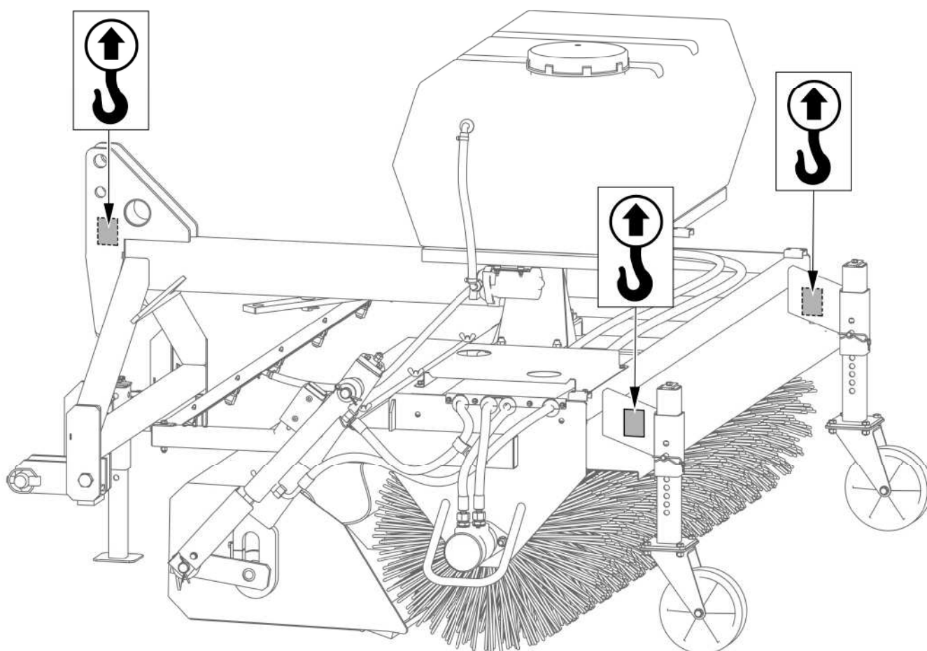
РИСУНОК 1.2 Транспортные захваты
