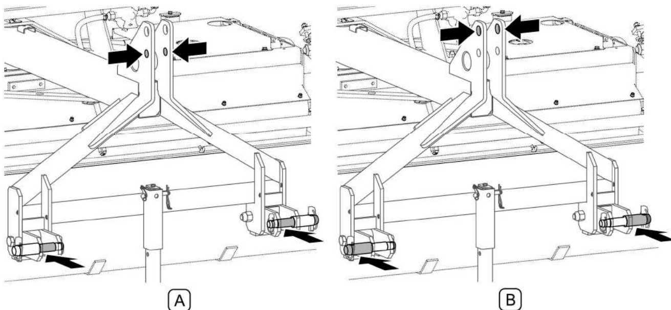
РИСУНОК 4.1 Категории трехточечной системы навески в соответствии с ISO 730- (А)- точки крепления кат. I ISO 730-1; (В)- точки крепления кат. II ISO 730-1;
