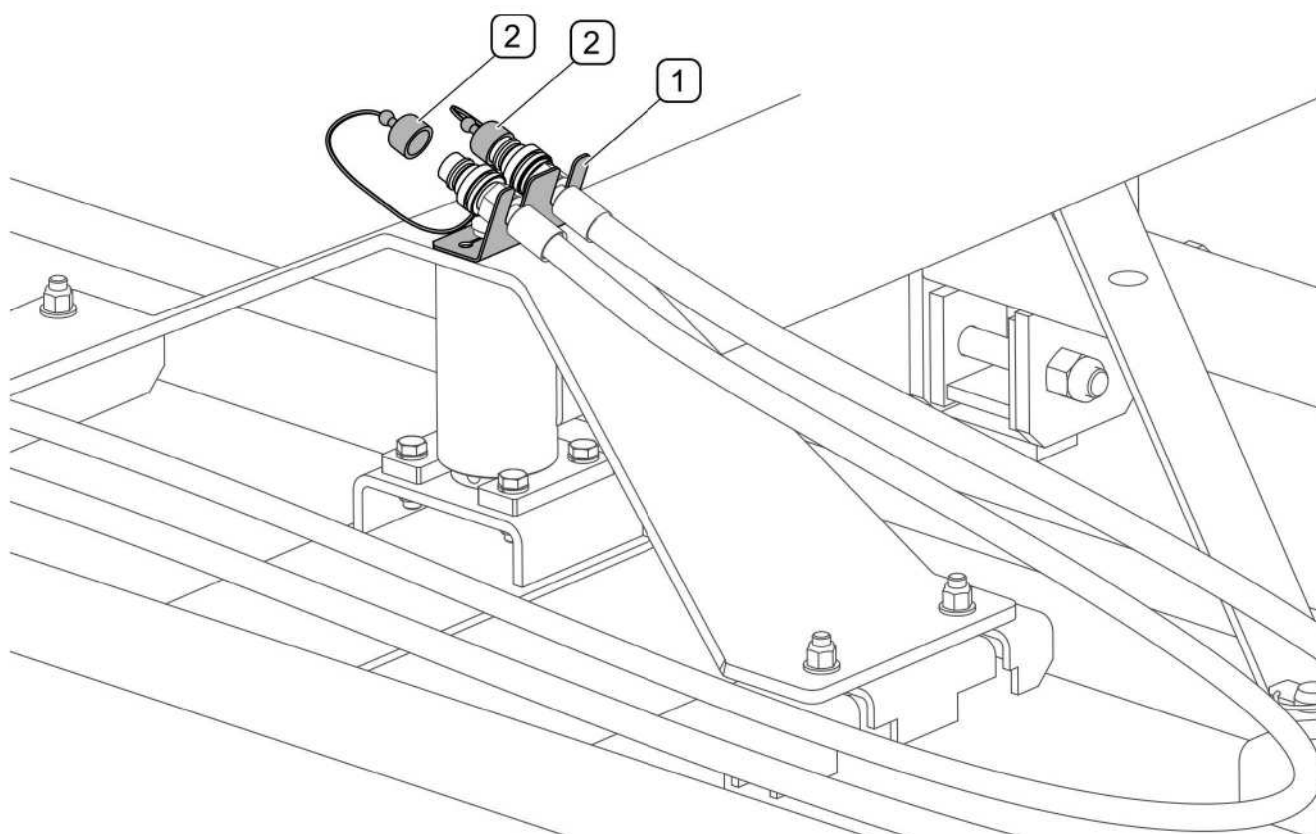
РИСУНОК 4.14 Предохранение штекеров после отсоединения от трактора
