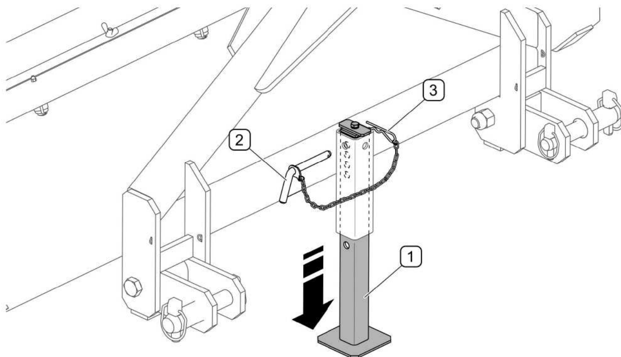
РИСУНОК 4.13 Стойночная опора
