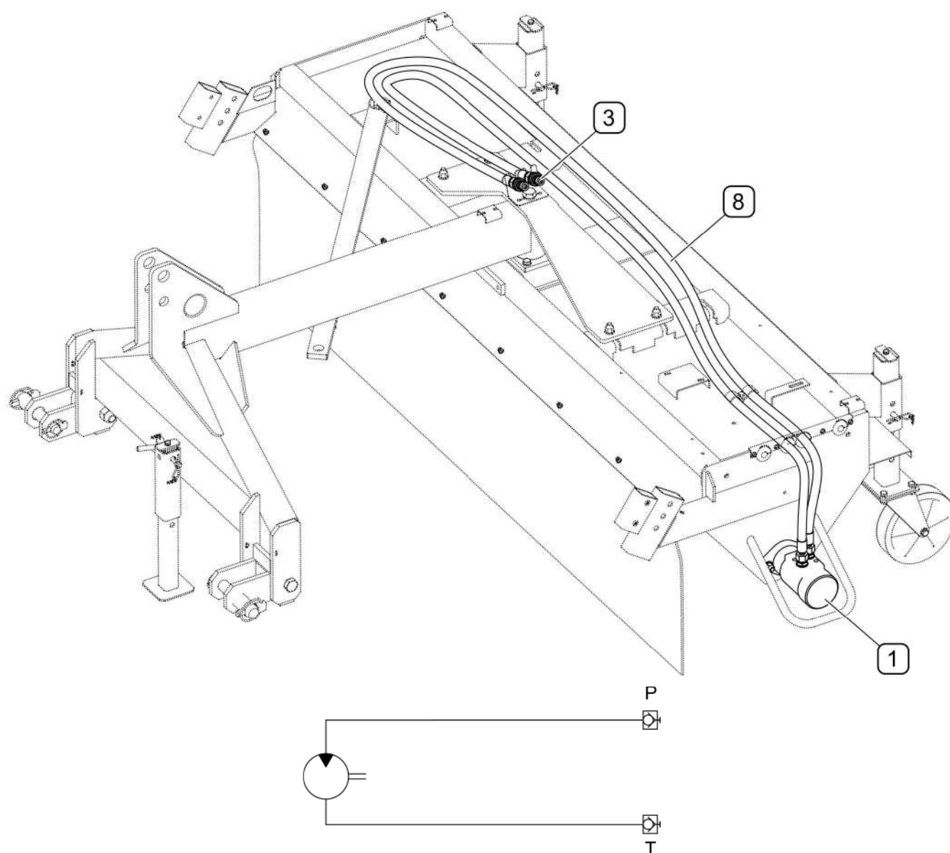
РИСУНОК 3.5 Устройство гидросистемы подметально-уборочной машины ZM- (1)- гидродвигатель привода подметающего валика; (3)- быстросъемные гидросоединения; (8)- гидропровода
