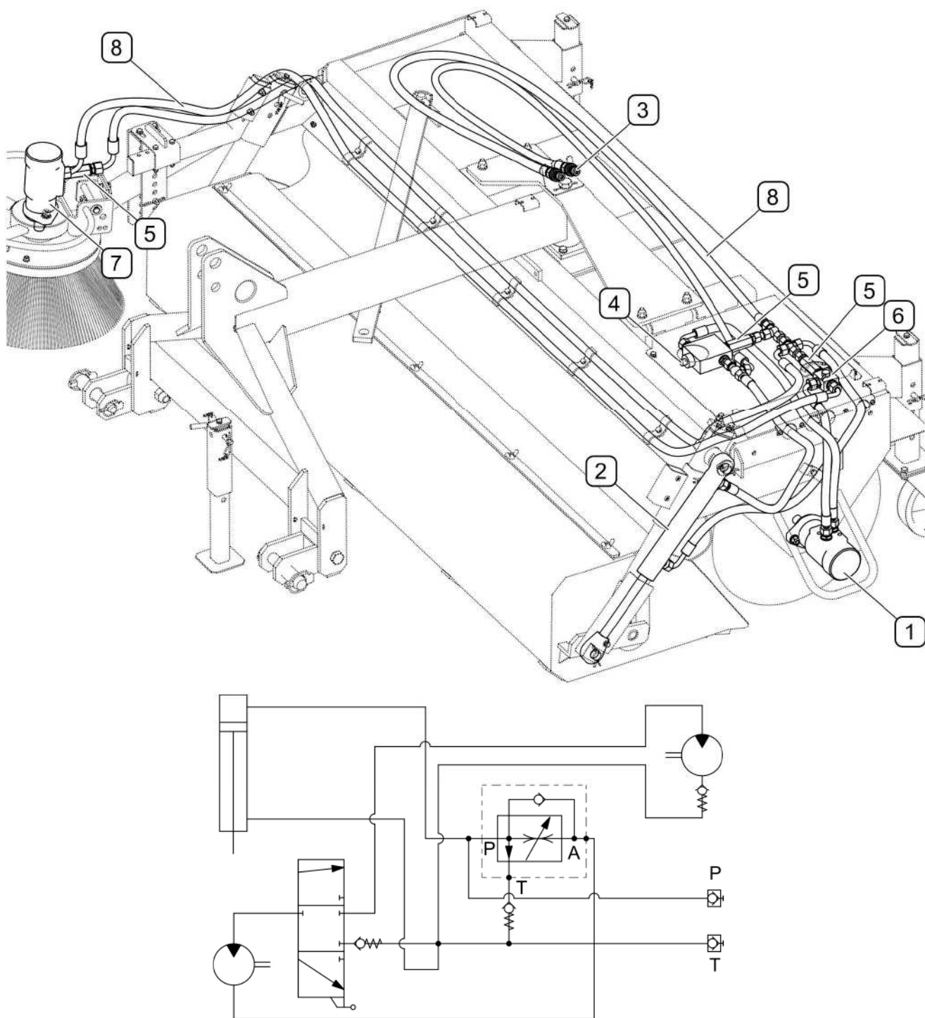
РИСУНОК 3.3 Устройство гидросистемы подметально-уборочных машин ZM-200- (1)- гидродвигатель привода подметающего валика; (2)- гидроцилиндр опорожнения
