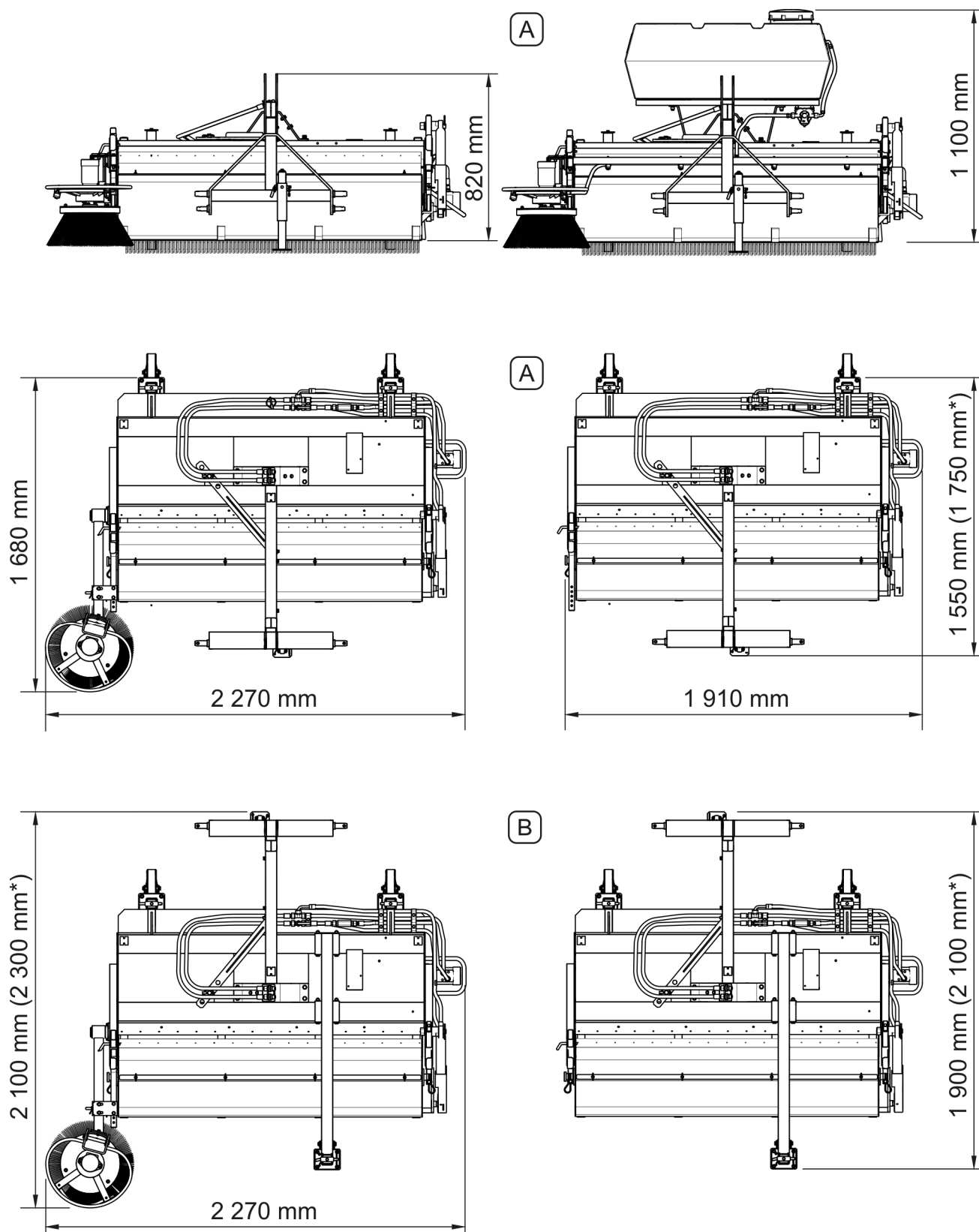
RYSUNEK 3.1 Wymiary zewnętrzne w zależności od wyposażenia
