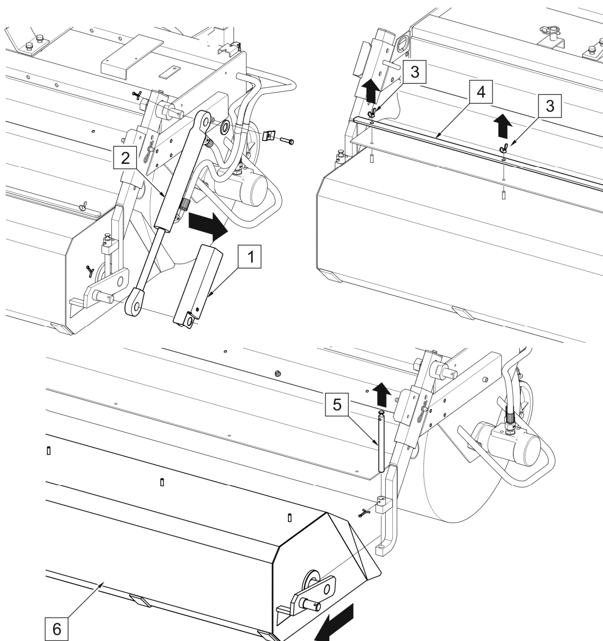
RYСУNEK 4.7 Demontaż cylindra hydraulicznego i listwy fartucha gumowego
