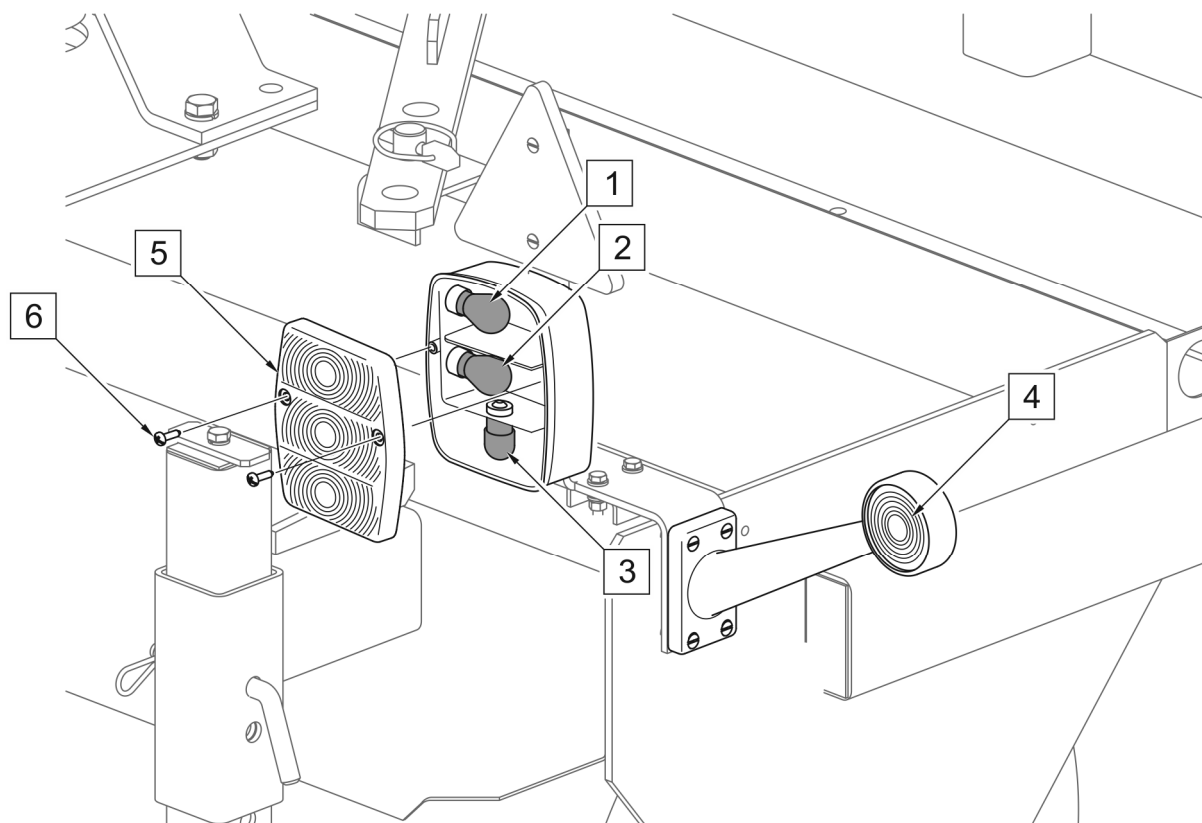
RYSUNEK 5.12 Wymiana żarówek
