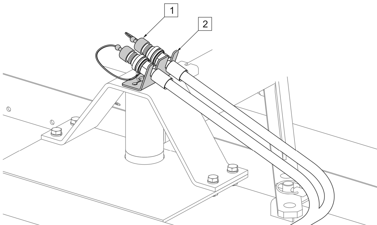
RYСУNEK 4.13 Zabezpieczenie wtyków po odłączeniu od nośnika
