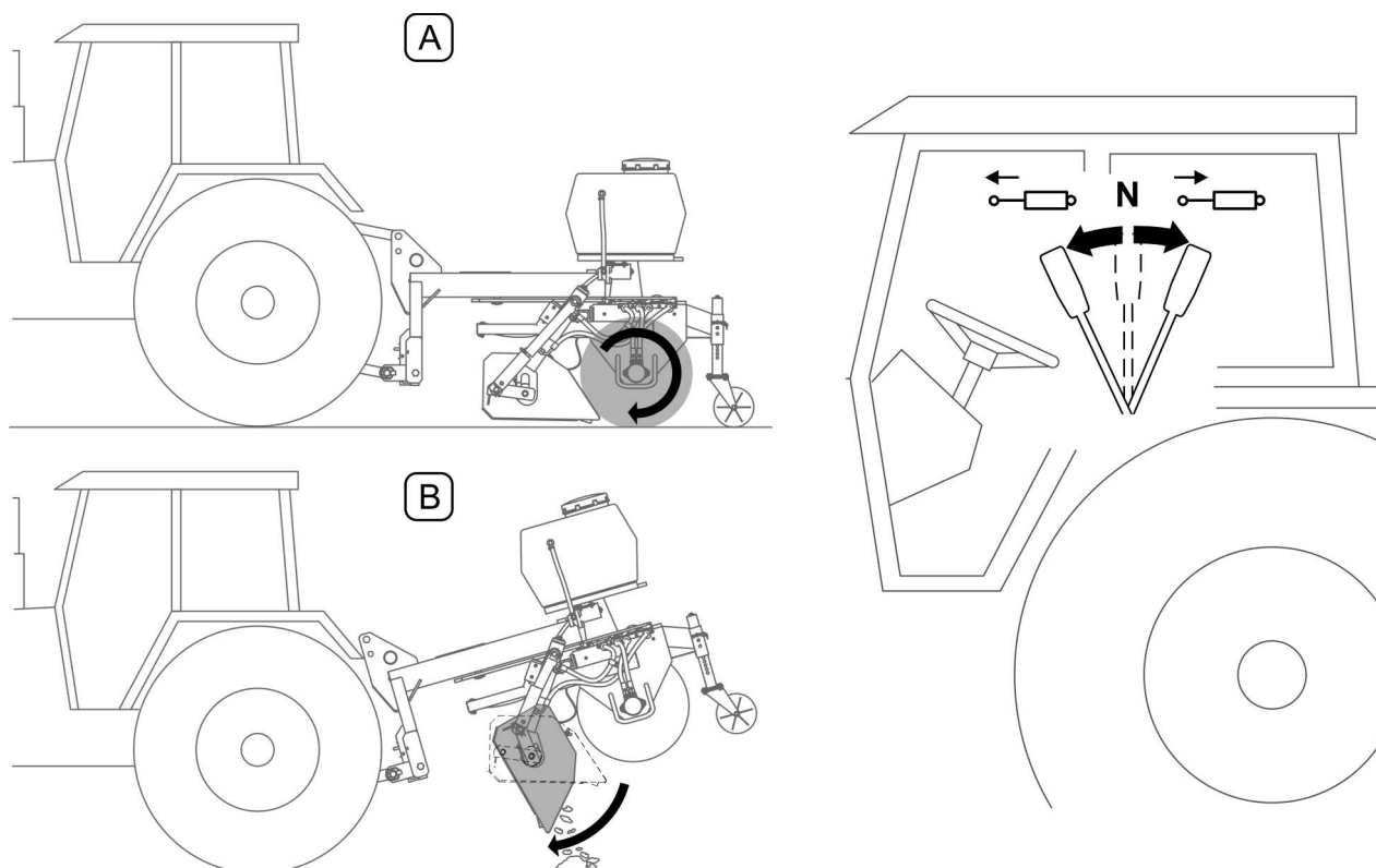
RYSUNEK 4.4 Opróżnianie zbiornika zanieczyszczeń
