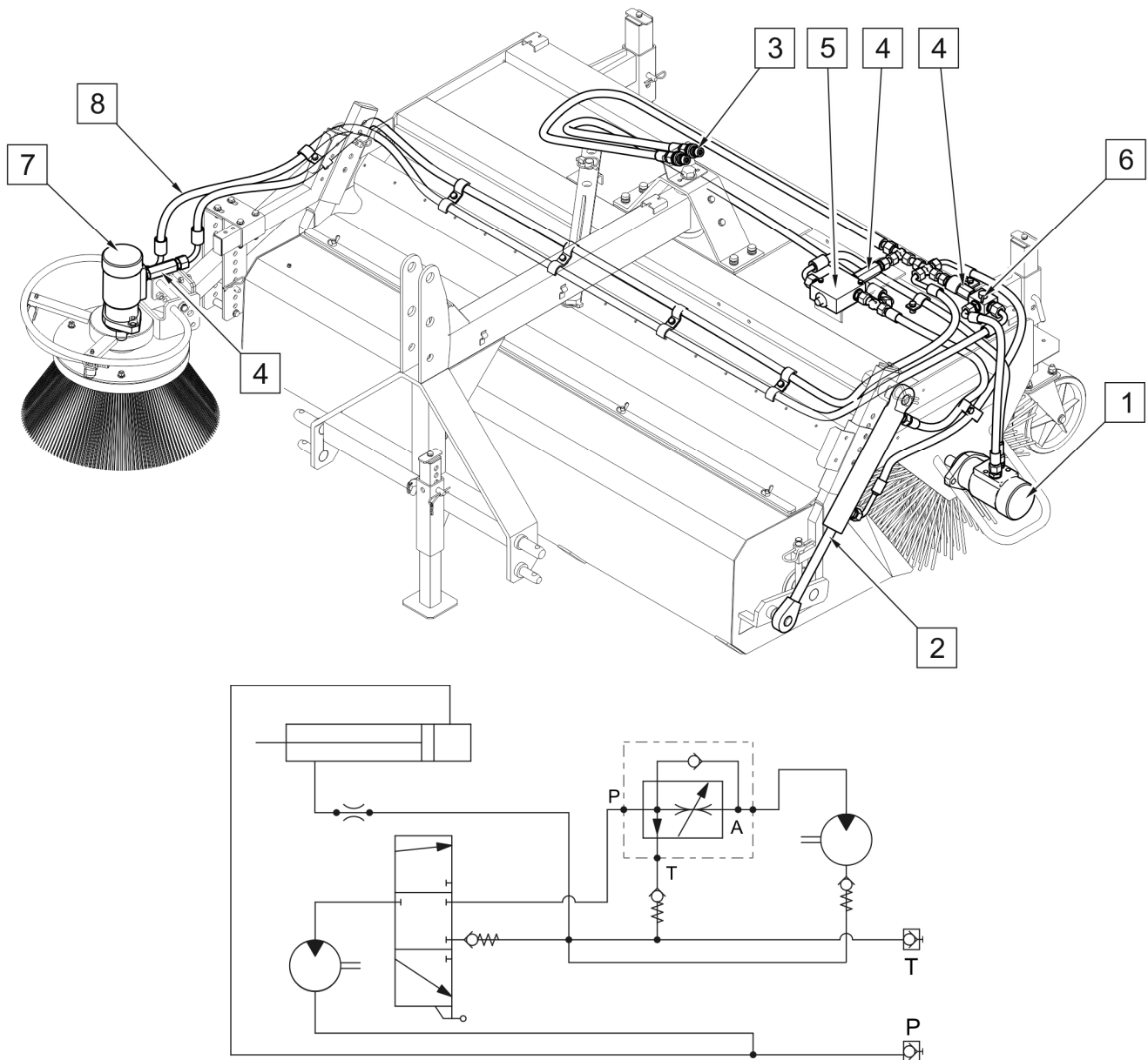
RYСУNEK 3.3 Budowa instalacji hydraulicznej zamiatarek ZM-1600-01; ZM-1600-03
