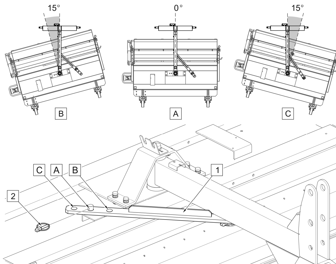
RYSUNEK 4.8 Zmiana kąta pracy zmiatarki
