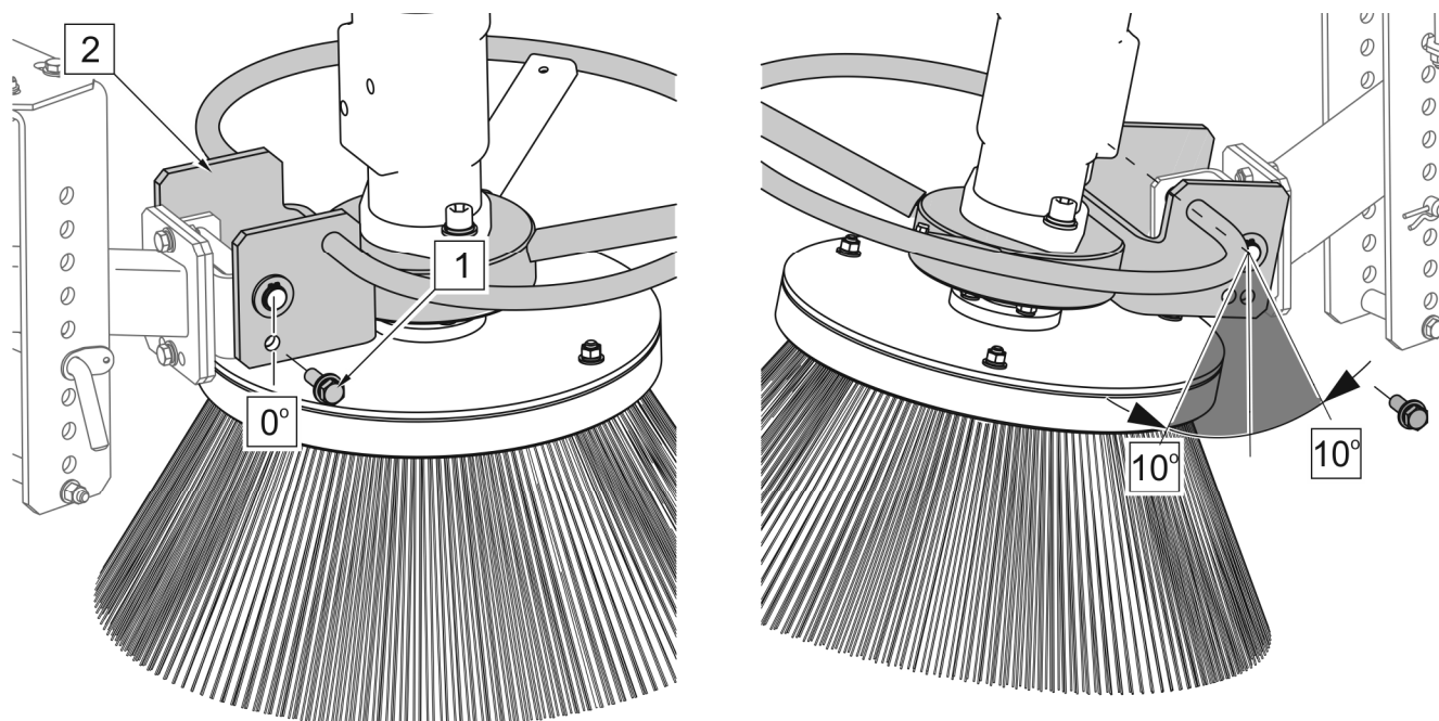
RYСУNEK 5.5 Regulacja pochylenia wzdłużnego
