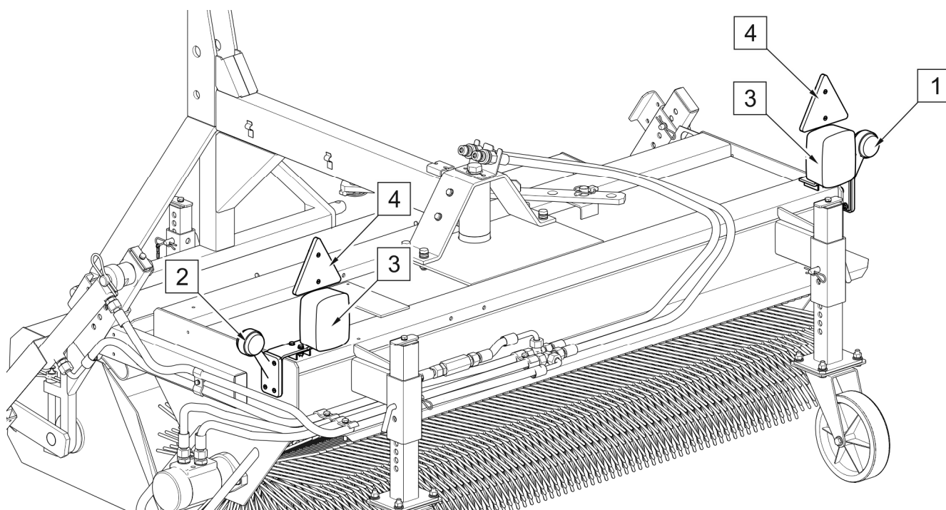
RYSUNEK 4.10 Dodatkowe oświetlenie zmiatarki pracującej za nośnikiem (opcja)
