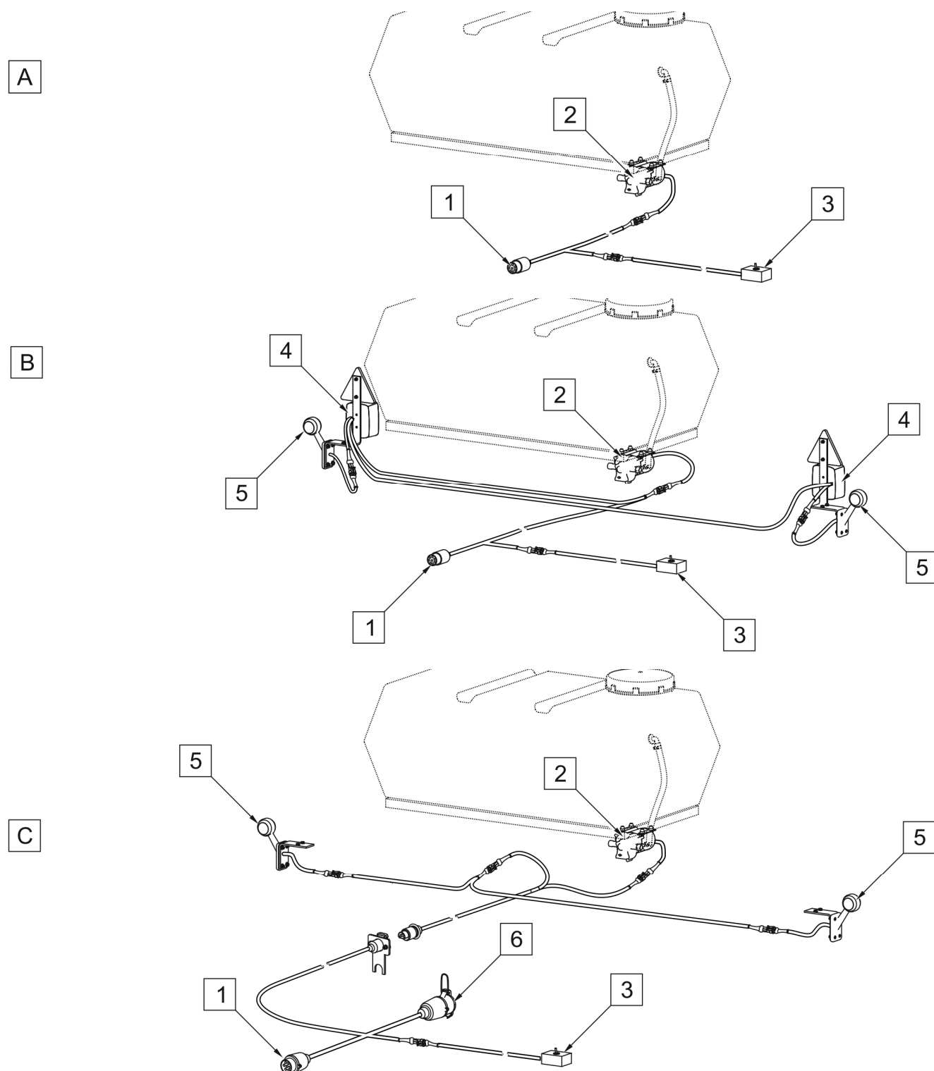
RYСУNEK 3.8 Budowa układu instalacji elektrycznej
