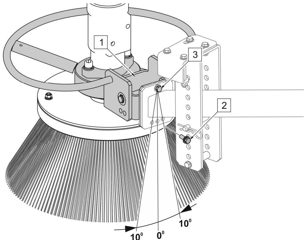
RYSUNEK 5.6 Regulacja pochylenia poprzecznego
