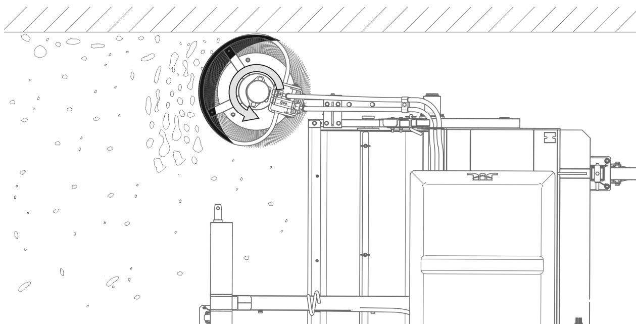
RYSUNEK 5.3 Schemat prawidłowego ustawienia szczotki bocznej
