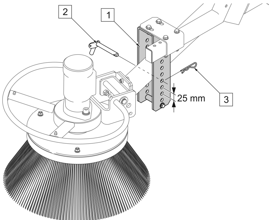
RYСУNEK 5.4 Ustawienie docisku szczotki bocznej
