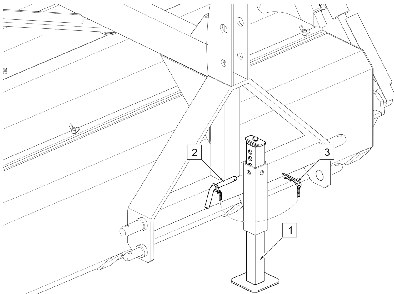
RYSUNEK 4.12 Podpórka postojowa
