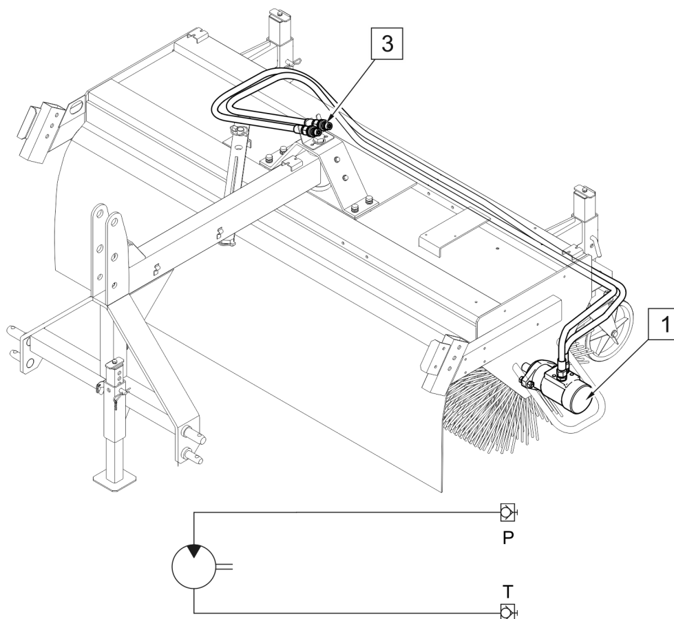
RYSUNEK 3.6 Budowa instalacji hydraulicznej zmiatarki ZM-1600-04
