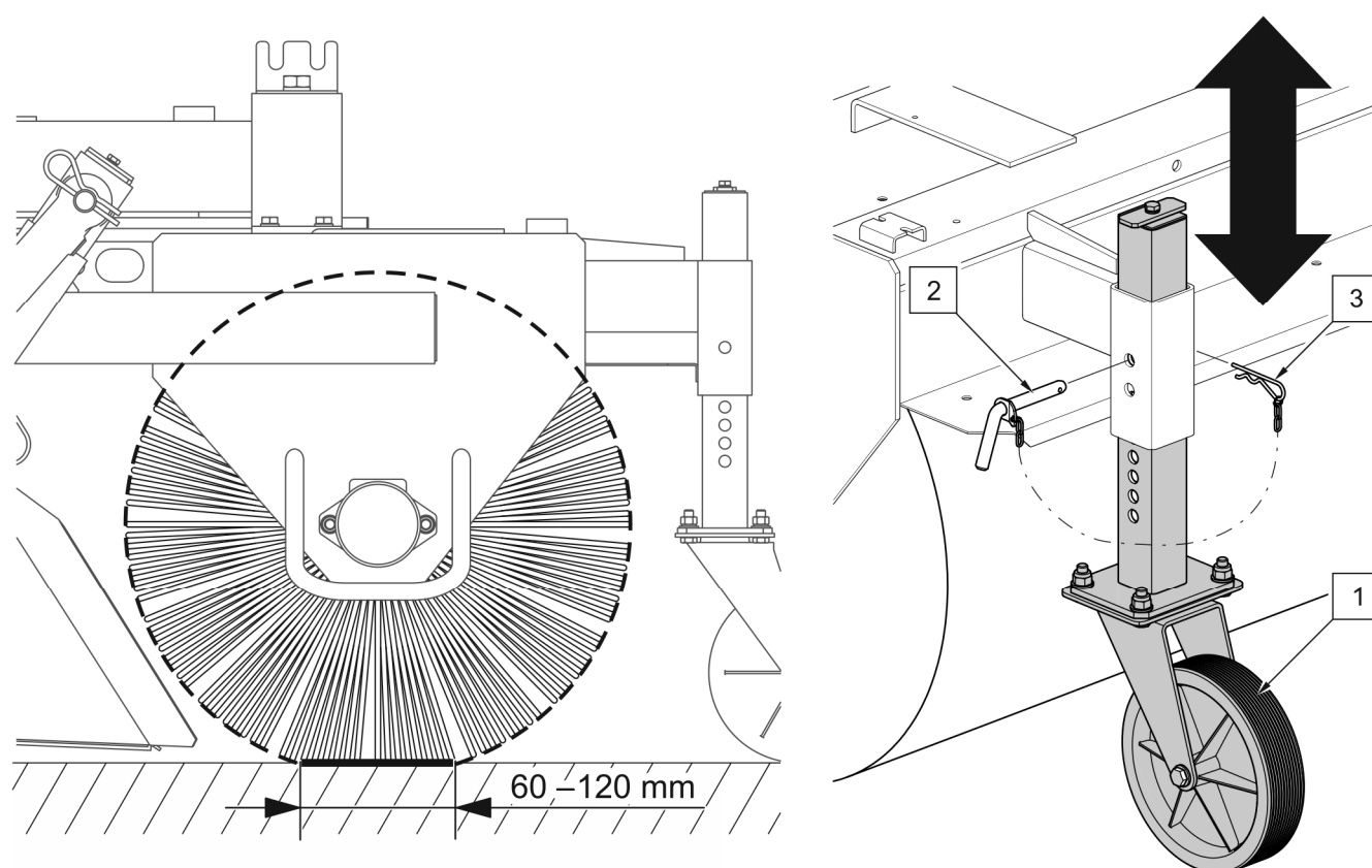
RYSUNEK 5.1 Regulacja docisku szczotki walcowej
