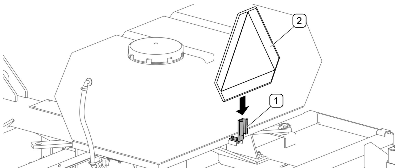
RYSUNEK 4.9 Dodatkowy spornik tablicy wyróżniającej (opcja)
