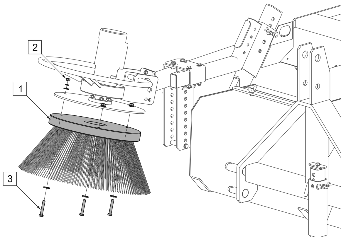
RYСУNEK 5.9 Wymiana szczotki bocznej
