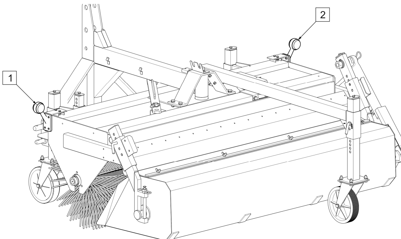
RYСУNEK 4.11 Dodatkowe oświetlenie zmiatarki pracującej przed nośnikiem (opcja)
