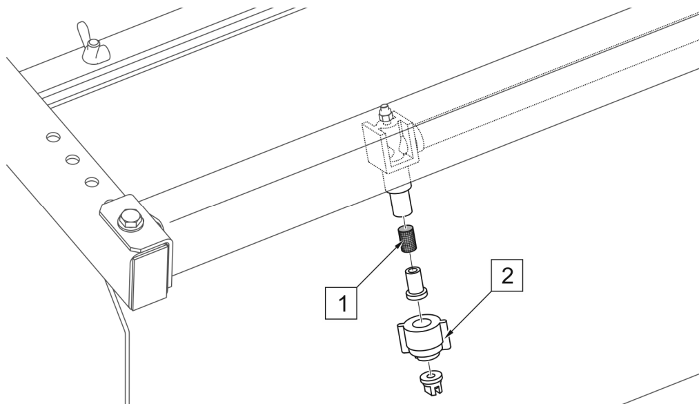
RYSUNEK 5.11 Filtry zraszaczy
