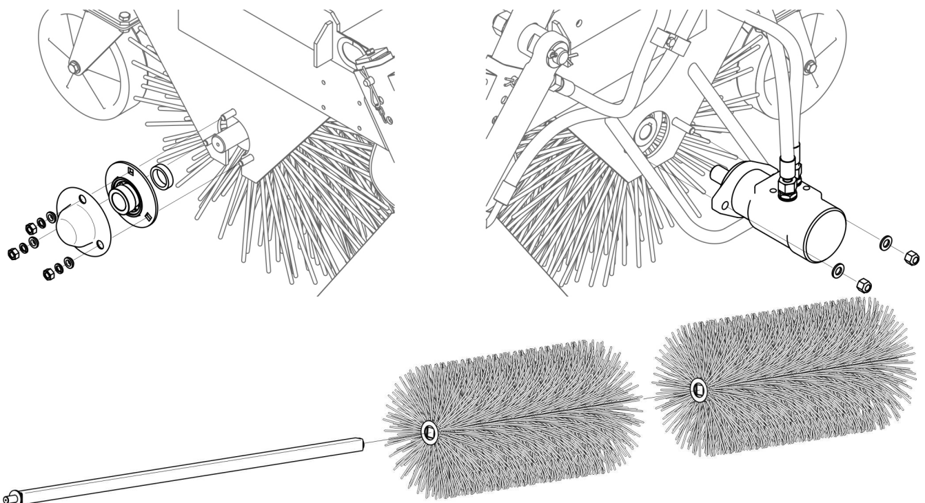
RYSUNEK 5.8 Wymiana szczotki walcowej
