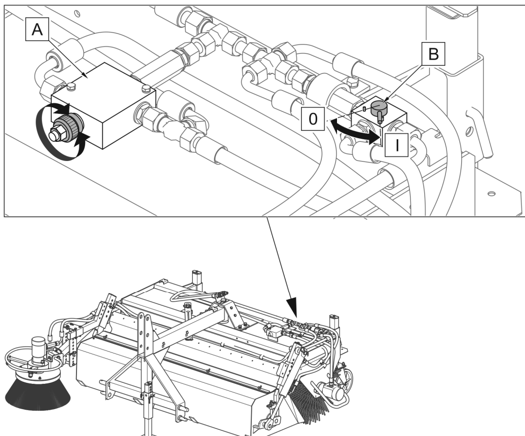
RYSUNEK 5.7 Regulator przepływu i rozdzielacz napędu szczotki
