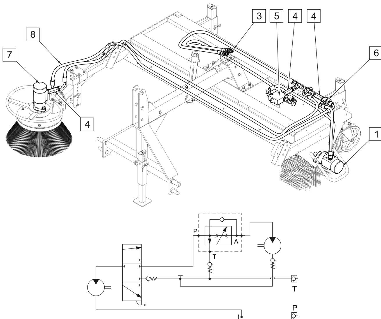
RYСУNEK 3.5 Budowa instalacji hydraulicznej zmiatarki ZM-1600-05
