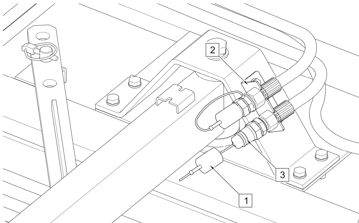
RYСУNEK 4.13 Zabezpieczenie wtyków po odłączeniu od nośnika
