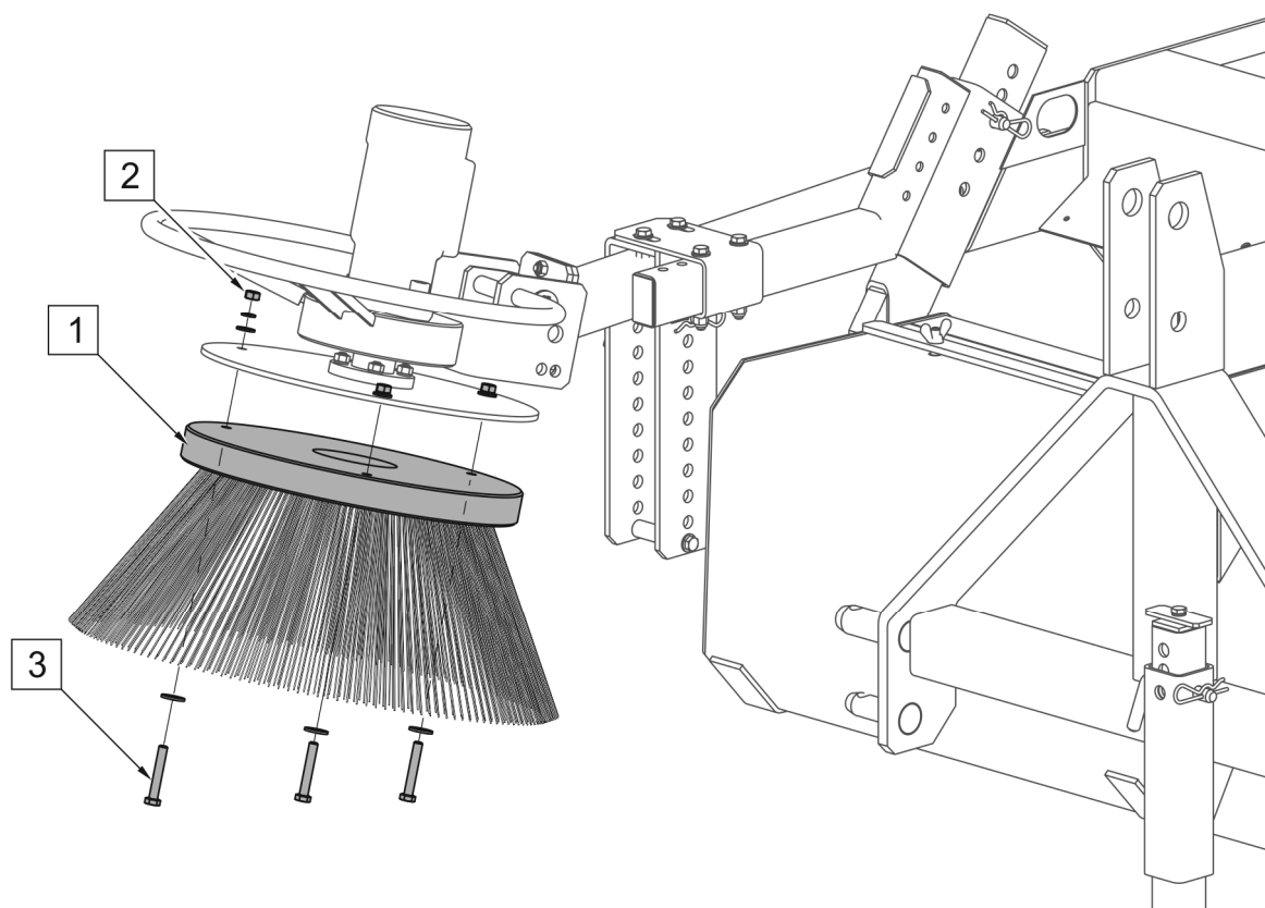
RYСУNEK 5.9 Wymiana szczotki bocznej
