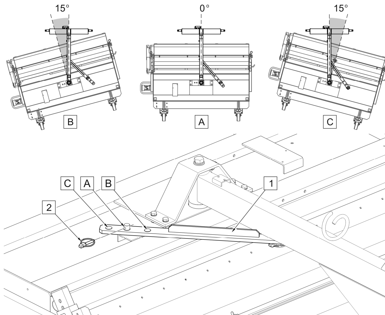
RYSUNEK 4.8 Zmiana kąta pracy zmiatarki
