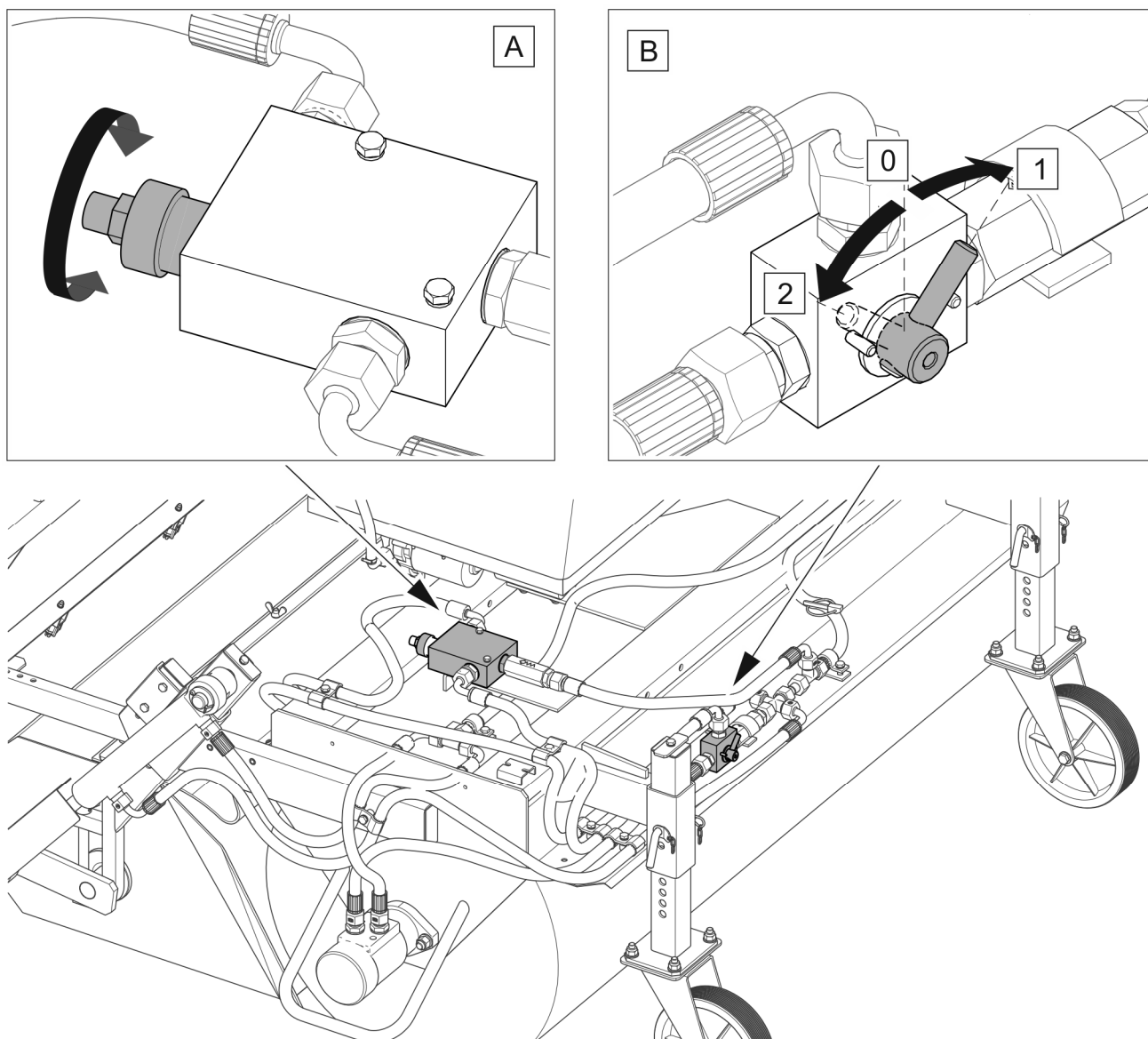
RYSUNEK 5.7 Regulator przepływu i rozdzielacz napędu szczotki
