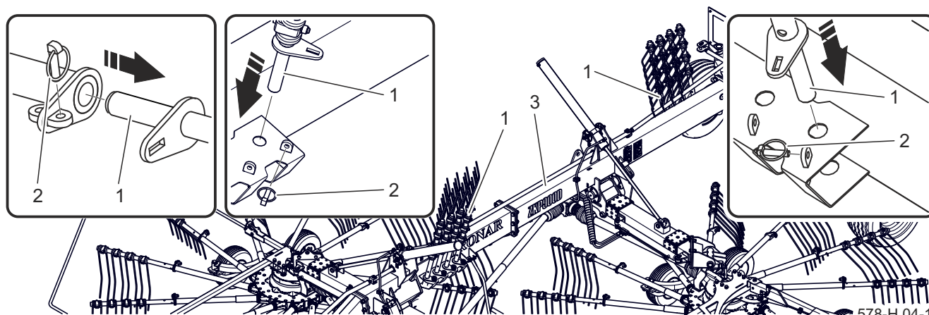
Rysunek 4.4 Montaż ramion grabiących
