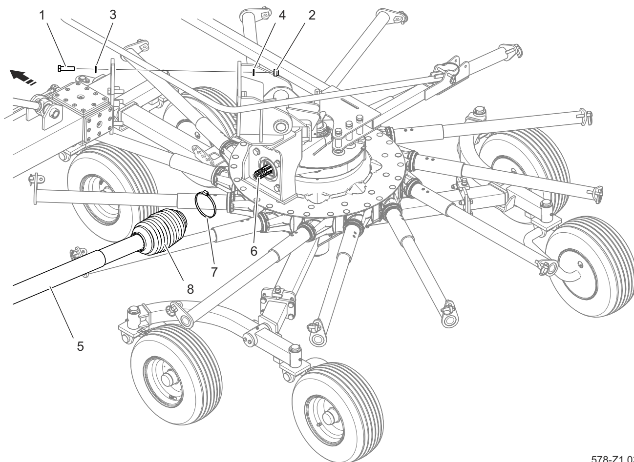
Rysunek A.3 Montaż zespołu grabiącego
