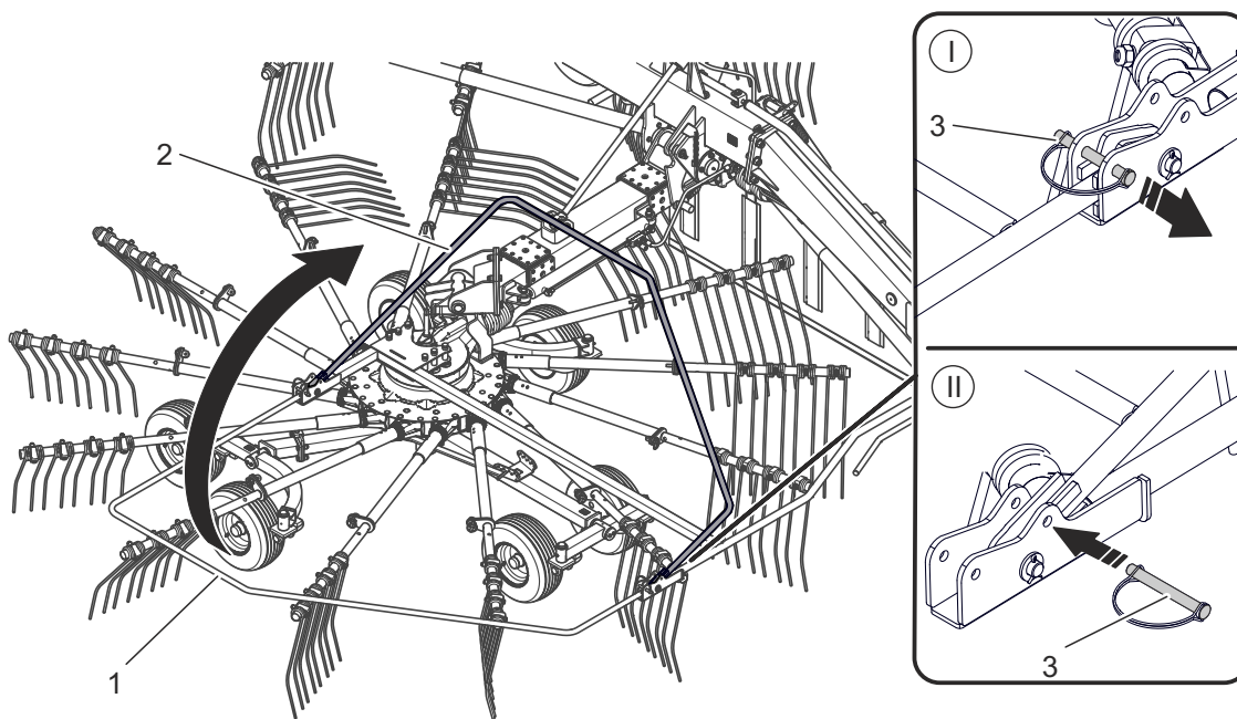
Rysunek 4.3 Obsługa osłon ochronnych
