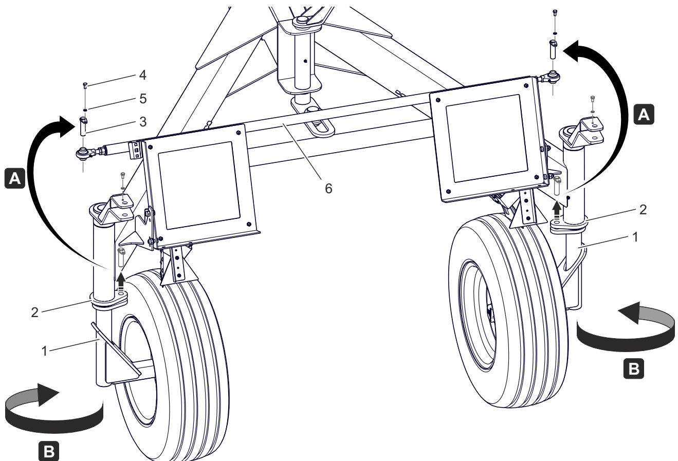
Rysunek A.1 Obrót kół
