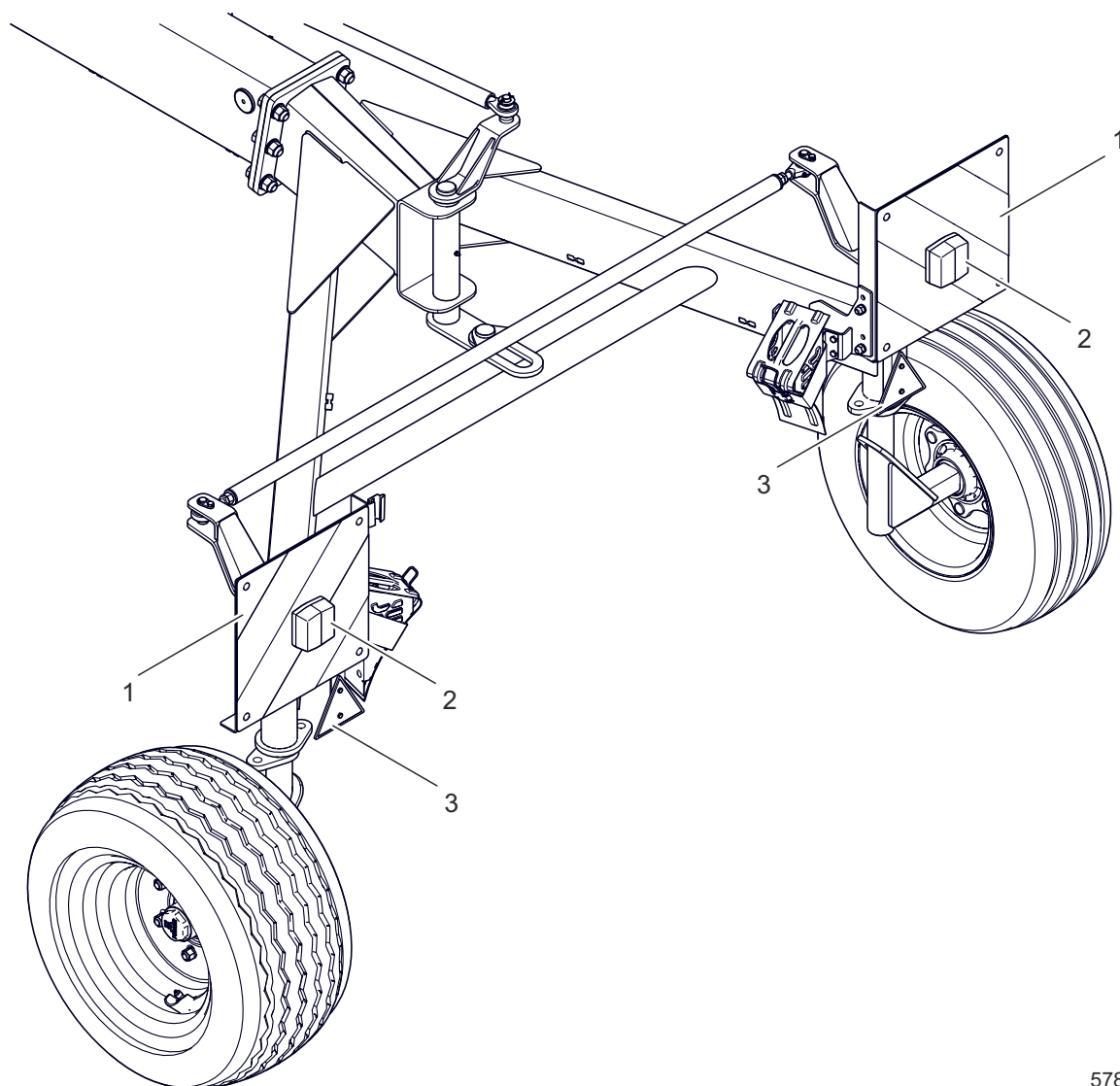
Rysunek 3.6 Rozmieszczenie elementów instalacji elektrycznej oraz elementów odblaskowych
