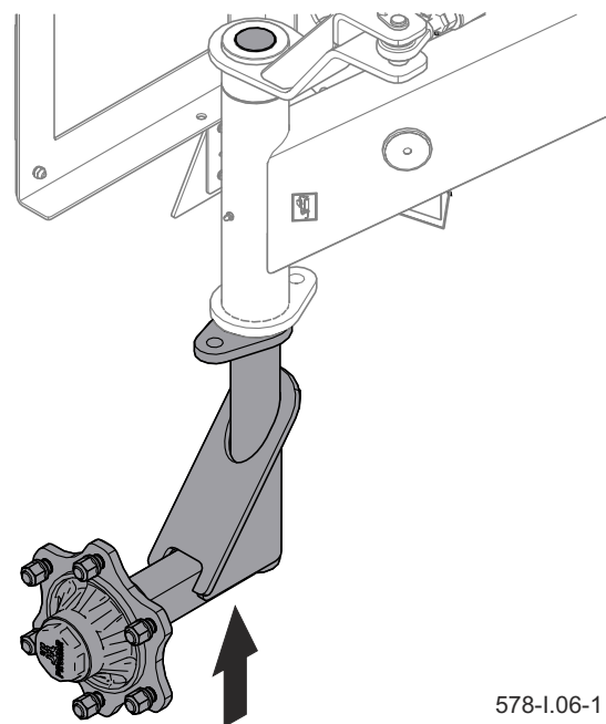
Rysunek 5.1 Punkt podparcia podnośnika
