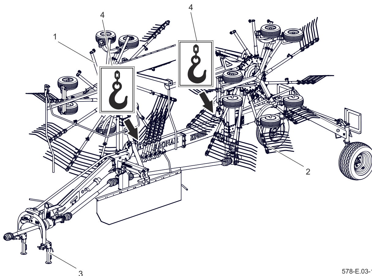
Rysunek 1.3 Lokalizacja uchwytów transportowych
