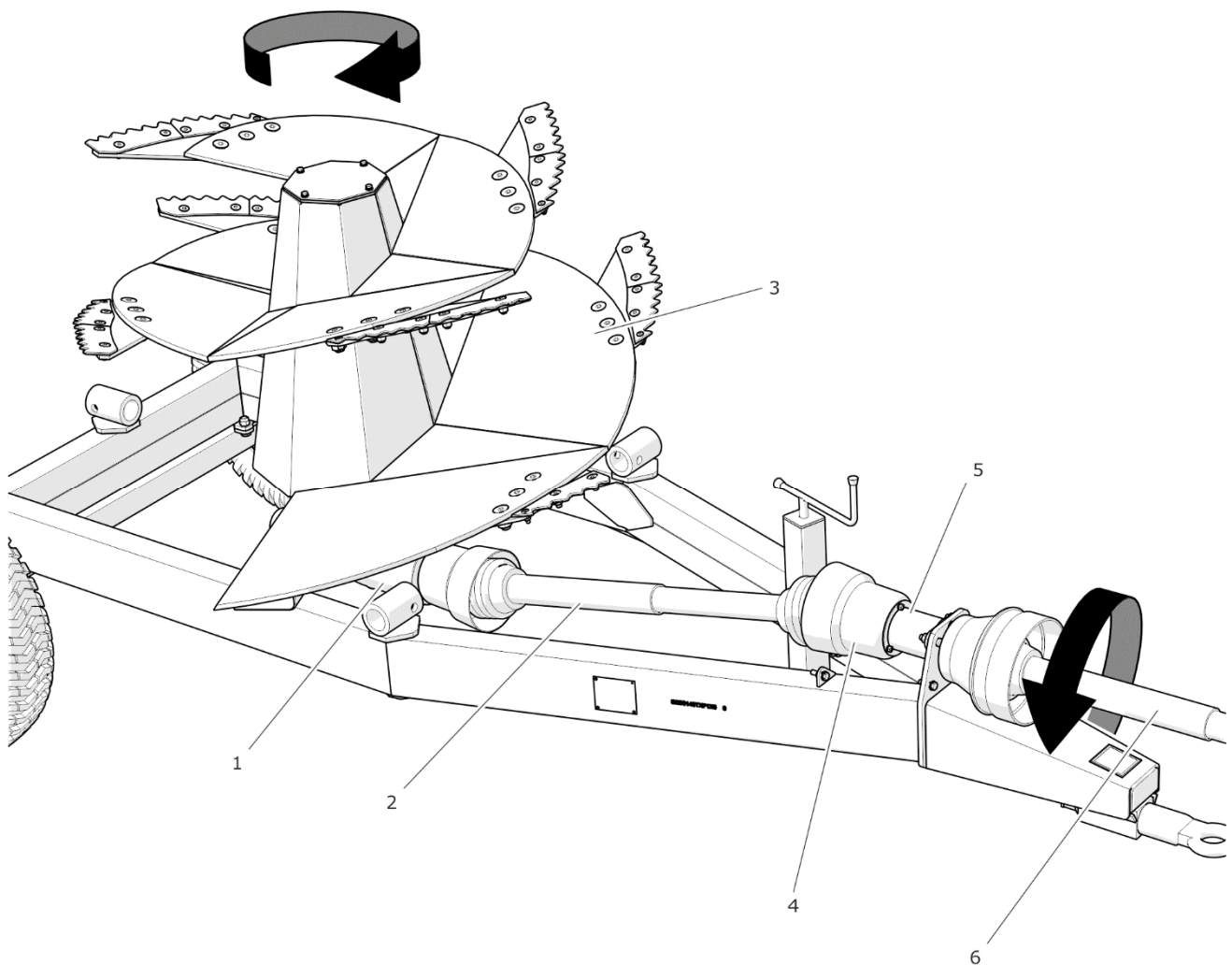
РИСУНОК 3.5 Система передачи привода
