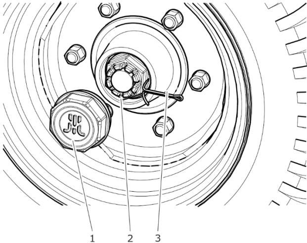
РИСУНОК 5.3 Регулировка подшипников в ходовой полуоси
