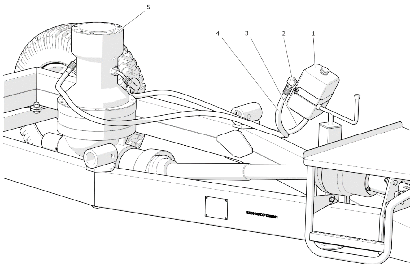
РИСУНОК 3.7 Система смазки передачи
