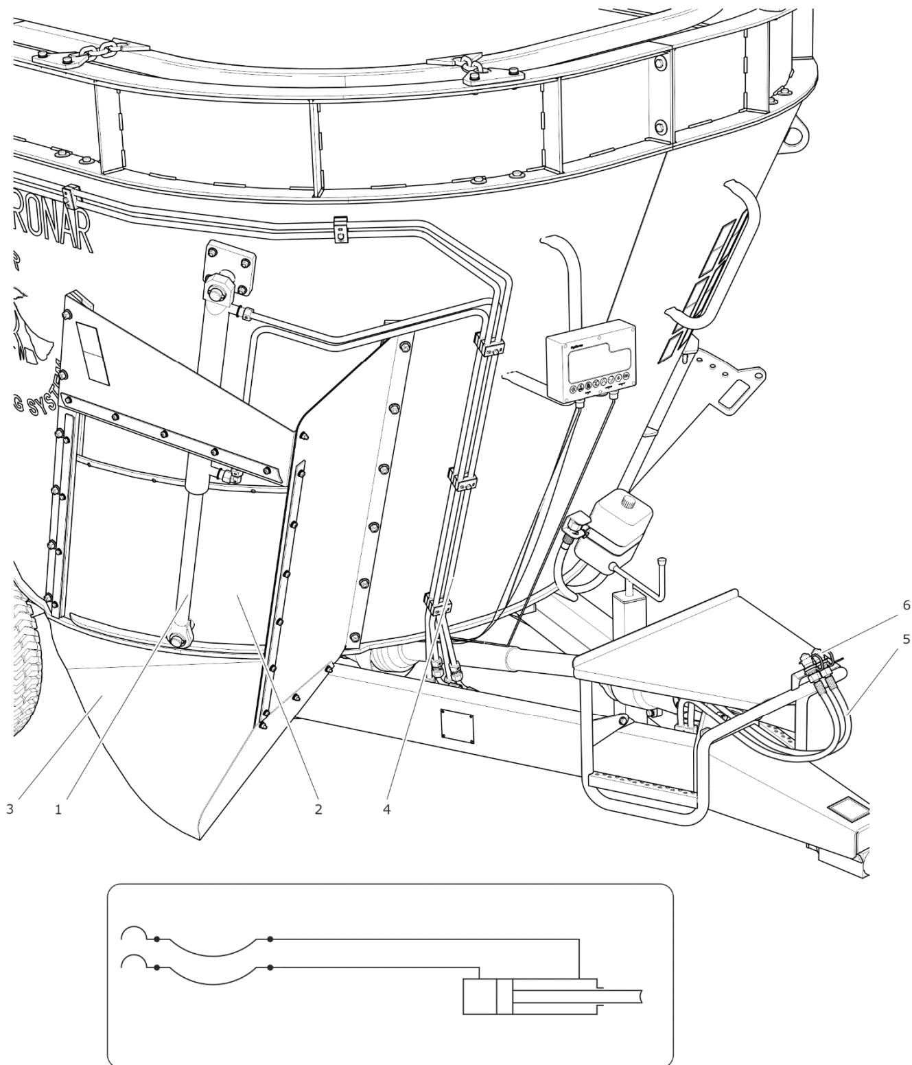
РИСУНОК 3.6 Схема и устройство гидравлической системы заслонки
