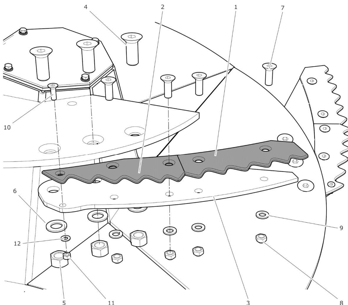
РИСУНОК 5.7 Демонтаж режущих ножей
