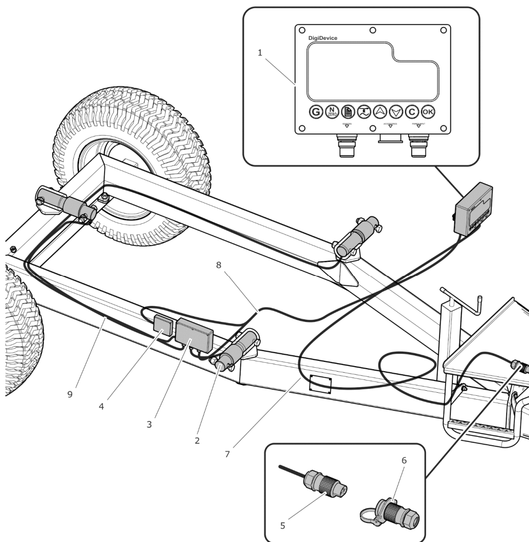
РИСУНОК 3.8 Размещение элементов световой сигнализации
