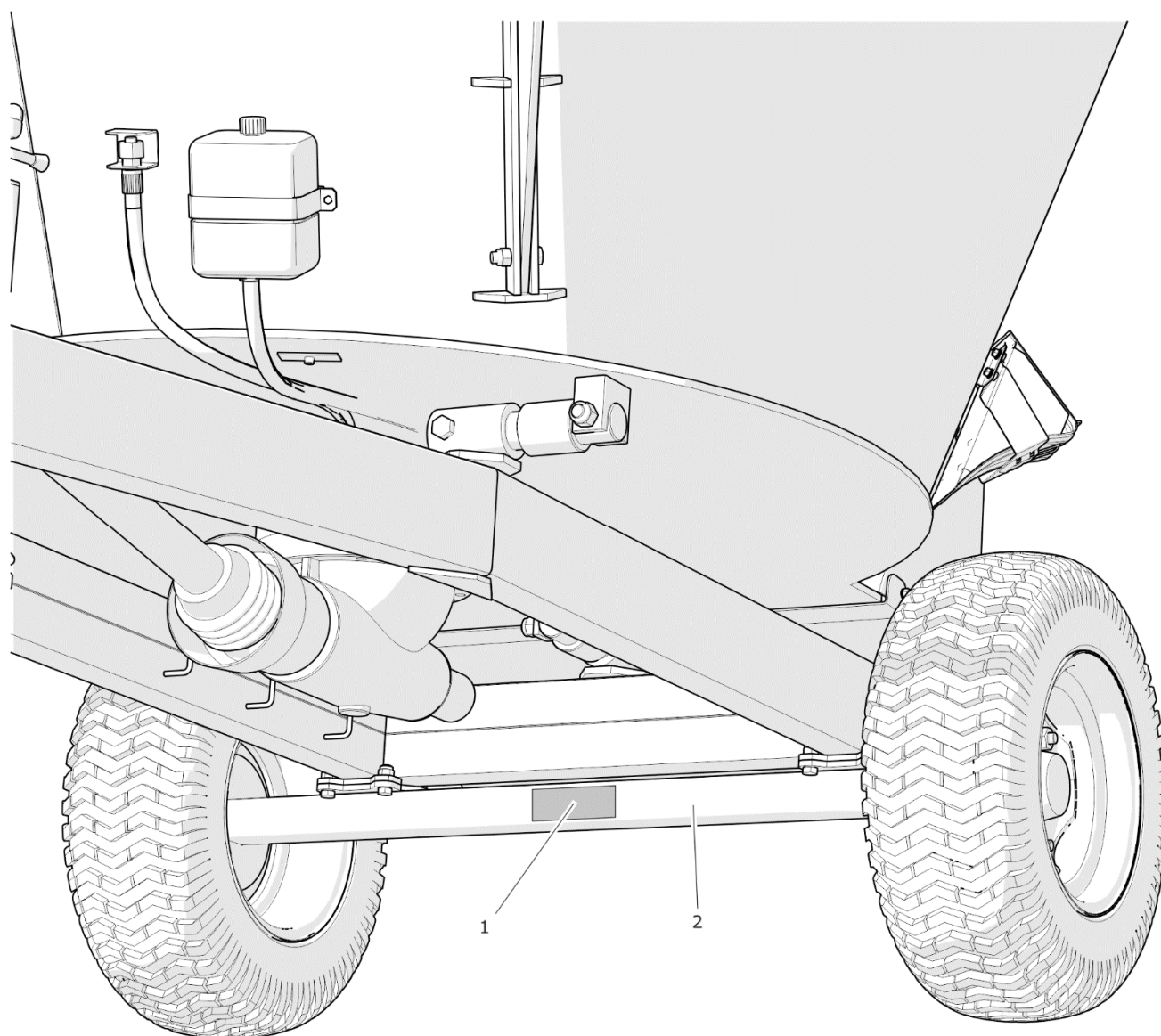
РИСУНОК 1.2 Размещение заводского щитка ходовой оси
