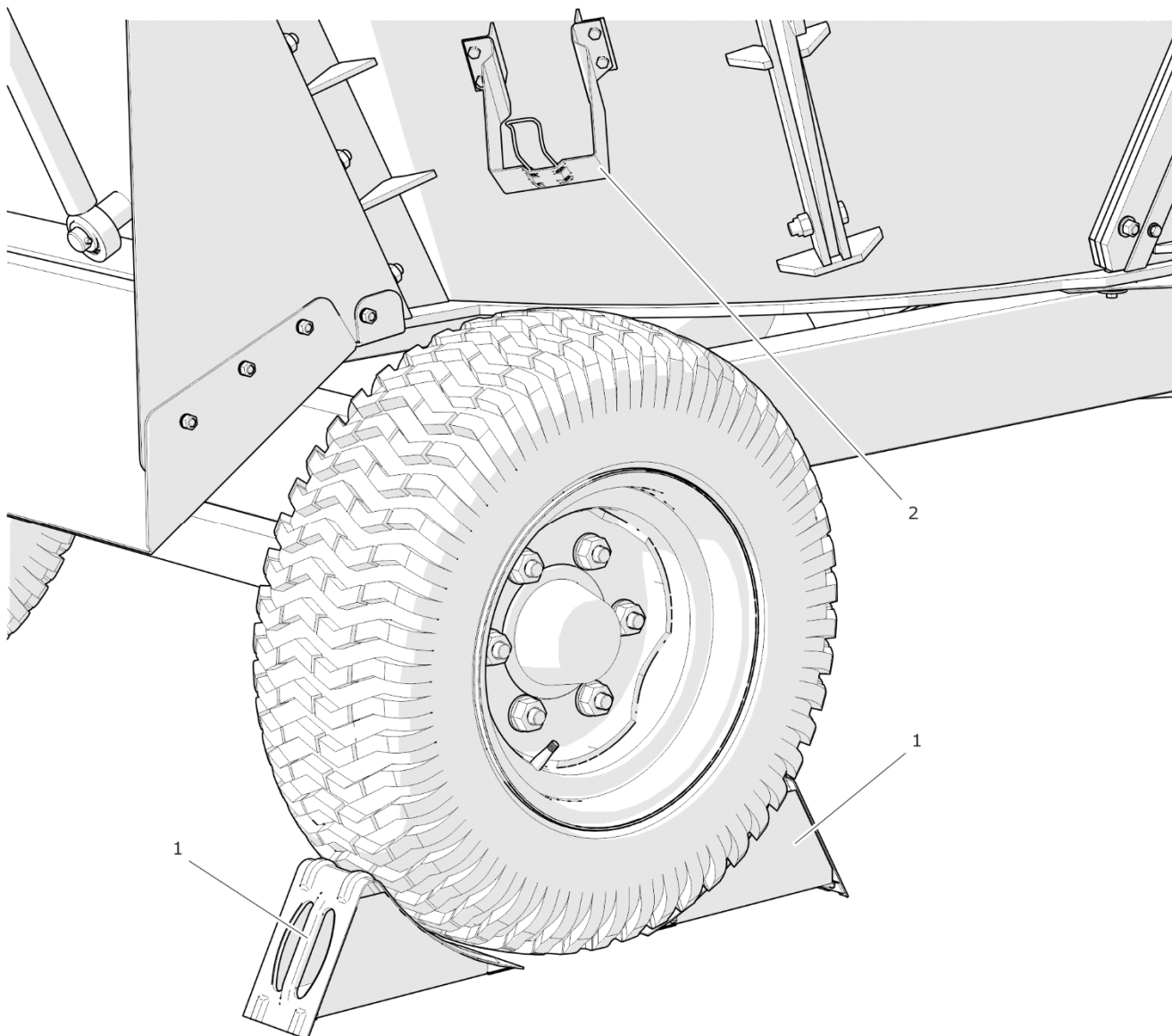
РИСУНОК 2.1 Способ установки клиньев
