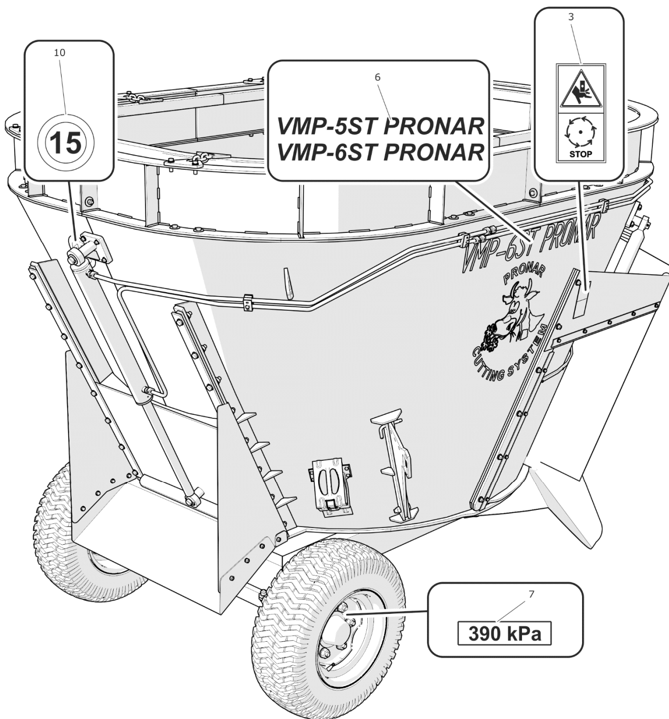
РИСУНОК 2.3 Размещение информационных и предупреждающих наклеек
