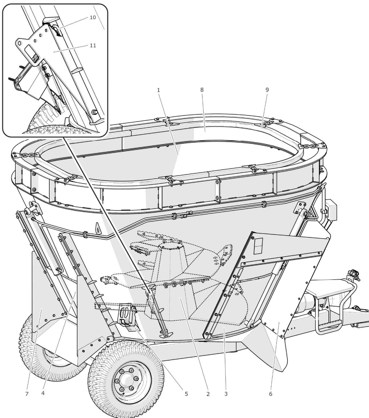
РИСУНОК 3.2 Бункер кормораздатчика
