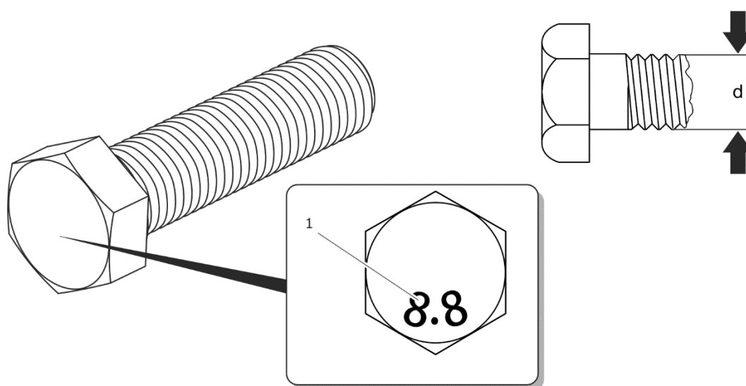
РИСУНОК 5.9 Болт с метрической резьбой
