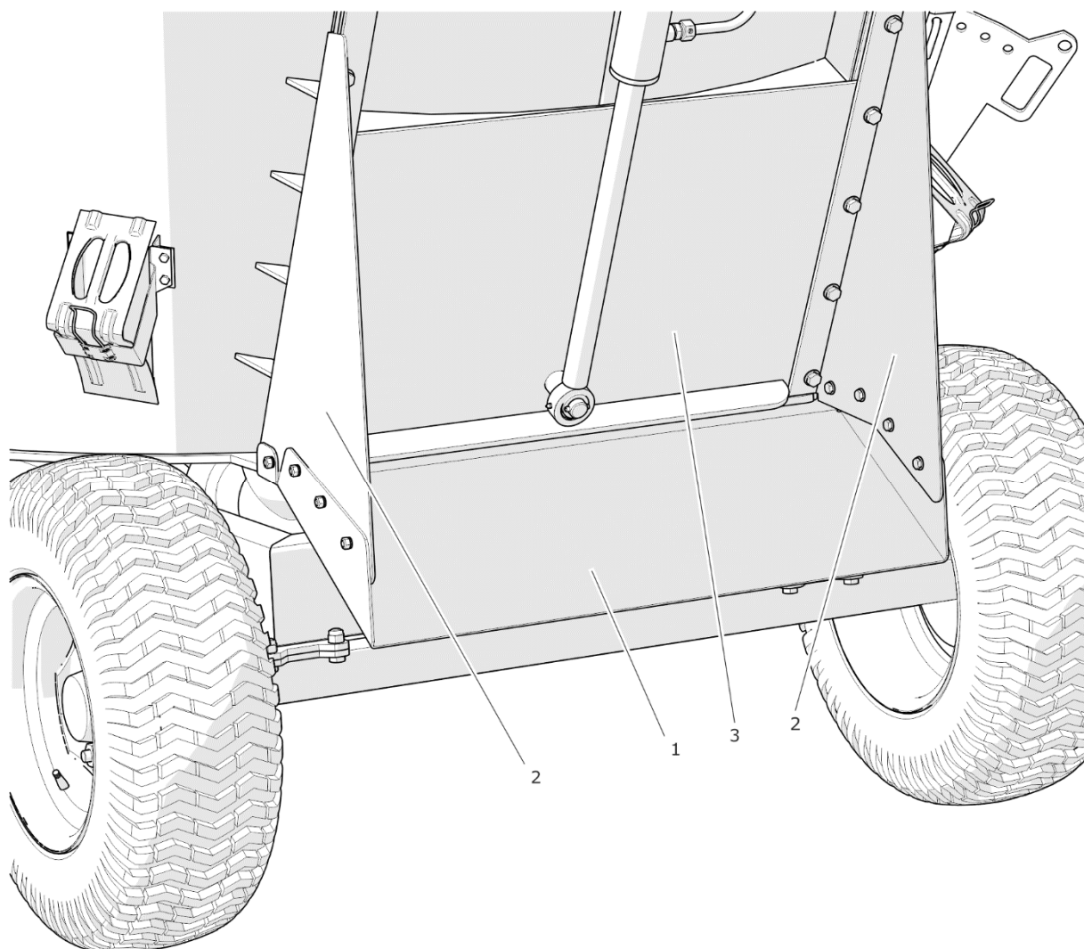
РИСУНОК 3.4 Дозирующее окно бункера - заднее
