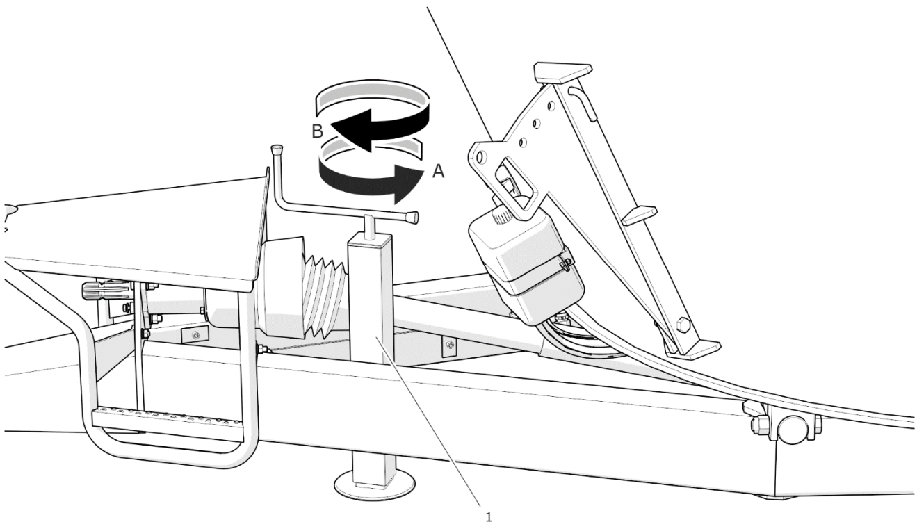
РИСУНОК 4.1 Обслуживание опоры
