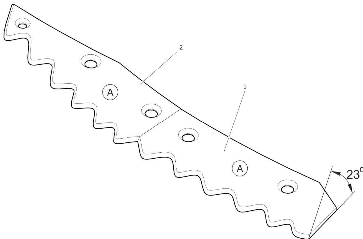
РИСУНОК 5.8 Правило заточки ножей
