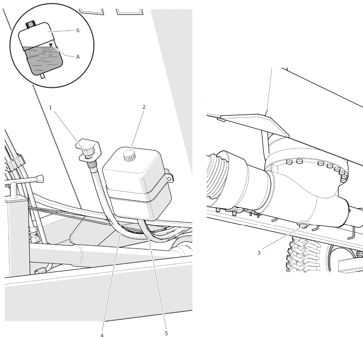
РИСУНОК 5.6 Замена масла
