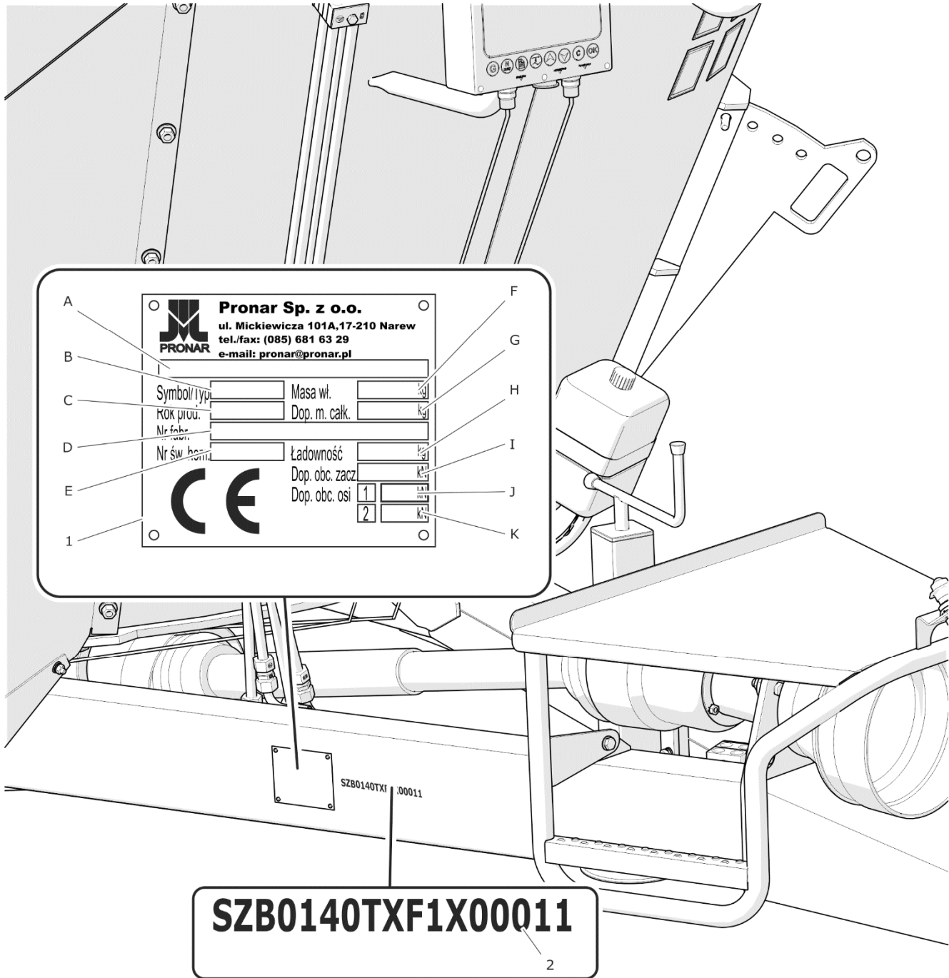
РИСУНОК 1.1 Размещение заводского щитка и серийного номера
