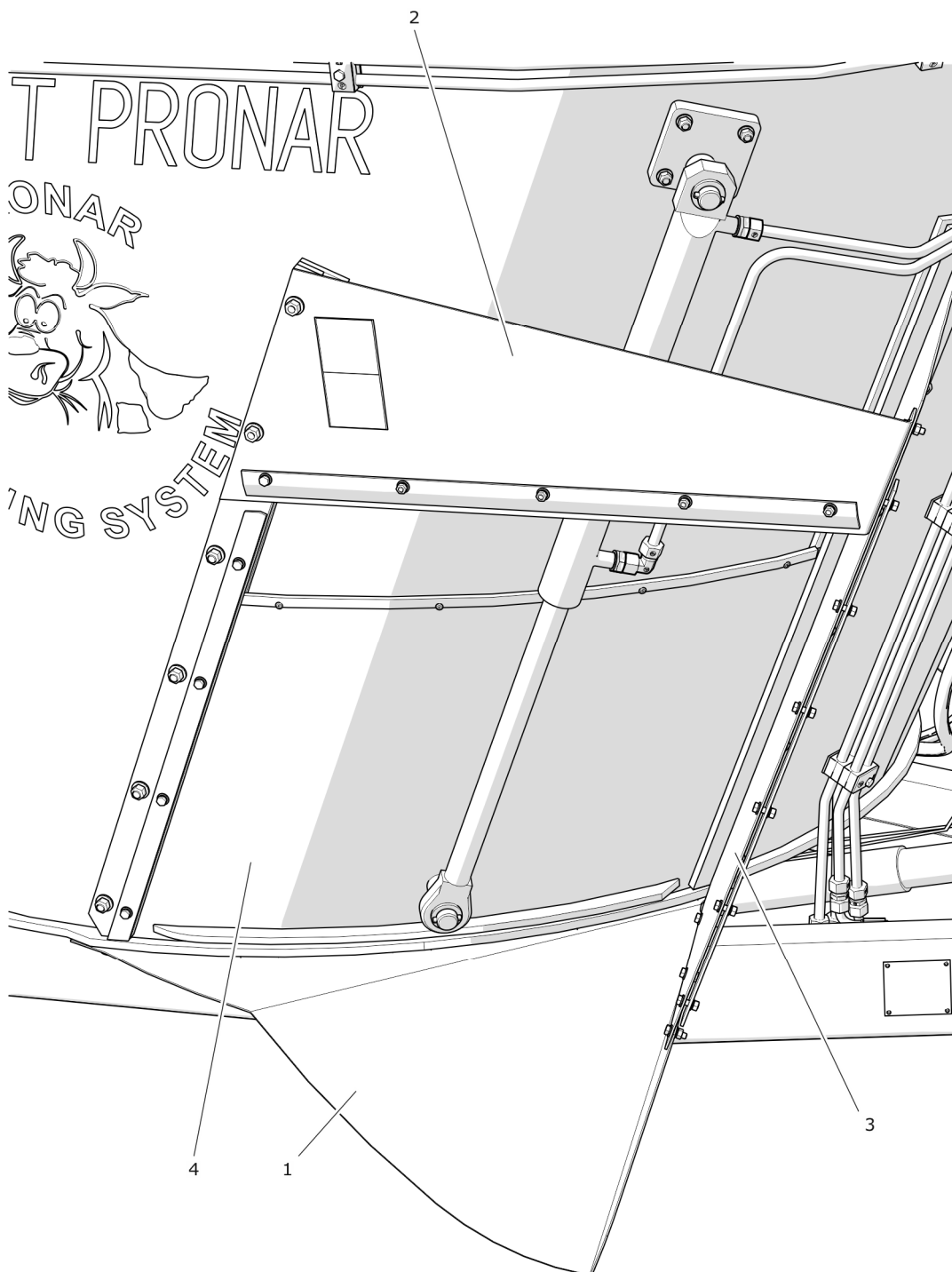
РИСУНОК 3.3 Окно для дозированной раздачи корма - переднее правое
