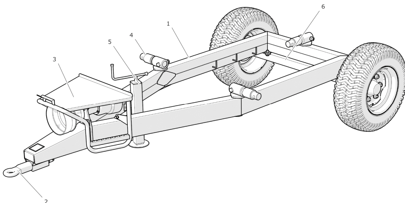
РИСУНОК 3.1 Шасси
