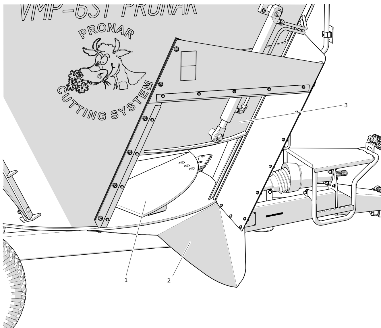
РИСУНОК 4.2 Окно для дозированной раздачи корма
