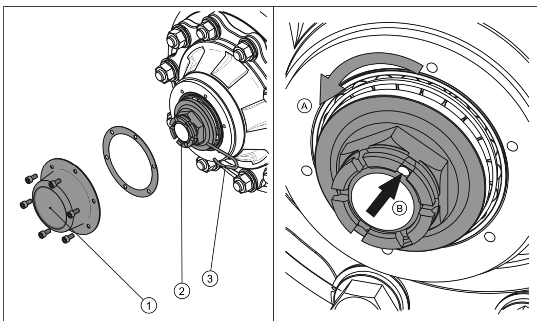
RYСУNEK 5.1A REGULACJA LUZU ŁOŻYSK OSI JEZDNEJ
