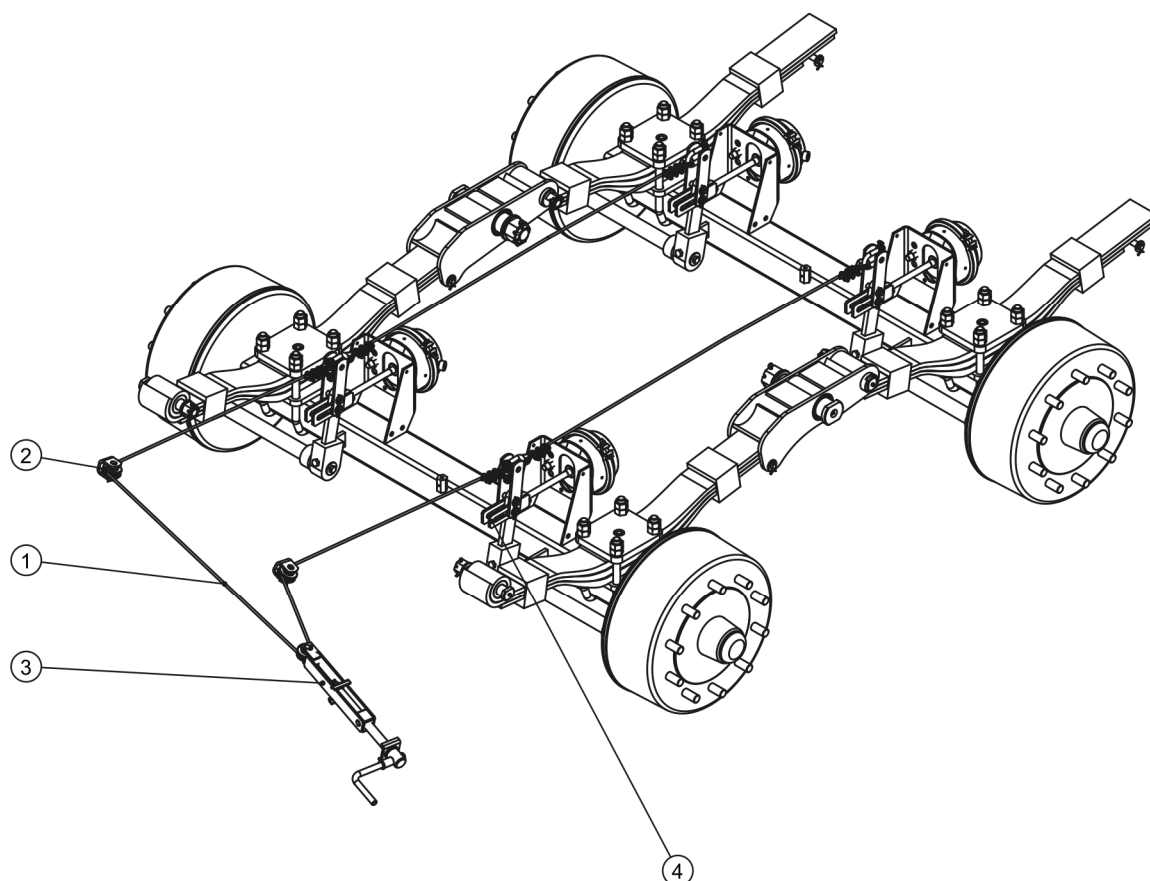
RYSUNEK 3.6A HAMULEC POSTOJOWY
