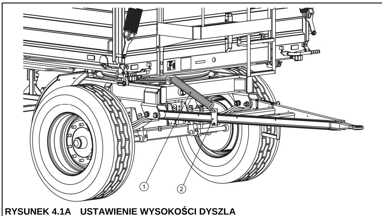
(1) sprężyna napinająca, (2) obejma
