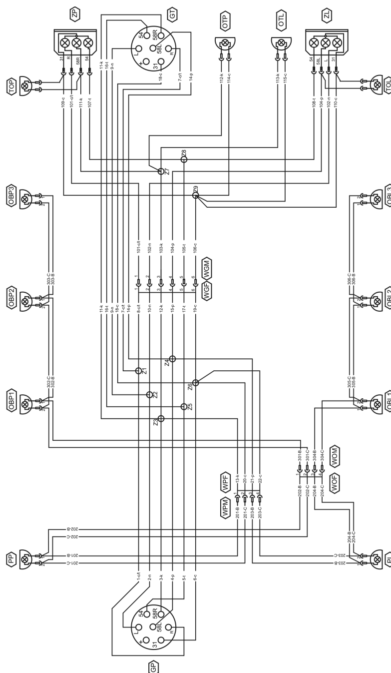
RYSUNEK 3.9A SCHEMAT INSTALACJI ELEKTRYCZNEJ
