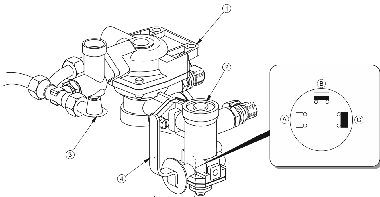
RYSUNEK 3.9 Zawór sterujący i regulator siły hamowania
