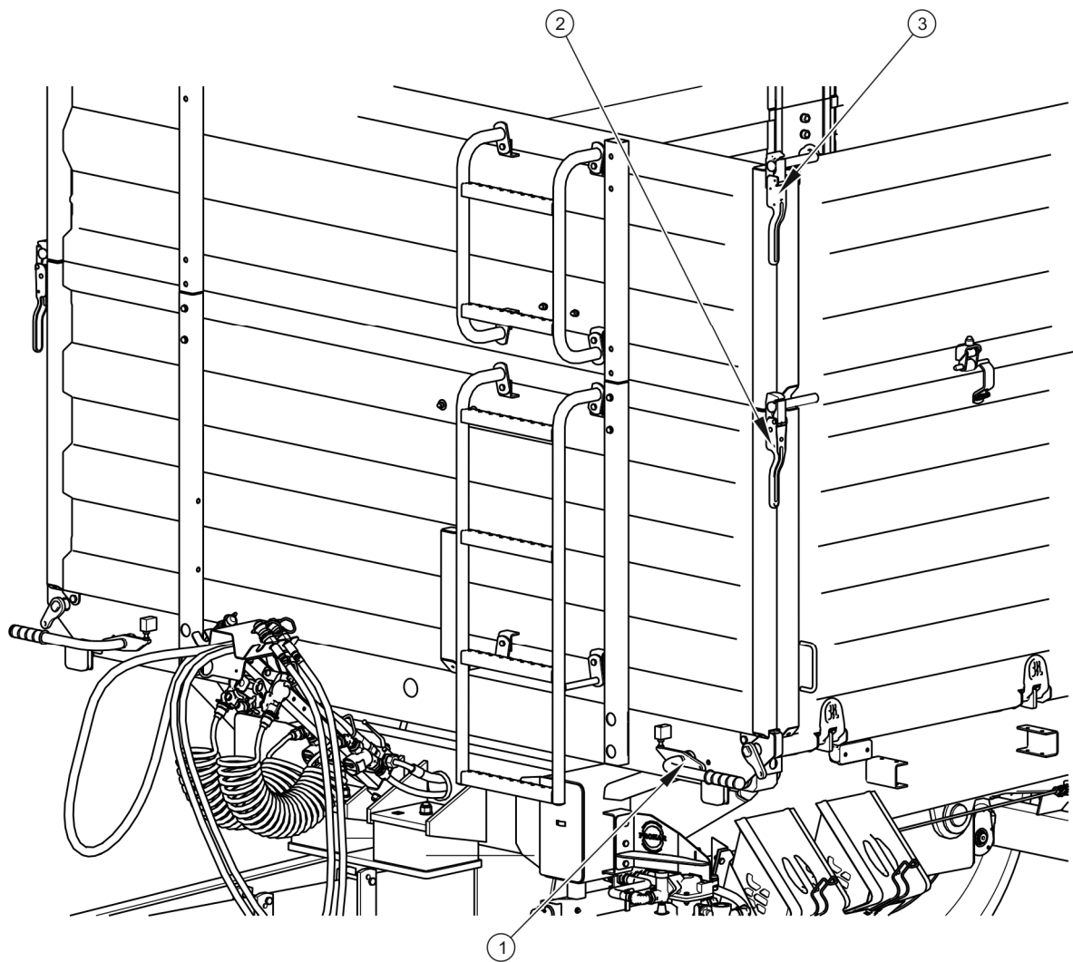
RYSUNEK 4.4 Zamki ścian i nadstaw skrzyniowych z przodu
