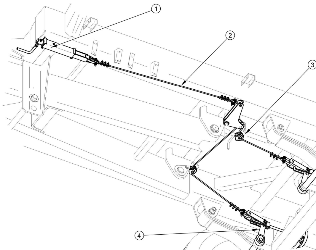
RYSUNEK 3.13 Budowa hamulca postojowego
