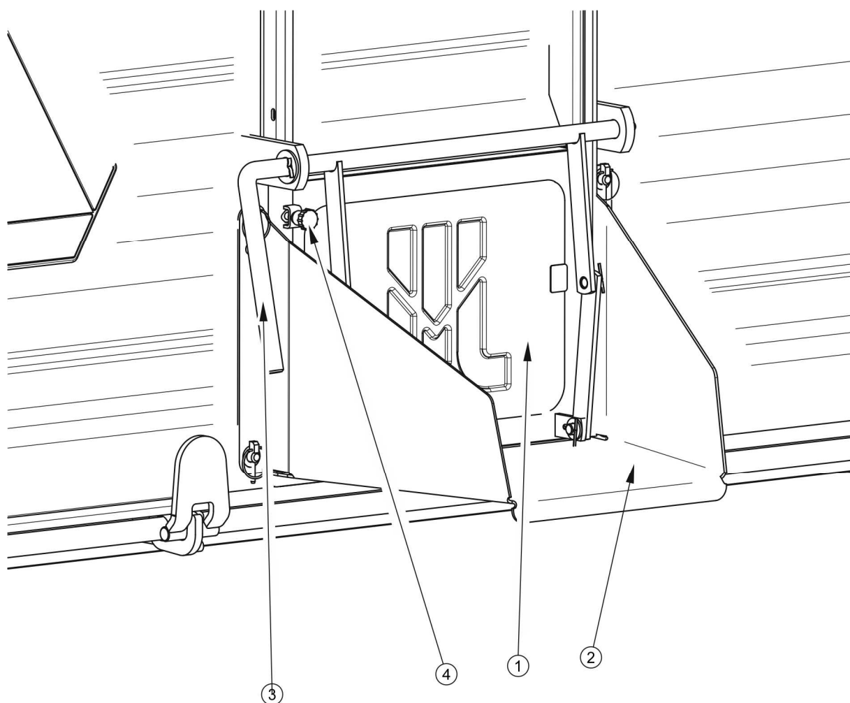
RYСУNEK 4.6 Zamki ścian i nadstaw skrzyniowych
