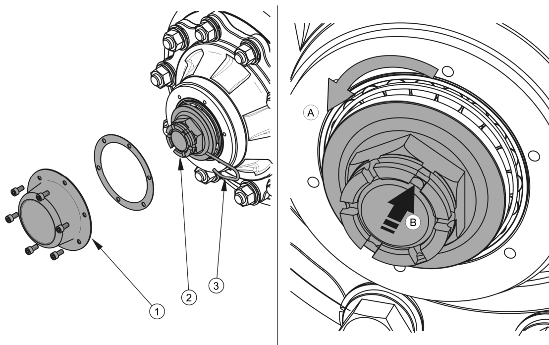
RYСУNEK 5.2 Regulacja łożysk osi jezdnej
