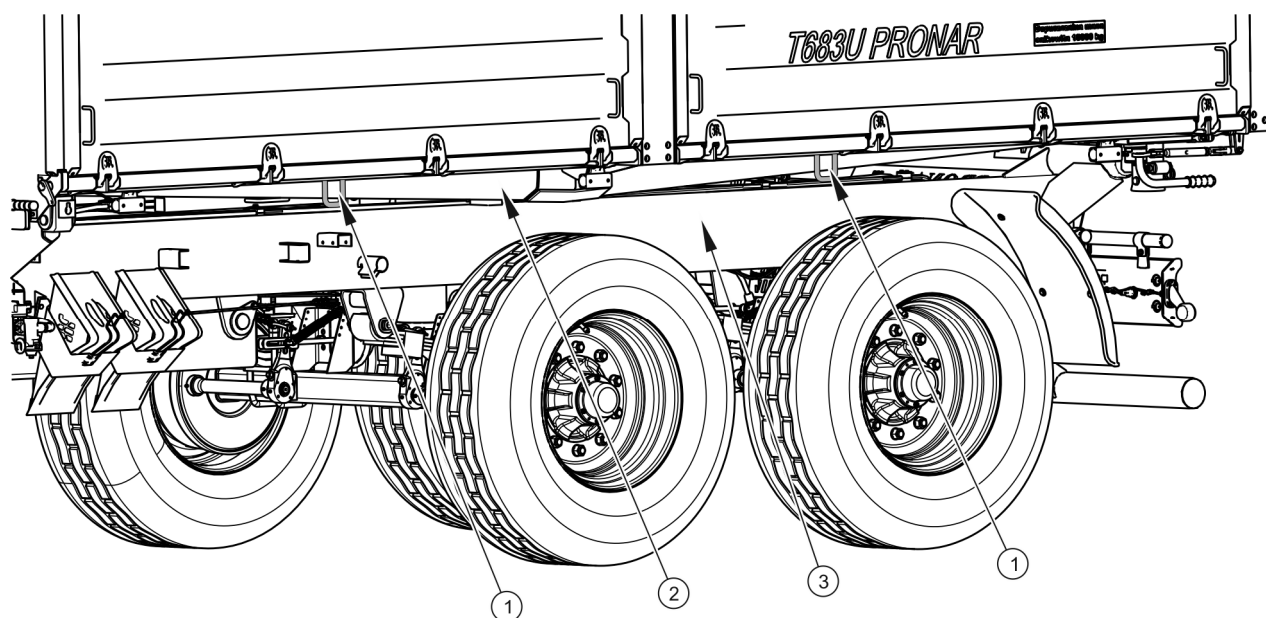
RYSUNEK 1.3 Rozmieszczenie uchwytów transportowych
