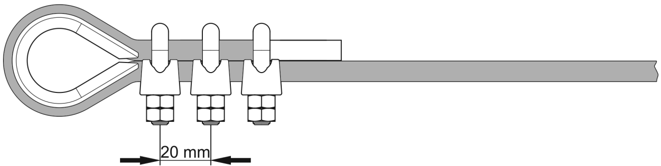
RYSUNEK 5.8 Montaż zacisków linki hamulcowej
