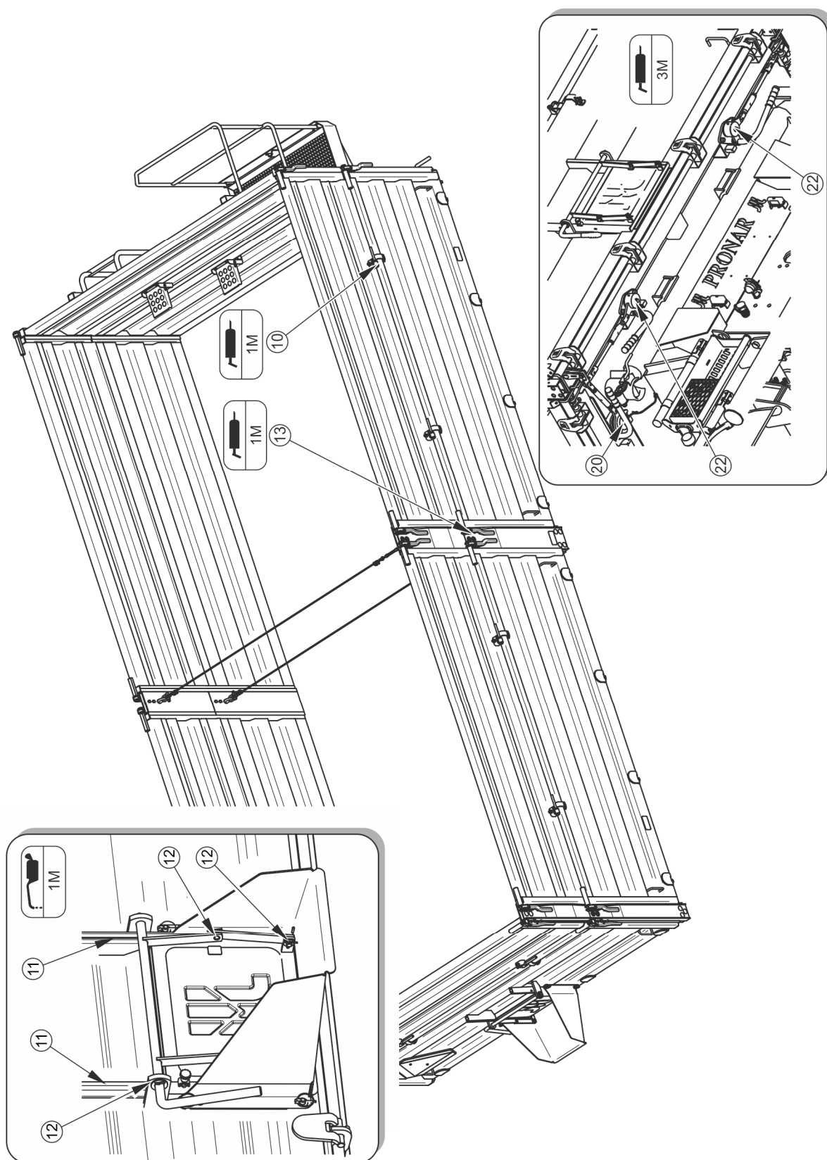
RYSUNEK 5.13 Punkty smarne przyczepy, część 2
