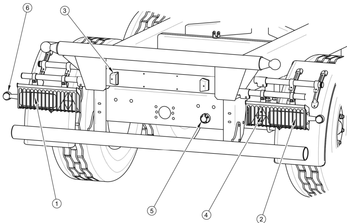
RYSUNEK 3.15 Rozmieszczenie elementów instalacji elektrycznej oraz świateł odblaskowych – widok z tyłu
