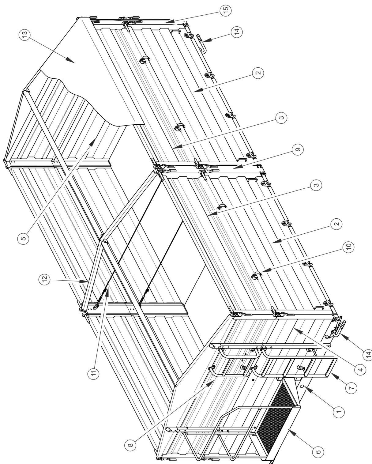
RYSUNEK 3.2 Skrzynia ładunkowa
