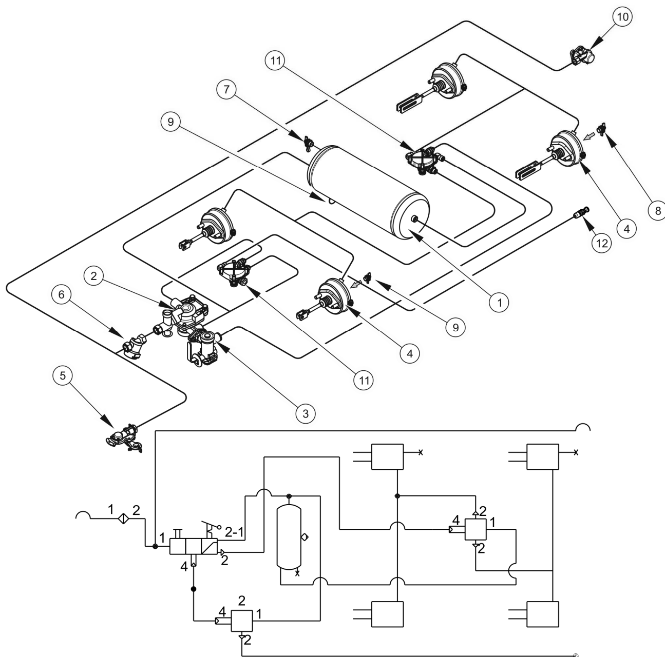
RYСУNEK 3.4 Budowa i schemat instalacji hamulcowej pneumatycznej jedнопроводowej
