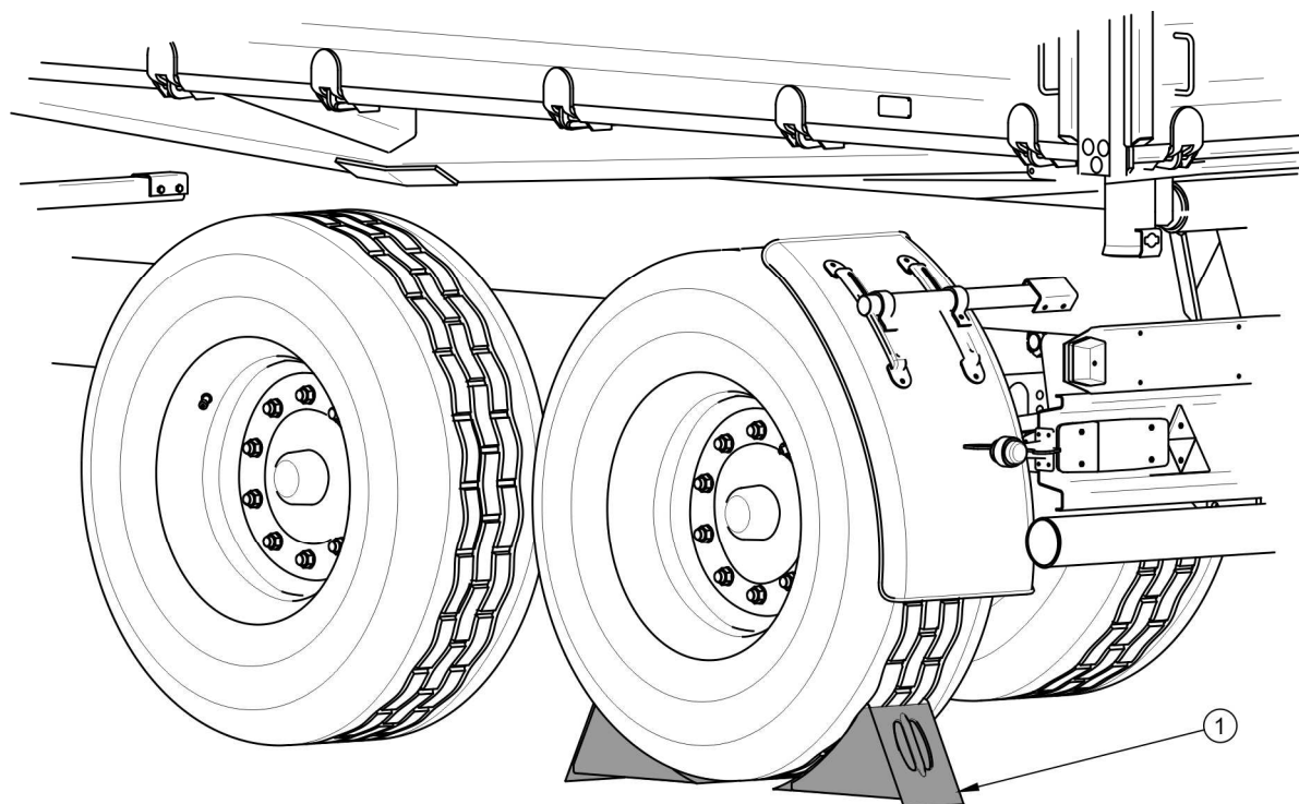
RYSUNEK 2.1 Sposób ustawiania klinów
