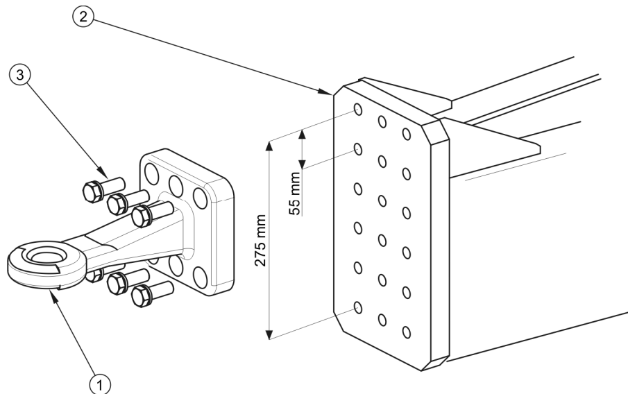
RYSUNEK 5.16 Regulacja położenia cięgna dyszla
