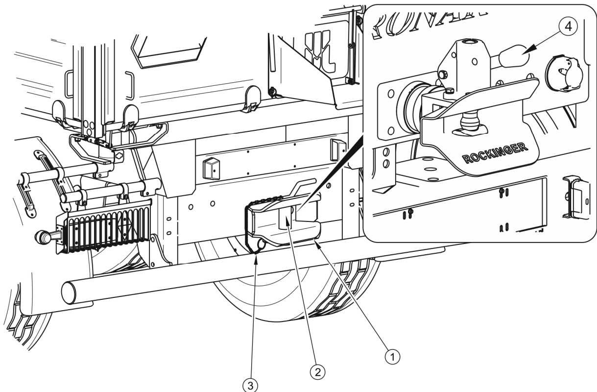
RYSUNEK 4.2 Zaczep tylny
