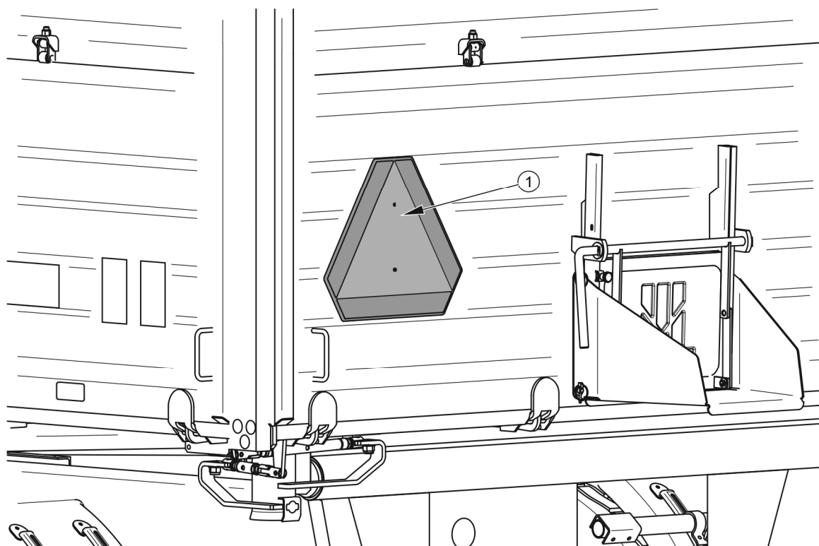
RYSUNEK 2.2 Miejsce montażu tablicy wyróżniającej pojazdy wolno poruszające się
