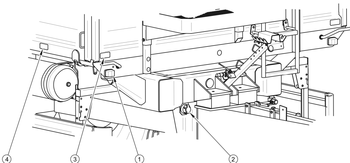
RYSUNEK 3.16 Rozmieszczenie elementów instalacji elektrycznej oraz świateł odblaskowych – widok z przodu
