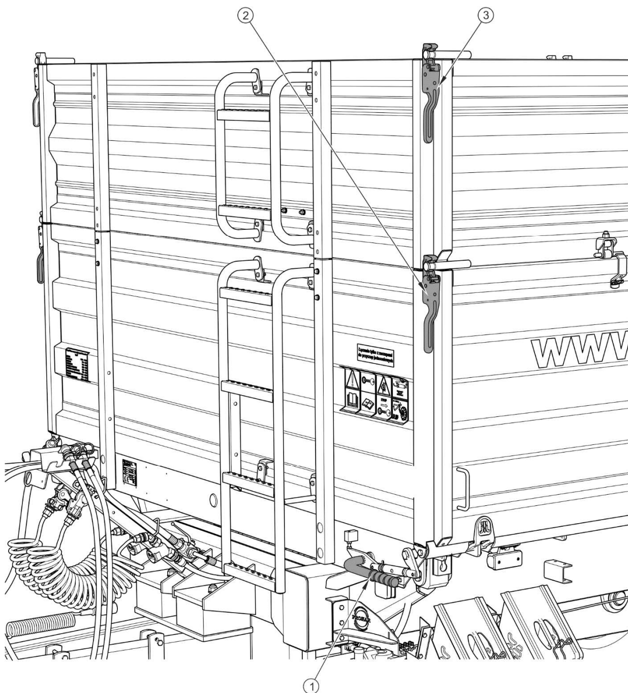
ABBILDUNG 4.4 Verschlüsse der Bordwände und Aufsätze der Ladekiste
