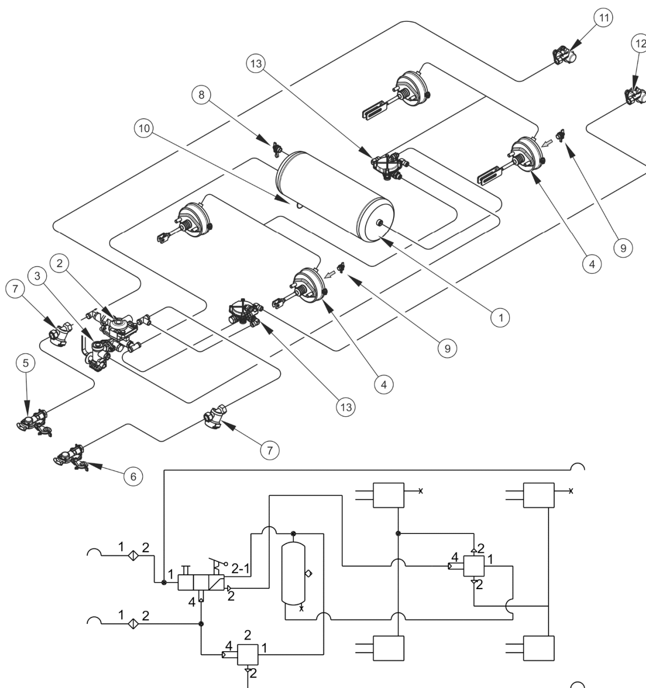
ABBILDUNG 3.5 Aufbau und Schema der Zweikreis-Druckluftbremse mit manuellem Bremskraftregler
