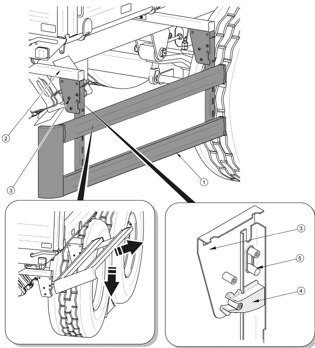
ABBILDUNG 4.7 Auffahrschutz links
