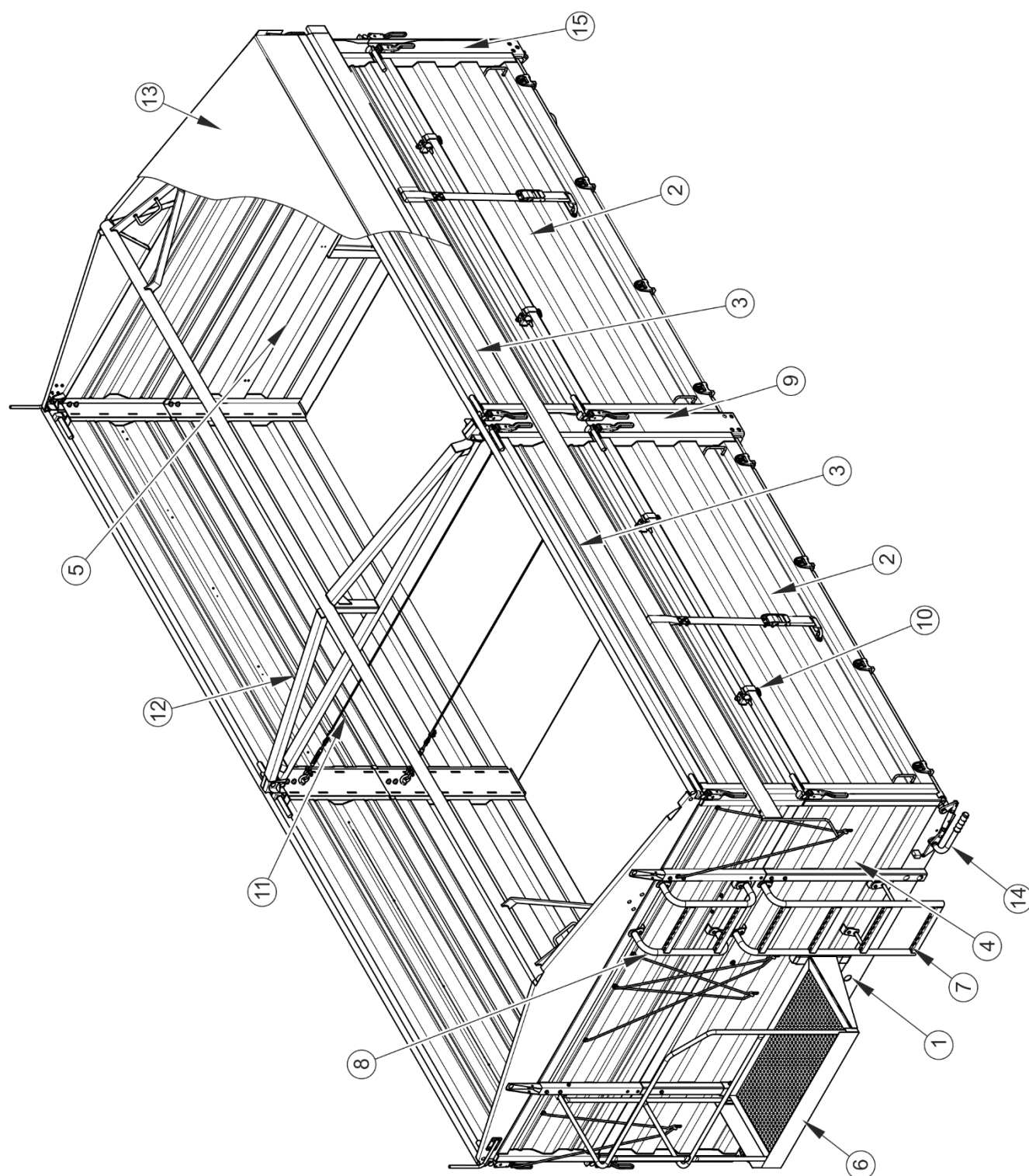
ABBILDUNG 3.2 Ladekasten - Rückansicht
