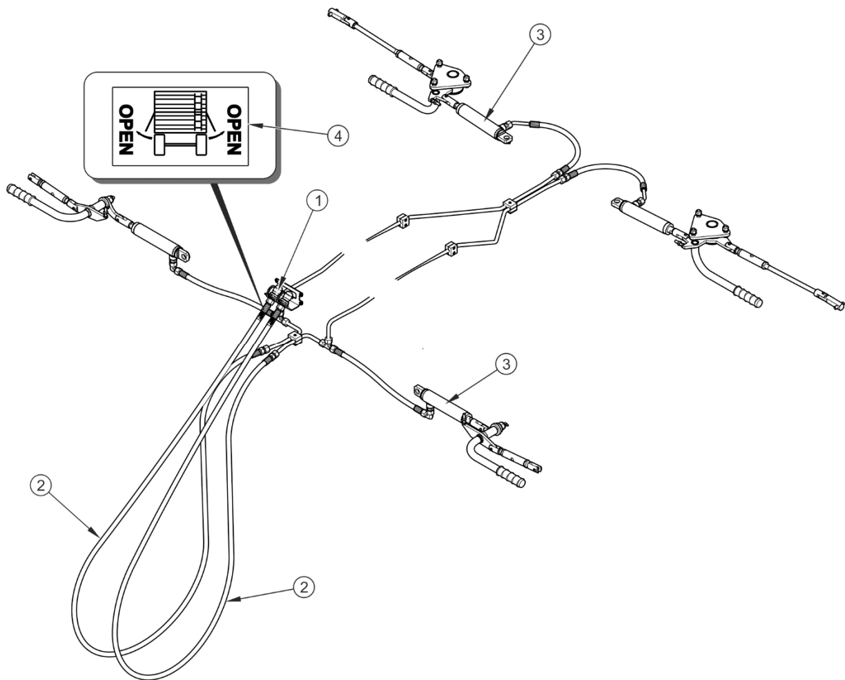
ABBILDUNG 3.13 Aufbau der Hydraulik zum Entriegeln der Bordwände
