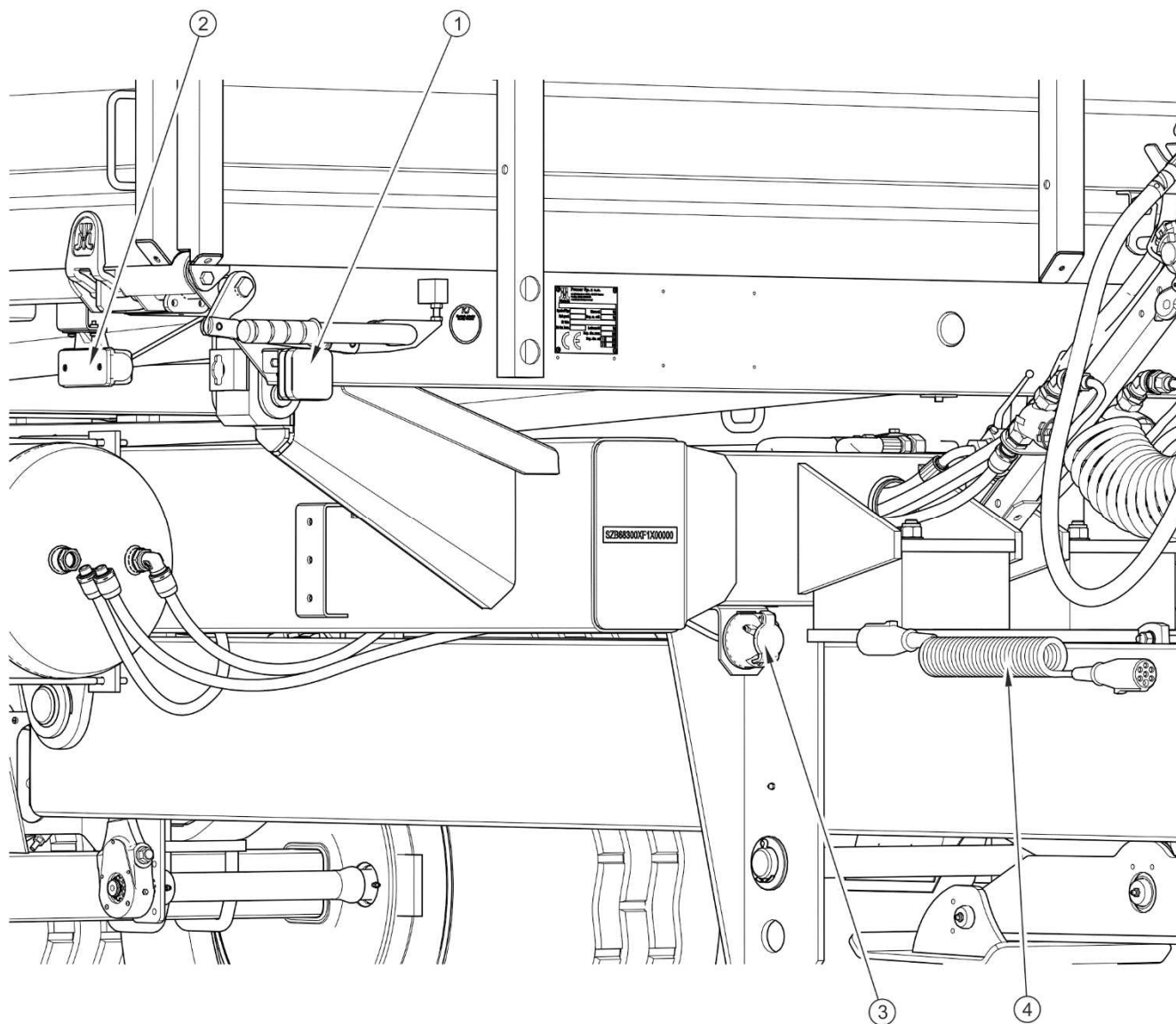
ABBILDUNG 3.18 Anordnung der Elemente der elektrischen Ausstattung – Vorderansicht
