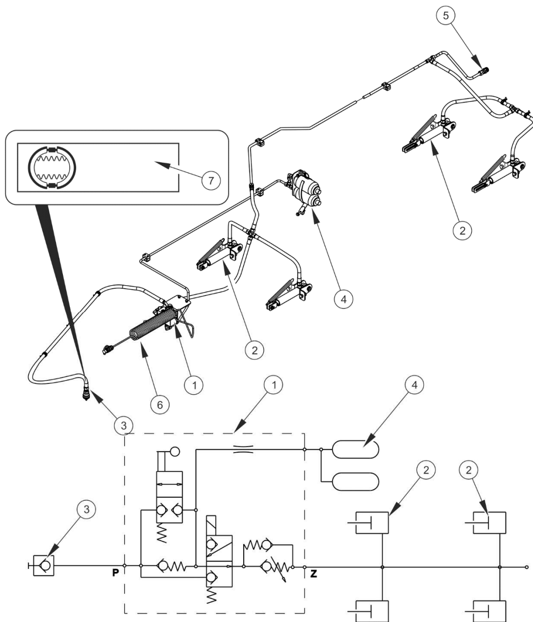
ABBILDUNG 3.7 Aufbau und Schema der Hydraulikbremse
