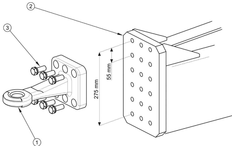
ABBILDUNG 5.17 Einstellung der Deichselhöhe
