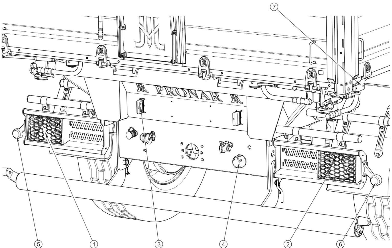
ABBILDUNG 3.17 Anordnung der Elemente der elektrischen Ausstattung – Rückansicht
