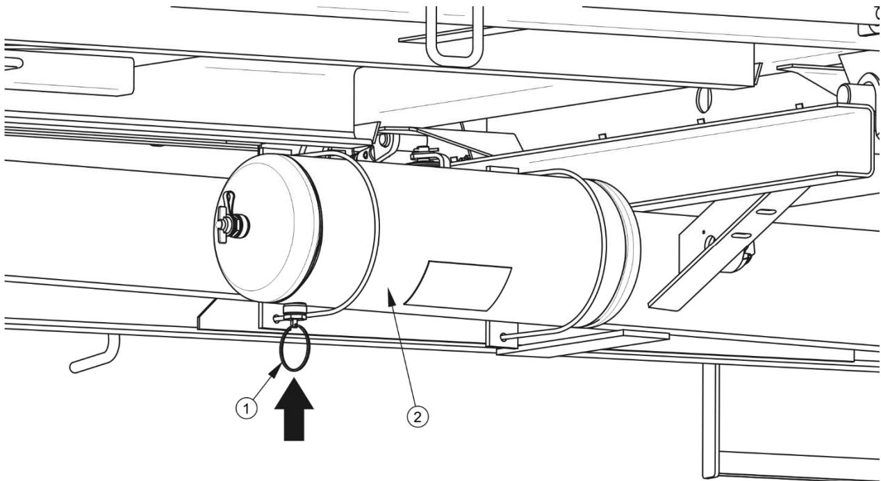
ABBILDUNG 5.10 Entwässerung des Druckluftbehälters
