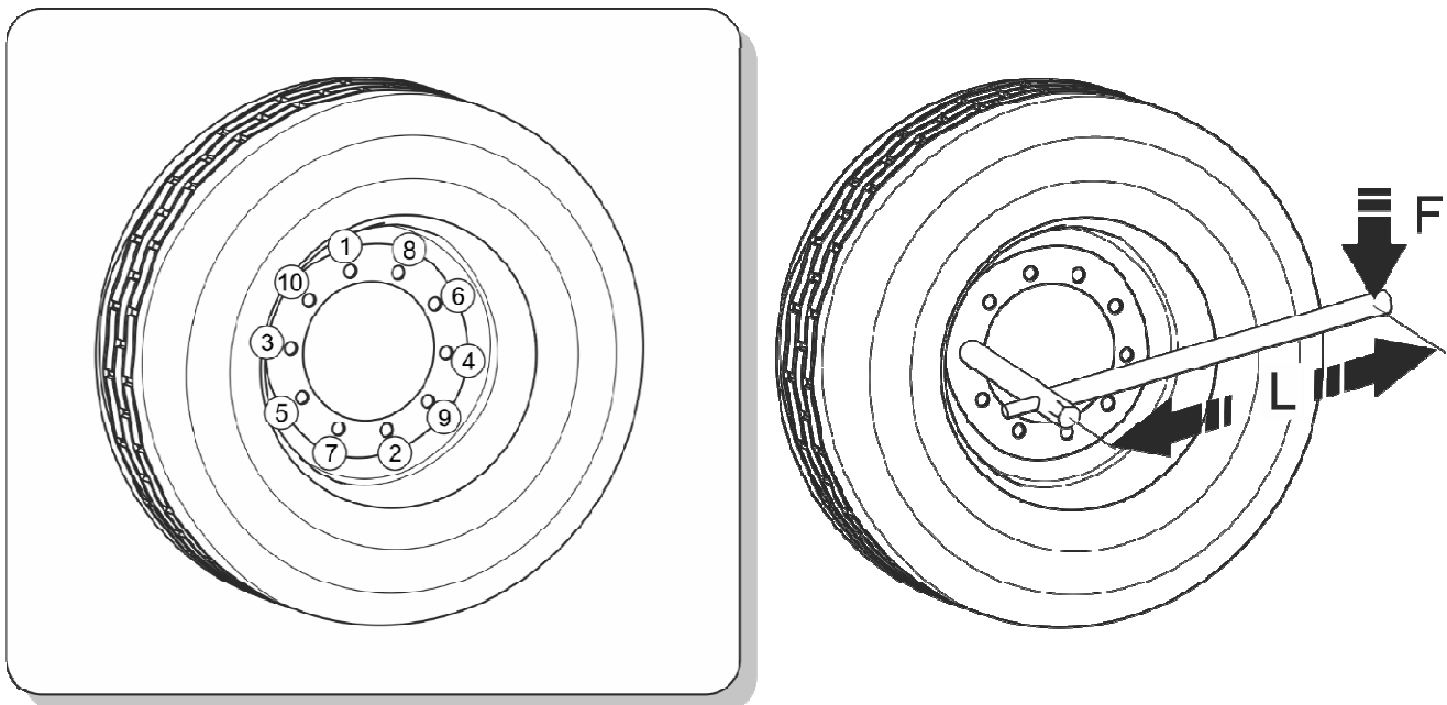
ABBILDUNG 5.3 Anziehreihenfolge der Muttern
