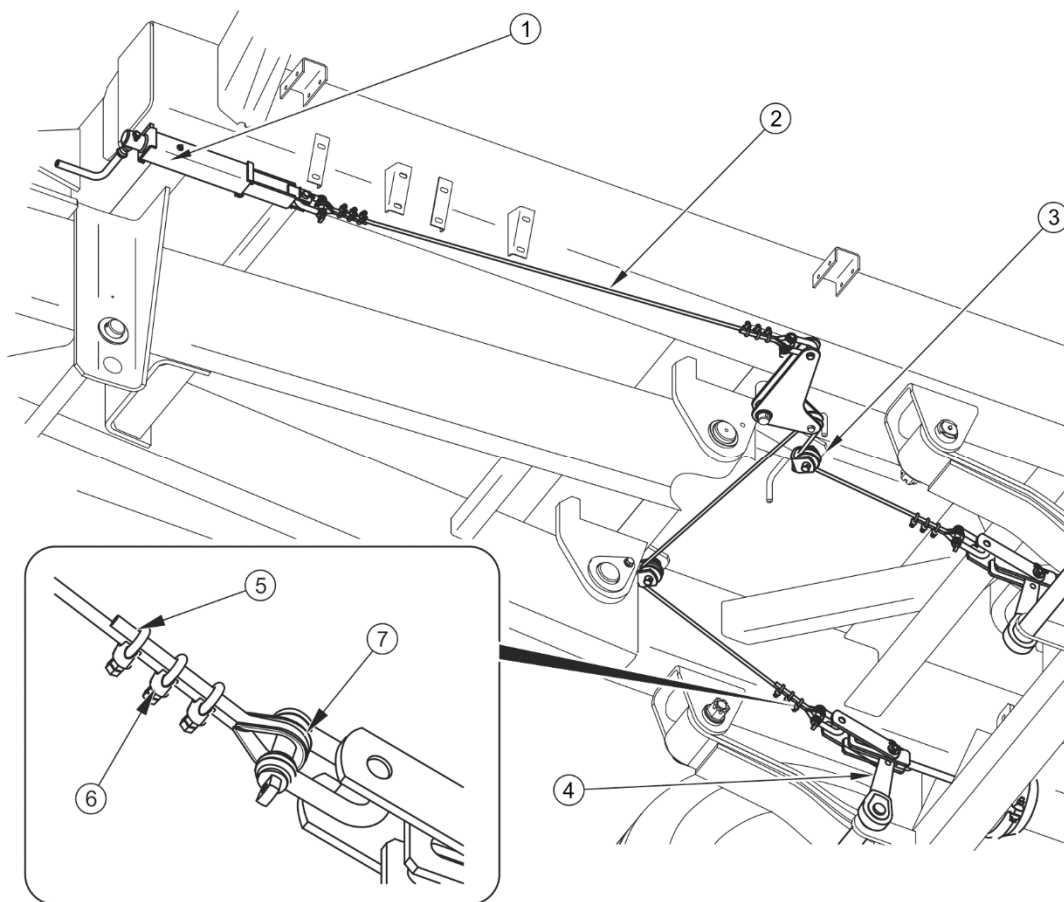
ABBILDUNG 5.7 Einstellung der Betriebsbremse
