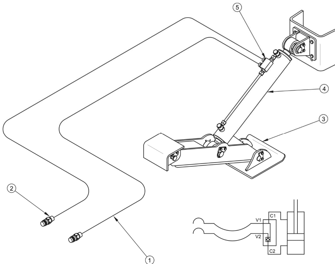
ABBILDUNG 3.12 Aufbau und Schema der Hydraulikanlage der Anhängerstütze
