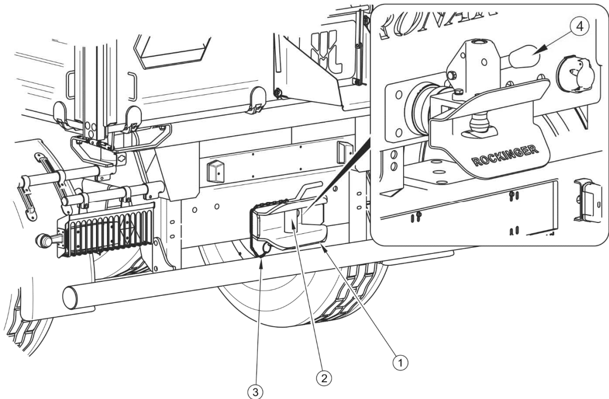
ABBILDUNG 4.2 Hintere Anhängerkupplung
