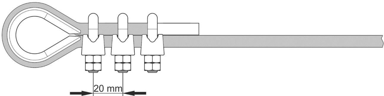
ABBILDUNG 5.8 Montage der Bremsseilklemmen
