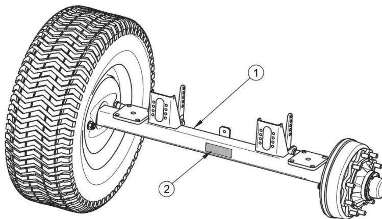
ABBILDUNG 1.2 Lokalisierung des Typenschildes an der Fahrachse
