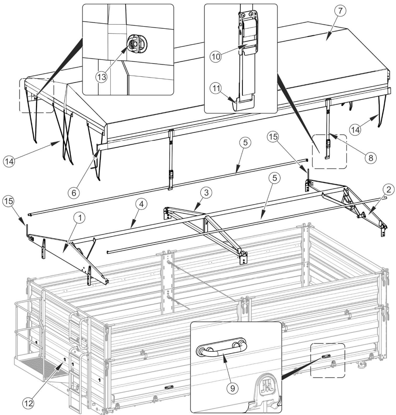
ABBILDUNG 5.16 Gestell mit Plane
