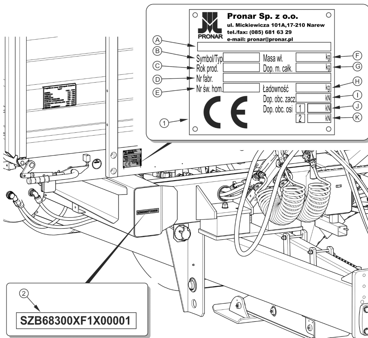
ABBILDUNG 1.1 Lokalisierung des Typenschilds und der eingeschlagenen Seriennummer
