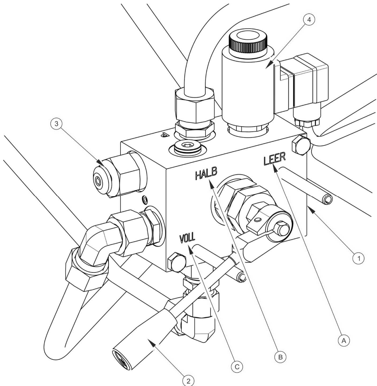
ABBILDUNG 3.10 Elektrohydraulisches Bremsventil
