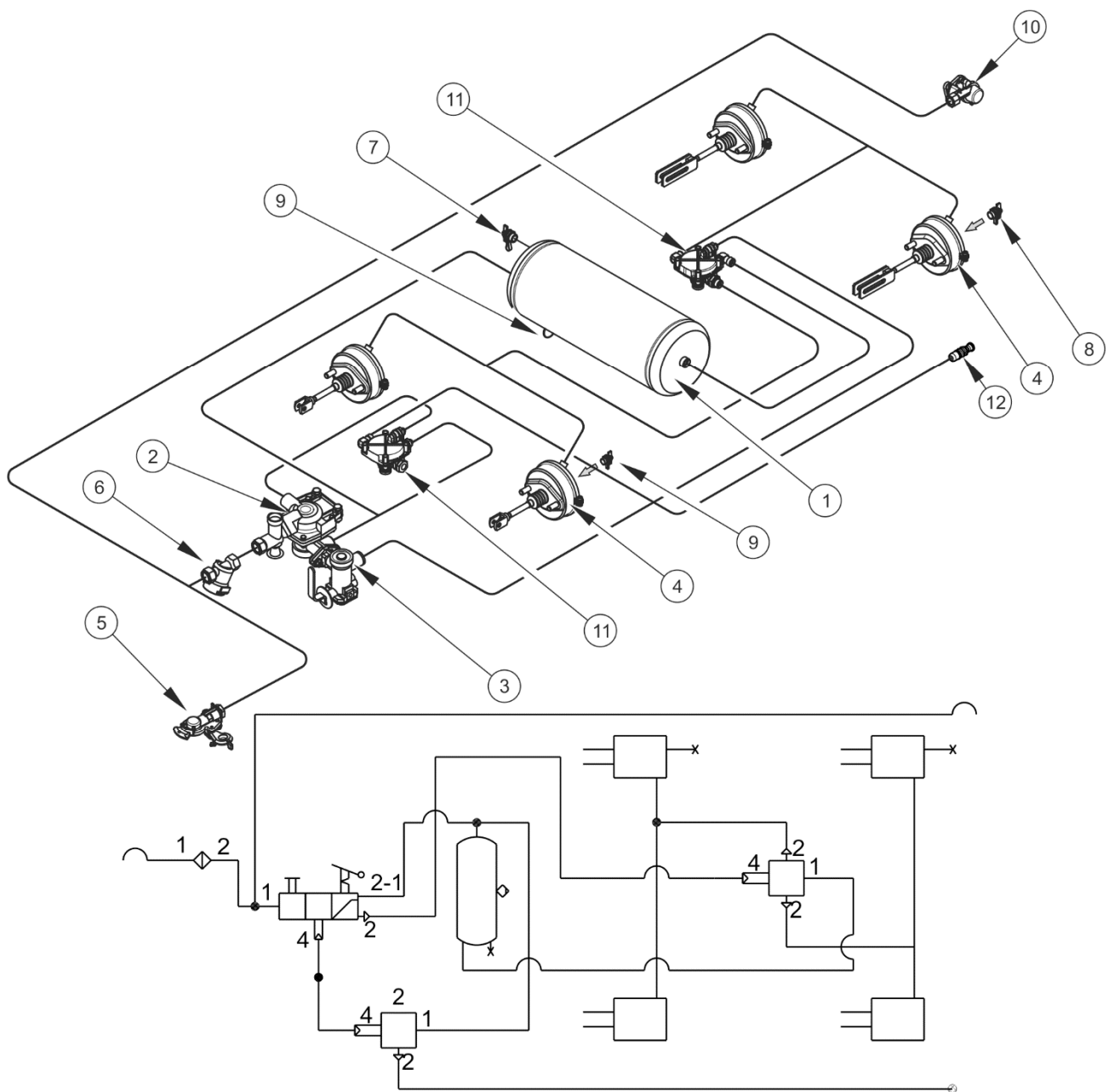
ABBILDUNG 3.4 Aufbau und Schema der Einkreisdruckluftbremse
