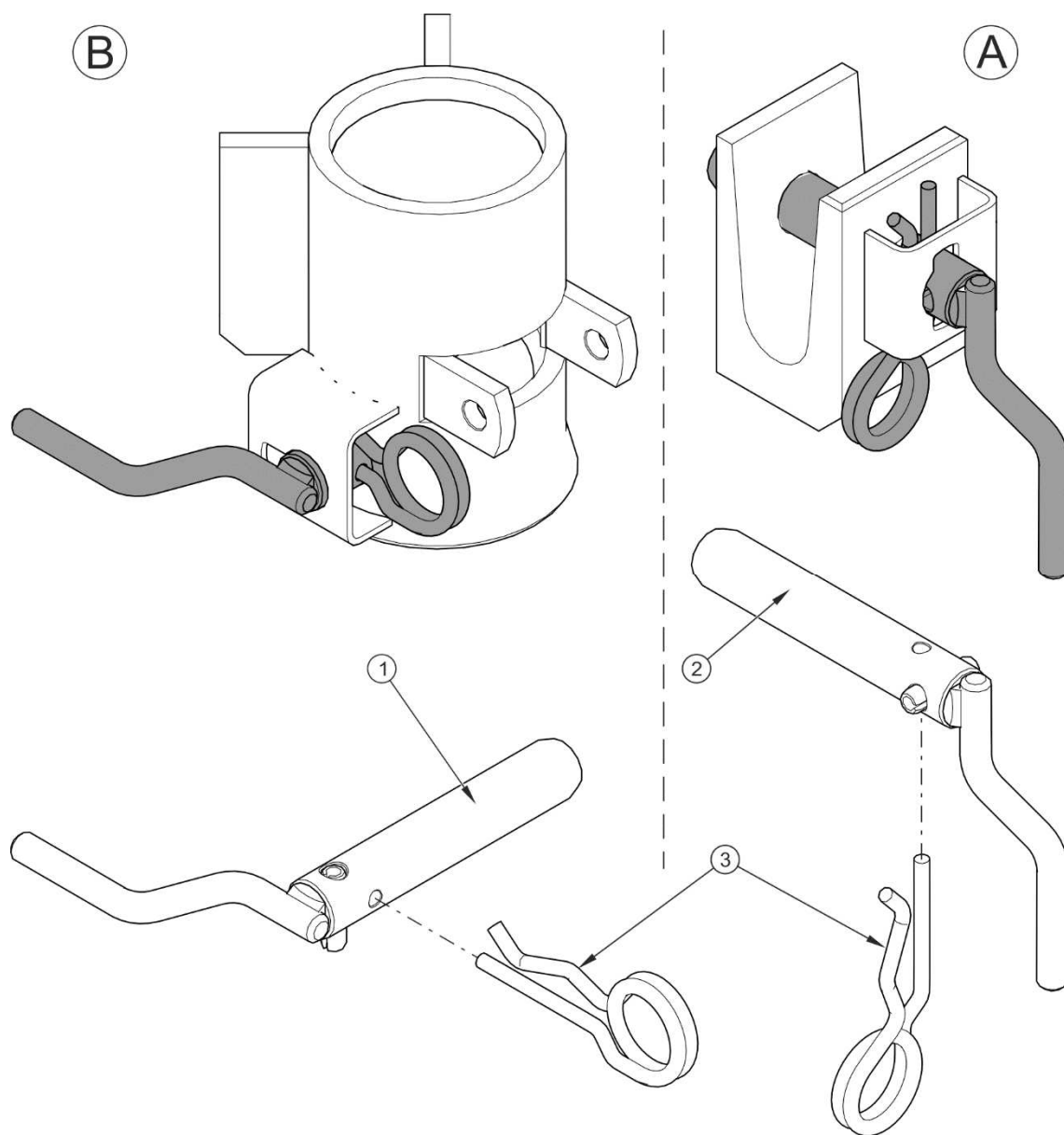
ABBILDUNG 4.3 Verriegelung der Kippbolzen
