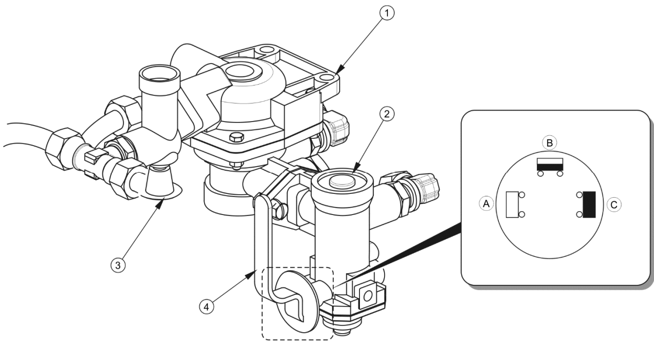
ABBILDUNG 3.9 Steuerventil und Bremskraftregler
