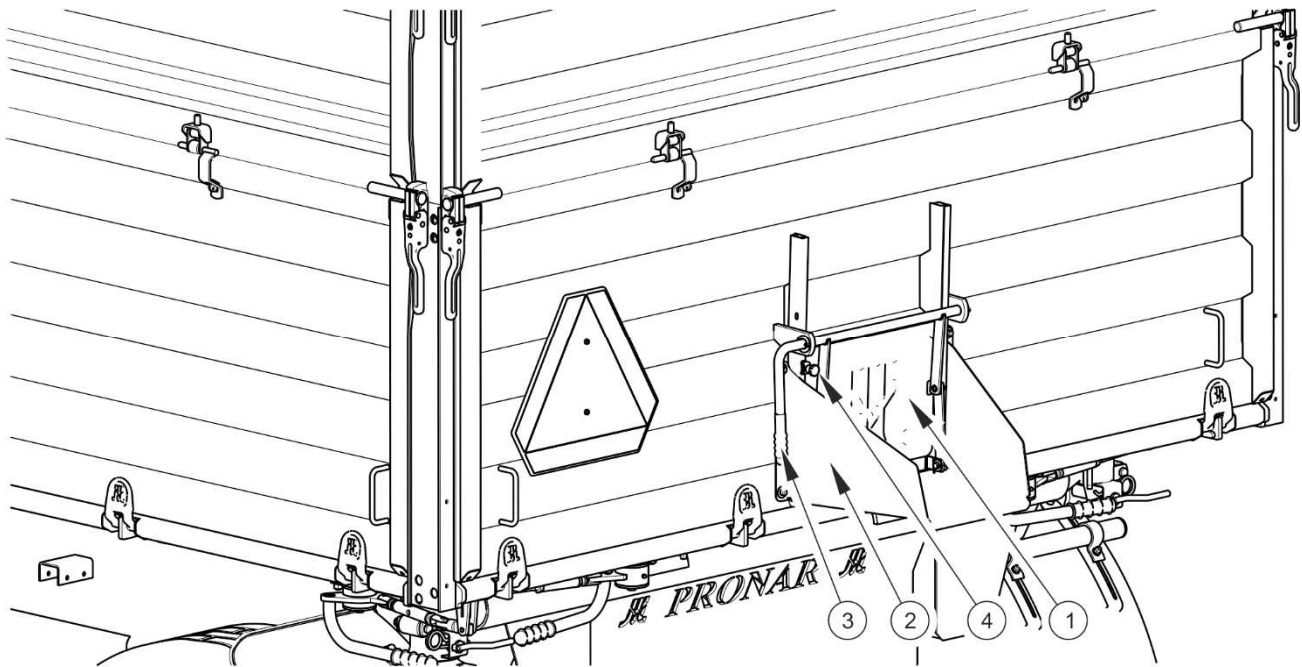
ABBILDUNG 3.3 Schieber der Heckbordwand
