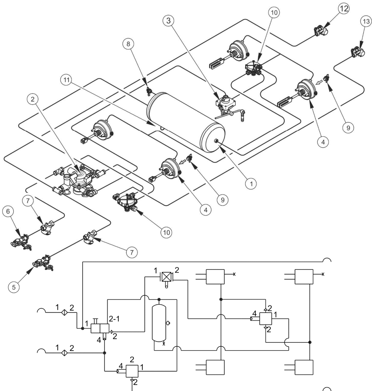
ABBILDUNG 3.6 Aufbau und Schema der Zweikreis-Druckluftbremse mit manuellem Bremskraftregler
