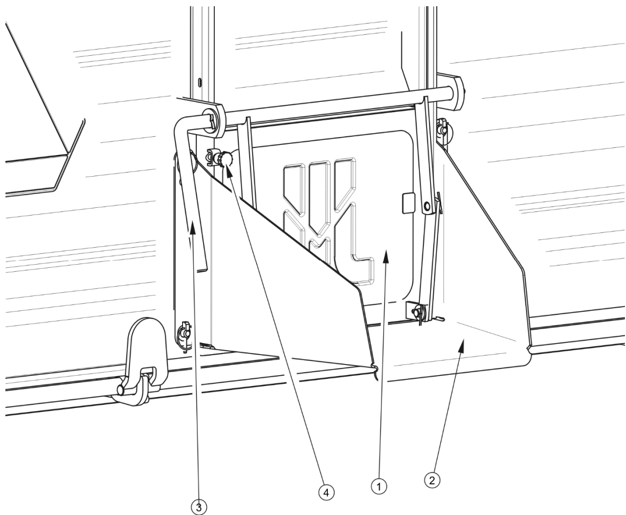
ABBILDUNG 4.6 Auslaufgosse
