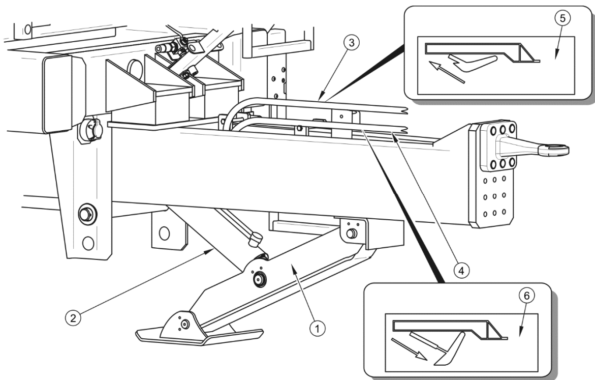
ABBILDUNG 4.1 Anhängerstütze
