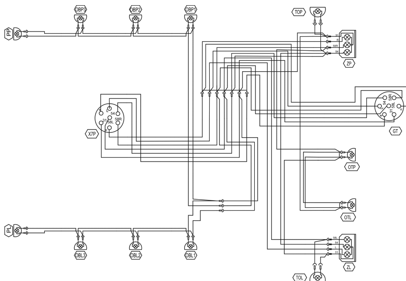
ABBILDUNG 3.16 Schaltplan der Elektroinstallation
