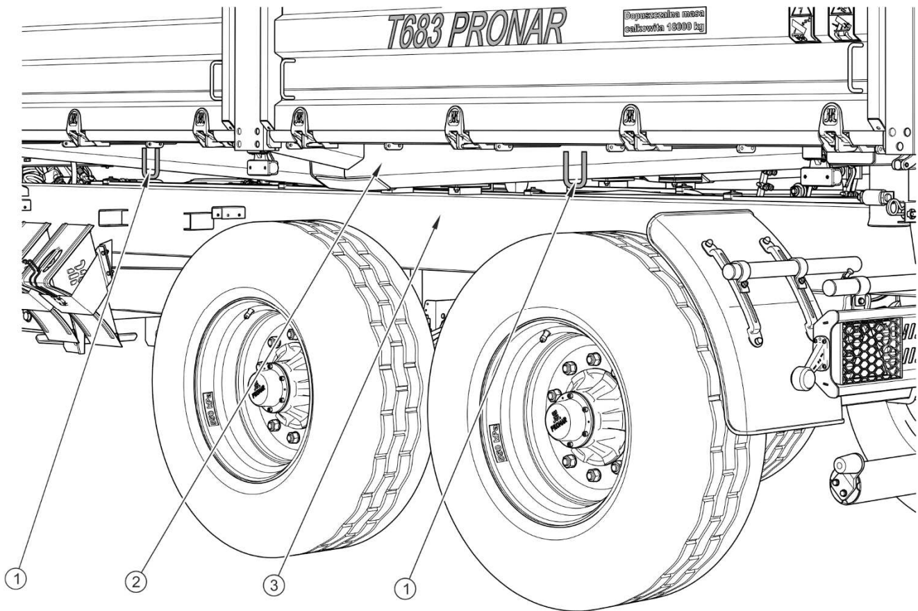
ABBILDUNG 1.3 Anordnung der Transporthalterungen
