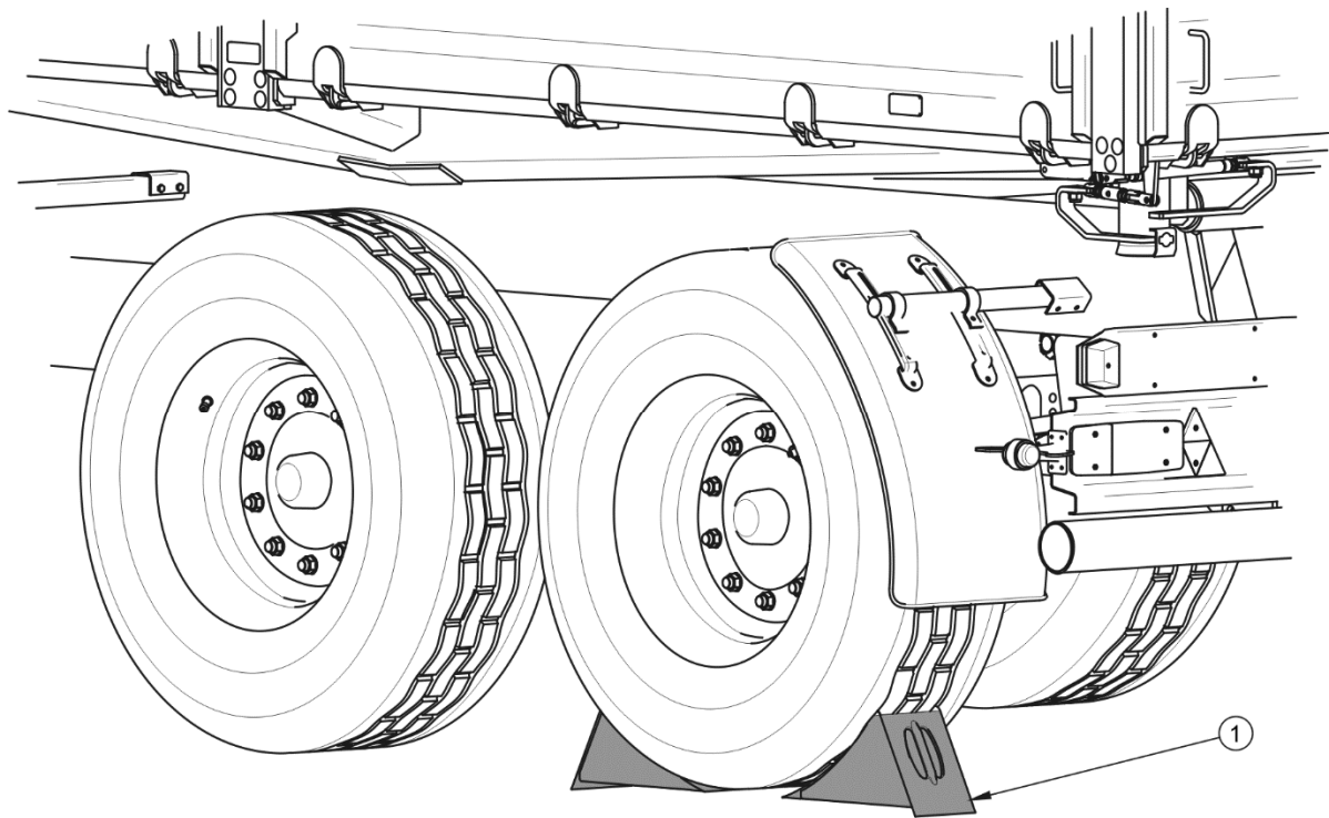
ABBILDUNG 2.1 Unterlegen der Keile
