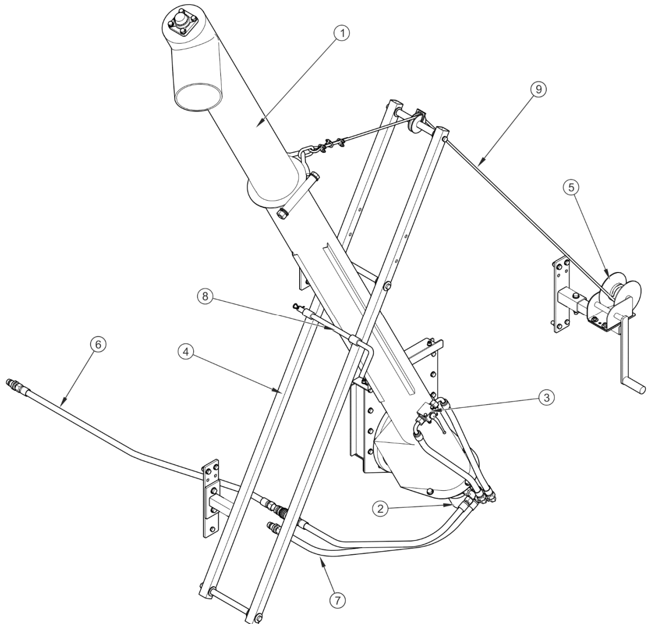
ABBILDUNG 3.14 Aufbau der Hydraulikanlage des Förderers
