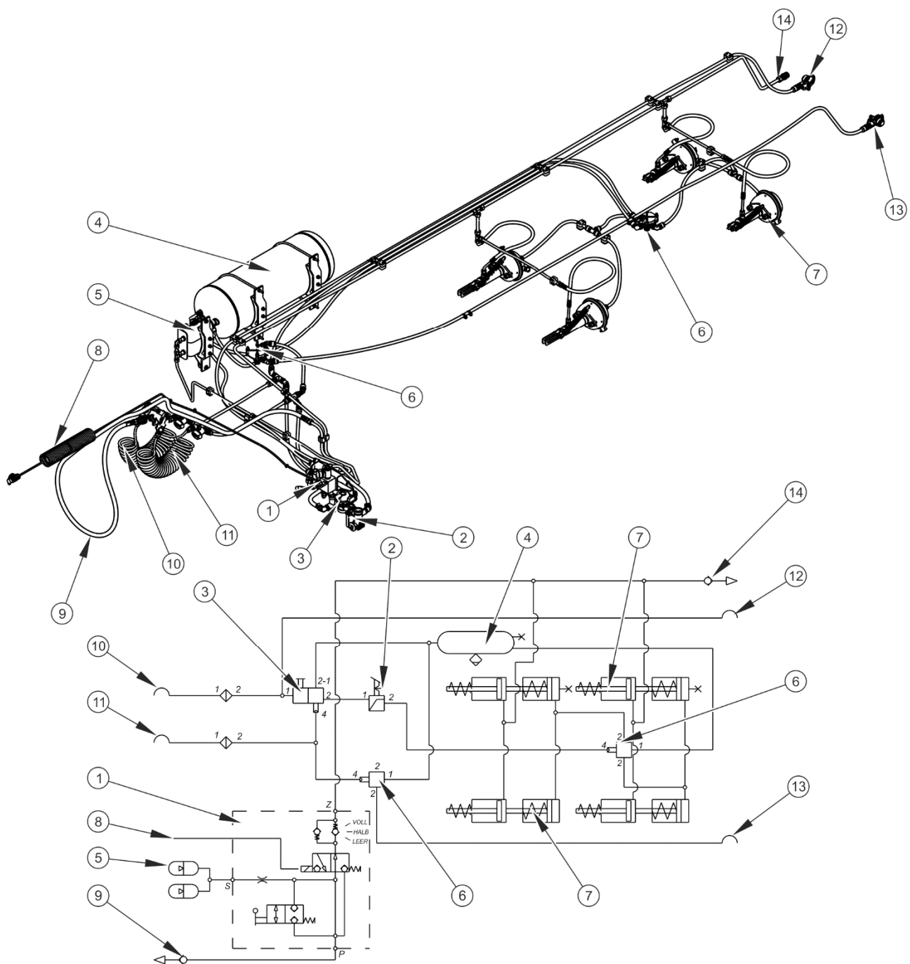
ABBILDUNG 3.8 Aufbau und Schema der kombinierten Bremsanlage – Hydraulik-/Druckluftanlage
