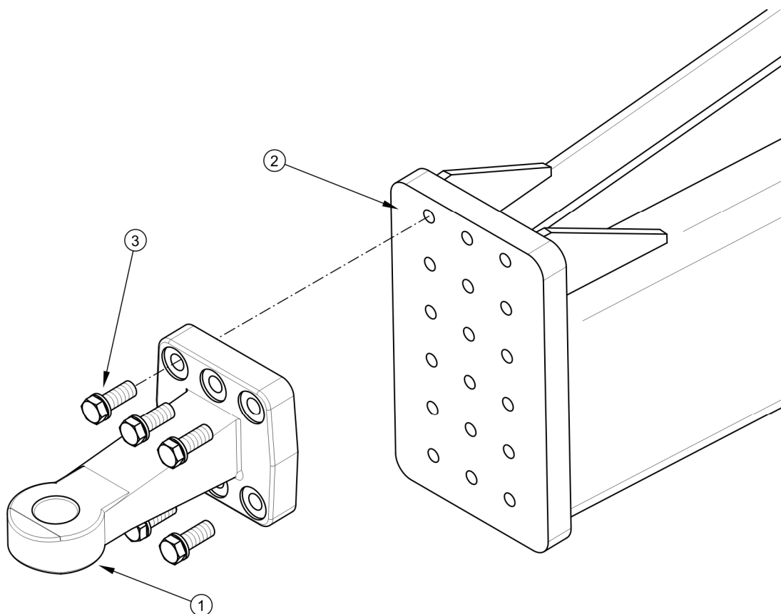
RYСУNEK 5.16 Regulacja położenia dyszla
