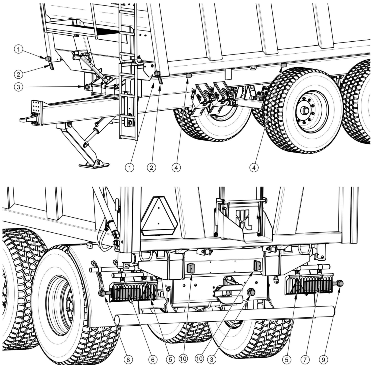
RYSUNEK 3.14 Rozmieszczenie elementów elektrycznych i odblaskowych
