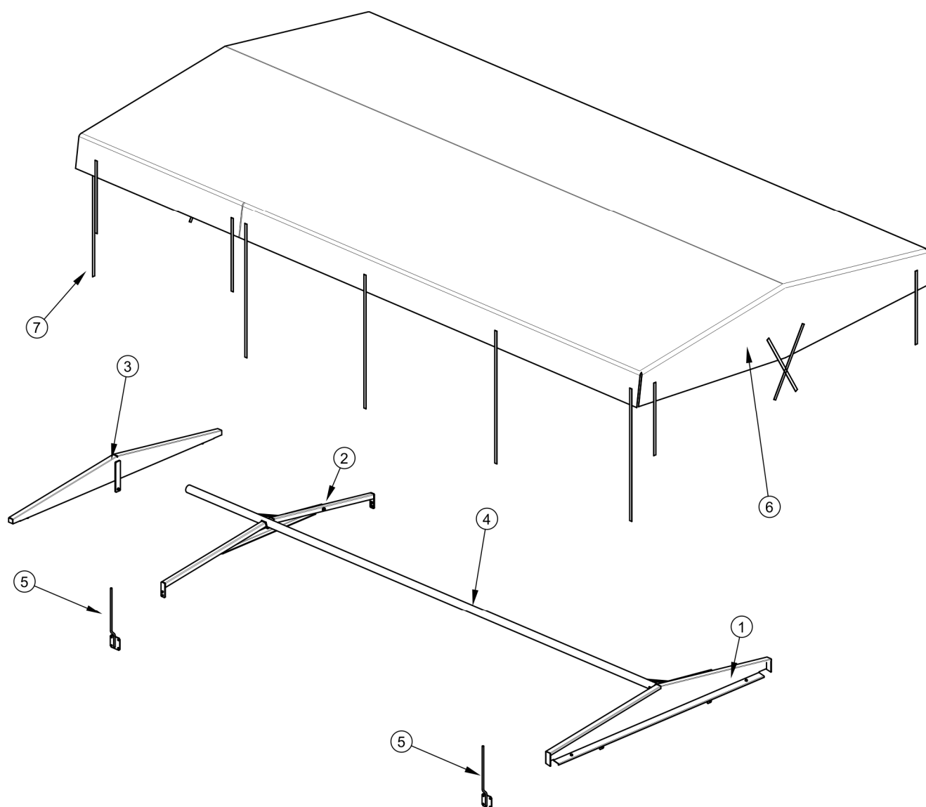
RYСУNEK 5.15 Stelaż z plancką
