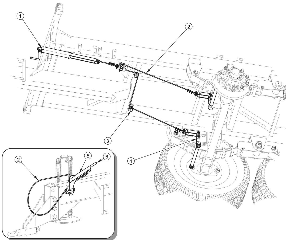
РИСУНОК 3.17 Устройство стояночного тормоза с кривошипным механизмом
