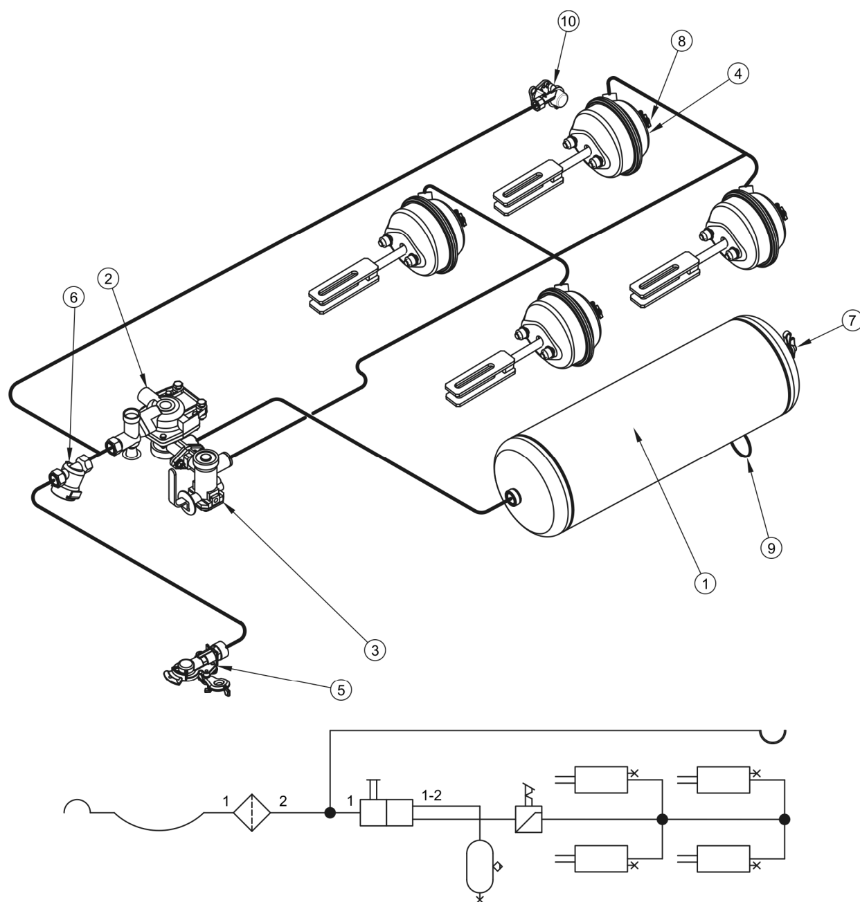
РИСУНОК 3.7 Устройство и схема однопроводной пневматической тормозной системы
