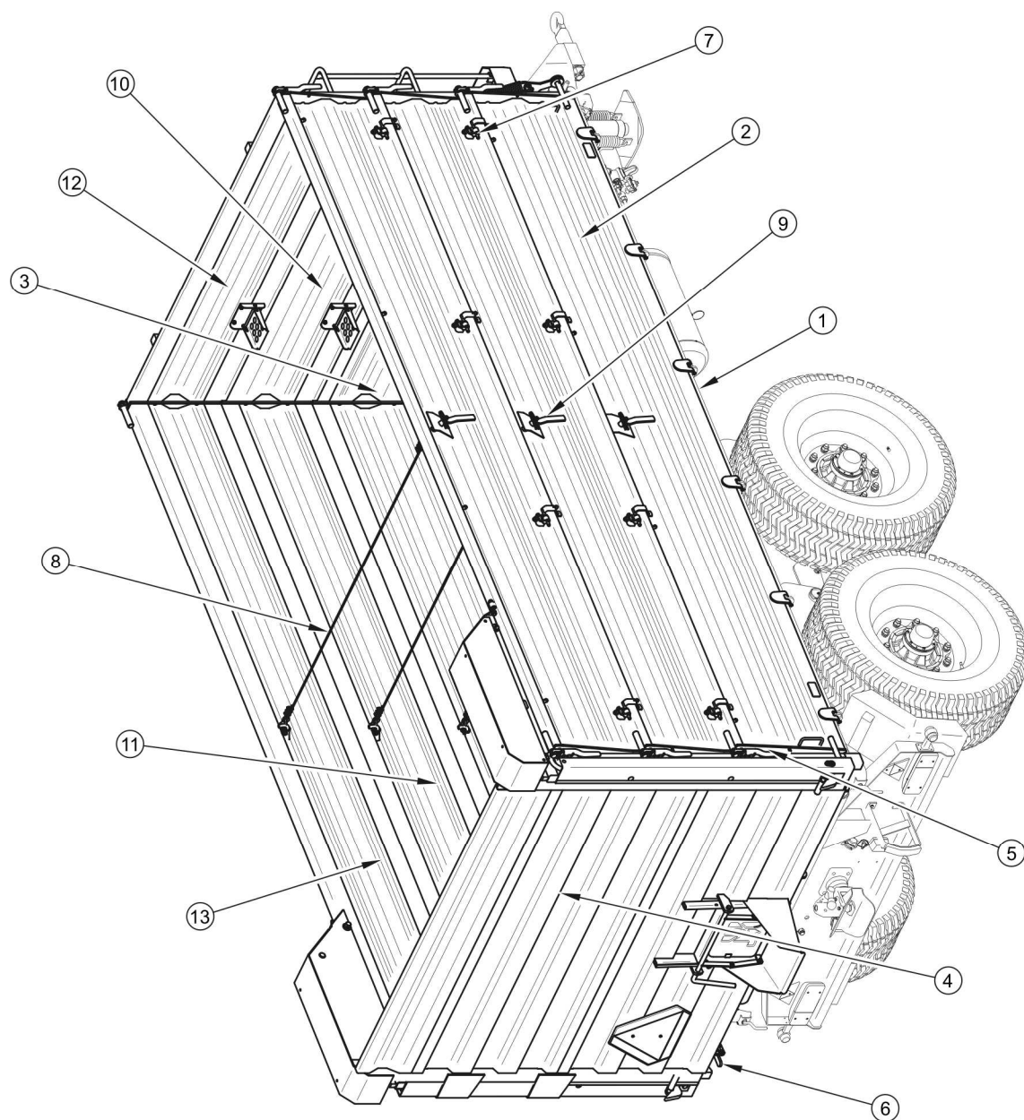
РИСУНОК 3.4 Грузовая платформа тип SILO
