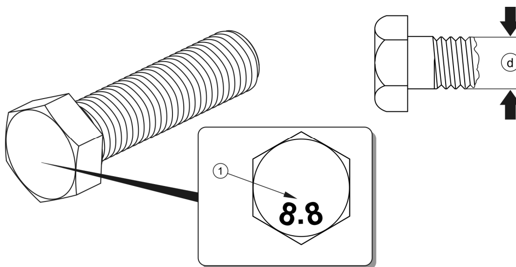
РИСУНОК 5.11 Болт с метрической резьбой
