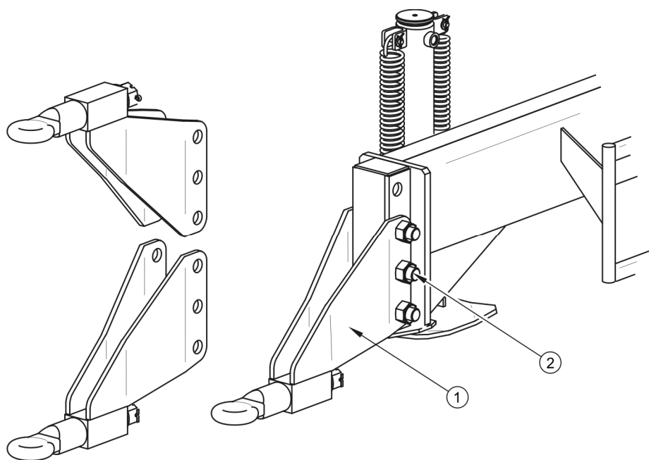
РИСУНОК 5.12 Регулирование положения дышла
