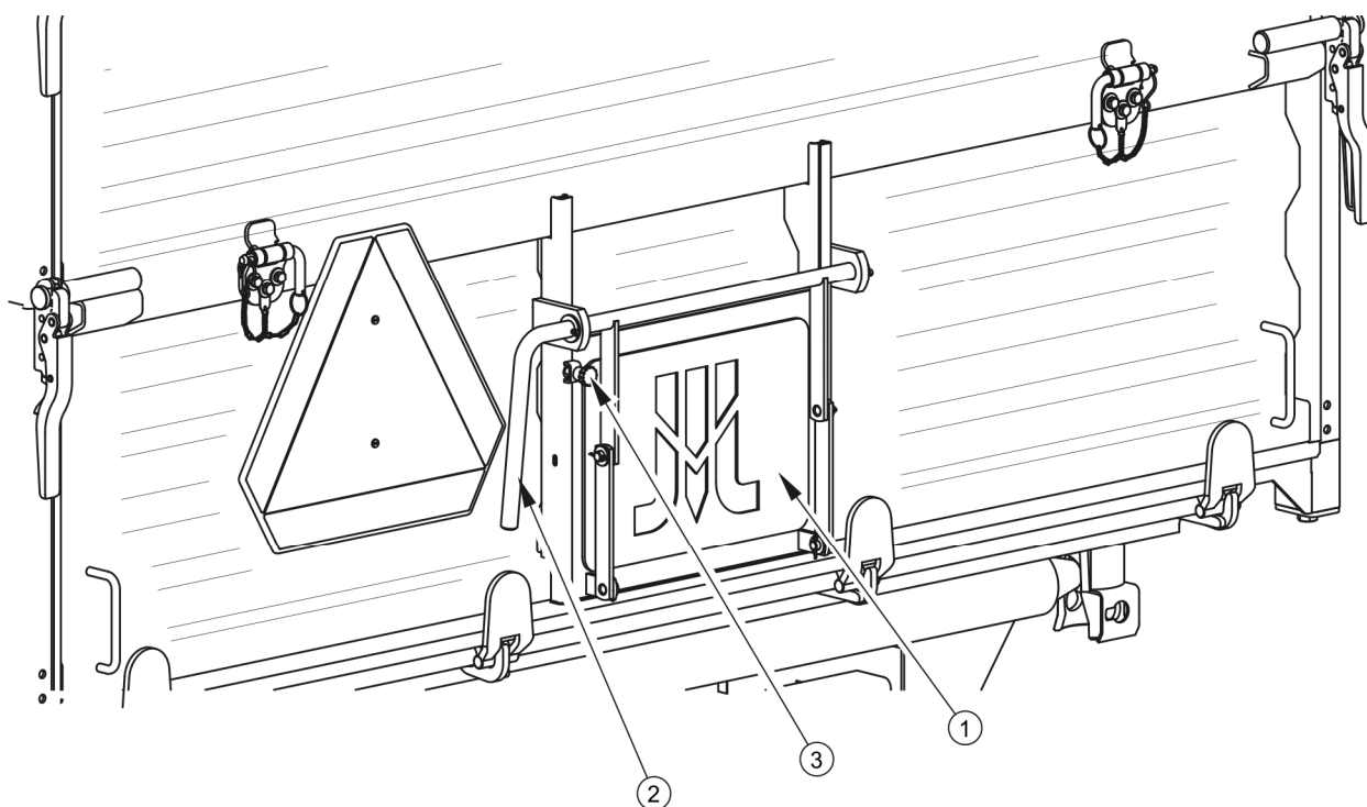
РИСУНОК 3.6 Разгрузочный люк в заднем борту
