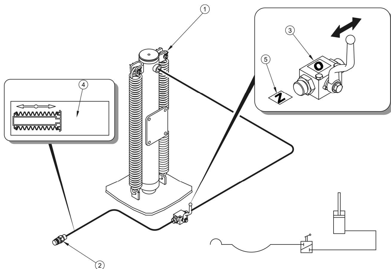
РИСУНОК 3.13 Устройство и схема гидравлической системы прямой опоры
