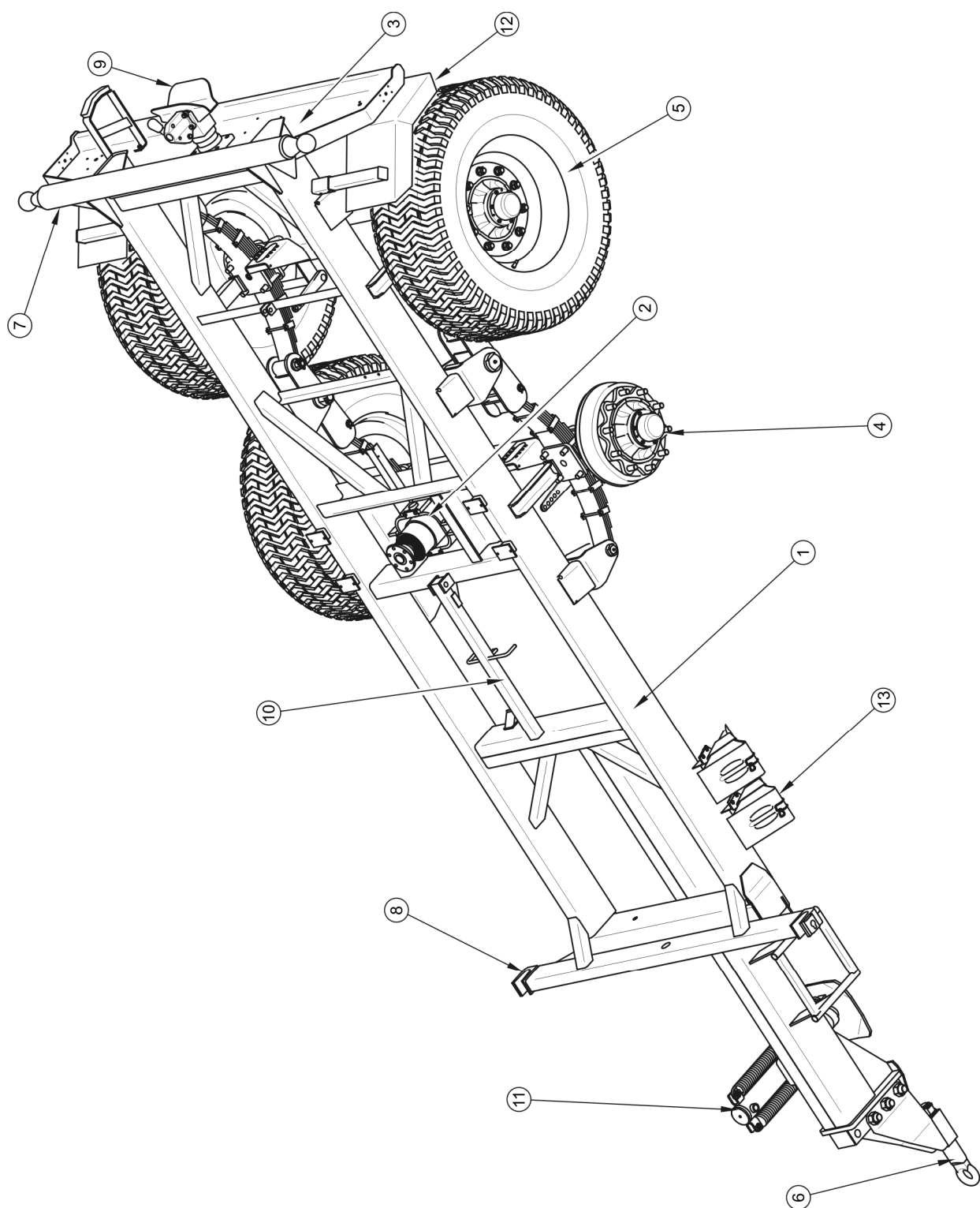
РИСУНОК 3.1 Шасси прицепа
