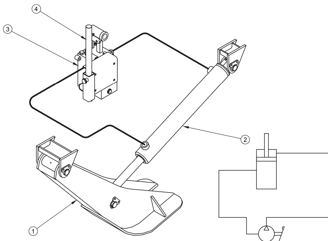
РИСУНОК 3.15 Устройство и схема гидравлической системы ножевой опоры с насосом
