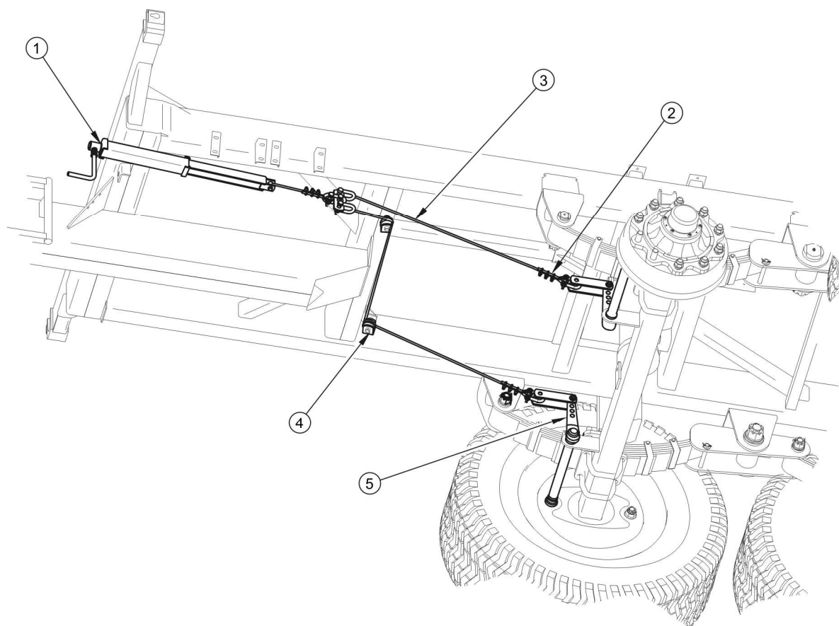
РИСУНОК 5.5 Регулирование натяжения тросов стояночного тормоза
