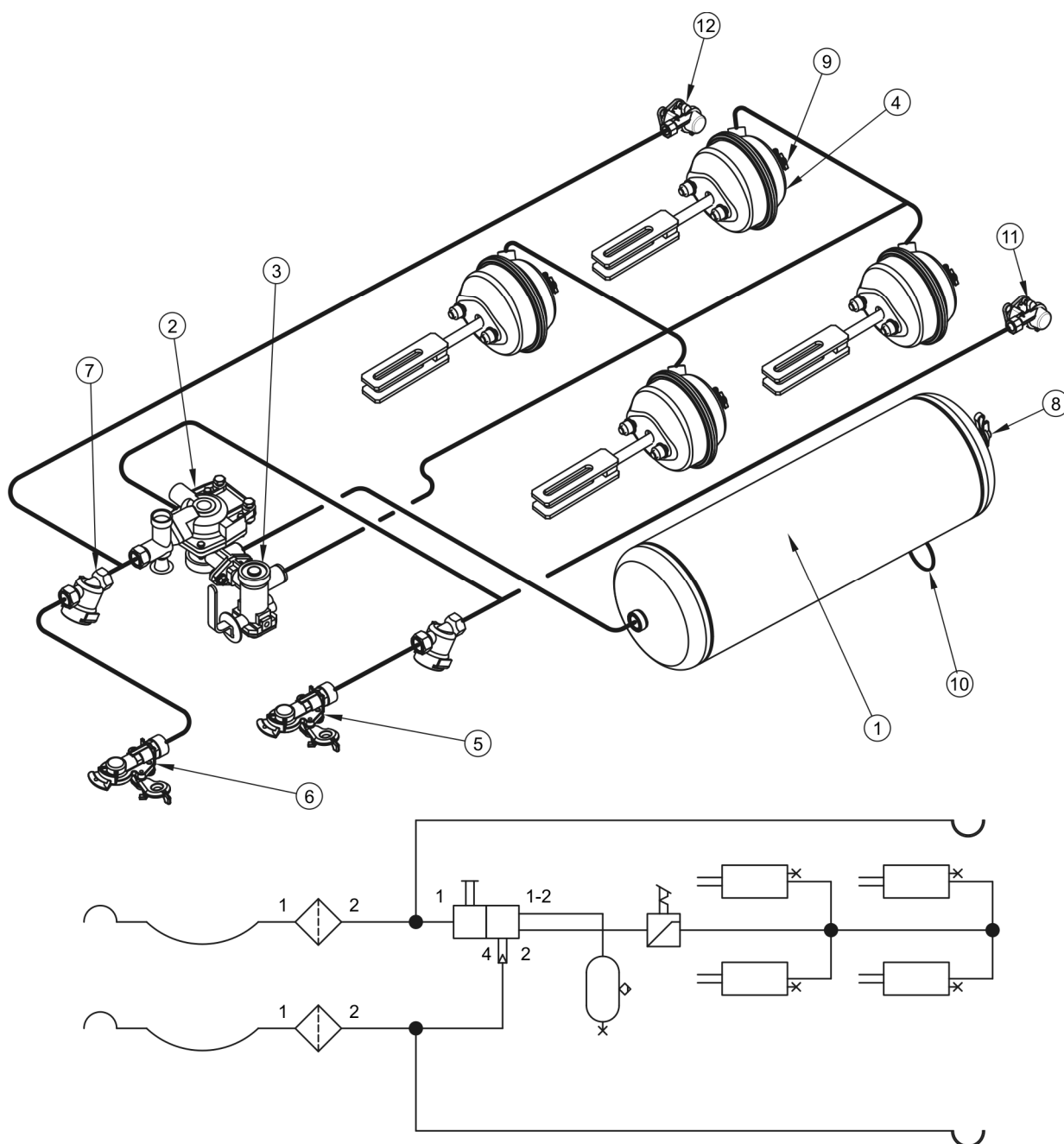
РИСУНОК 3.8 Устройство и схема двухпроводной пневматической тормозной системы с ручным регулятором силы торможения
