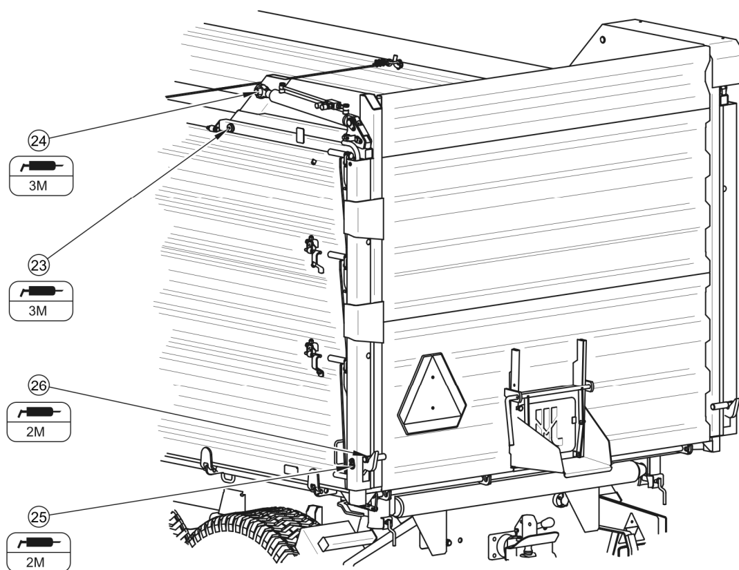
РИСУНОК 5.10 Точки смазки прицепа, часть 3
