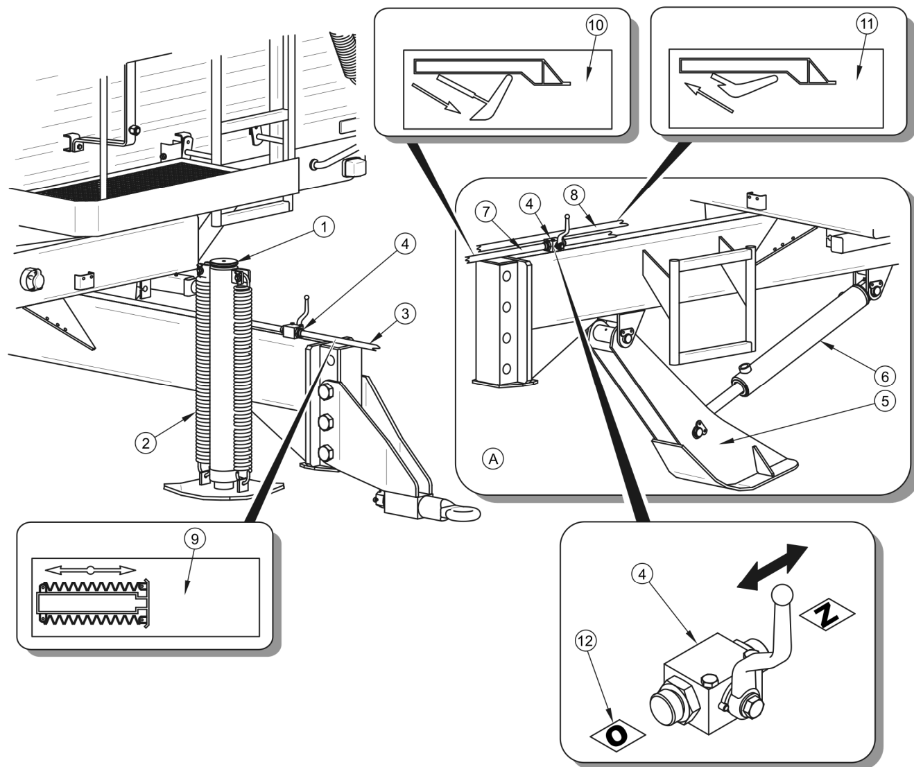
РИСУНОК 4.1 Опора прицепа
