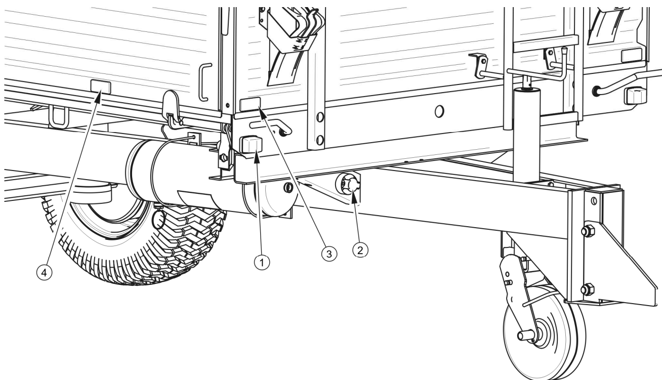
РИСУНОК 3.20 Размещение элементов системы световой сигнализации и катафотов прицепа – вид спереди
