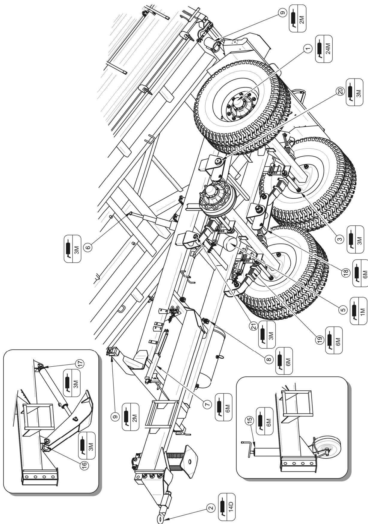
РИСУНОК 5.8 Точки смазки прицепа, часть 1
