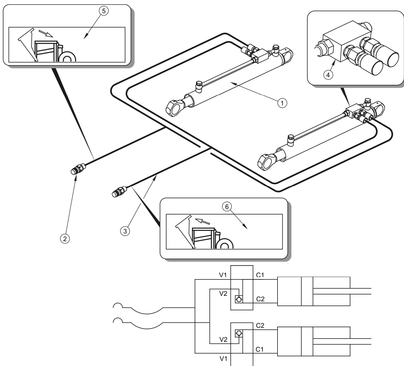
РИСУНОК 3.16 Устройство и схема гидравлической системы заднего борта
