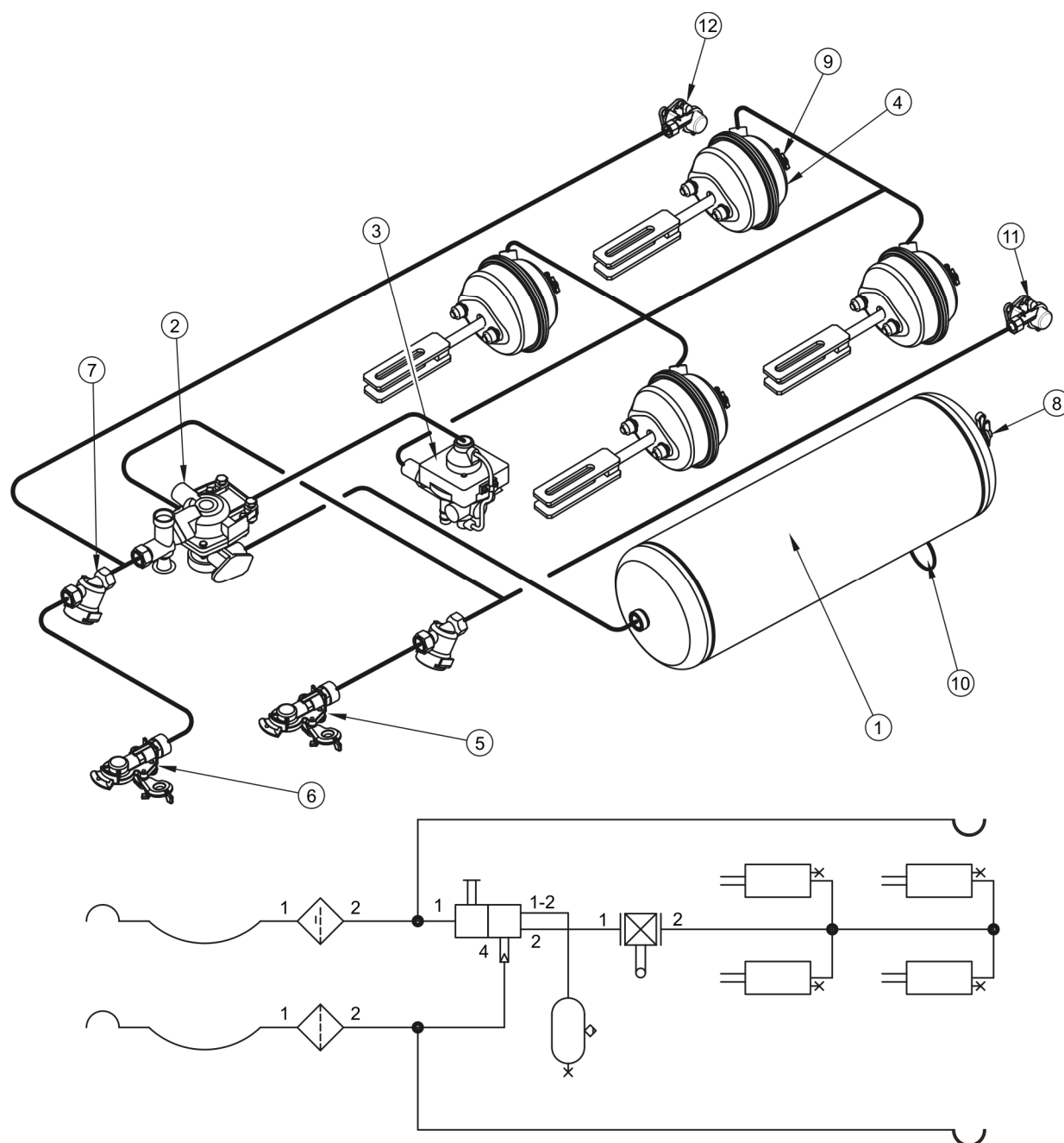
РИСУНОК 3.9 Устройство и схема двухпроводной пневматической тормозной системы с автоматическим регулятором силы торможения
