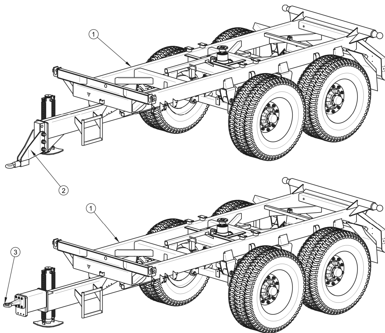
РИСУНОК 3.2 Версии нижней рамы
