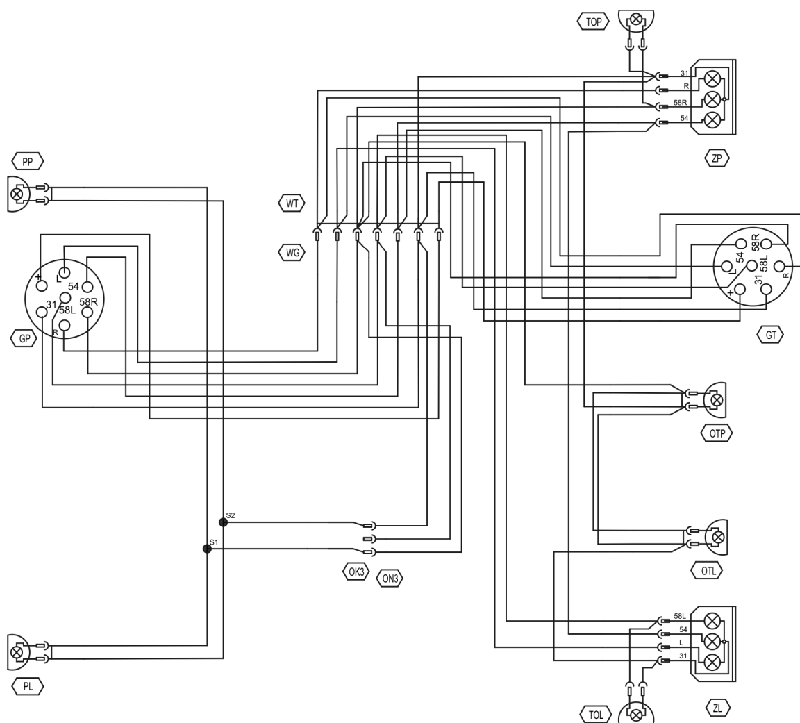
РИСУНОК 3.18 Принципиальная схема электрической системы
