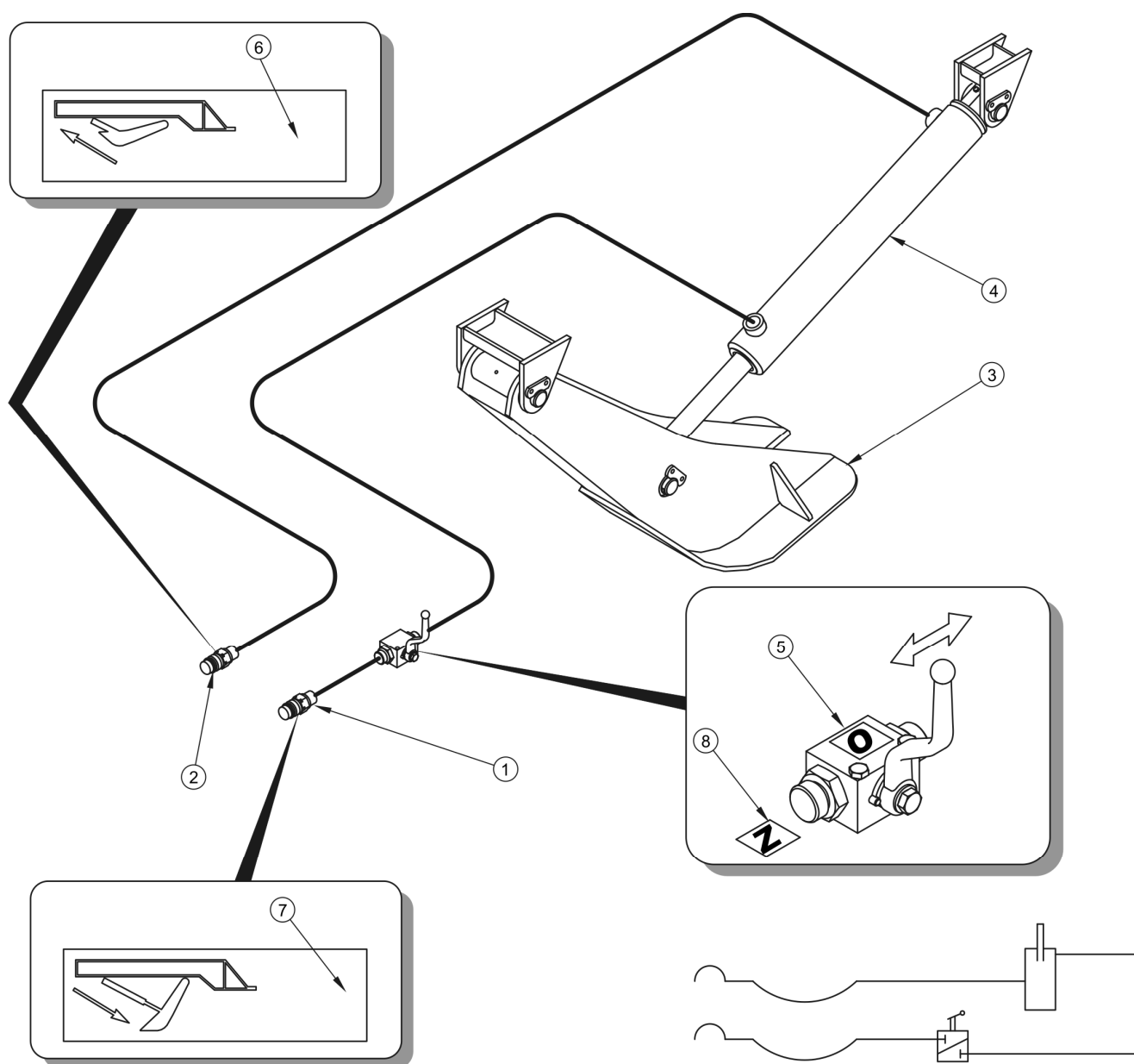
РИСУНОК 3.14 Устройство и схема гидравлической системы ножевой опоры
