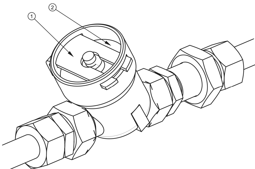
РИСУНОК 5.6 Воздушный фильтр
