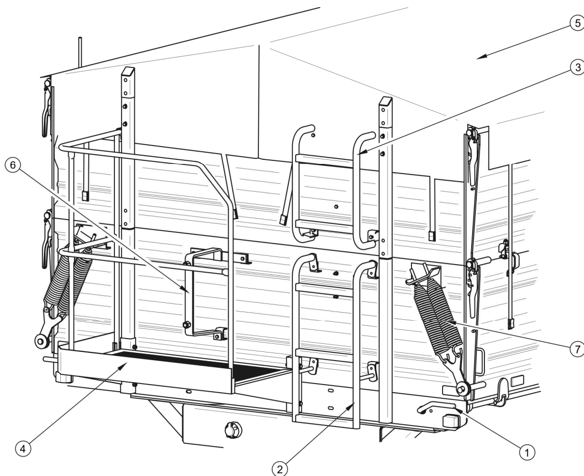
РИСУНОК 3.5 Платформа прицепа - вид спереди
