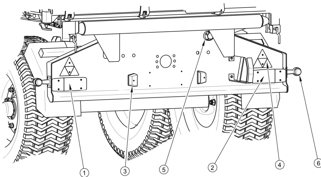
РИСУНОК 3.19 Размещение элементов системы световой сигнализации и катафотов прицепа – вид сзади
