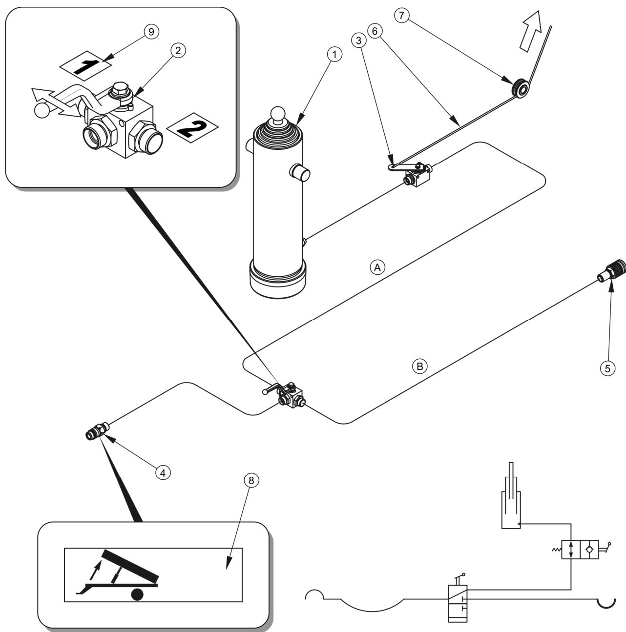
РИСУНОК 3.12 Устройство и схема гидравлической системы опрокидывания
