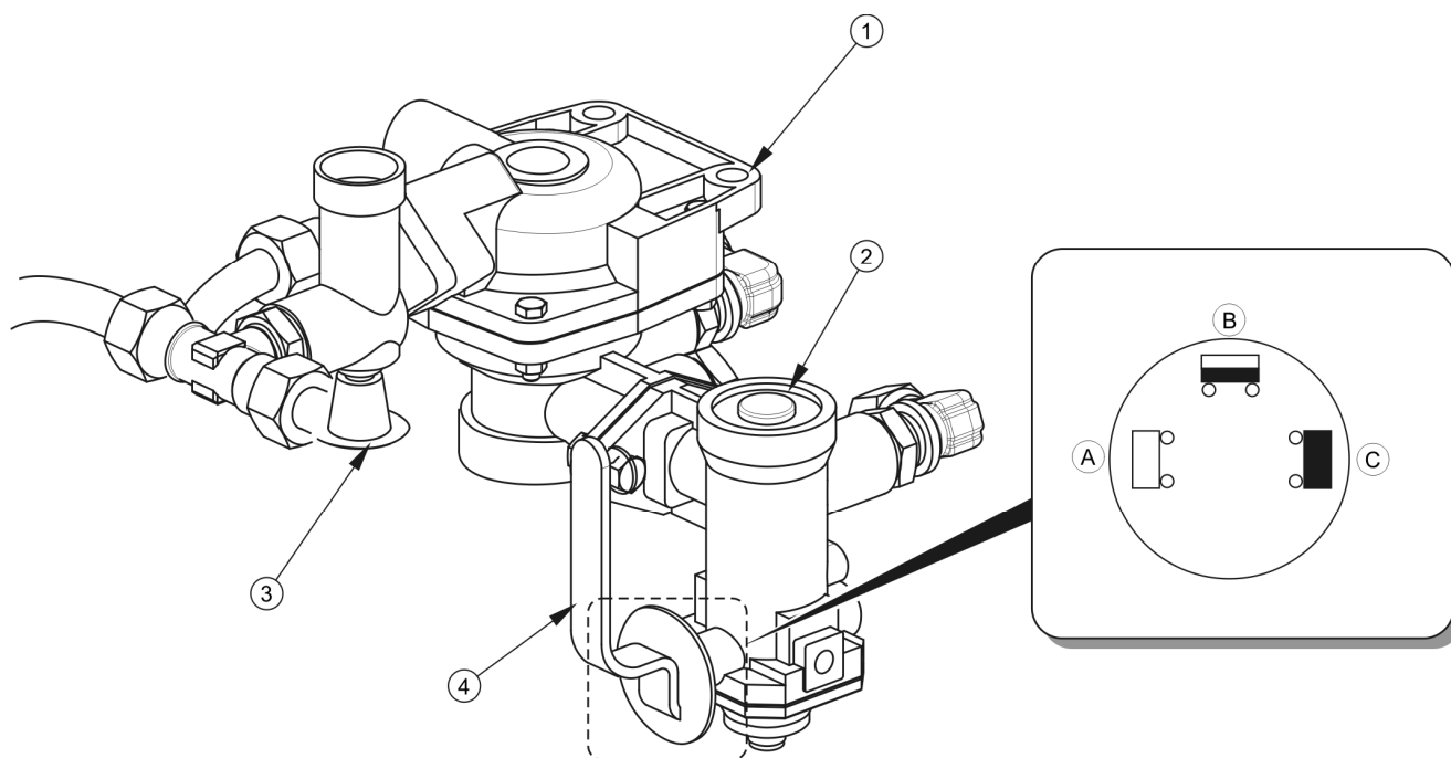
РИСУНОК 3.11 Управляющий клапан и регулятор силы торможения
