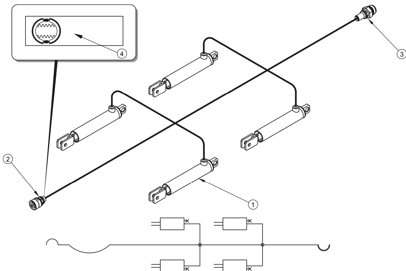
РИСУНОК 3.10 Устройство и схема гидравлической тормозной системы
