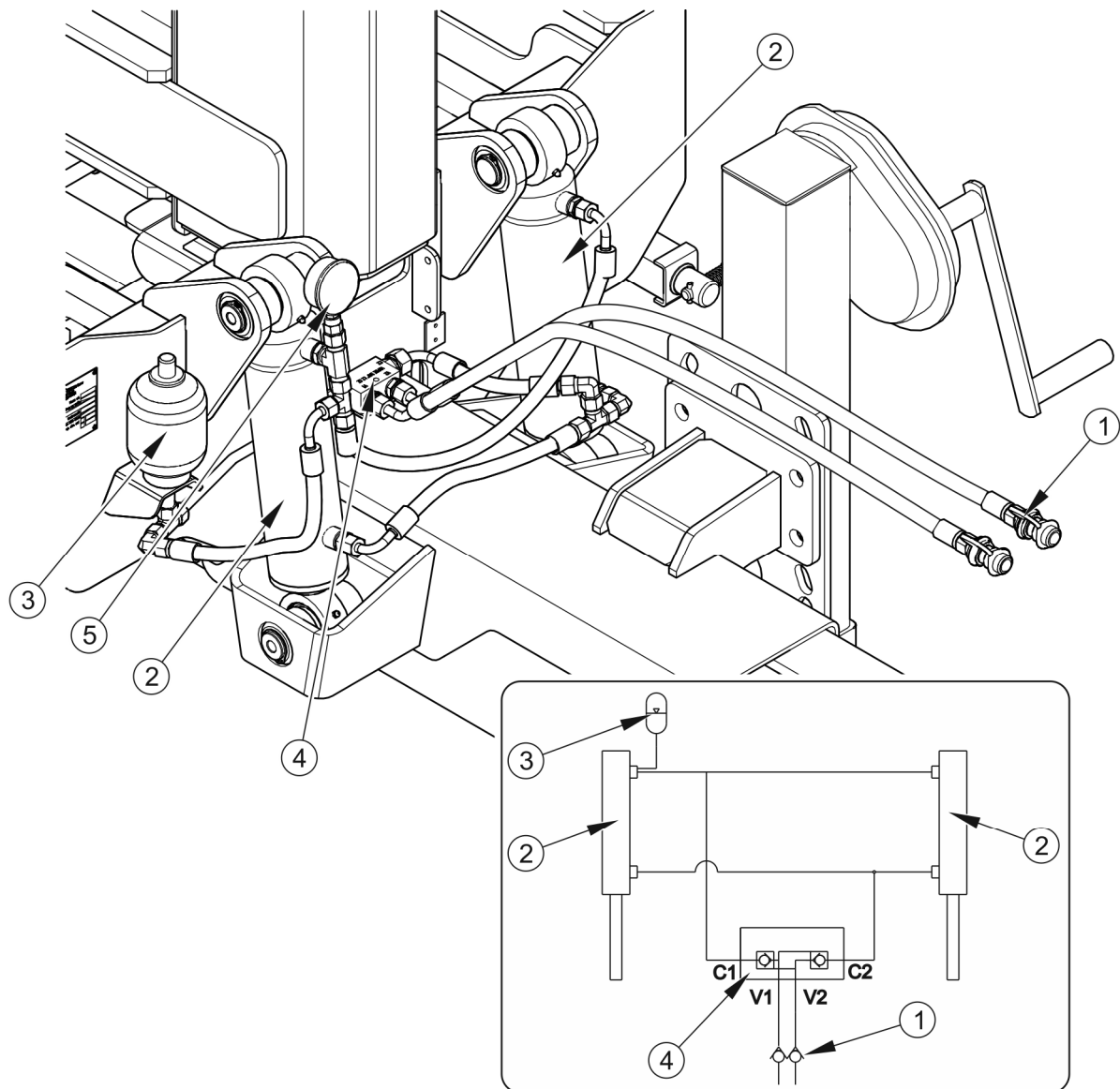
RYSUNEK 3.11 Budowa i schemat instalacji hydraulicznej dyszla
