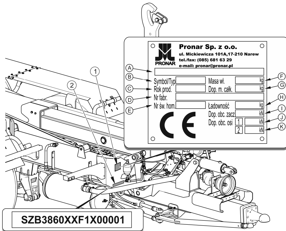
RYSUNEK 1.1 Miejsce umieszczenia tabliczki znamionowej i wybitcia numeru fabrycznego
