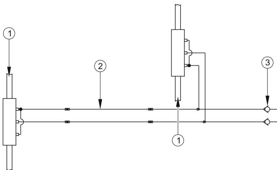
RYСУNEK 3.18 Schemat instalacji hydraulicznej blokady skrętu osi zewnętrznych
