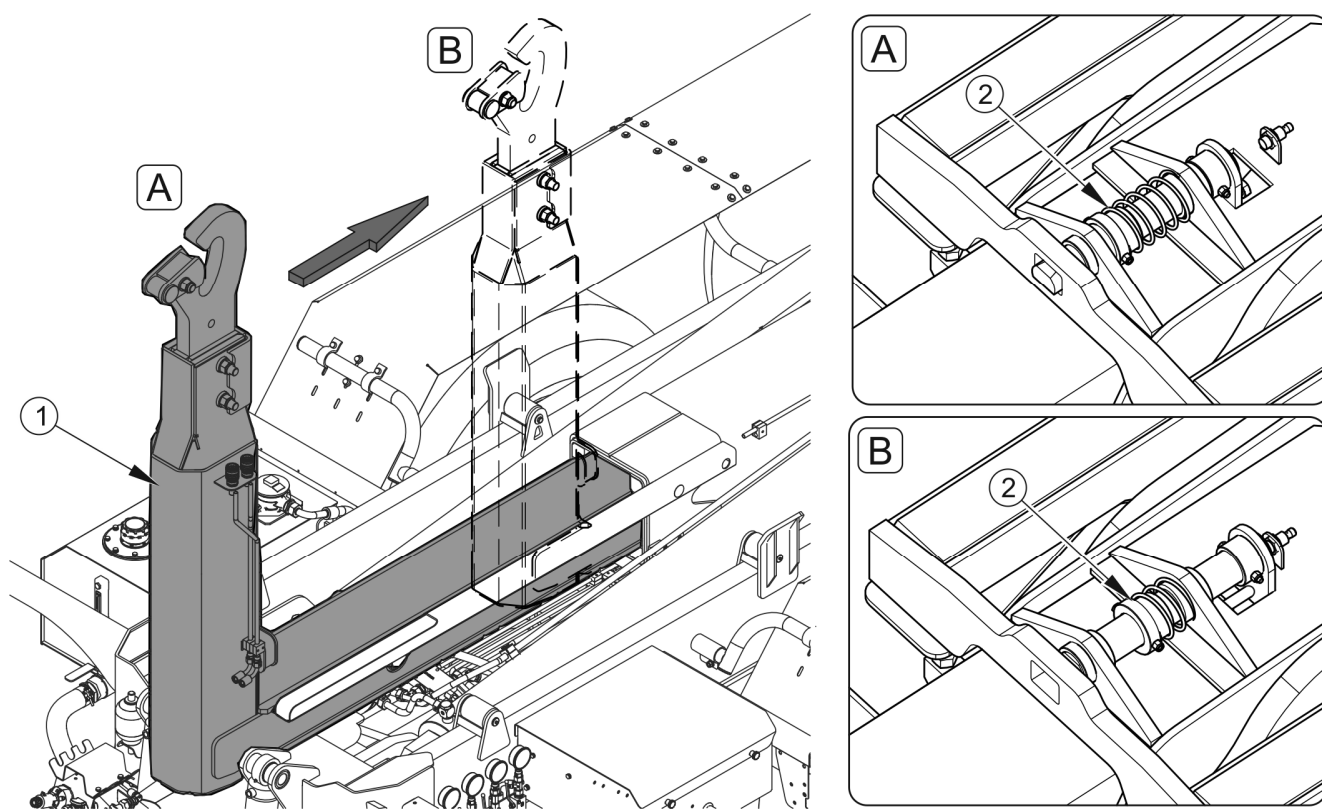
RYСУNEK 3.3 Przelączanie przyczepy do trybu „hakowiec”
