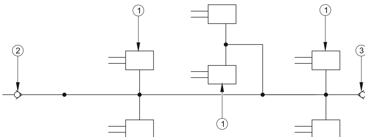
RYSUNEK 3.6 Schemat instalacji hamulcowej hydraulicznej
