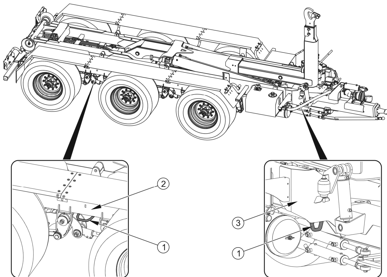
RYSUNEK 1.2 Rozmieszczenie uchwytów transportowych
