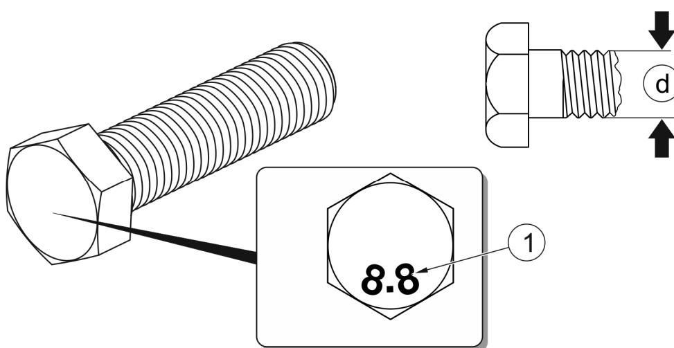
RYSUNEK 5.16 Śruba z gwintem metrycznym
