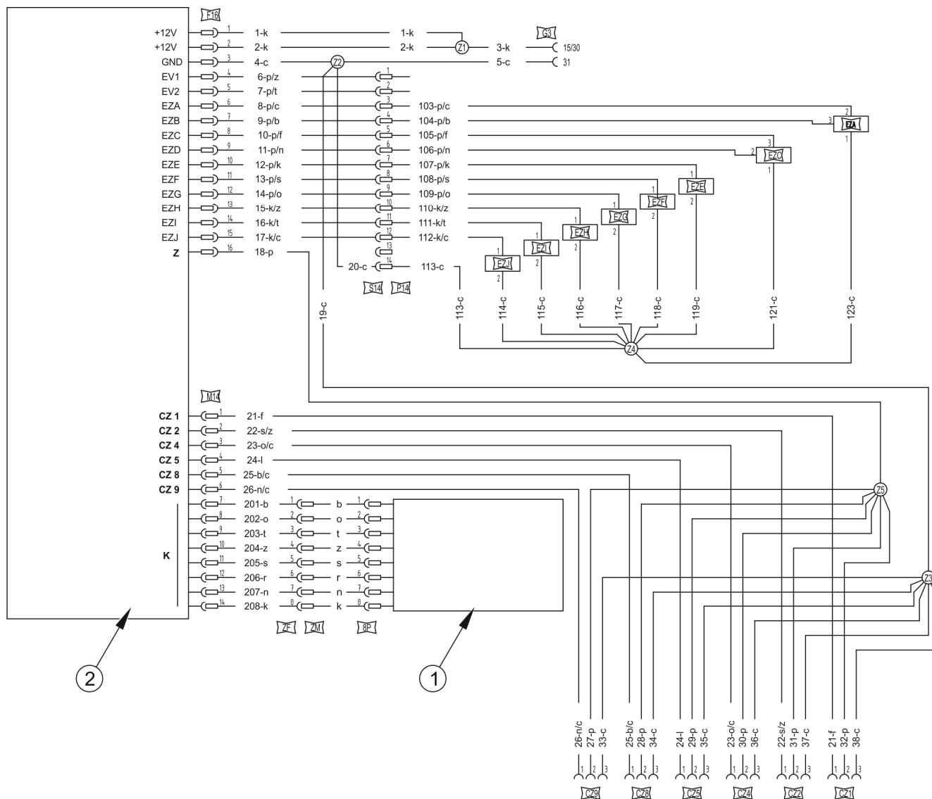
RYSUNEK 3.15 Schemat instalacji elektrycznej układu hydraulicznego
