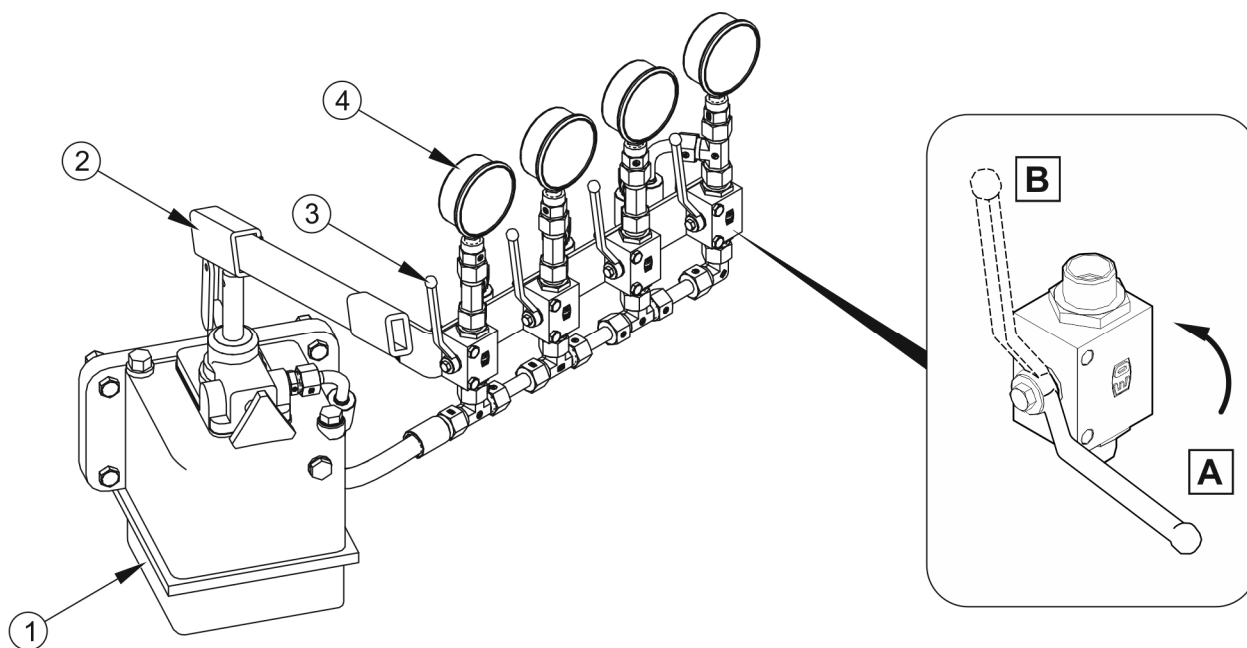
RYSUNEK 4.6 Hydrauliczna pompka ręczna
