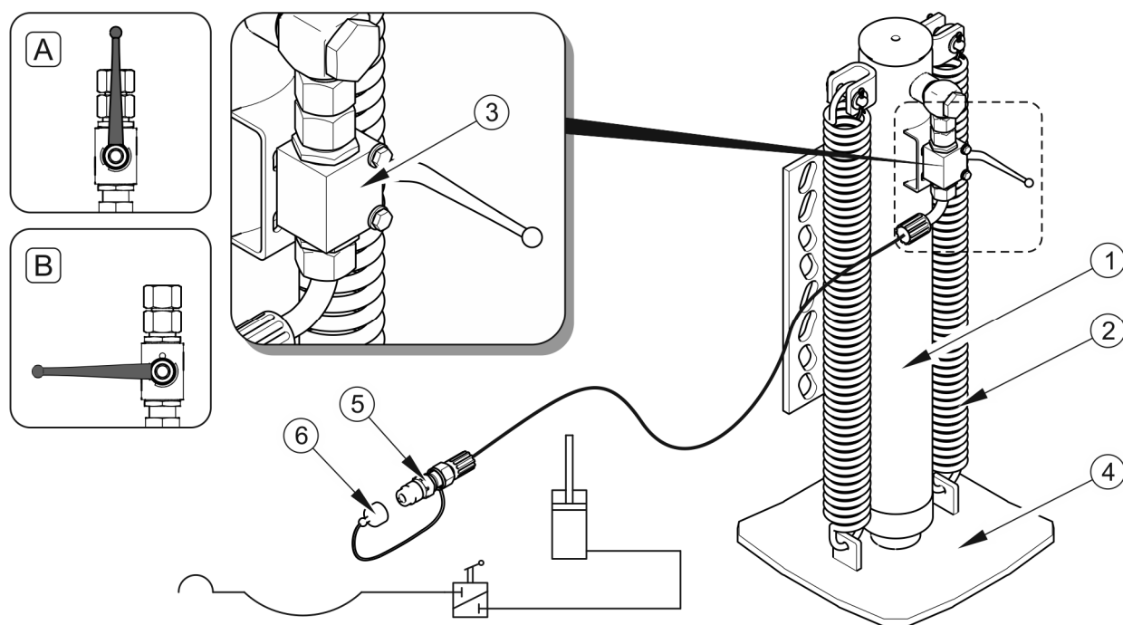
RYSUNEK 3.9 Budowa i schemat instalacji hydraulicznej podpory prostej
