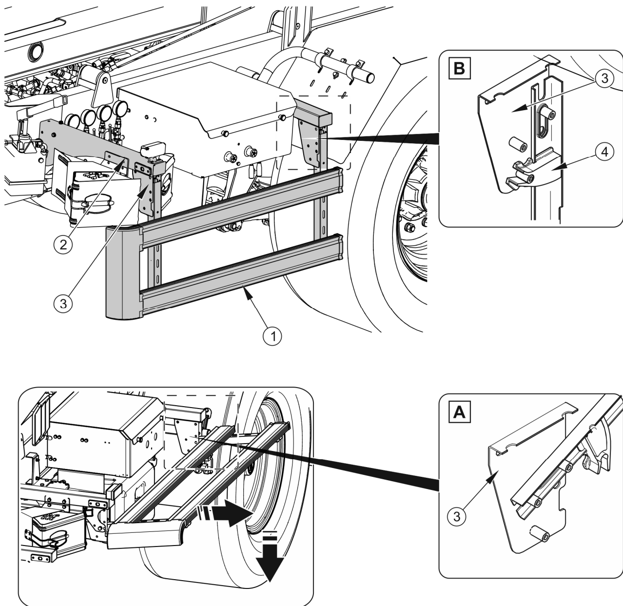
RYSUNEK 4.9 Ośłona przeciwnajazdowa lewa
