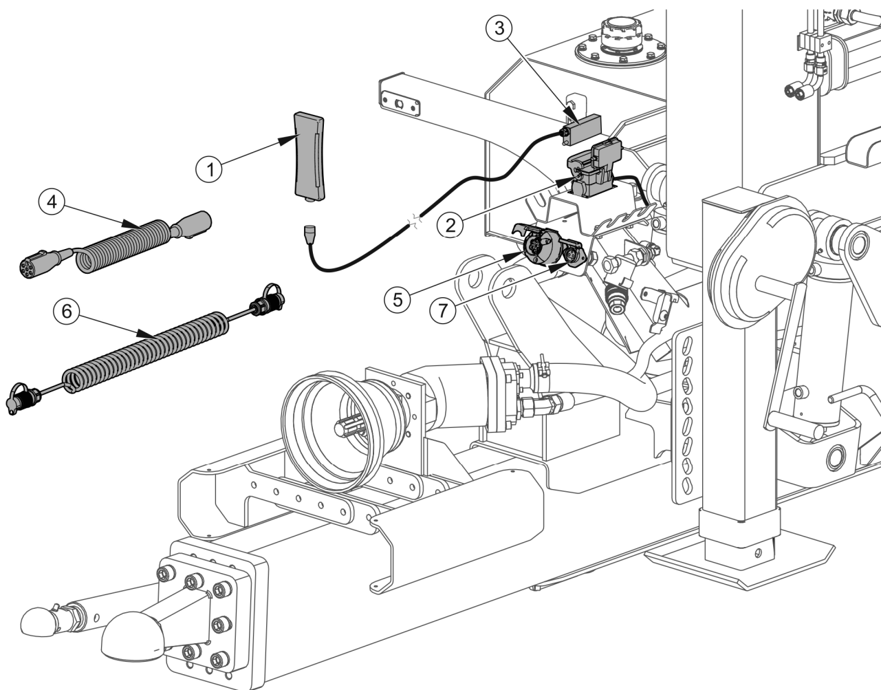
RYSUNEK 4.3 Podłączenie instalacji elektrycznej
