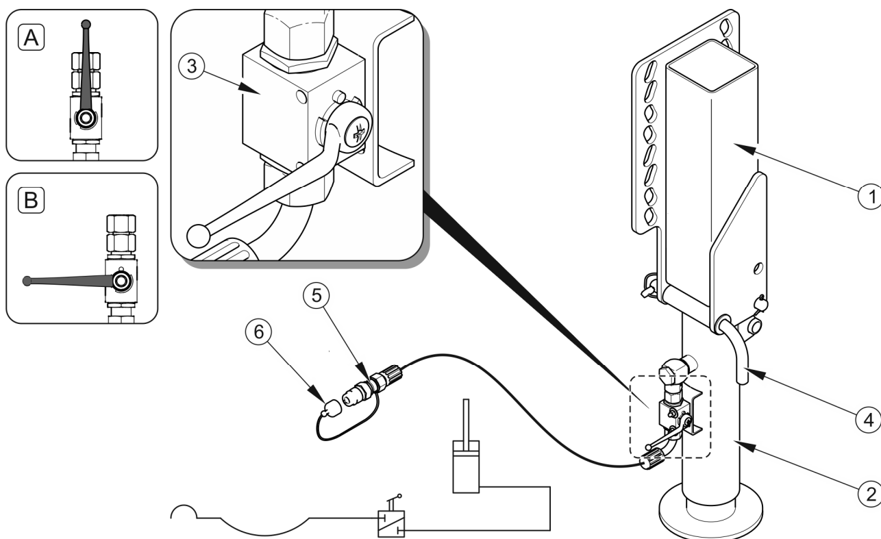
RYСУNEK 3.10 Budowa i schemat instalacji hydraulicznej podпоры łamanej
