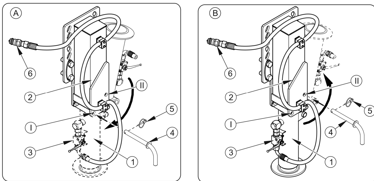
RYSUNEK 4.5 Obsługa podpory hydraulicznej łamanej
