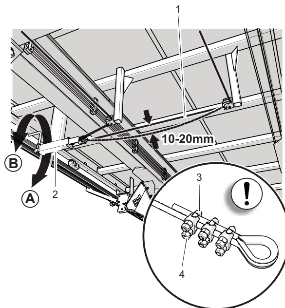
Abbildung 5.13 Kontrolle der Bremsseilspannung
