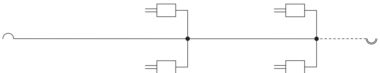
Abbildung 3.6 Schema der hydraulischen Bremsanlage
