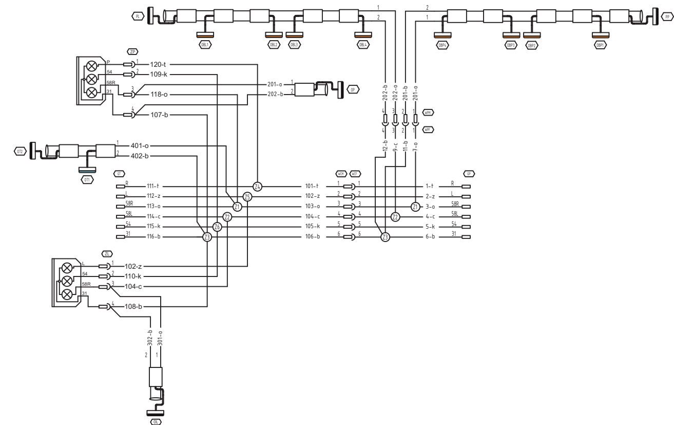
Abbildung 3.12 Schaltplan der elektrischen Installation
