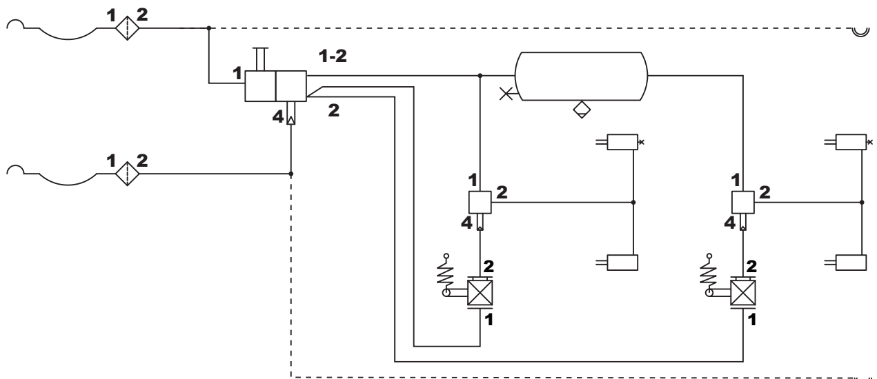
Abbildung 3.5 Schema der Zweikreis-Bremsanlage mit automatischem Bremskraftregler
