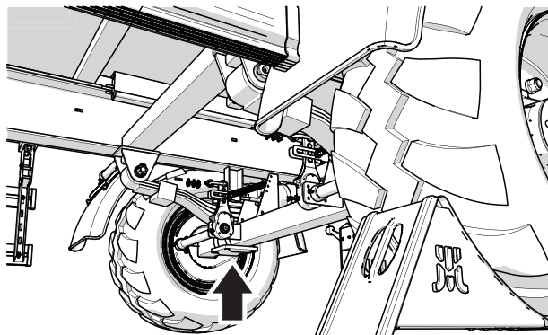
Abbildung 5.1 Empfohlene Ansetzpunkte für den Fahrzeugheber
