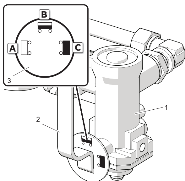
Abbildung 3.8 Dreistufiger Bremskraftregler
