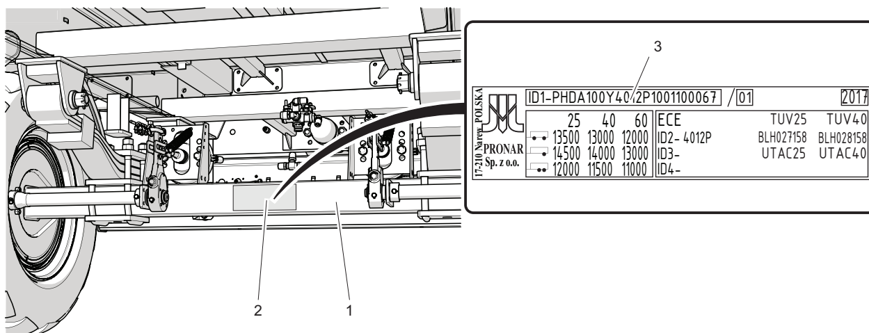
Abbildung 1.2 Identifikation der Fahrachsen
