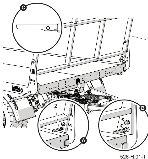
Abbildung 4.1 Einstellen der Leitern
