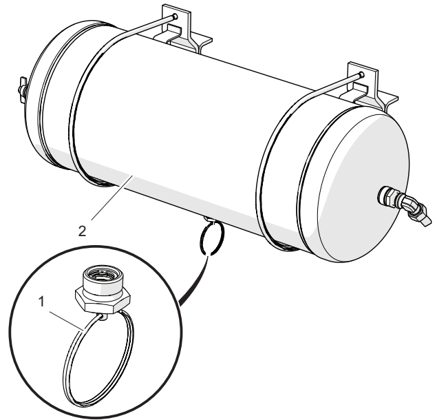
Abbildung 5.12 Druckluftbehälter (1) Entwässerungsventil (2) Behälter,
