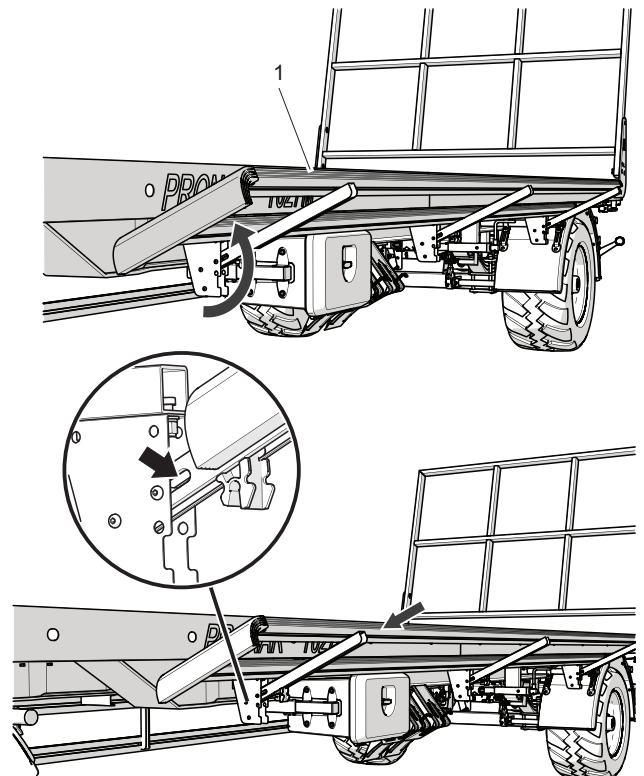
Abbildung 4.2 Linker Auffahrschutz
