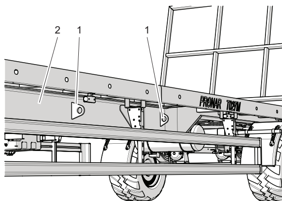
Abbildung 1.3 Befestigungsstellen des Anhängers (1) Transporthalterung, (2) Rahmen
