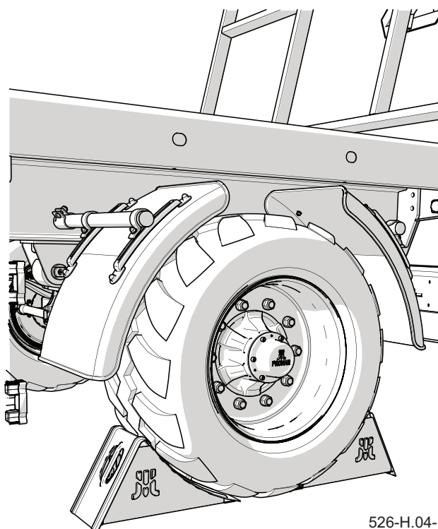
Abbildung 4.4 Radkeile
