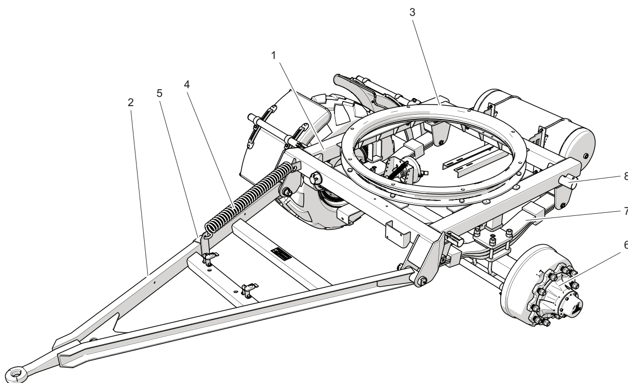
Abbildung 3.3 Aufbau des Anhängers
