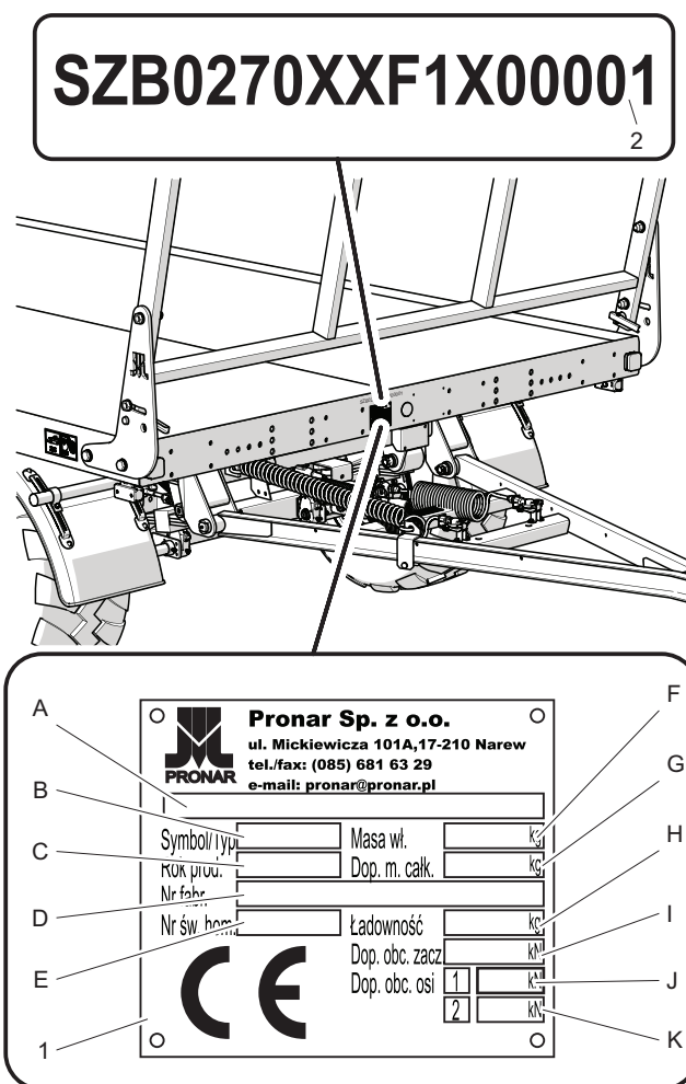
Abbildung 1.1 Lokalisierung des Typenschildes
