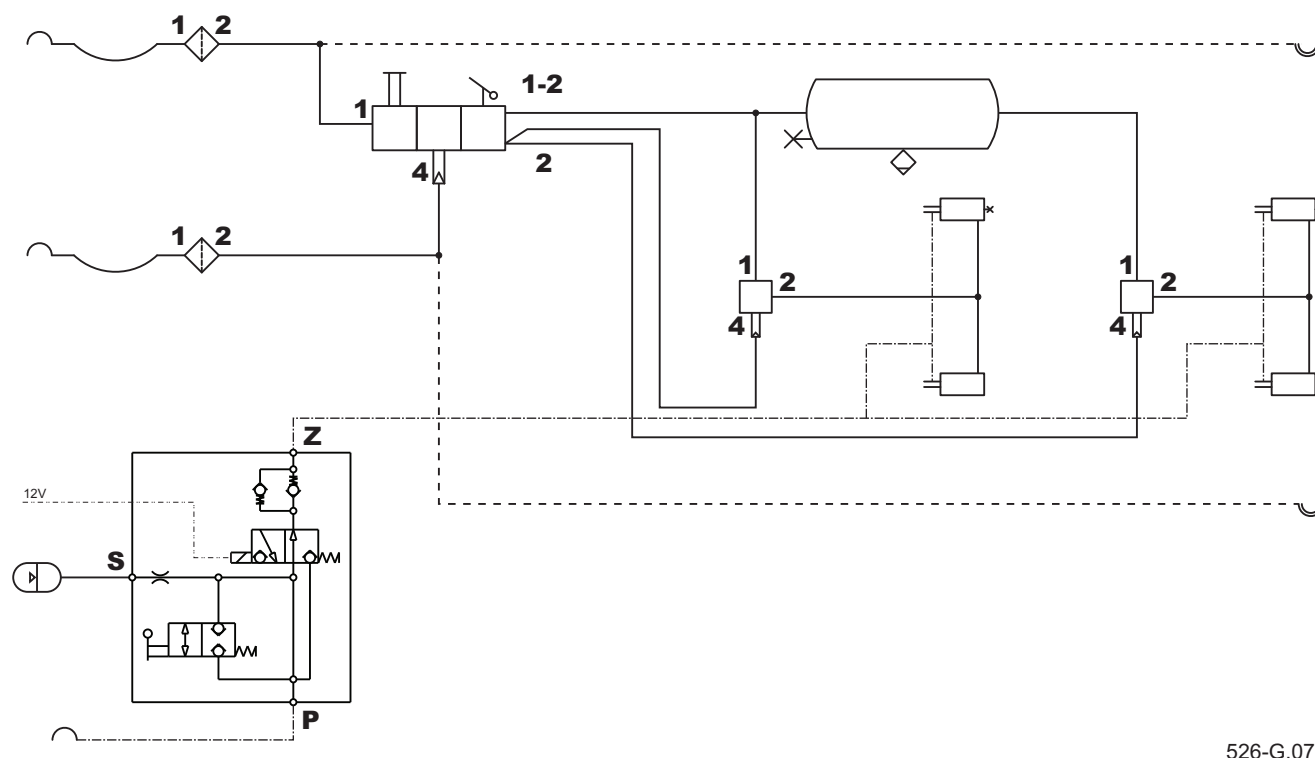
Abbildung 3.7 Schaltbild der kombinierten Bremsanlage mit elektronischer Sicherung
