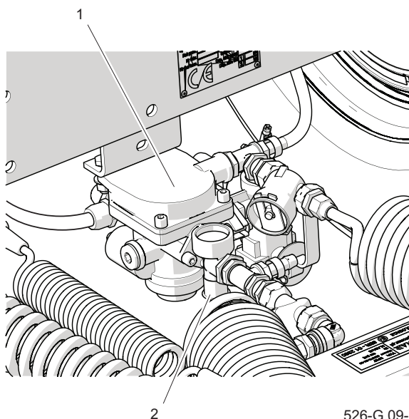
Abbildung 3.9 Steuerventil
