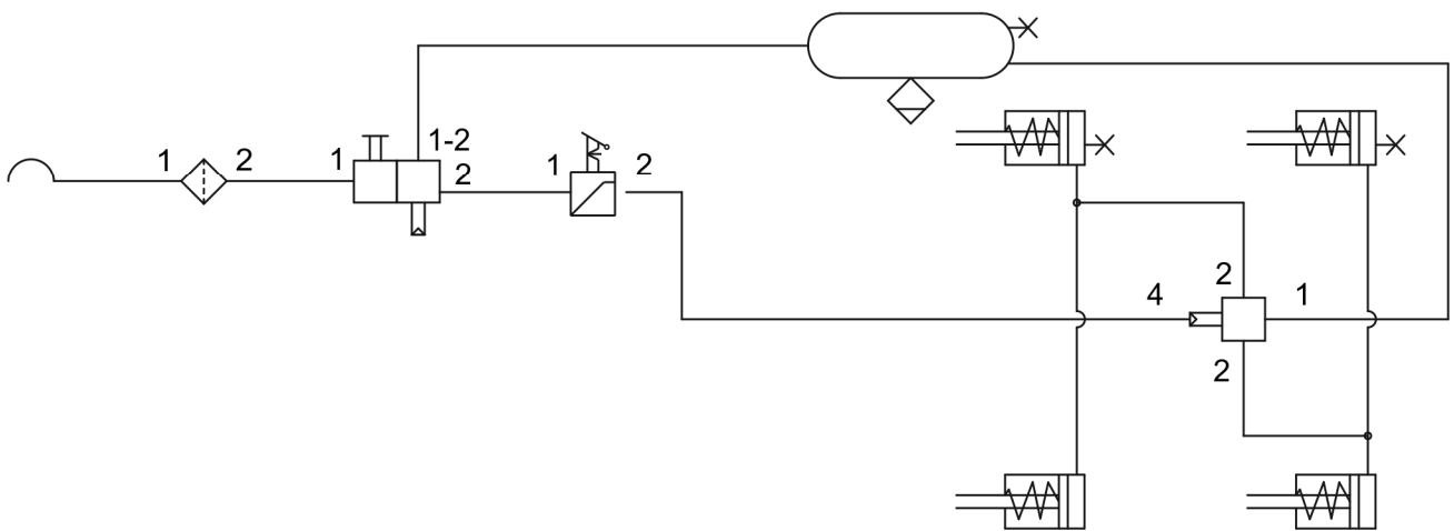
RYSUNEK 3.7 Budowa i schemat instalacji hamulcowej pneumatycznej jedнопrzewodowej z regulatorem ręcznym
