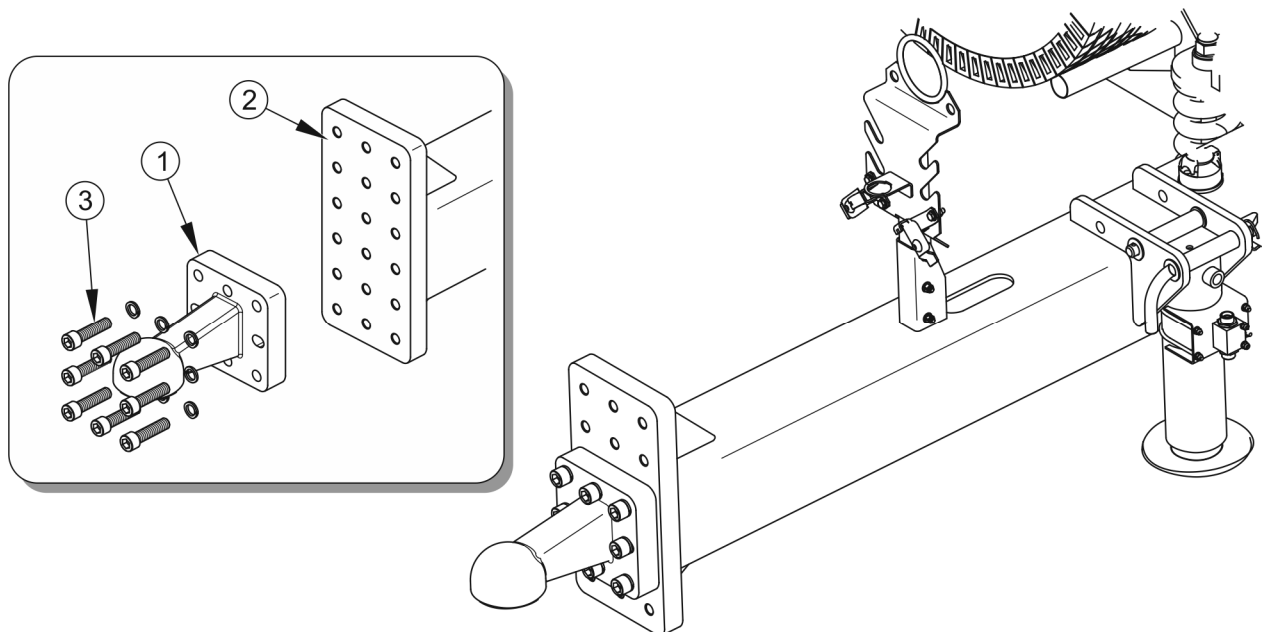
RYСУNEK 5.12 Regulacja położenia dyszla
