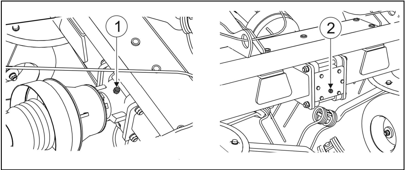
BILD 5.1A Getriebeölwechsel
