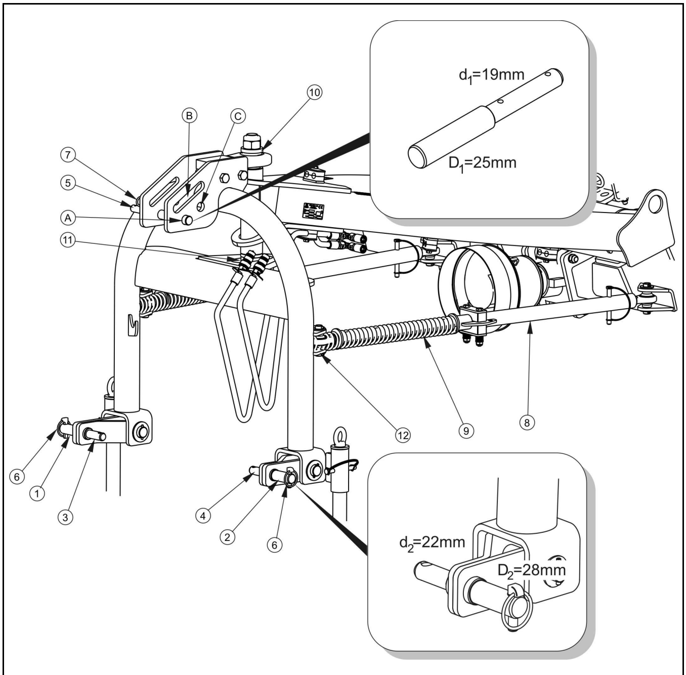
BILD 3.2A Aufhängung
