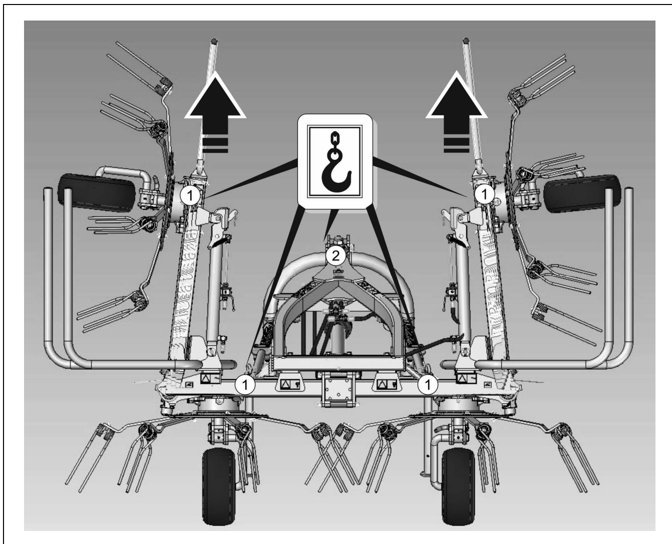
BILD 1.2A Stellen zum Aufhängen des Schwaders
