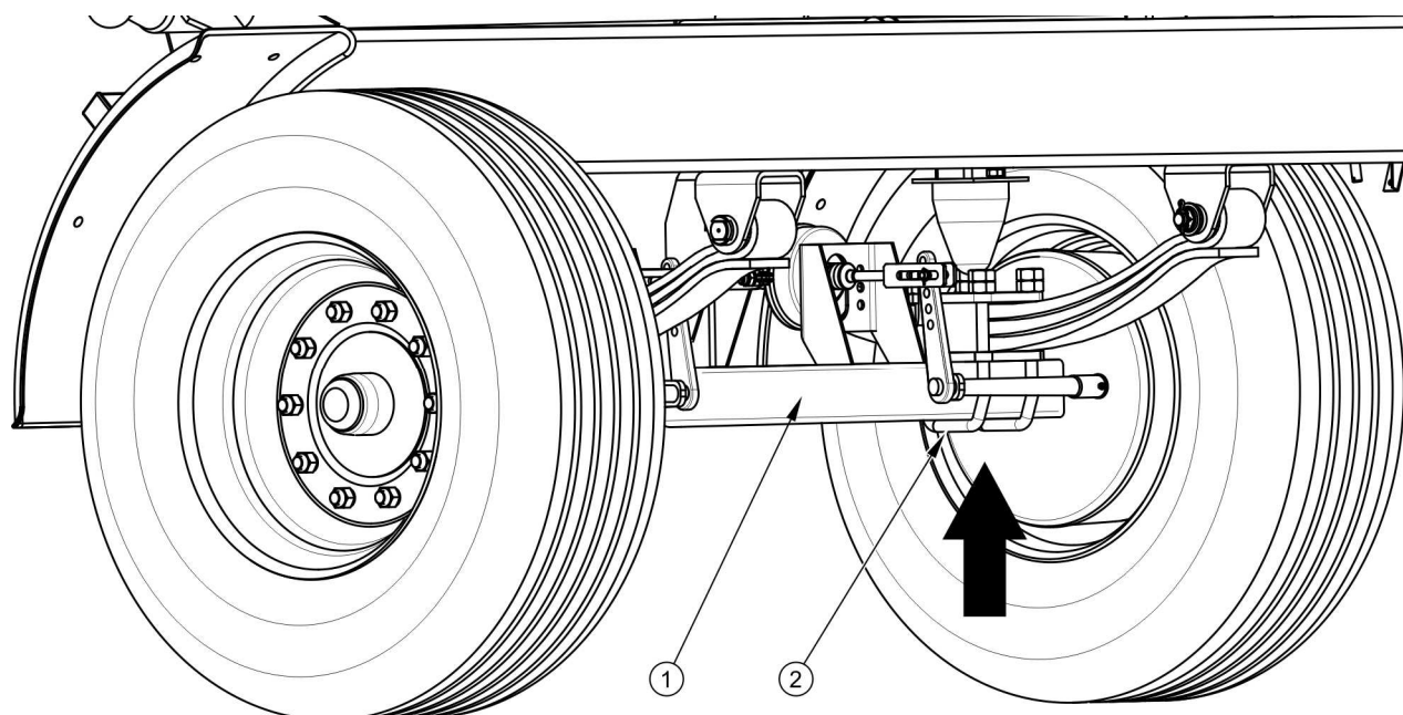
РИСУНОК 5.2 Точка поддомкрачивания
