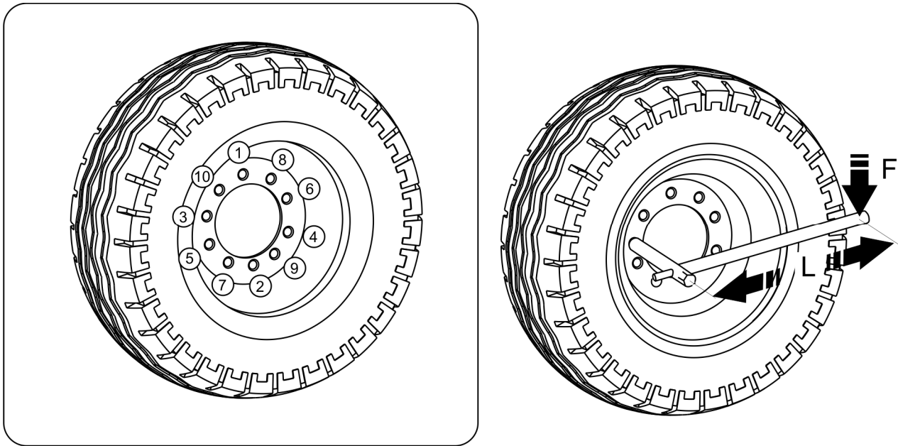
РИСУНОК 5.4 очередность затяжки гаек
