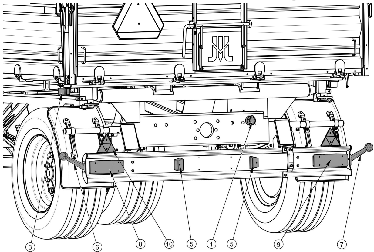
РИСУНОК 3.10 Размещение элементов электрической системы и светоотражающей сигнализации
