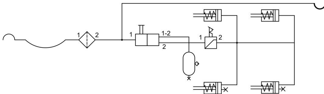
РИСУНОК 3.6 Устройство и схема однопроводной пневматической тормозной системы
