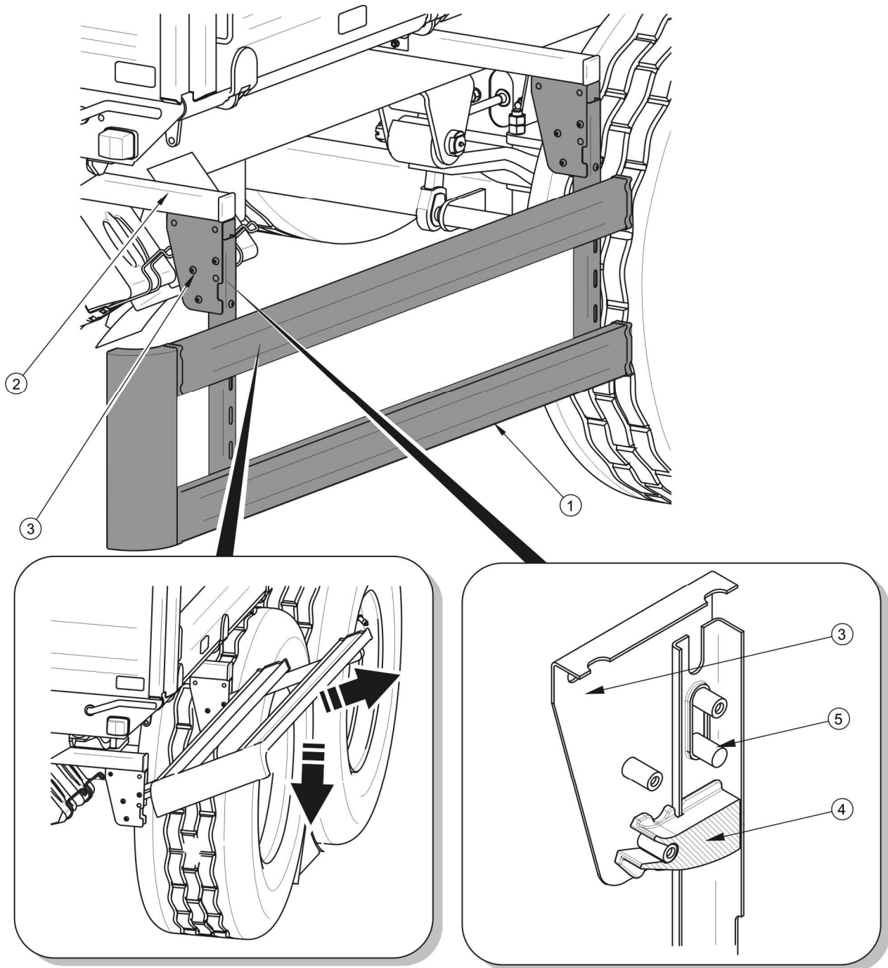
RYСУNEK 4.7 Osłona przeciwnajazdowa lewa
