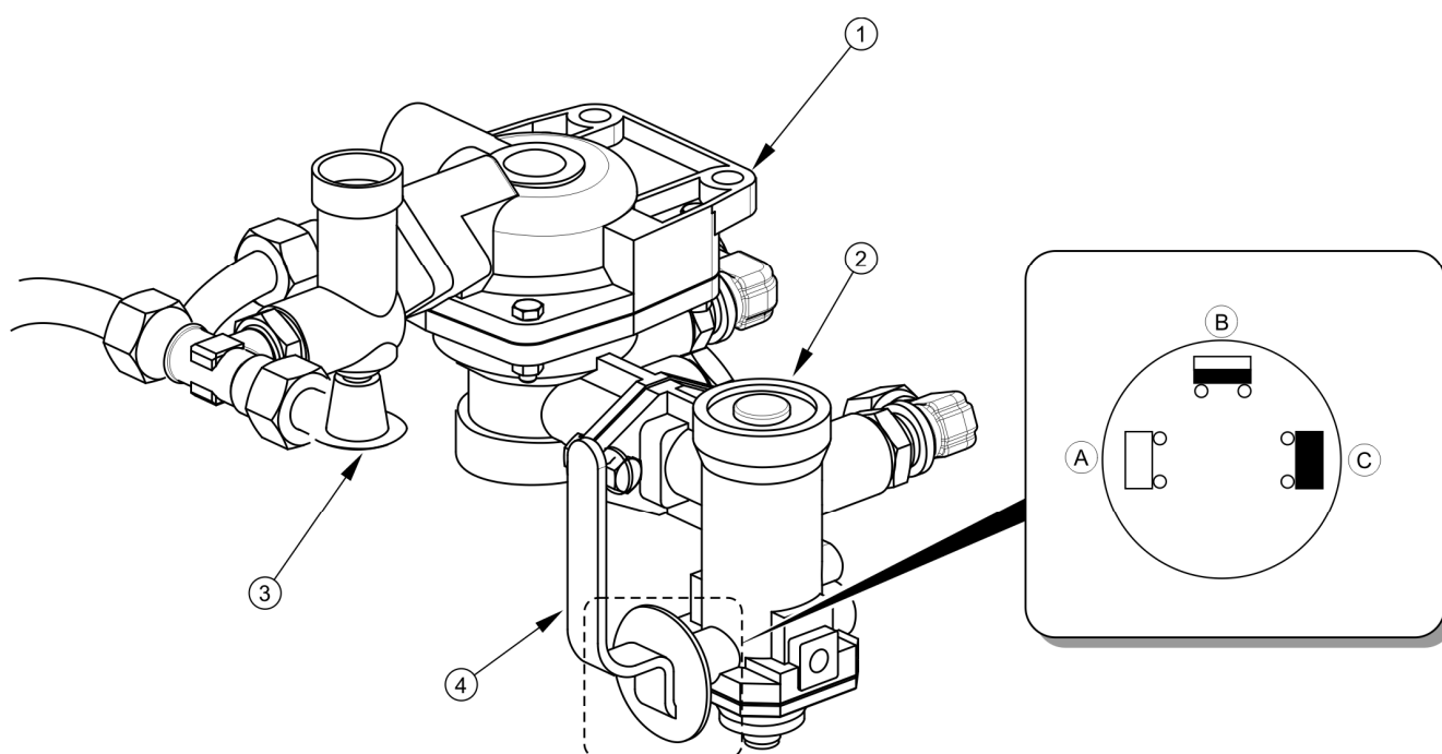
RYSUNEK 3.7 Zawór sterujący i regulator siły hamowania
