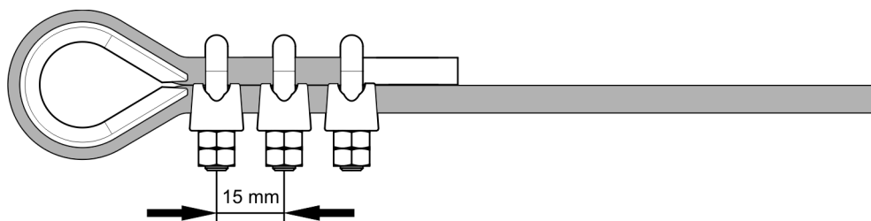
RYСУNEK 5.6 Montaż zacisków linki hamulcowej
