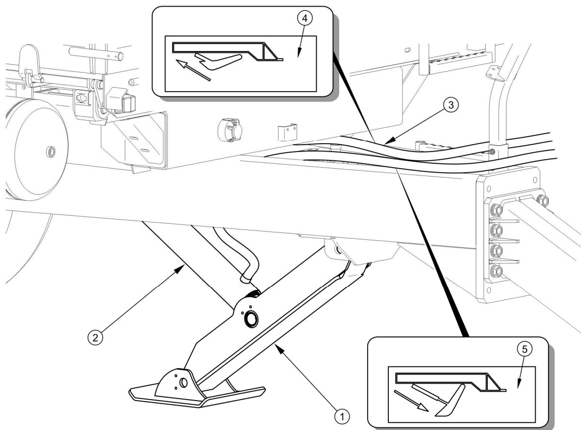
RYСУNEK 4.1 Podpora przyczepy
