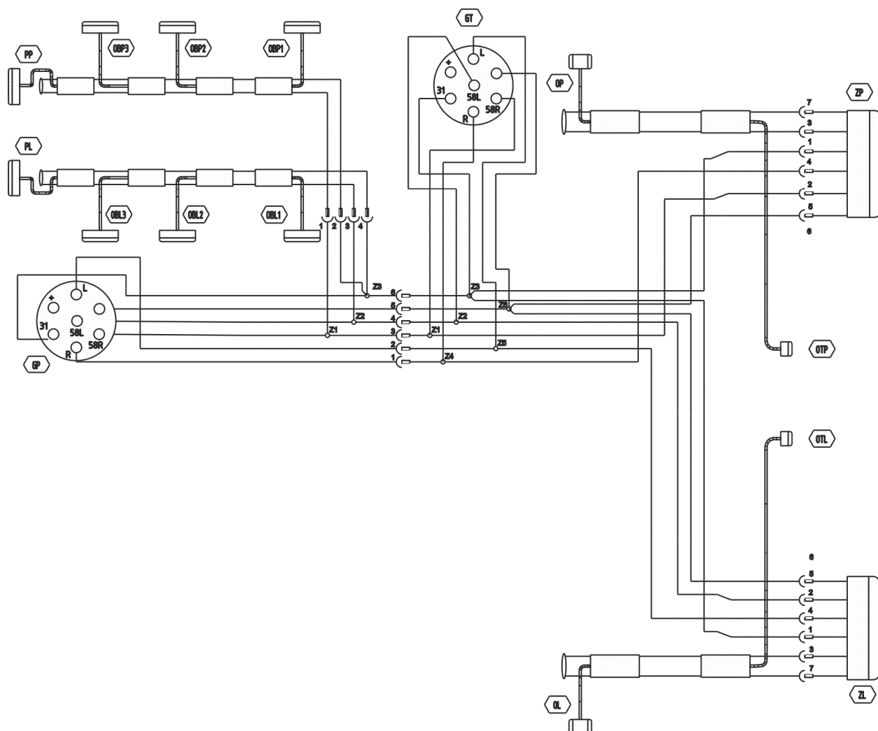
RYСУNEK 3.13 Schemat ideowy instalacji elektrycznej
