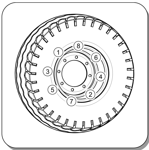
RYСУNEK 5.3 Kolejność dokręcania nakrętek
