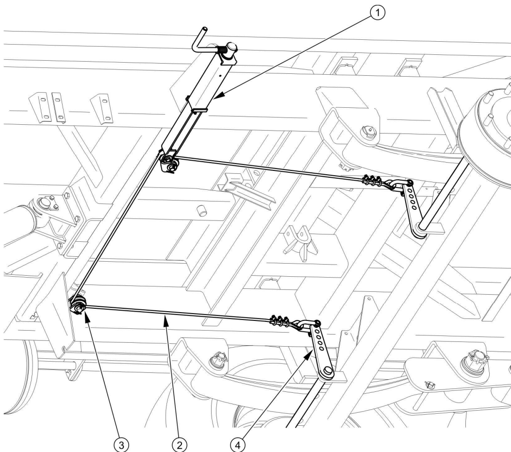
RYSUNEK 3.12 Budowa hamulca postojowego
