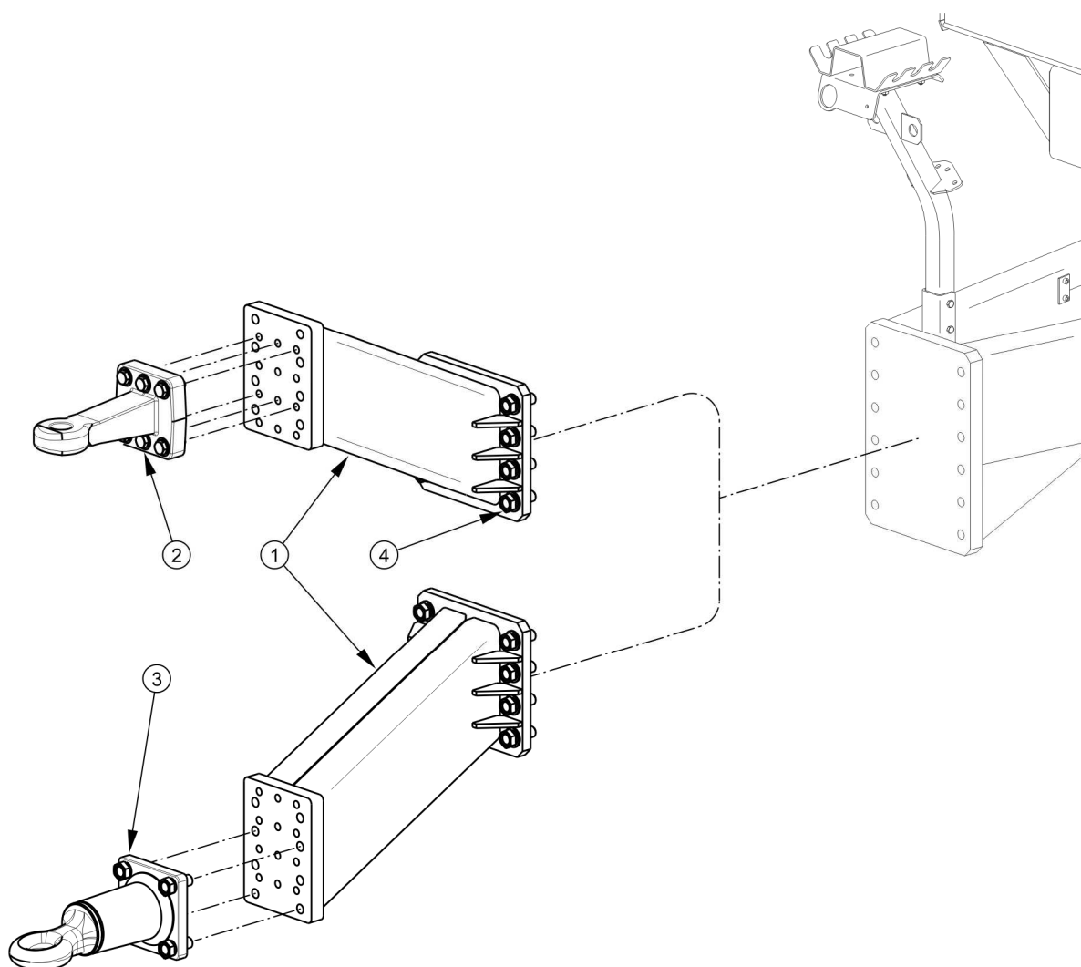
RYСУNEK 5.15 Regulacja położenia dyszla
