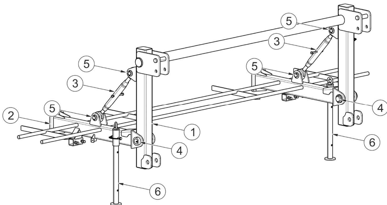
РИСУНОК 3.2 Несущая система
