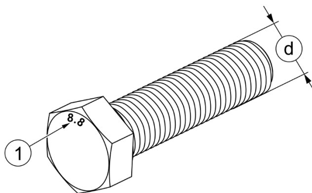
РИСУНОК 5.6 Болт с метрической резьбой
