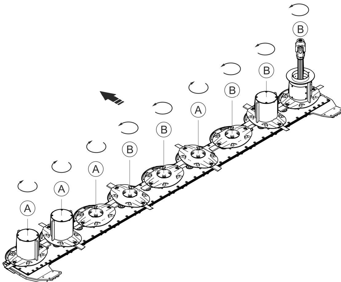
РИСУНОК 5.2 Типы срезающих ножей
