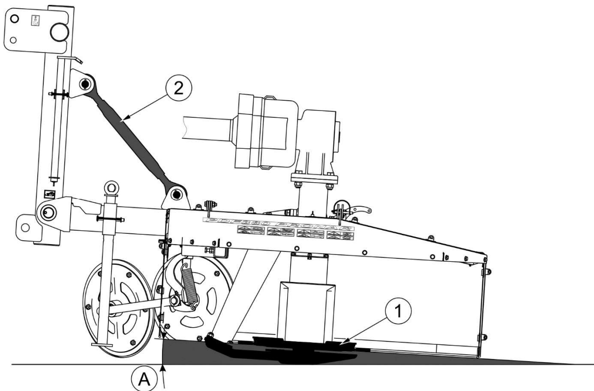
РИСУНОК 4.7 Регулировка высоты кошения
