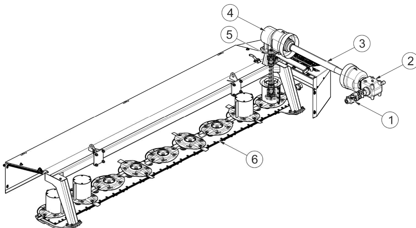
РИСУНОК 3.3 Система передачи привода
