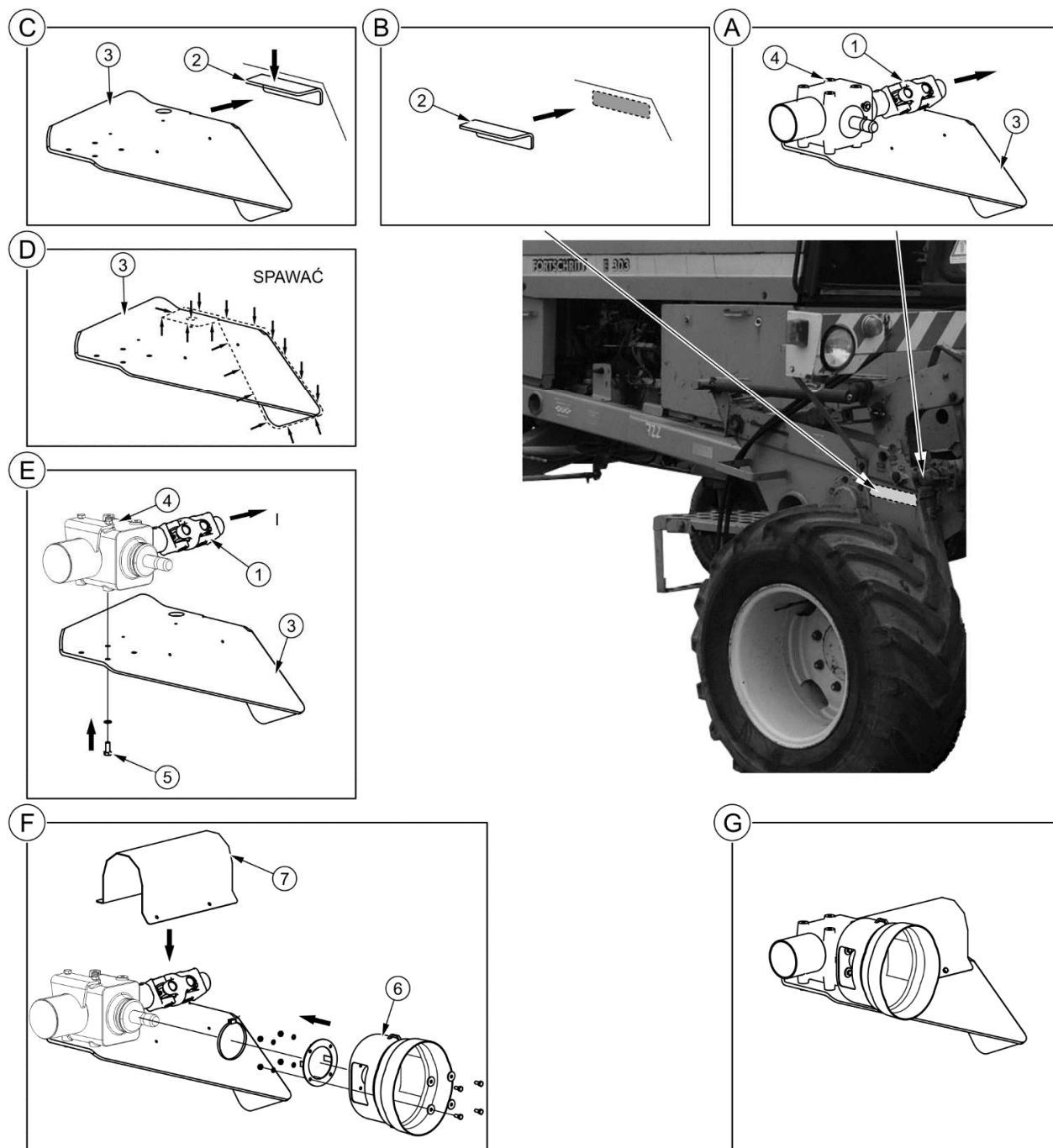
РИСУНОК 4.1 Монтаж основания угловой передачи на самоходной машине FORTSCHRITT
