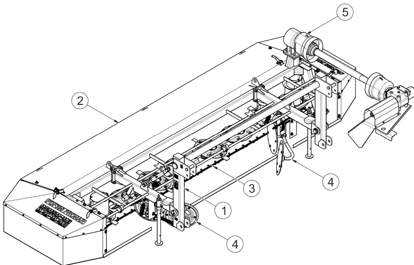
РИСУНОК 3.1 Общее устройство
