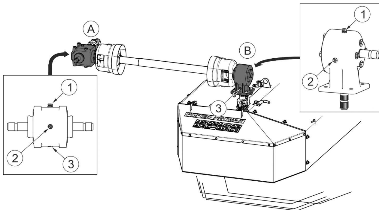
РИСУНОК 5.4 Проверка и замена масла в угловых передачах
