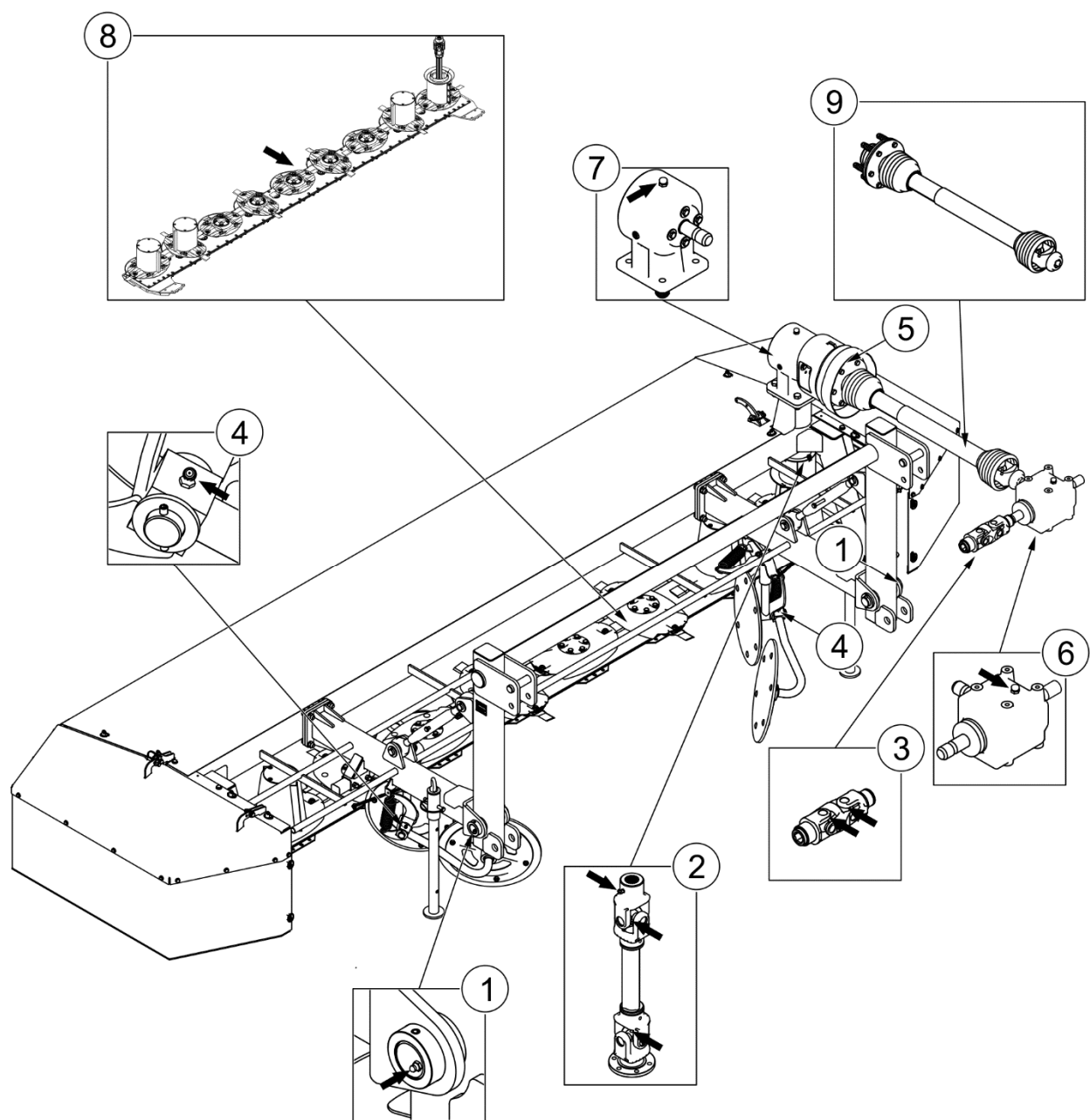
РИСУНОК 5.5 Точки смазки
