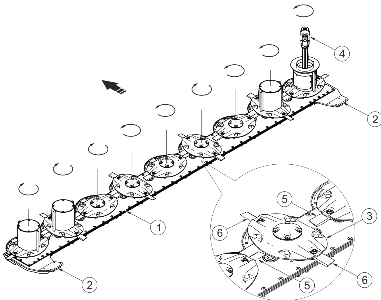
РИСУНОК 3.4 Режущий узел
