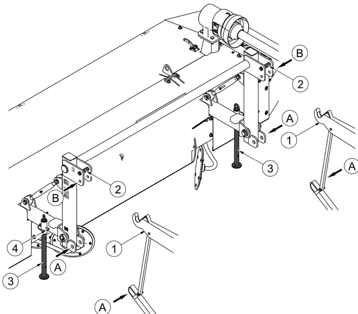
РИСУНОК 4.2 Подсоединение к самоходной машине FORTSCHRITT
