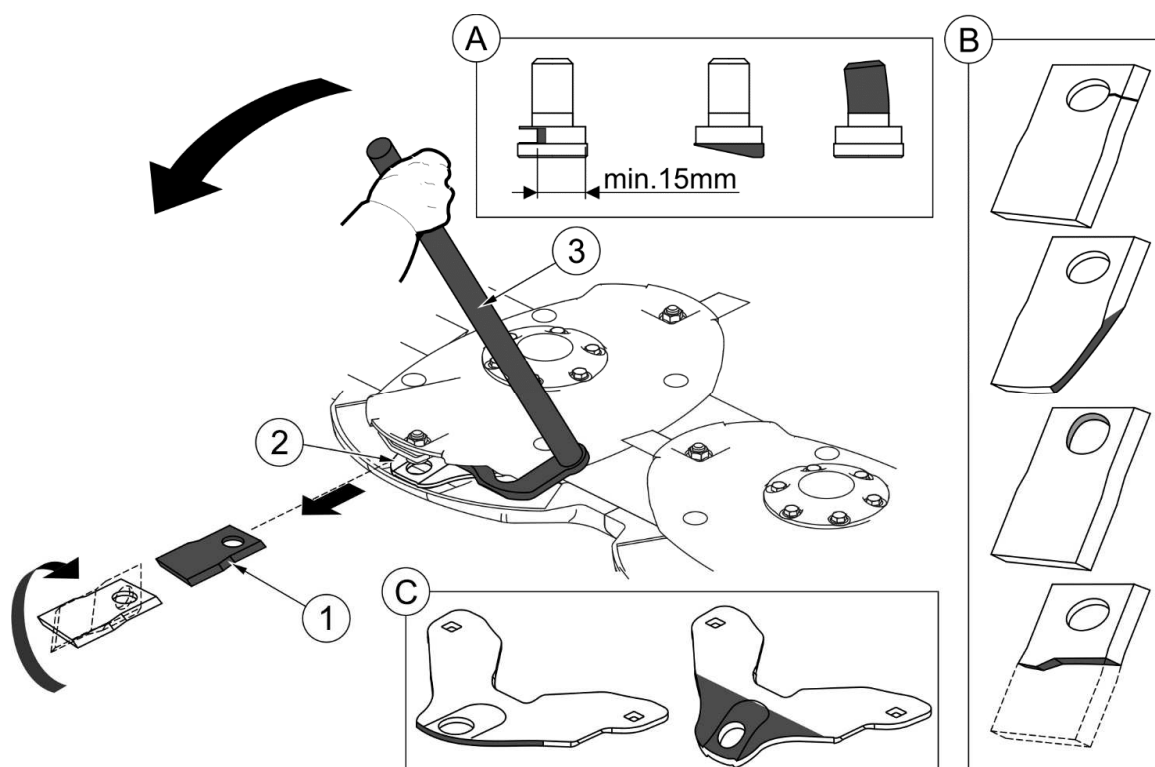
РИСУНОК 5.1 Замена срезающих ножей
