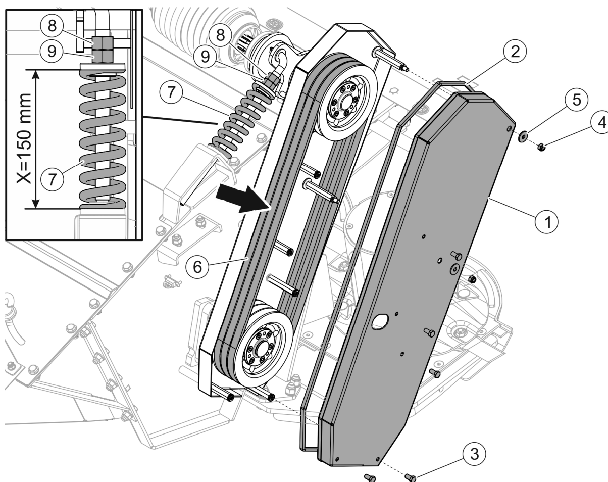
RYСУNEK 5.6 Regulacja napięcia przekładni pasowej PDF301C / PDF340C
