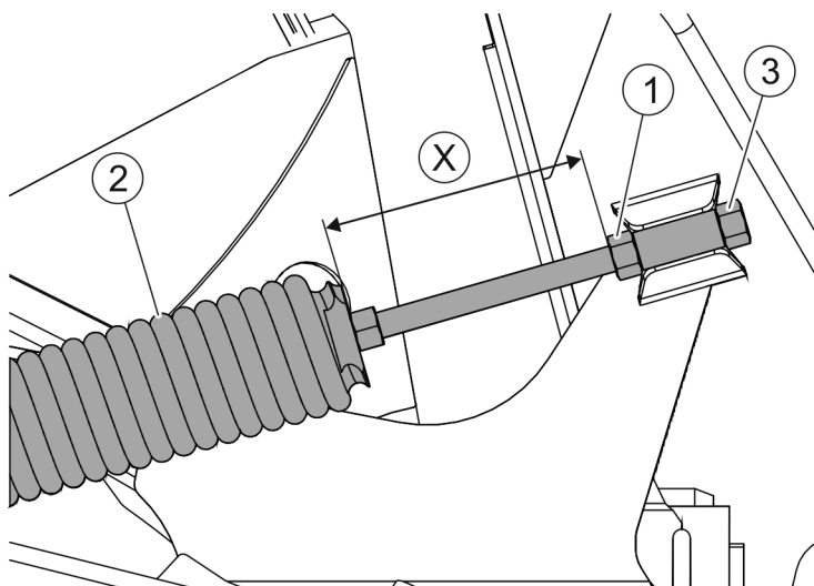
RYSUNEK 4.7 Regulacja nacisku listy tnącej
