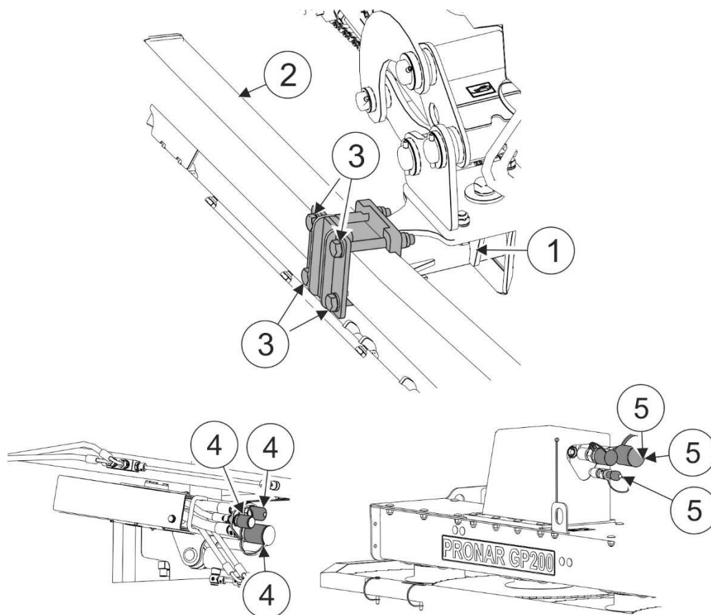
РИСУНОК 4.1 Подсоединение к универсальной стреле
