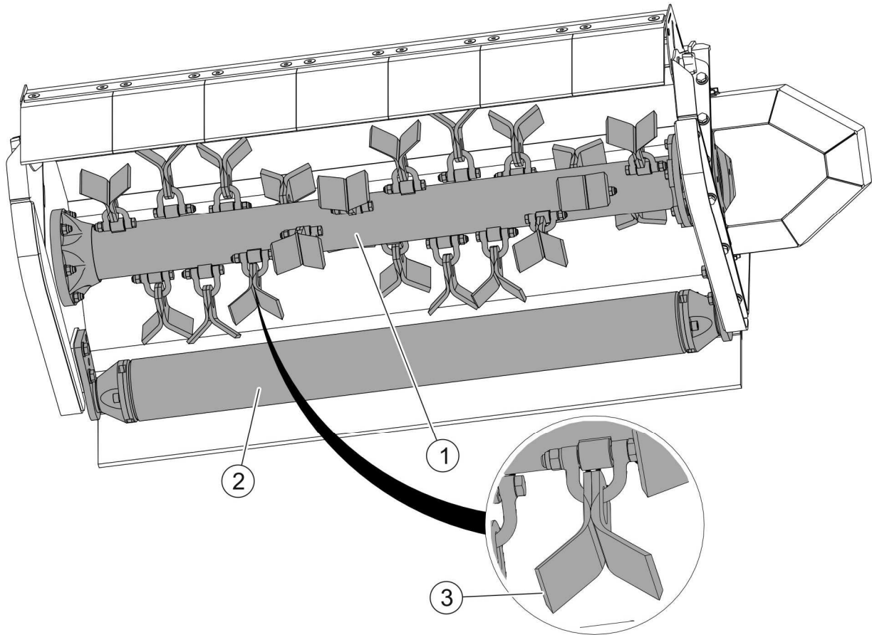
RYSUNEK 3.3 Zespół tnący
