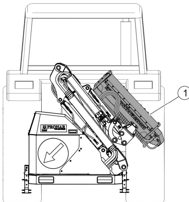
RYСУNEK 4.2 Przykładowa pozycja transportowa głowicy koszącej na wyciągniku wielofunkcyjnym
