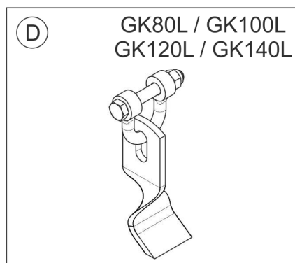
RYSUNEK 5.3 Kontrola i wymiana noży.
