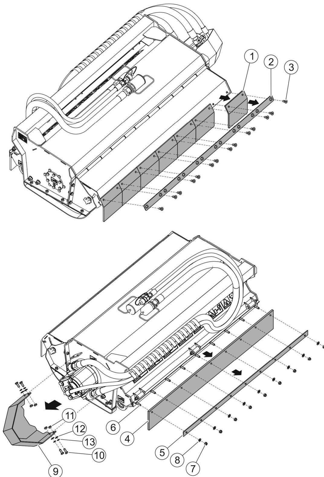
RYSUNEK 5.1 Demontaż osłon.
