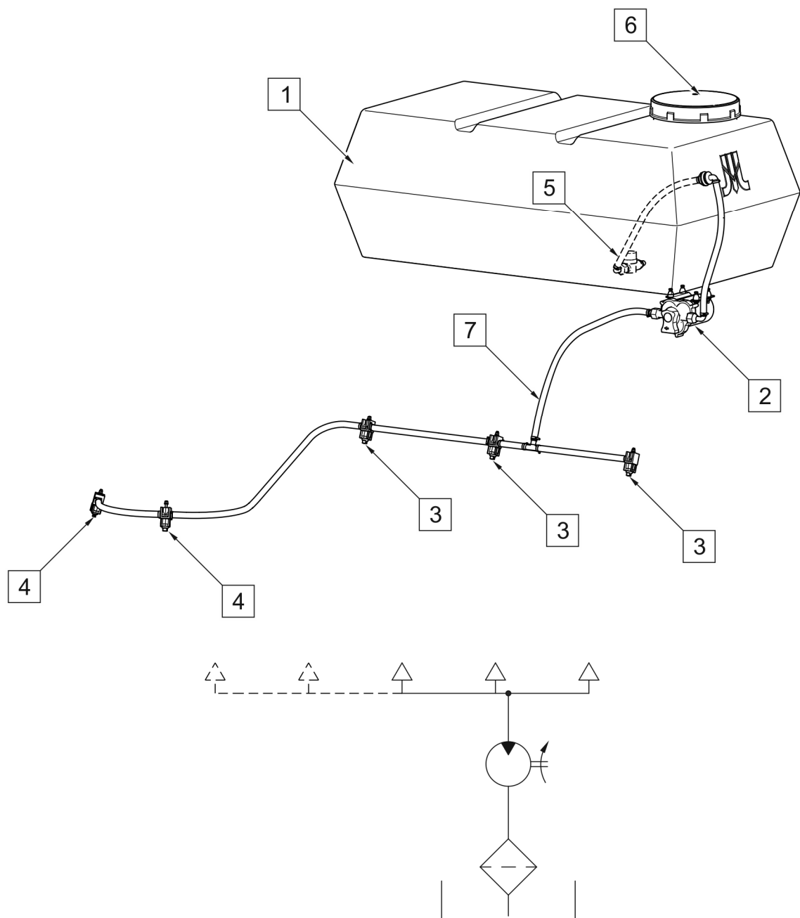
RYSUNEK 3.7 Budowa układu zraszania
