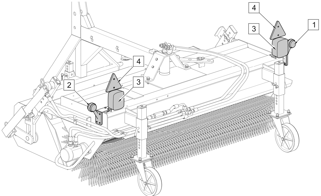
RYSUNEK 4.10 Dodatkowe oświetlenie zmiatarki pracującej za nośnikiem
