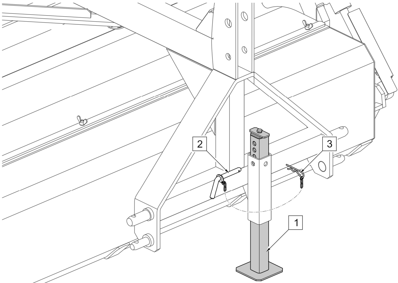
RYSUNEK 4.12 Podpórka postojowa
