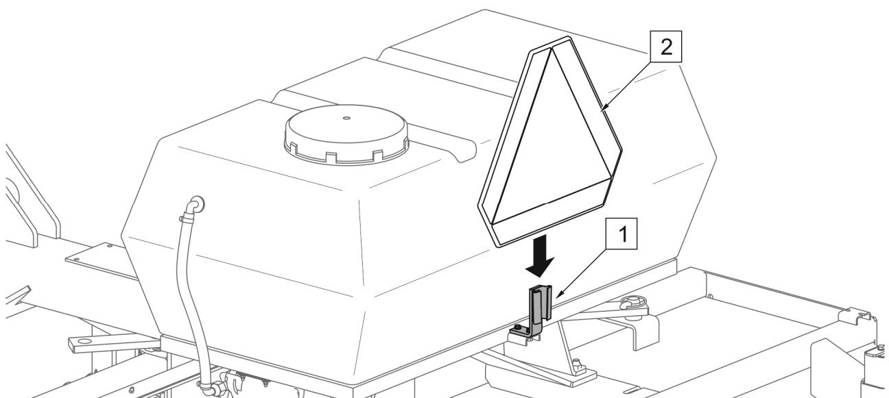
RYSUNEK 4.9 Dodatkowy wspornik tablicy wyróżniającej (opcja)
