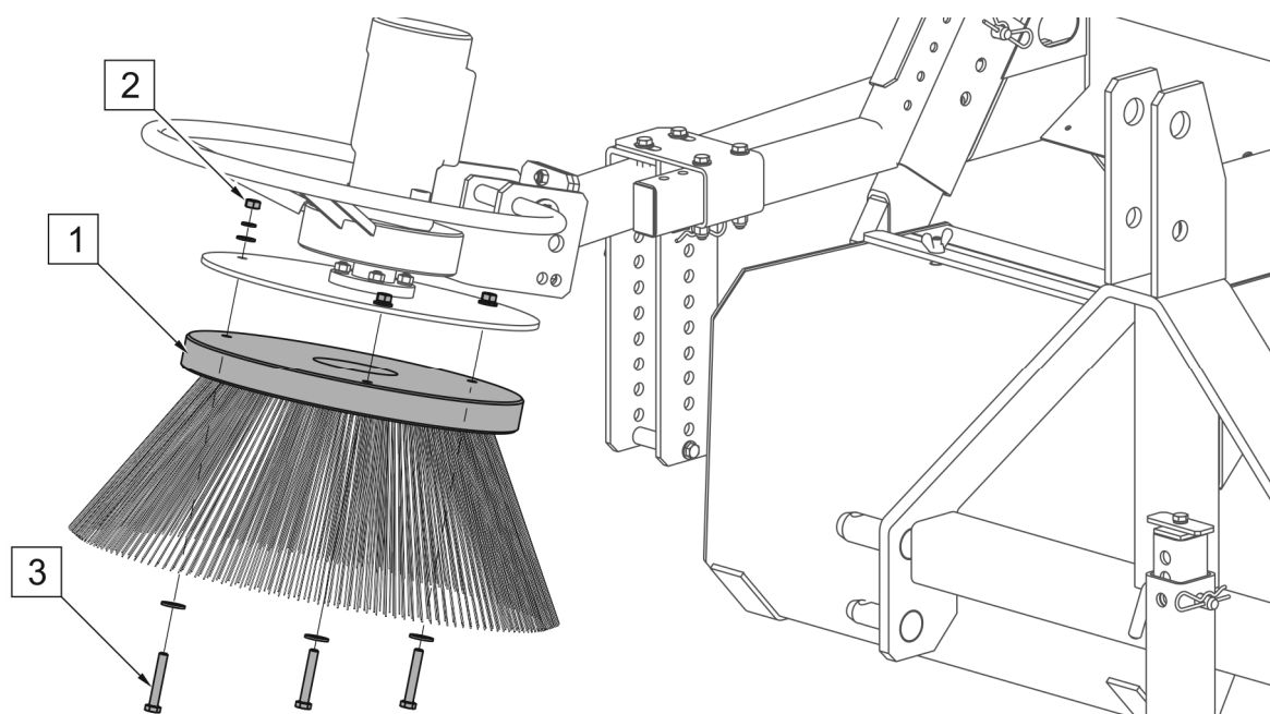
RYСУNEK 5.10 Wymiana szczotki bocznej
