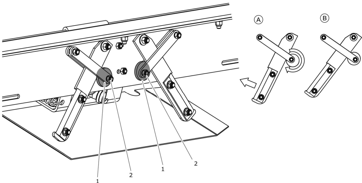
RYSUNEK 5.10 Zasada regulacji, widok z tyłu.
