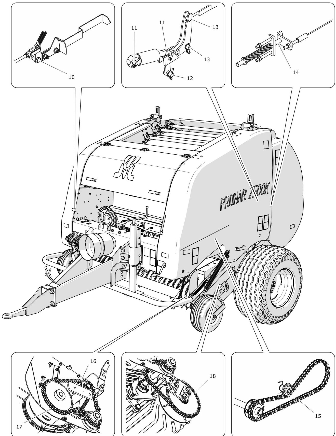
RYСУNEK 5.36 Punkty smarne prasy, część 2
