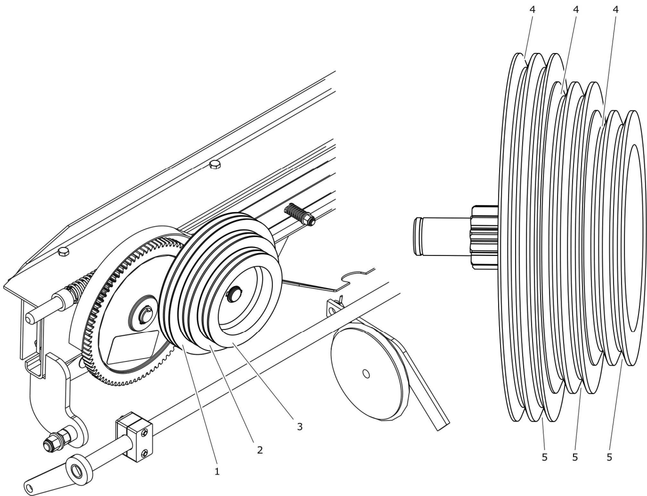
RYSUNEK 4.9 Regulacja gęstości owinięć
