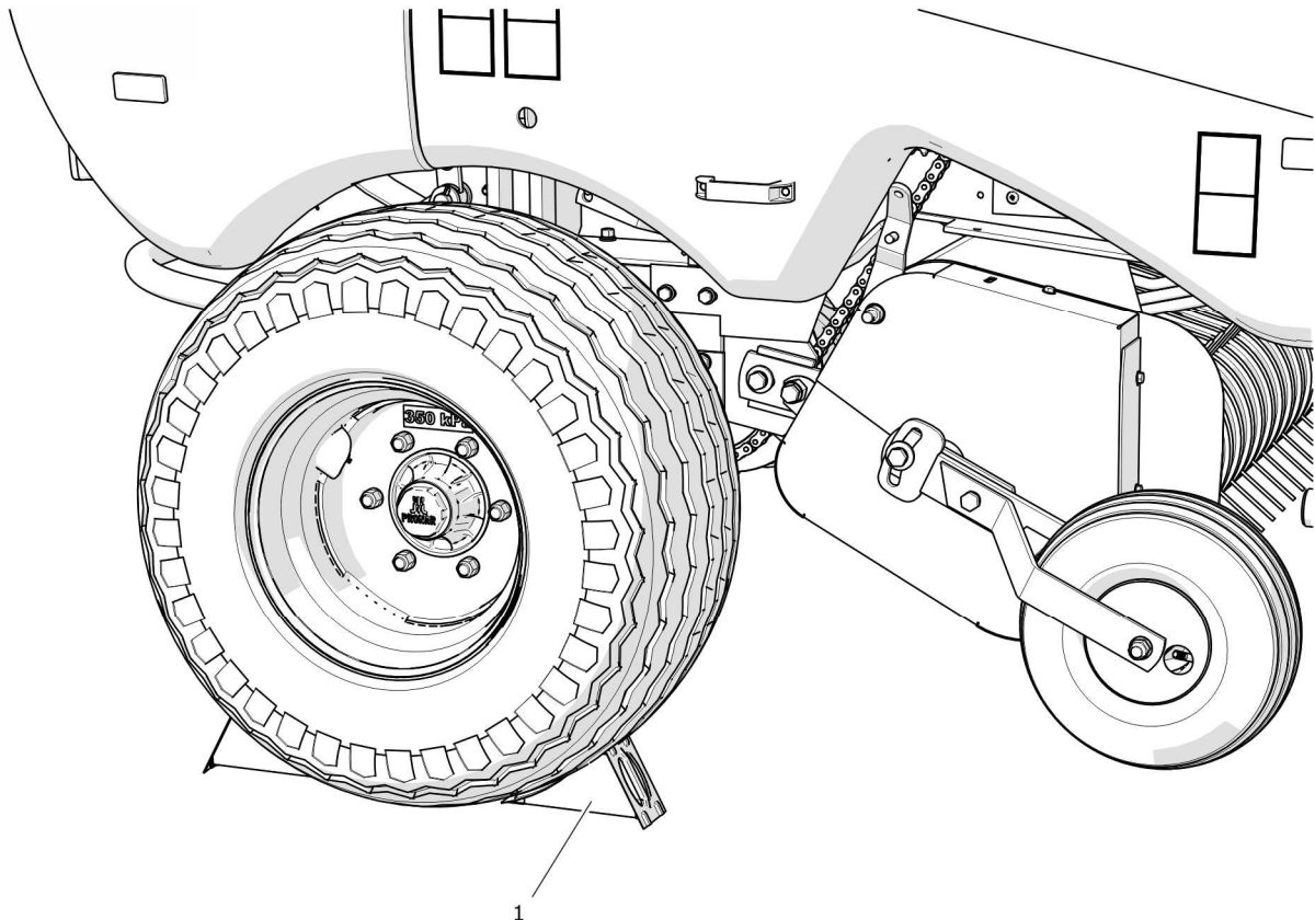
RYСУNEK 2.3 Sposób ustawiania klinów
