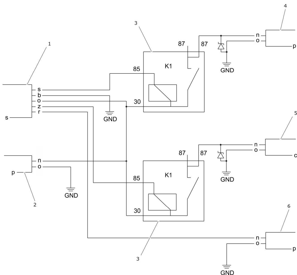
RYSUNEK 3.18 Schemat skrzynki przekaźnikowej sterownika (wersja standardowa)
