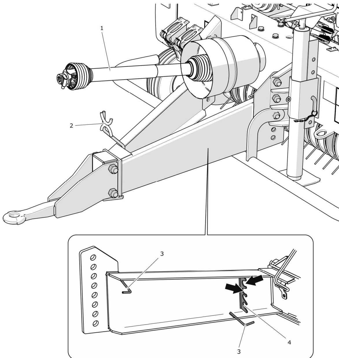
RYSUNEK 4.3 Wspornik wału przegubowo teleskopowego
