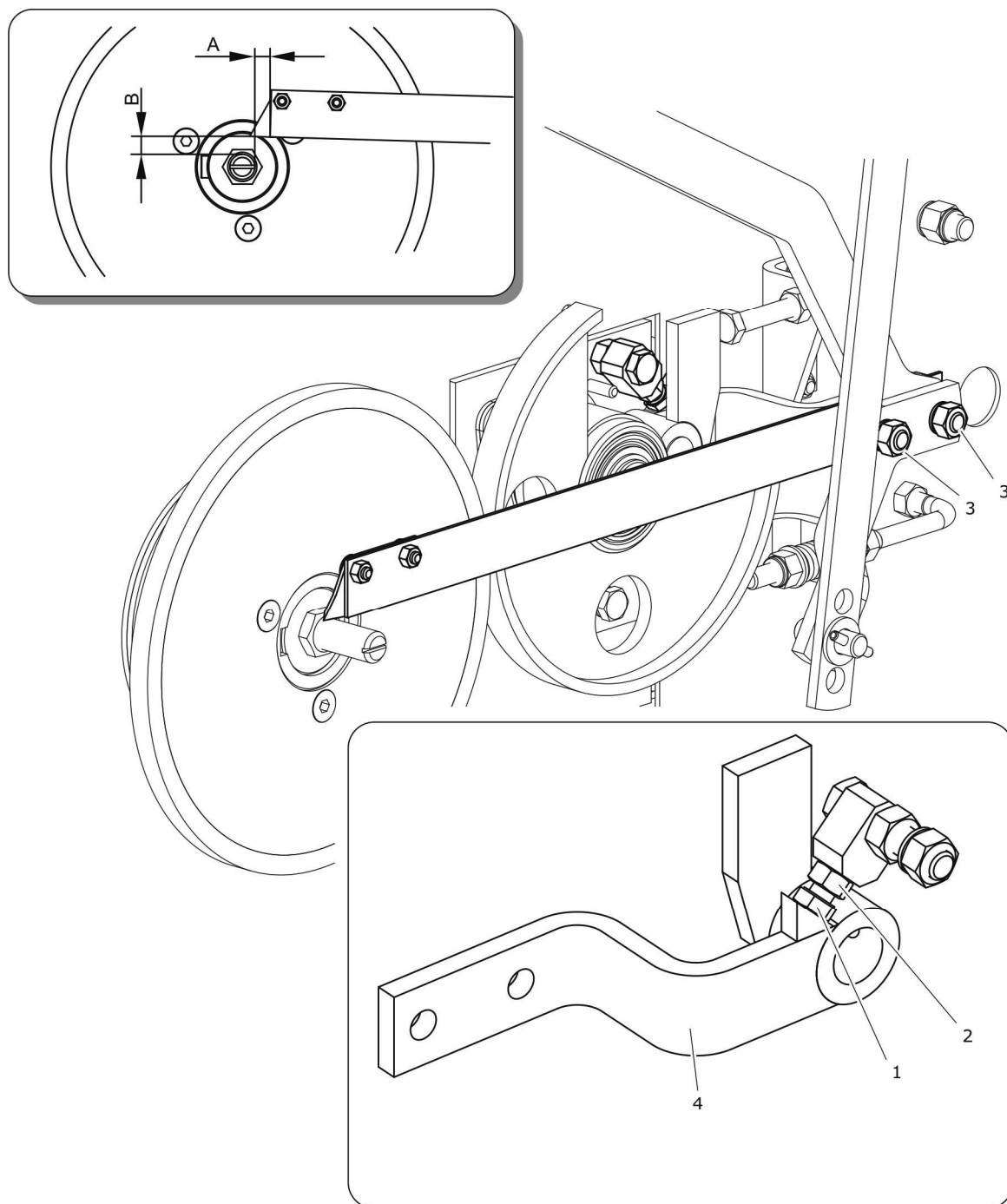
RYSUNEK 5.32 Regulacja położenia ramienia sprężystego
