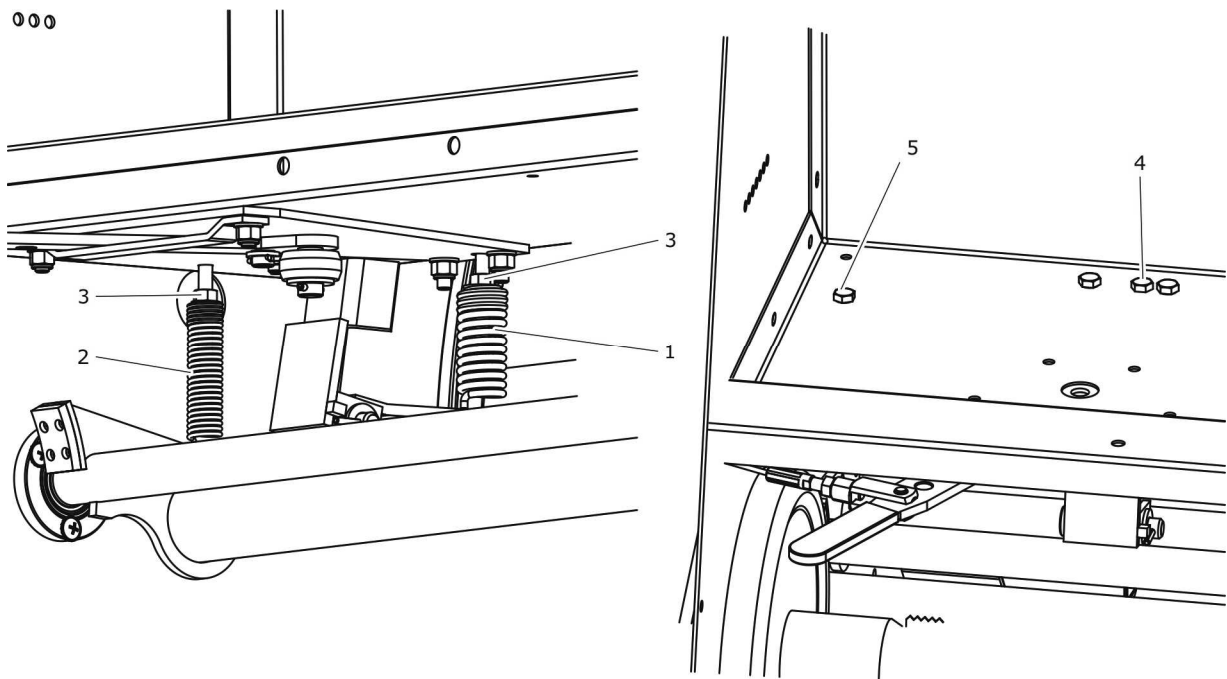
RYСУNEK 5.30 Regulacja napięcia sprężyny głównej i pomocniczej
