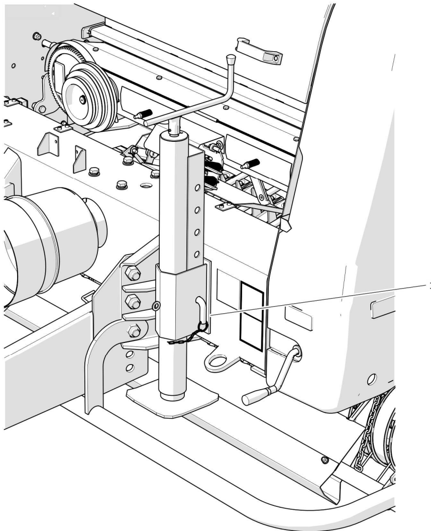
RYSUNEK 4.2 Podpora postojowa w pozycji transportowej
