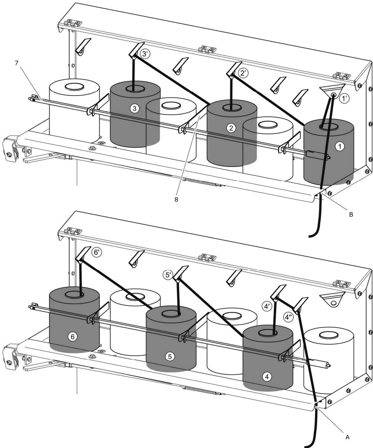
RYСУNEK 4.4 Prowadzenie sznurka w zasobniku
