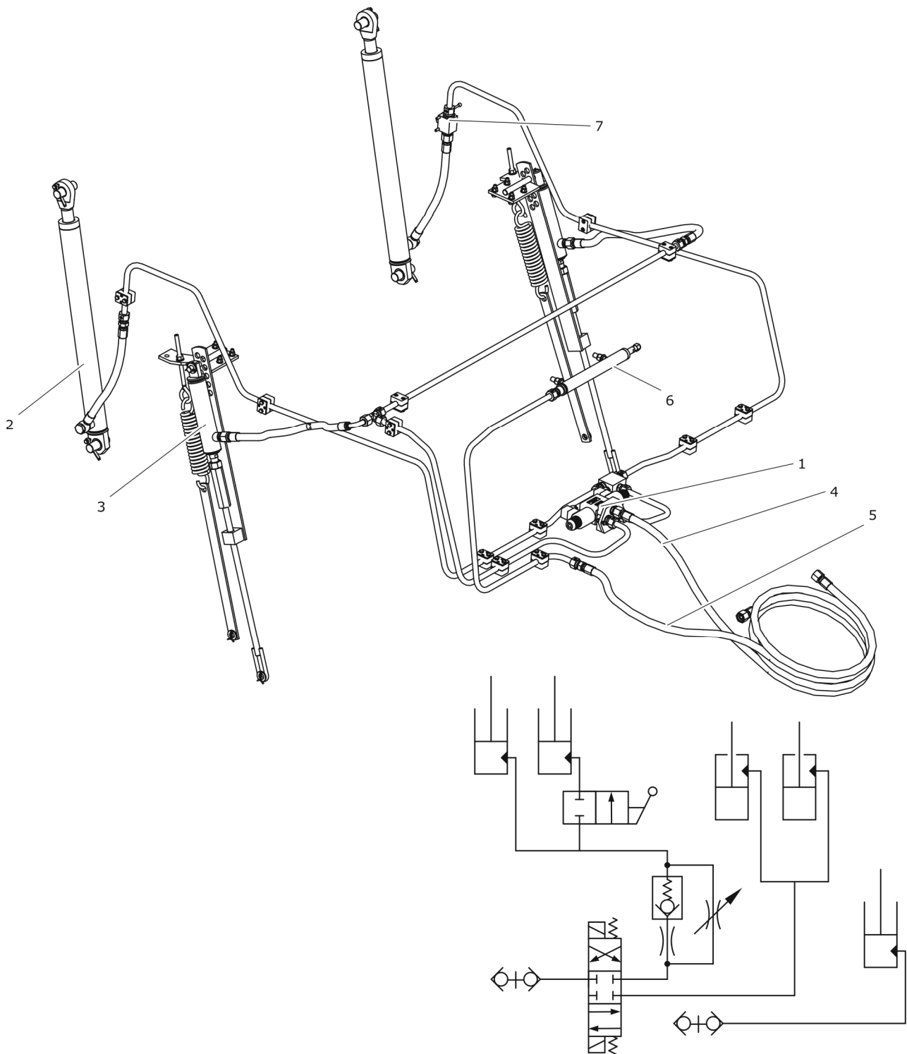
RYSUNEK 3.19 Budowa i schemat instalacji hydraulicznej
