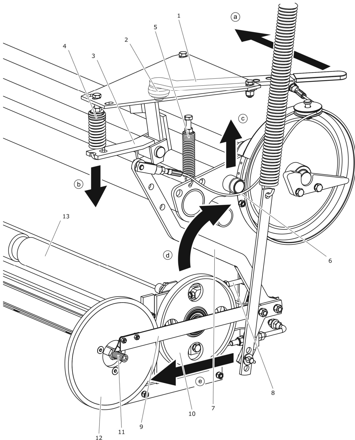
RYSUNEK 3.8 Zasad działania mechanizmu owijania siatką
