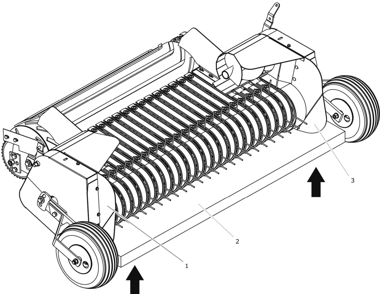
RYSUNEK 5.14 Miejsce ustawienia podnośników
