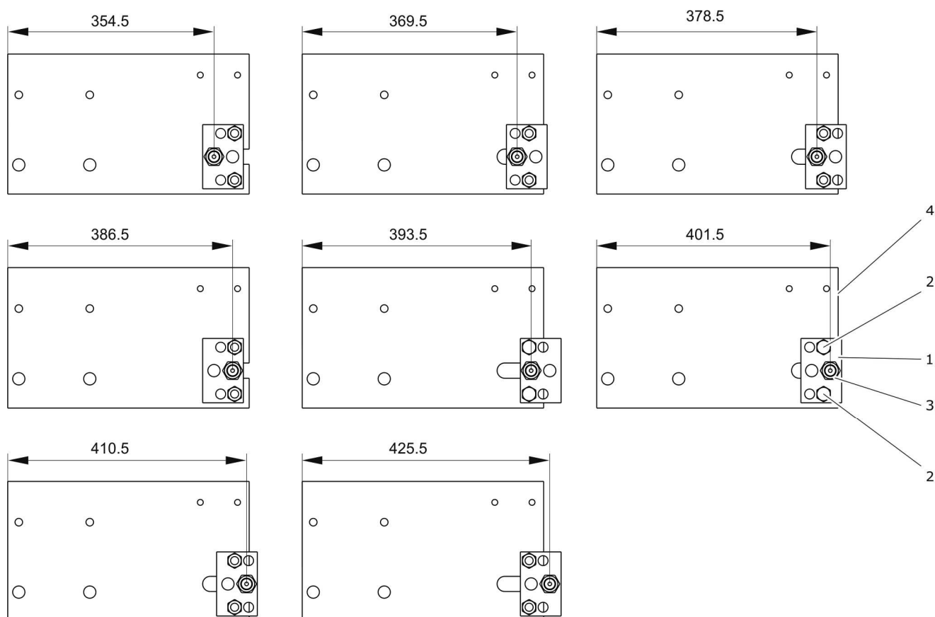
RYSUNEK 5.23 Warianty ustawienia płytki regulacyjnej
