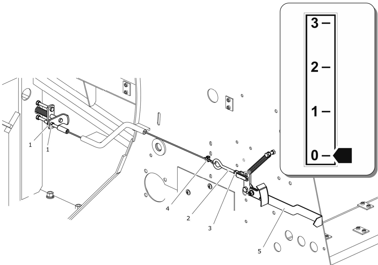
RYSUNEK 5.16 Regulacja wskaźnika zagęszczenia
