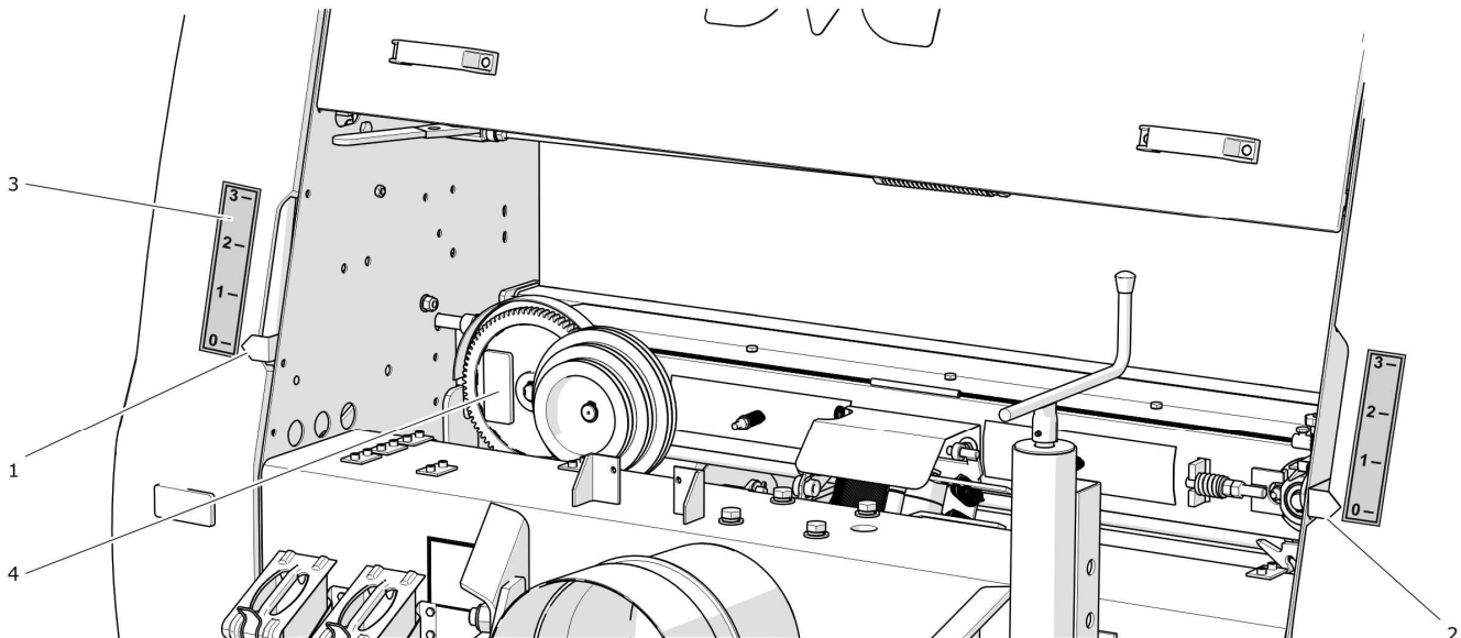
RYSUNEK 4.15 Wskaźnik zagęszczenia balotów
