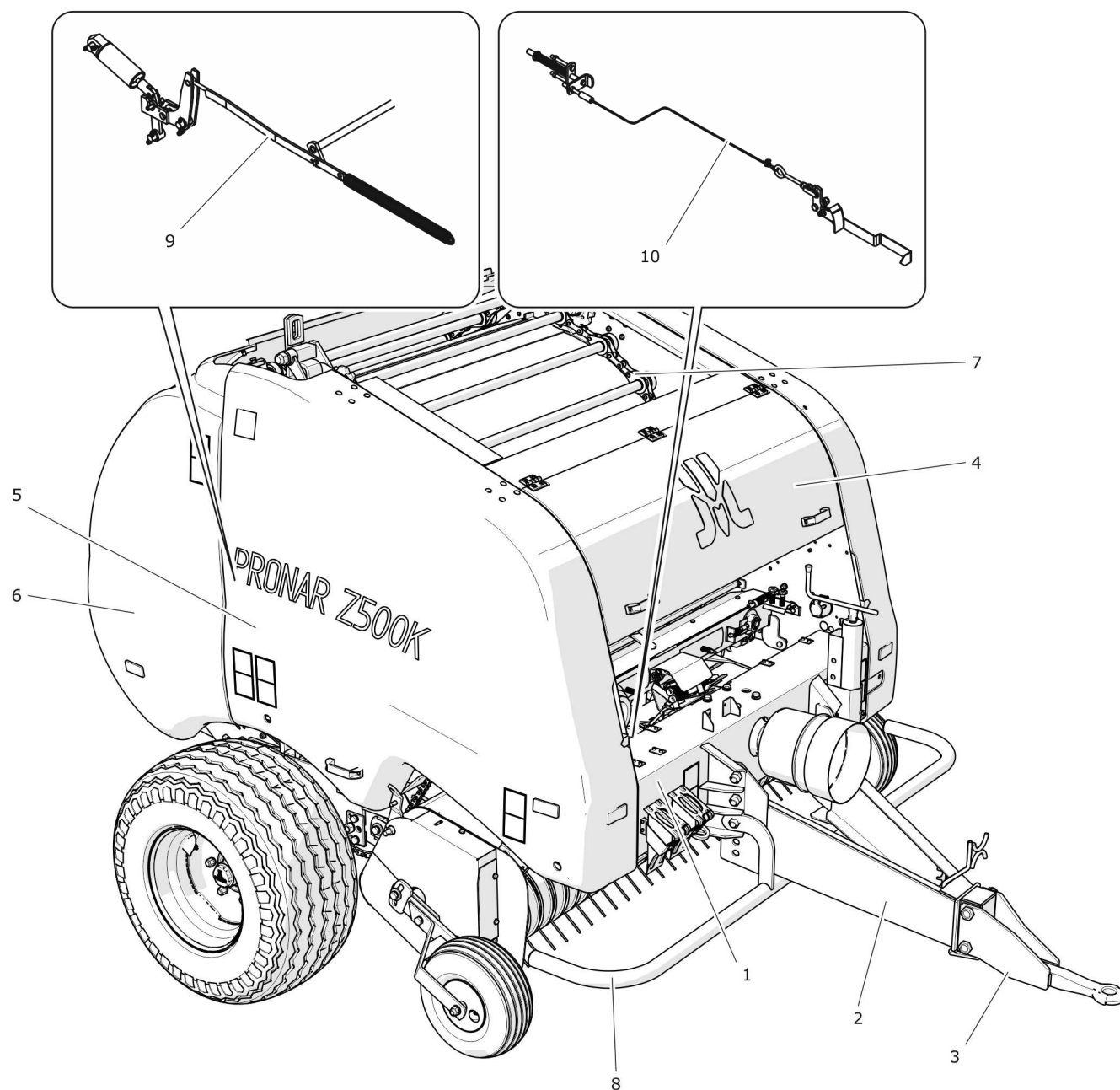
RYСУNEK 3.1 Budowa prasy belującej, część 1
