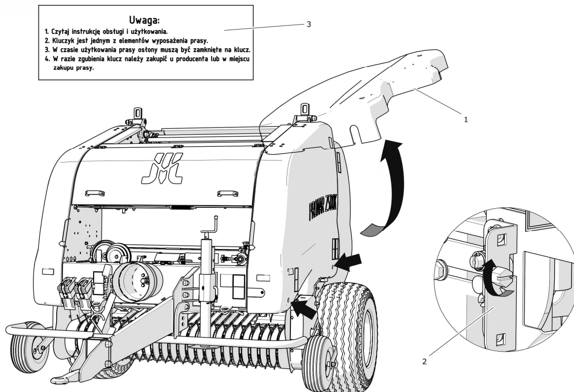
RYSUNEK 5.1 Osłona boczna lewa.
