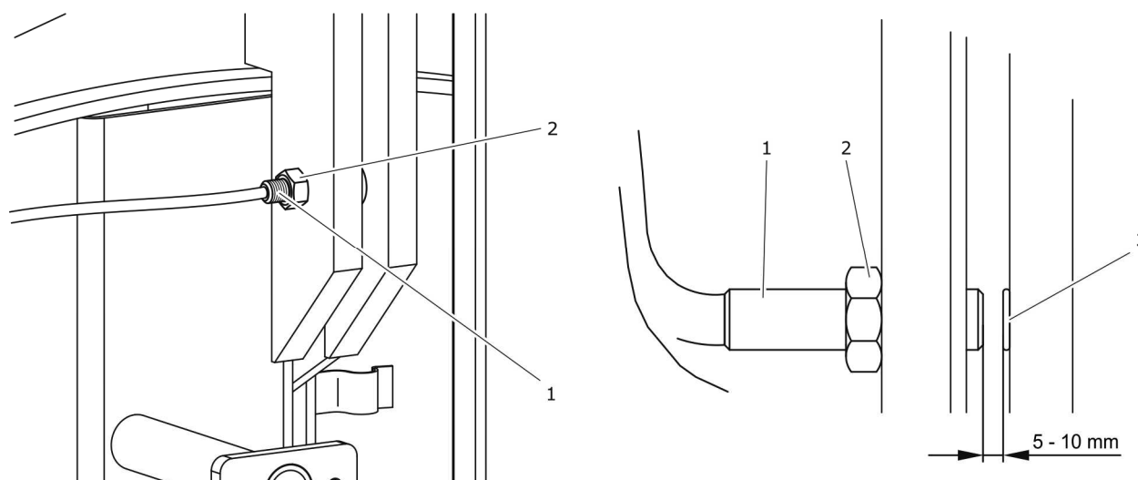
RYSUNEK 5.26 Regulacja czujnika
