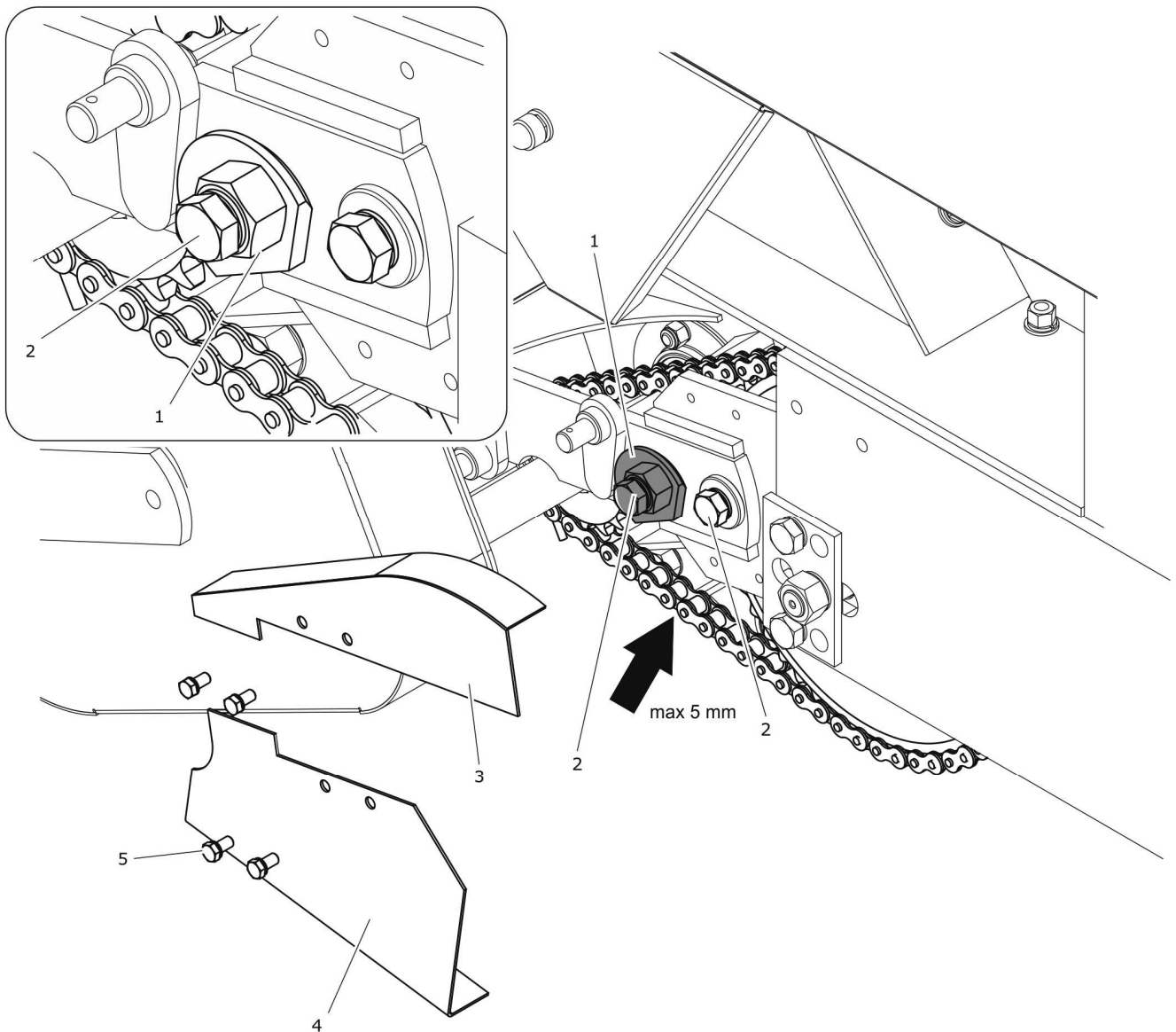
RYСУNEK 5.21 Regulacja napięcia łańcucha napędu motowideł, widok z lewej
