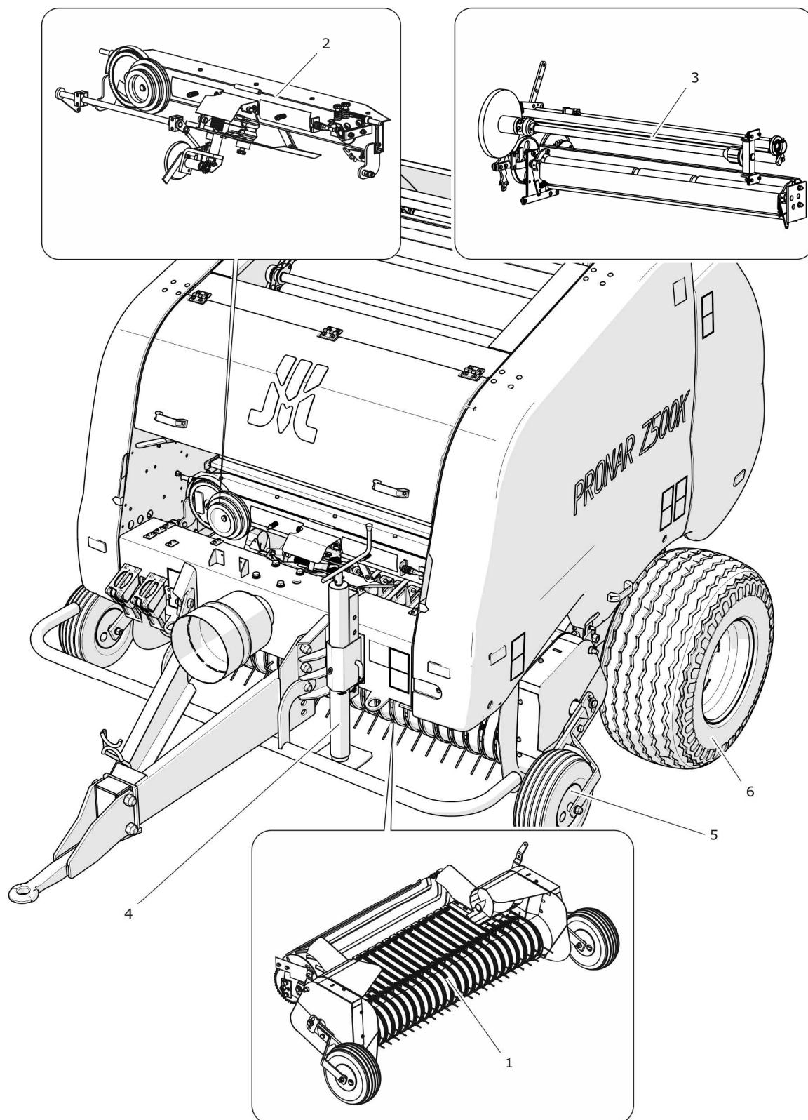
RYSUNEK 3.2 Budowa prasy belującej, część 2
