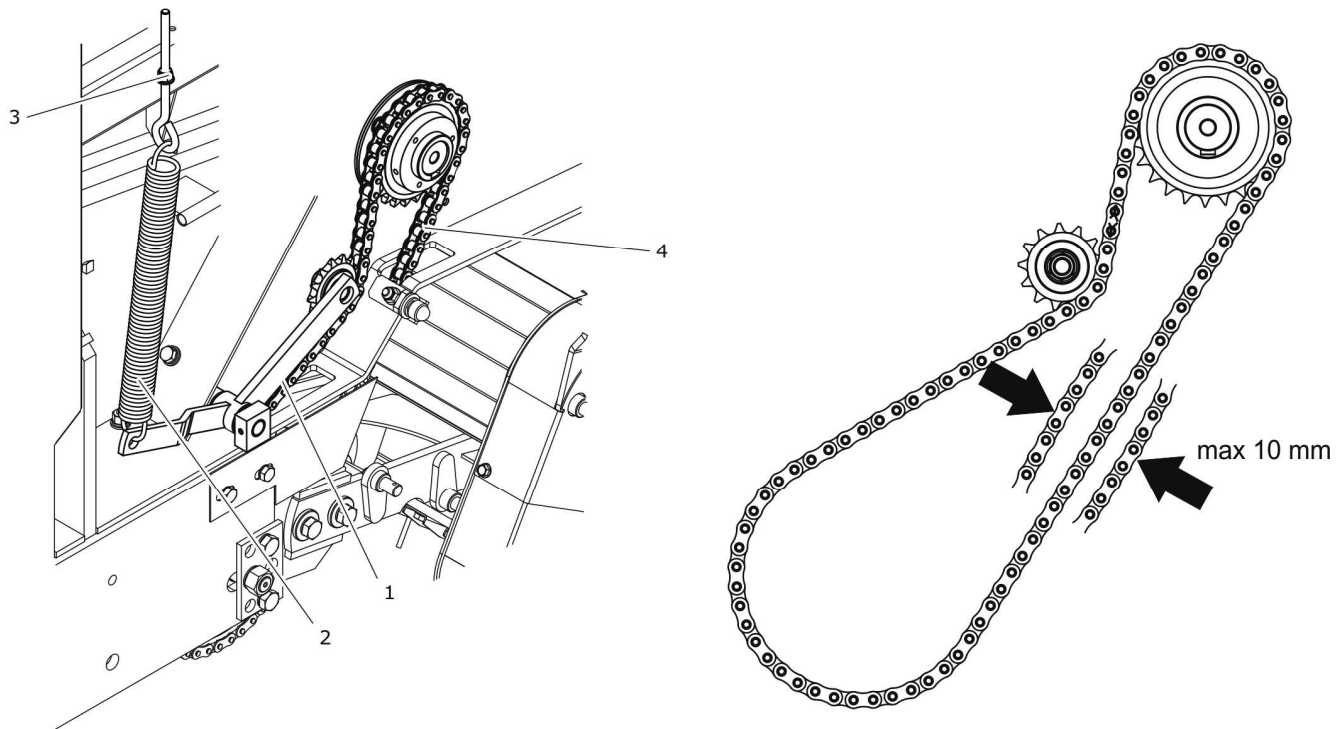
RYSUNEK 5.20 Regulacja łańcucha napędu podbieraka
