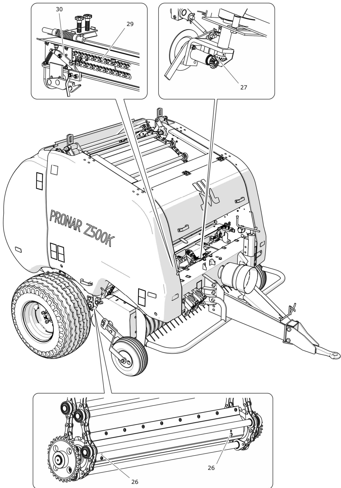
RYСУNEK 5.38 Punkty smarne prasy, część 4
