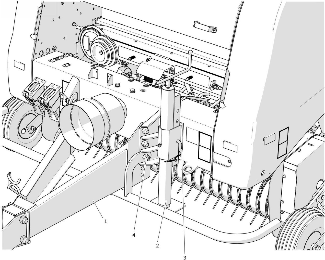
RYSUNEK 5.7 Przygotowanie prasy do regulacji wysokości dyszła
