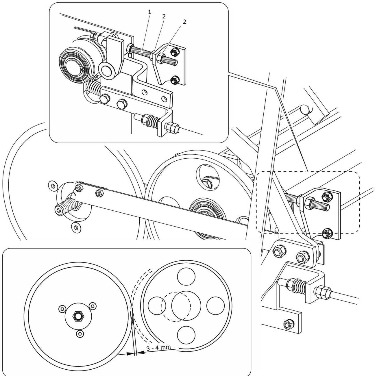
RYСУNEK 5.29 Regulacja docisku koła startowego do koła napędowego
