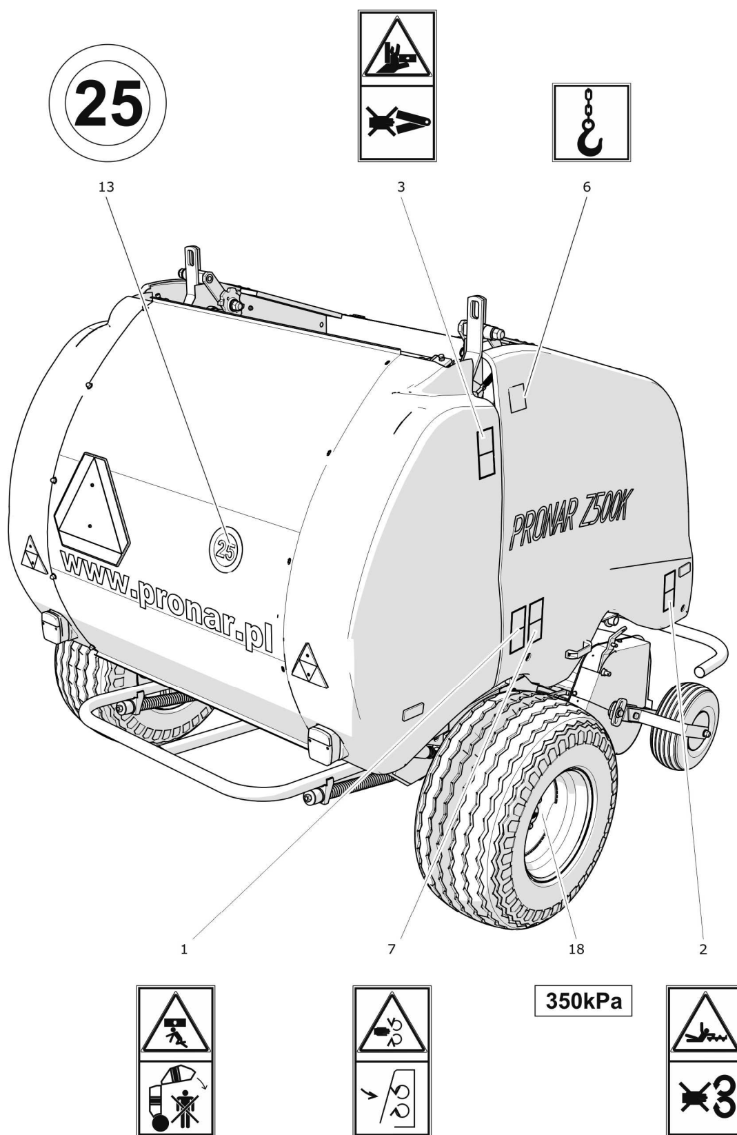
RYSUNEK 2.6 Rozmieszczenie naklejek informacyjnych i ostrzegawczych, część 3
