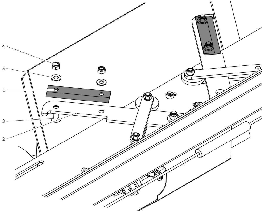
RYСУNEK 5.11 Wymiana noży, widok z dołu po otwarciu mechanizmu.
