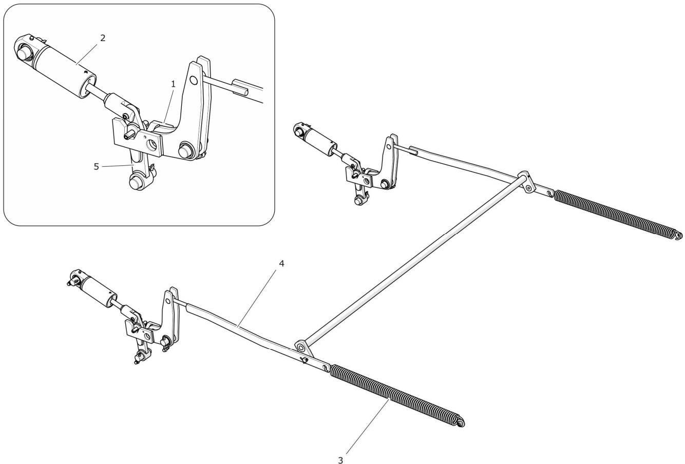
RYSUNEK 3.13 Budowa układu ryglowania klapy tylnej
