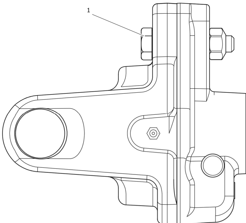
RYSUNEK 5.33 Sprzęgło ze śrubą ścinaną
