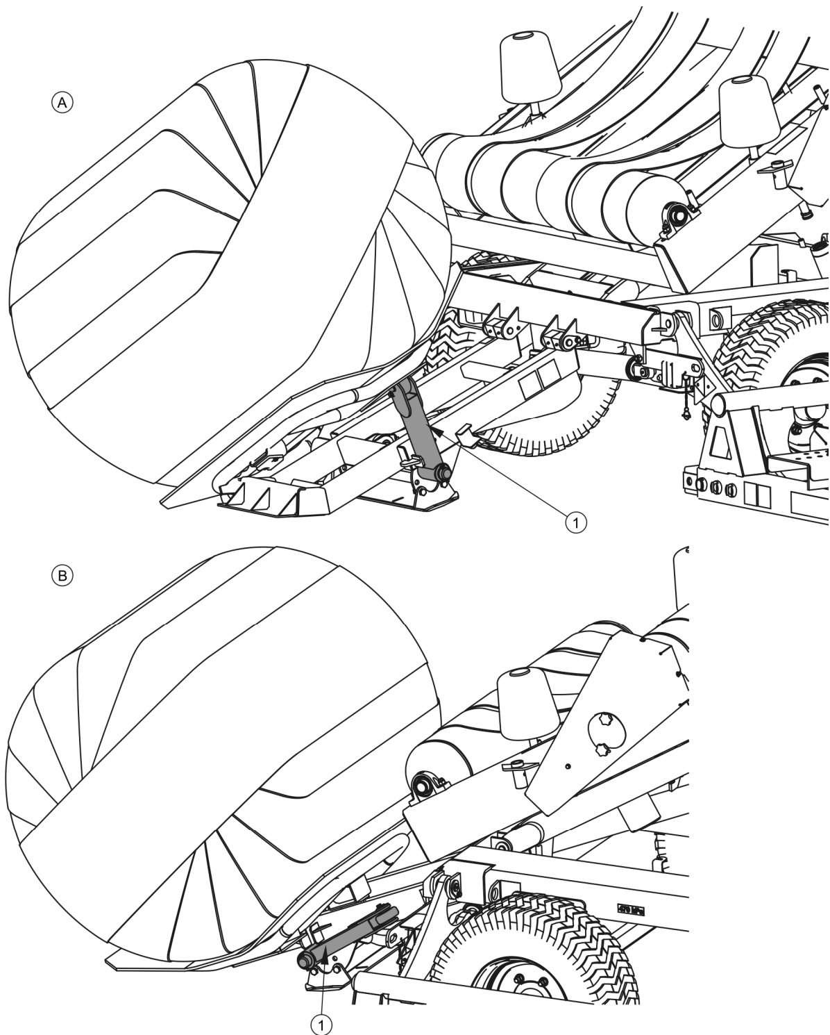
RYСУNEK 3.6 Wyładunek beli
