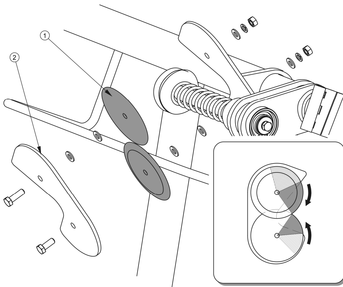
RYSUNEK 5.23 Wymiana noży tnących
