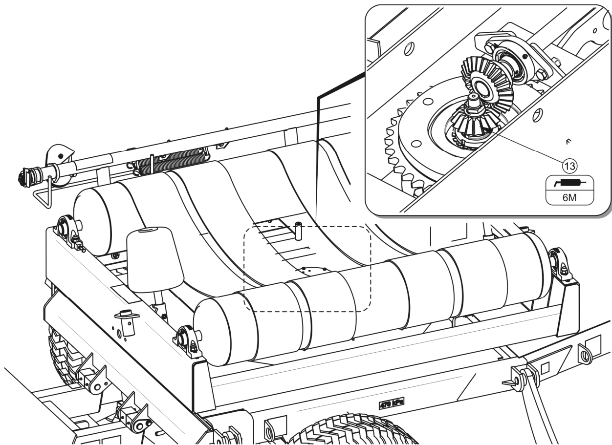
RYSUNEK 5.17 Punkty smarne owijarki, część 2
