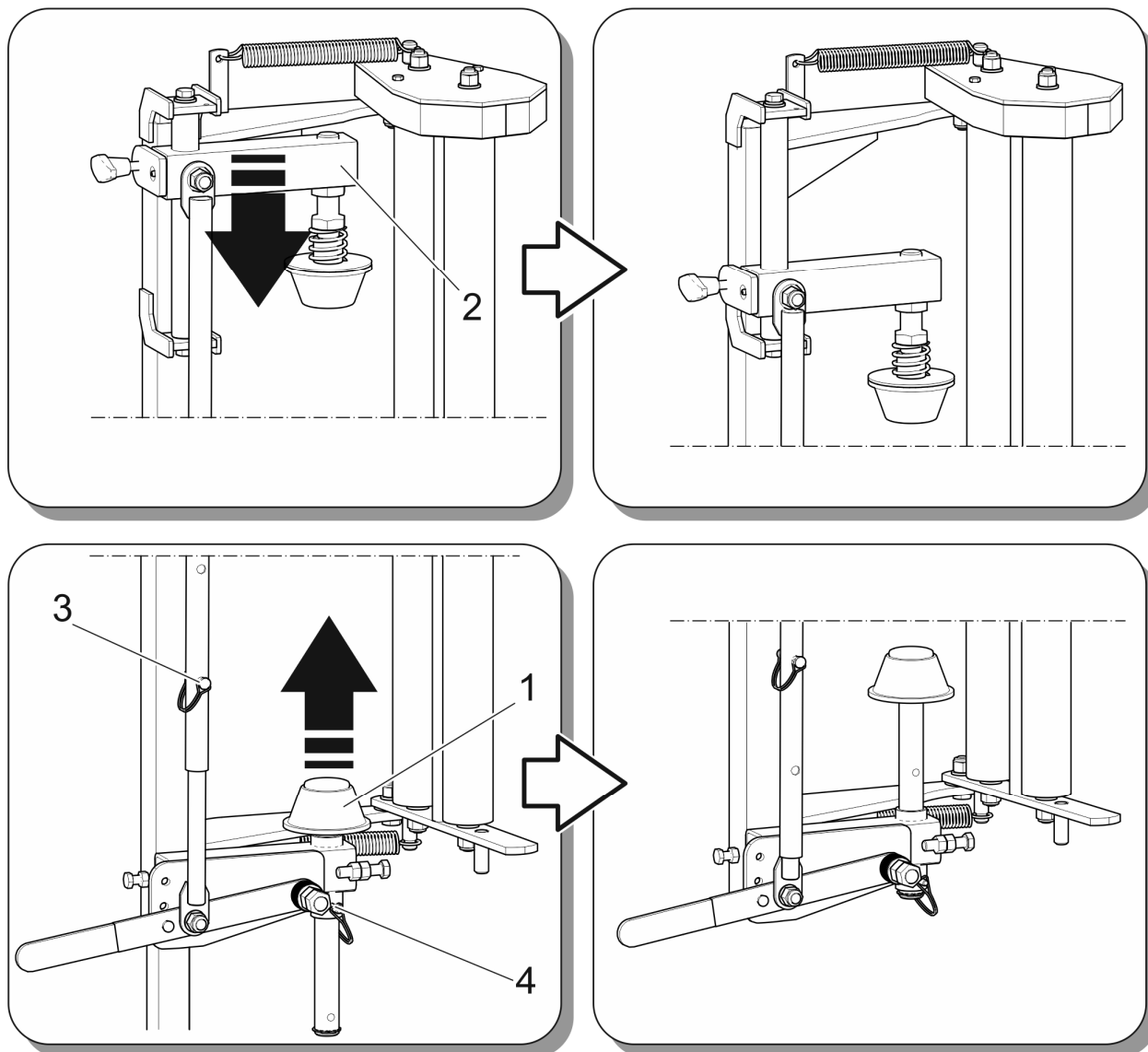
RYСУNEK 5.9 Podajnik folii
