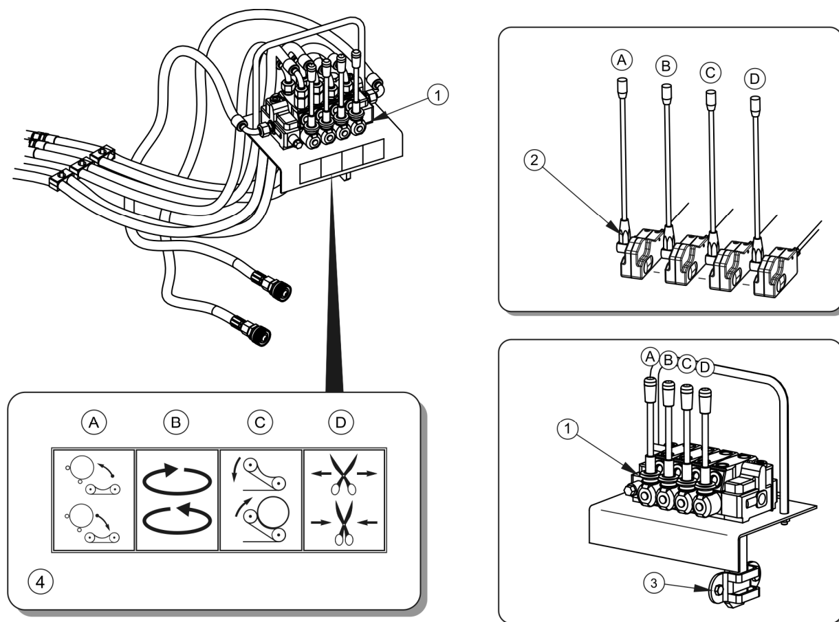
RYSUNEK 3.11 Elementy sterujące
