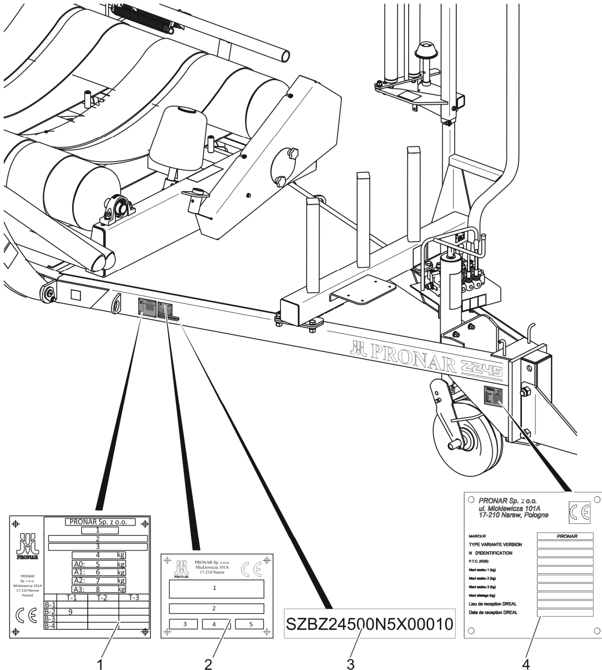
RYSunEK 1.1 Miejsce umieszczenia tabliczek znamionowych i wybicia numeru VIN
