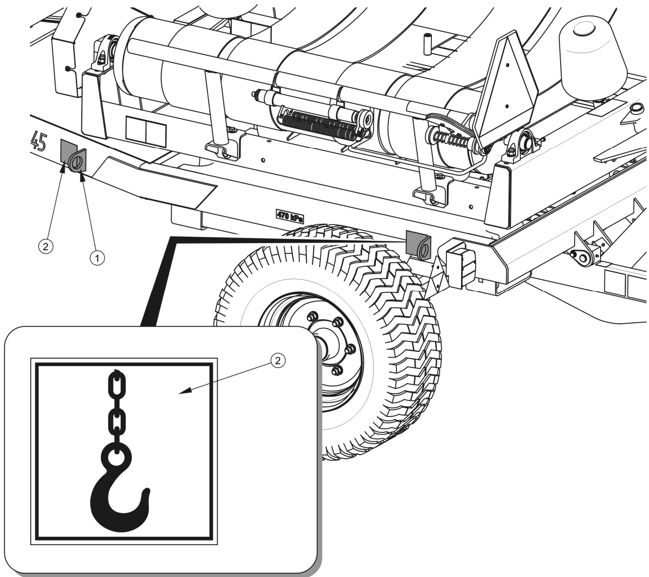
RYSUNEK 1.6 Rozmieszczenie uchwytów transportowych
