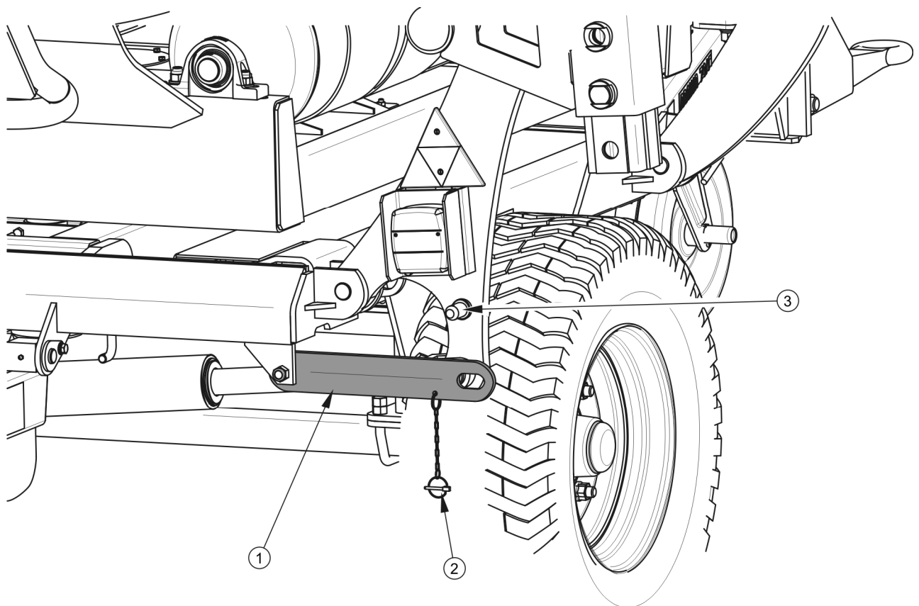
RYSUNEK 2.3 Blokada ramienia załadowniczego
