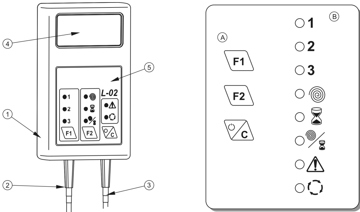
RYSUNEK 4.11 Budowa licznika L02
