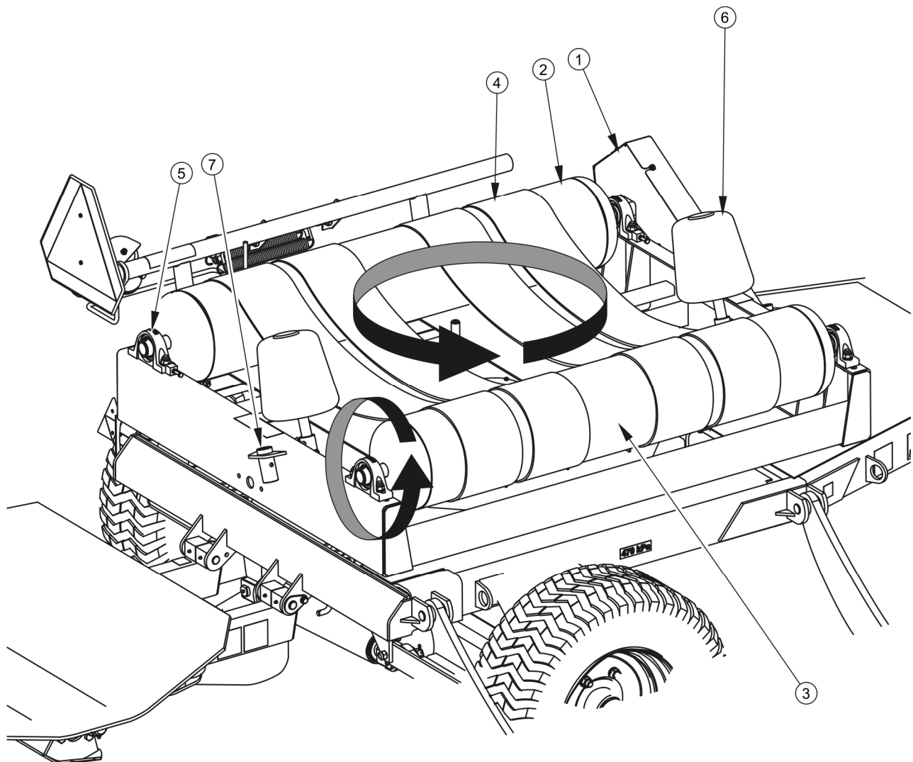
RYСУNEK 3.4 Budowa stołu obrotowego, widok z góry
