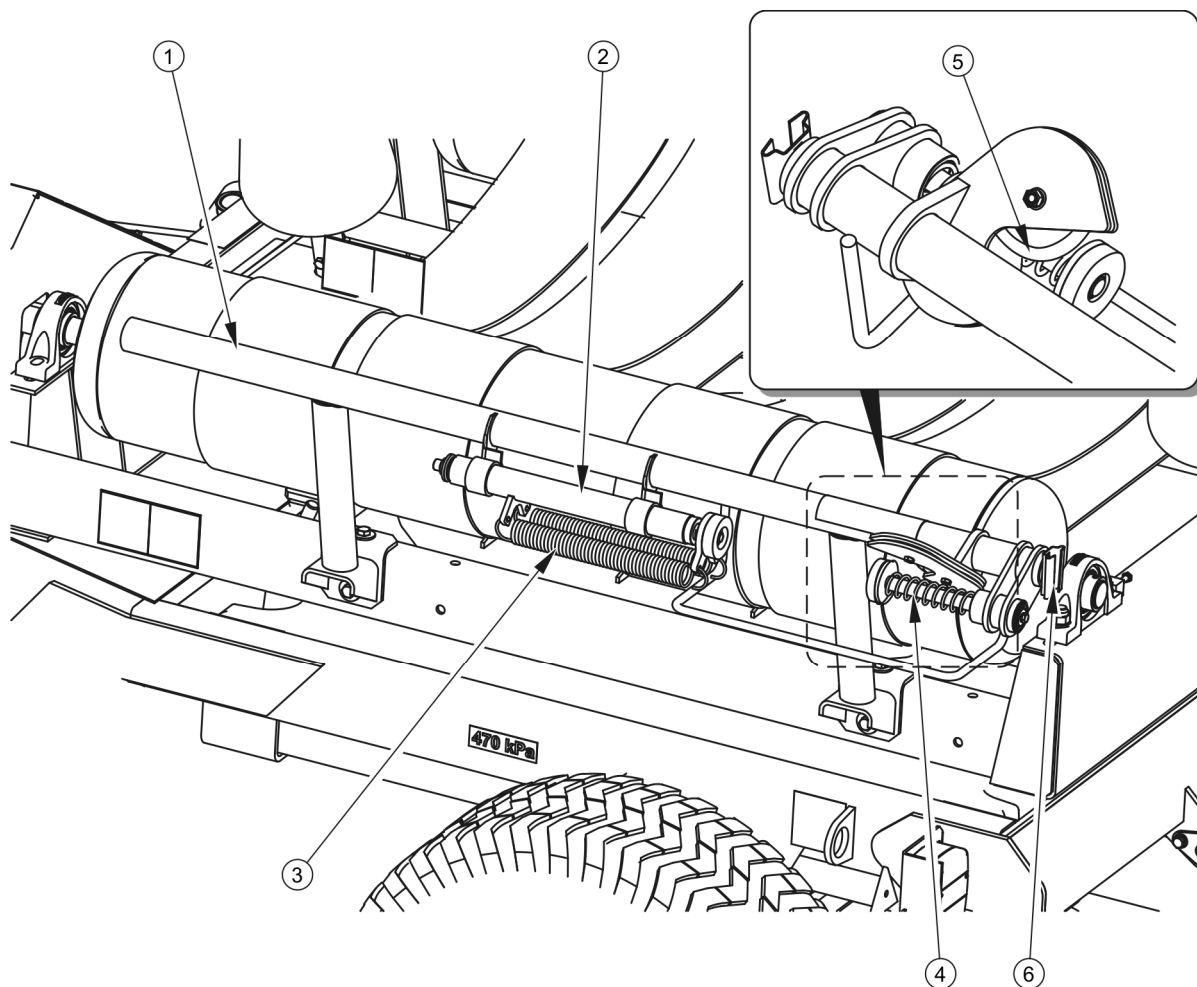
RYСУNEK 3.7 Mechanizm tnący
