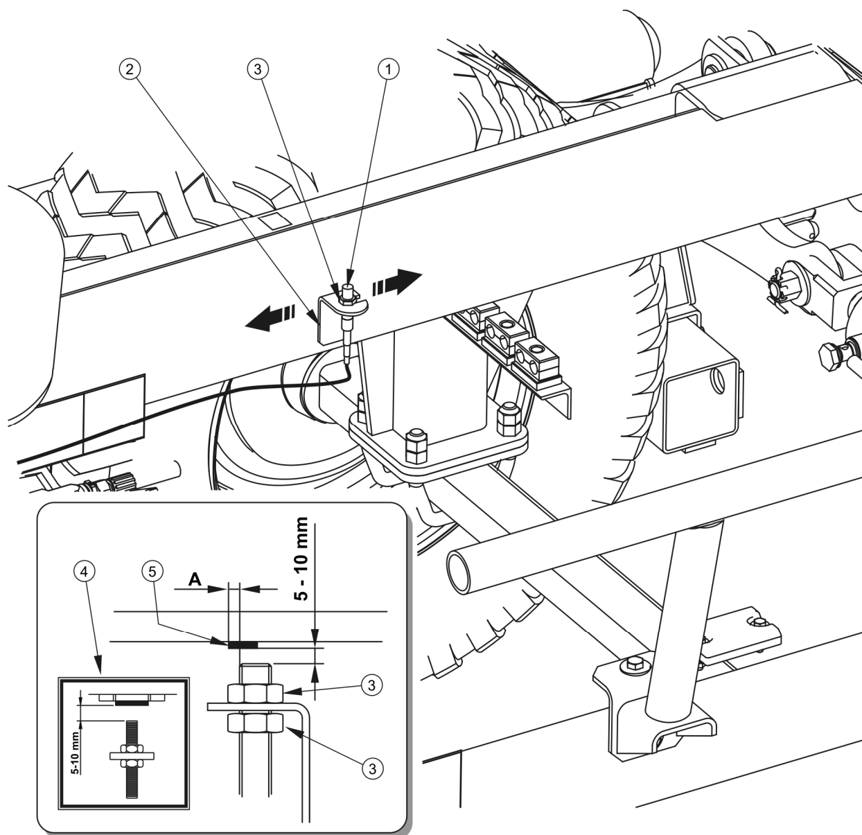
RYSUNEK 5.13 Zasada regulacji czujnika obrotów
