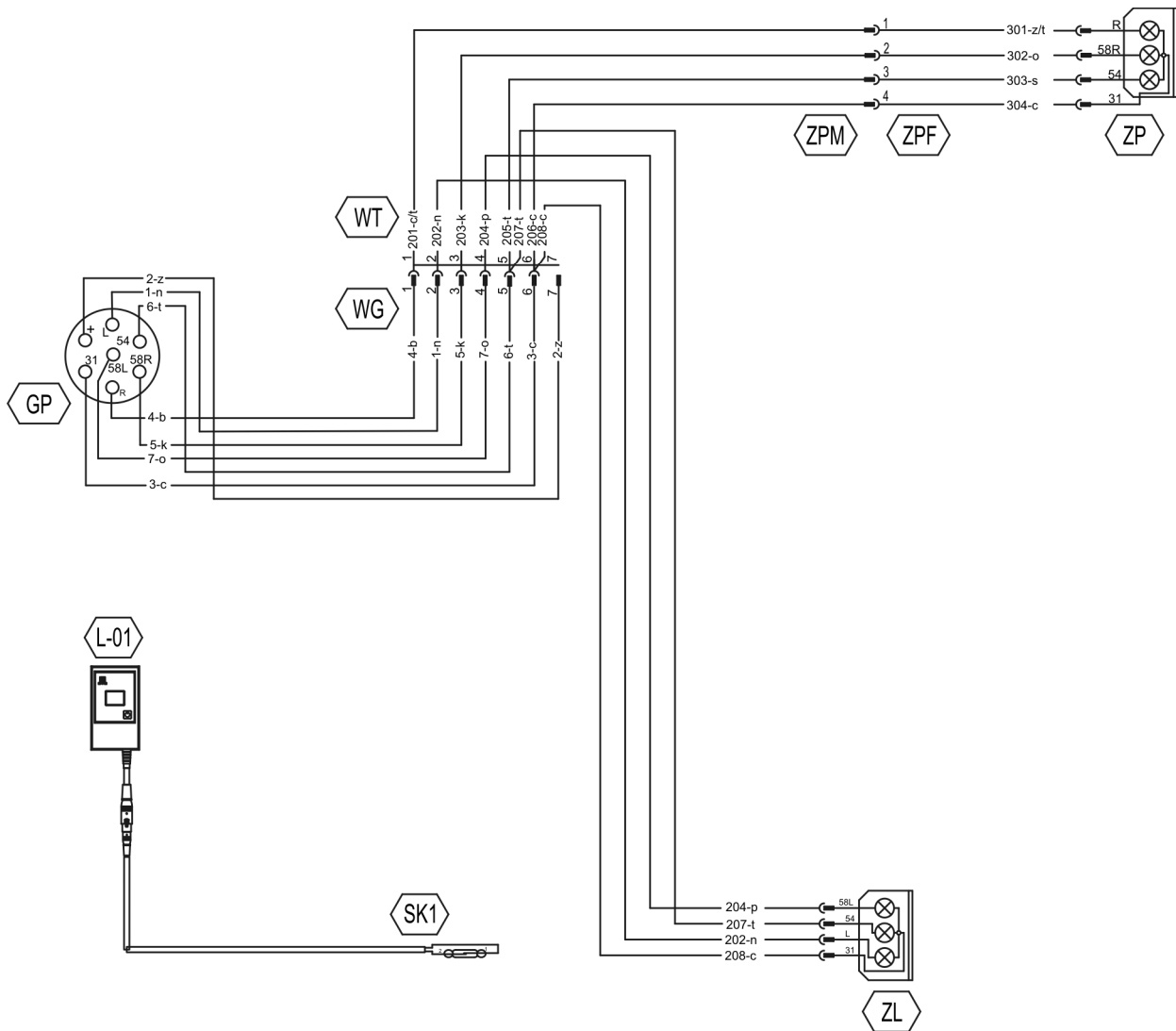
RYСУNEK 3.9 Schemat instalacji elektrycznej
