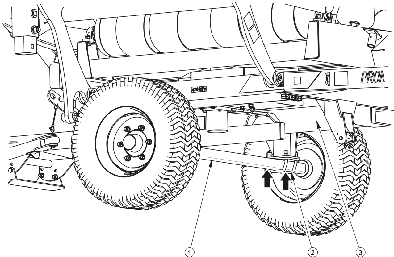
RYSUNEK 5.1 Punkt podparcia podnośnika
