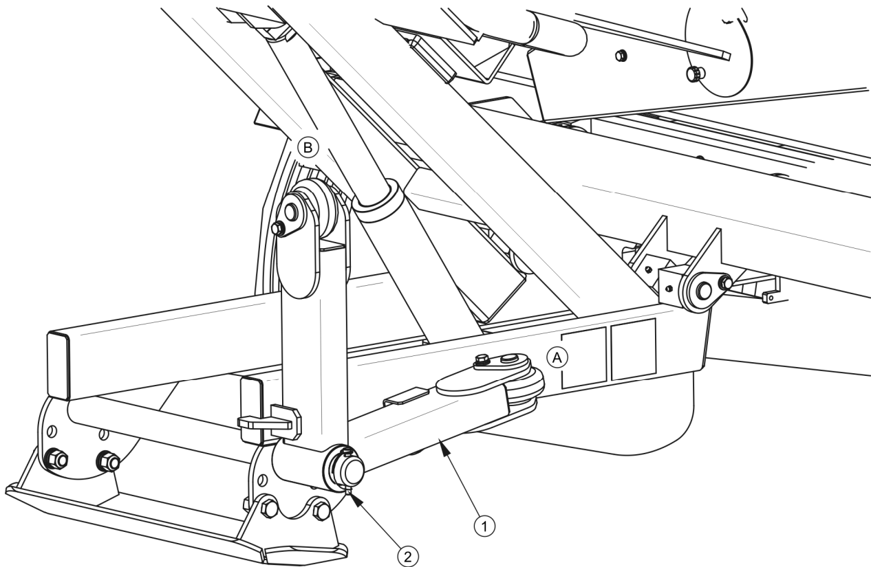
RYSUNEK 5.12 Zmian pozycji łapy wywrotu boczego
