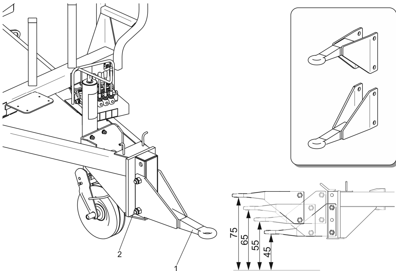
RYSUNEK 5.19 Regulacja położenia dyszla
