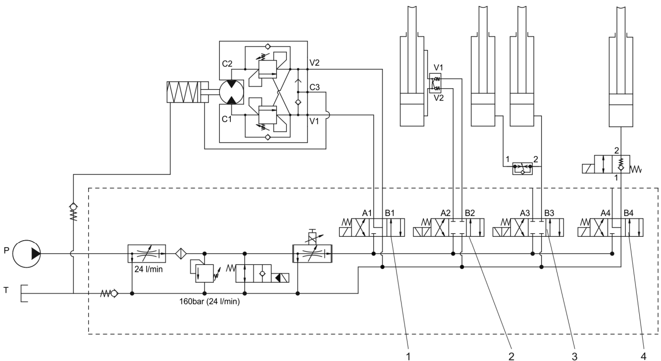
RYSUNEK 3.13 Schemat instalacji hydraulicznej ze sterowaniem elektrycznym
