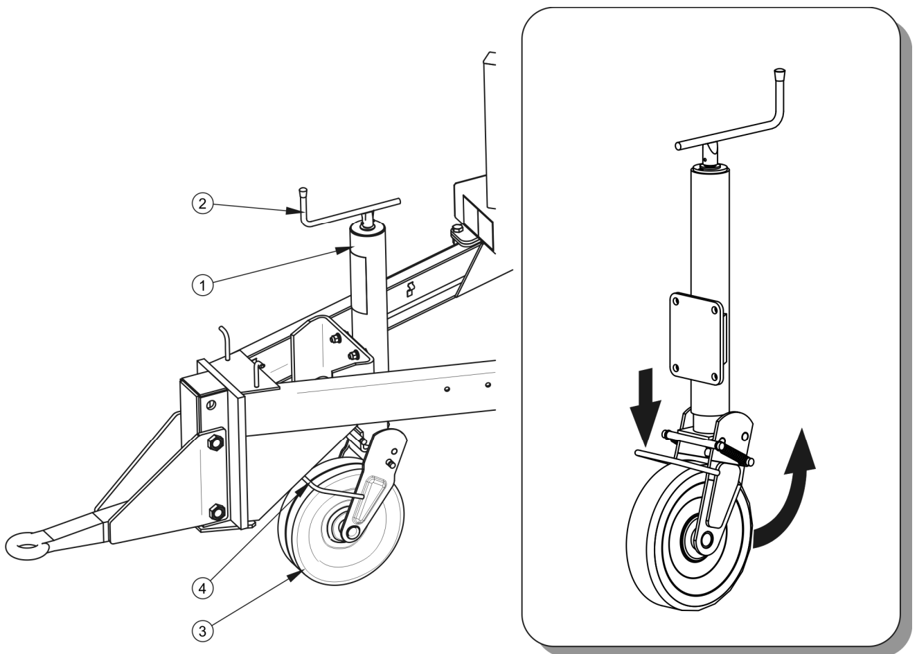
RYSUNEK 4.1 Podpora owijarki
