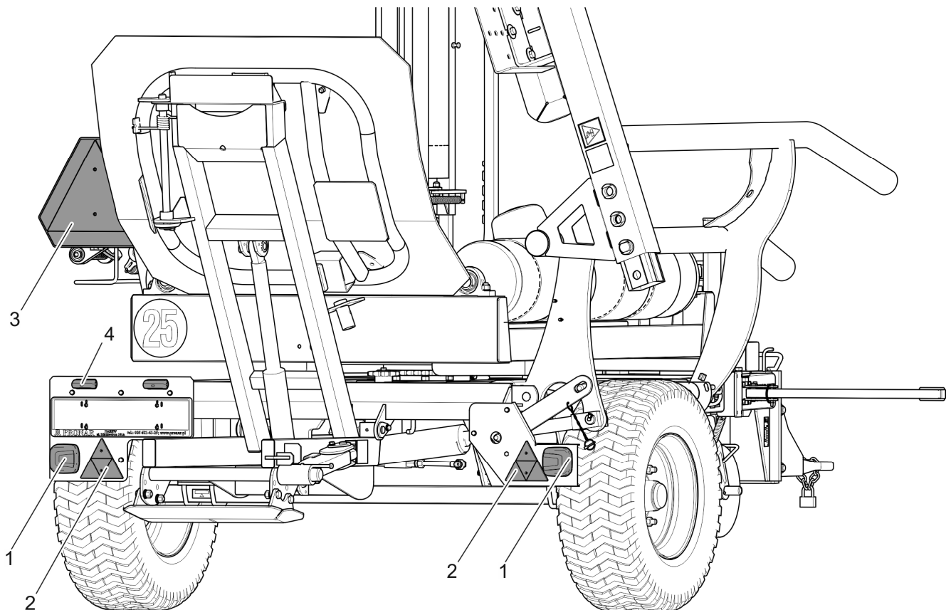
RYSUNEK 3.8 Rozmieszczenie elementów oświetlenia elektrycznego i świateł odblaskowych
