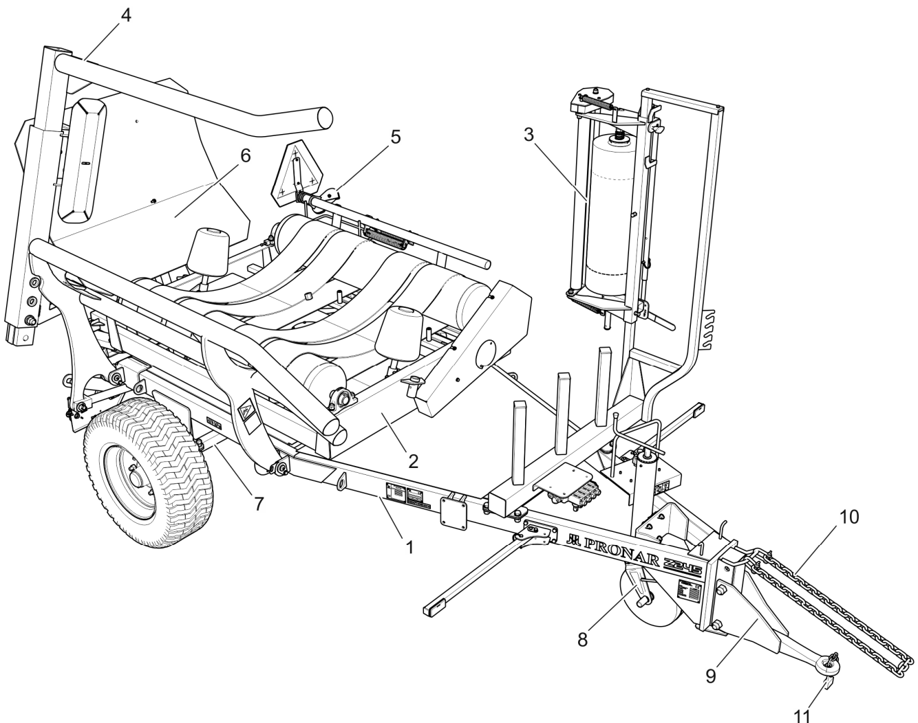
RYСУNEK 3.1 Budowa owijarki PRONAR Z245
