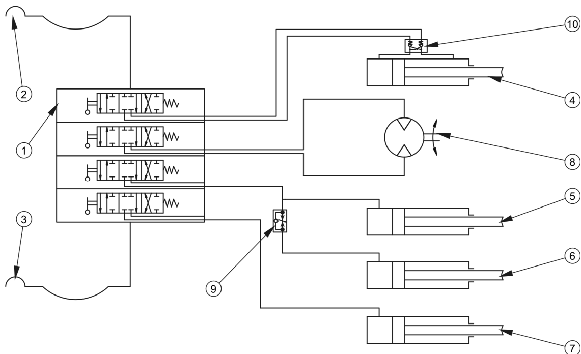
RYSUNEK 3.12 Schemat instalacji hydraulicznej ze sterowaniem mechanicznym
