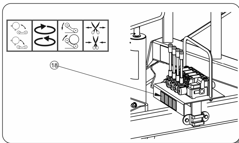
RYSUNEK 2.5 Rozmieszczenie naklejek informacyjnych i ostrzegawczych, widok z tyłu
