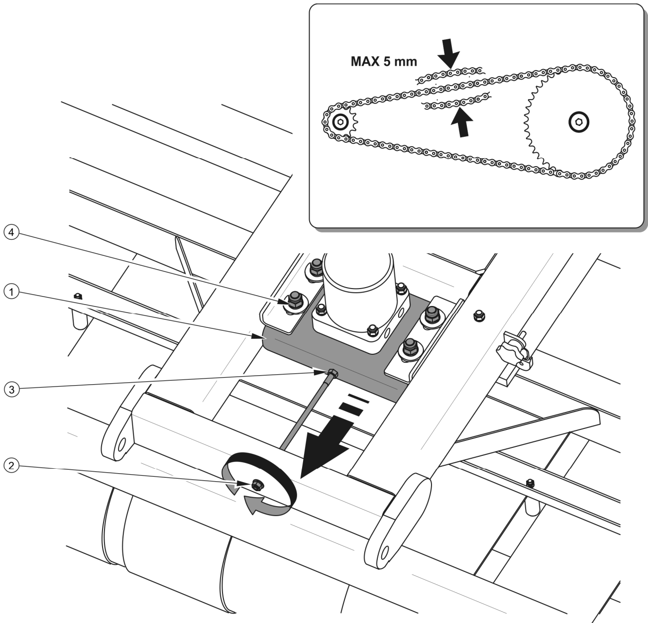
RYSUNEK 5.5 Regulacja łańcuch napędu stołu obrotowego.
