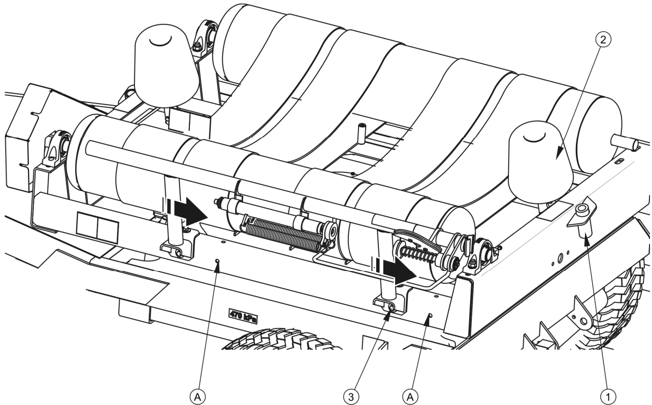
RYSUNEK 5.10 Dostosowanie elementów stołu obrotowego
