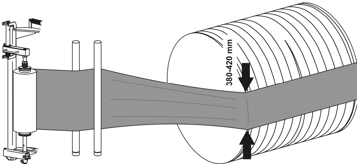
RYСУNEK 5.20 Metoda 1 kontroli napięcia folii
