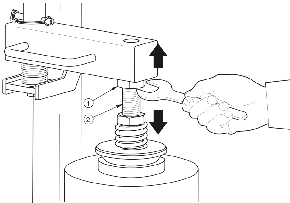
RYSUNEK 5.22 Regulacja napięcia
