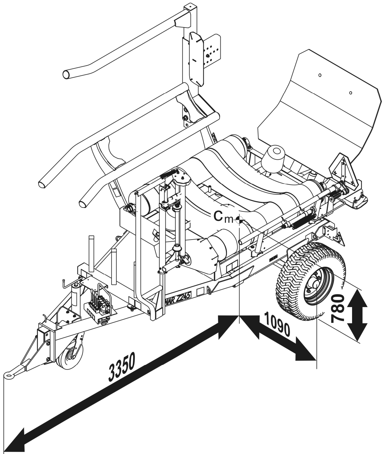
RYСУNEK 1.7 Położenie środka ciężkości owijarki przygotowanej do transportu
