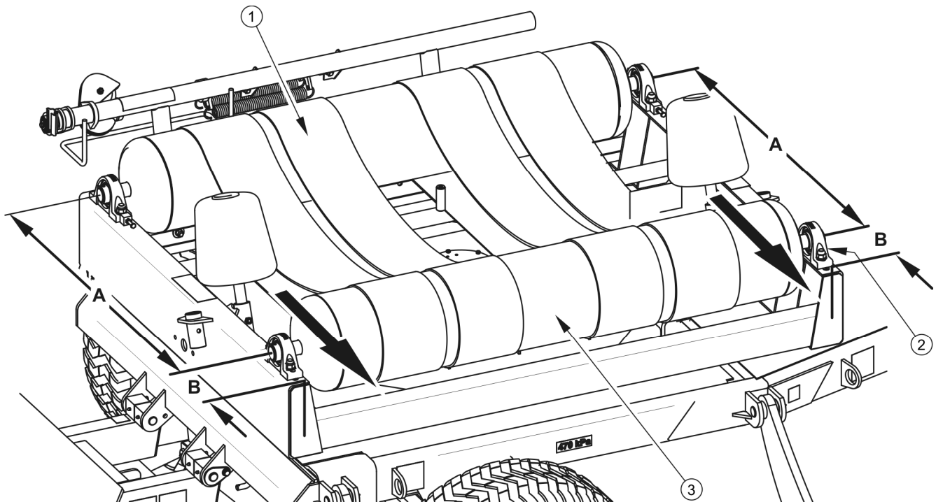
RYСУNEK 5.15 Regulacja napięcia pasów
