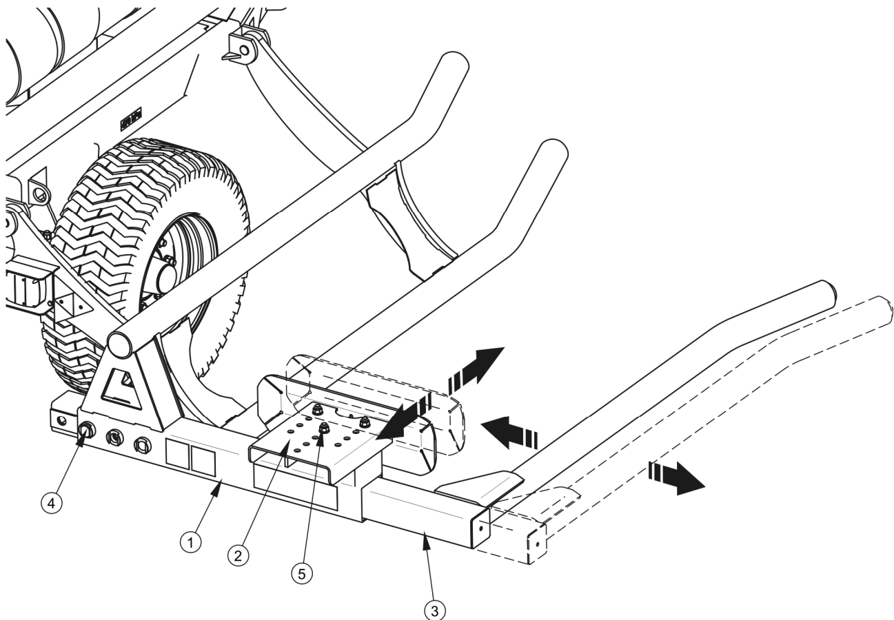
RYСУNEK 5.11 Regulacja ramienia załadowczego
