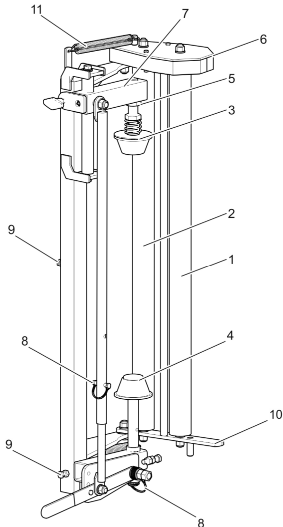
RYSUNEK 3.2 Budowa podajnika folii
