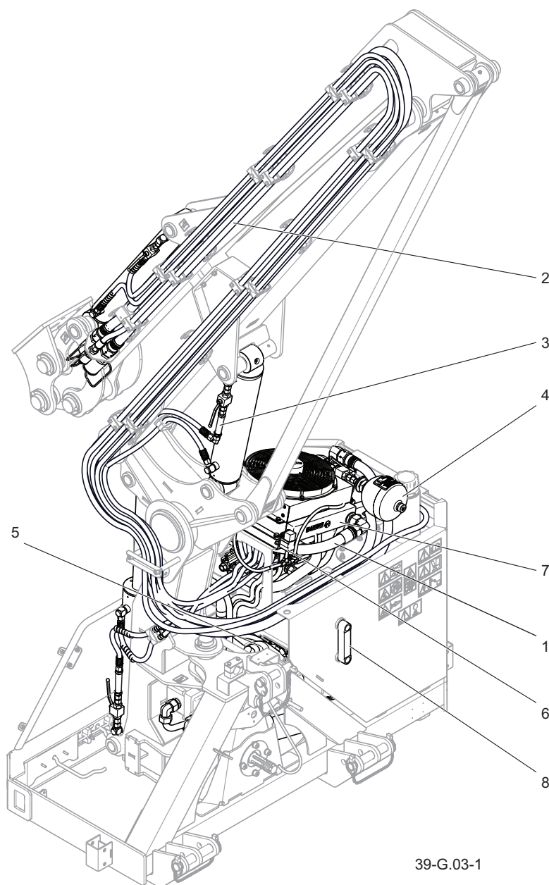
Rysunek 3.3 Budowa układu hydraulicznego
