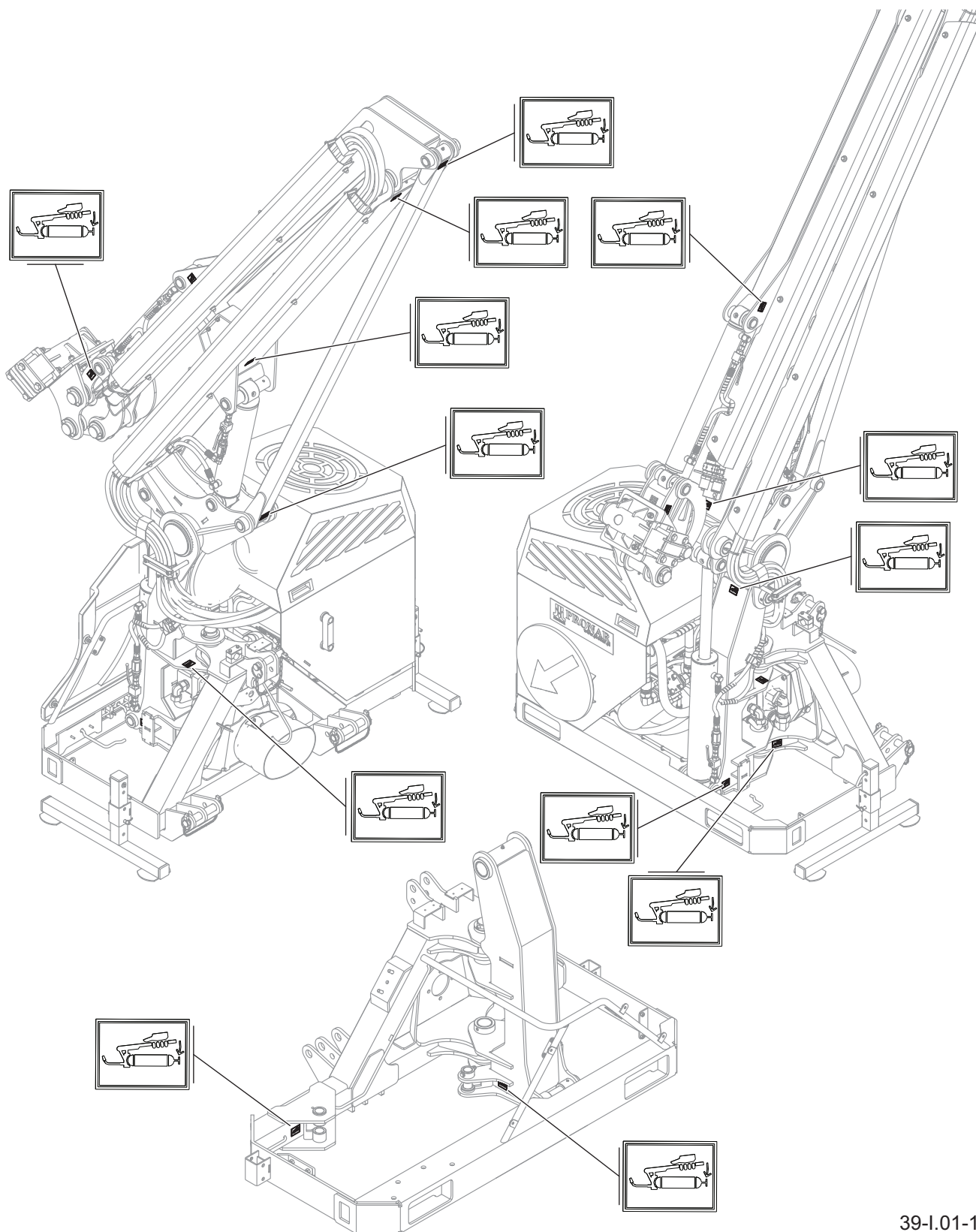
Rysunek 5.5 Położenie piktoqramów punktów smarowania
