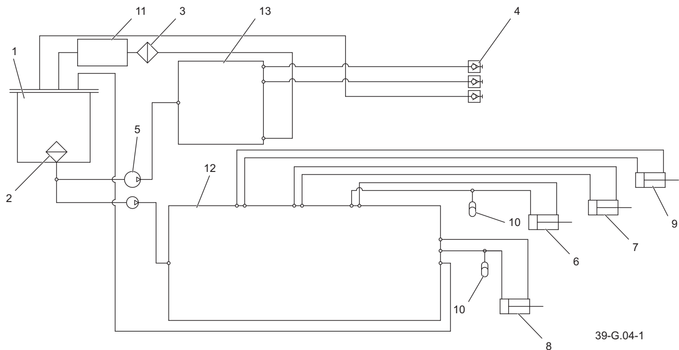
Rysunek 3.4 Schemat instalacji hydraulicznej wsięgnika wielofunkcyjnego WWT600P
