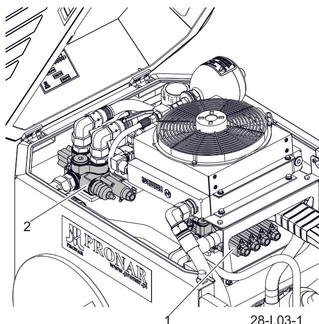
Rysunek 5.3 Rozdzielacza hydrauliczne WWT600P
