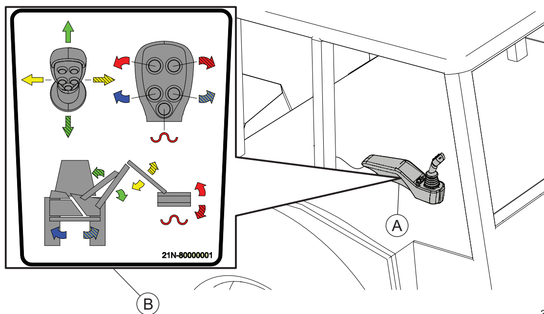
Rysunek 4.4 Układ sterowania wysięgnika wewnątrz kabiny nośnika narzędzi (ciągnika) wraz z piktogramem.
