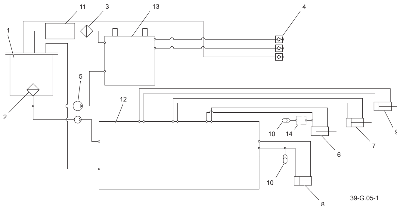
Rysunek 3.5 Schemat instalacji hydraulicznej wyciągnika wielofunkcyjnego WWT604P
