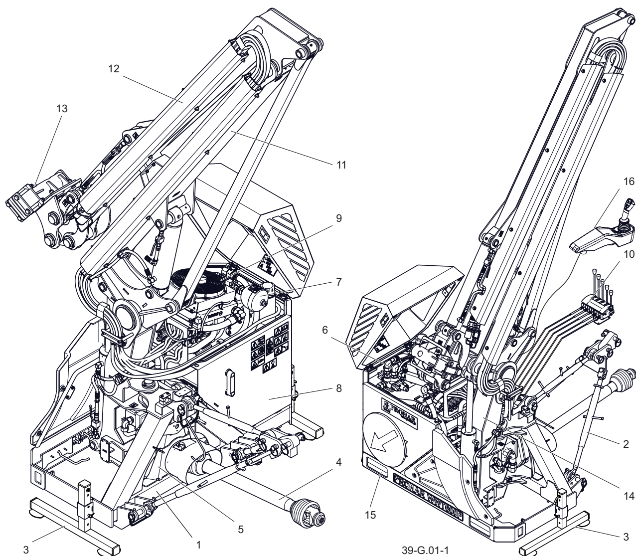
Rysunek 3.2 Budowa wysięgnika
