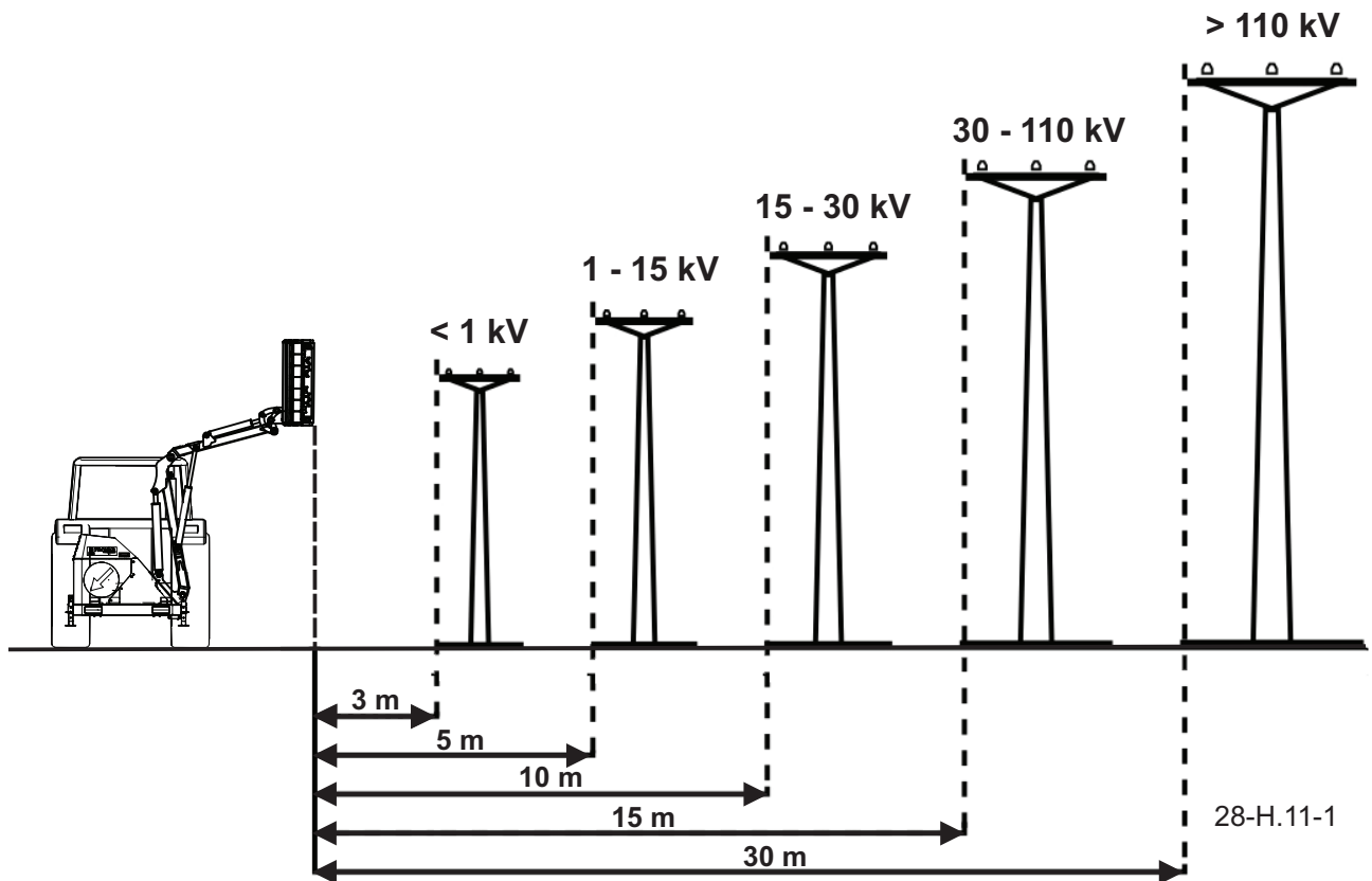
Rysunek 4.13 Bezpieczne odległości maszyny od linii elektroenergetycznych.
