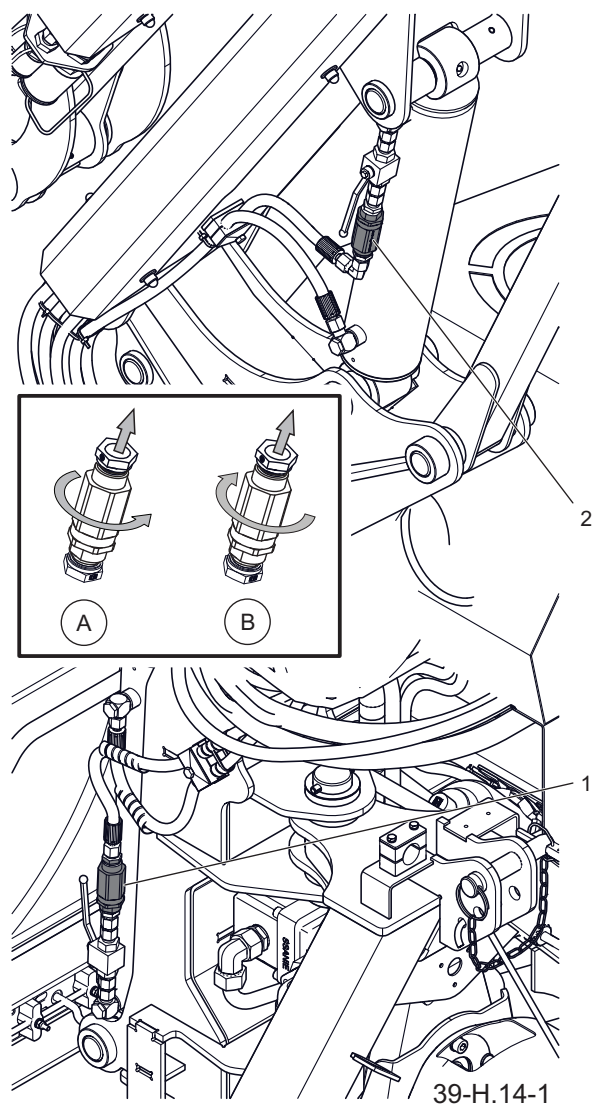
Rysunek 4.16 Zawory dławiąco-zwrotne siłowników wychyłu ramion.
