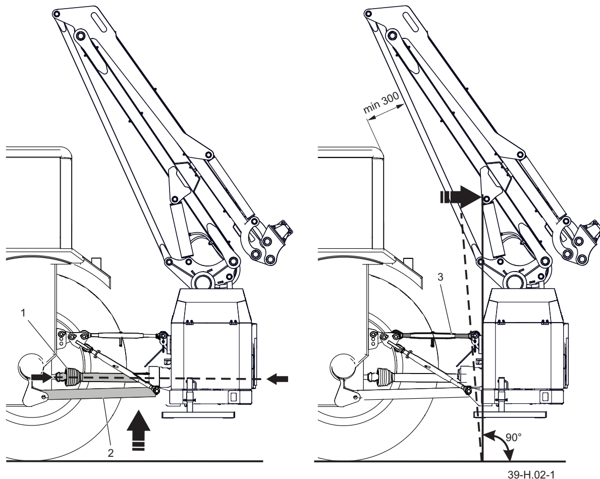
Rysunek 4.2 Sposób ustawienia wyciągnika wielofunkcyjnego względem podłoża (1) wał napędowy (2) cięgła dolne tylnego TUZ (3) łącznik centralny
