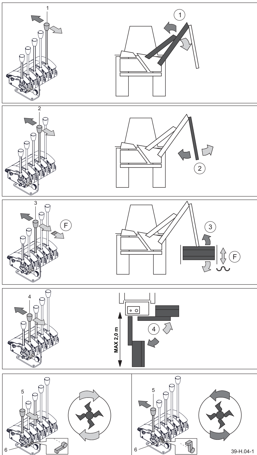
Rysunek 4.6 Sposób ustawienia wysięgnika wielofunkcyjnego względem podłoża
