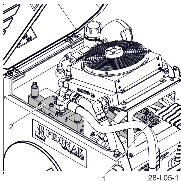
Rysunek 5.4 Rozdzielacza hydrauliczne WWT604P
