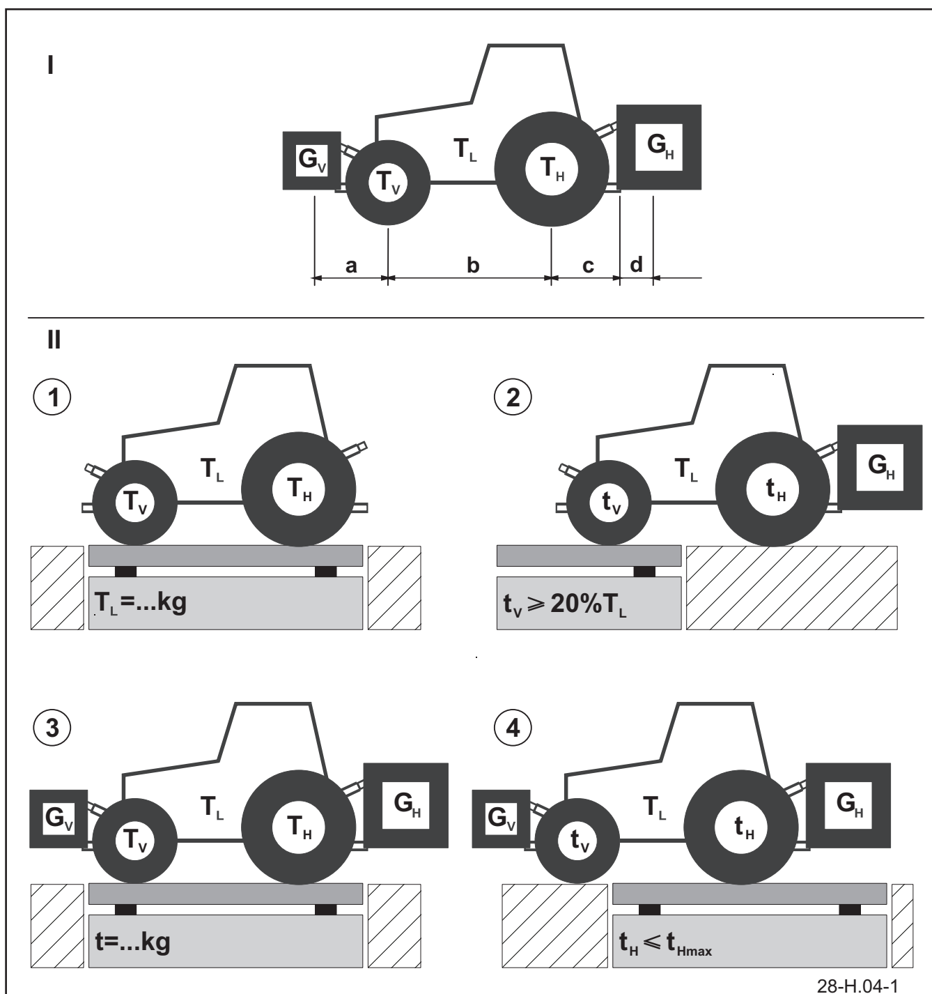
Rysunek 4.5 Dociążenie przedniej osi nośnika narzędzi (ciągnika).
