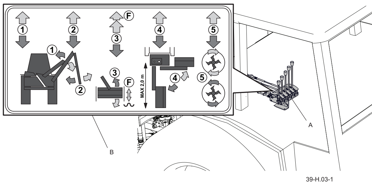
Rysunek 4.3 Układ sterowania wysięgnika wewnątrz kabiny nośnika narzędzi (ciągnika) wraz z piktogramem.
