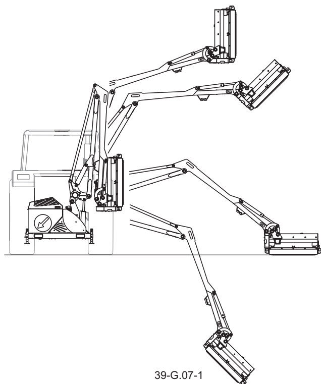
Rysunek 4.11 Przykładowe pozycje robocze wysięgnika wielofunkcyjnego z głowicą koszącą GK110.
