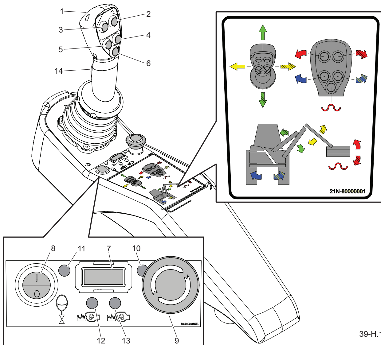
Rysunek 4.7 Sposób sterowania wsięgnikiem wielofunkcyjnym WWT604P
