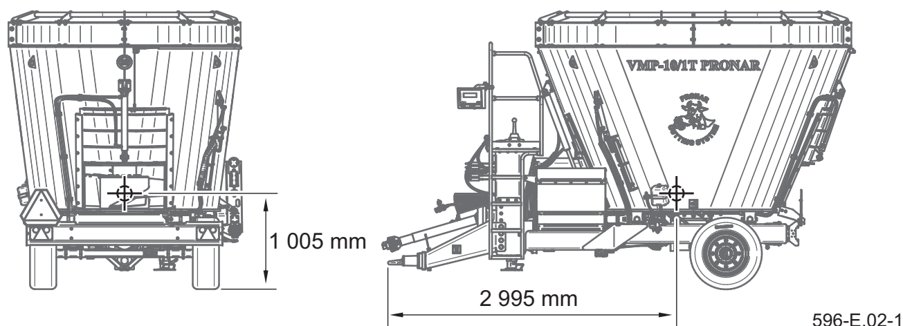
Rysunek 1.2 Położenie środka ciężkości
