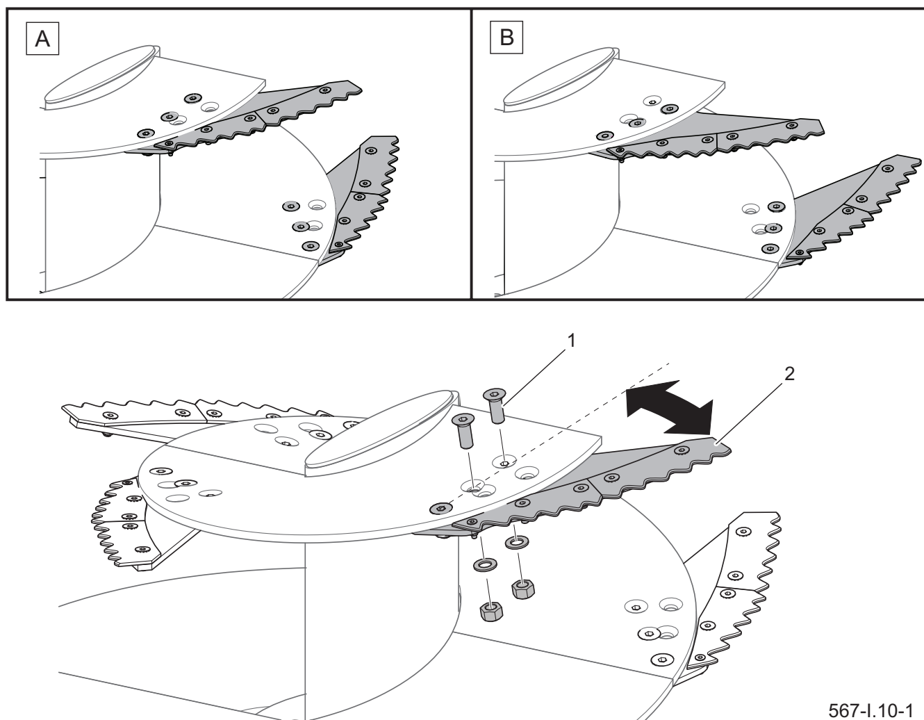
Rysunek 5.10 Regulacja położenia noży tnących
