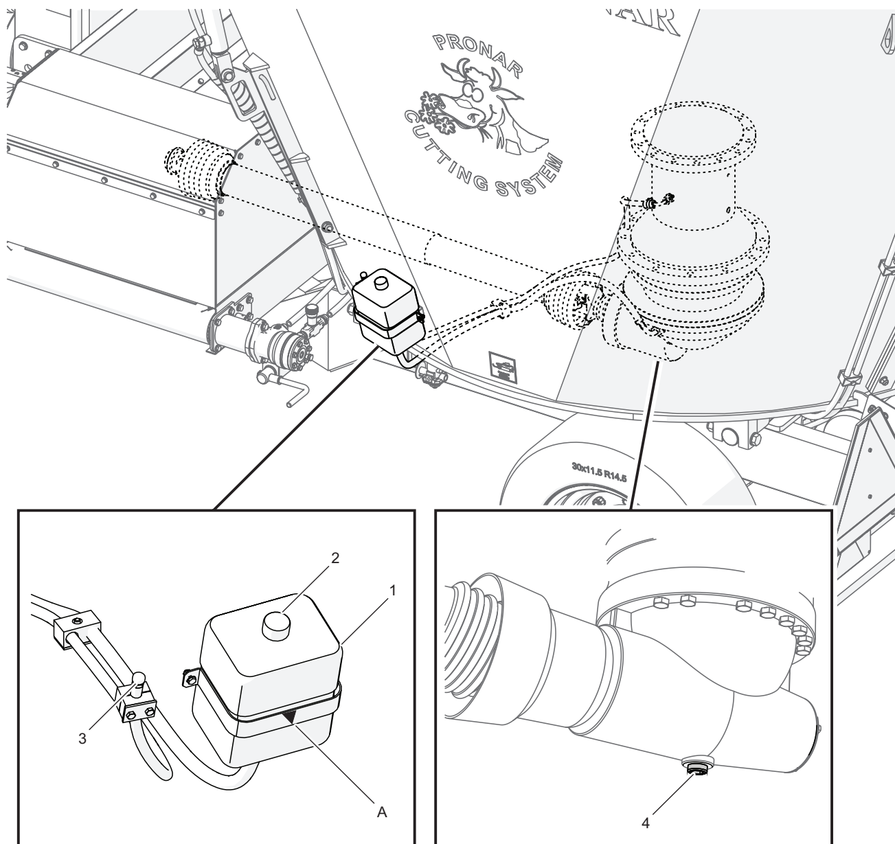
Rysunek 5.6 Wymiana oleju w przekładni planetarnej
