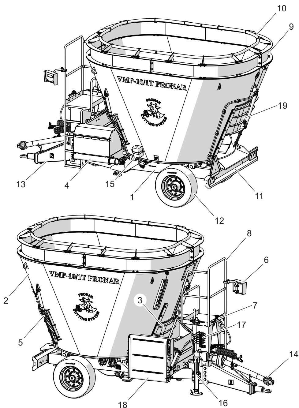
Rysunek 3.1 Budowa ogólna
