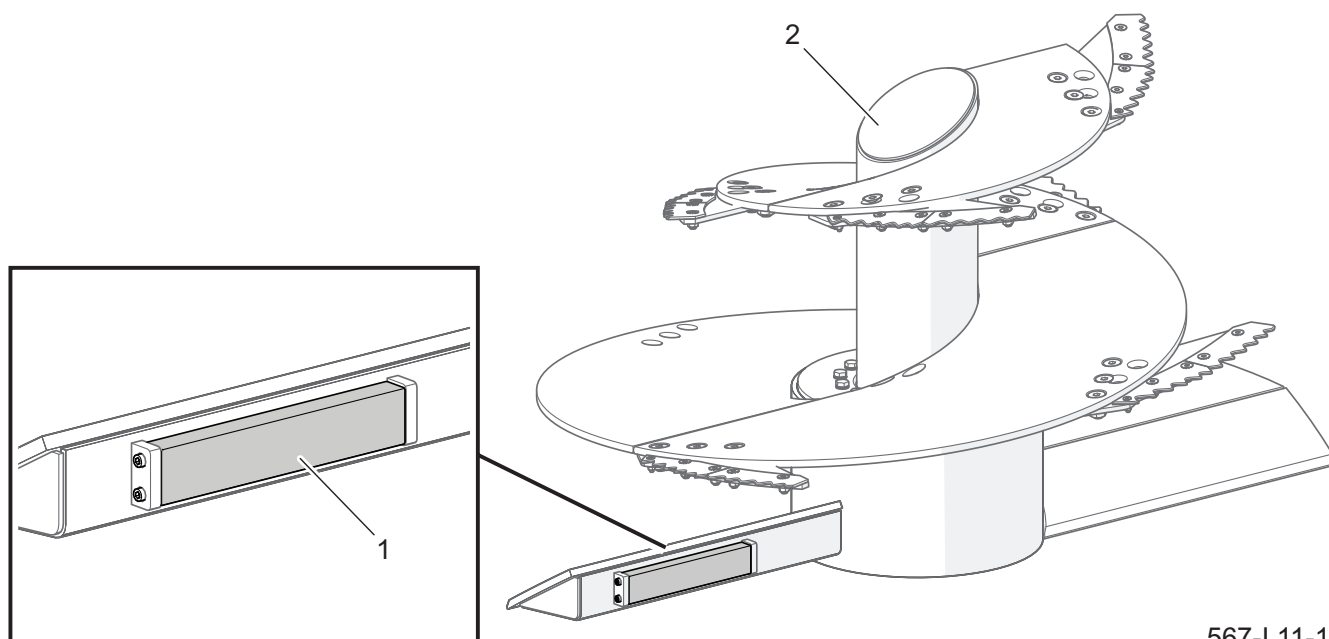
Rysunek 5.12 Magnesy mieszadeł ślimakowych (1) magnes neodymowy (2) mieszadło ślimakowe
