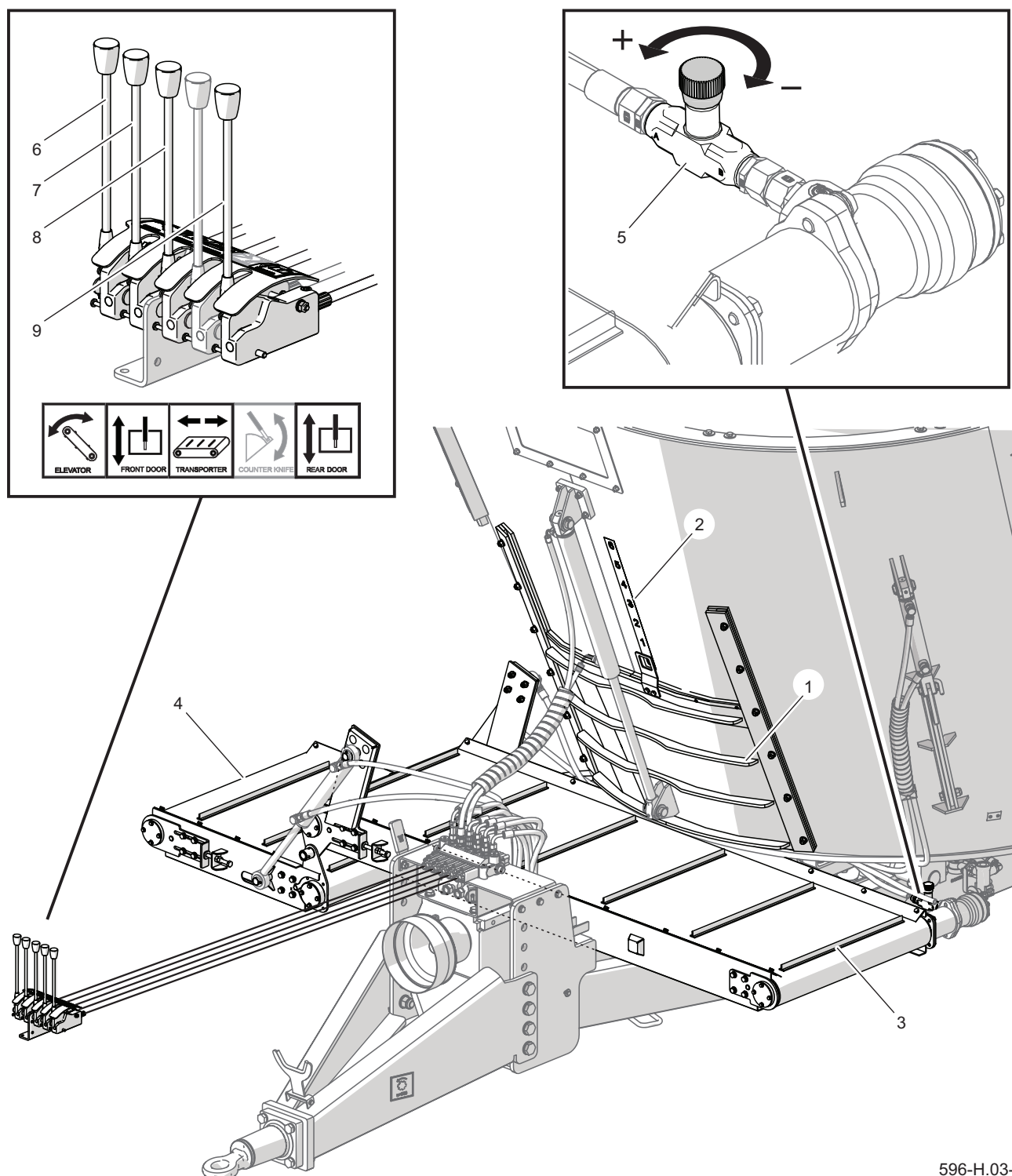
Rysunek 4.3 Wyładunek mieszanki paszowej
