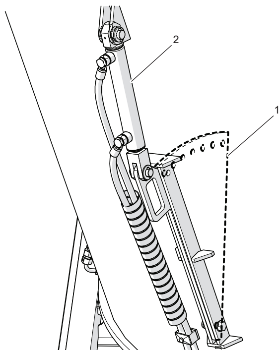
Rysunek 4.5 Przeciwnoże regulowane hydraulicznie (opcja)
