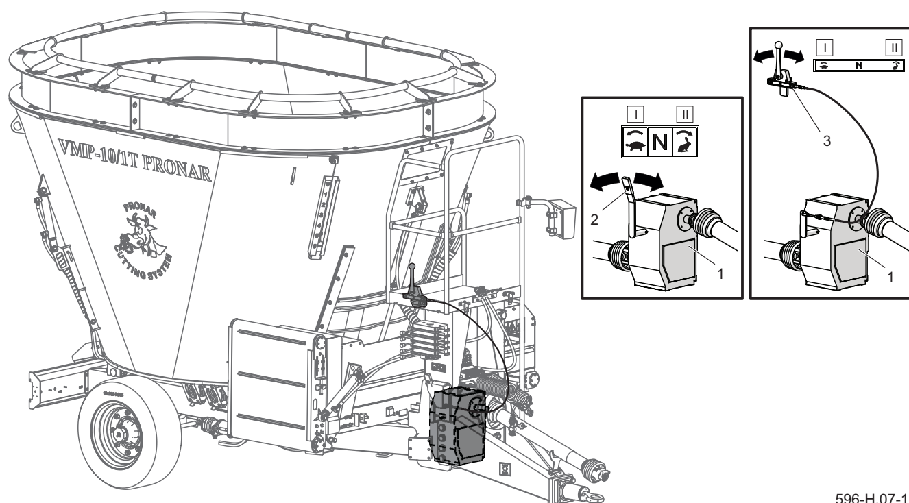
Rysunek 4.6 Zmiana prędkości napędu mieszadeł ślimakowych
