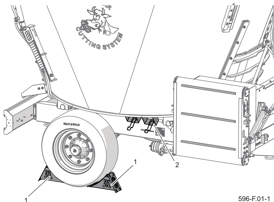
Rysunek 2.1 Sposób ustawienia klinów do kół (1) klin (2) kieszeń klina
