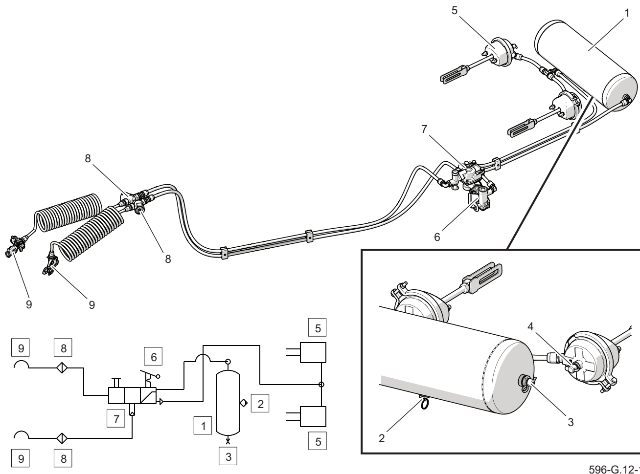
Rysunek 3.13 Instalacja hamulcowa pneumatyczna dwuprzewodowa (wyposażenie dodatkowe)
