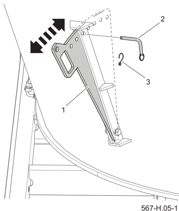
Rysunek 4.4 Przeciwnoże mechanicznie regulowane (1) przeciwnóż ustalający (2) sworzeń (3) zawleczka
