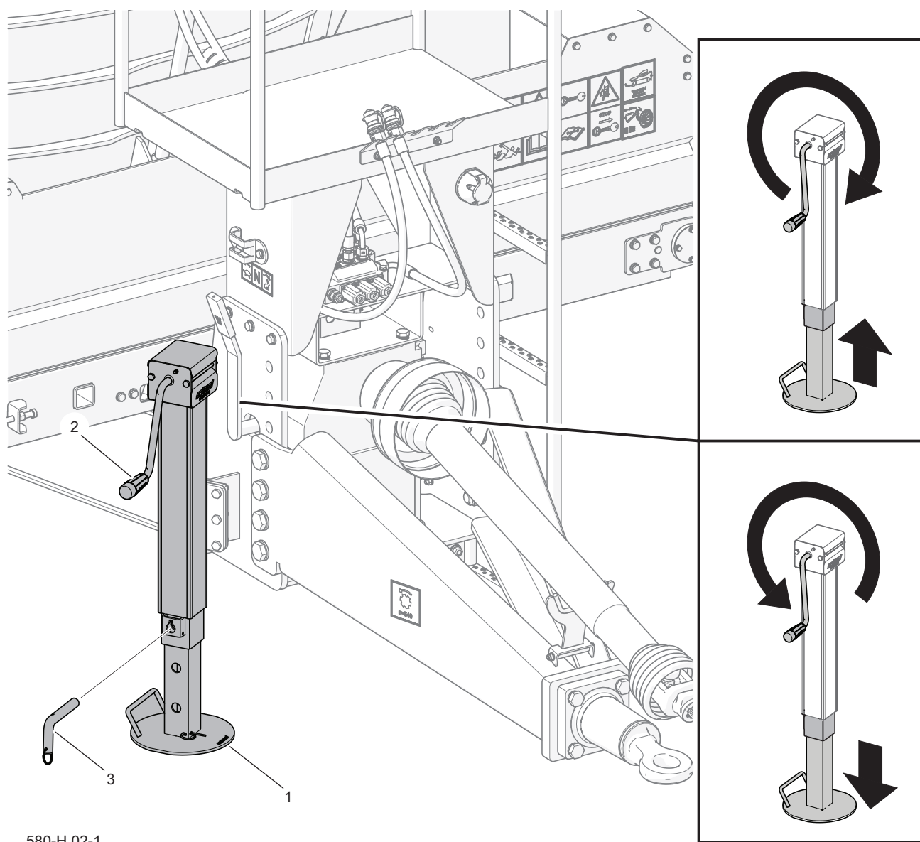
Rysunek 4.2 Podpora postojowa
