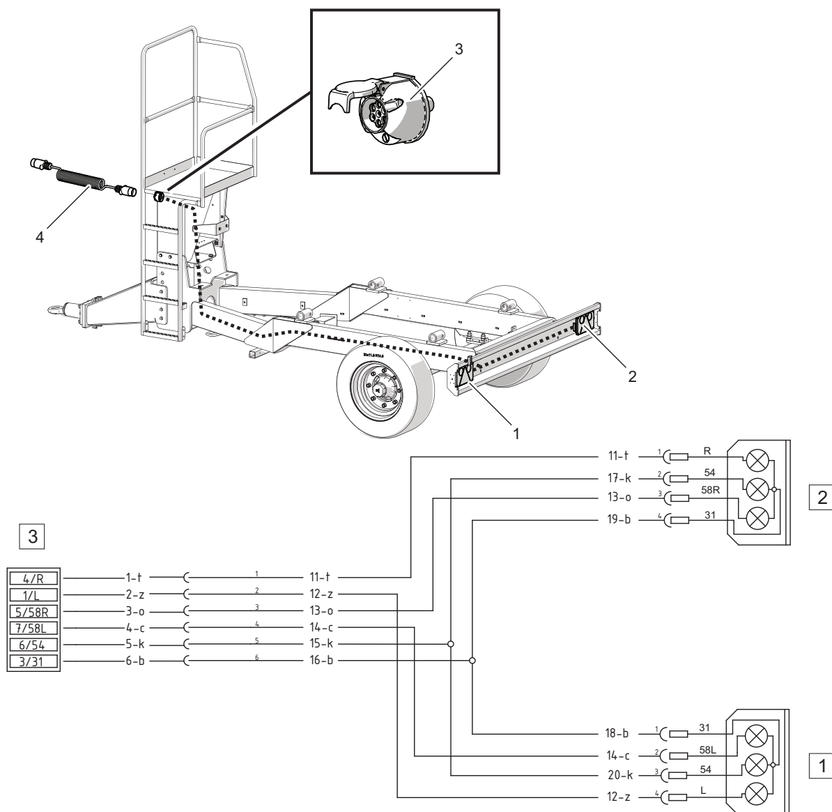
Rysunek 3.11 Instalacja elektryczna oświetleniowa (wyposażenie dodatkowe)
