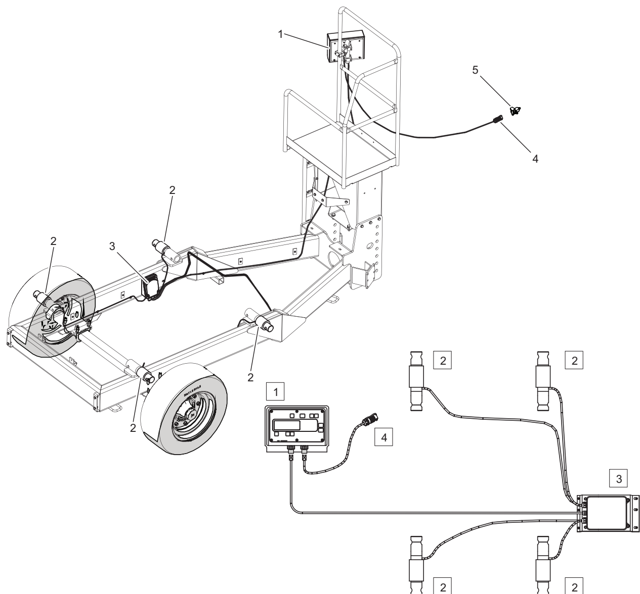
Rysunek 3.10 Układ ważenia
