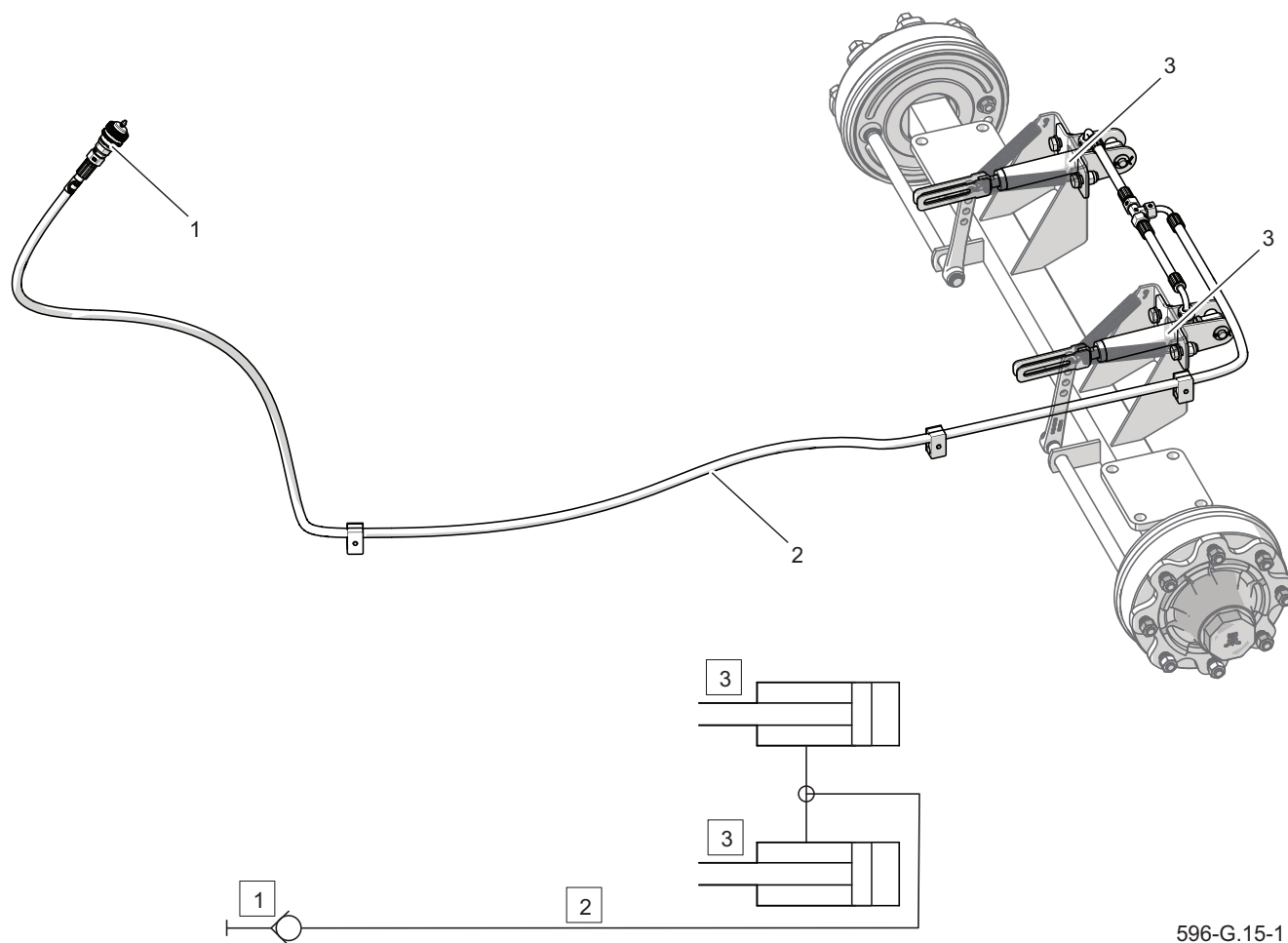
Rysunek 3.15 Instalacja hamulcowa hydrauliczna (wyposażenie dodatkowe)
