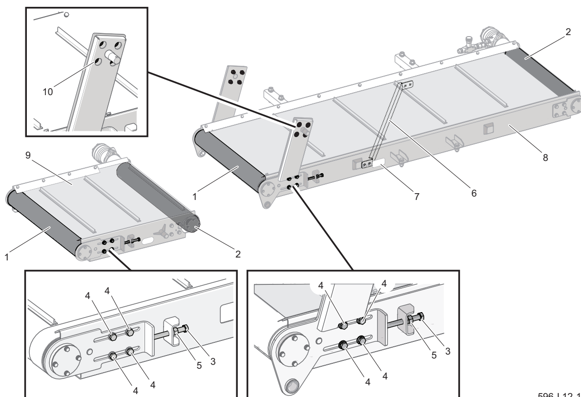
Rysunek 5.11 Regulacja taśmy przenośnika
