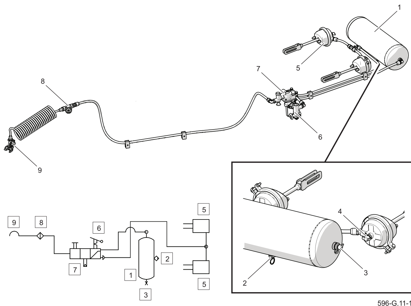
Rysunek 3.12 Instalacja hamulcowa pneumatyczna jedнопrzewodowa (wyposażenie dodatkowe)
