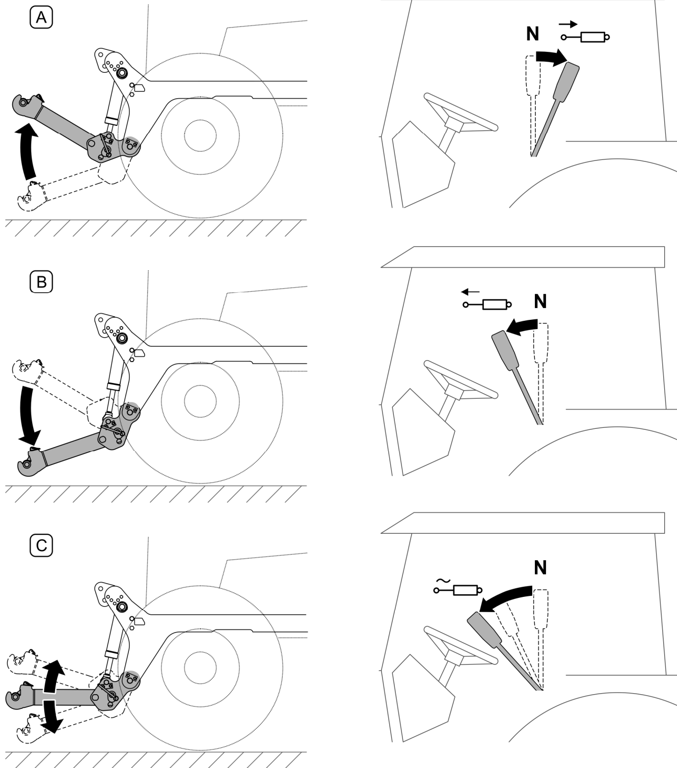
RYСУNEK 4.17 Sterowanie ramionami przedniego TUZ
