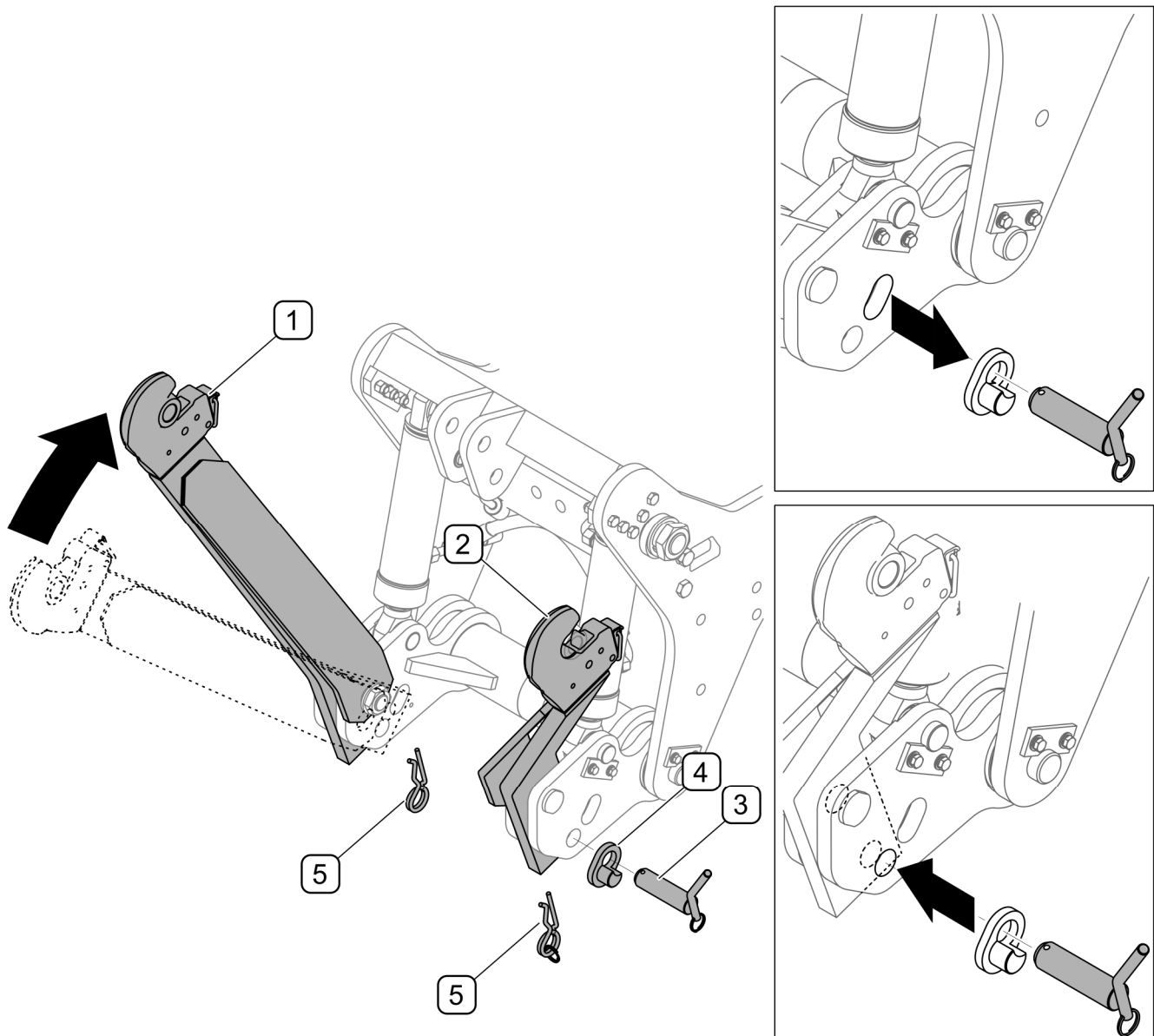
RYSUNEK 4.18 Ustawienie cięgieł do pozycji transportowej
