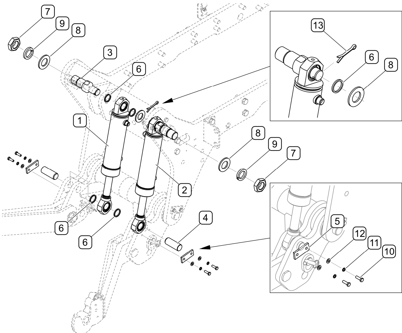
RYСУNEK 4.8 Montaż siłowników hydraulicznych
