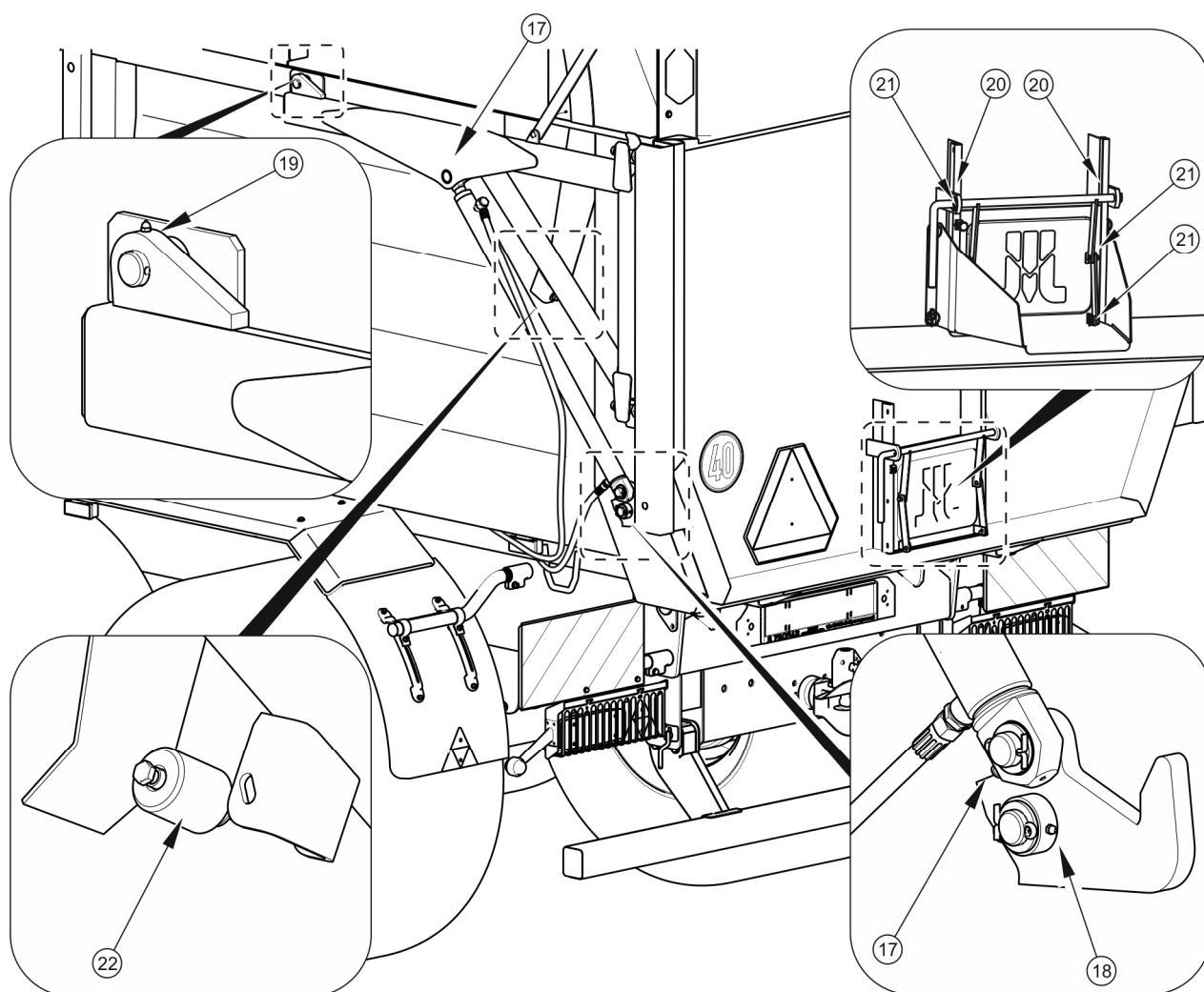
RYSUNEK 5.12 Punkty smarne przyczepek
