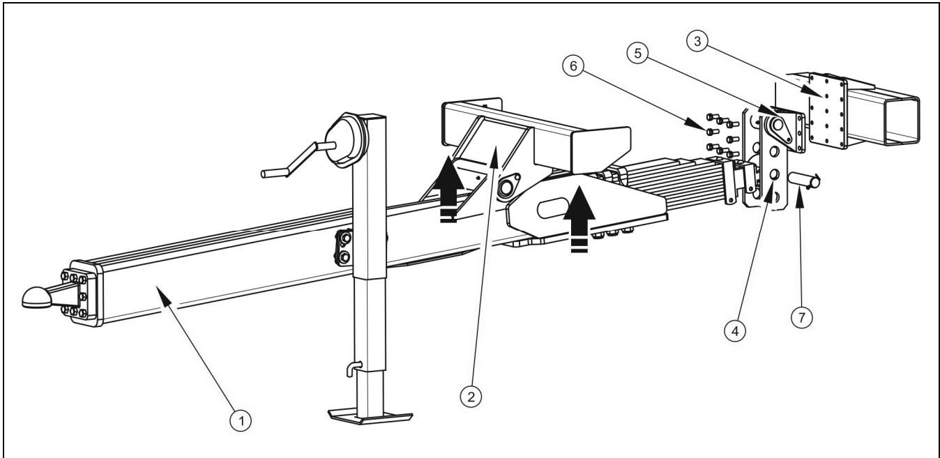
RYSUNEK 5.14 Ustawienie wysokości dyszla
