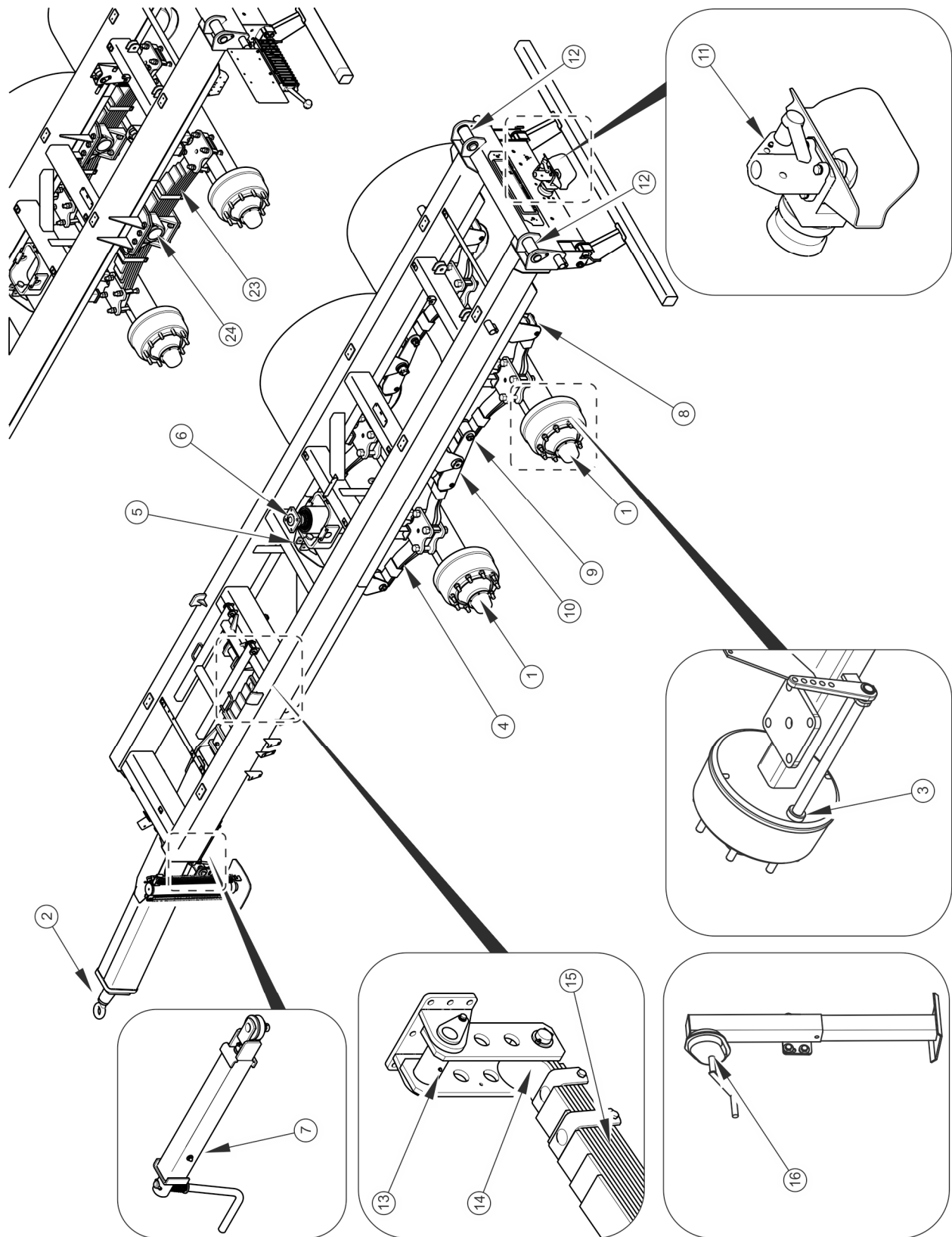
RYSUNEK 5.11 Punkty smarne przyczepty
