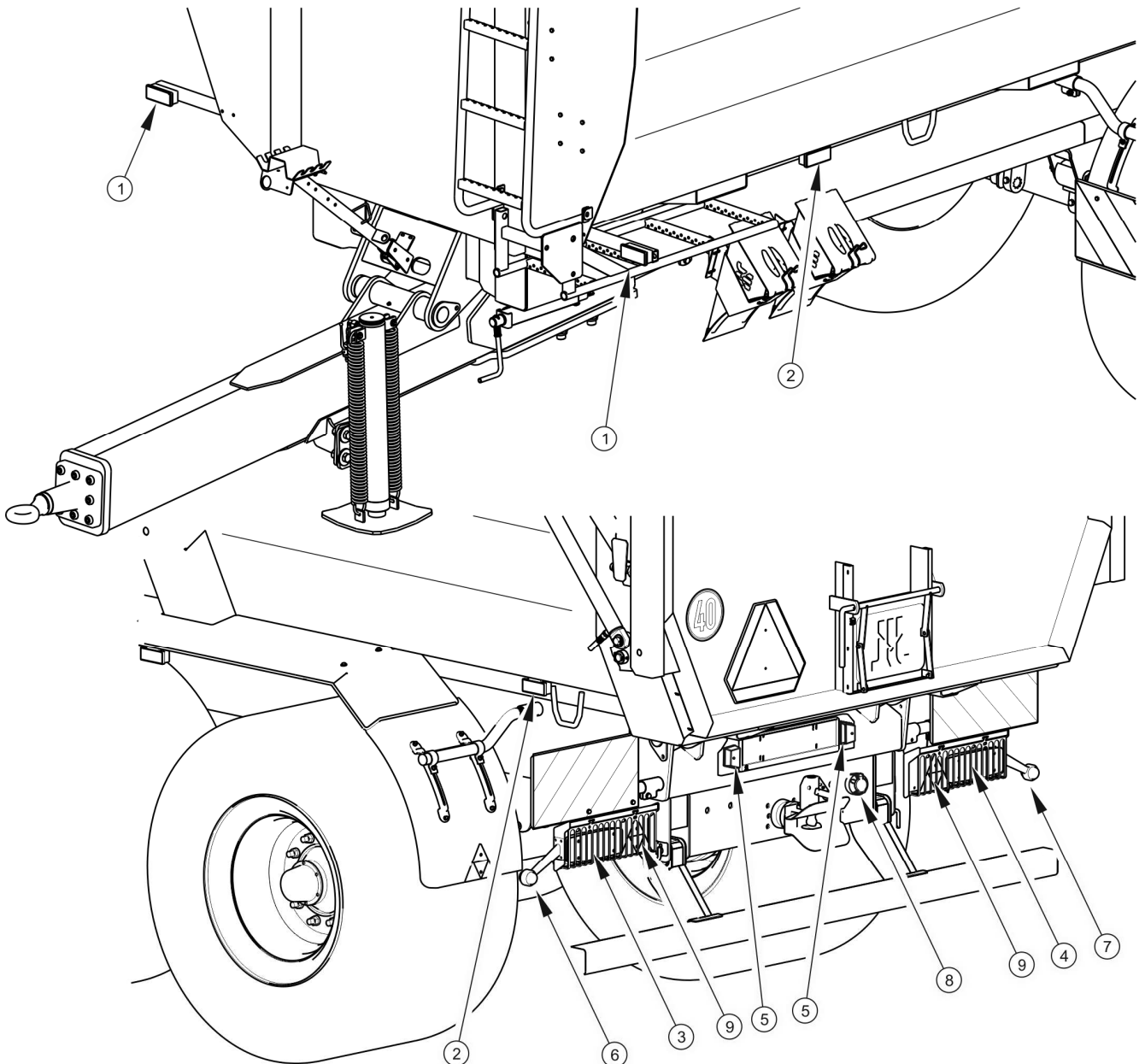
RYSUNEK 3.14 Rozmieszczenie elementów elektrycznych i odblaskowych
