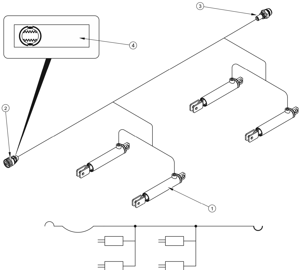
RYСУNEK 3.6 Budowa i schemat instalacji hamulcowej hydraulicznej
