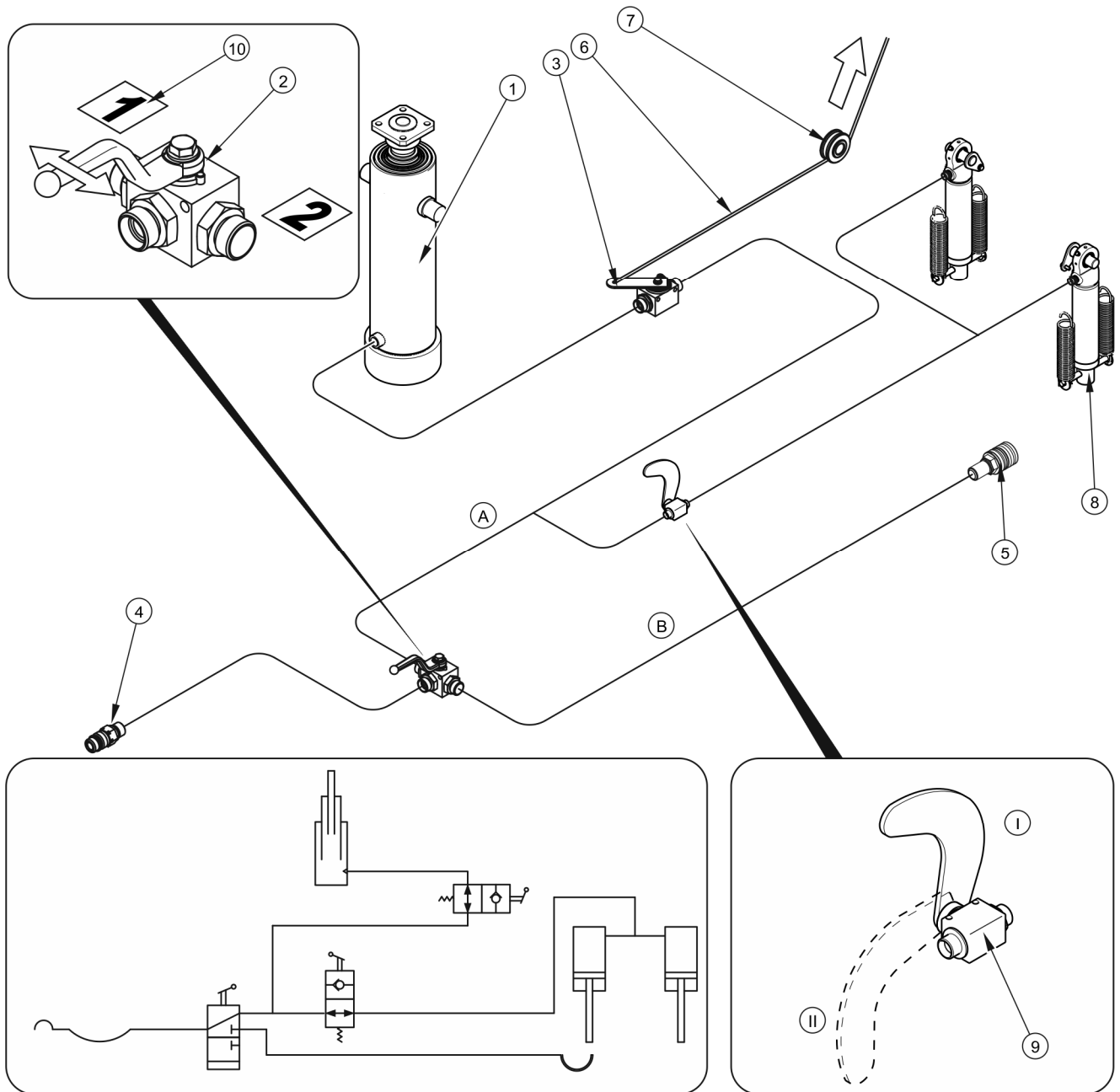
RYSUNEK 3.9 Budowa i schemat instalacji hydraulicznej wyrotu bogie
