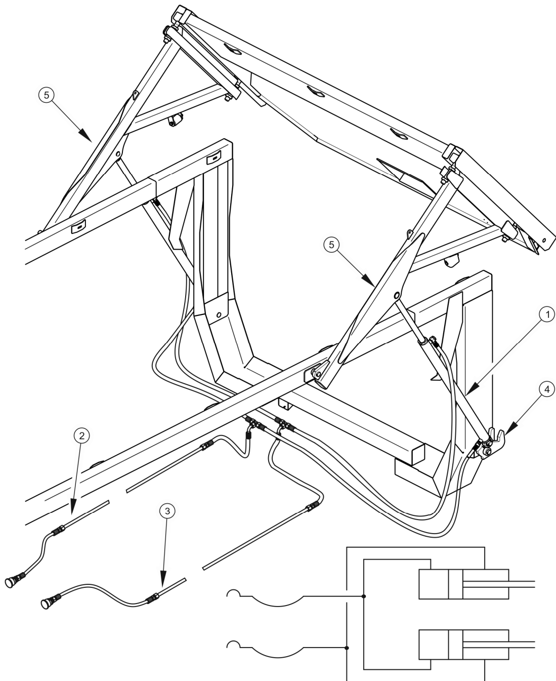
RYSunEK 3.12 Budowa i schemat instalacji hydraulicznej kłapy tylnej
