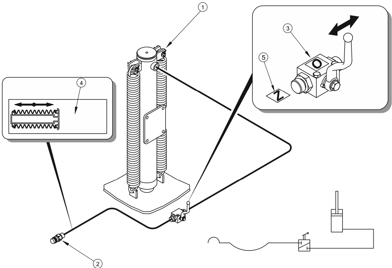
RYСУNEK 3.10 Budowa i schemat instalacji hydraulicznej podpory prostej
