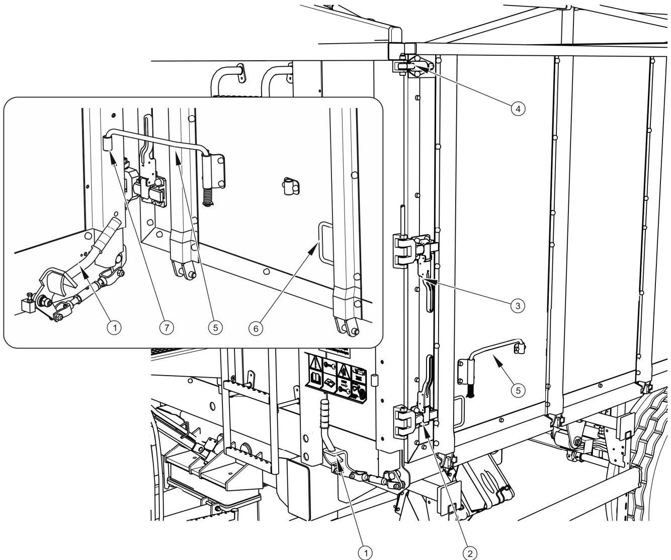
RYSUNEK 4.4 Otwieranie lewej ściany portalowej skrzyni ładunkowej
