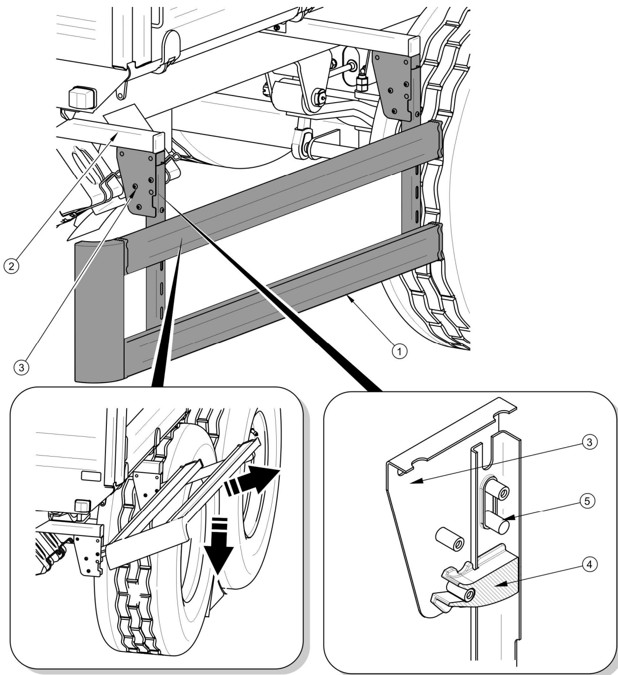
RYSUNEK 4.8 Ośłona przeciwnajazdowa lewa
