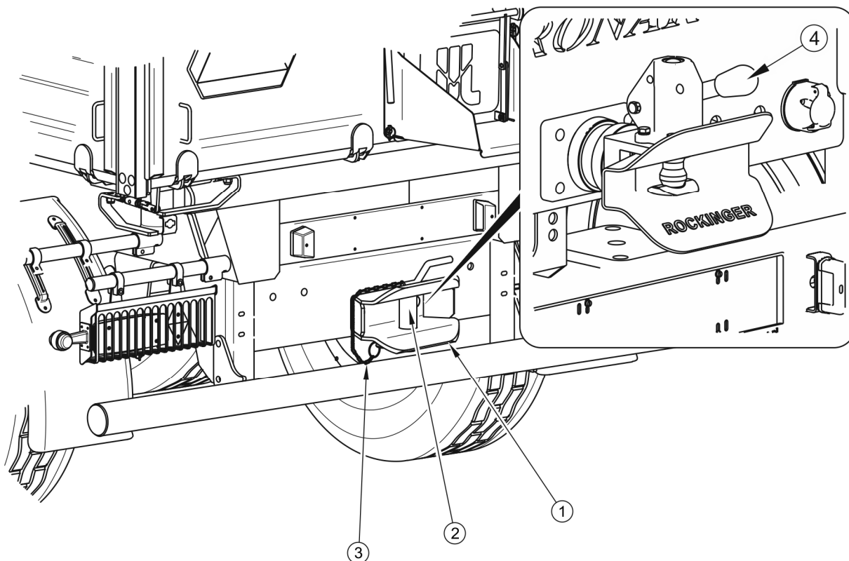
RYSUNEK 4.2 Zaczep tylny
