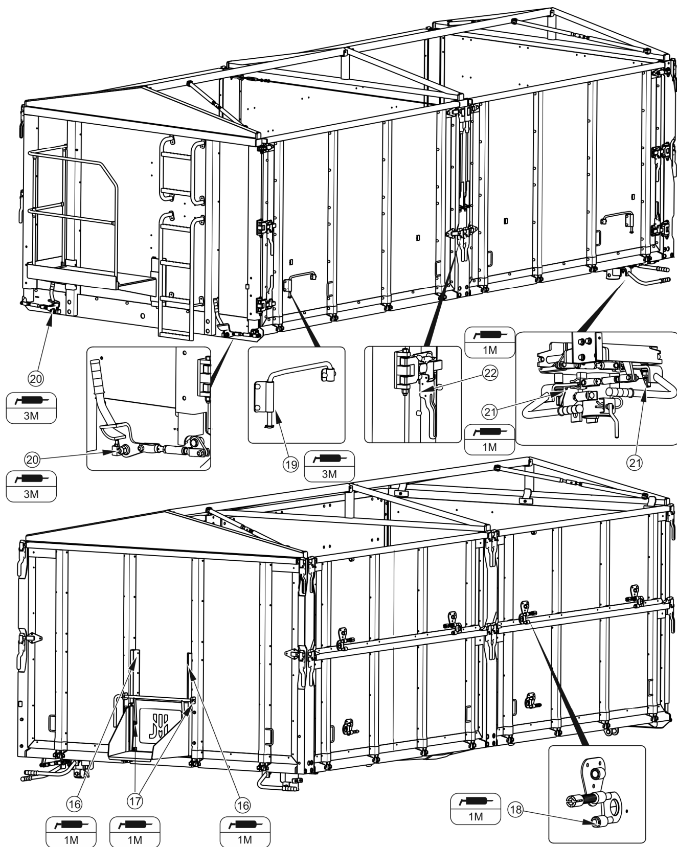
RYSUNEK 5.13 Punkty smarne przyczepy, część 2
