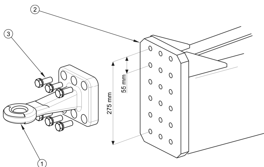
RYСУNEK 5.15 Regulacja położenia cięgna dyszla
