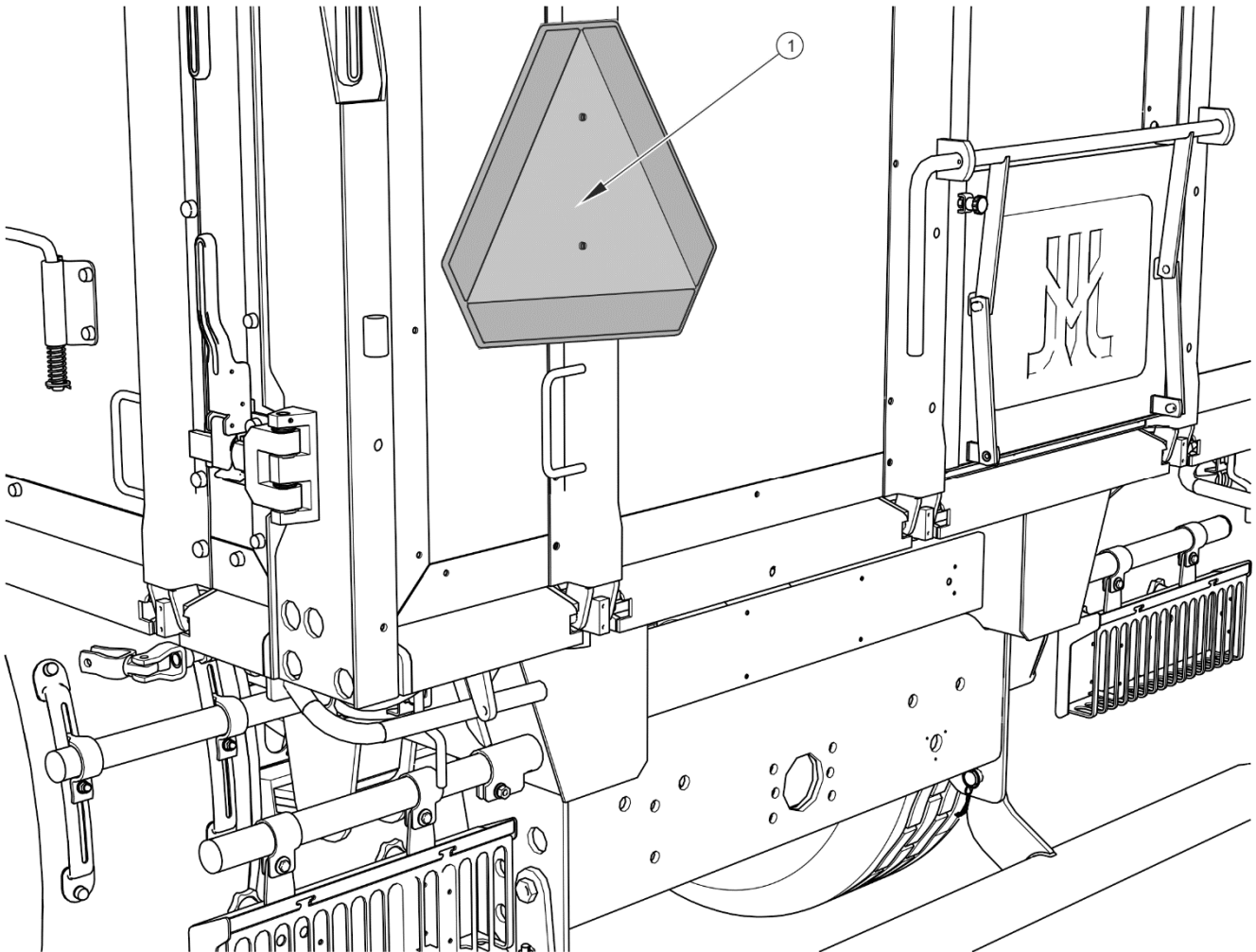
FIGURE 2.2 Lieu de montage de la plaque distinctive véhicules lents
