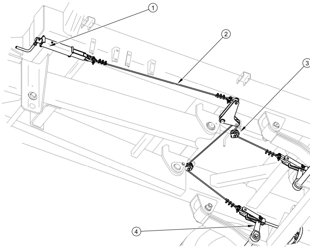
FIGURE 3.11 Construction du frein de stationnement
