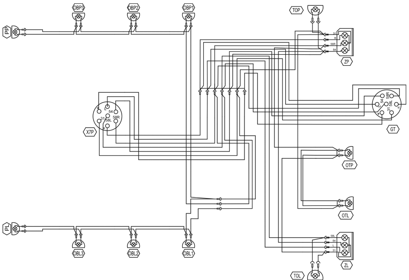
FIGURE 3.12 Schéma de principe de l'installation électrique
