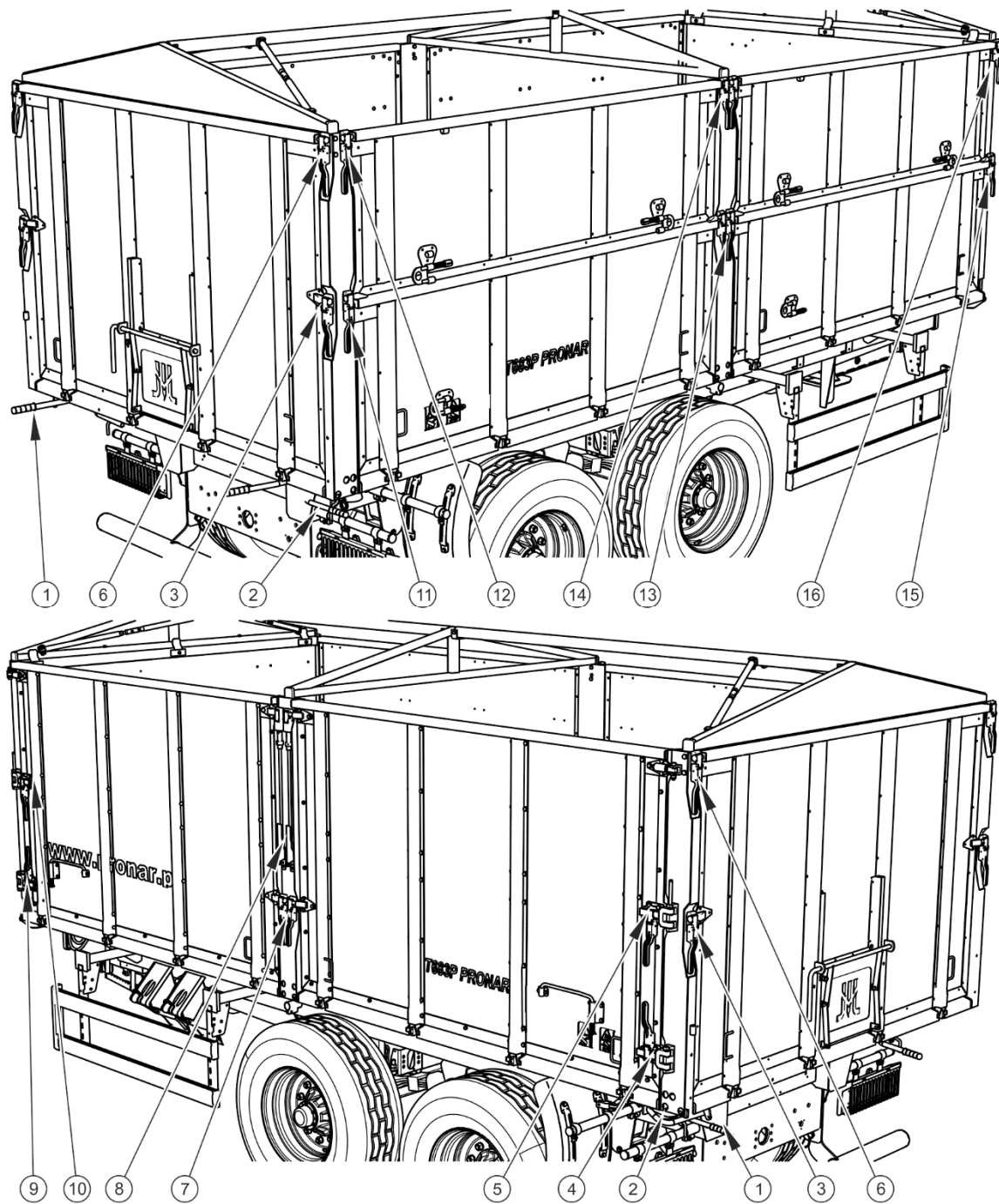
FIGURE 4.5 Emplacement des serrures et verrous des parois de la remorque
