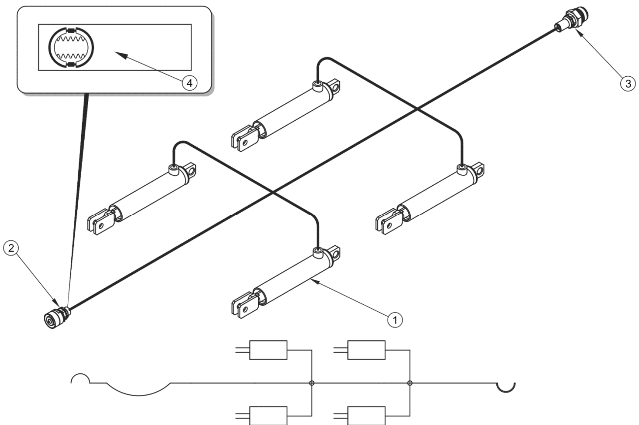
FIGURE 3.7 Construction et schéma du système de freinage hydraulique
