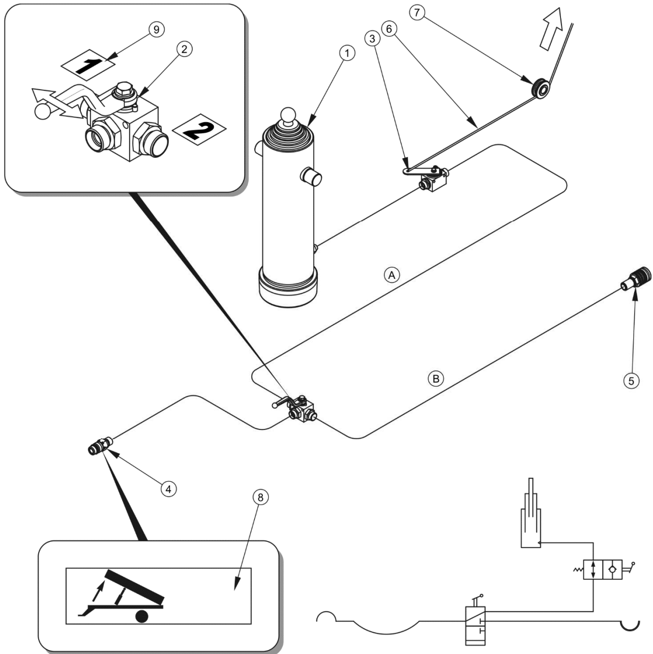
FIGURE 3.9 Construction et schéma de l'installation hydraulique du dispositif de basculement
