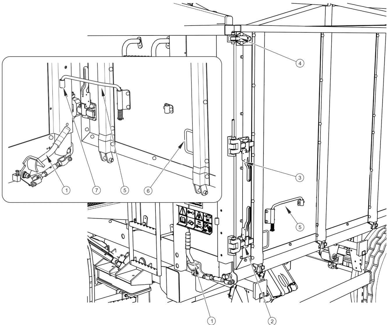
FIGURE 4.4 Ouverture de la paroi à portail gauche de la benne
