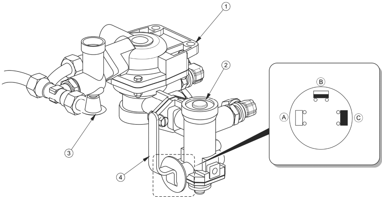
FIGURE 3.8 Vanne de commande et régulateur de la force de freinage
