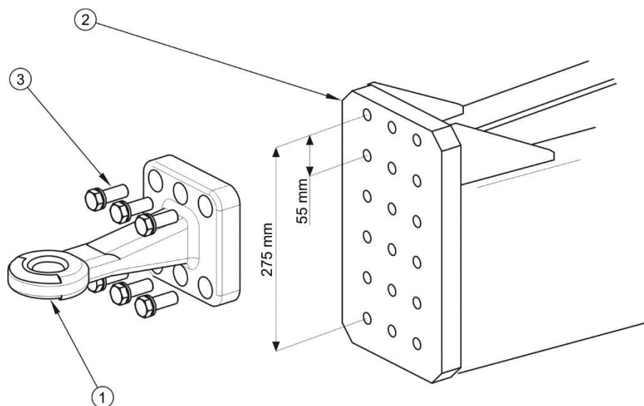
FIGURE 5.15 Réglage de la position de l'anneau d'attelage du timon
