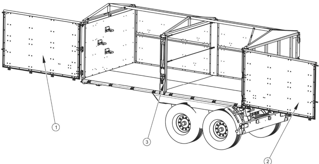
FIGURE 4.6 Ouverture des parois portails (côté gauche)
