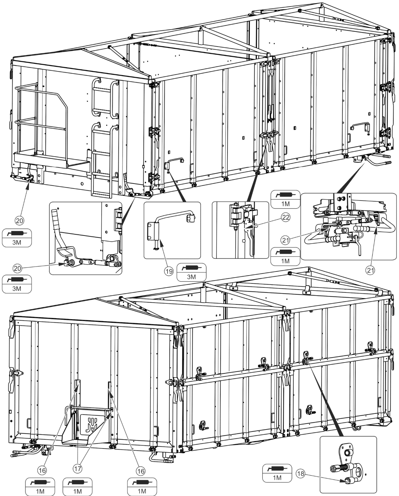
FIGURE 5.13 Points de lubrification de la remorque, partie 2
