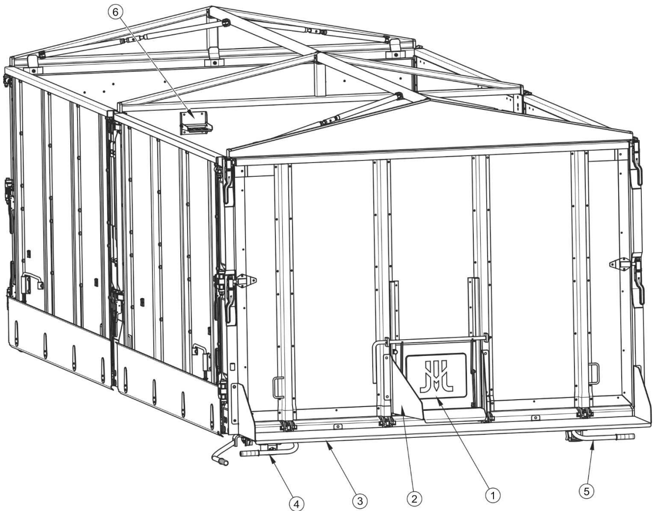
FIGURE 3.3 Paroi arrière de la benne
