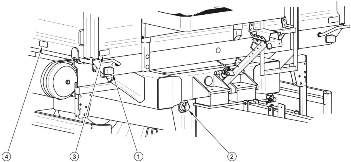
FIGURE 3.14 Emplacement des éléments de l'installation électrique et des réflecteurs – vue avant
