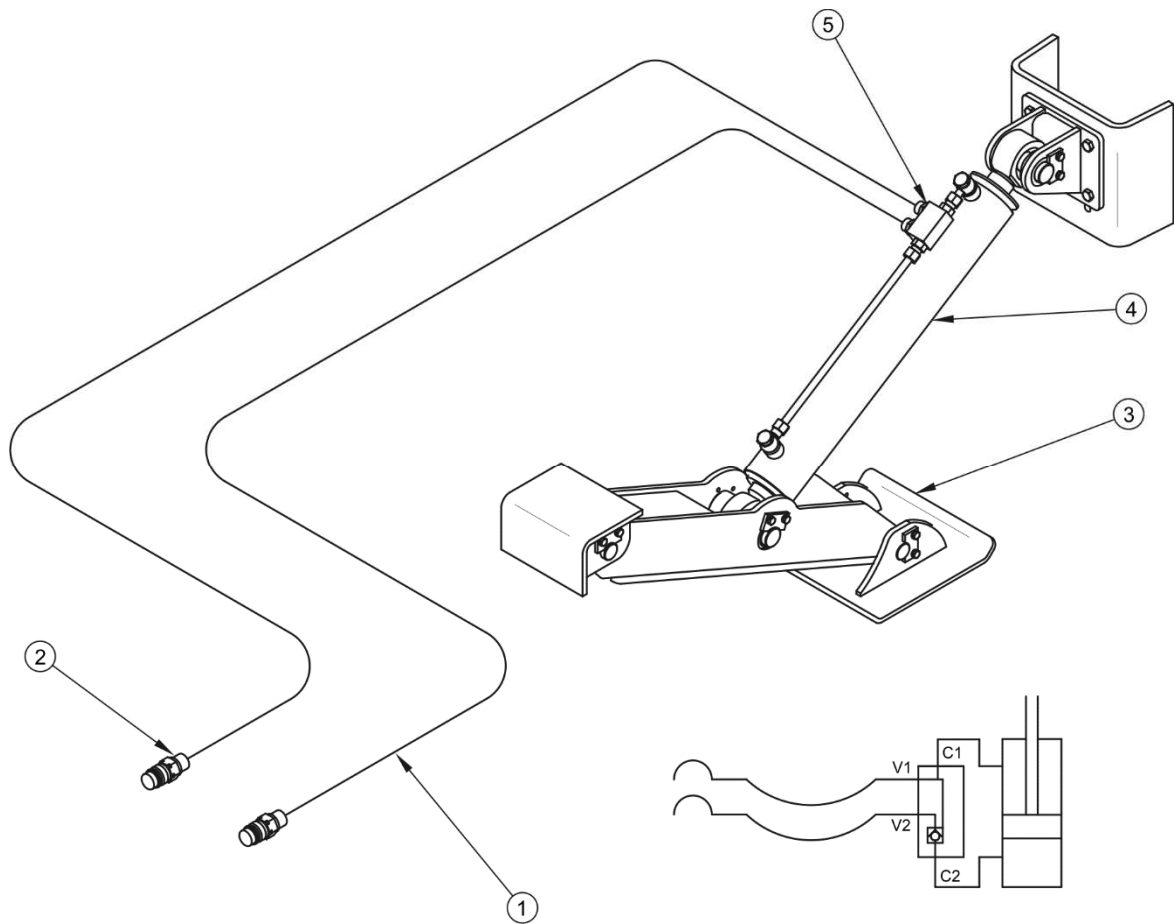
FIGURE 3.10 Construction et schéma de l'installation hydraulique de la béquille ciseaux
