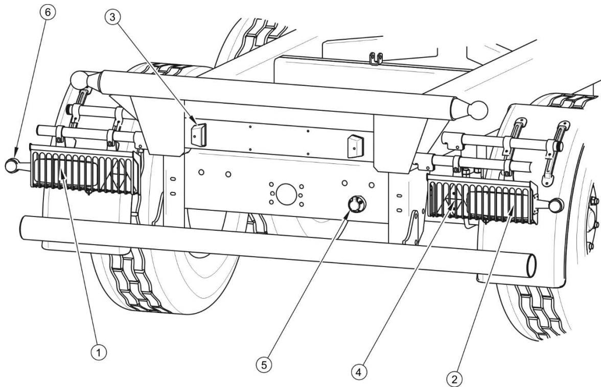
FIGURE 3.13 Emplacement des éléments de l'installation électrique et des réflecteurs – vue arrière
