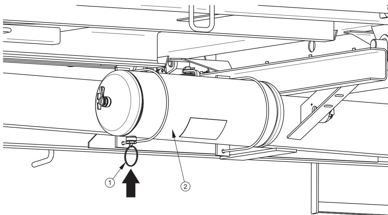
RYSUNEK 5.7 Odwadnianie zbiornika powietrza
