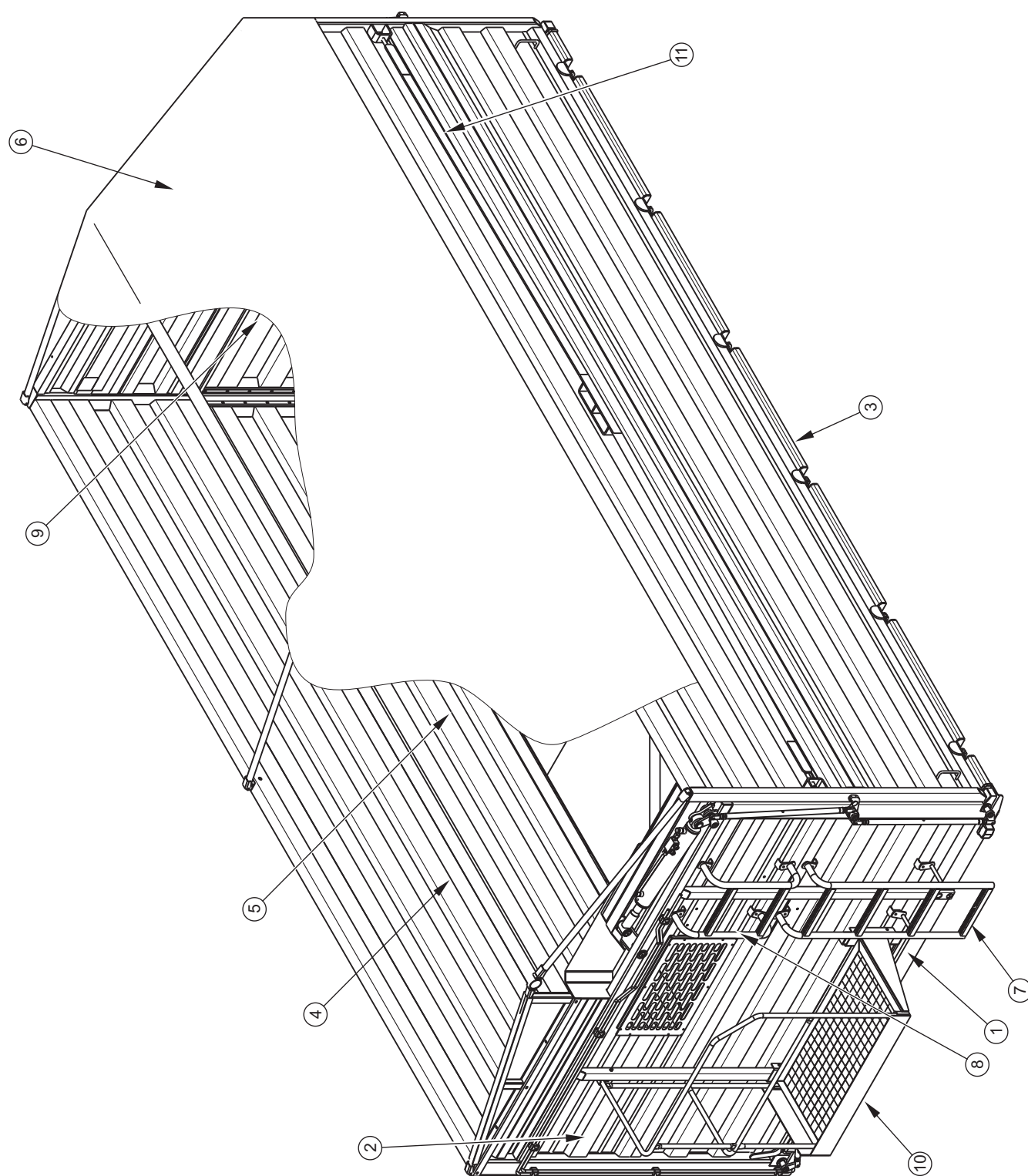
RYСУNEK 3.2 Skrzynia ładunkowa
