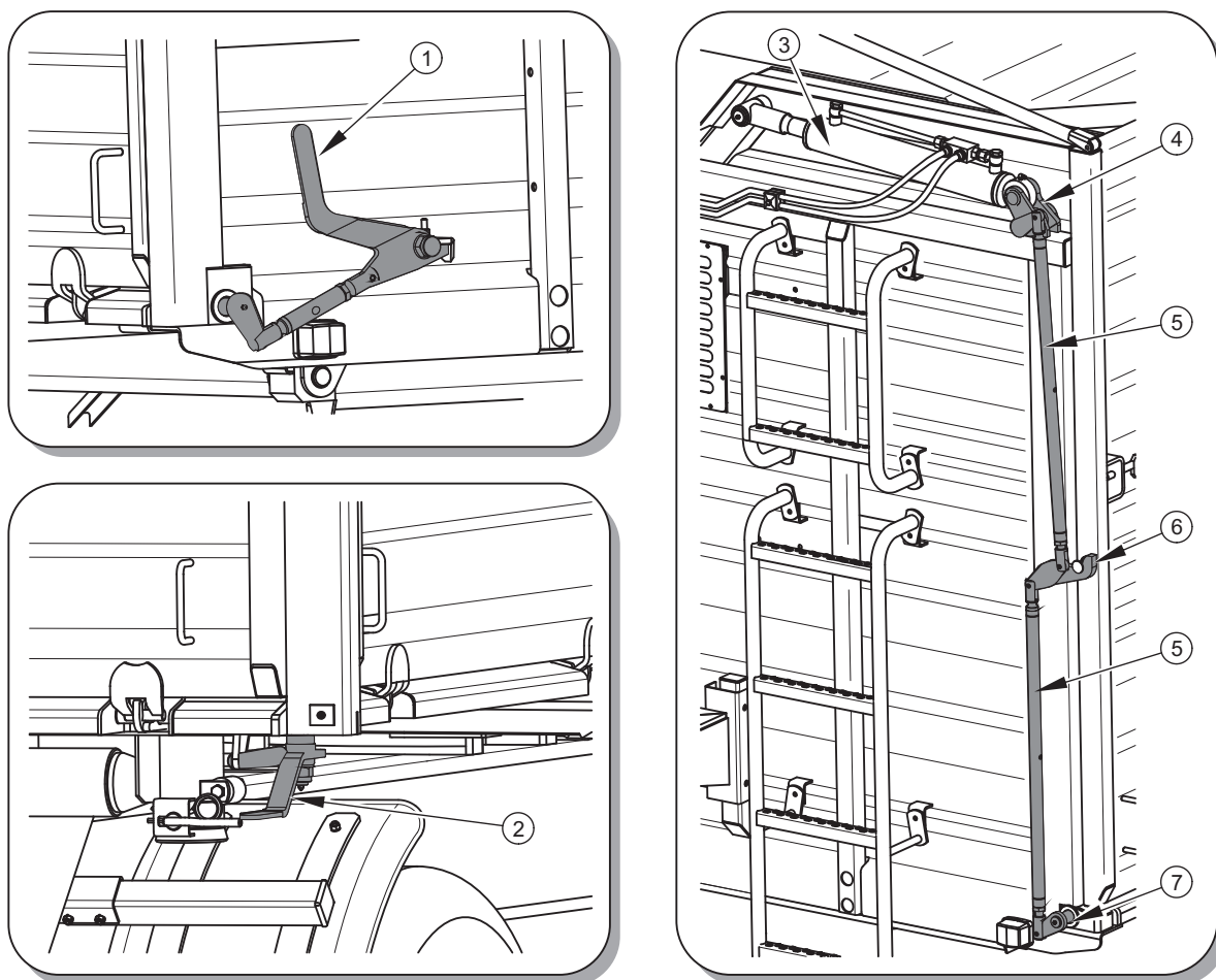
RYСУNEK 3.13 Otwieranie i zamykanie ścian
