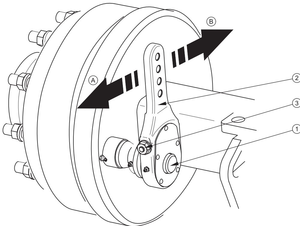
RYSUNEK 5.4 Regulacja hamulca zasadniczego
