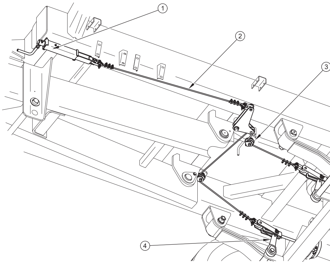
RYSUNEK 3.12 Budowa hamulca postojowego
