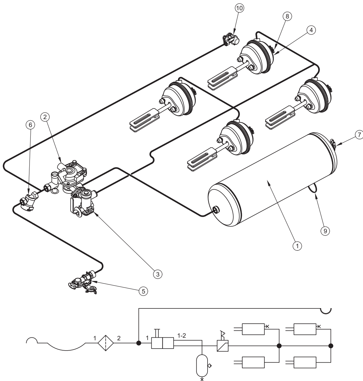
RYСУNEK 3.4 Budowa i schemat instalacji hamulcowej pneumatycznej jedнопроводowej
