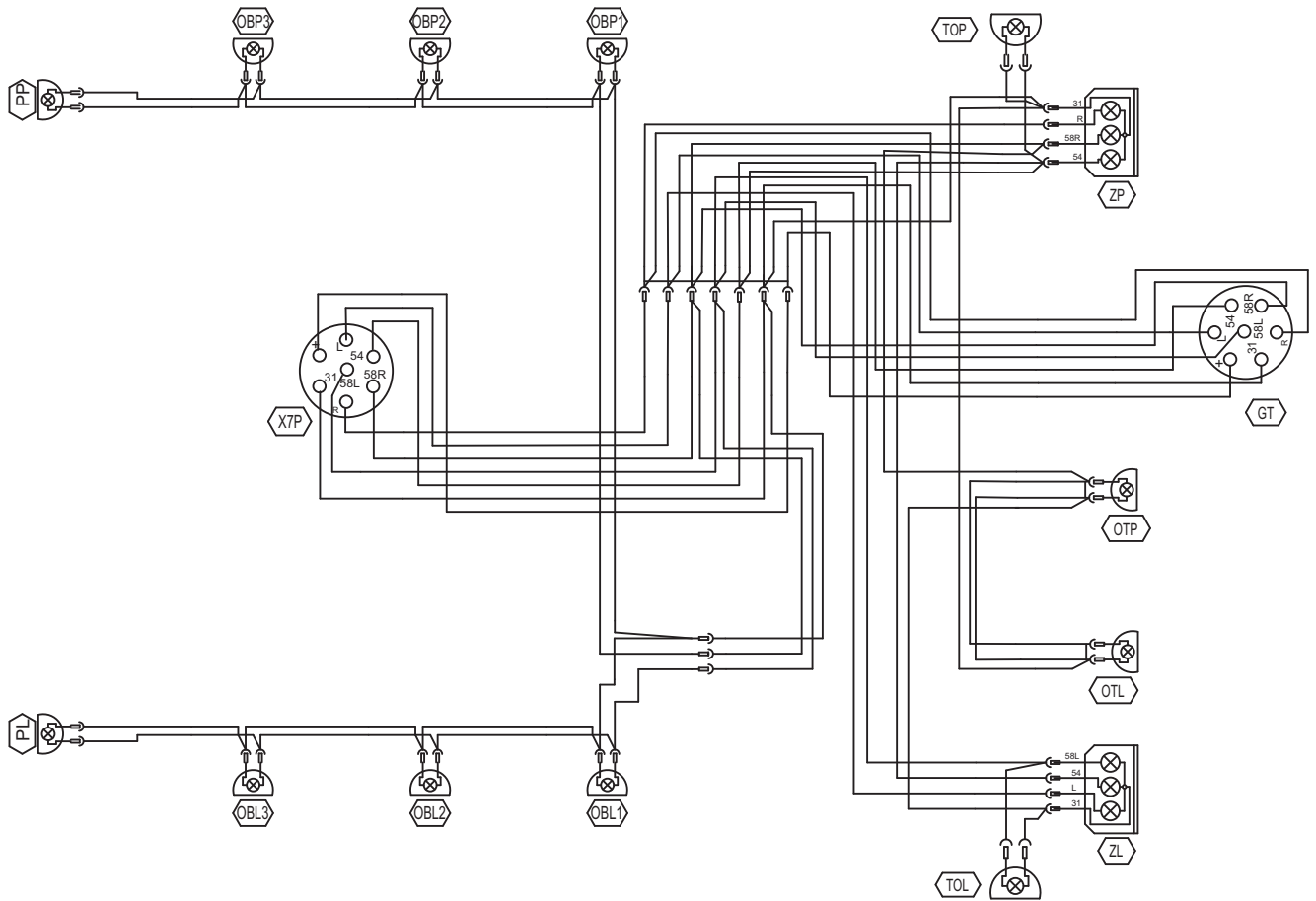
RYSUNEK 3.14 Schemat ideowy instalacji elektrycznej
