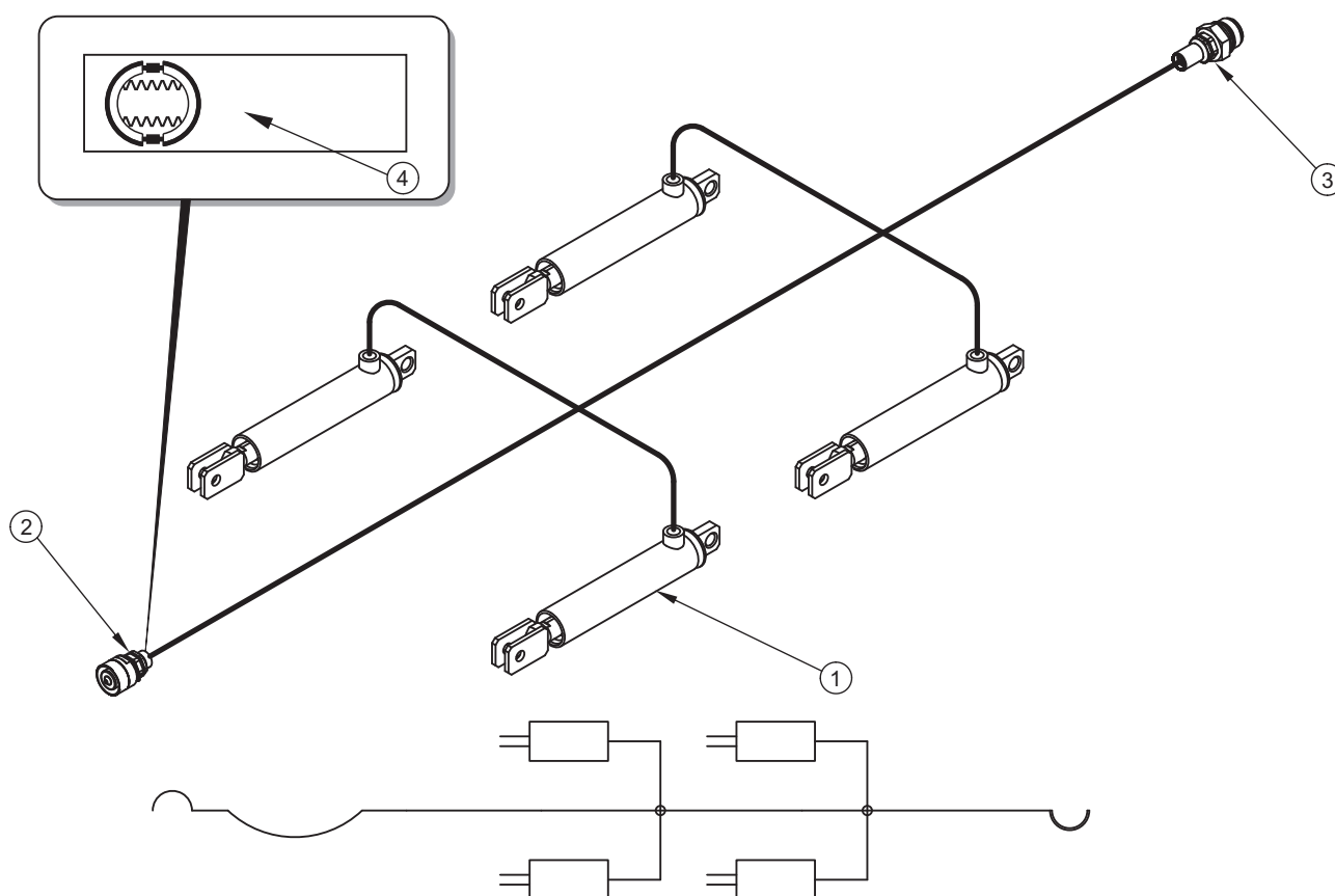
RYСУNEK 3.7 Budowa i schemat instalacji hamulcowej hydraulicznej
