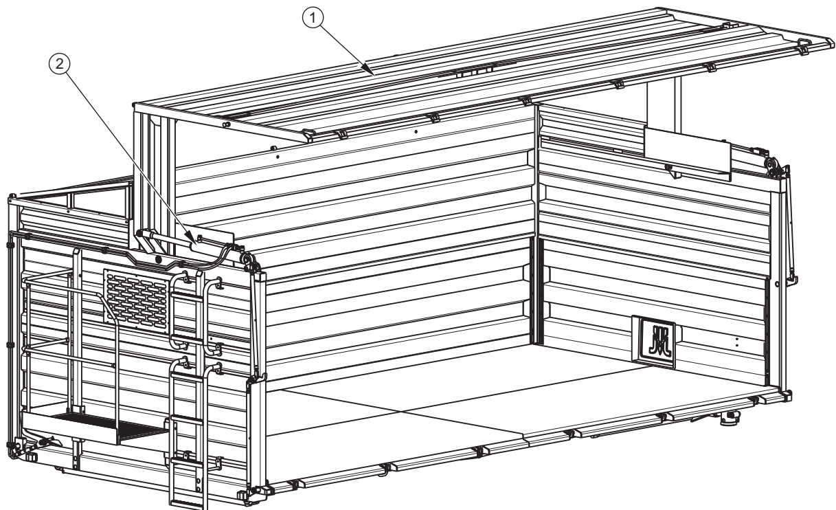
RYSUNEK 4.6 Ściana lewa hydrauliczna
