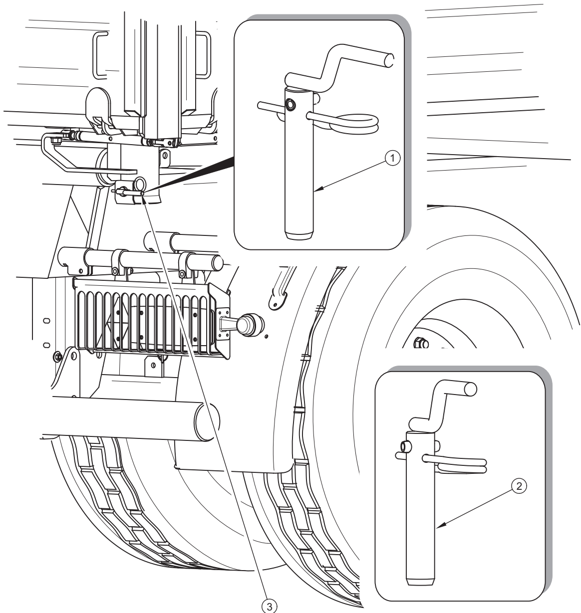
RYSUNEK 4.4 Ryglowanie sworzni wywrotu
