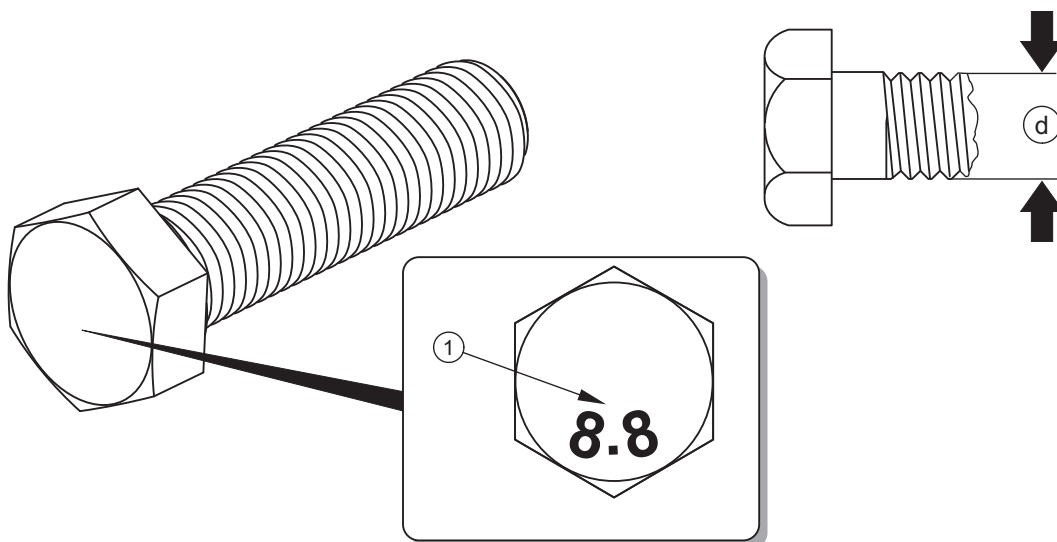
RYSUNEK 5.10 Śruba z gwintem metrycznym
