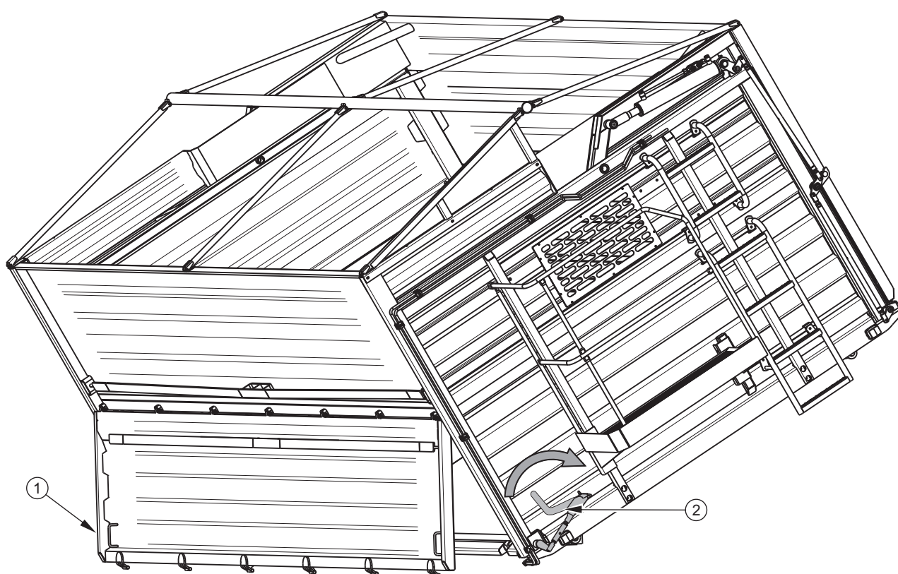
RYSUNEK 4.5 Otwierania prawej ściany skrzyni ładunkowej
