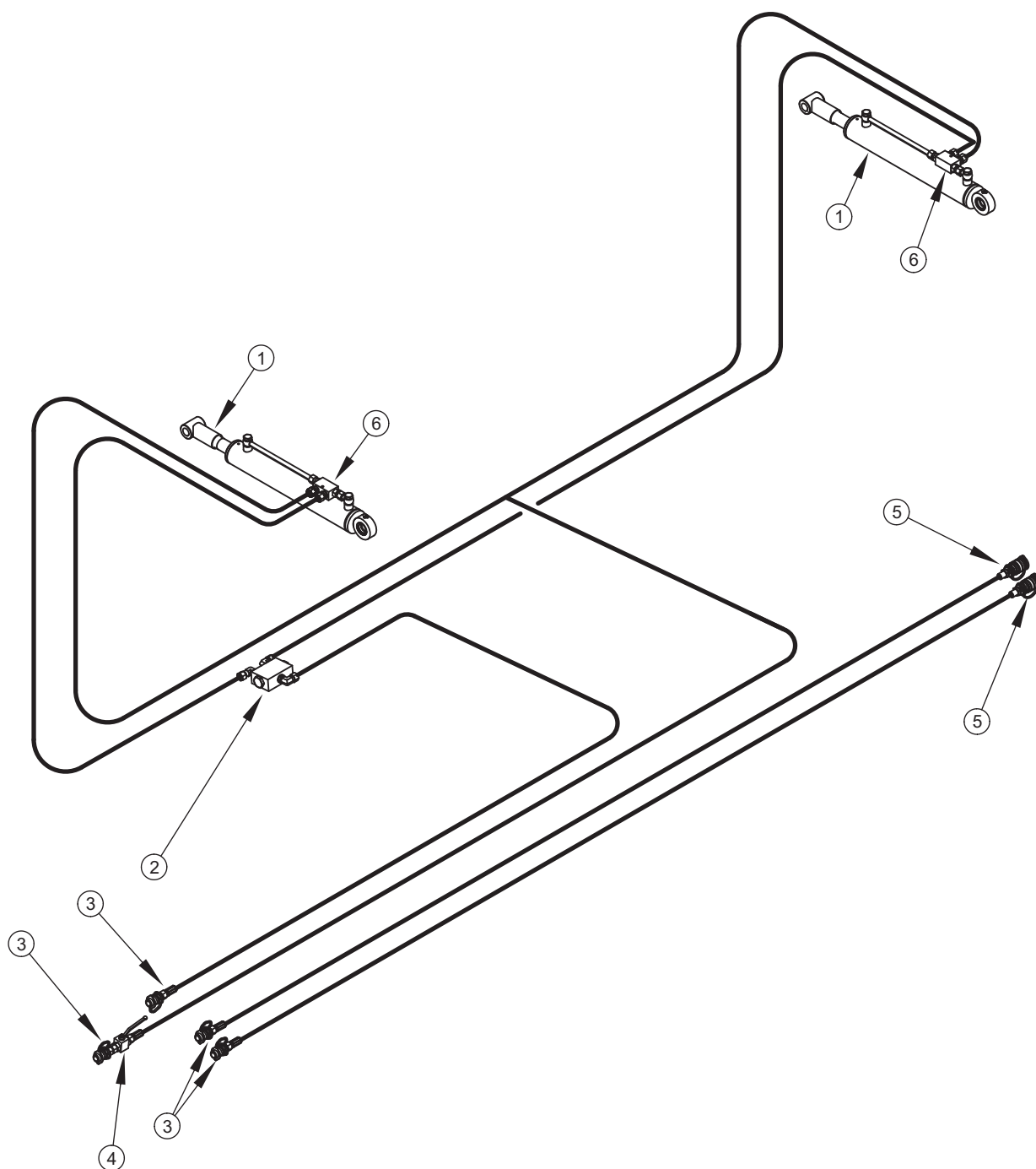
RYSUNEK 3.11 Budowa i schemat instalacji hydraulicznej otwierania burt
