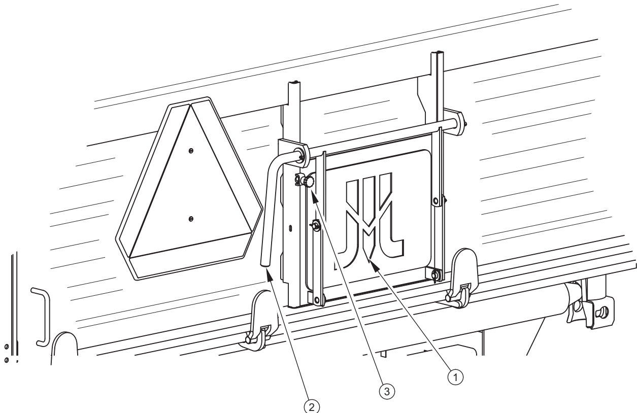
RYСУNEK 3.3 Zasuwa ściany tylnej
