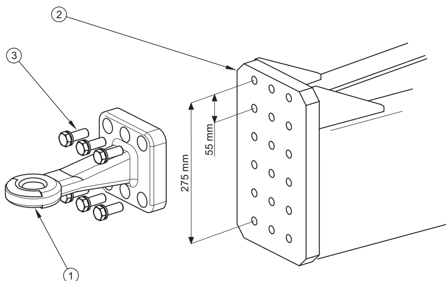
RYSUNEK 5.11 Regulacja położenia cięgna dyszla
