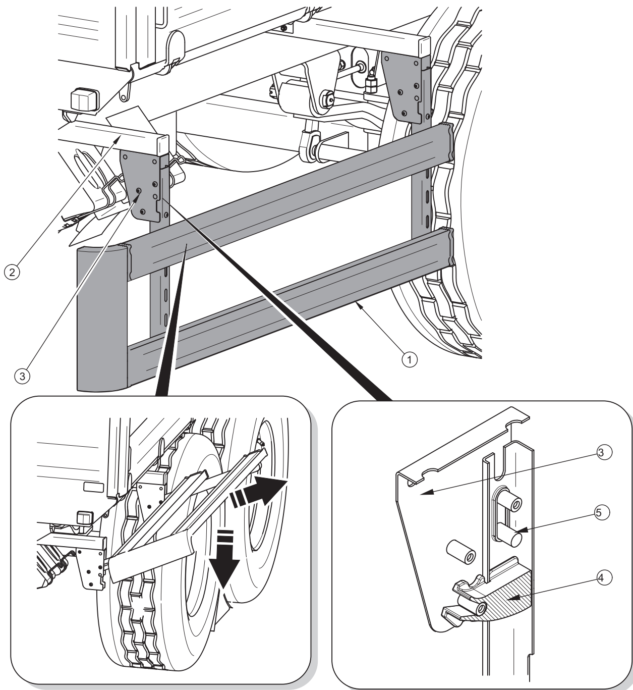
RYSUNEK 4.8 Osłona przeciwnajazdowa lewa
