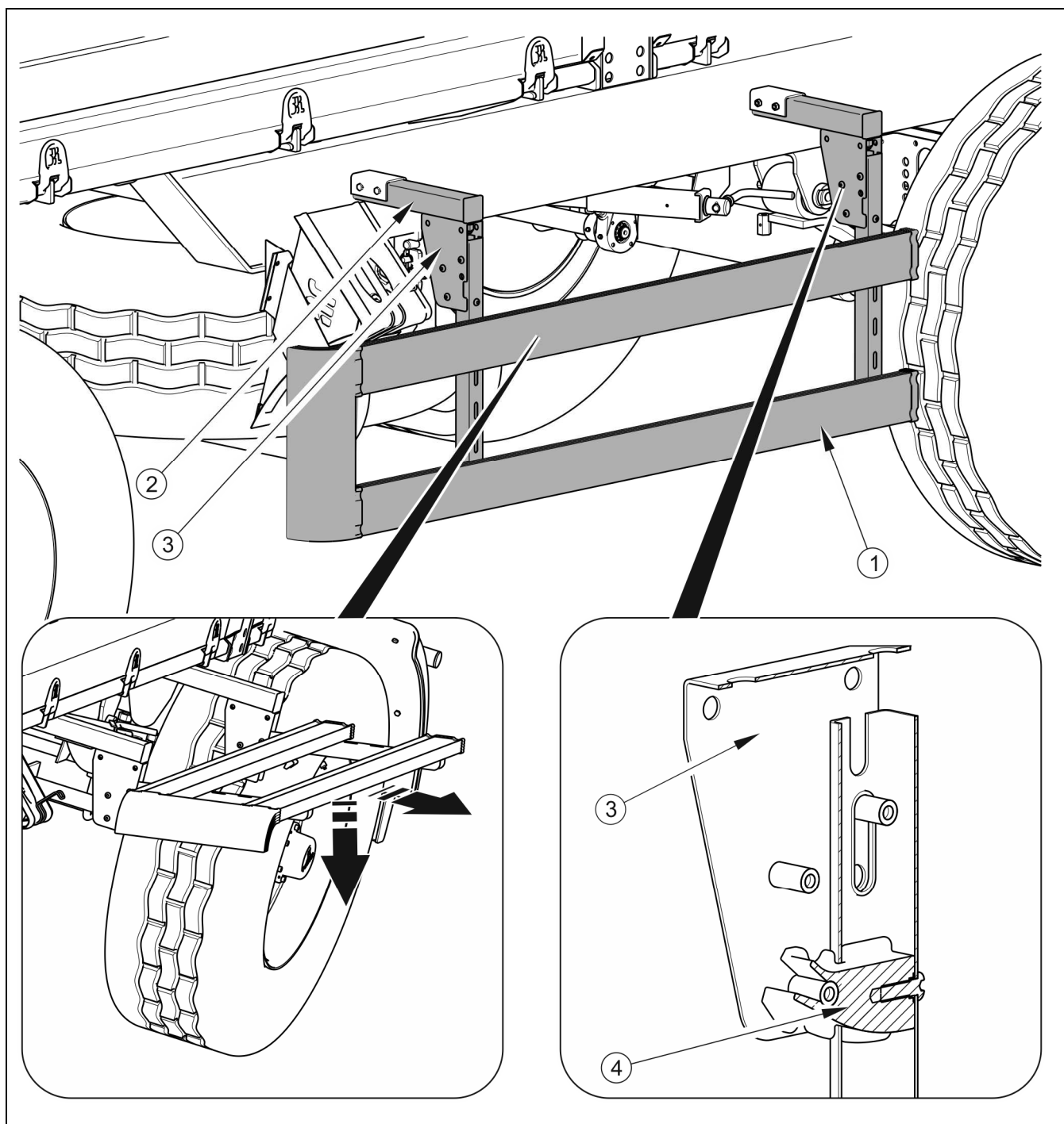
Obrázek 4.6 Protinájezdová zábrana
