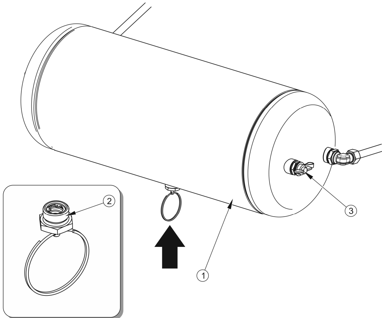
Obrázek 5.10 Odvodňování vzdušníku
