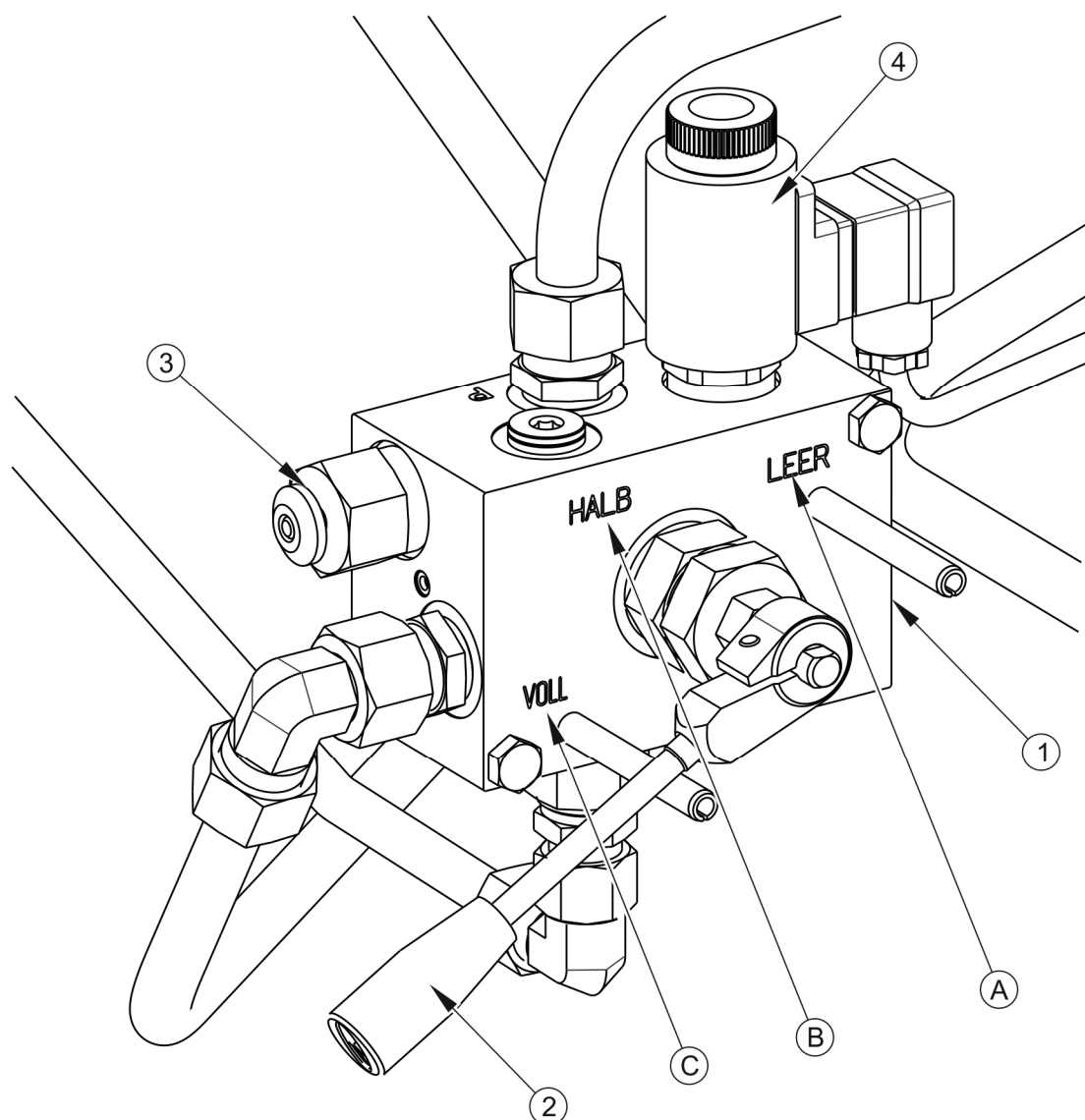
Obrázek 3.9 Elektrohydraulický brzdový ventil
