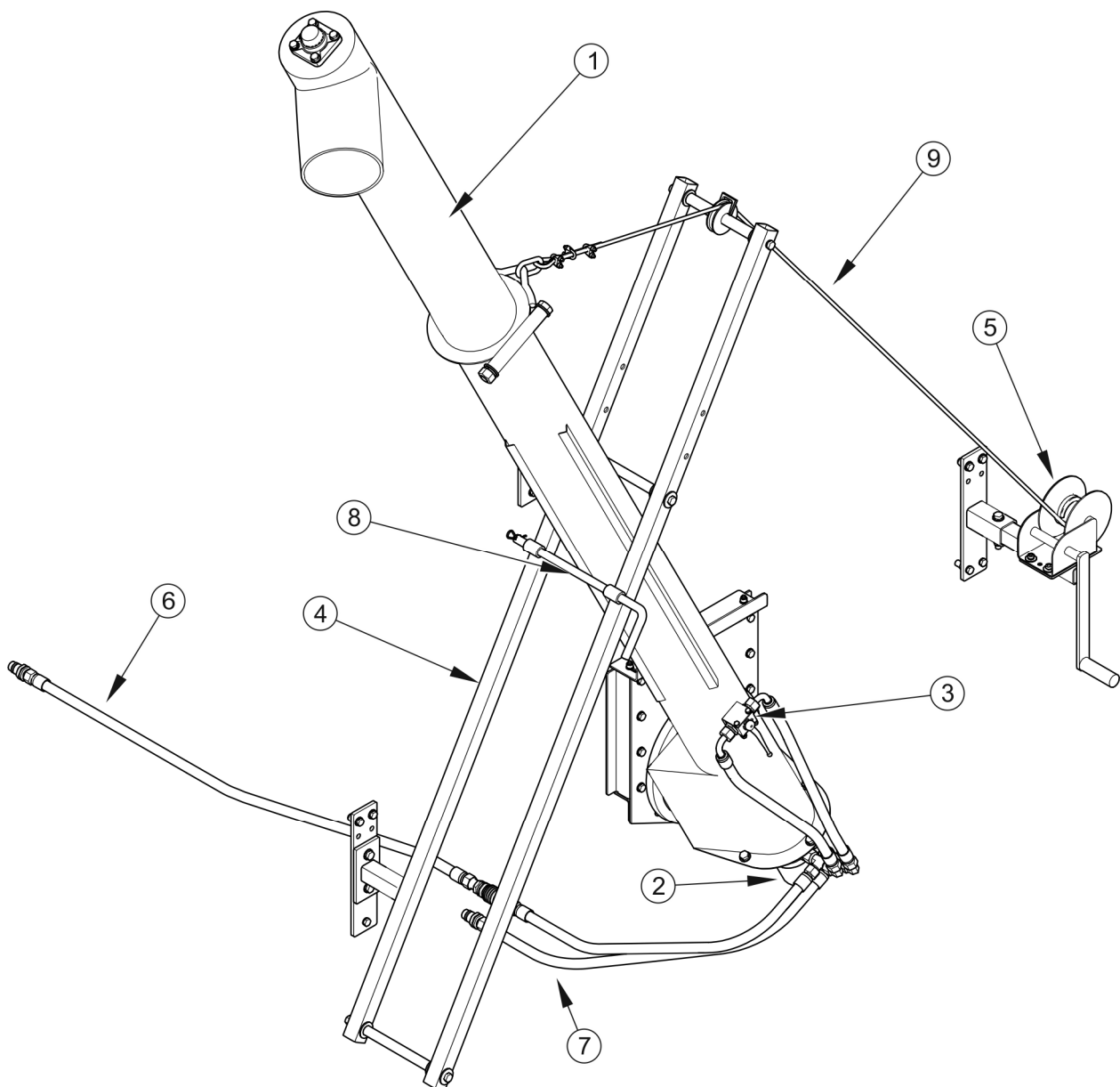
Obrázek 3.12 Konstrukce instalace hydraulické zásobníku
