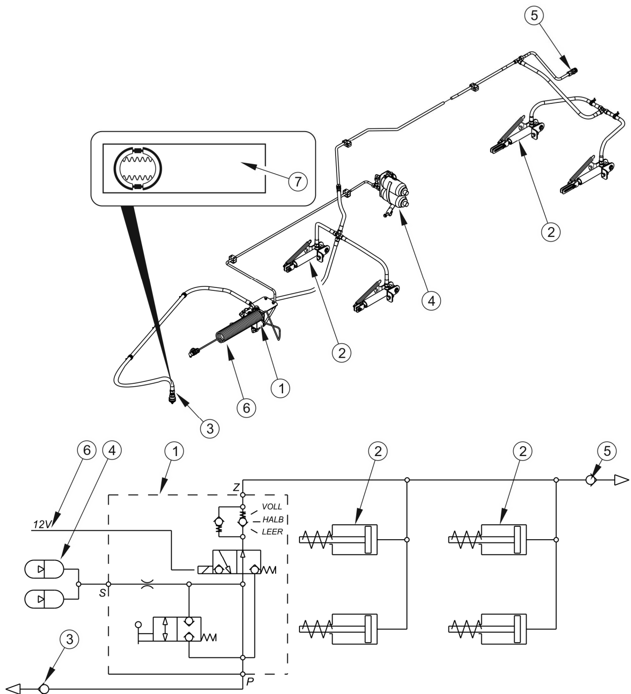
Obrázek 3.7 Konstrukce a schéma hydraulické brzdové instalace
