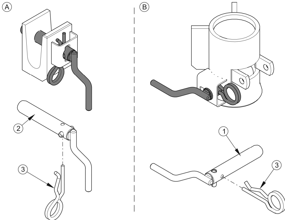
Obrázek 4.2 Zajišťování čepů sklápění
