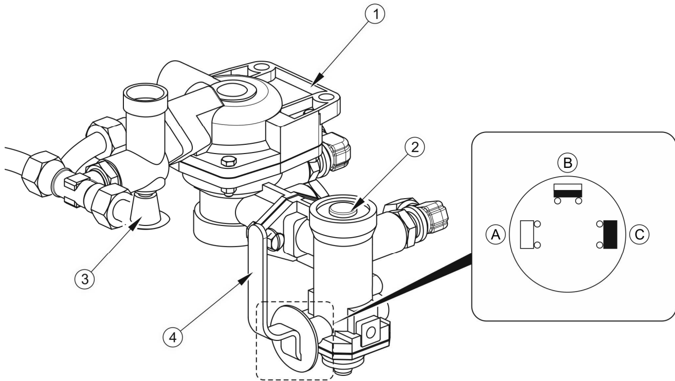
Obrázek 3.8 Ovládací ventil a regulátor brzdové síly
