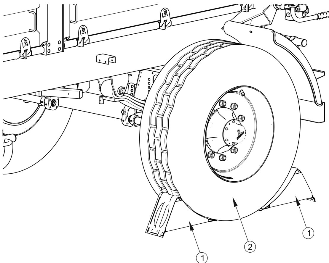
Obrázek 2.1 Způsob podložení klínů
