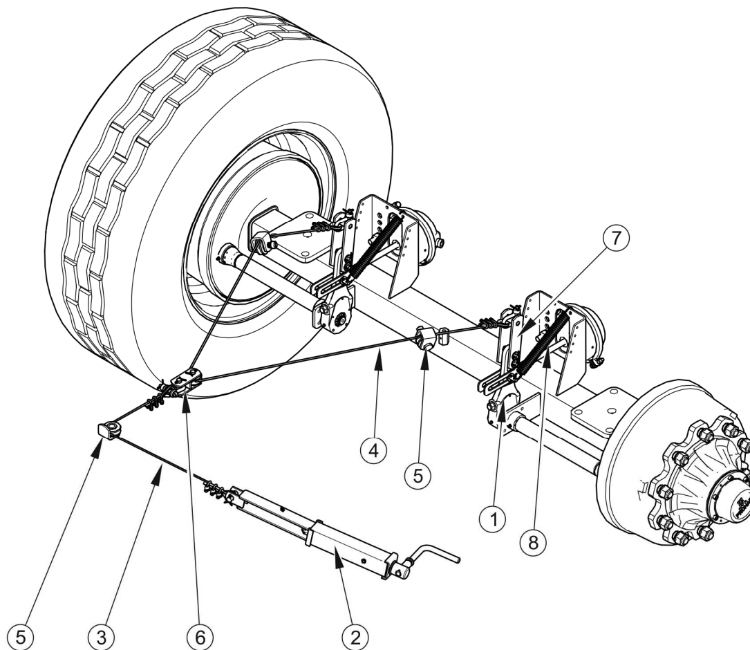
Obrázek 3.13 Konstrukce parkovací brzdy
