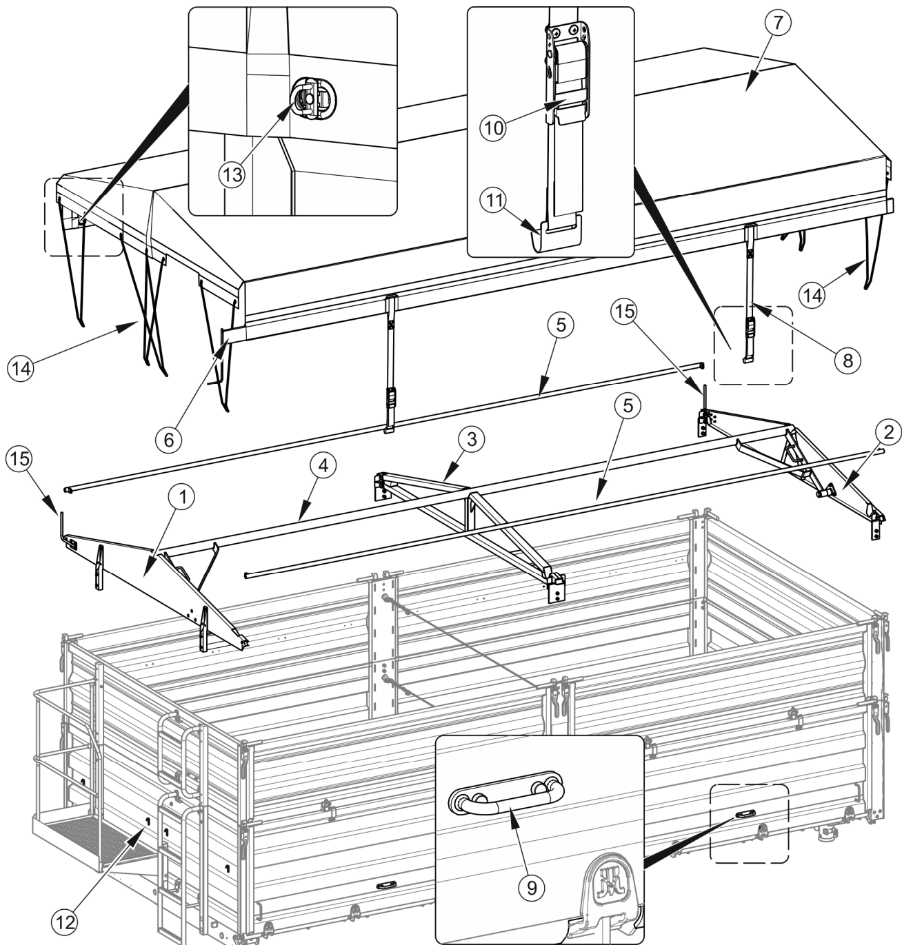
Obrázek 5.15 Podpěrná konstrukce s plachtou
