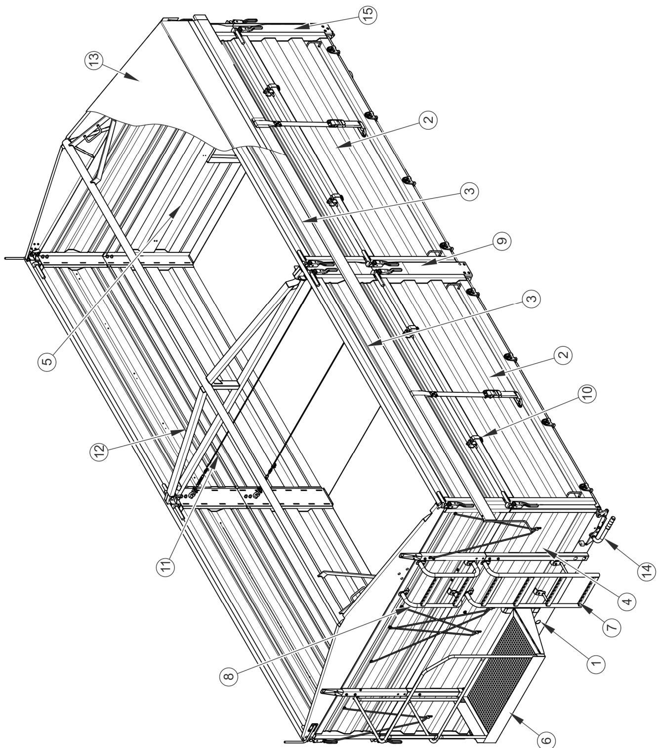
Obrázek 3.2 Nákladní prostor s dělenými stěnami.
