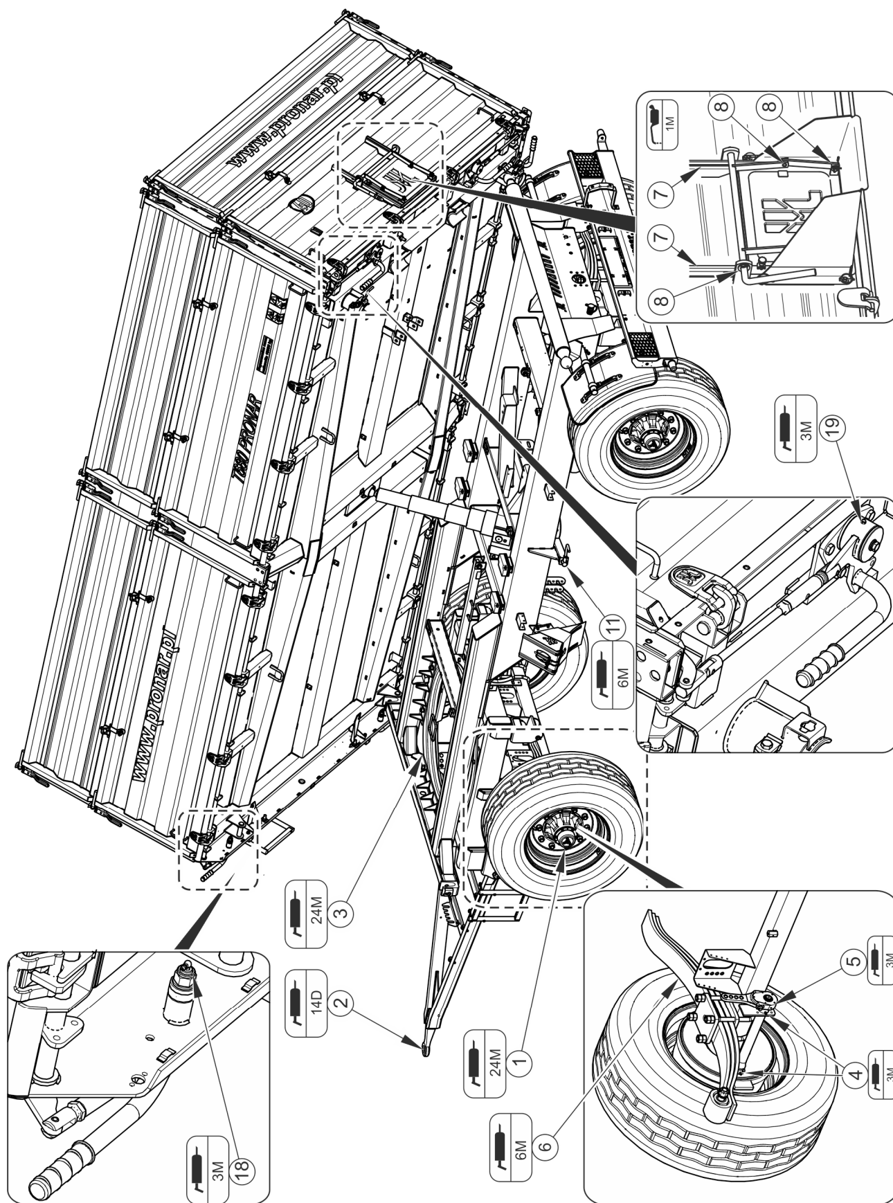
Obrázek 5.12 Mazací body přívěsu, část 1
