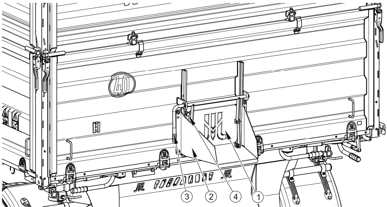
Obrázek 3.3 Zadní bočnice
