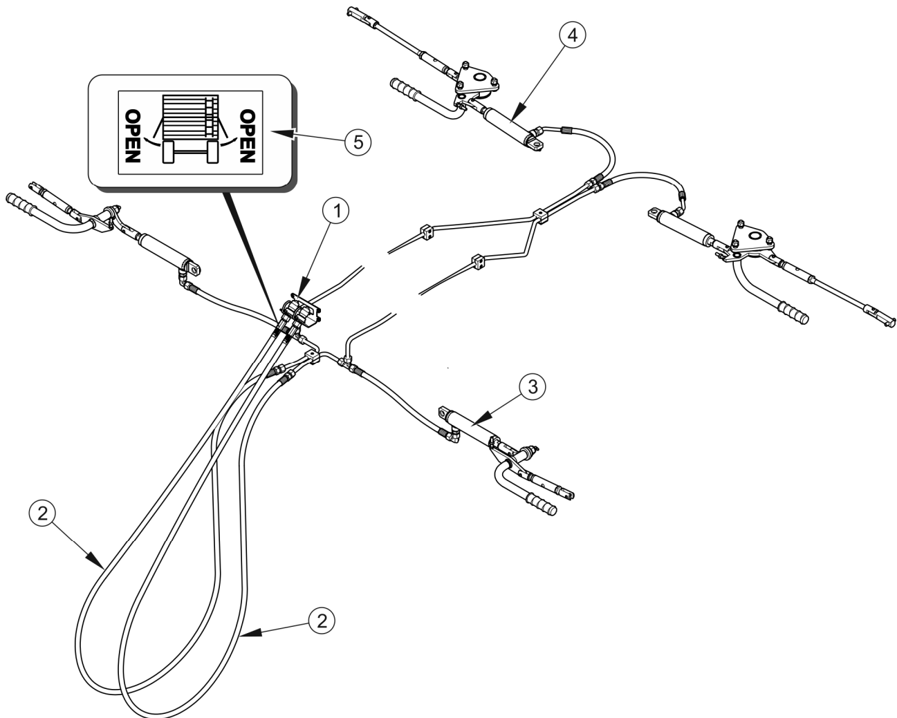
Obrázek 3.11 Konstrukce hydraulické instalaci odemykání bočnic
