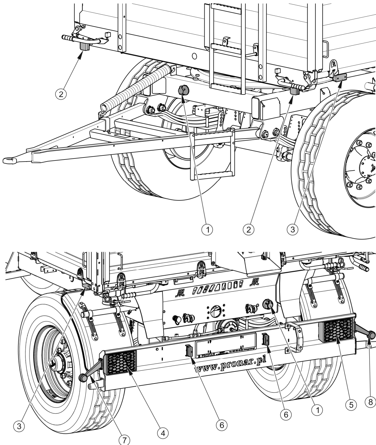
Obrázek 3.14 Rozmístění elektrických a odrazových prvků
