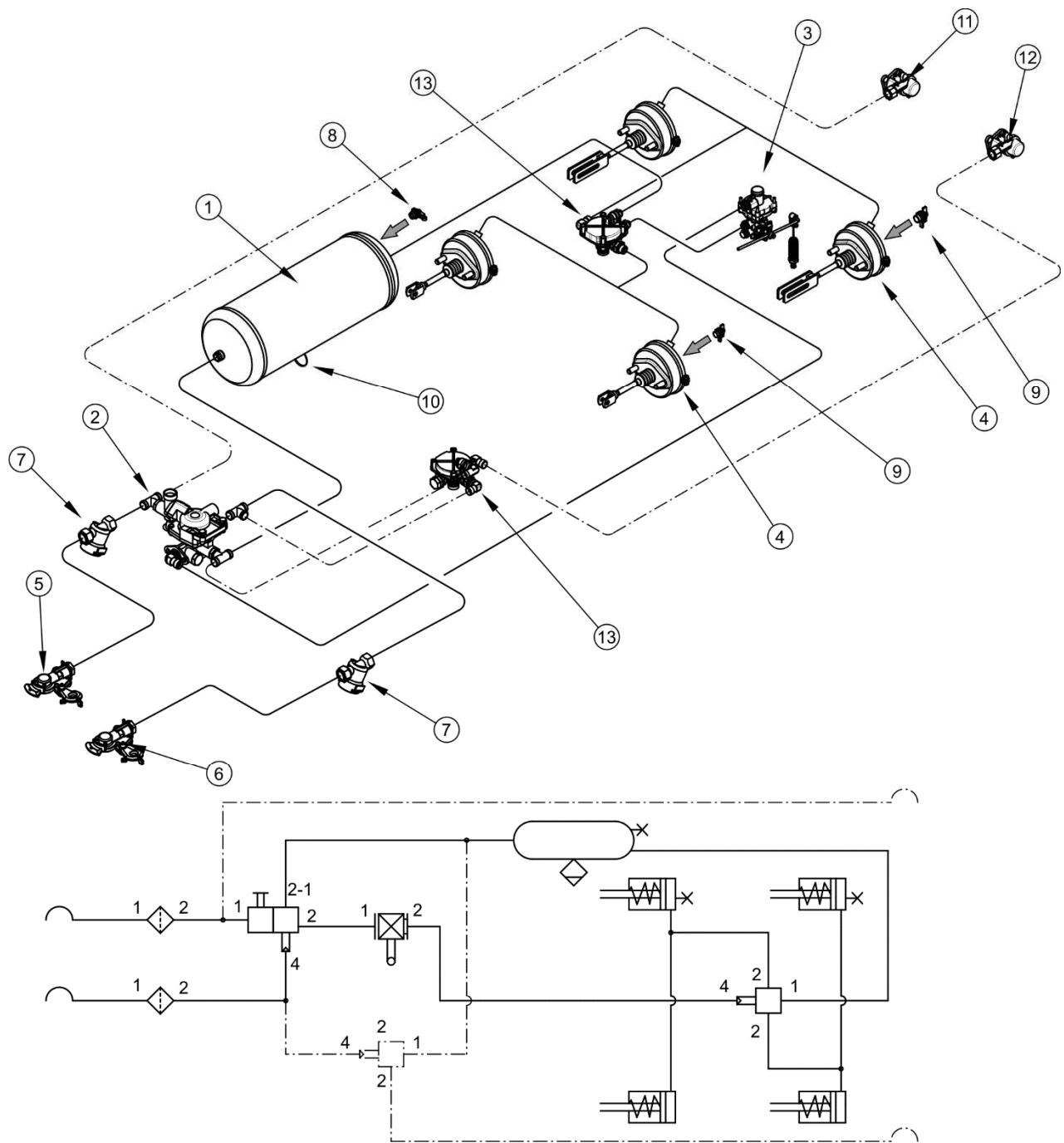
FIGURE 3.5 Construction et schéma du système de freinage pneumatique double circuit, régulateur automatique
