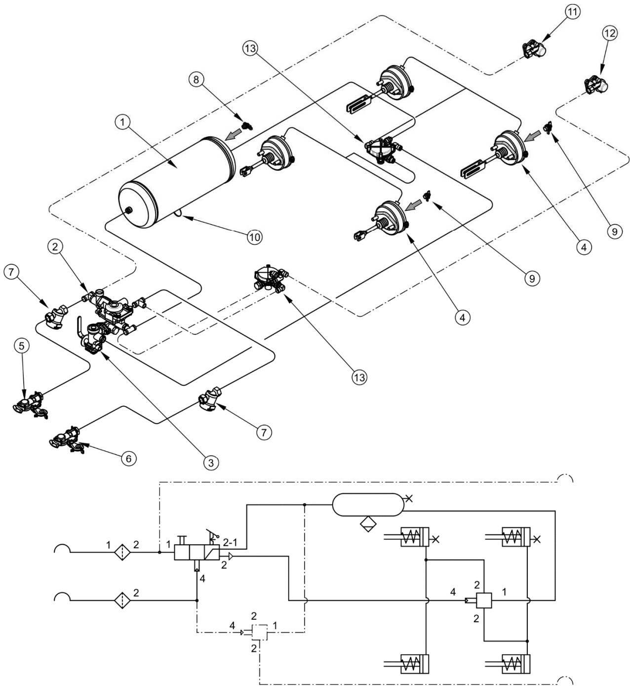
FIGURE 3.4 Construction et schéma du système de freinage pneumatique à double circuit
