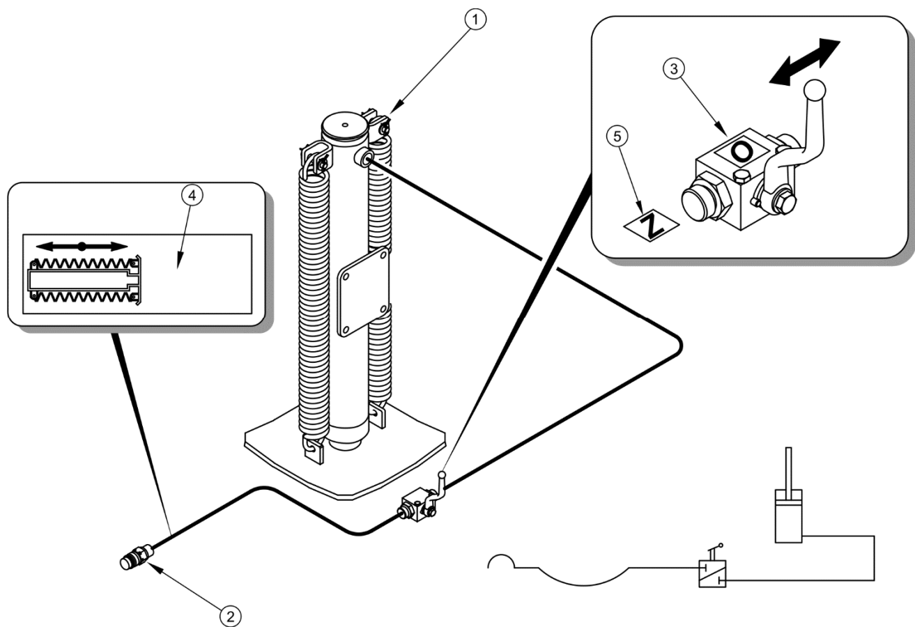
FIGURE 3.9 Construction et schéma de l'installation hydraulique de la béquille droite
