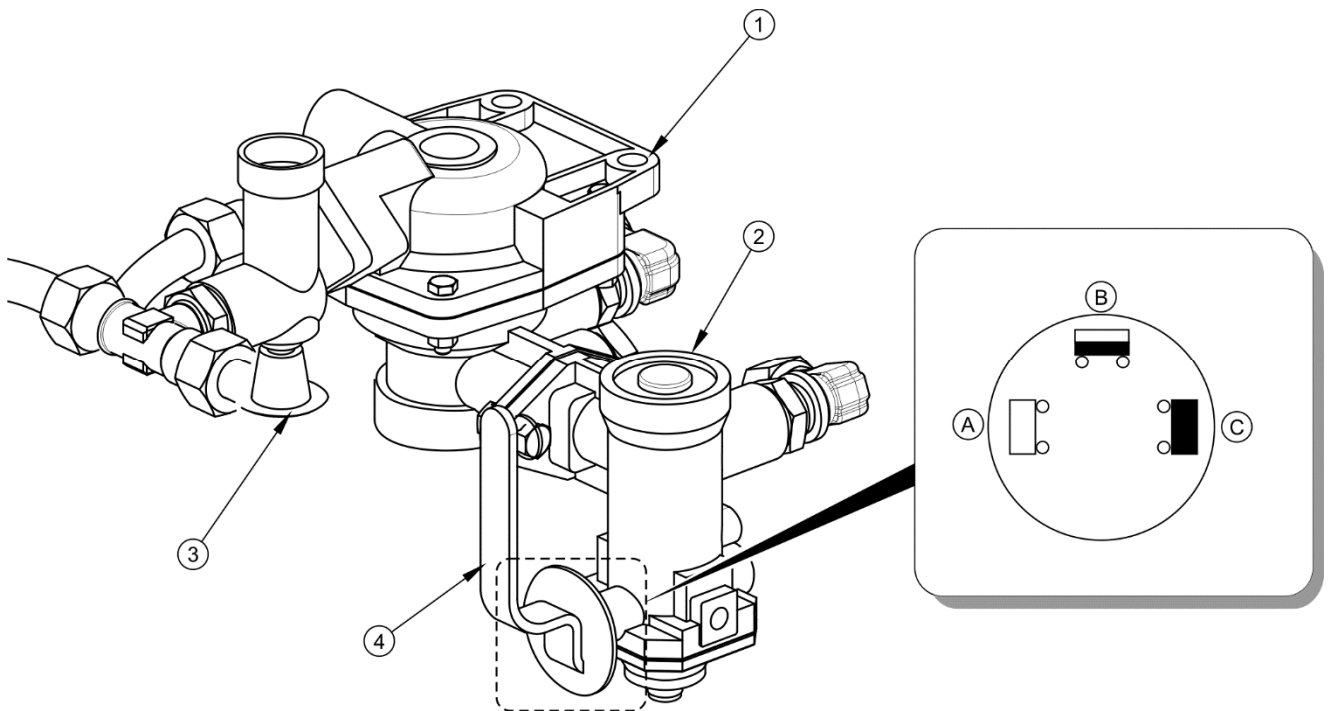
FIGURE 3.7 Vanne de commande et régulateur de la force de freinage
