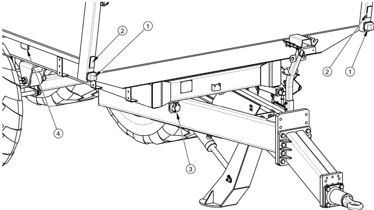
FIGURE 3.13 Emplacement des éléments électriques et réfléchissants à l'avant
