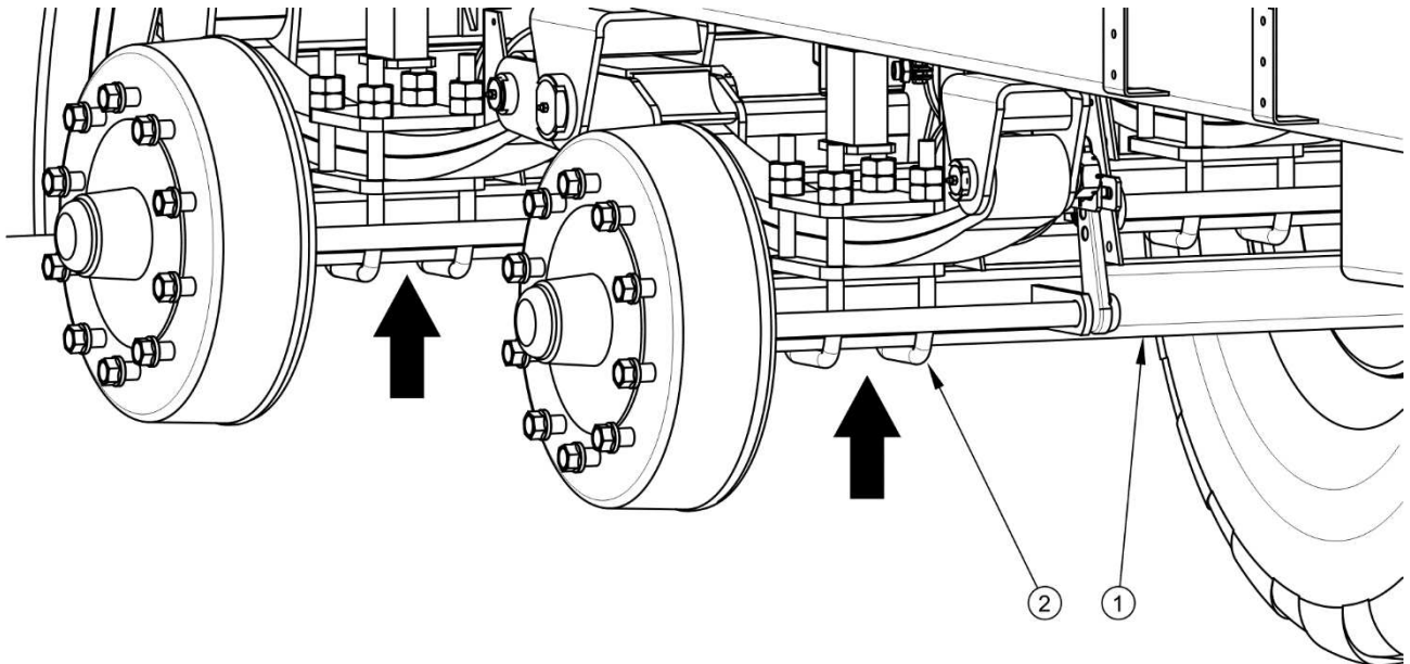
FIGURE 5.2 Point d'appui du support
