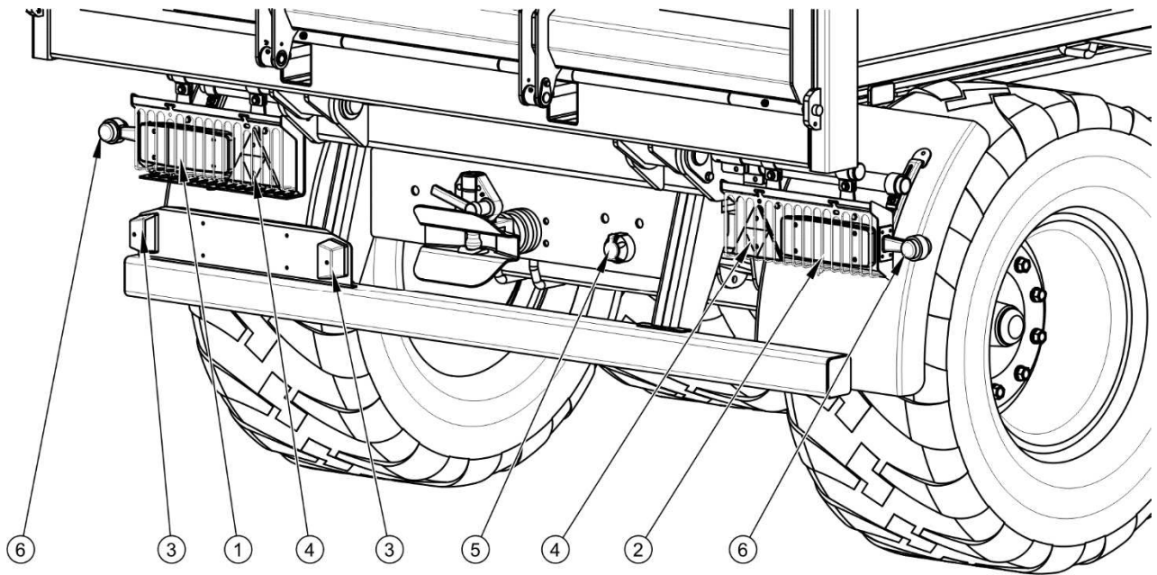
FIGURE 3.14 Emplacement des éléments électriques et réfléchissants à l'arrière
