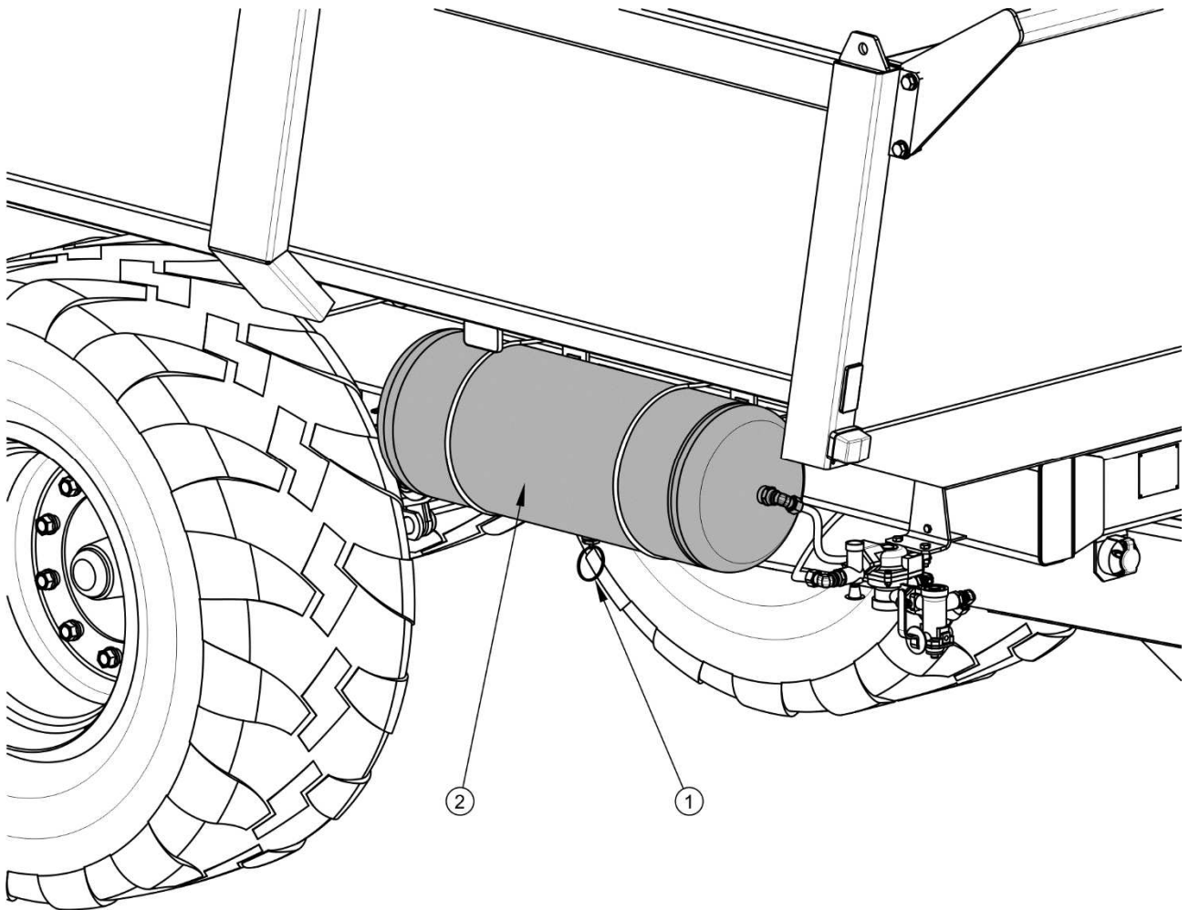
FIGURE 5.9 Purge du réservoir d'air
