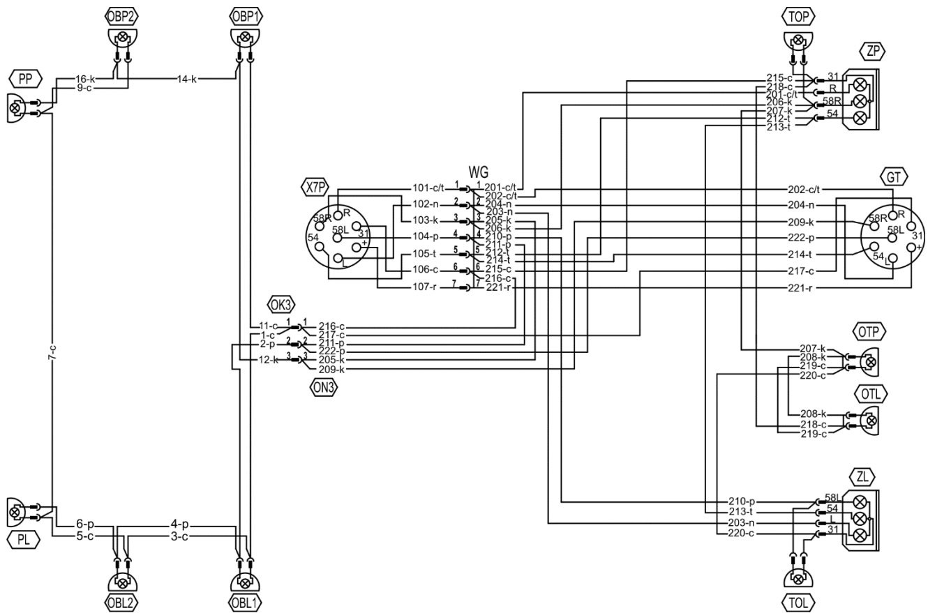
FIGURE 3.15 Schéma de principe de l'installation électrique
