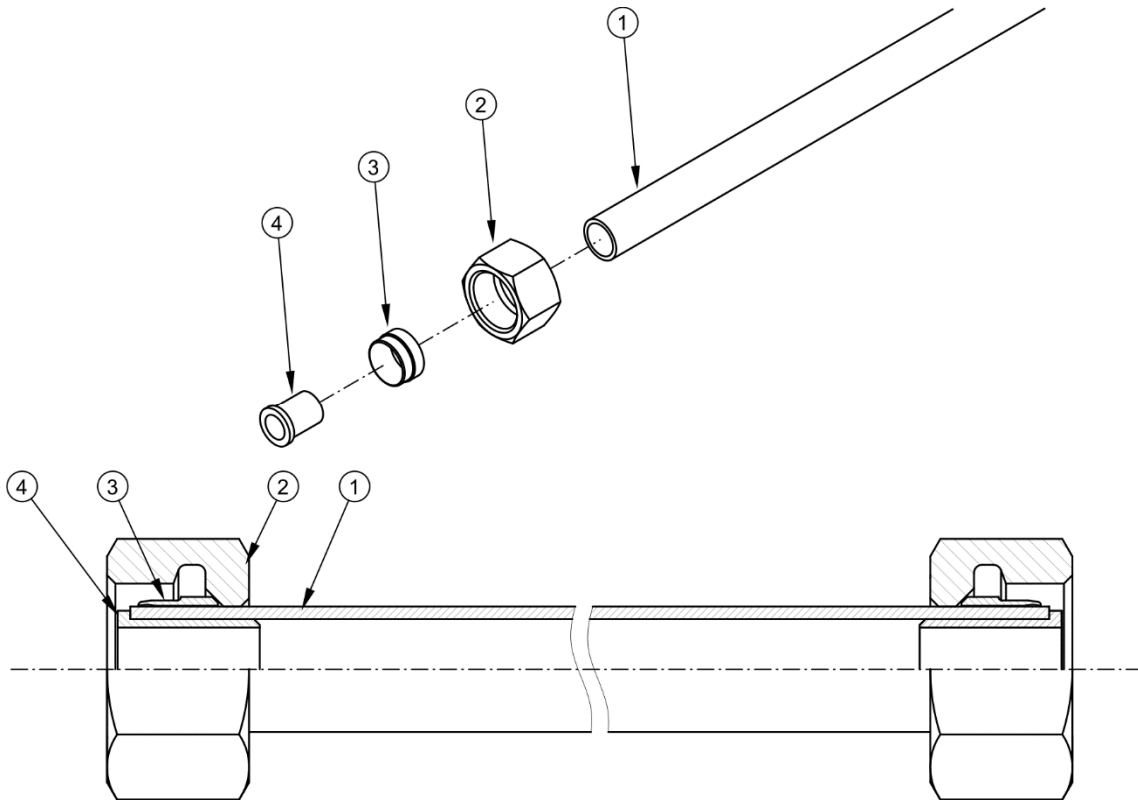
FIGURE 5.10 Montage du tuyau pneumatique
