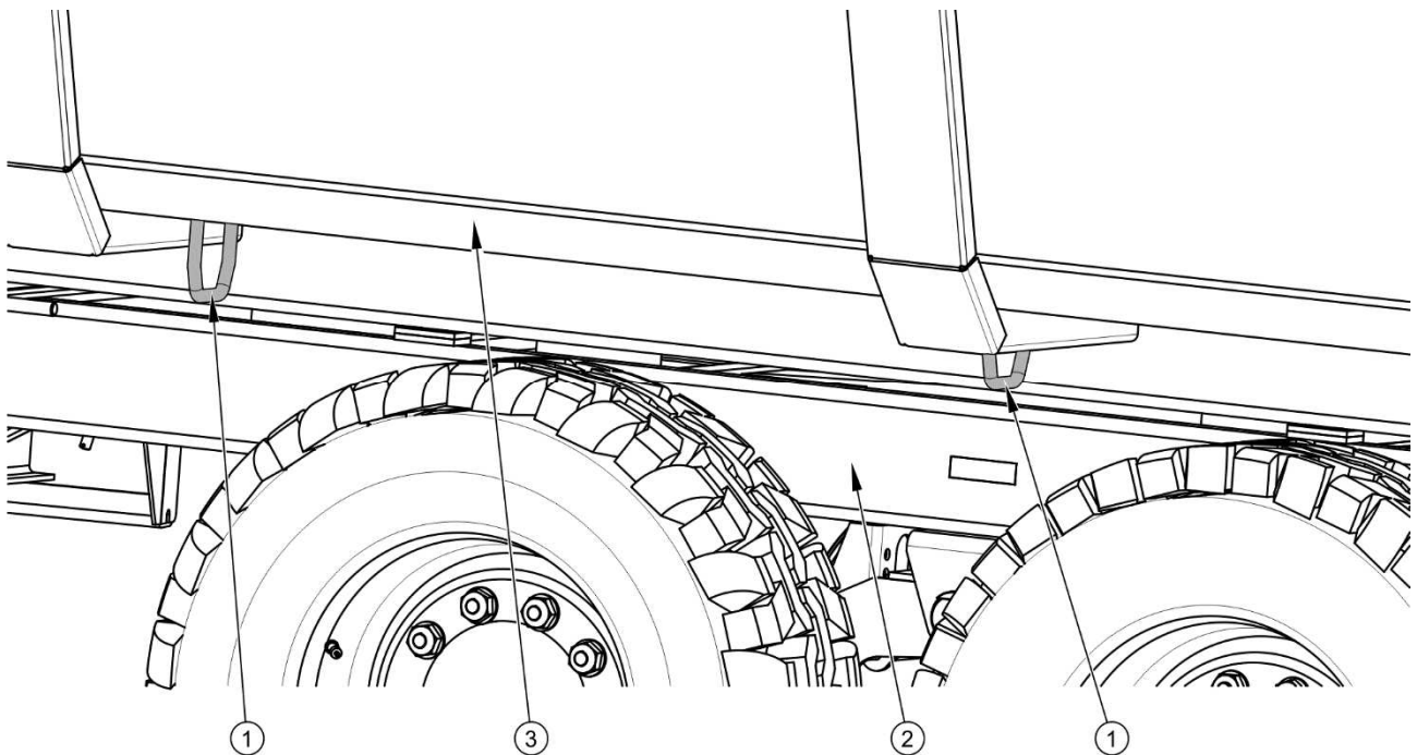
FIGURE 1.3 Emplacement des anneaux de transport
