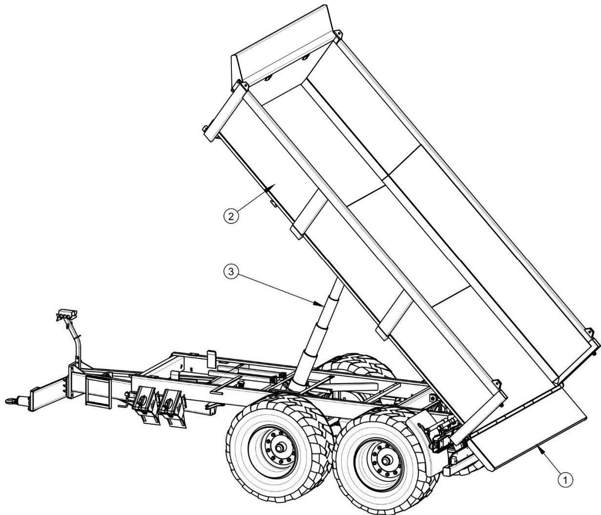
FIGURE 4.1 Déchargement de la benne avec hayon hydraulique arrière
