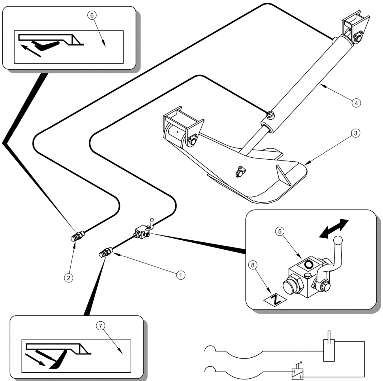
FIGURE 3.10 Construction et schéma de l'installation hydraulique de la béquille ciseaux
