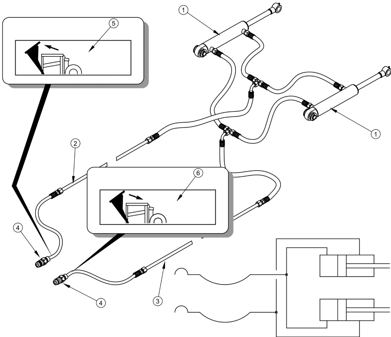
FIGURE 3.11 Construction et schéma de l'installation hydraulique du hayon arrière (1) cylindre hydraulique, (2) conduit d'alimentation, (3) conduit de retour, (4) raccord rapide, (5), (6) autocollant d'information
