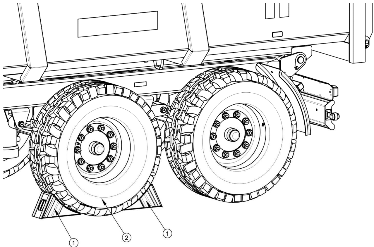
FIGURE 2.1 Méthode de placer les cales
