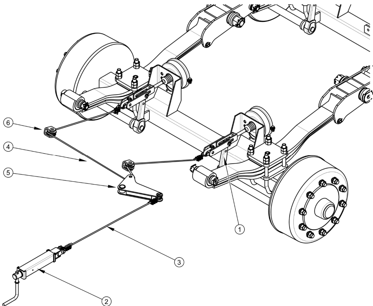
FIGURE 3.12 Construction du frein de stationnement
