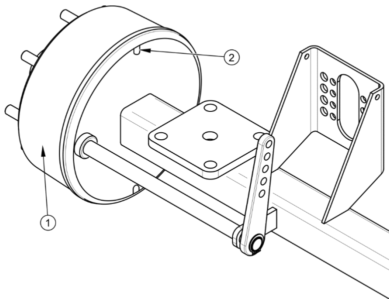
FIGURE 5.1 Contrôle des garnitures de freins
