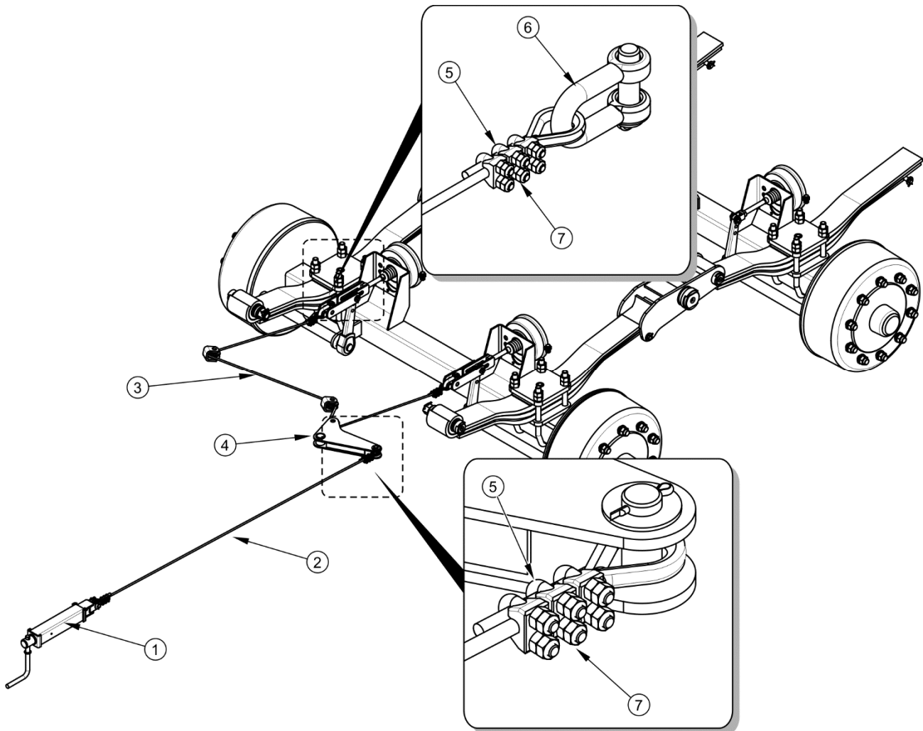
FIGURE 5.6 Réglage de la tension de câble du frein de stationnement
