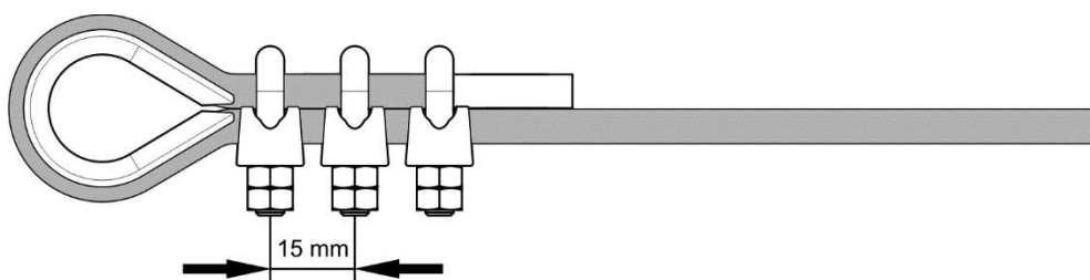
FIGURE 5.7 Montage des serre-câbles du câble d'acier
