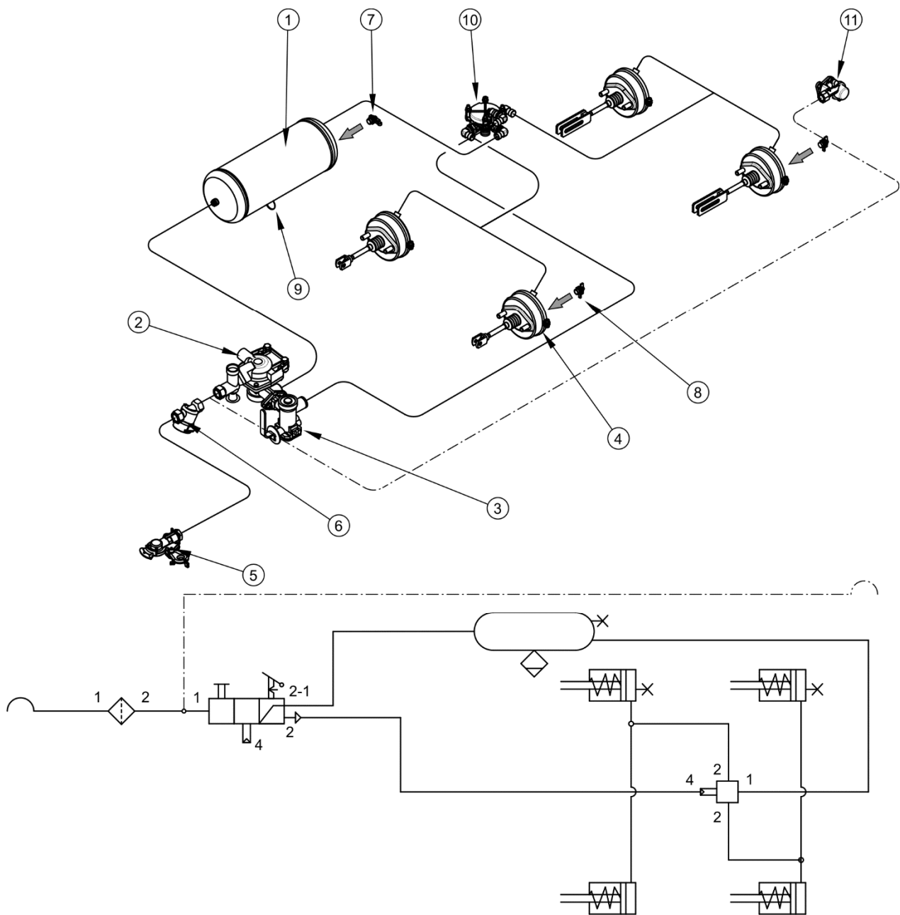
FIGURE 3.3 Construction et schéma du système de freinage hydraulique à circuit simple
