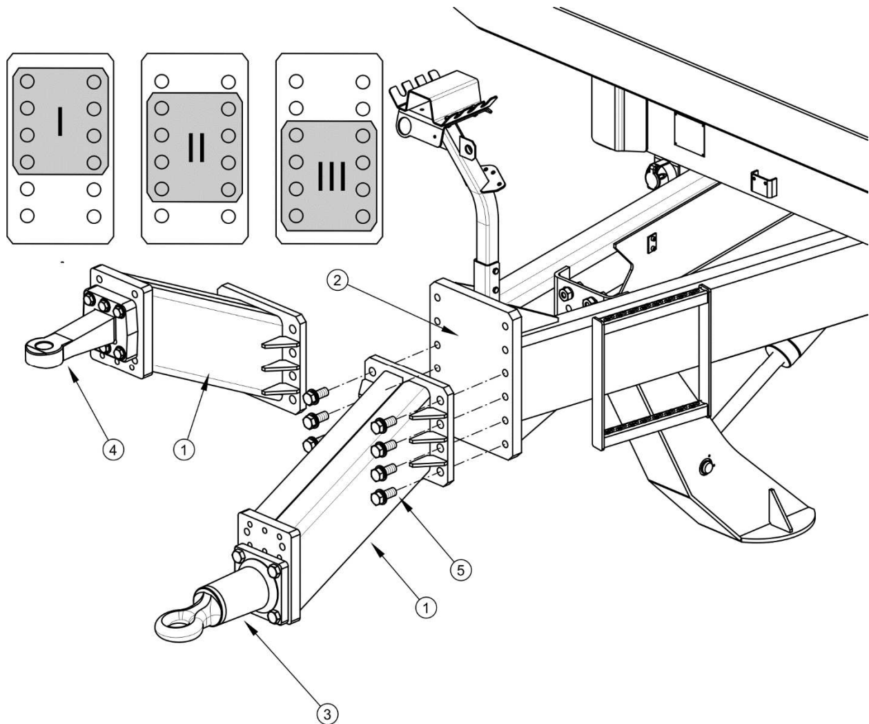
FIGURE 5.13 Réglage de la position du timon
