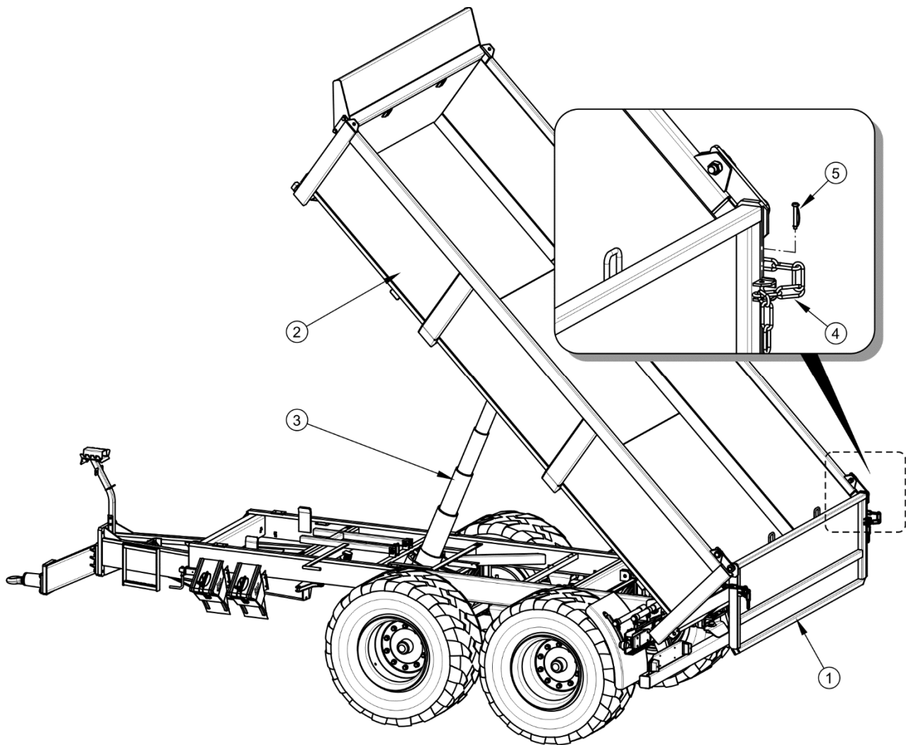
FIGURE 4.2 Déchargement de la benne avec hayon pivotant
