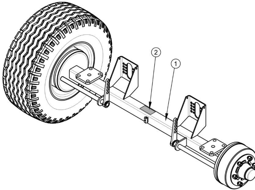
FIGURE 1.2 Emplacement de la plaque signalétique de l'essieu moteur
