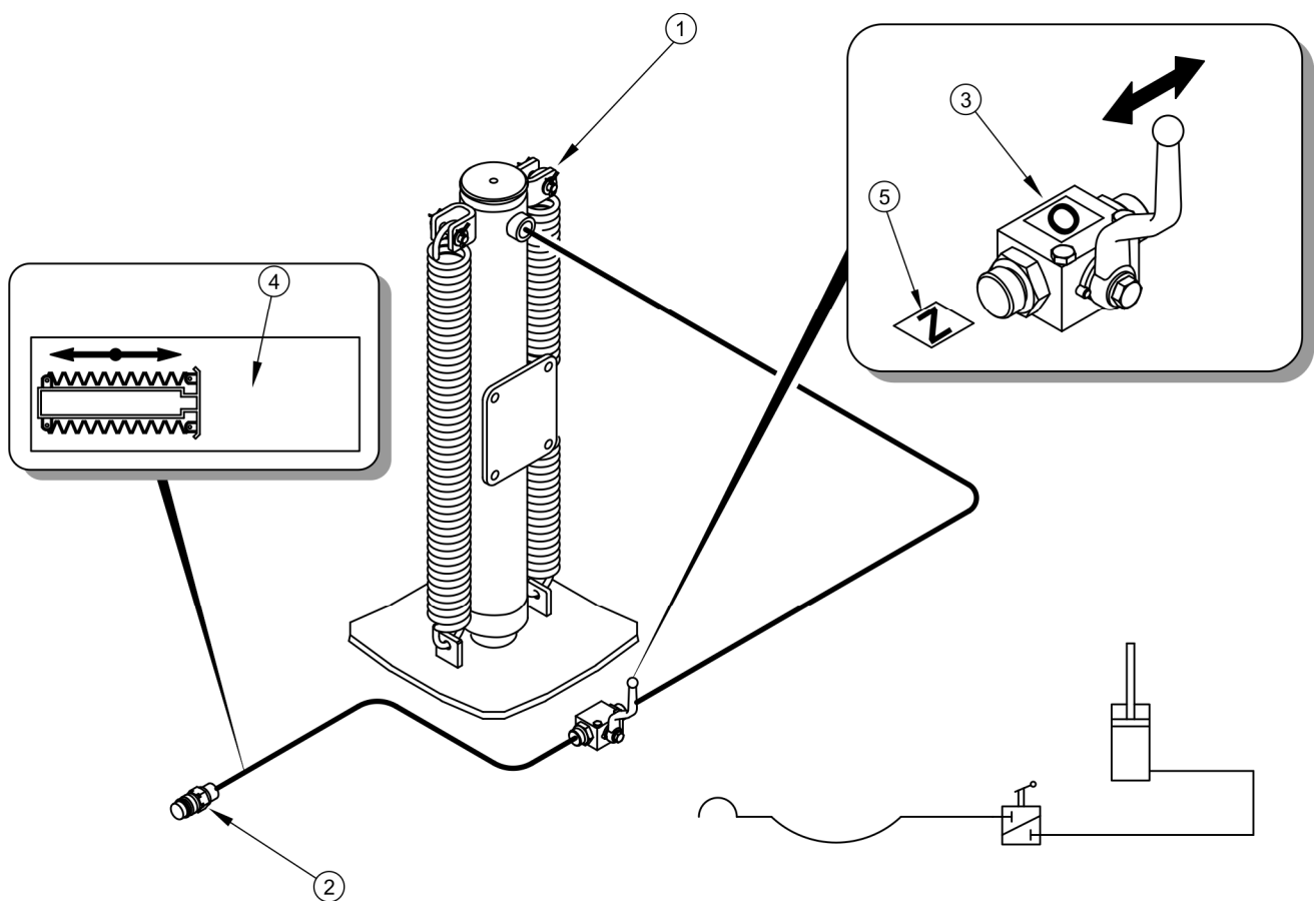
RYSunEK 3.10 Budowa i schemat instalacji hydraulicznej podпоры prostej
