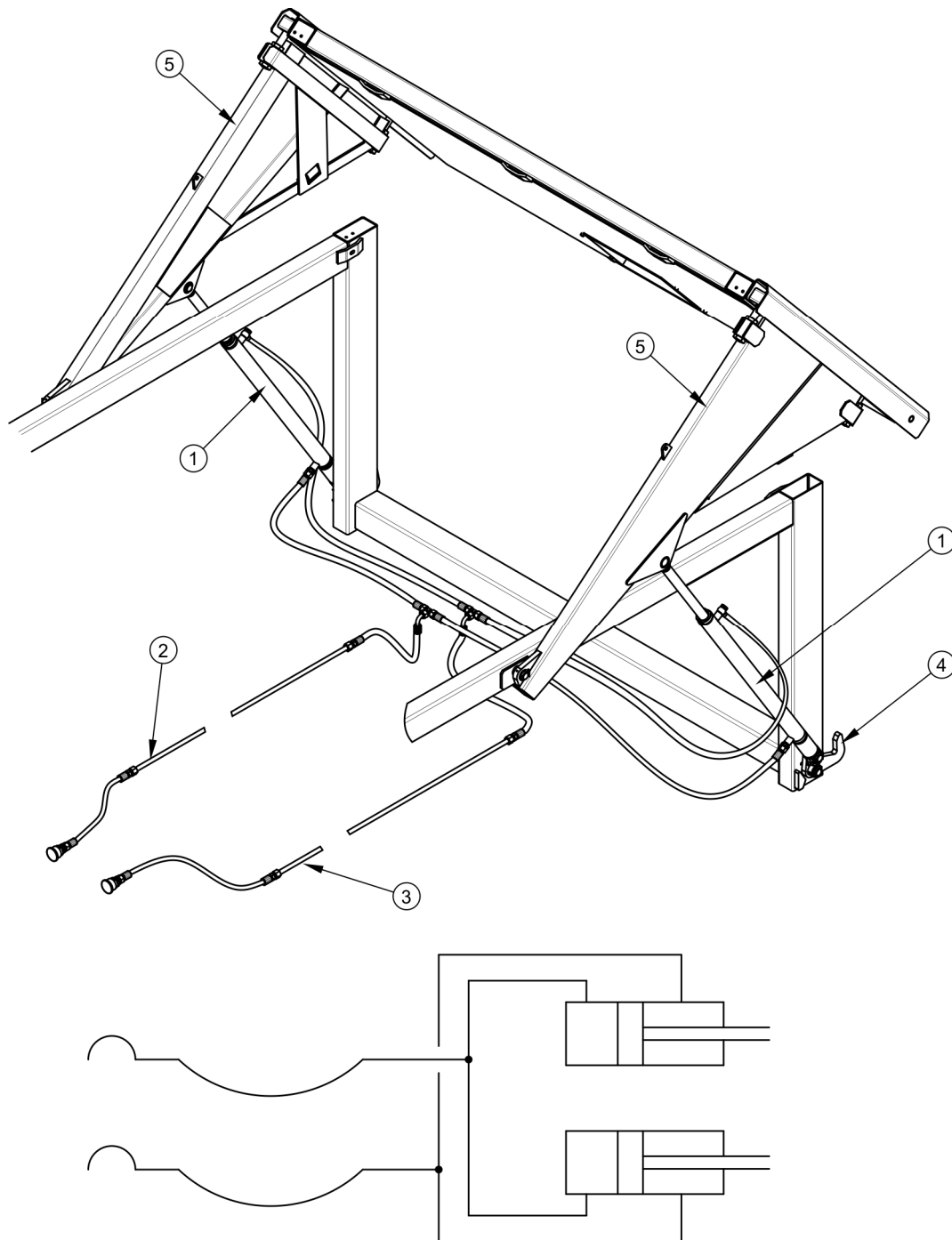
RYСУNEK 3.12 Budowa i schemat instalacji hydraulicznej klapy tylnej
