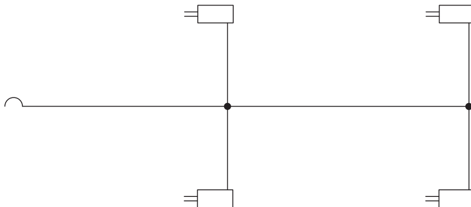
Rysunek 3.10 Schemat instalacji hamulcowej hydraulicznej
