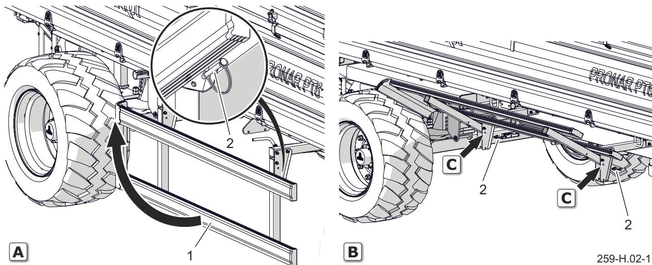
Rysunek 4.2 Obsługa osłon najazdowych
