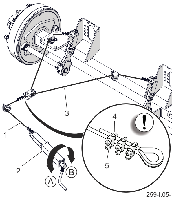
Rysunek 5.13 Kontrola napięcia linki
