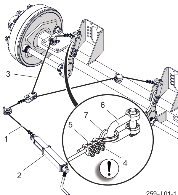
Rysunek 6.2 Wymiana linki hamulca postojowego
