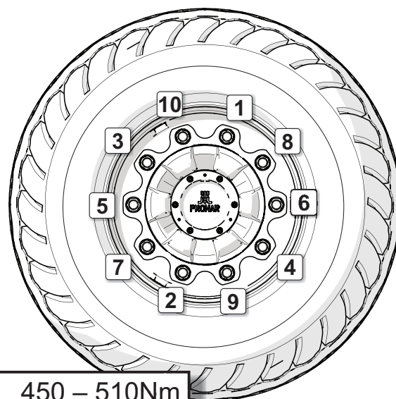
Rysunek 5.15 Zasada dokręcania koła
