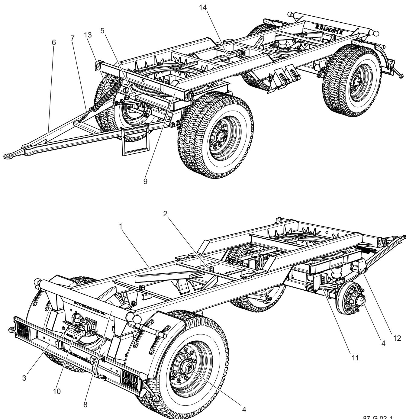
Rysunek 3.2 Podwozie przyczepy
