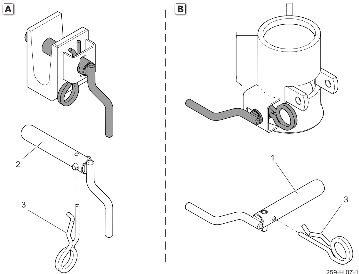
Rysunek 4.9 Ryglowanie sworzni wywrotu
