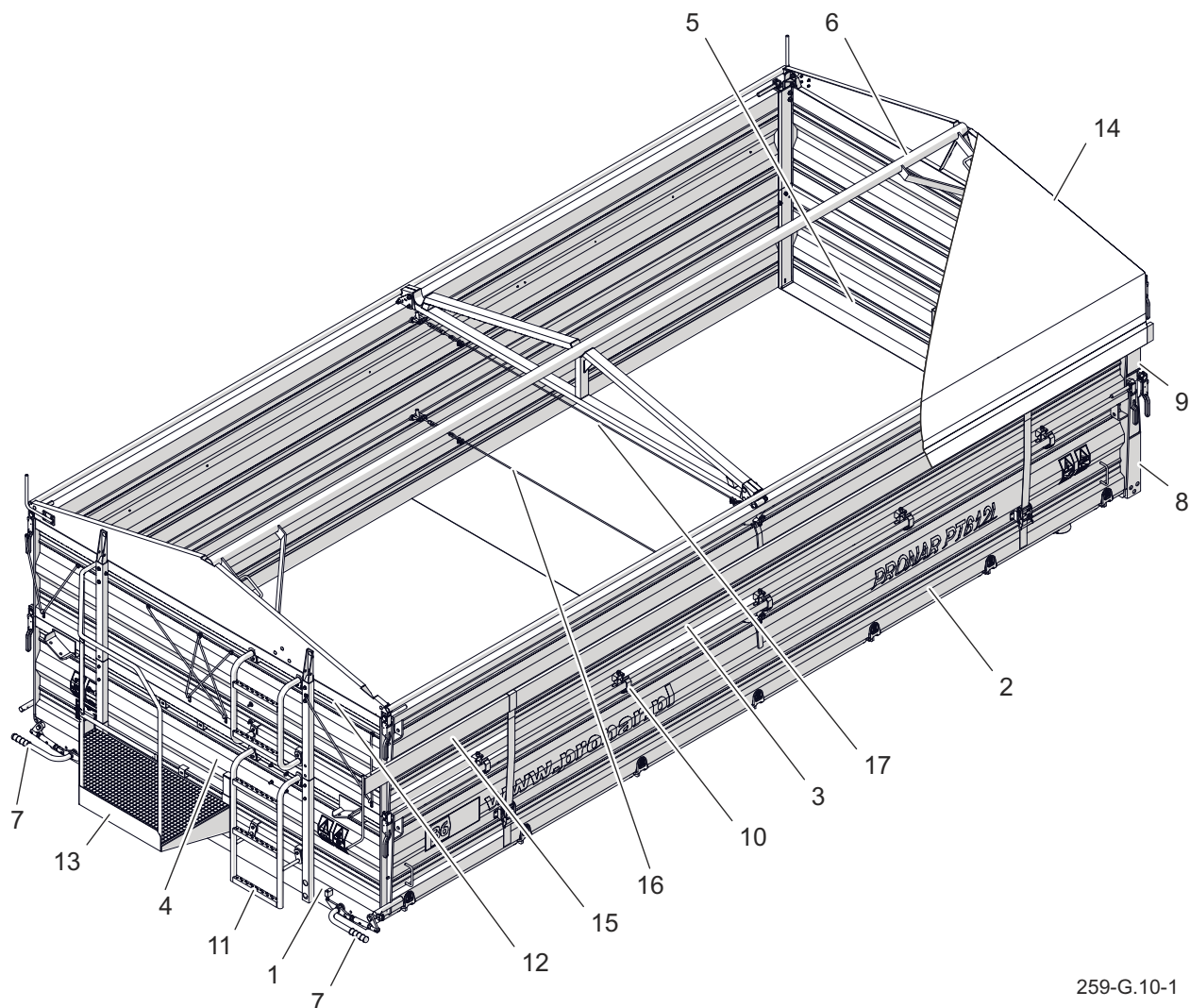
Rysunek 3.3 Skrzynia ładunkowa
