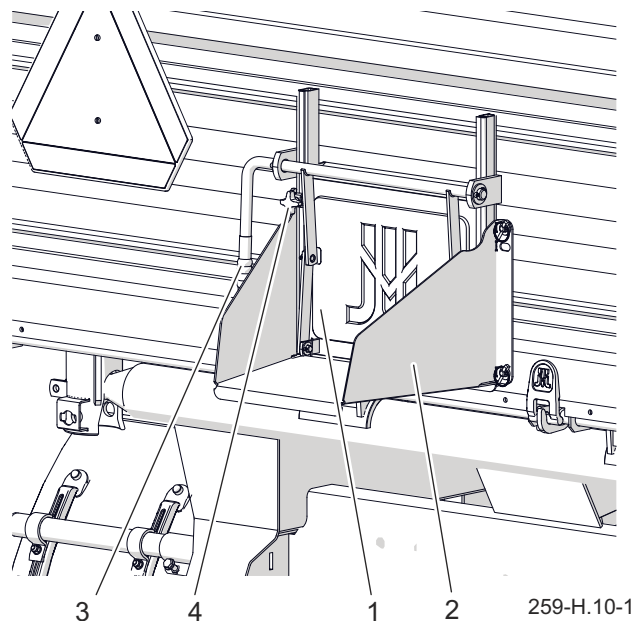
Rysunek 4.11 Zasuwa zsywu
