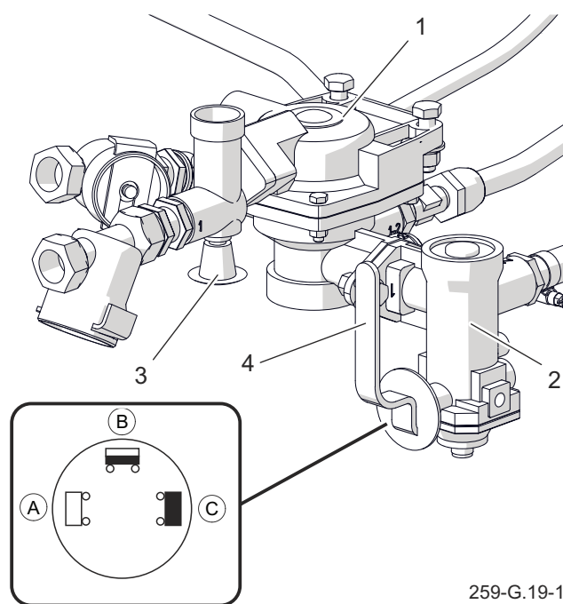
Rysunek 3.5 Zawór sterujący i regulator siły hamowania
