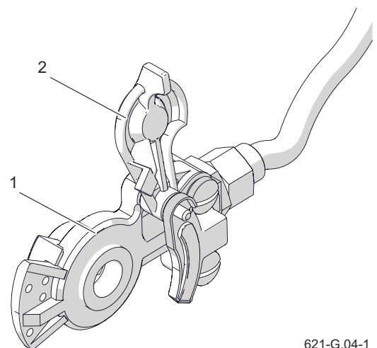
Rysunek 3.9 Przyłącze pneumatyczne (1) korpus przyłączy (2) przykrywka przyłączy
