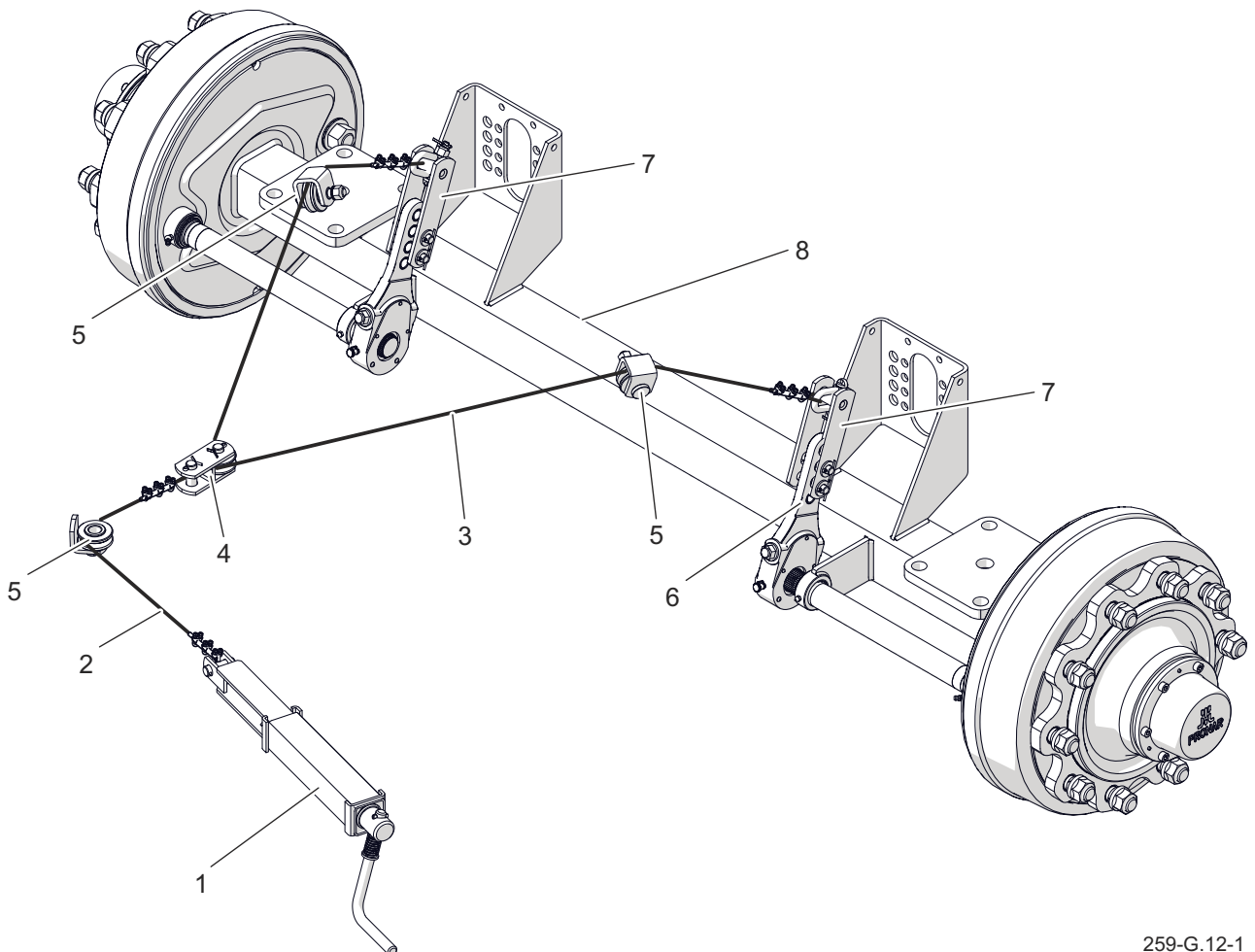
Rysunek 3.12 Hamulec postojowy
