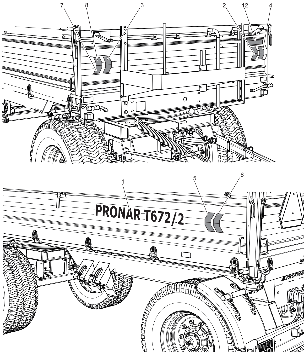
Rysunek 2.3 Rozmieszczenie nalepek informacyjnych i ostrzegawczych
