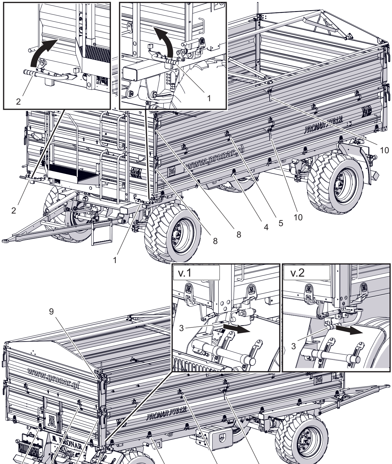
Rysunek 4.13 Obsługa plandeki
