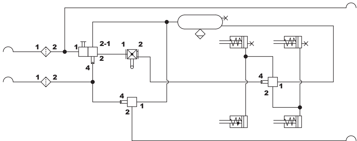
Rysunek 3.8 Schemat instalacji hamulcowej pneumatycznej 2-przewodowej ALB
