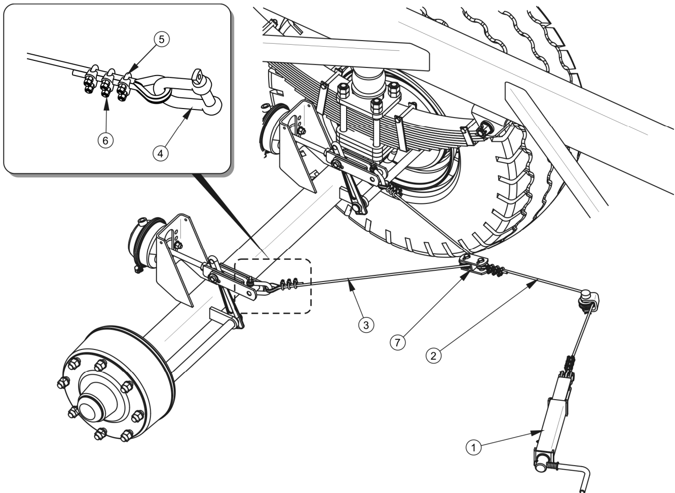
Obrázek 5.5 Seřízení napnutí lanka parkovací brzdy
