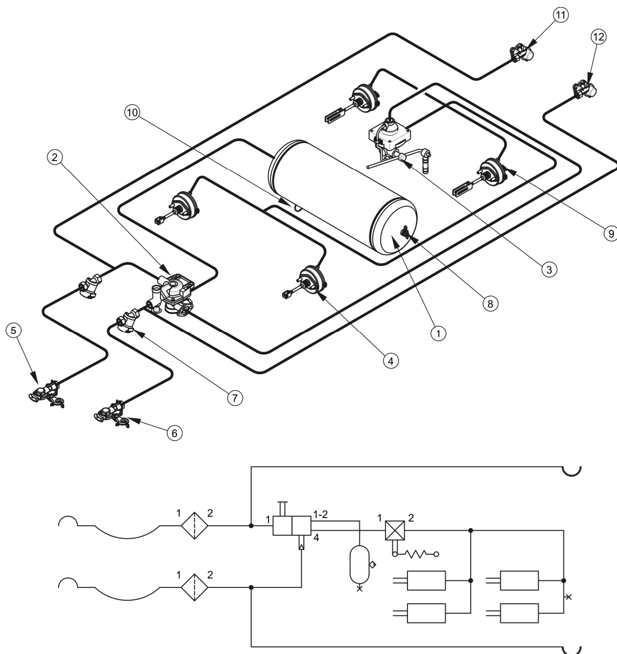
Obrázek 3.7 Konstrukce a schéma vzduchové brzdové dvouhadicové instalace s automatickým regulátorem
