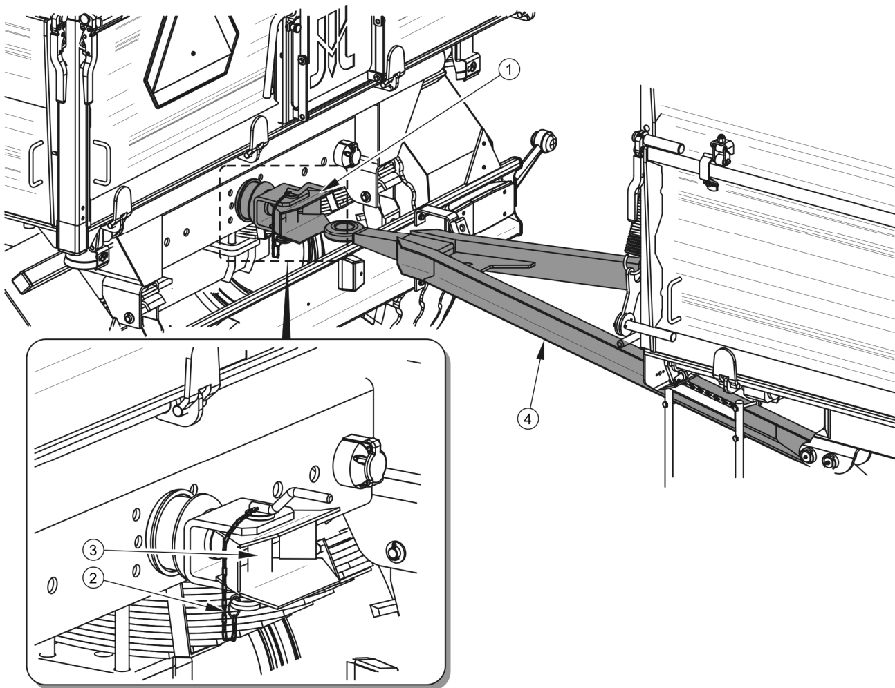
Obrázek 4.2 Agregace druhého přívěsu
