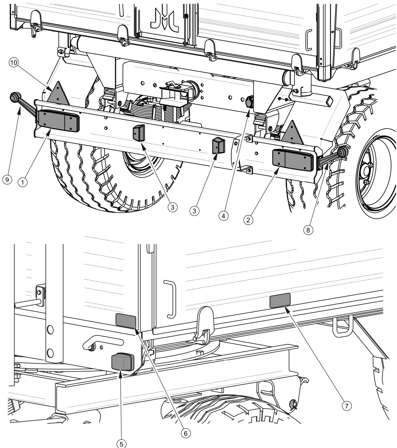
Obrázek 5.8 Součástí elektrovybavení a odrazová světla.
