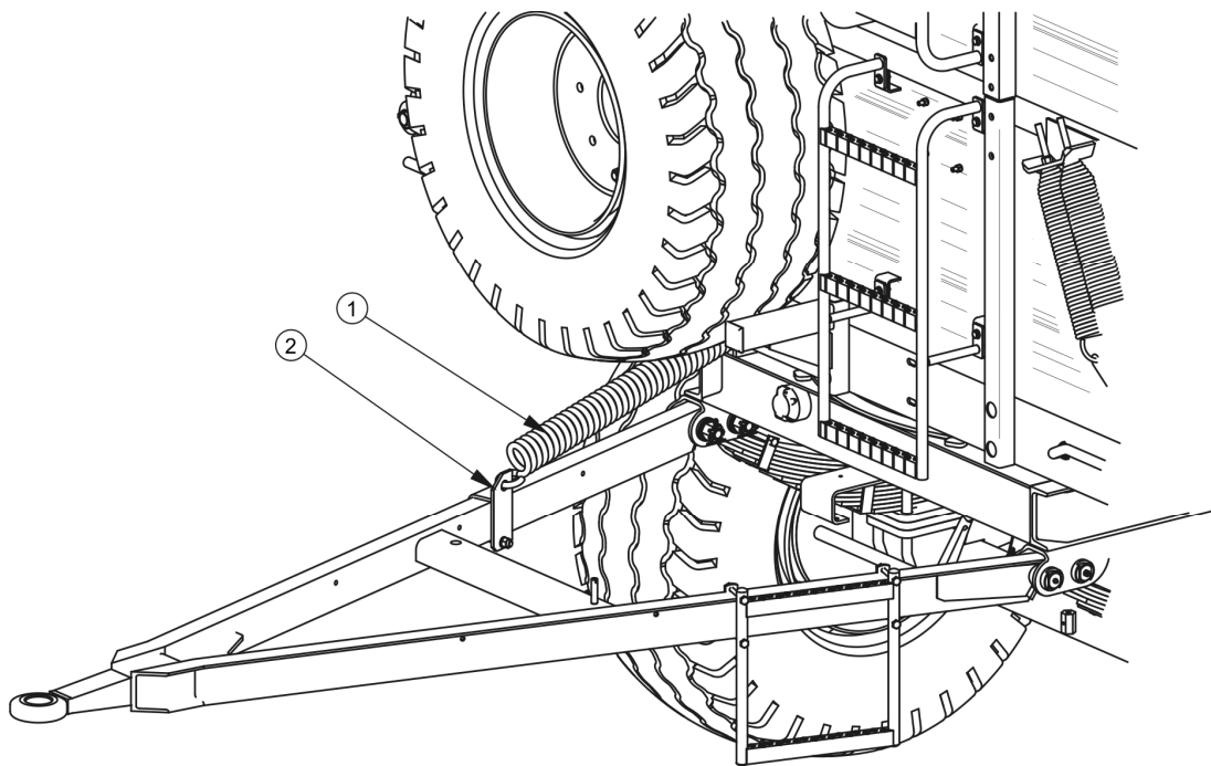
Obrázek 5.13 Seřízení polohy oje
