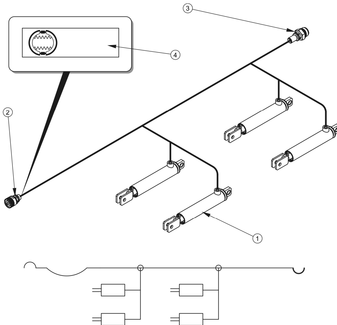
Obrázek 3.6 Konstrukce a schéma hydraulické brzdové instalace
