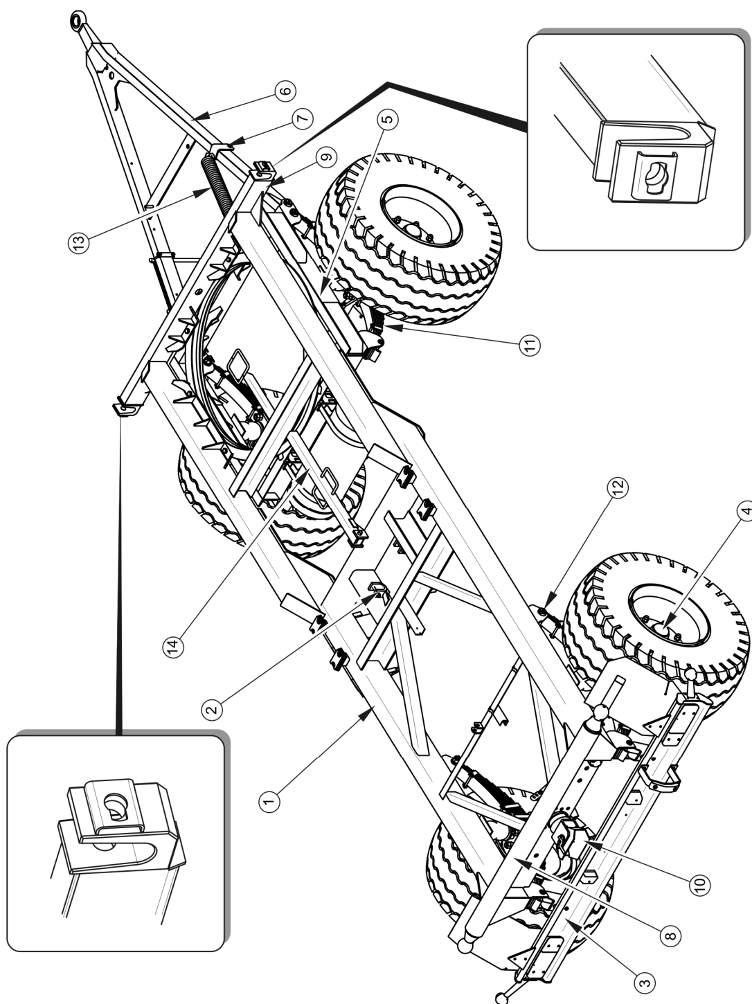
Obrázek 3.1 Podvozek přívěsu
