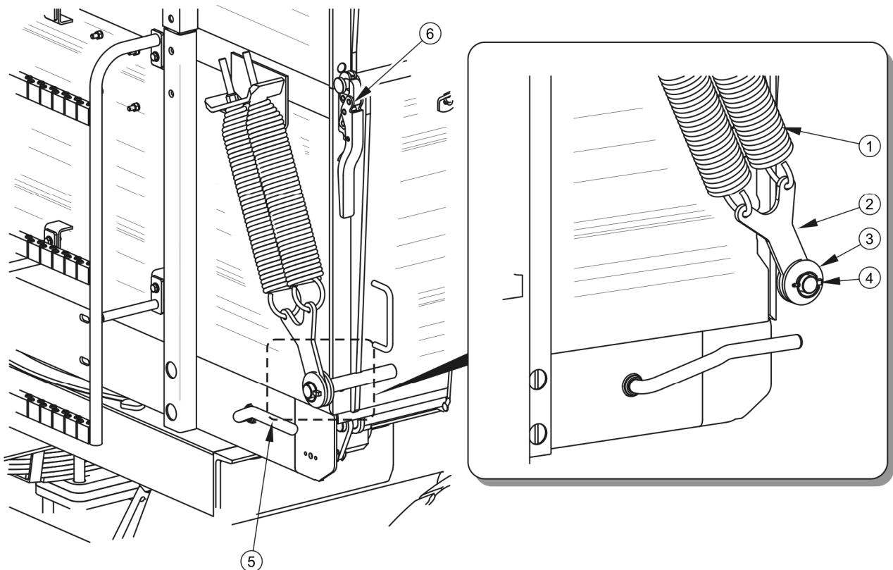
Obrázek 4.7 Kotevní mechanismus
