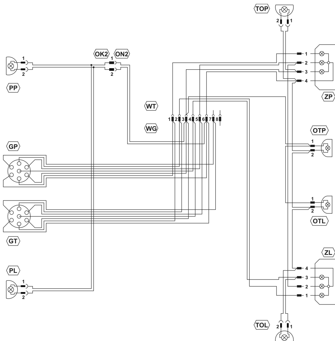
Obrázek 3.10 Ideové schéma elektroinstalace
