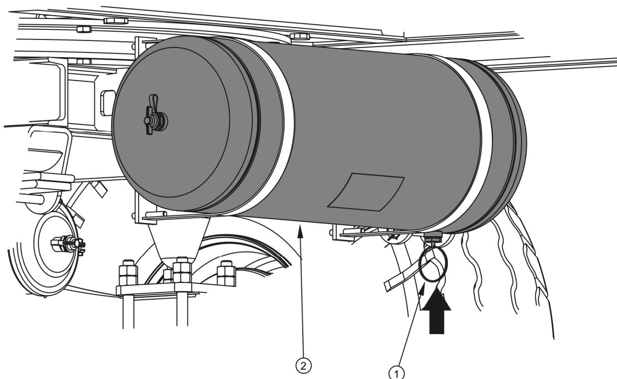
Obrázek 5.7 Odvodňování vzdušníku
