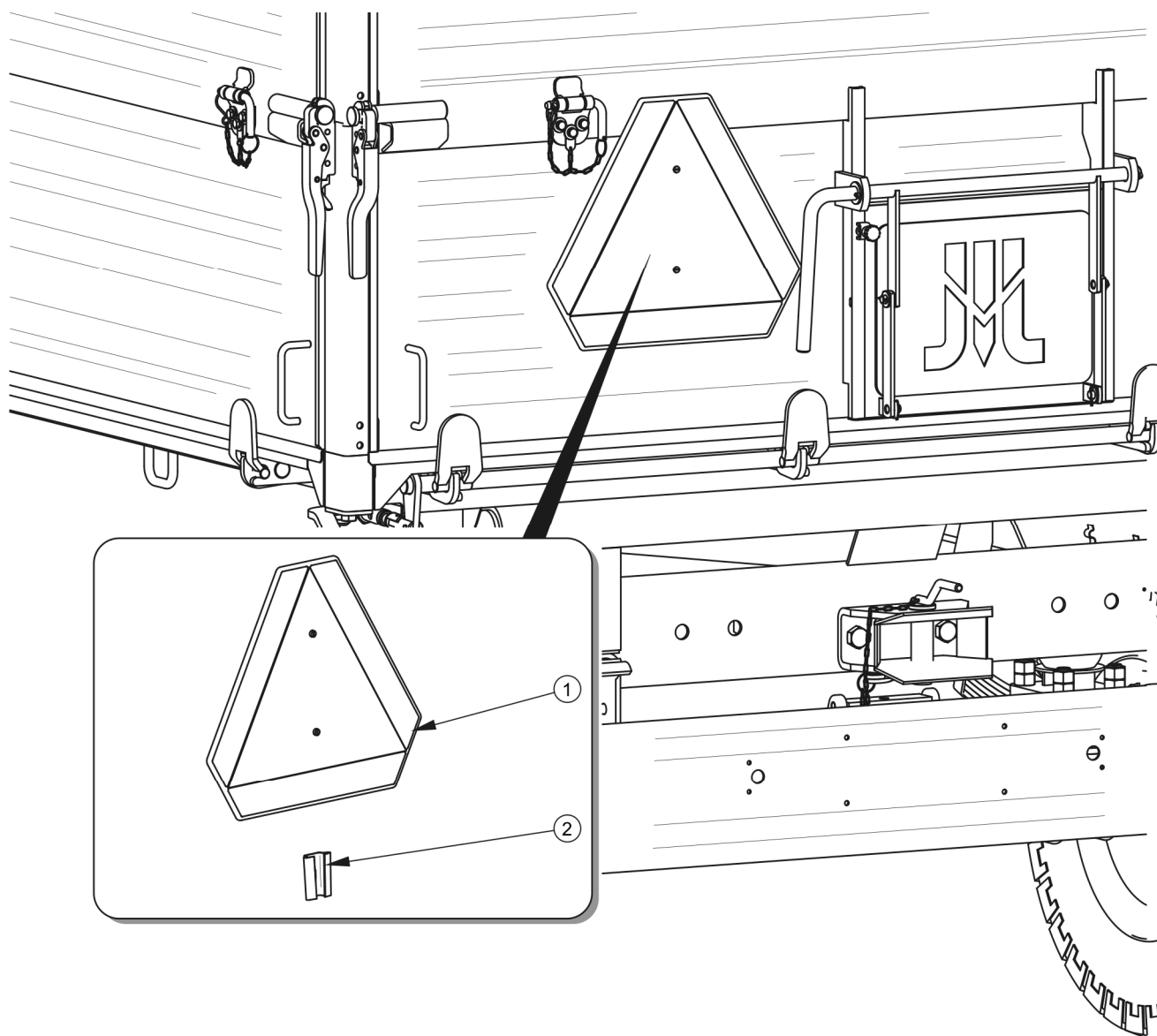
Obrázek 2.2 Místo montáže tabulky označující pomalá vozidla
