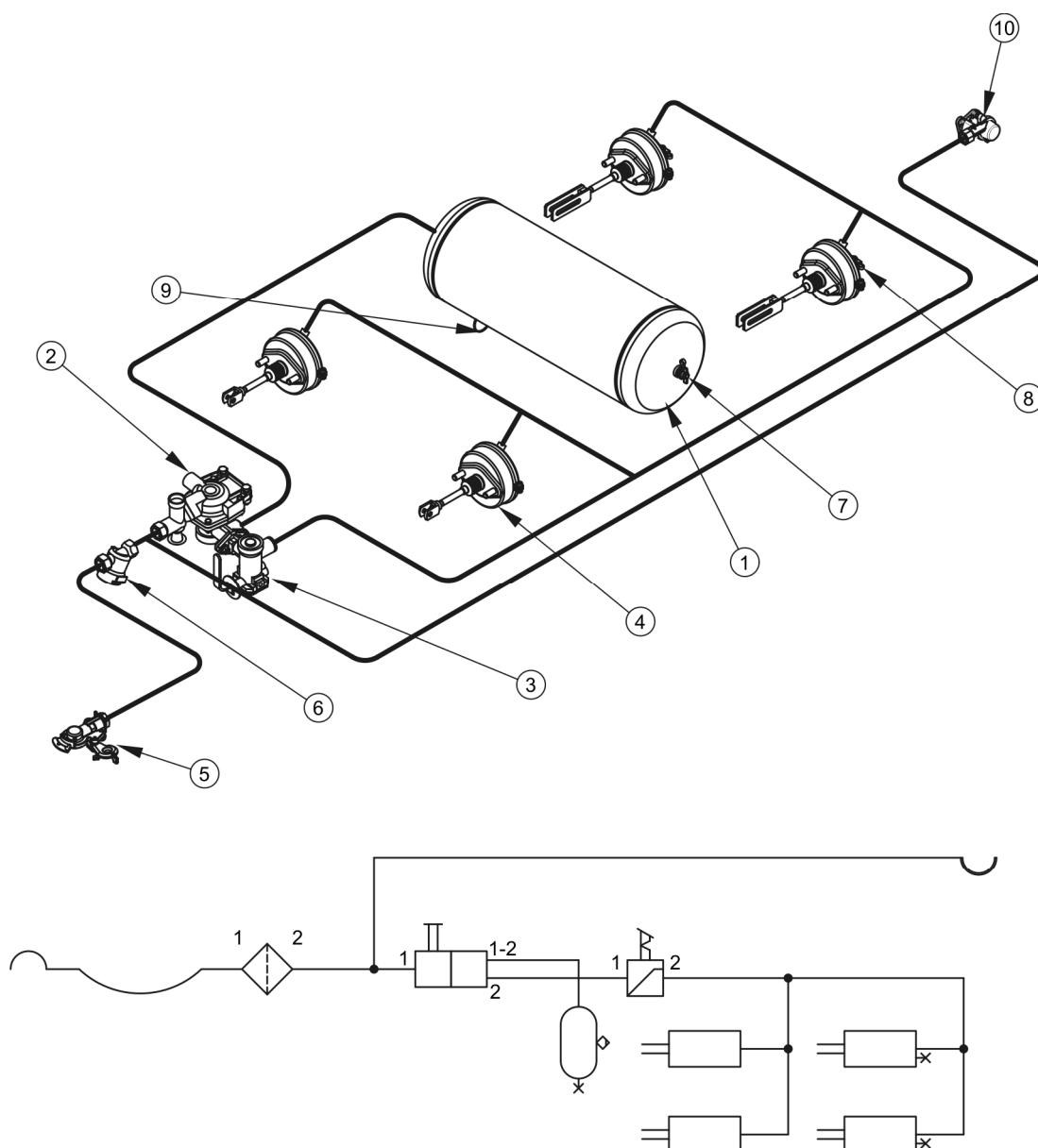
Obrázek 3.5 Konstrukce a schéma vzduchové jednohadicové brzdové instalace
