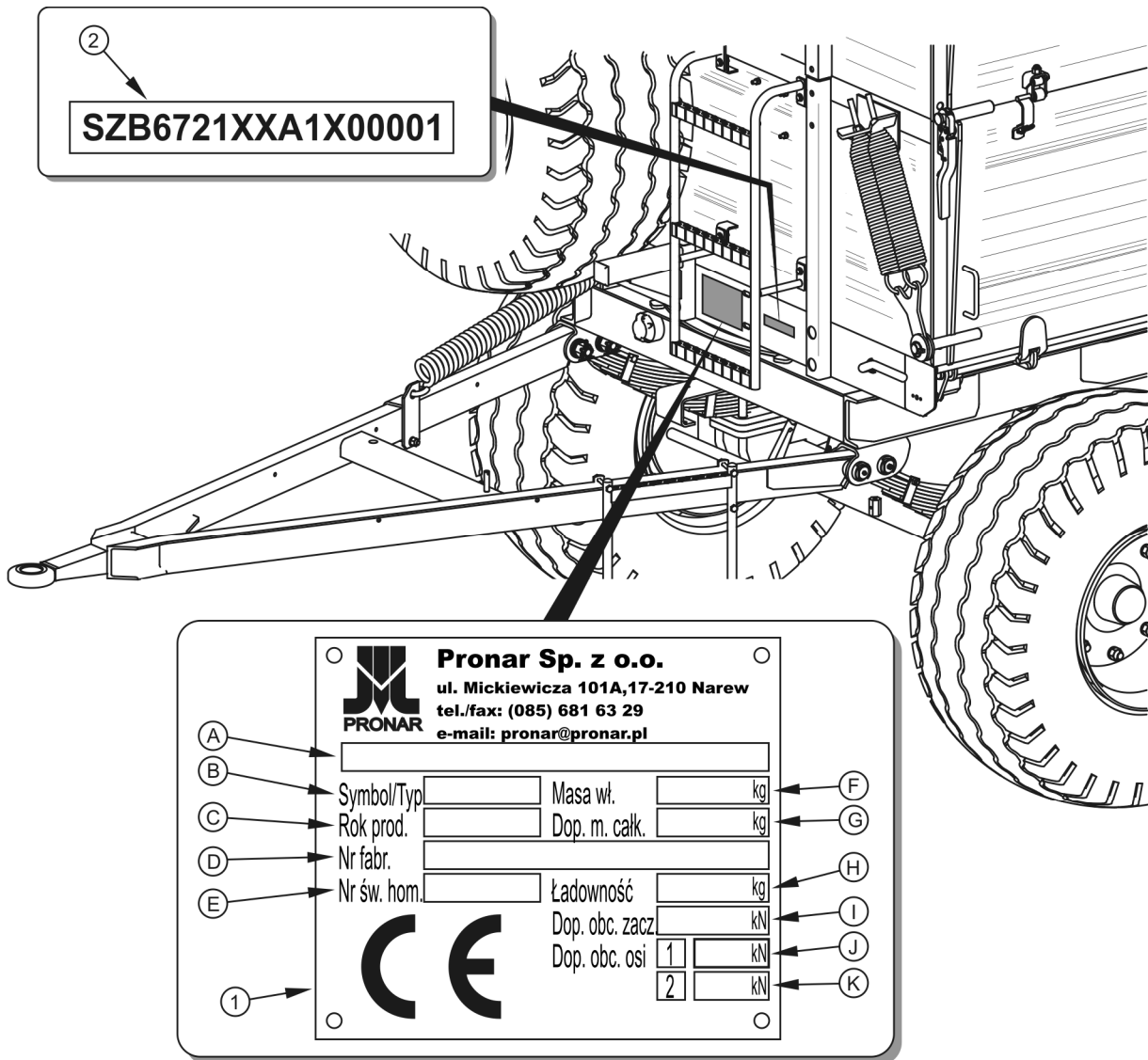
Obrázek 1.1 Místa umístění údajového štítku a vyznačení výrobního čísla
