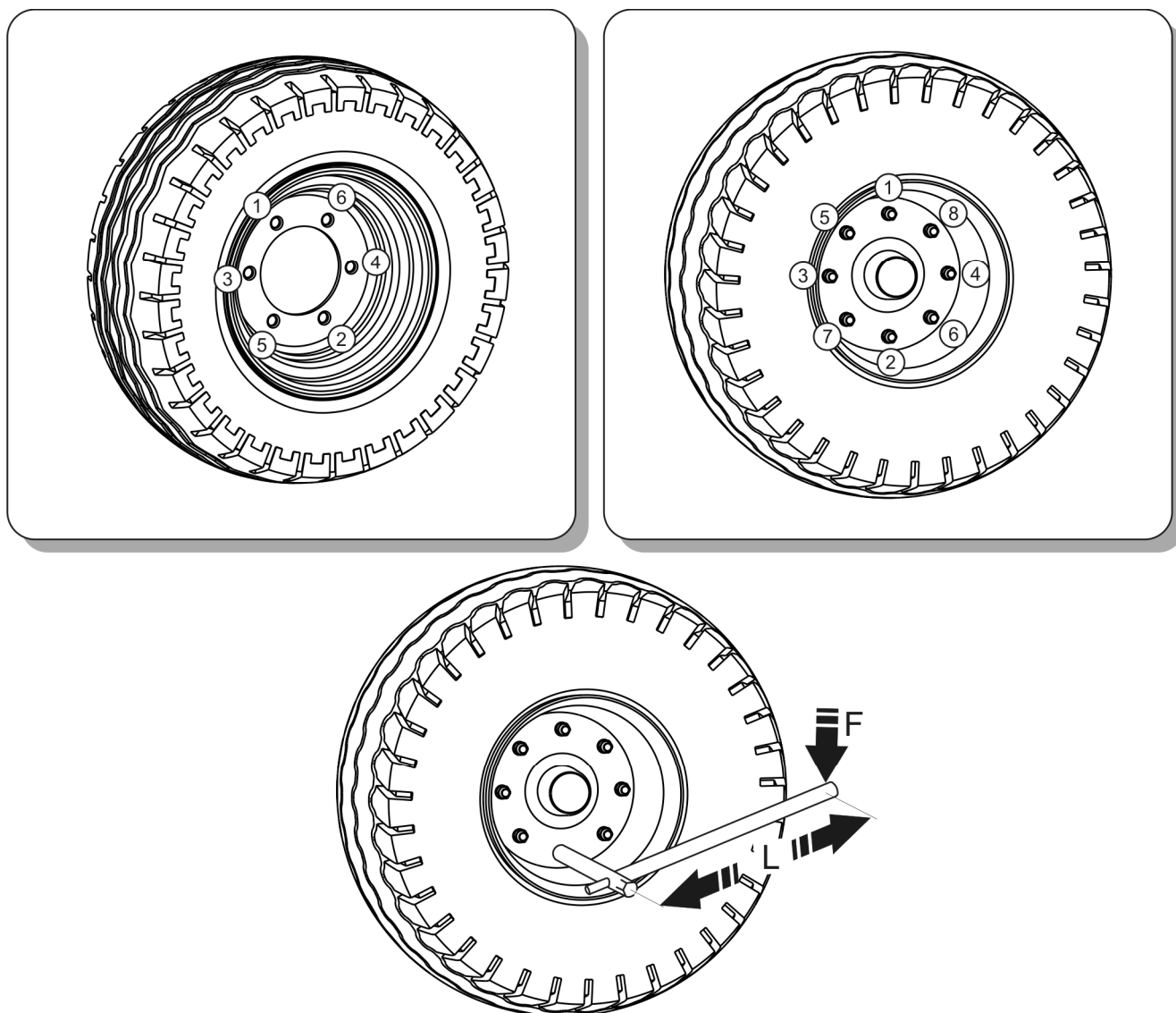
Obrázek 5.3 Pořadí dotahování matic, nápravy z 6 a 8 jehlicemi M18x1.5
