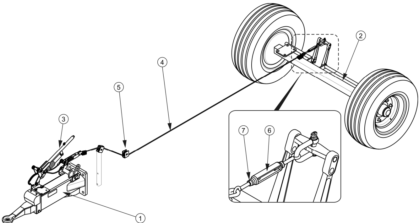
РИСУНОК 5.5 Регулирование натяжения троса тормоза инерционного типа
