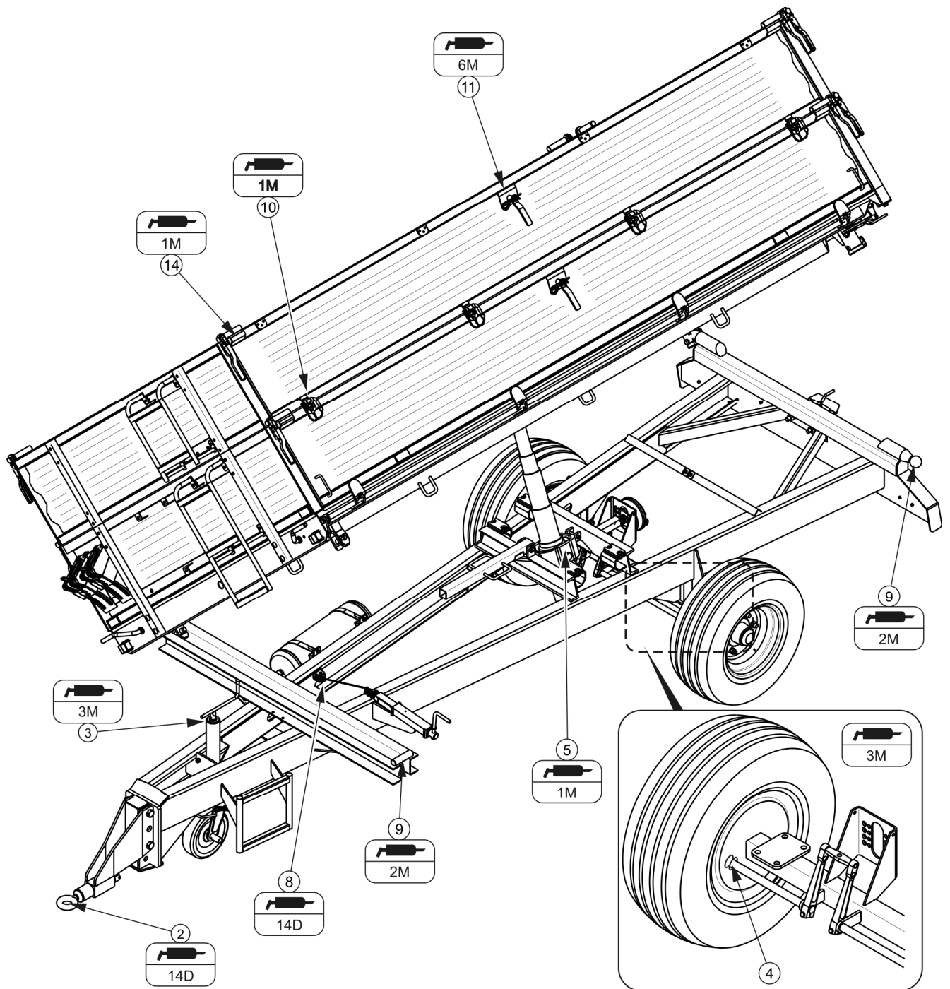
РИСУНОК 5.9 Точки смазки прицепа, часть 1
