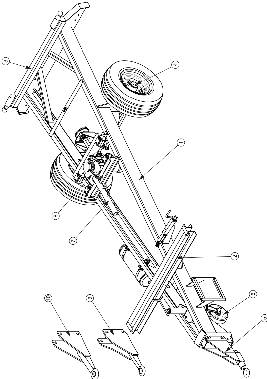
РИСУНОК 3.1 Шасси прицепа с нижним дышлом
