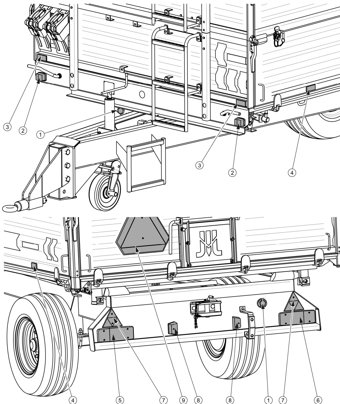
РИСУНОК 3.15 Размещение элементов электрической системы и светоотражающей сигнализации
