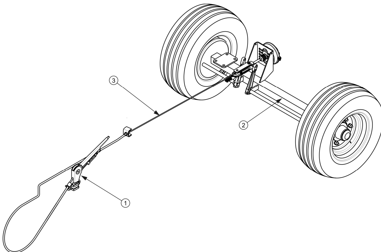
РИСУНОК 3.14 Ручной рычажный тормоз
