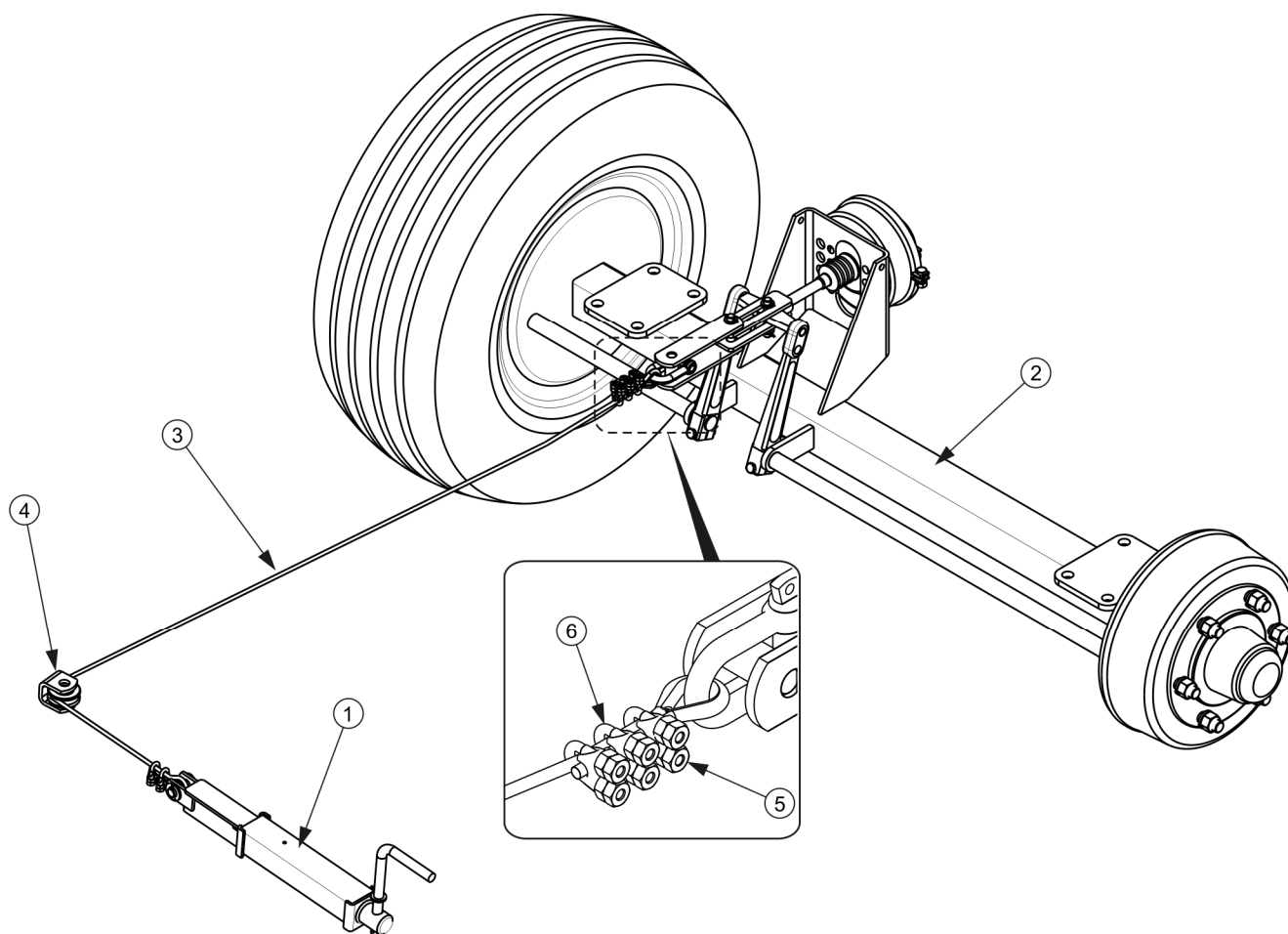
РИСУНОК 5.6 Регулирование натяжения троса стояночного тормоза
