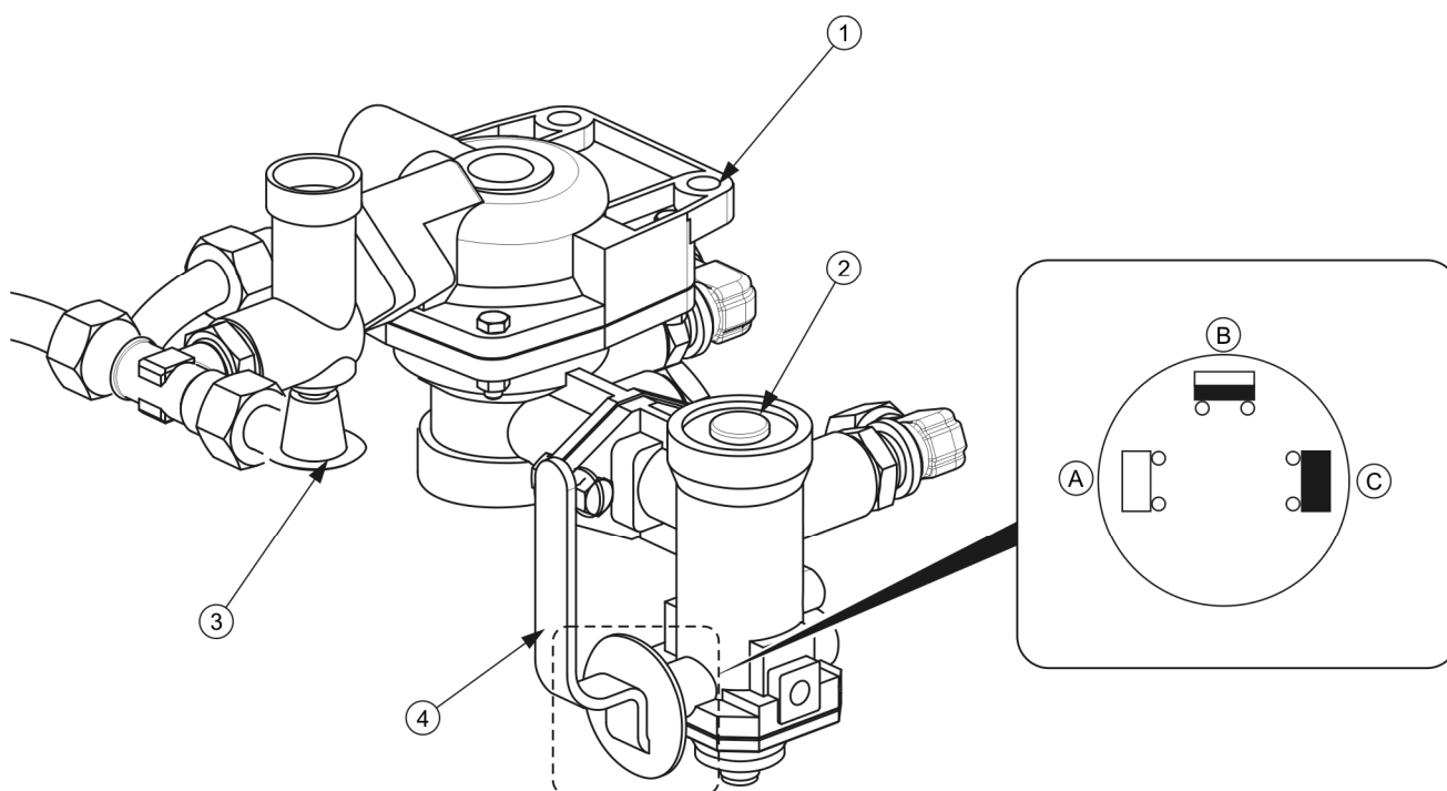
РИСУНОК 3.11 Управляющий клапан и регулятор силы торможения
