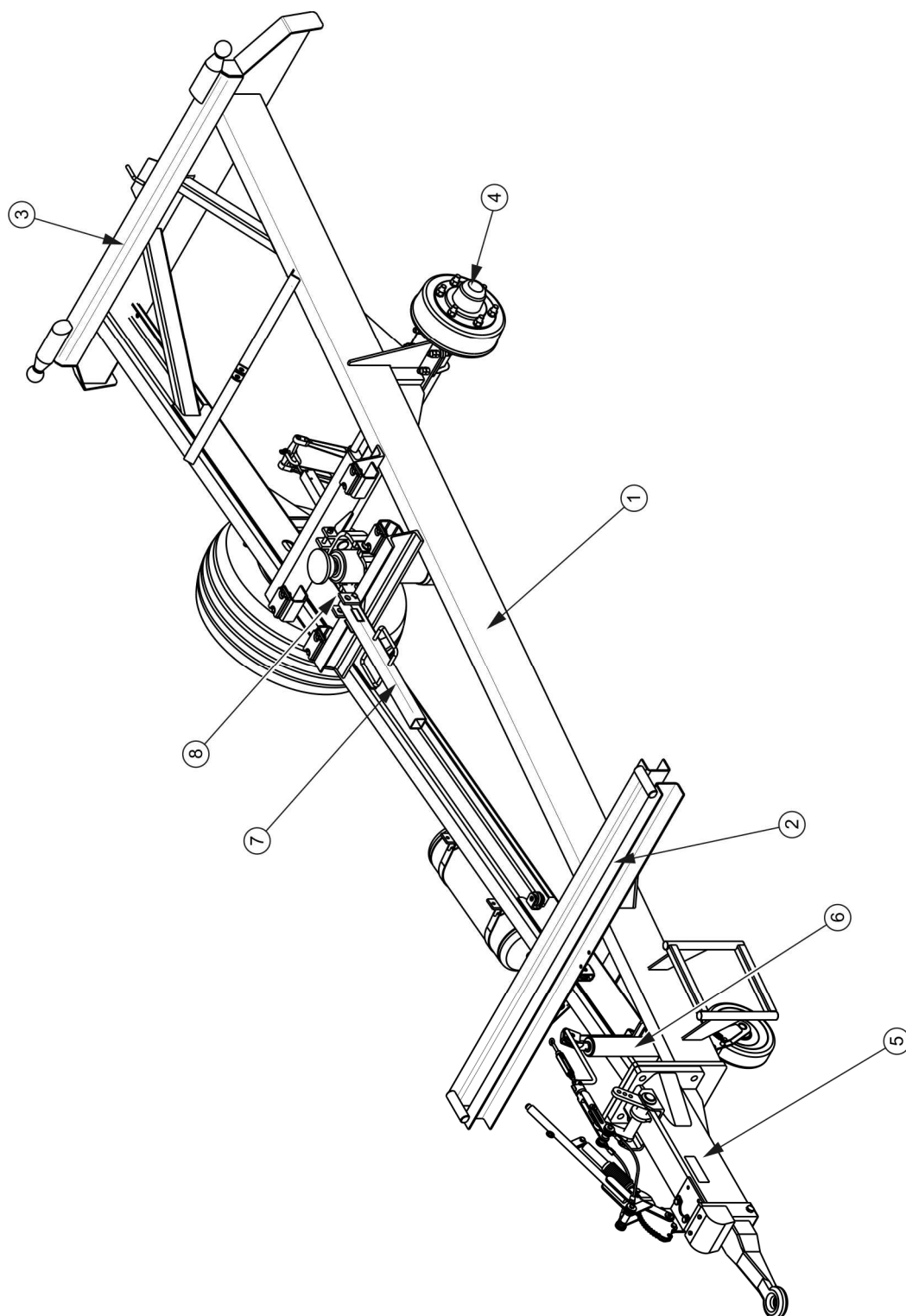
РИСУНОК 3.3 Шасси прицепа с инерционным дышлом
