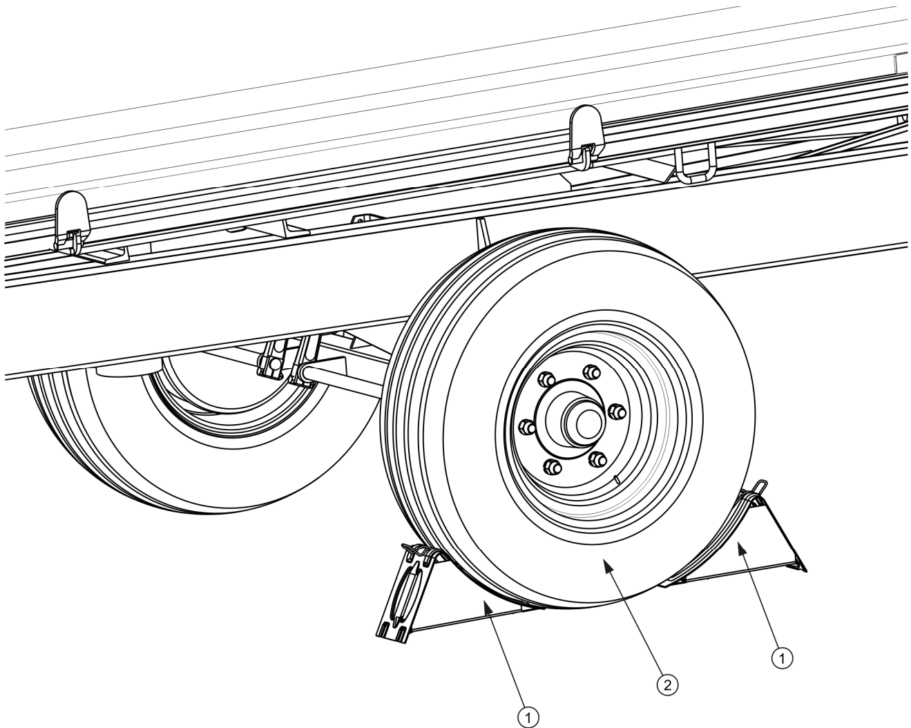
РИСУНОК 2.1 Способ установки клиньев
