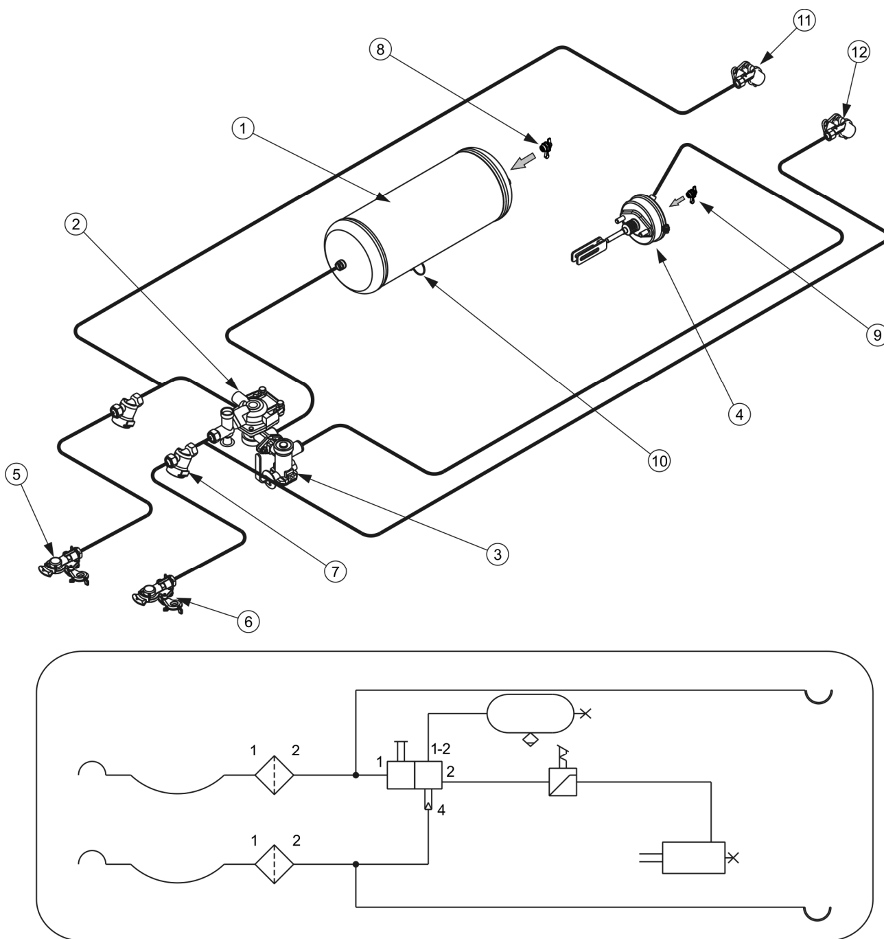
РИСУНОК 3.7 Устройство и схема пневматической двухпроводной тормозной системы
