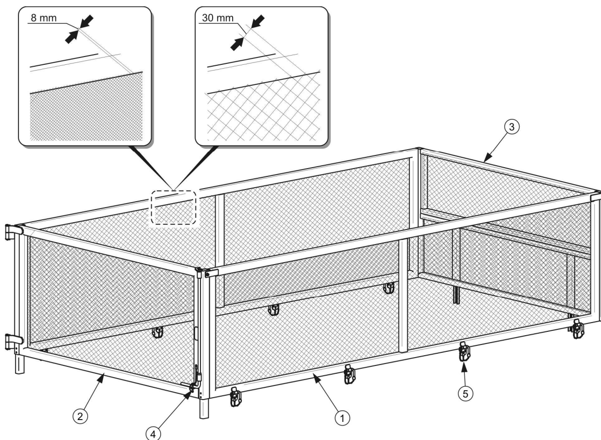
РИСУНОК 3.6 Сетчатые надставки высотой 1,000 мм
