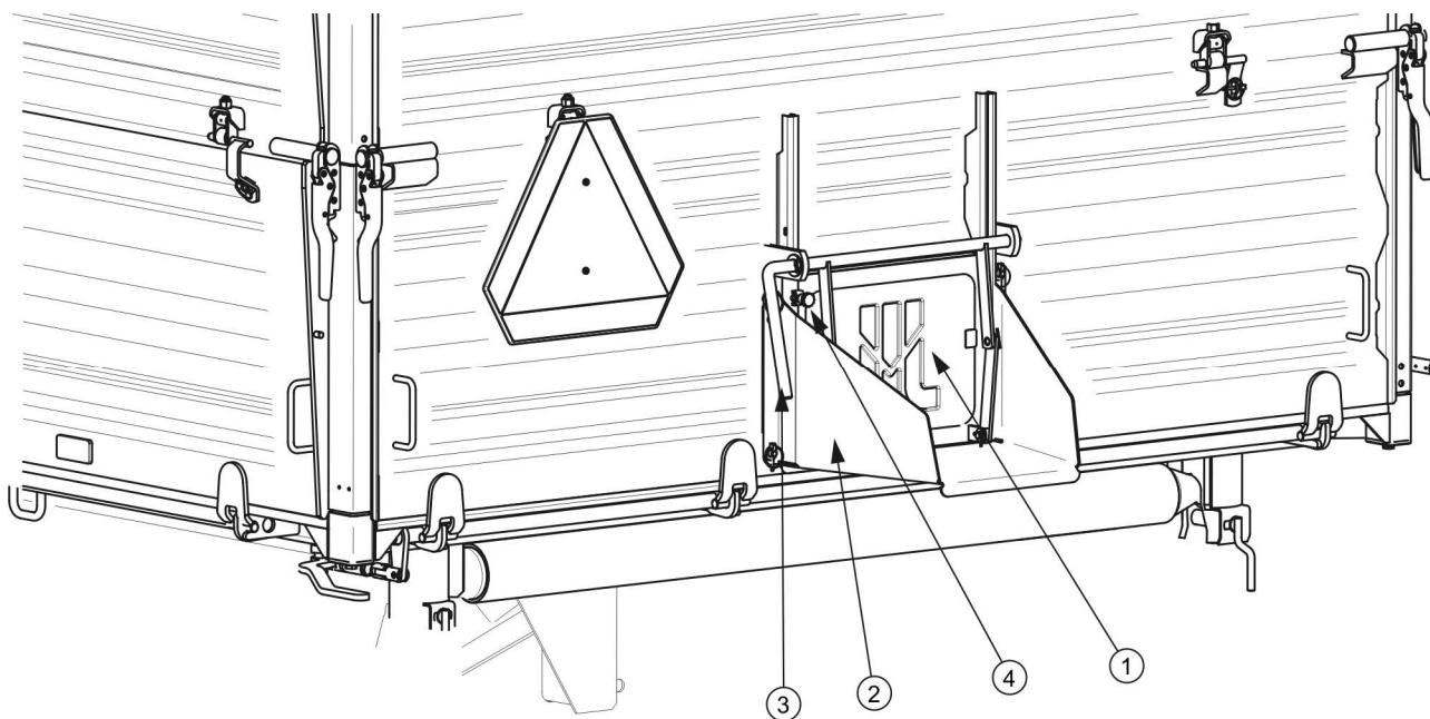
РИСУНОК 3.5 Задний борт
