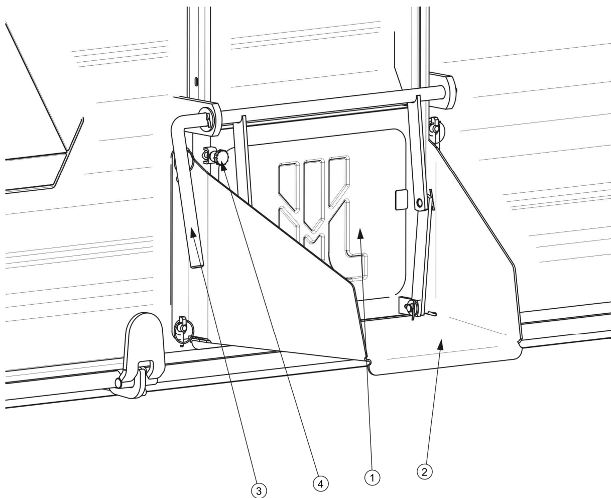
РИСУНОК 4.6 Разгрузочный люк
