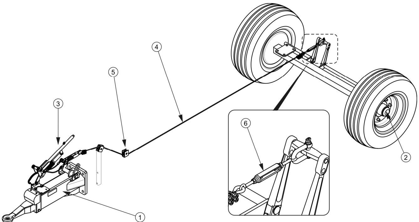
РИСУНОК 3.10 Тормоз инерционного типа
