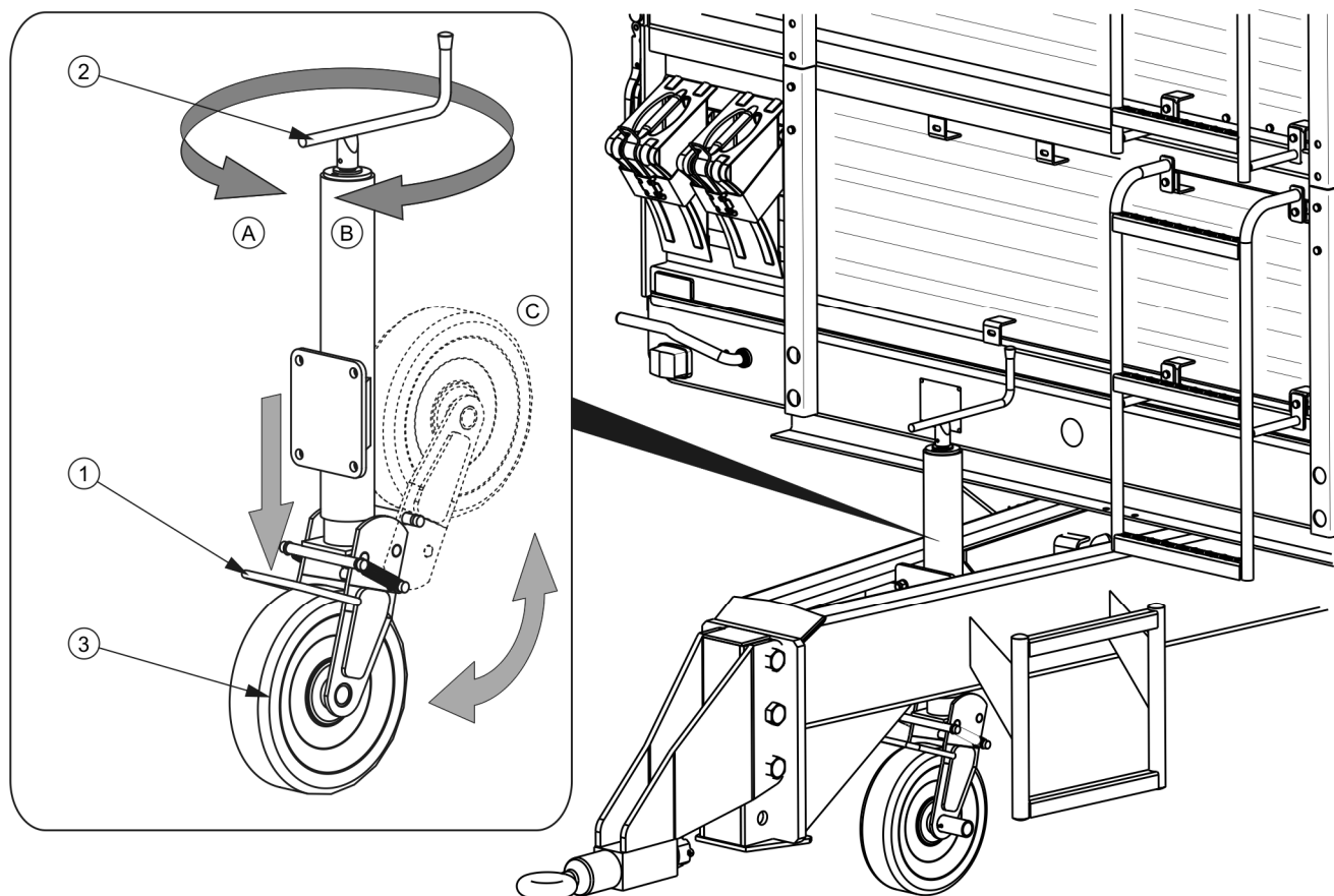
РИСУНОК 4.2 Подсоединение к трактору
