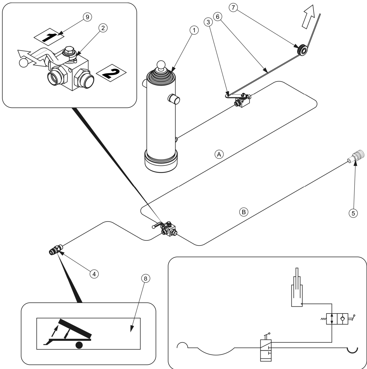
РИСУНОК 3.12 Устройство и схема гидравлической системы опрокидывания
