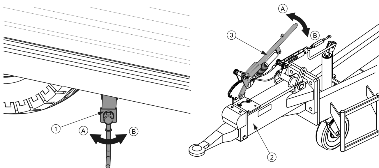
РИСУНОК 4.1 Стояночный тормоз
