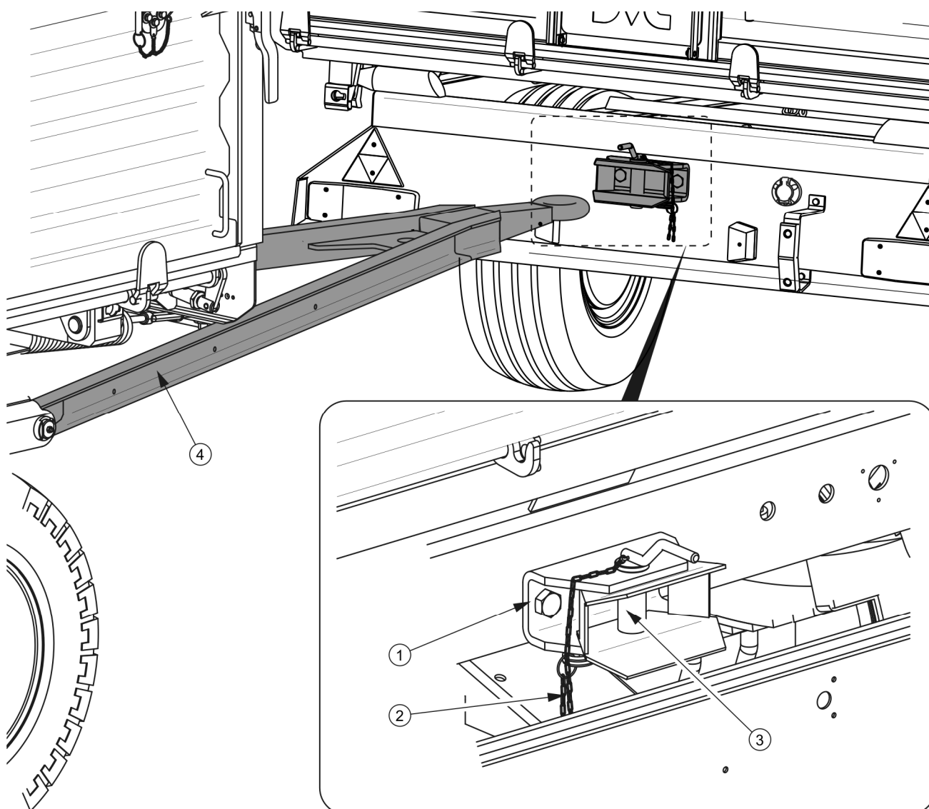
РИСУНОК 4.3 Агрегирование второго прицепа
