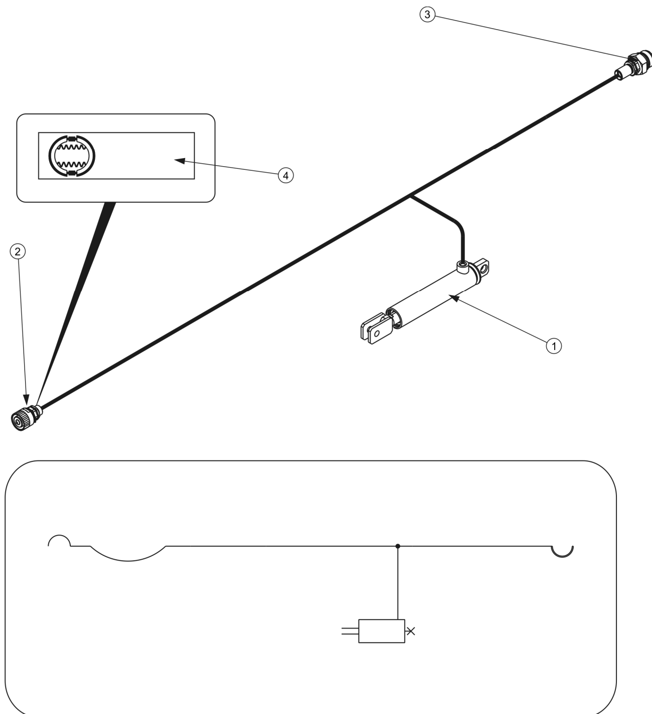
РИСУНОК 3.9 Устройство и схема гидравлической тормозной системы
