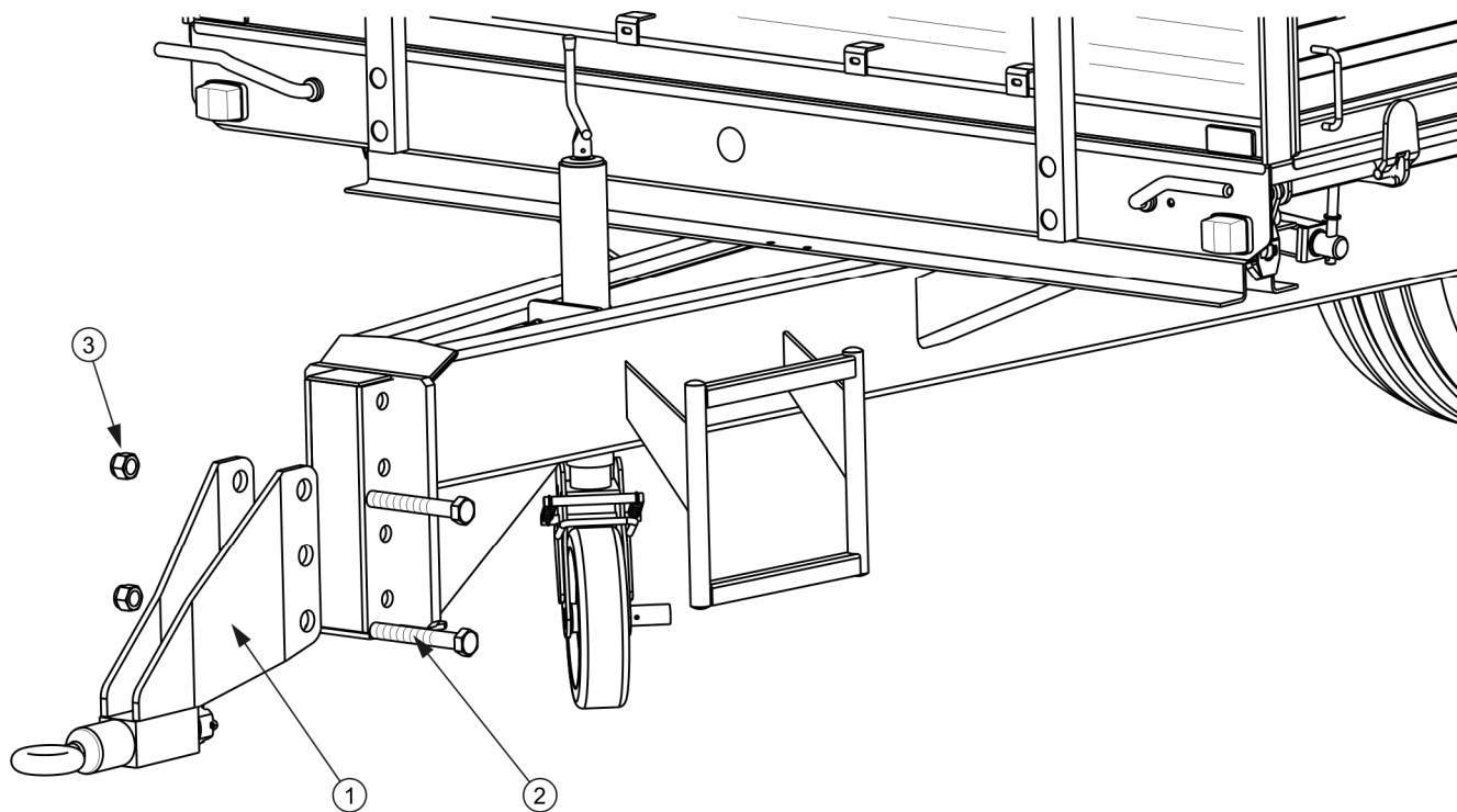
РИСУНОК 5.13 Регулирование положения дышла
