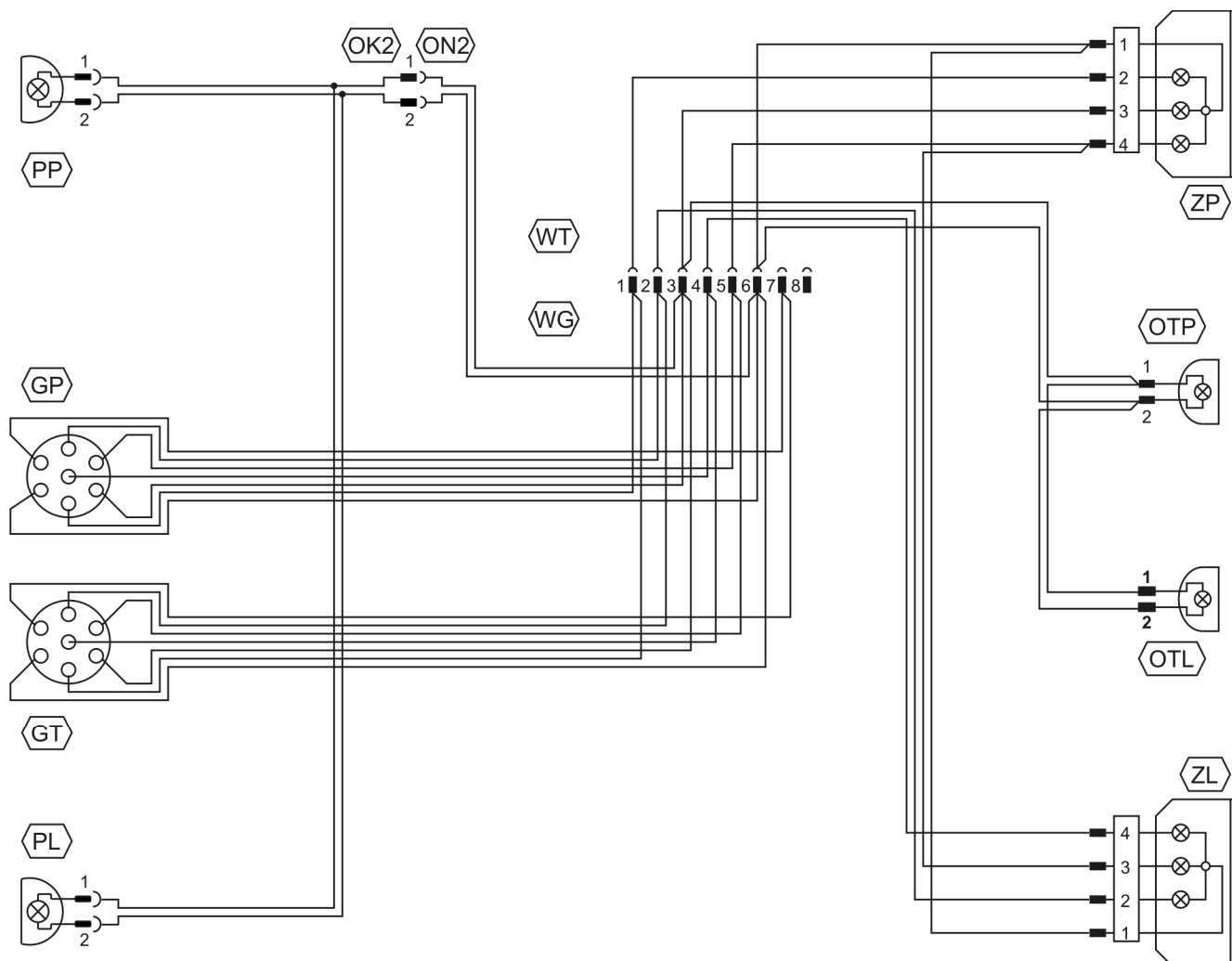
РИСУНОК 3.16 Принципиальная схема электрической системы
