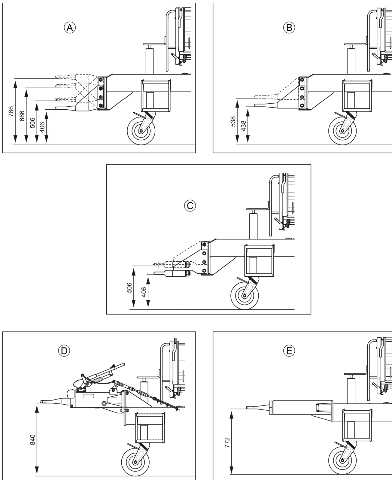
РИСУНОК 5.14 Регулирование положения дышла по высоте
