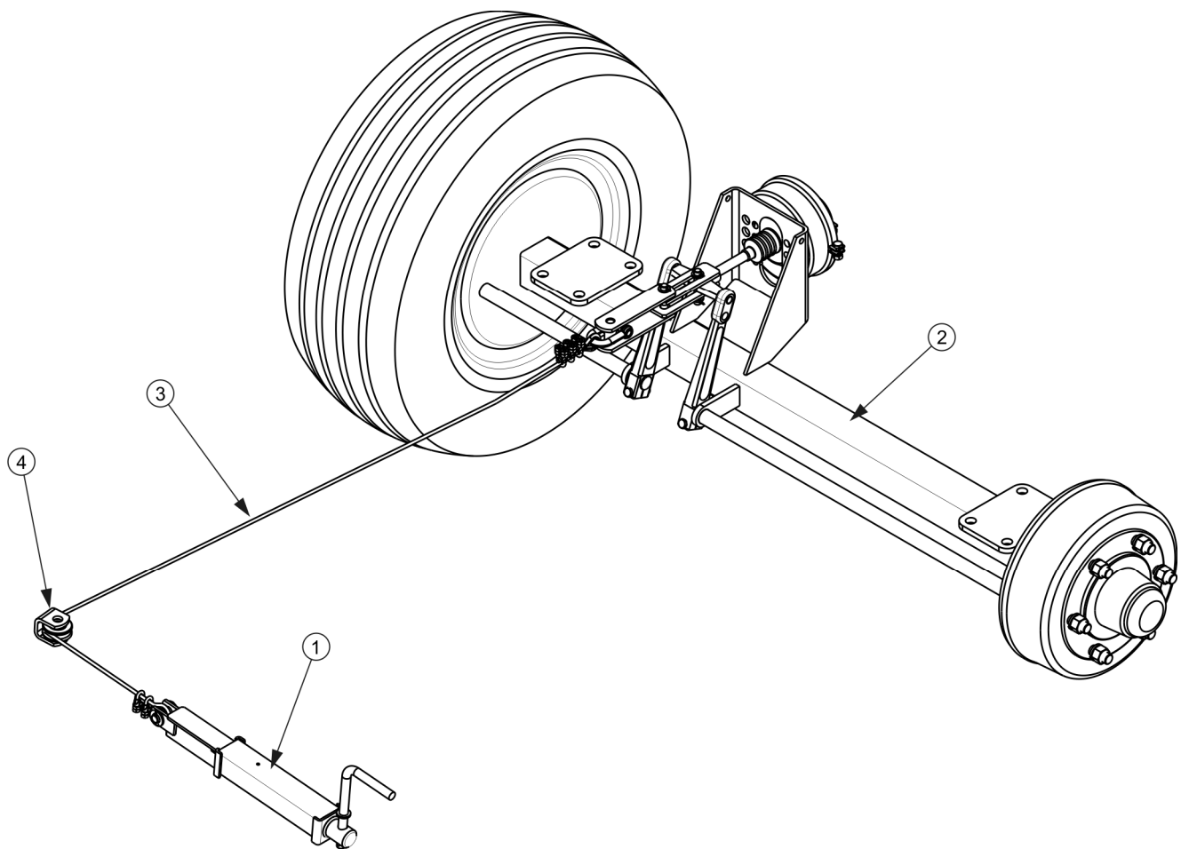
РИСУНОК 3.13 Ручной тормоз с кривошипным механизмом
