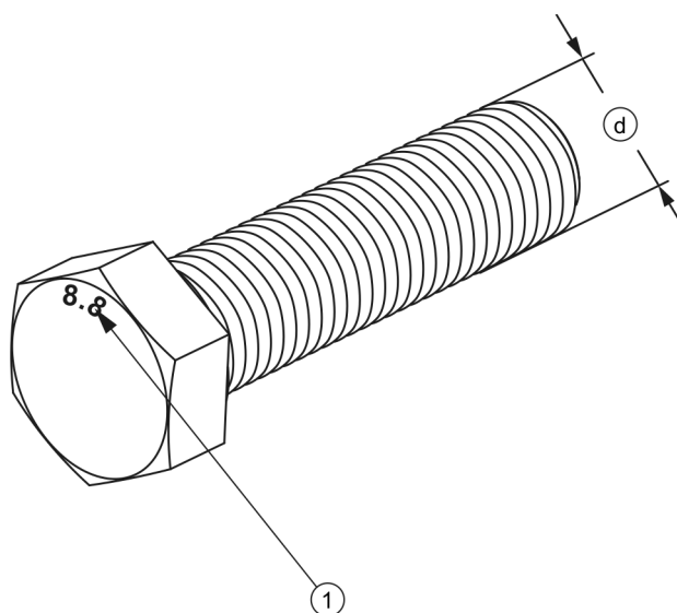
РИСУНОК 5.11 Болт с метрической резьбой
