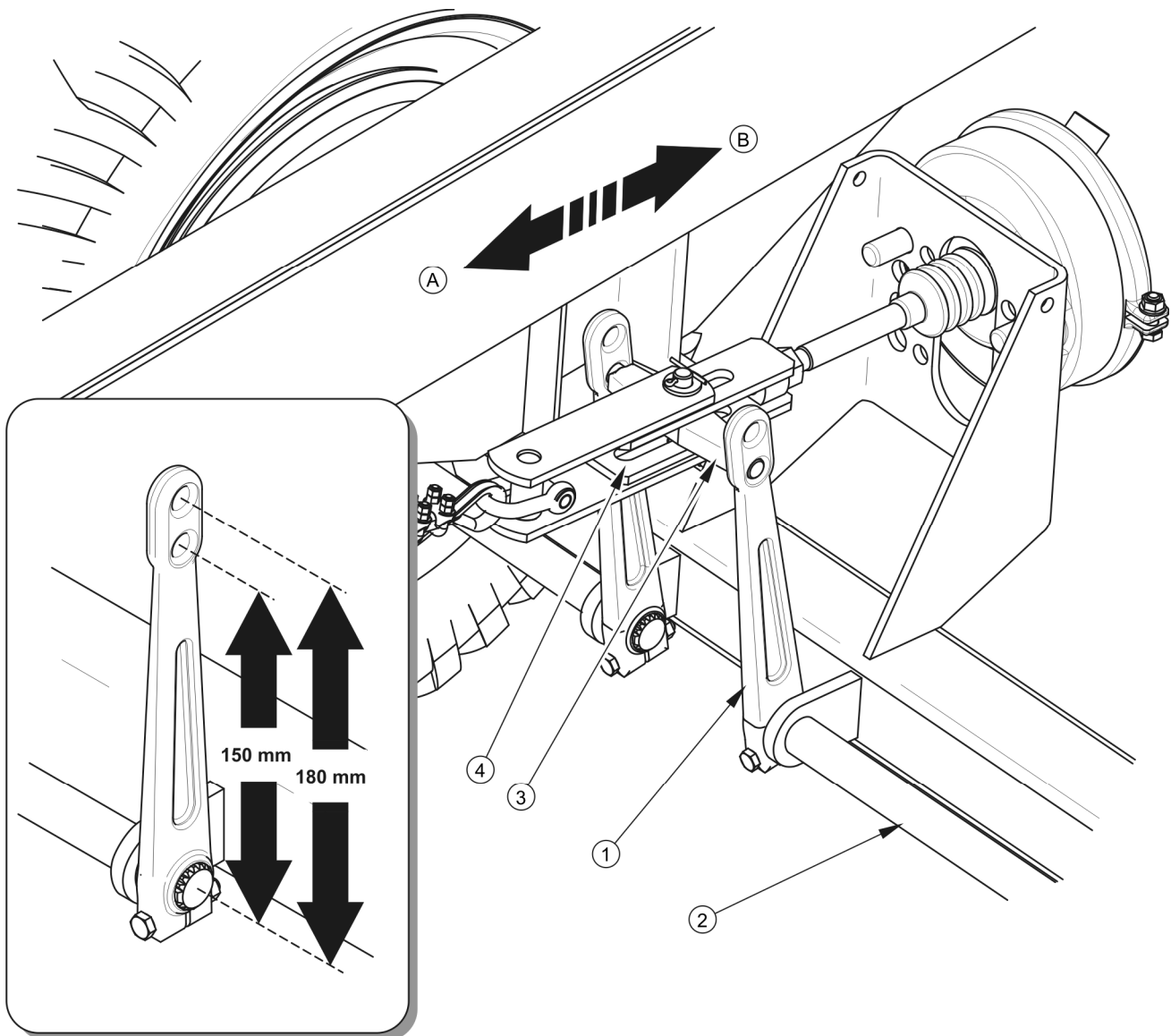
РИСУНОК 5.4 Регулирование механических тормозов ходовых осей
