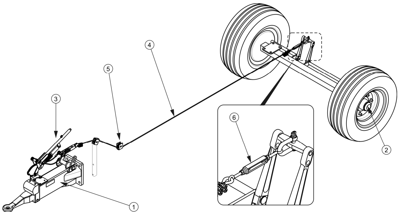
RYСУNEK 3.10 Hamulec najazdowy
