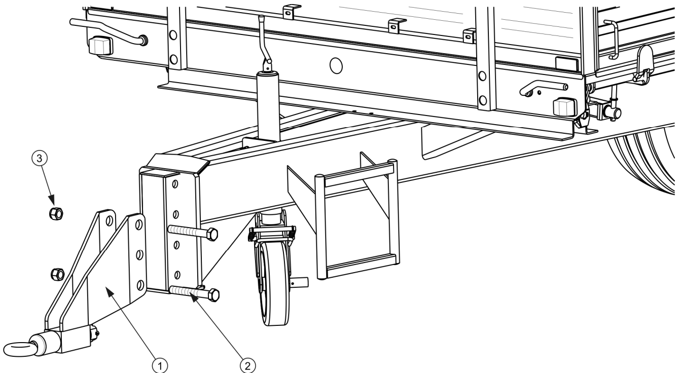
RYSunEK 5.13 Regulacja położenia dyszla
