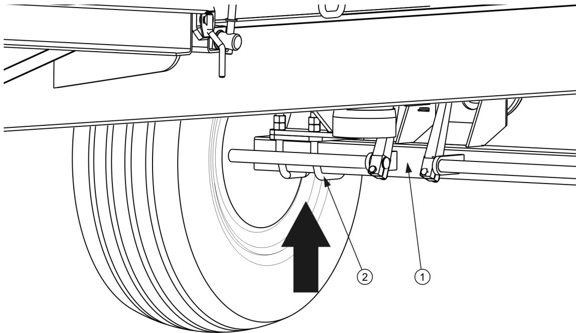
RYSUNEK 5.1 Punkt podparcia podnośnika
