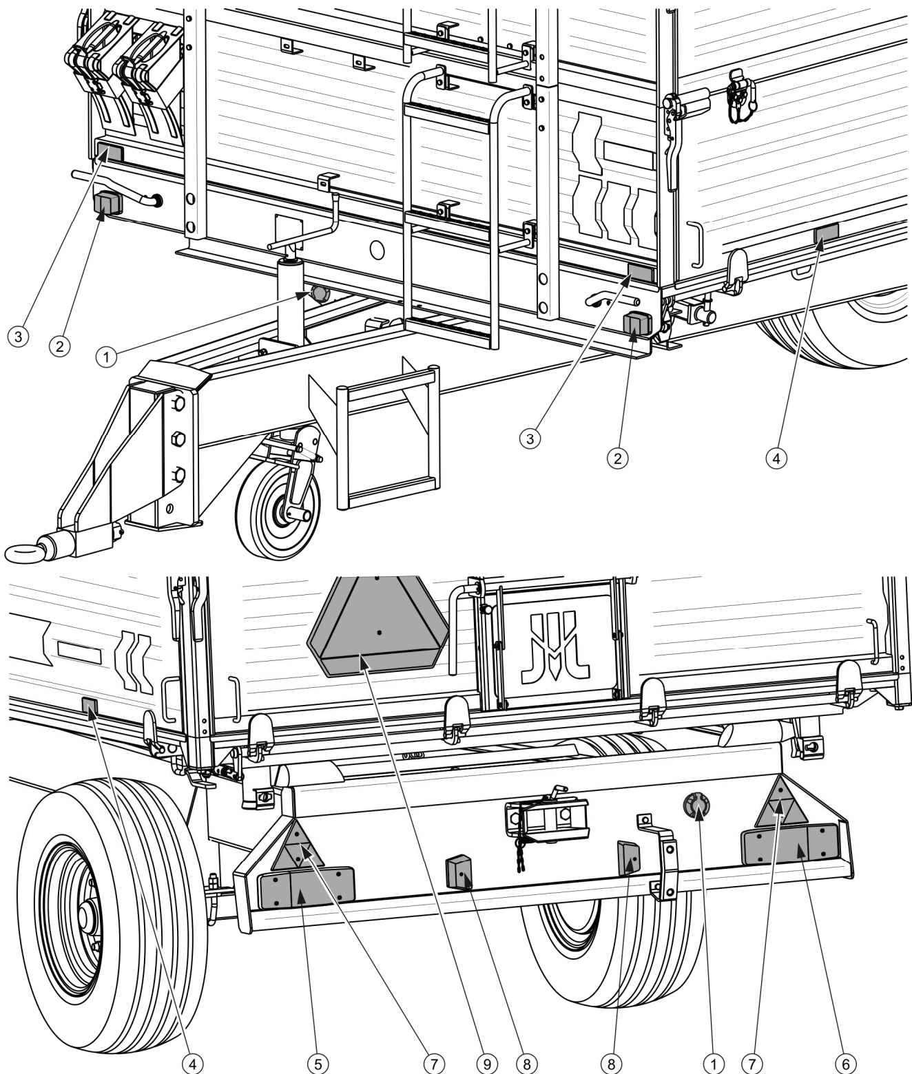
RYСУNEK 3.15 Rozmieszczenie elementów elektrycznych i odblaskowych
