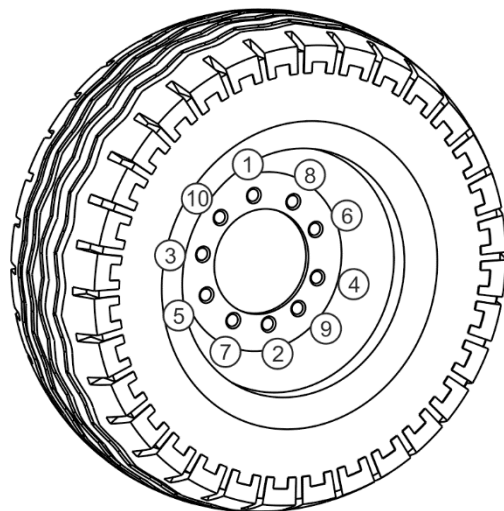
РИСУНОК 5.5 Очередность отвинчивания и завинчивания гаек
