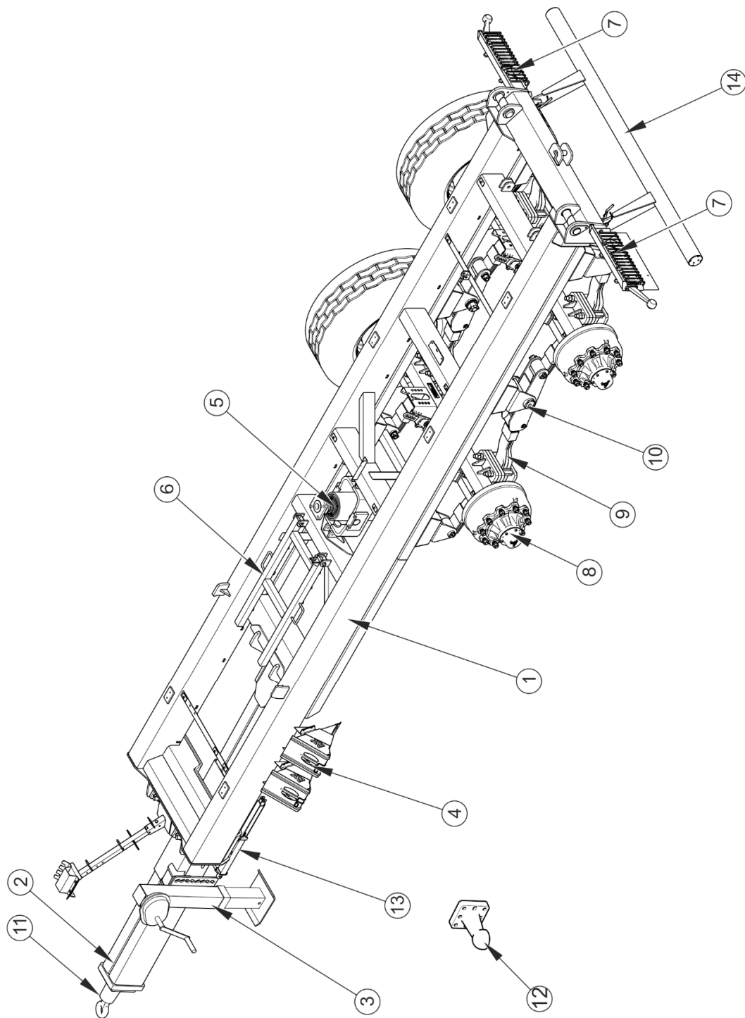
РИСУНОК 3.1 Шасси прицепа
