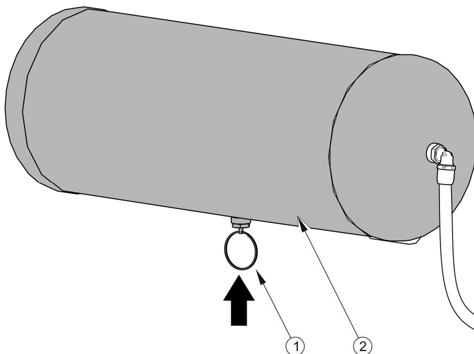
РИСУНОК 5.13 Отвод конденсата из емкости для сжатого воздуха
