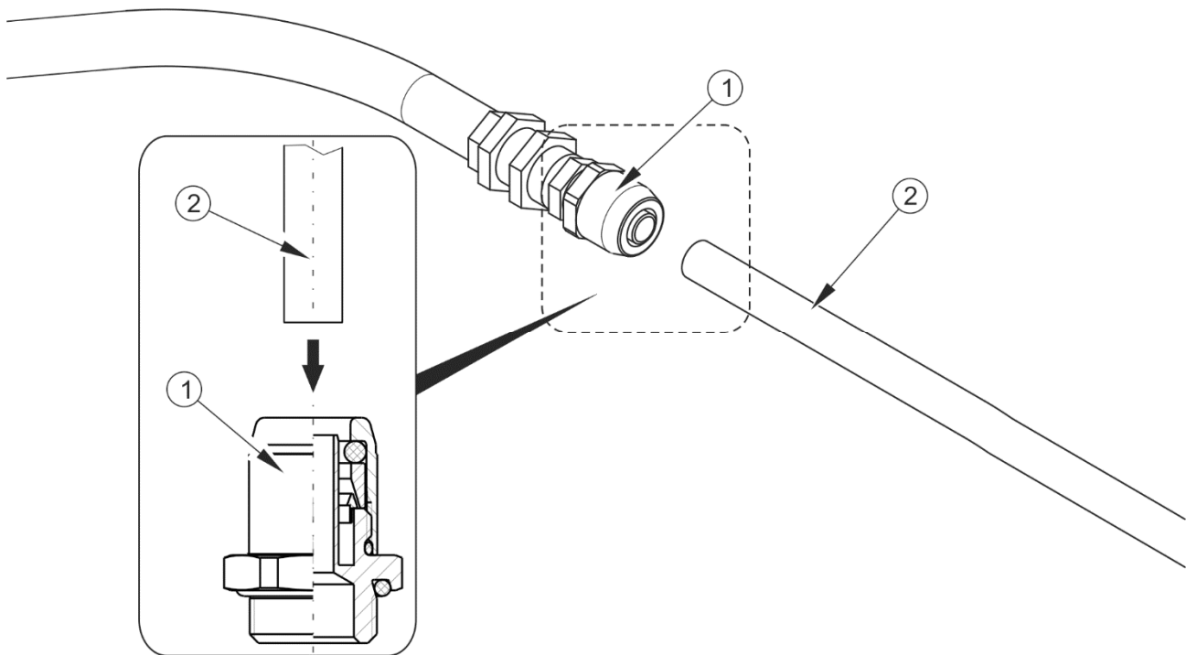
РИСУНОК 5.14 Монтаж пневмопровода
