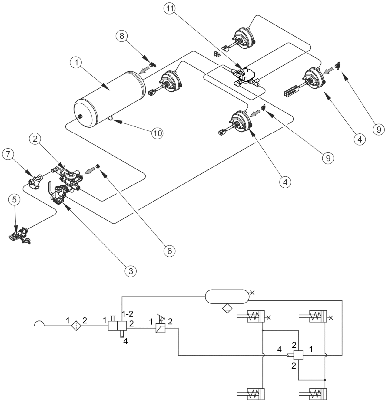
РИСУНОК 3.4 Устройство и схема однопроводной пневматической тормозной системы
