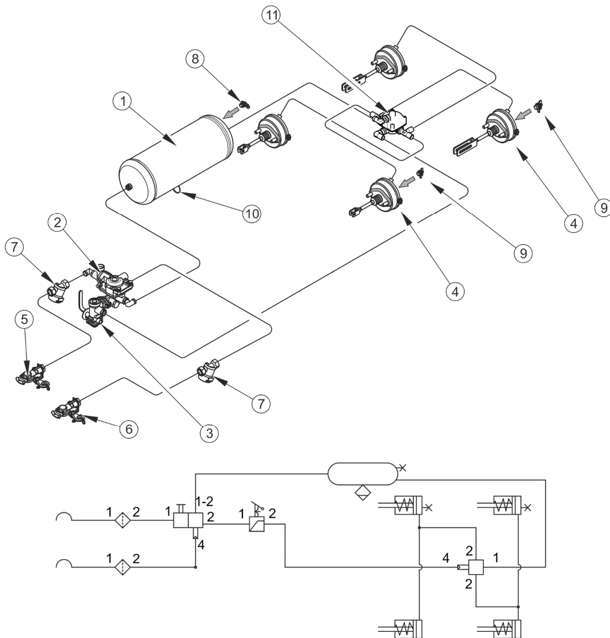
РИСУНОК 3.3 Устройство и схема пневматической двухпроводной тормозной системы
