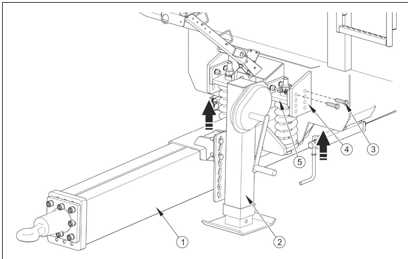
РИСУНОК 5.19 Регулировка высоты дышла
