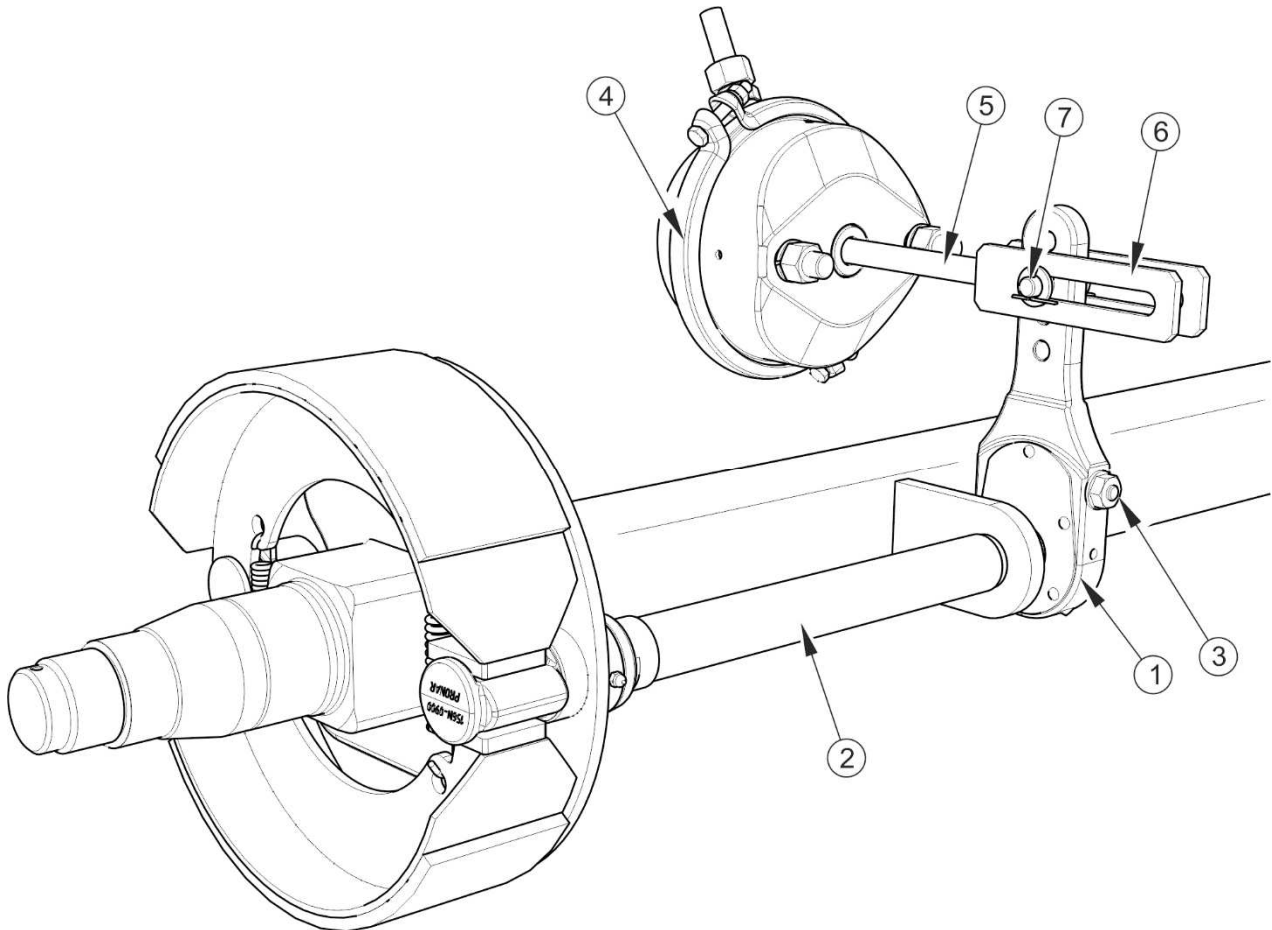
РИСУНОК 5.6 Устройство пневматического тормоза ходовой оси
