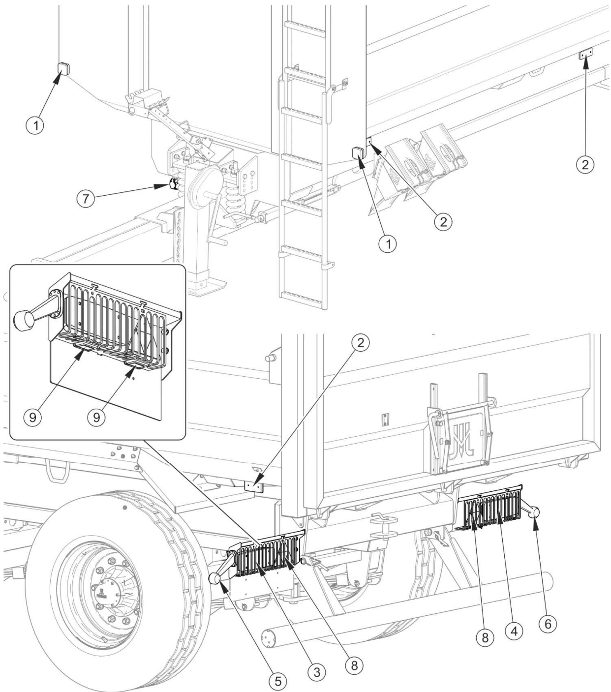
РИСУНОК 3.14 Размещение элементов электрической системы и светоотражающей сигнализации
