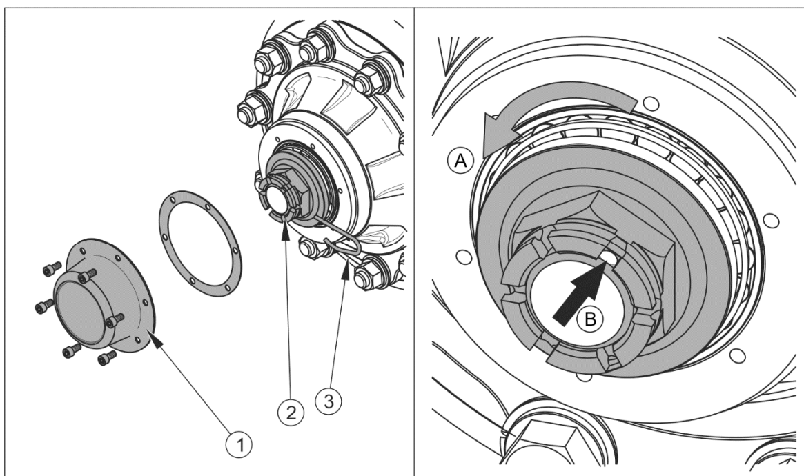
РИСУНОК 5.4 Регулирование зазора в ходовой оси
