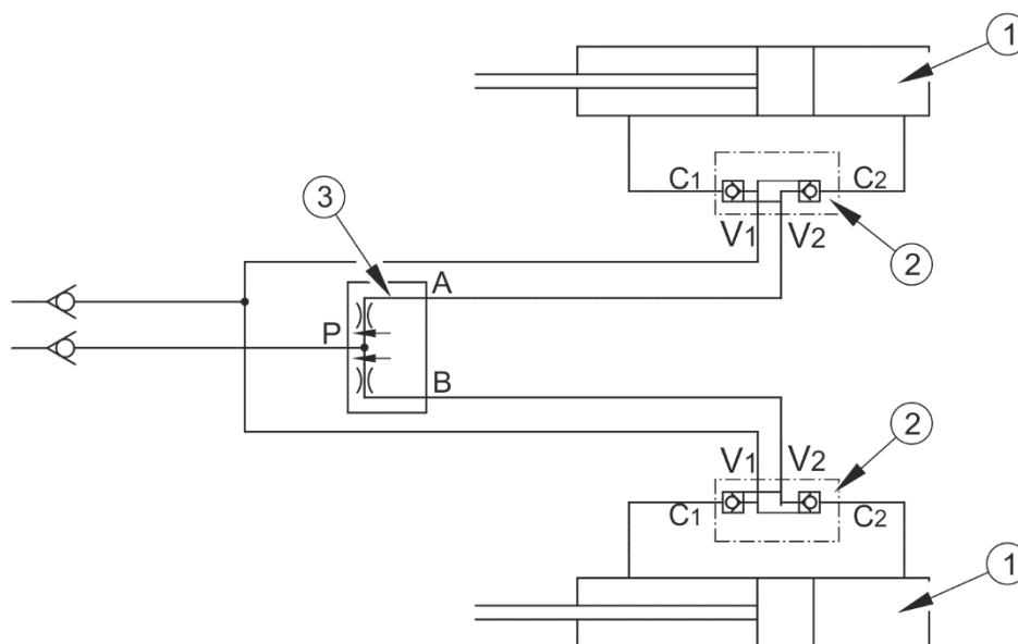
РИСУНОК 3.13 Схема гидравлической системы заднего борта
