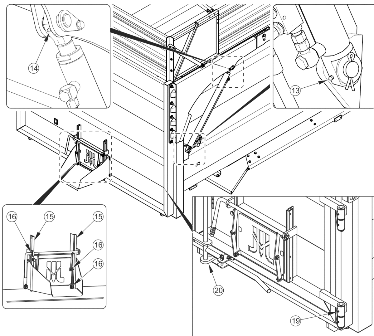
РИСУНОК 5.16 Точки смазки прицепа
