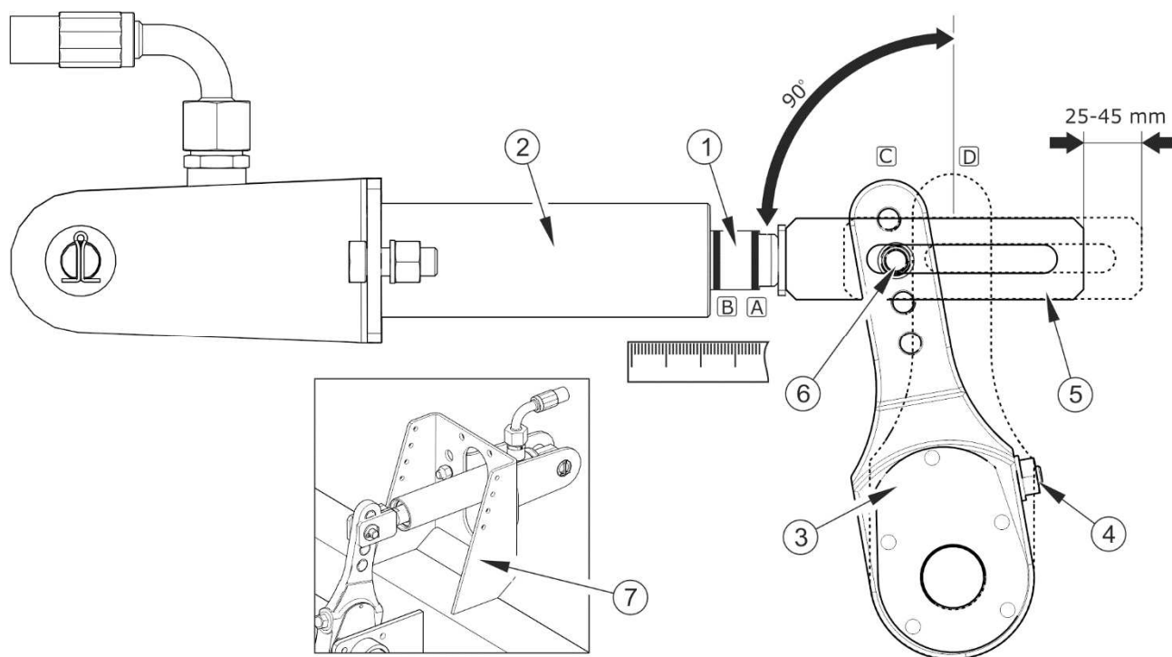
РИСУНОК 5.9 Принцип регулировки гидравлического тормоза
