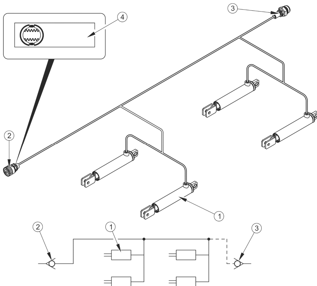
РИСУНОК 3.5 Устройство и схема гидравлической тормозной системы
