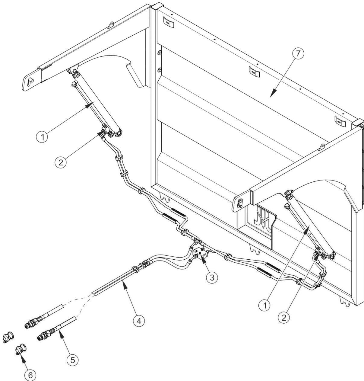
РИСУНОК 3.12 Схема гидравлической системы заднего борта
