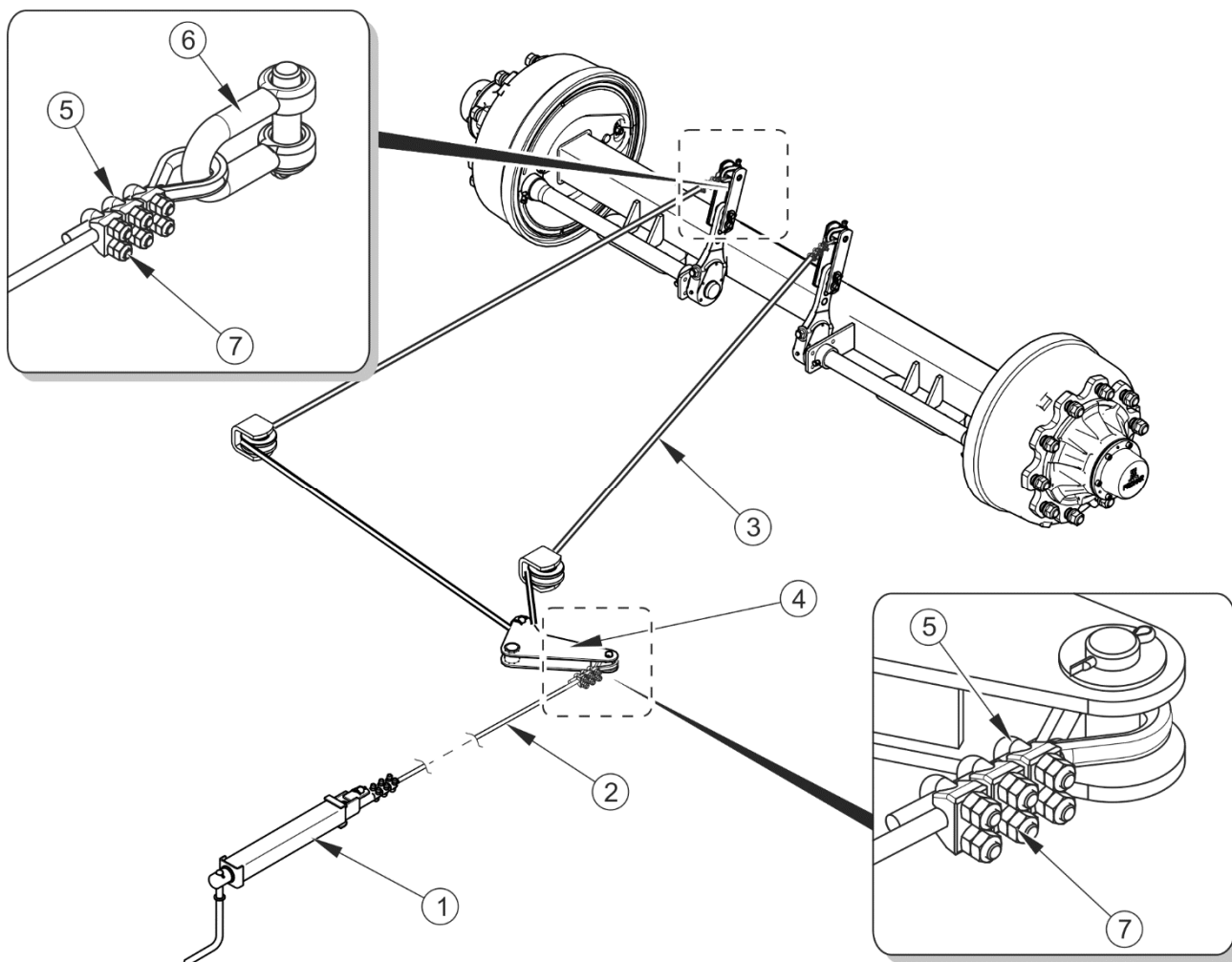
РИСУНОК 5.10 Регулирование натяжения троса стояночного тормоза
