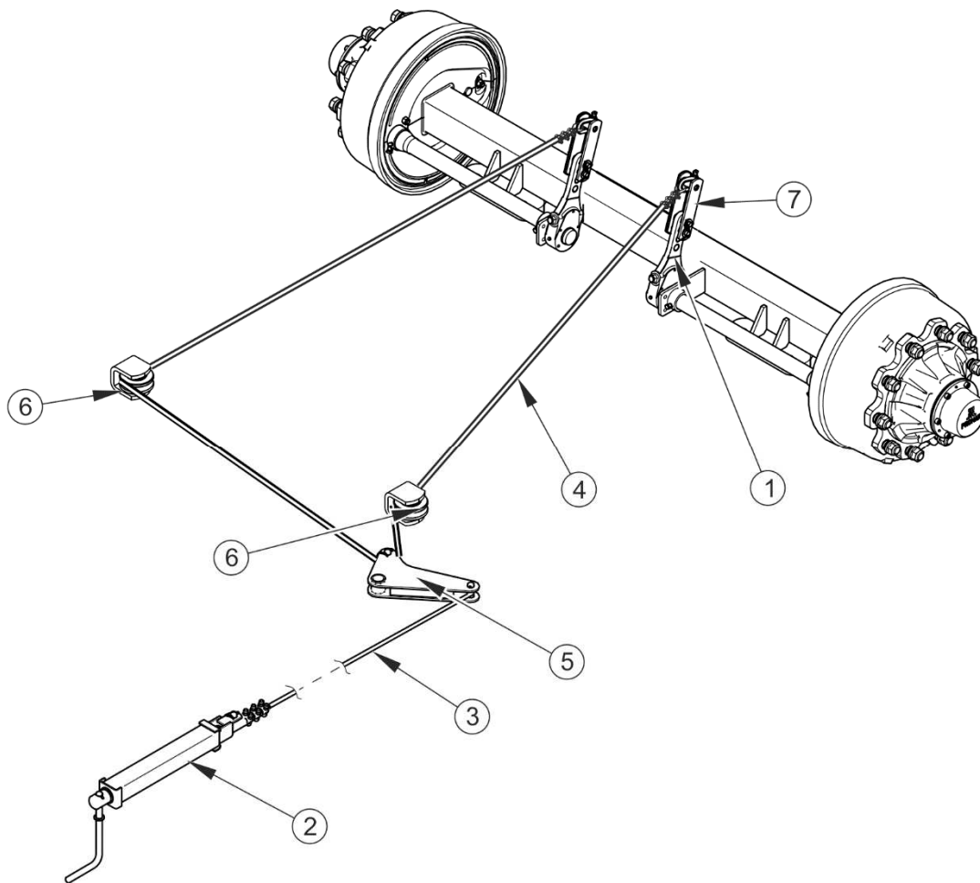
РИСУНОК 3.8 Устройство стояночного тормоза
