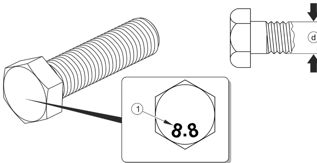
РИСУНОК 5.18 Болт с метрической резьбой
