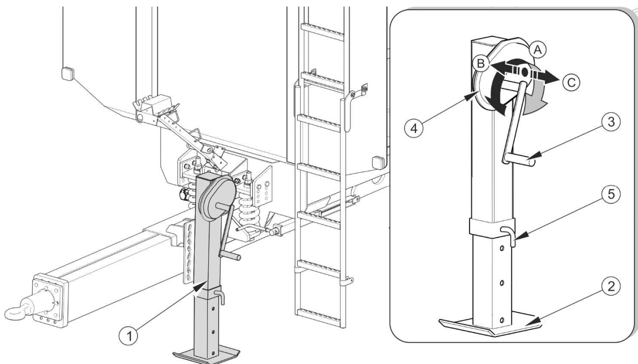
РИСУНОК 4.1 Регулировка высоты дышла
