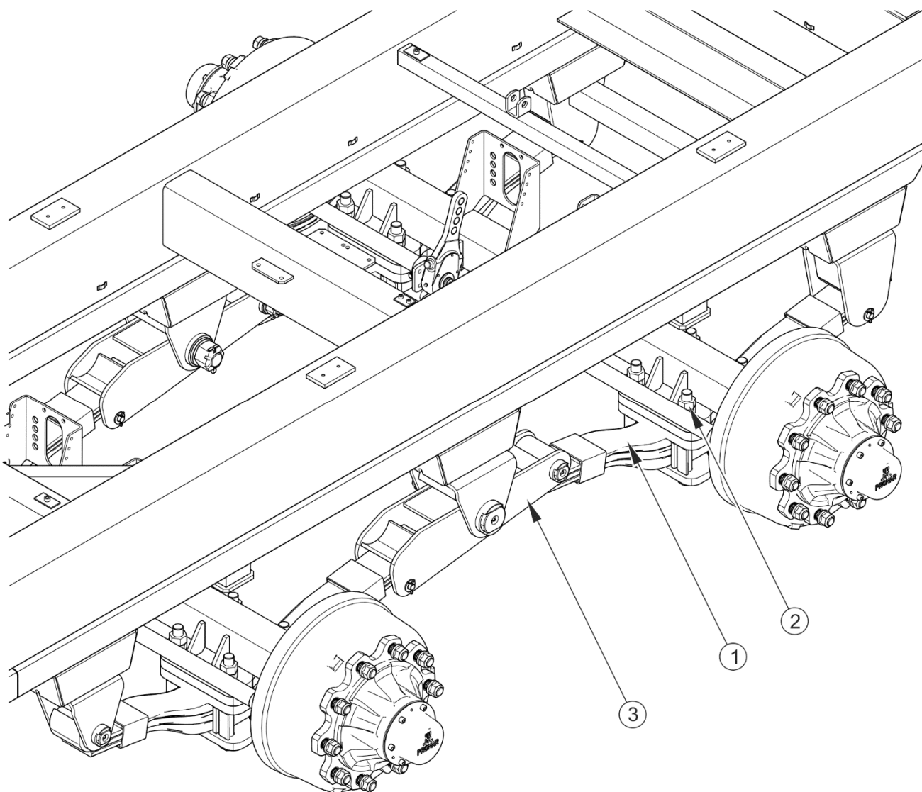
РИСУНОК 5.17 Подвеска тип "тандем"
