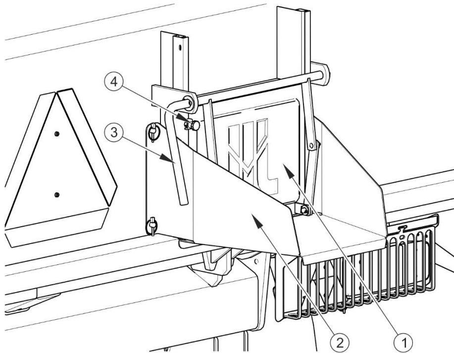
РИСУНОК 4.2 Разгрузочный желоб
