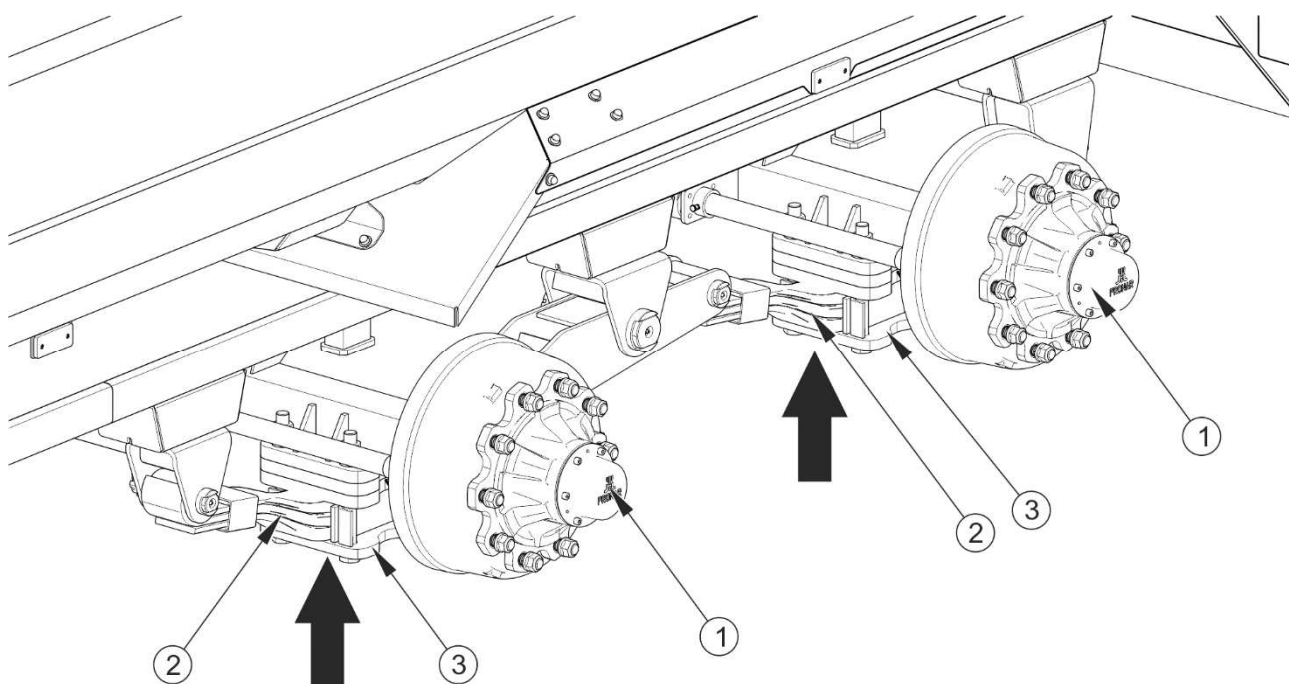
РИСУНОК 5.2 Точка поддомкрачивания
