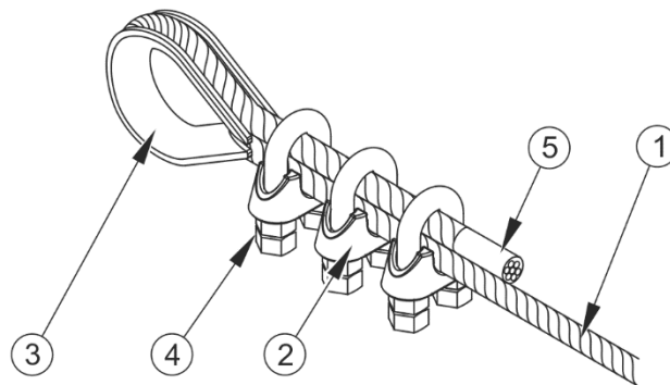
РИСУНОК 5.11 Монтаж тормозного троса
