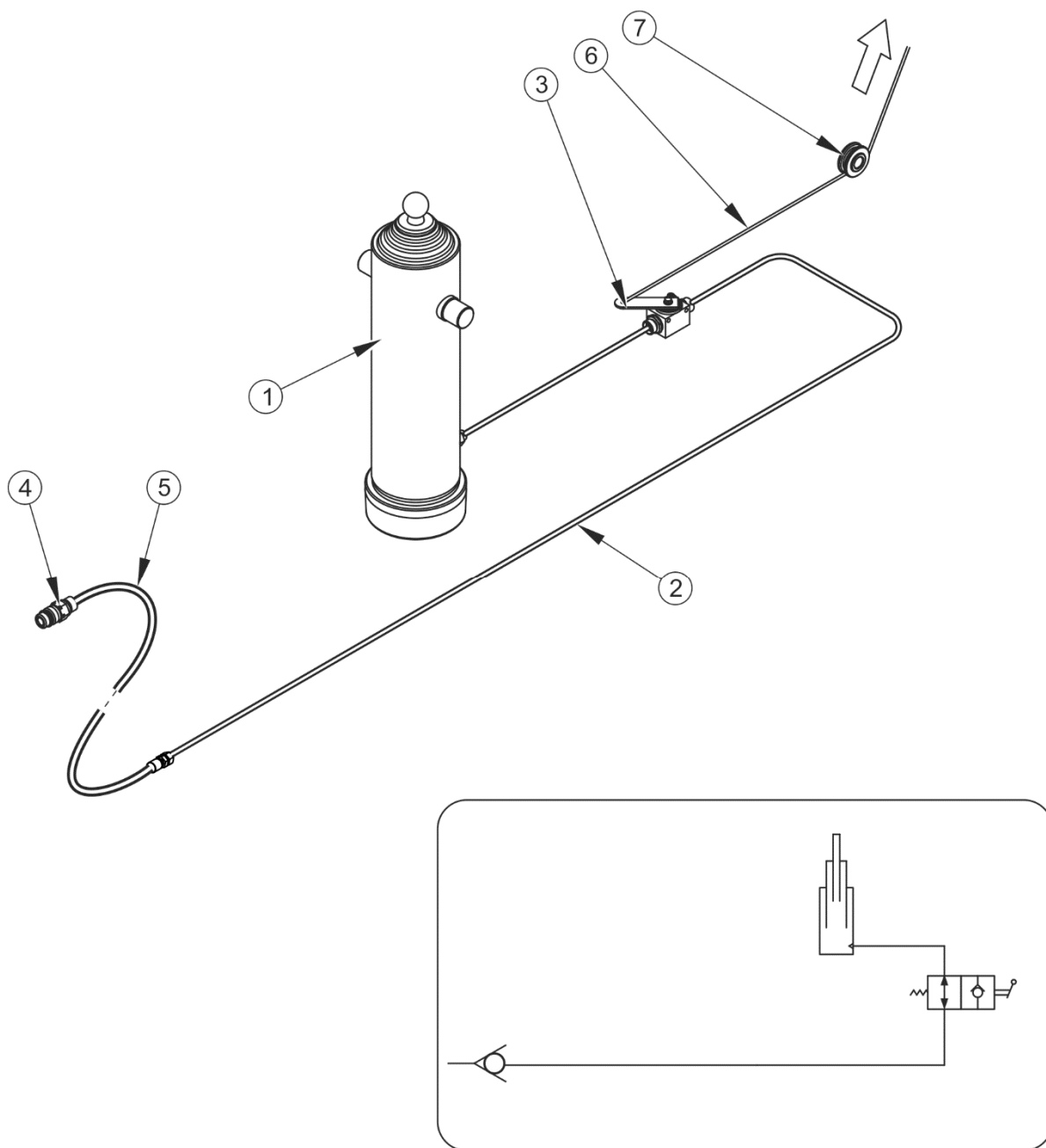
РИСУНОК 3.9 Устройство и схема гидравлической системы опрокидывания "тандем"
