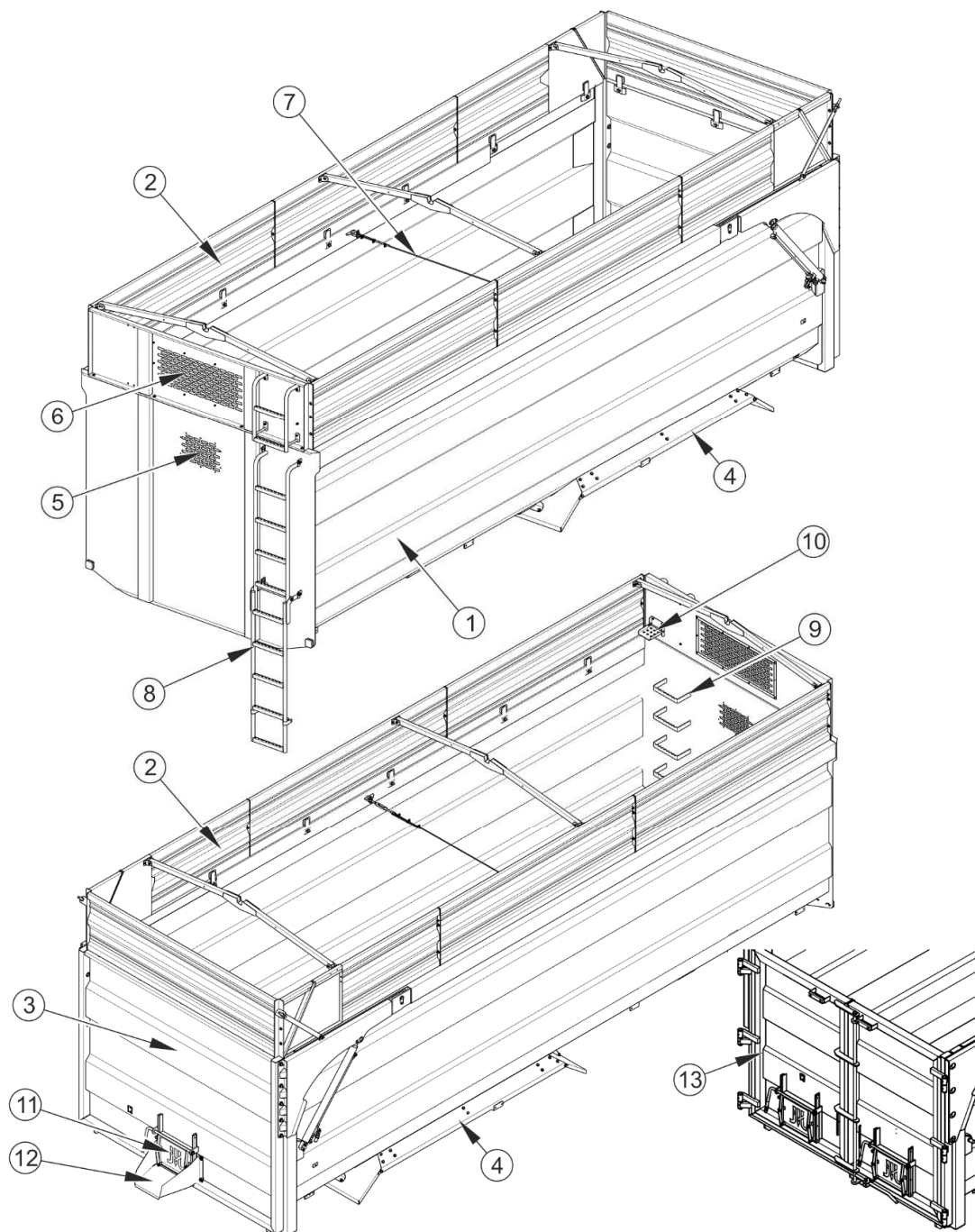
РИСУНОК 3.2 Грузовая платформа
