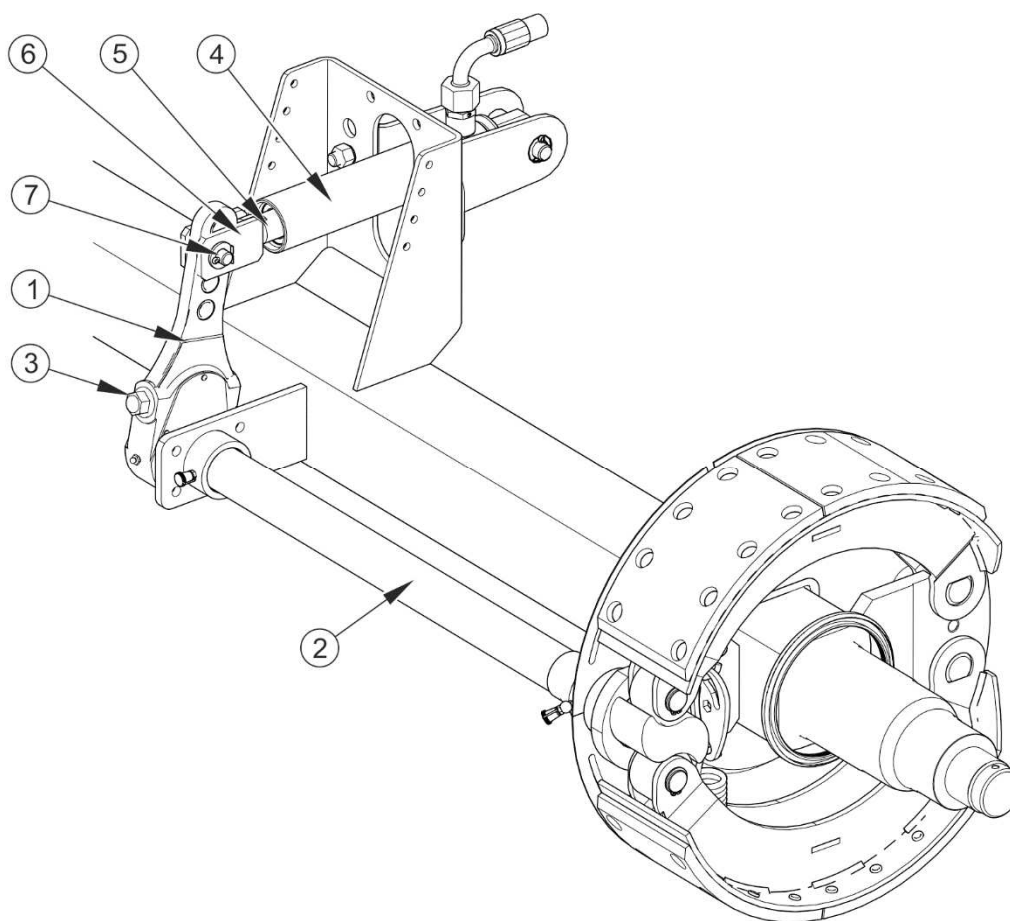
РИСУНОК 5.7 Устройство гидравлического тормоза ходовой оси
