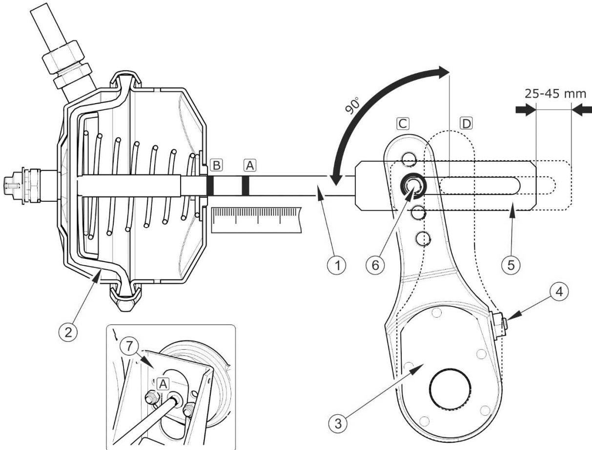
РИСУНОК 5.8 Принцип регулировки пневматического тормоза
