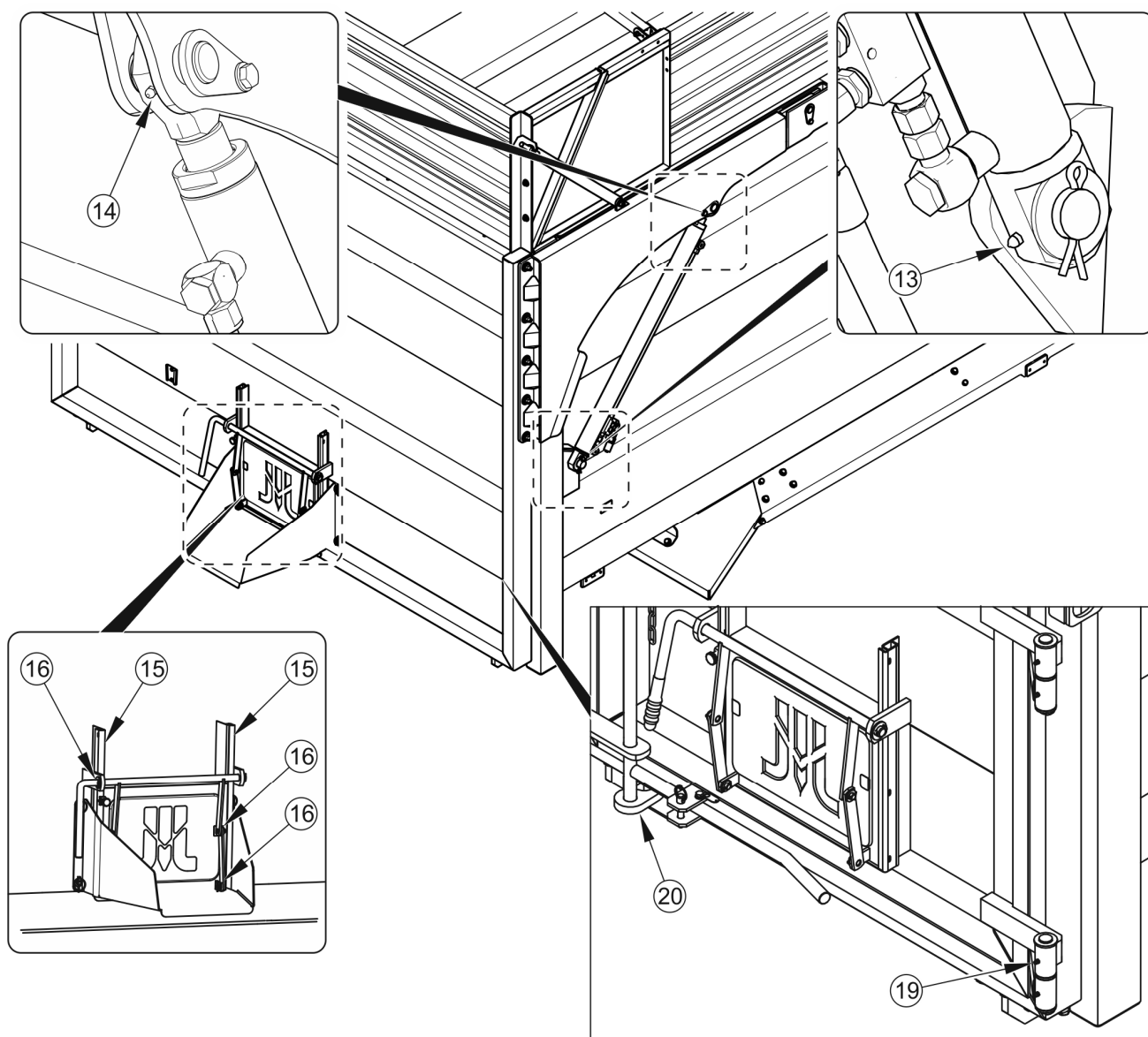
Obrázek 5.16 Mazací místa přívěsu
