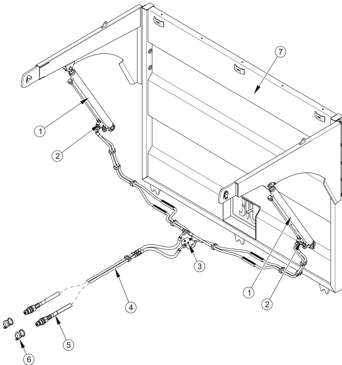
Obrázek 3.12 Konstrukce a schéma hydraulické instalace zadního poklopu
