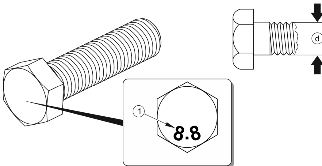
Obrázek 5.18 Šroub s metrickým závitem
