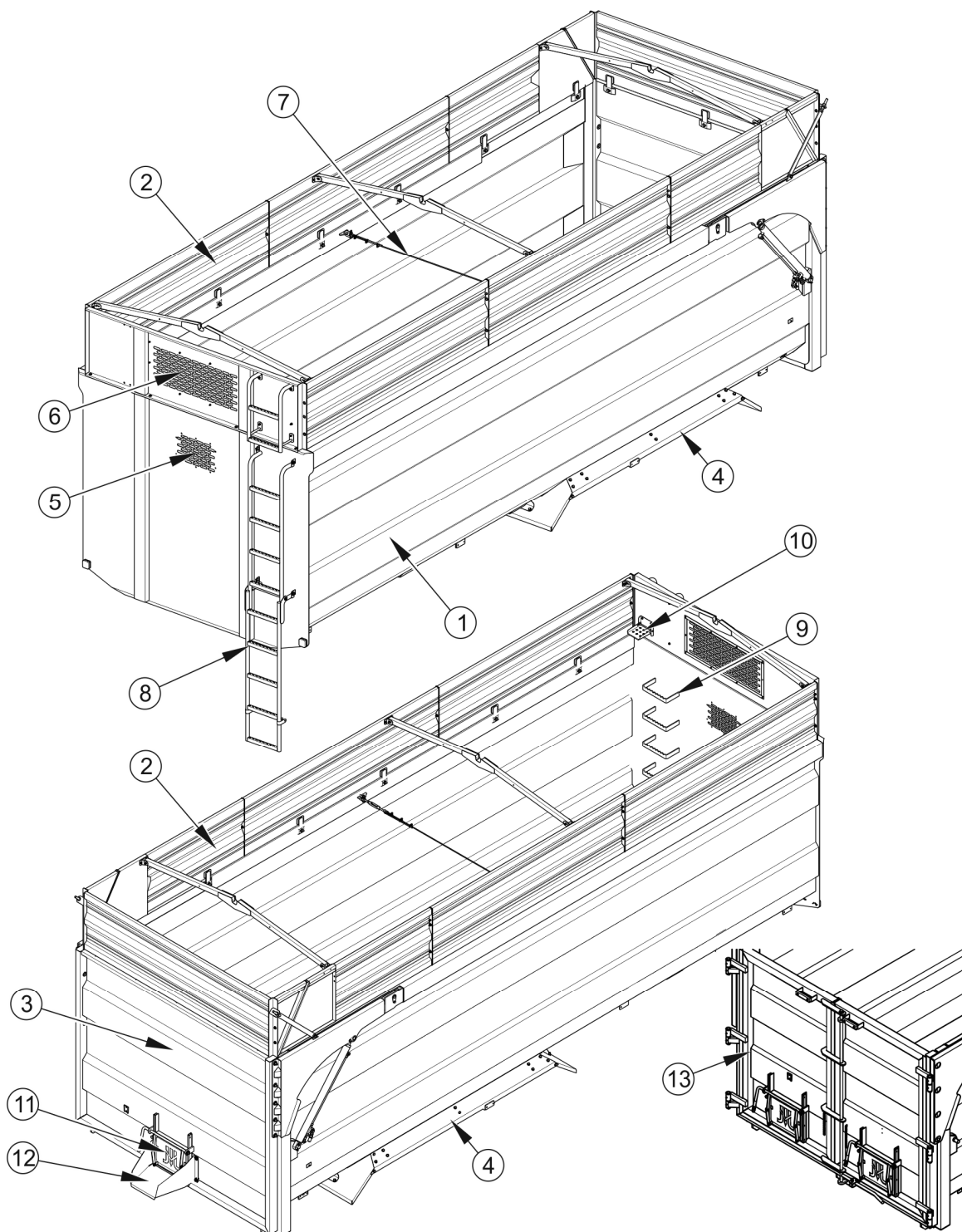
Obrázek 3.2 Korba
