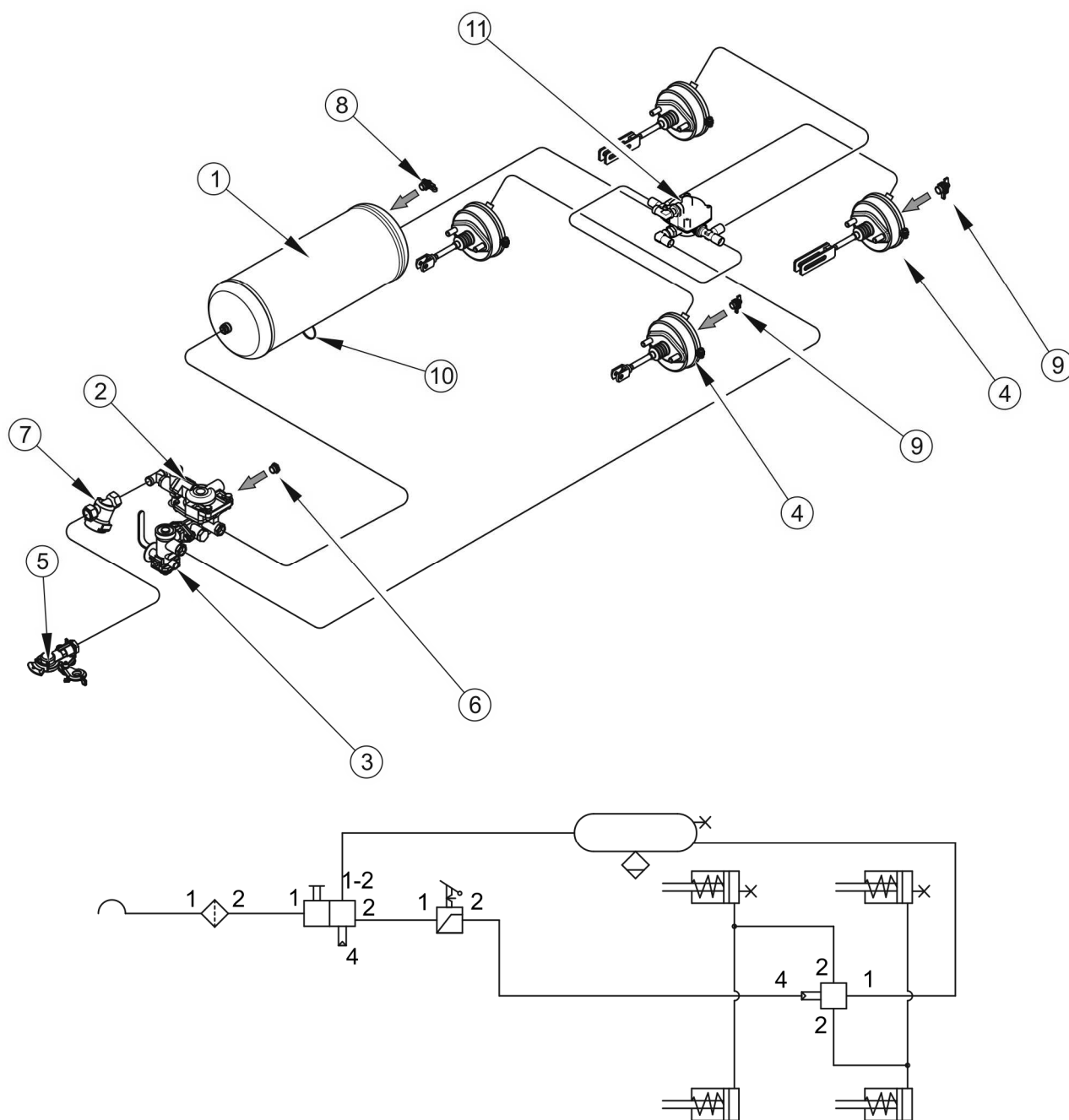
Obrázek 3.4 Konstrukce a schéma vzduchové jednoduché brzdové instalace
