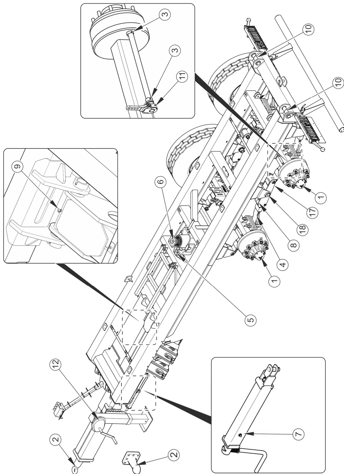
Obrázek 5.15 Mazací místa přivěsu
