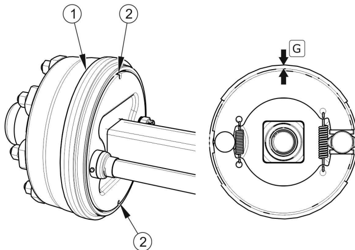
Obrázek 5.1 Kontrola brzdového obložení
