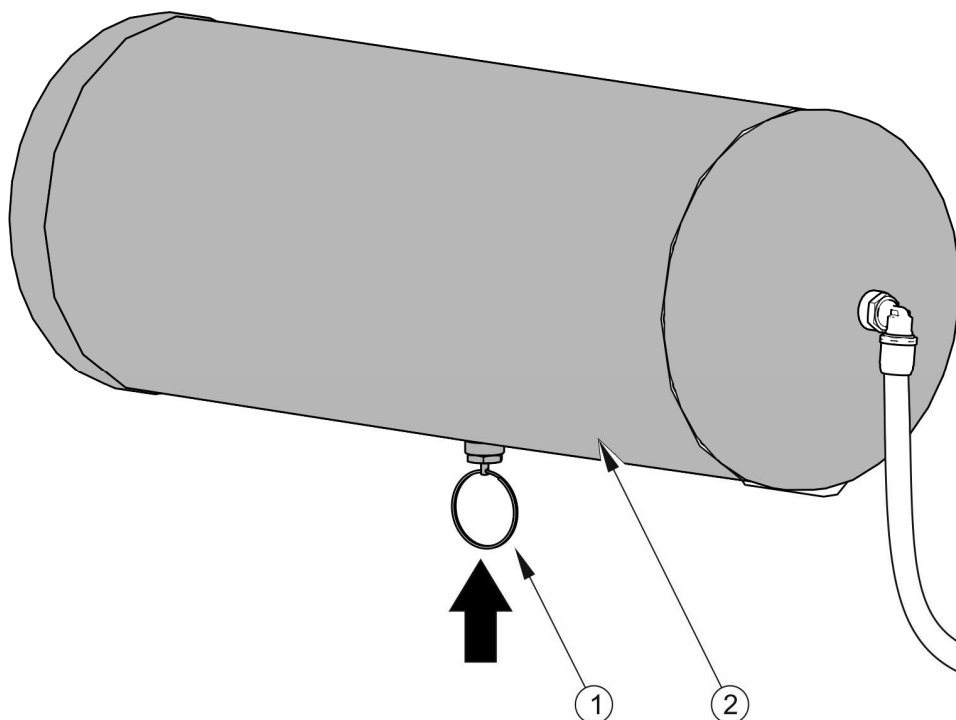
Obrázek 5.13 Odvodňování vzdušníku
