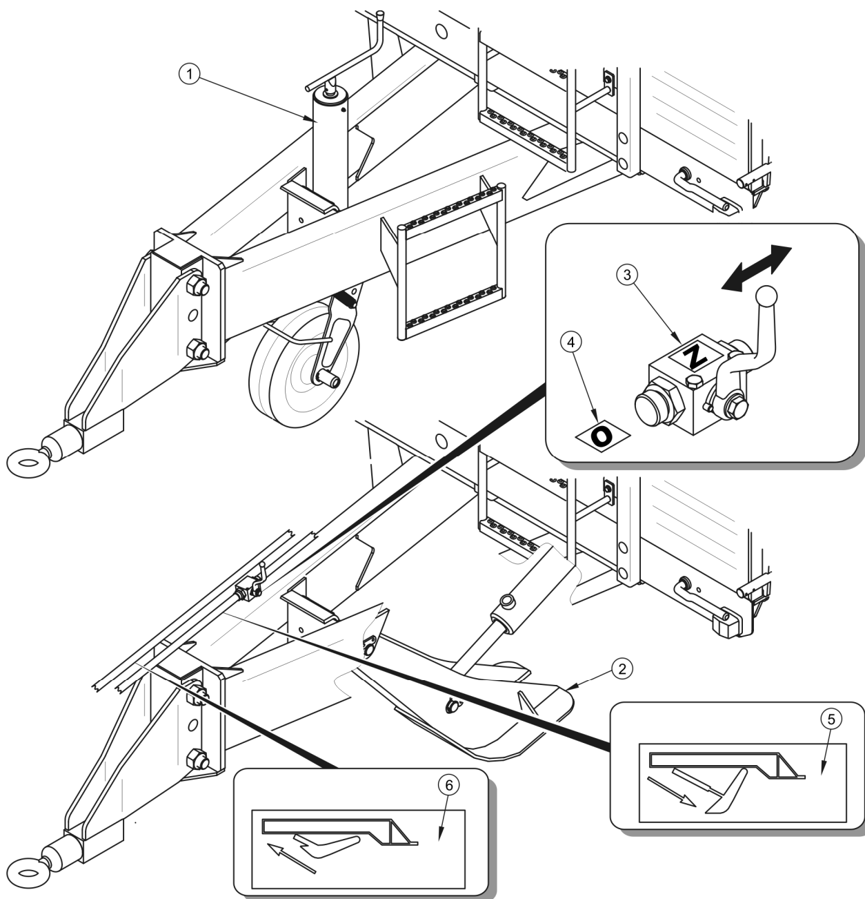
РИСУНОК 4.1 Опора прицепа
