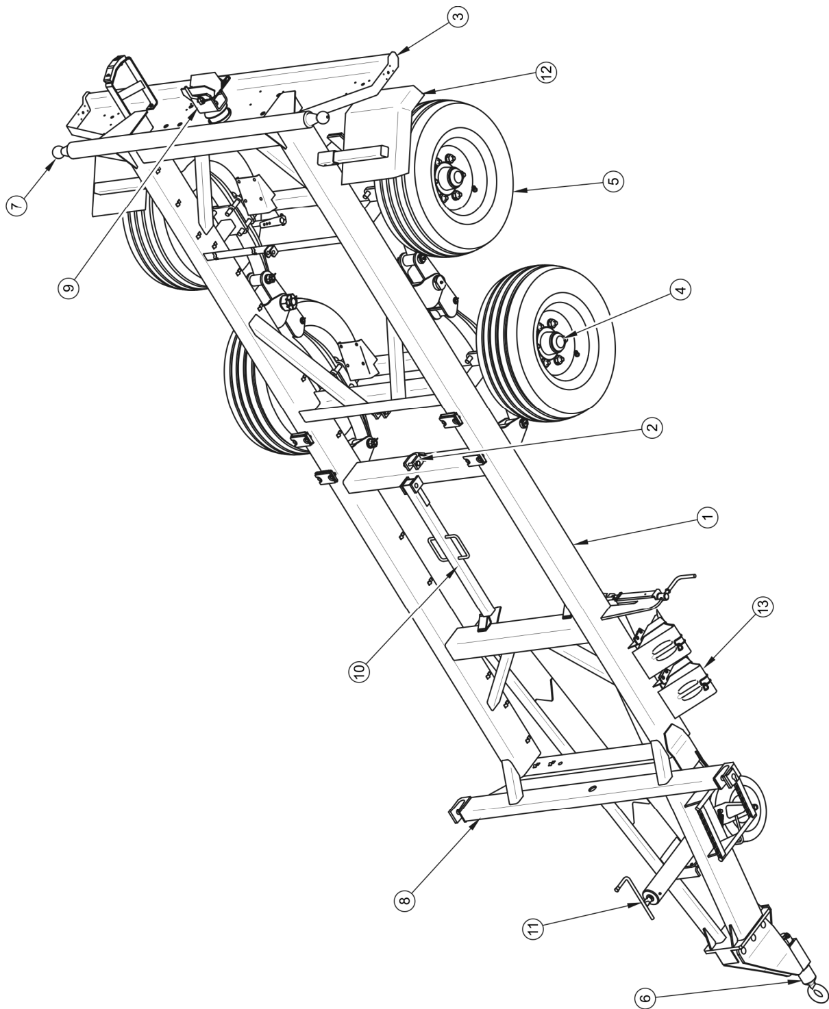
РИСУНОК 3.1 Шасси прицепа
