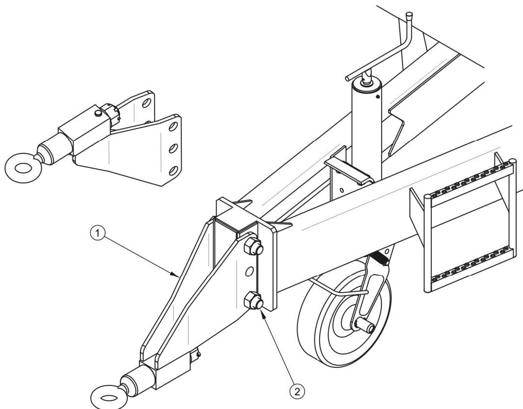
РИСУНОК 5.12 Регулирование положения дышла
