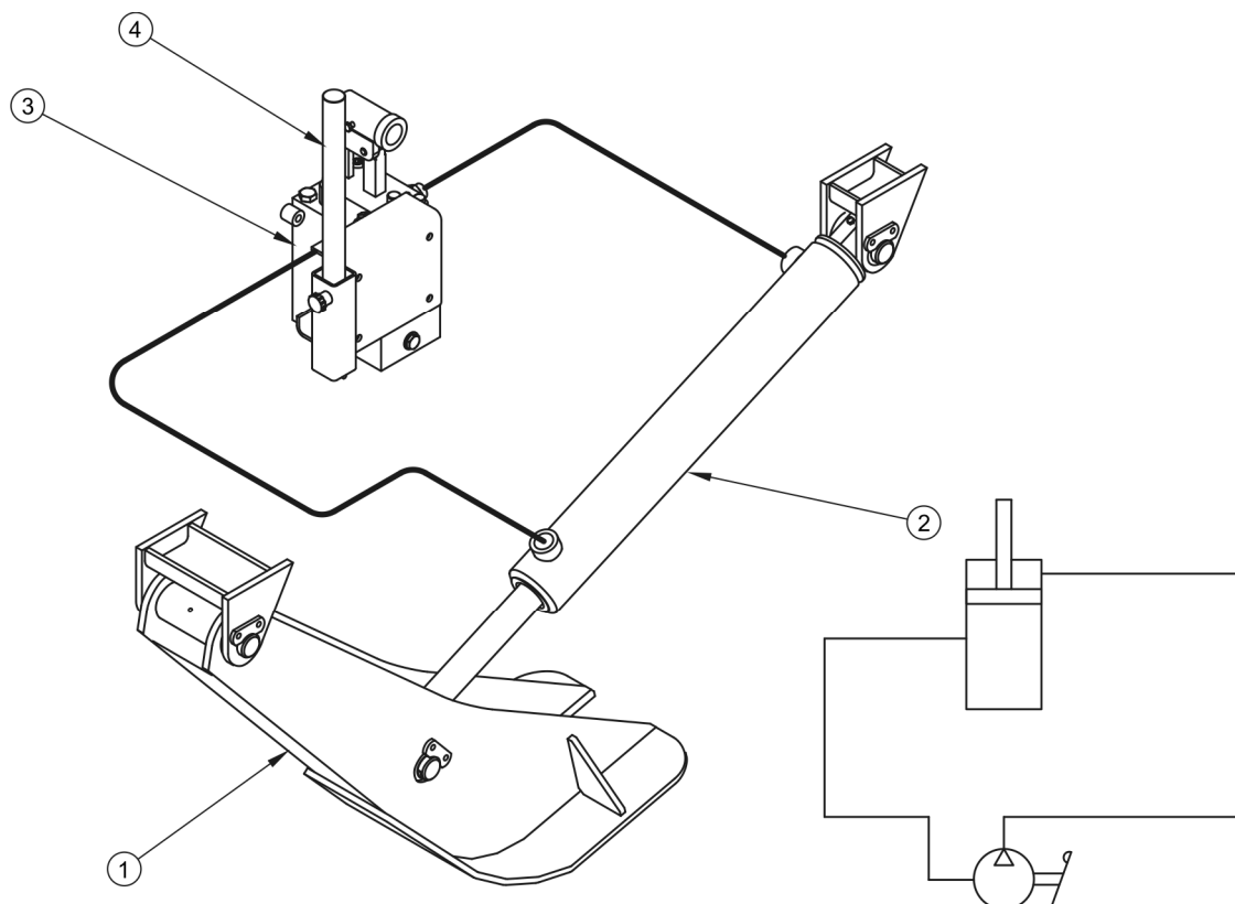
РИСУНОК 3.14 Устройство и схема гидравлической системы ножевой опоры с насосом (1) ножевая опора, (2) гидроцилиндр опоры, (3) ручной насос, (4) рычаг насоса
