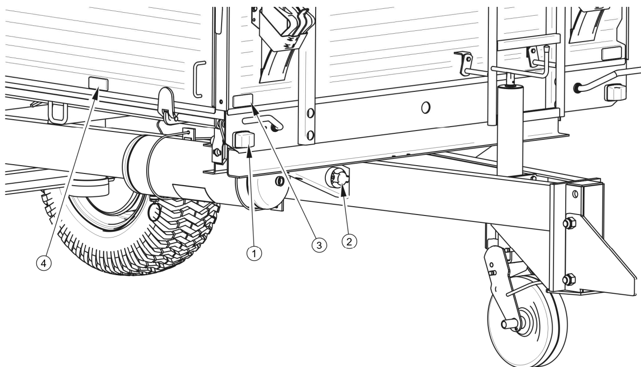
РИСУНОК 3.18 Размещение элементов системы световой сигнализации и катафотов прицепа – вид спереди
