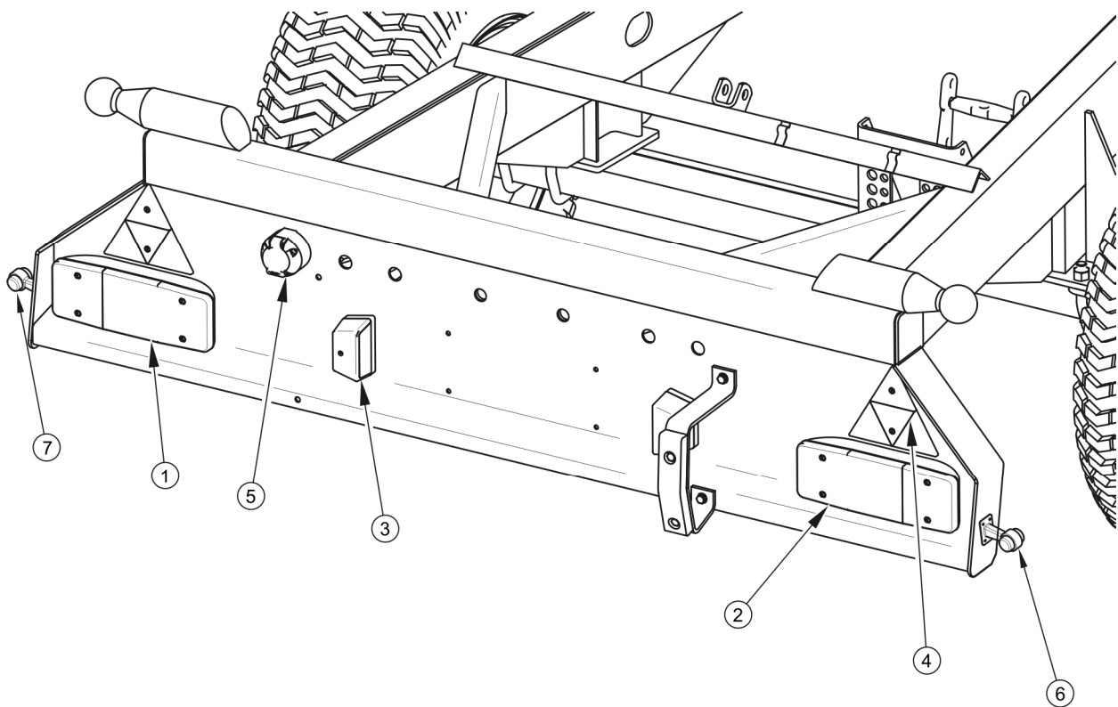
РИСУНОК 3.17 Размещение элементов системы световой сигнализации и катафотов прицепа – вид сзади
