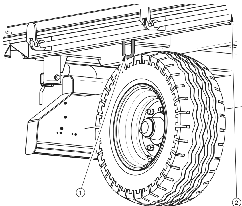
РИСУНОК 1.3 Расположение транспортных захватов
