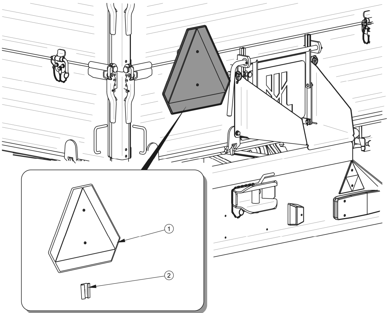
РИСУНОК 2.2 Размещение трехугольного знака медленно движущегося транспортного средства.
