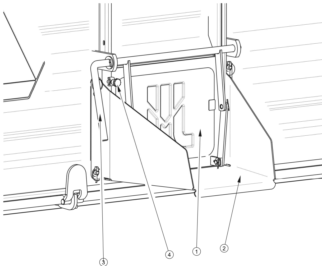
РИСУНОК 4.6 Разгрузочный люк
