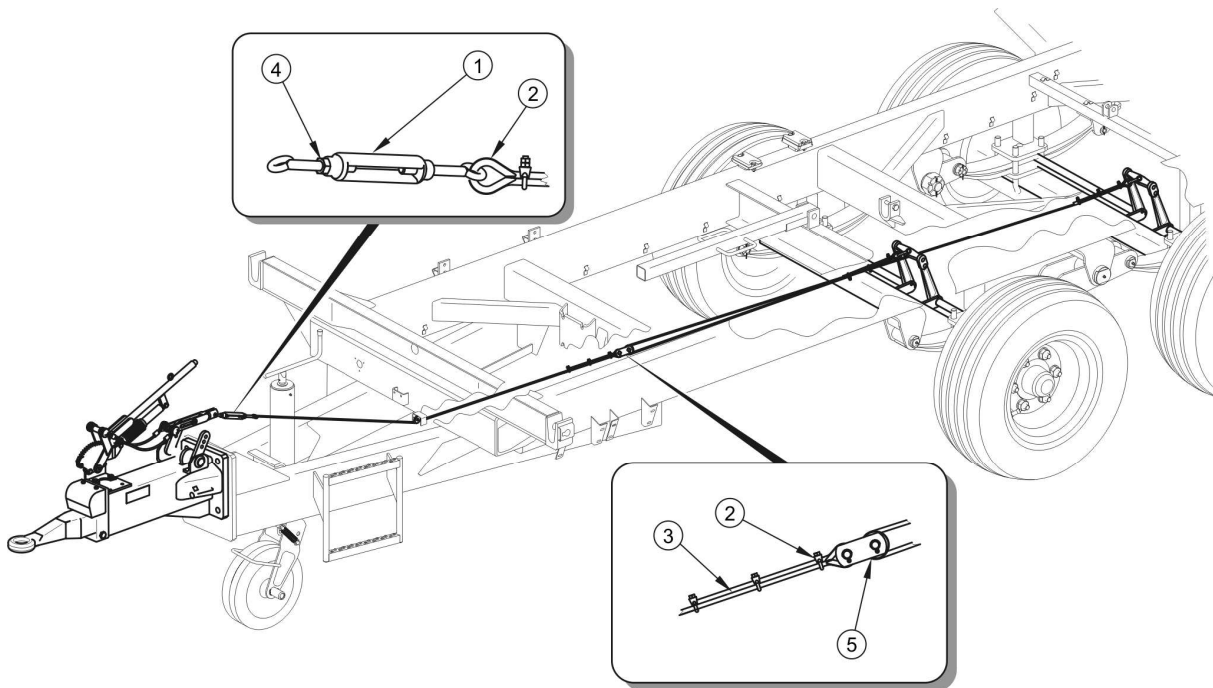
РИСУНОК 5.5 Регулирование натяжения троса тормоза инерционного типа
