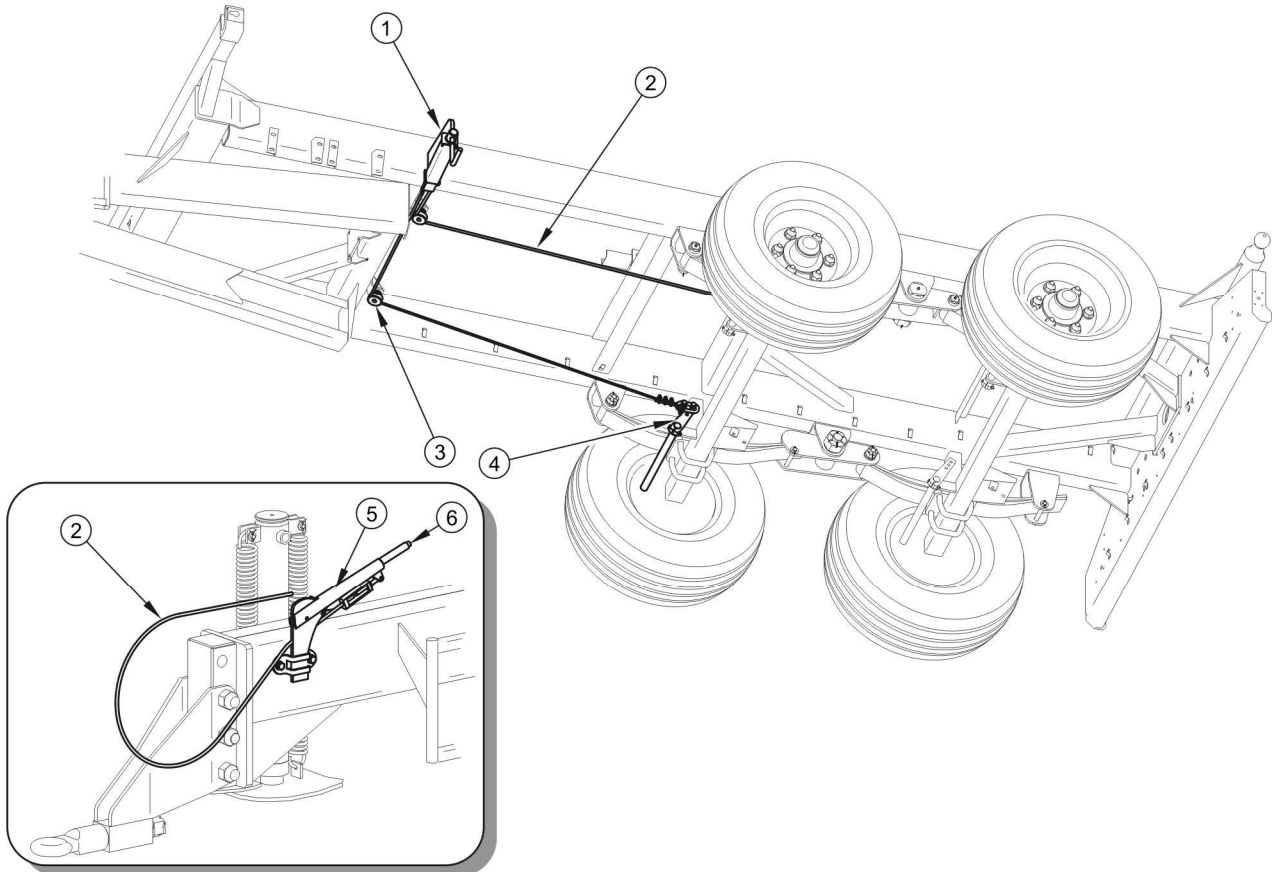
РИСУНОК 3.15 Устройство стояночного тормоза с кривошипным механизмом
