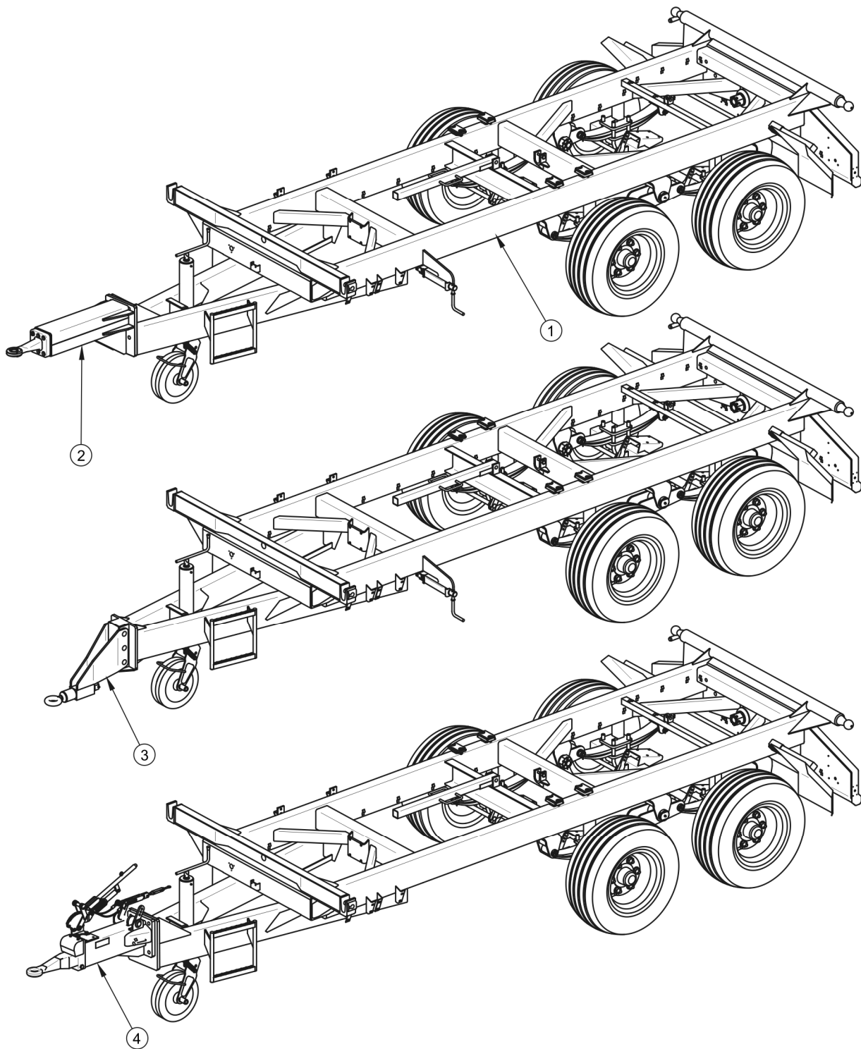
РИСУНОК 3.2 Версии нижней рамы
