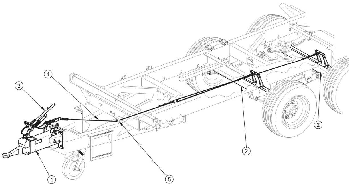
РИСУНОК 3.10 Тормоз инерционного типа
