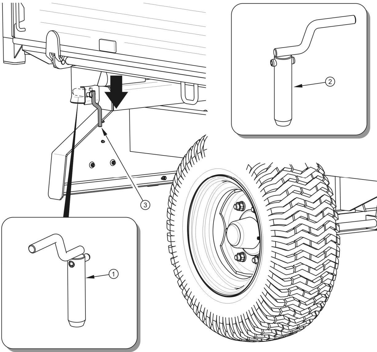
РИСУНОК 4.4 Блокировка болтов опрокидывающего механизма
