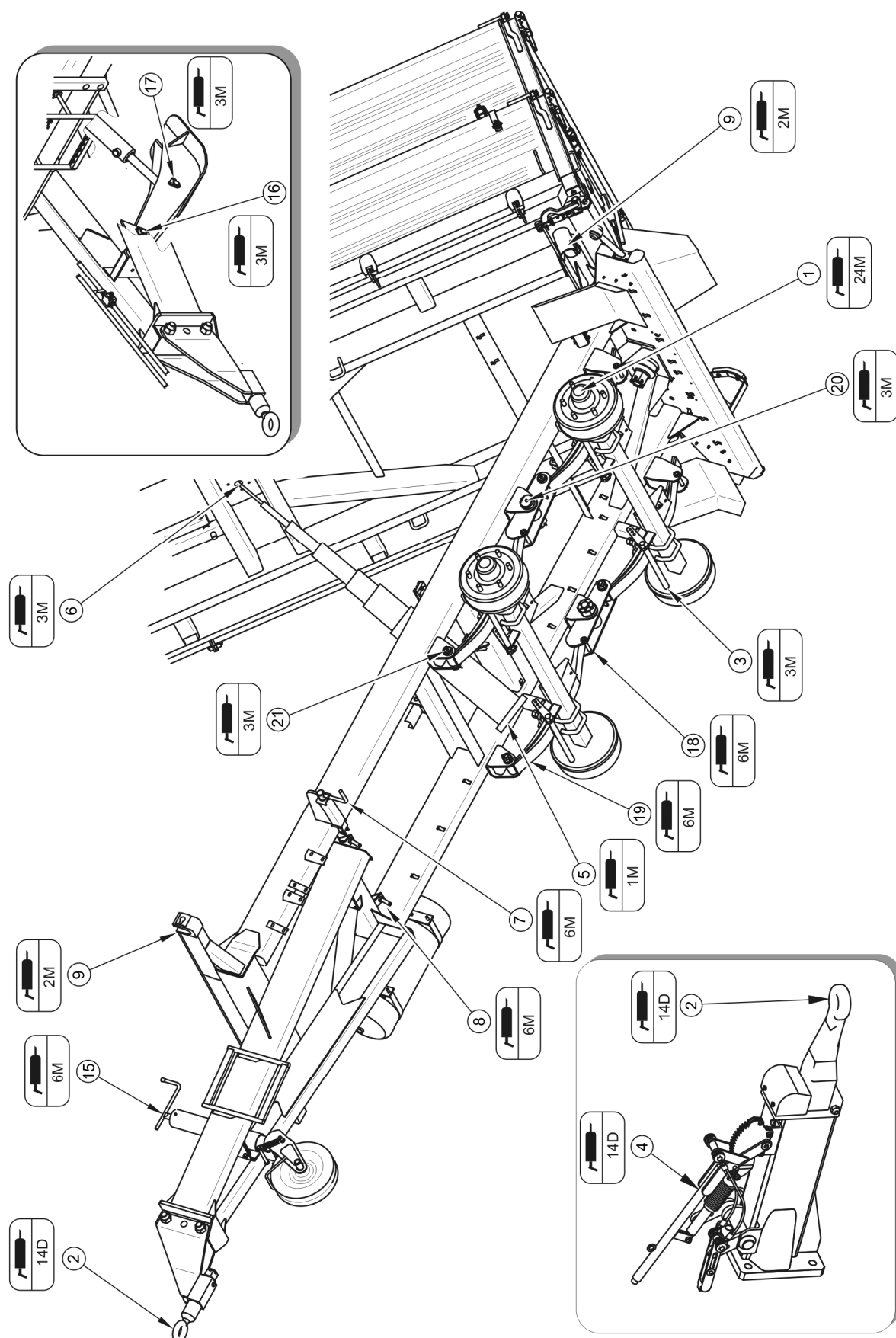
РИСУНОК 5.9 Точки смазки прицепа, часть 1
