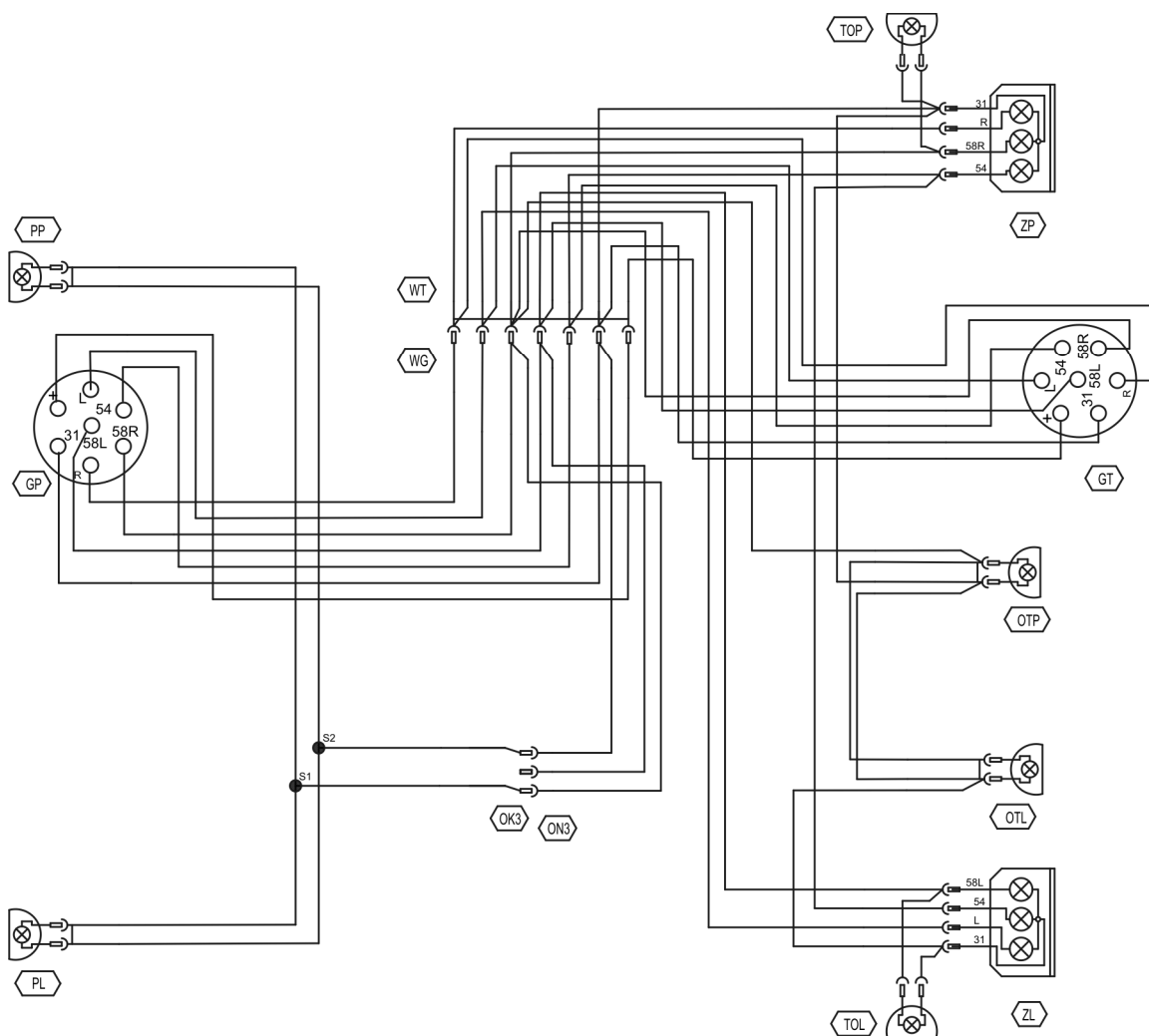
РИСУНОК 3.16 Принципиальная схема электрической системы
