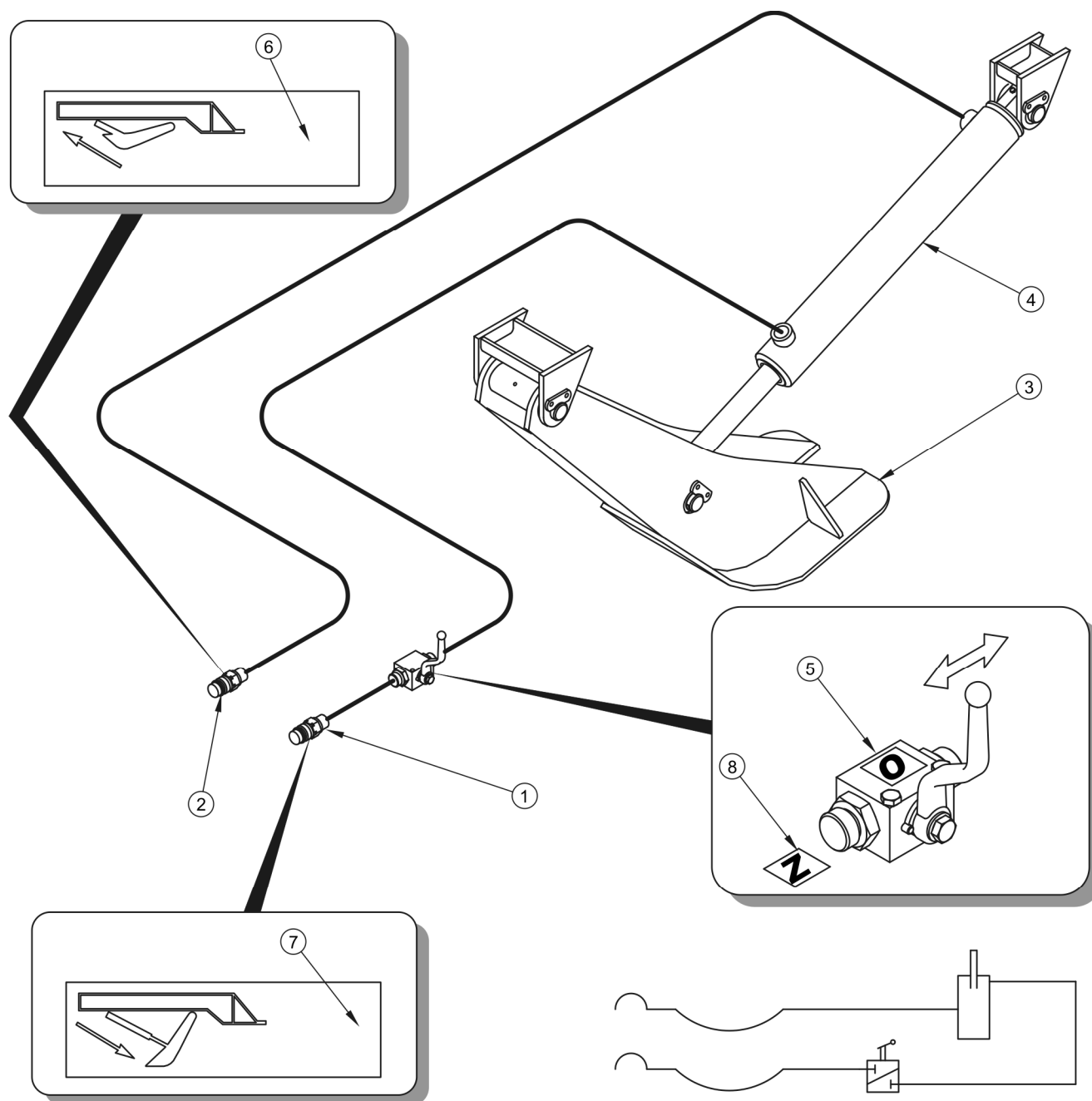
РИСУНОК 3.13 Устройство и схема гидравлической системы ножевой опоры
