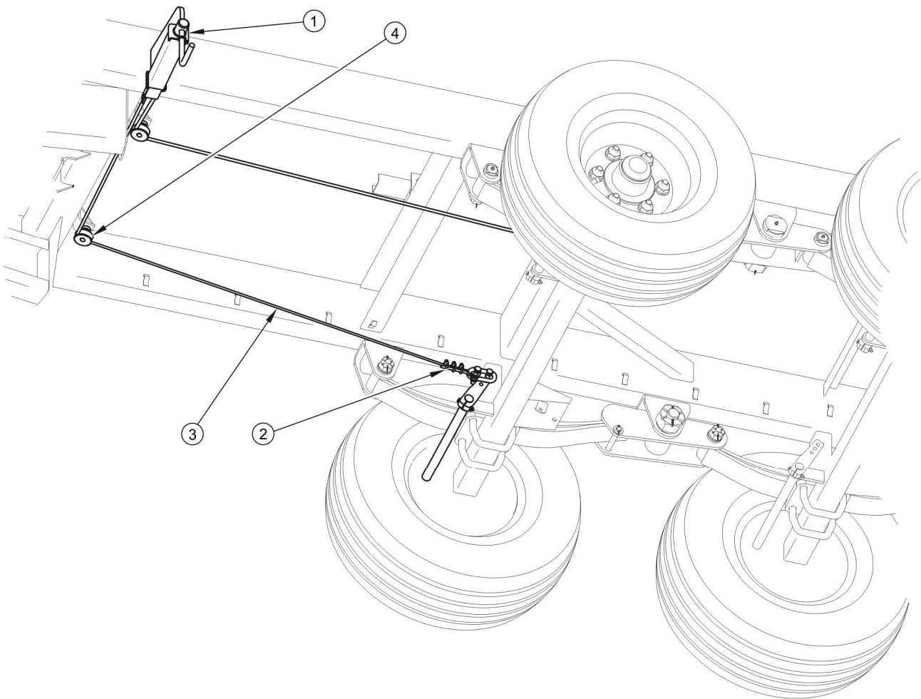
РИСУНОК 5.6 Регулирование натяжения тросов стояночного тормоза
