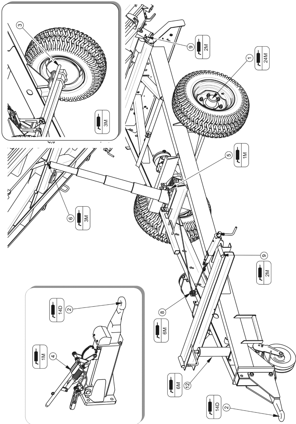
ABBILDUNG 5.9 Schmierpunkte des Anhängers, Teil 1
