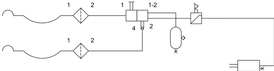
ABBILDUNG 3.5 Aufbau und Schema der Zweikreis-Druckluftbremse
