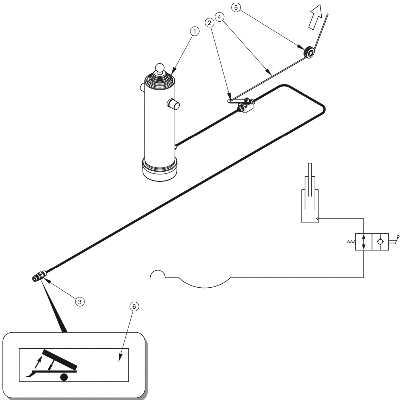
ABBILDUNG 3.10 Aufbau und Schema der Hydraulikanlage der Kippvorrichtung
