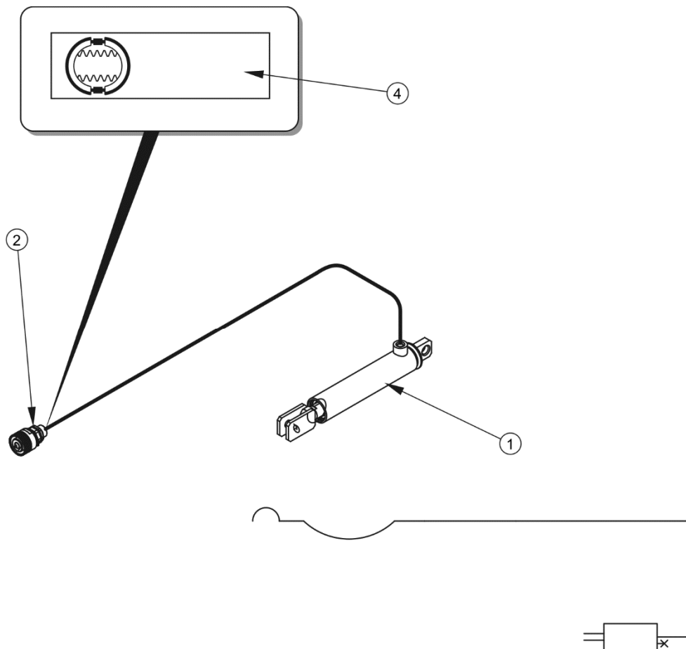
ABBILDUNG 3.7 Aufbau und Schema der Hydraulikbremse
