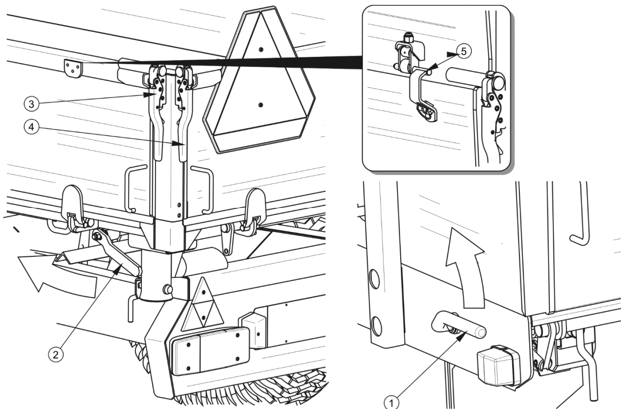
ABBILDUNG 4.4 Wandverschluss
