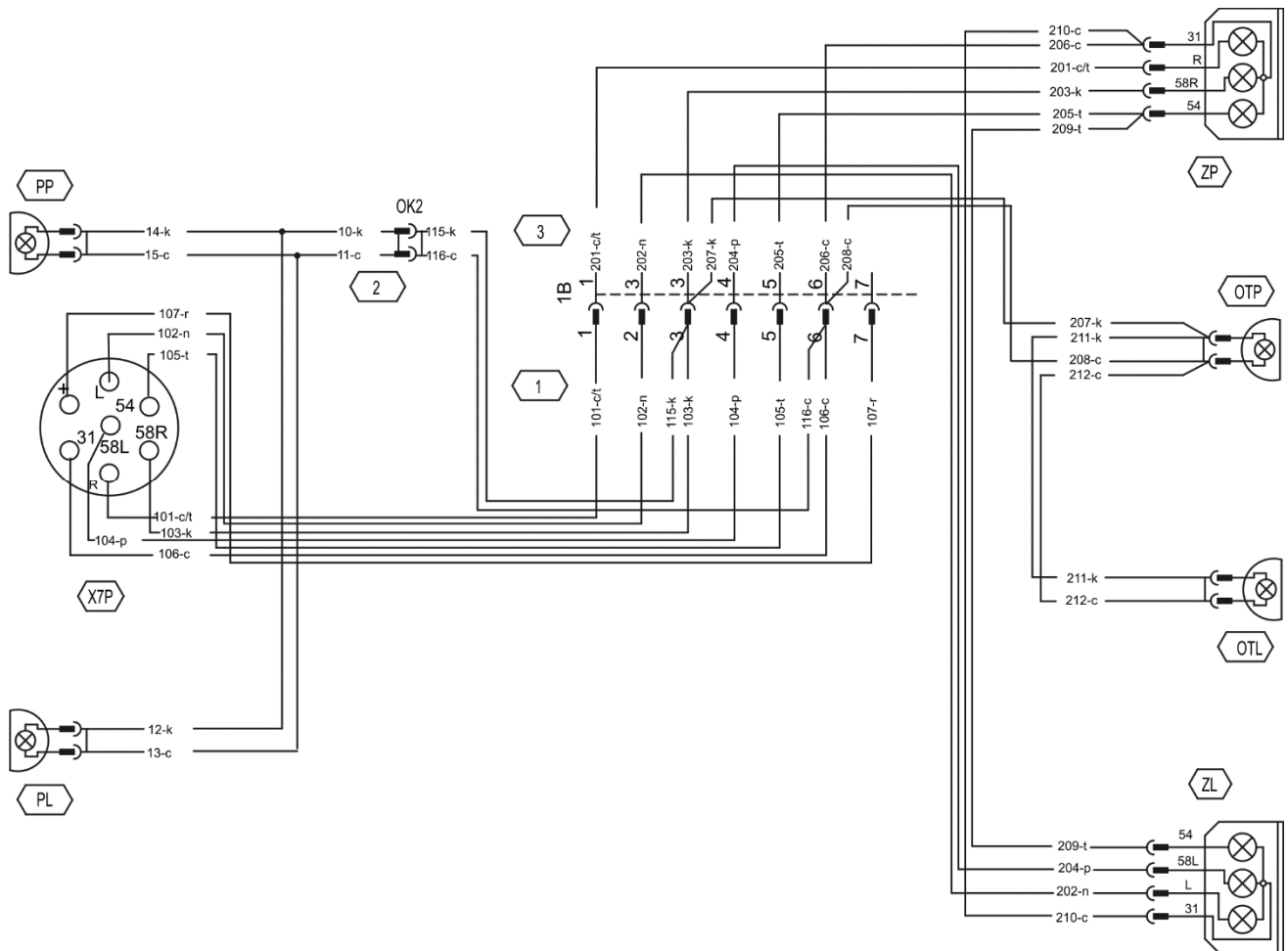
ABBILDUNG 3.12 Schaltplan der Elektroinstallation
