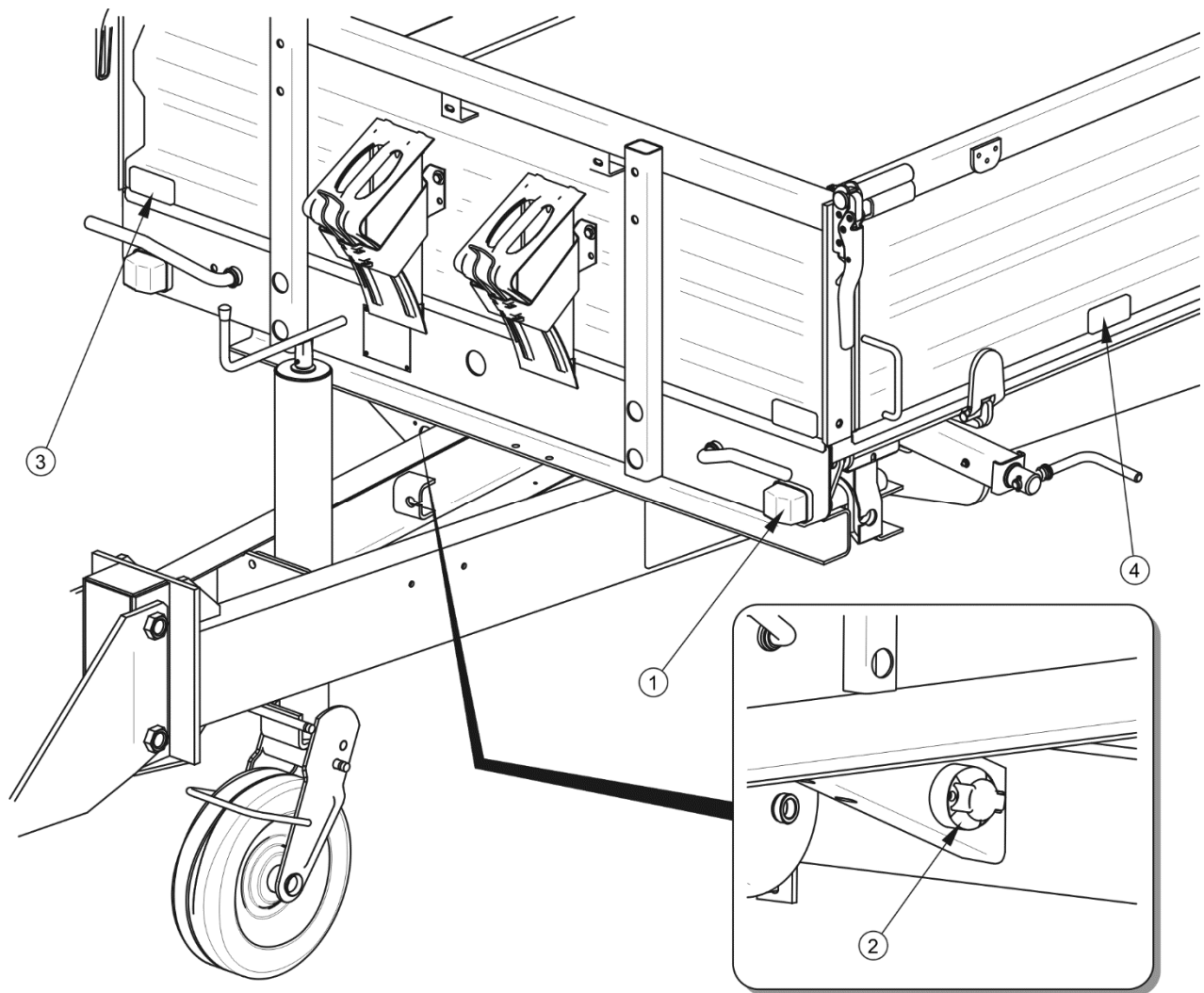
ABBILDUNG 3.14 Anordnung der Elemente der Elektroinstallation und der Rückstrahler – Vorderansicht
