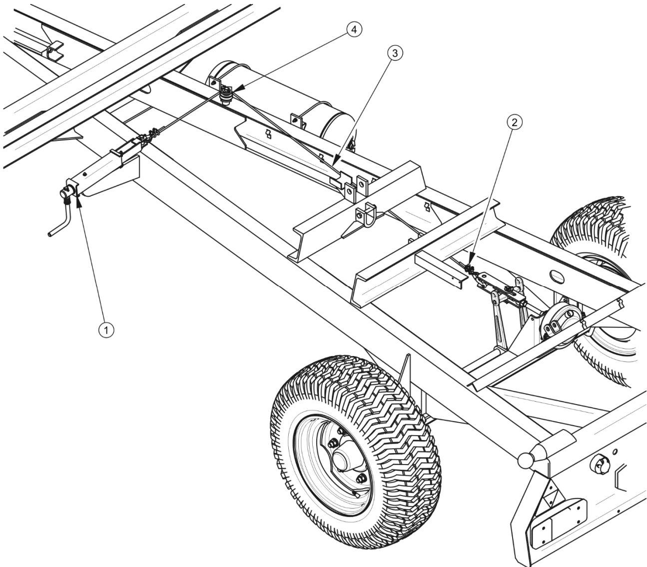
ABBILDUNG 5.6 Einstellen Bremsseilspannung der Feststellbremse
