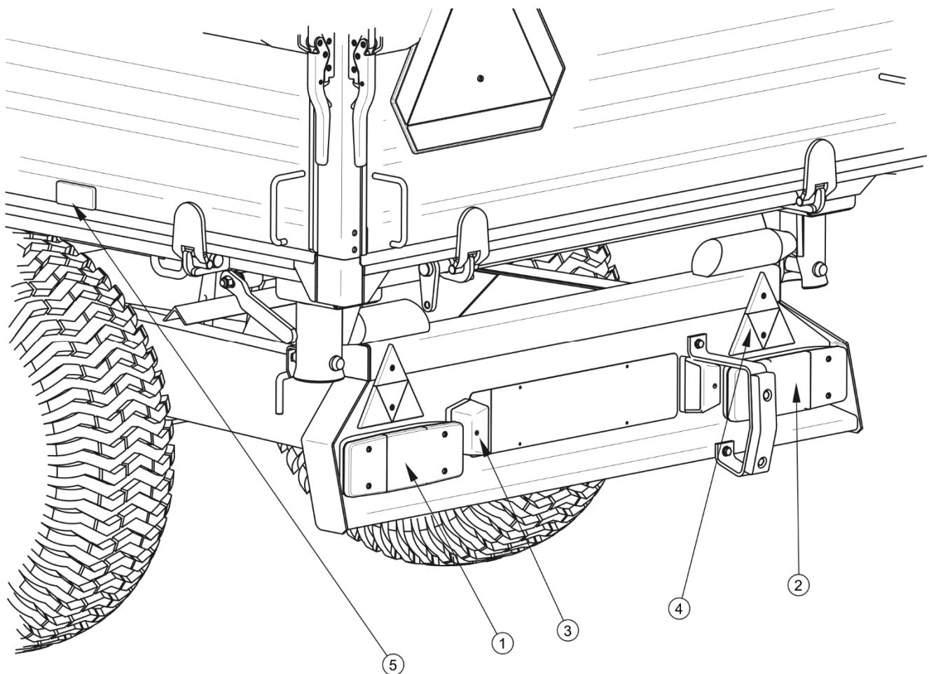
ABBILDUNG 3.13 Anordnung der Elemente der Elektroinstallation und der Rückstrahler – Rückansicht
