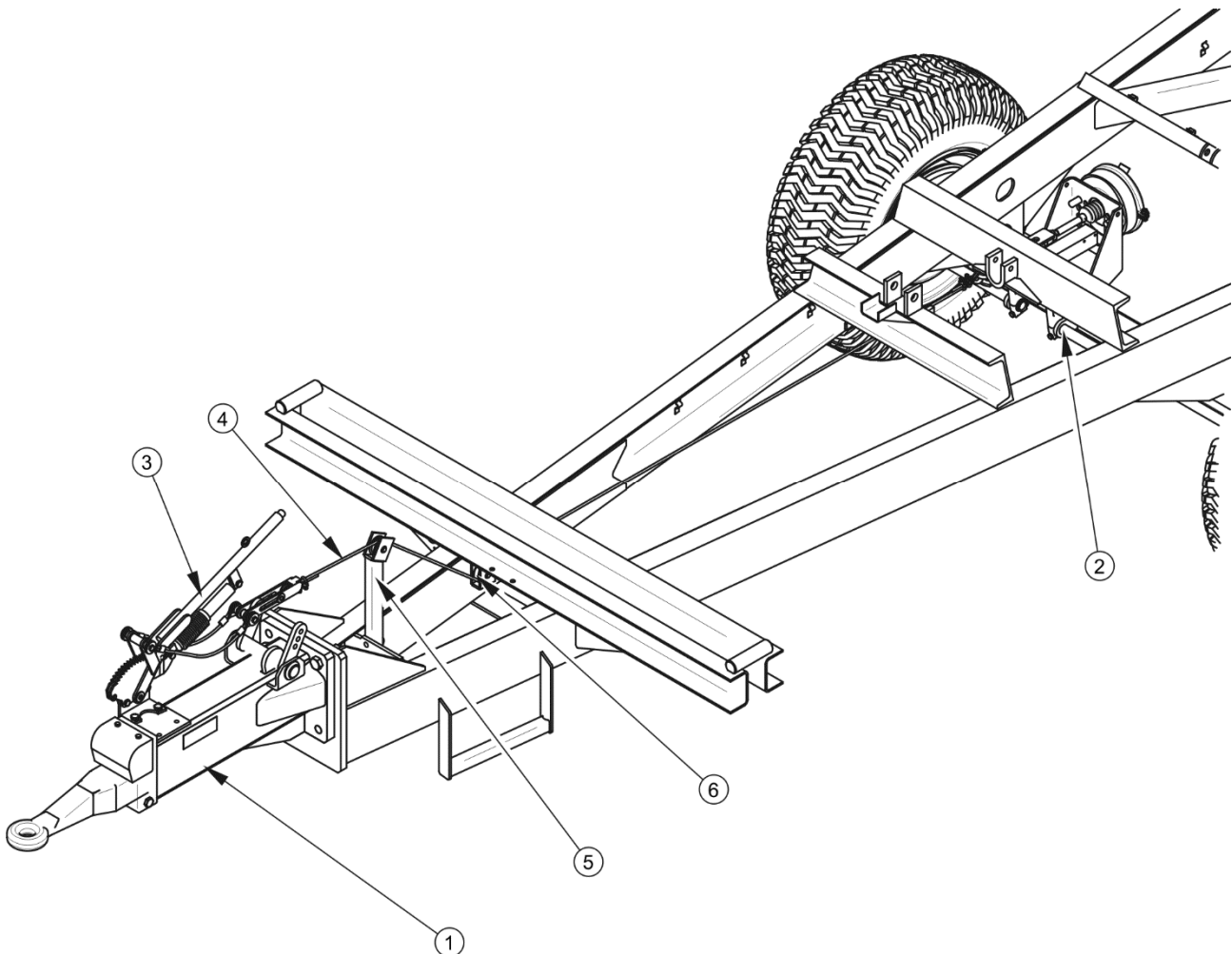
ABBILDUNG 3.8 Auffahrbremse
