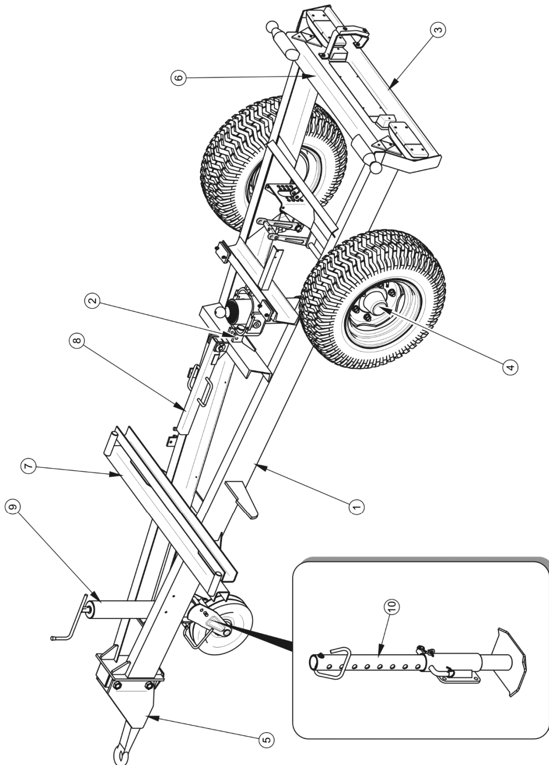
ABBILDUNG 3.1 Fahrgestell des Anhängers
