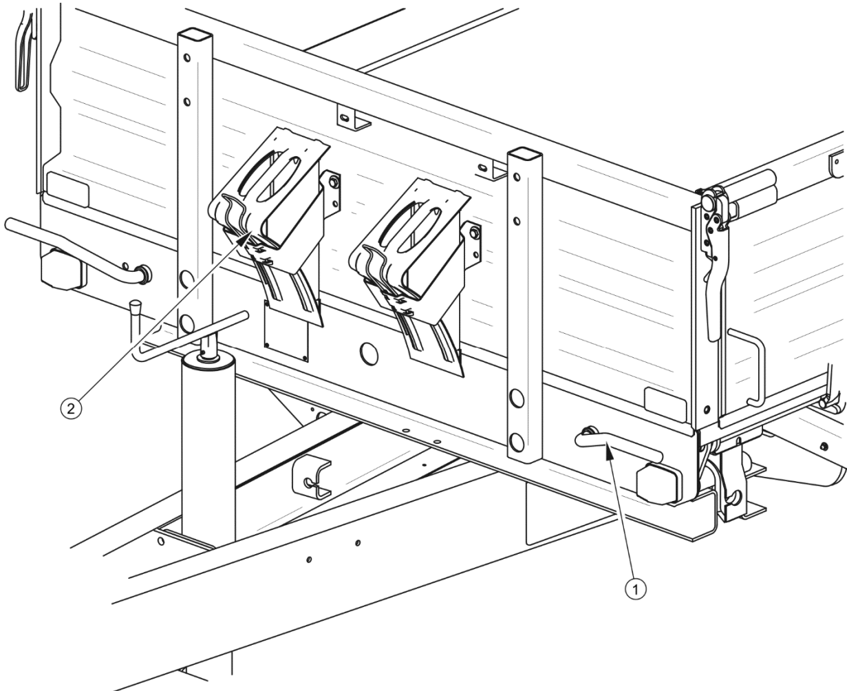
ABBILDUNG 3.4 Ladekasten - Vorderansicht
