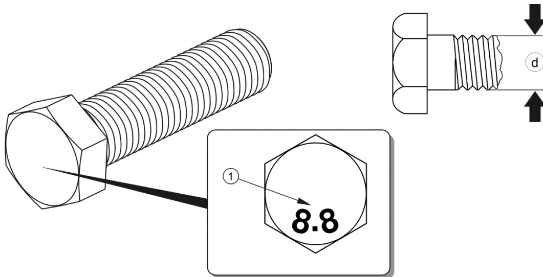
ABBILDUNG 5.11 Schraube mit metrischem Gewinde
