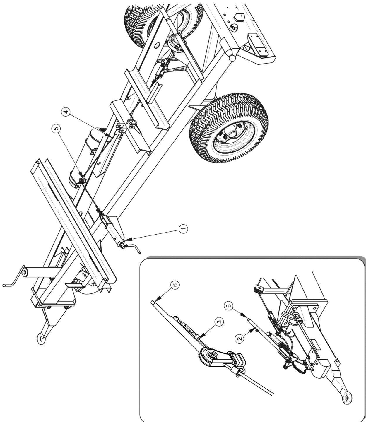
ABBILDUNG 3.11 Aufbau der Feststellbremse mit dem Kurbelmechanismus
