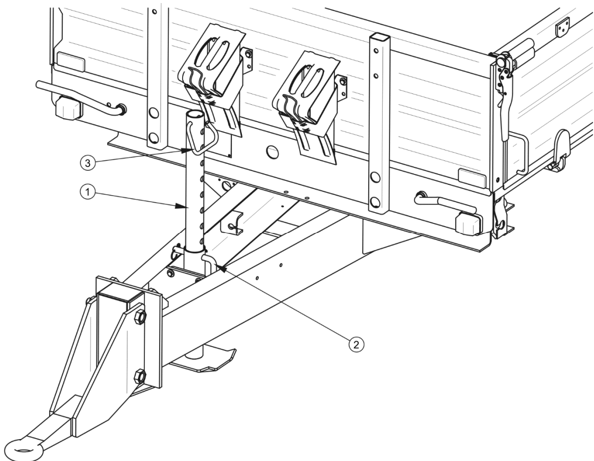
ABBILDUNG 4.2 Gerade Stütze des Anhängers
