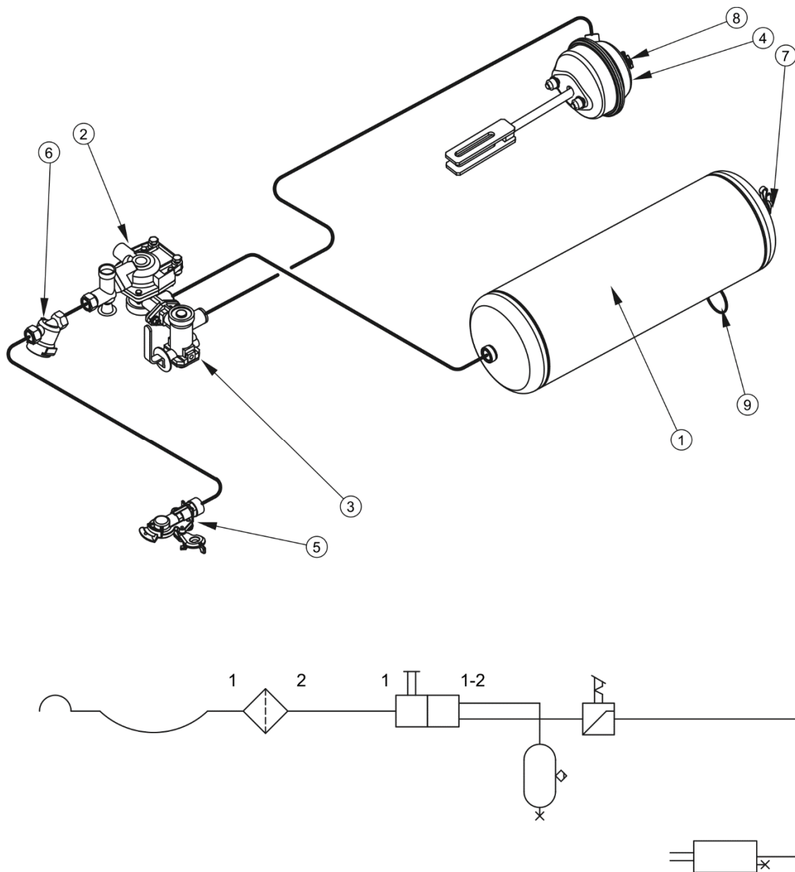
ABBILDUNG 3.6 Aufbau und Schema der Einkreis-Druckluftbremse
