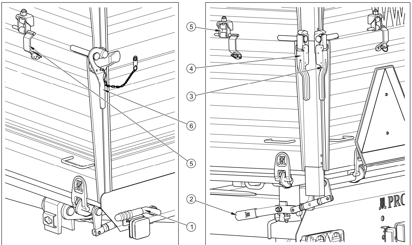
RYSUNEK 4.4 Zamki ścian i nadstaw skrzyniowych
