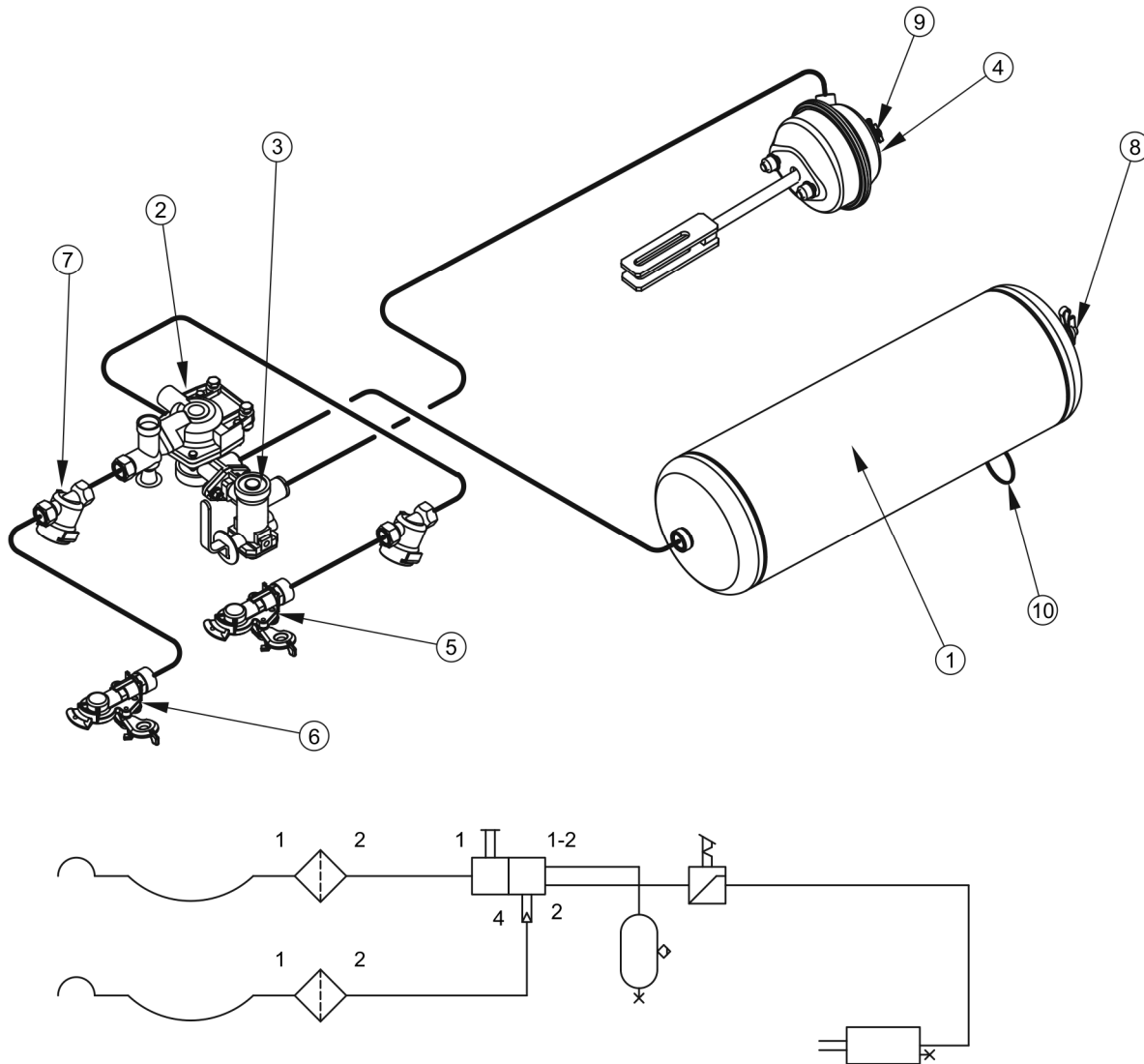
RYSUNEK 3.6 Budowa i schemat instalacji hamulcowej pneumatycznej dwuprzewodowej
