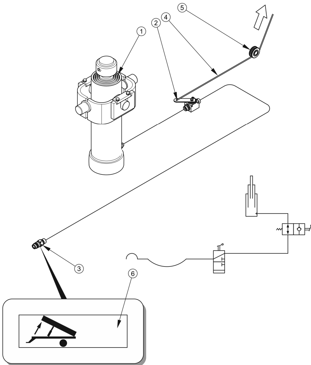
RYСУNEK 3.11 Budowa i schemat instalacji hydraulicznej wywrotu
