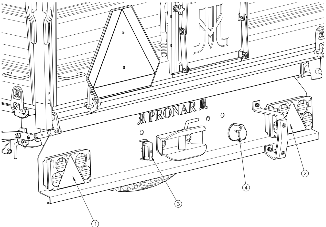
RYSUNEK 3.14 Rozmieszczenie elementów instalacji oświetleniowej – widok z tyłu
