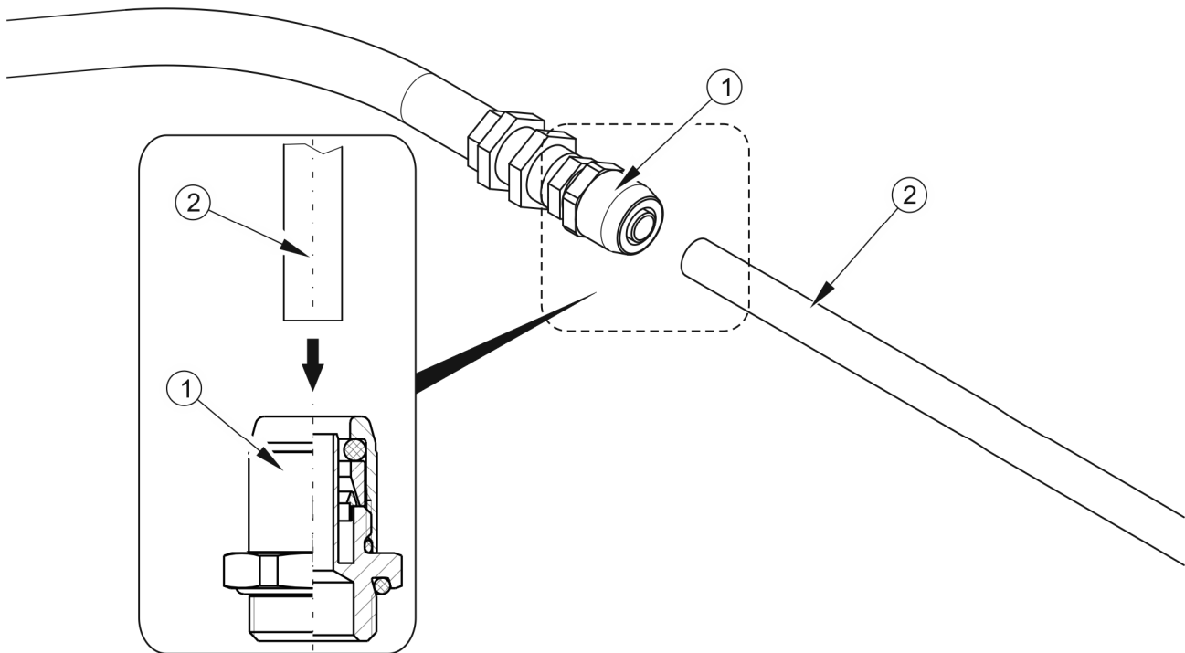
RYSUNEK 5.12 Montaż przewodu pneumatycznego
