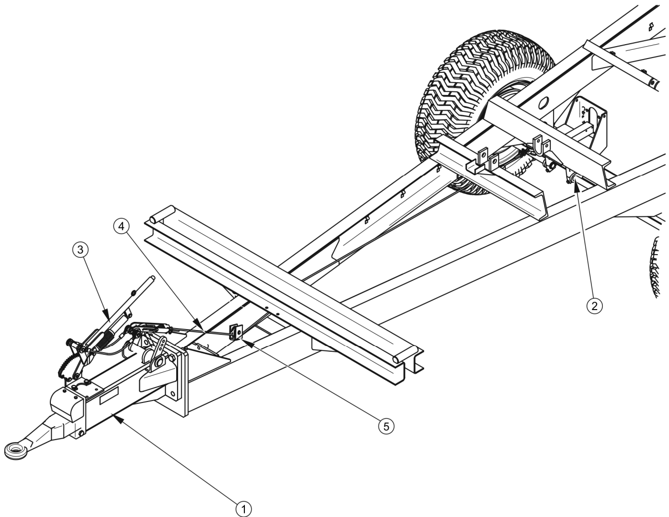
RYСУNEK 3.9 Hamulec najzdowy
