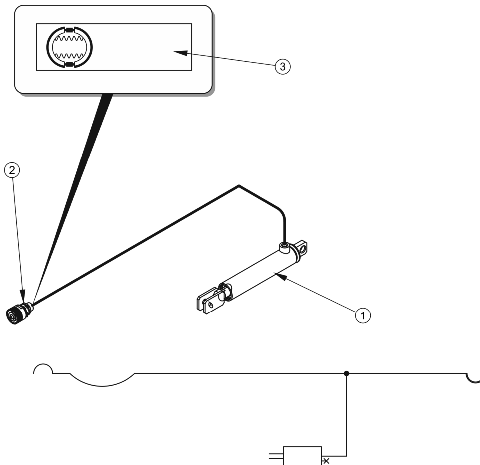
RYSUNEK 3.8 Budowa i schemat instalacji hamulcowej hydraulicznej
