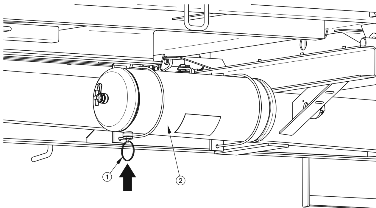
RYСУNEK 5.11 Odwadnianie zbiornika powietrza
