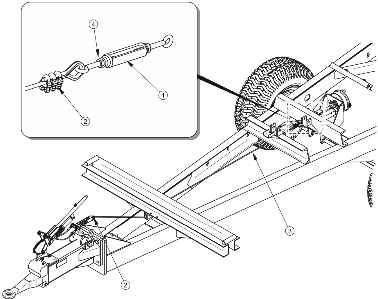
RYSUNEK 5.7 Regulacja napięcia linki hamulca najzdowego
