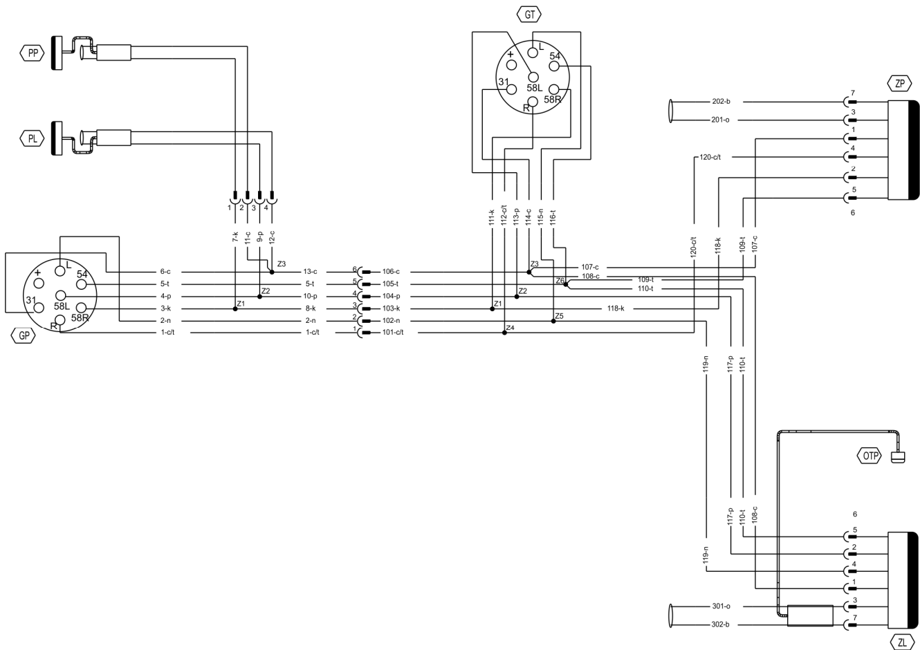
RYSUNEK 3.13 Schemat ideowy instalacji elektrycznej
