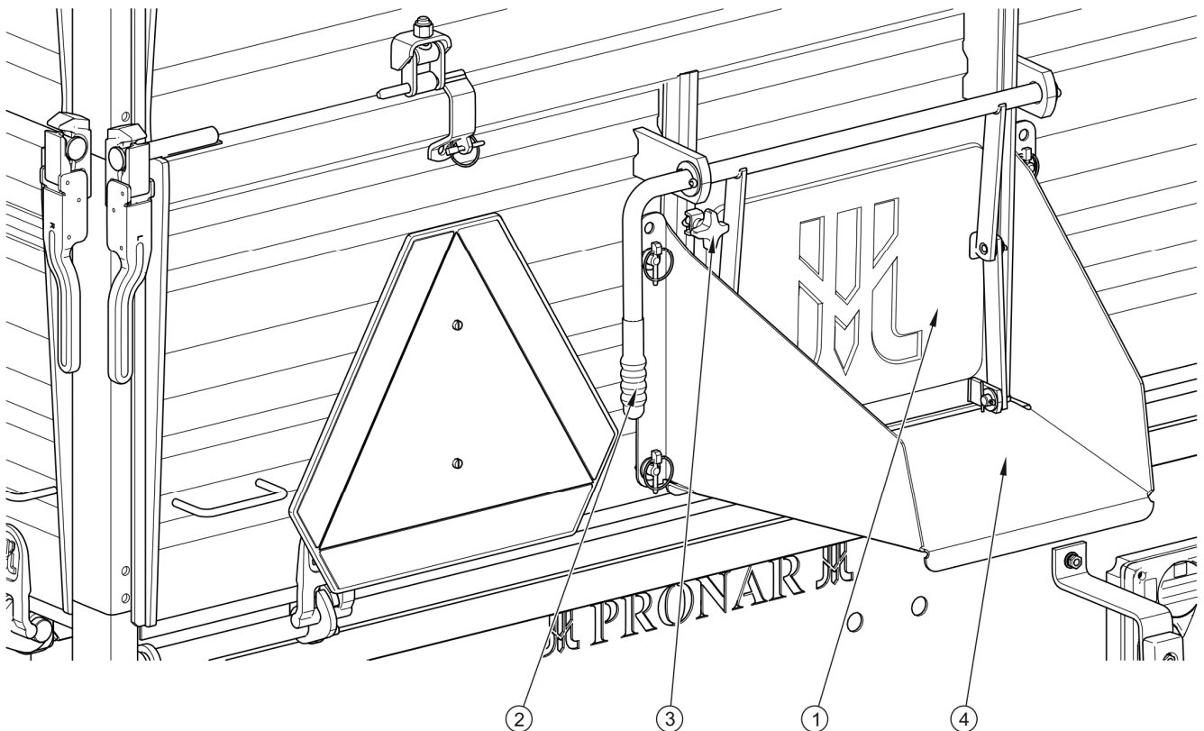
RYСУNEK 3.5 Zasuwa ściany tylnej z blokadą i rynna zsypową
