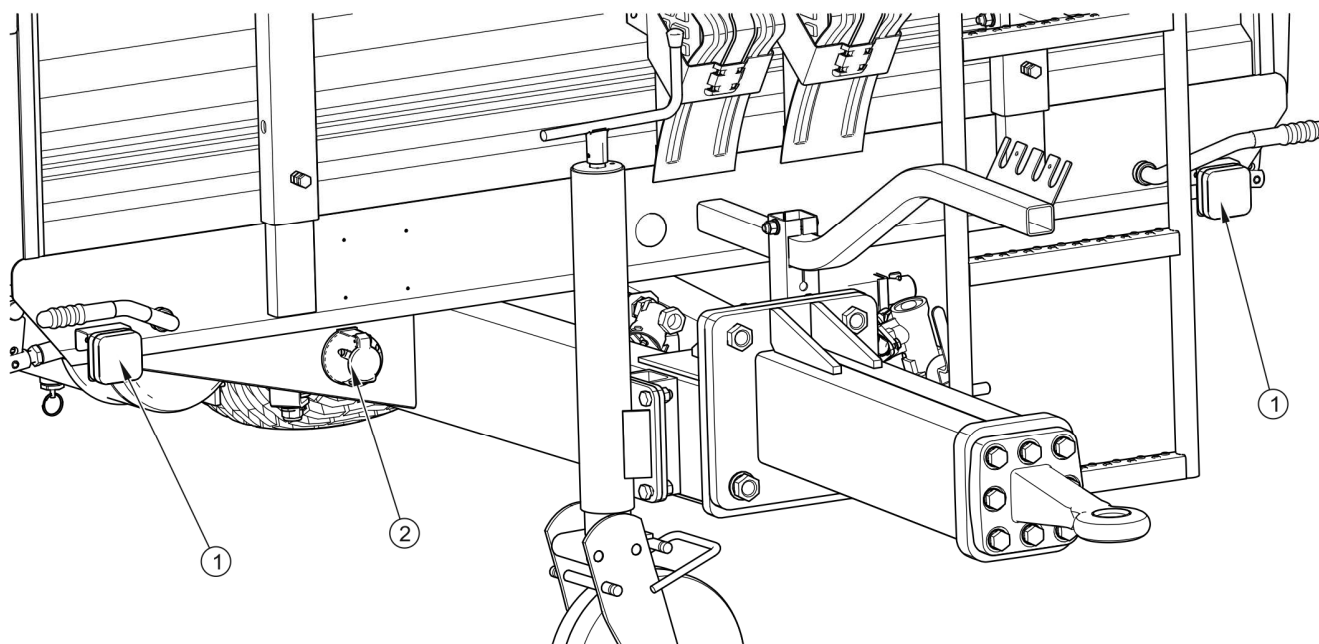
RYSUNEK 3.15 Rozmieszczenie elementów instalacji oświetleniowej – widok z przodu
