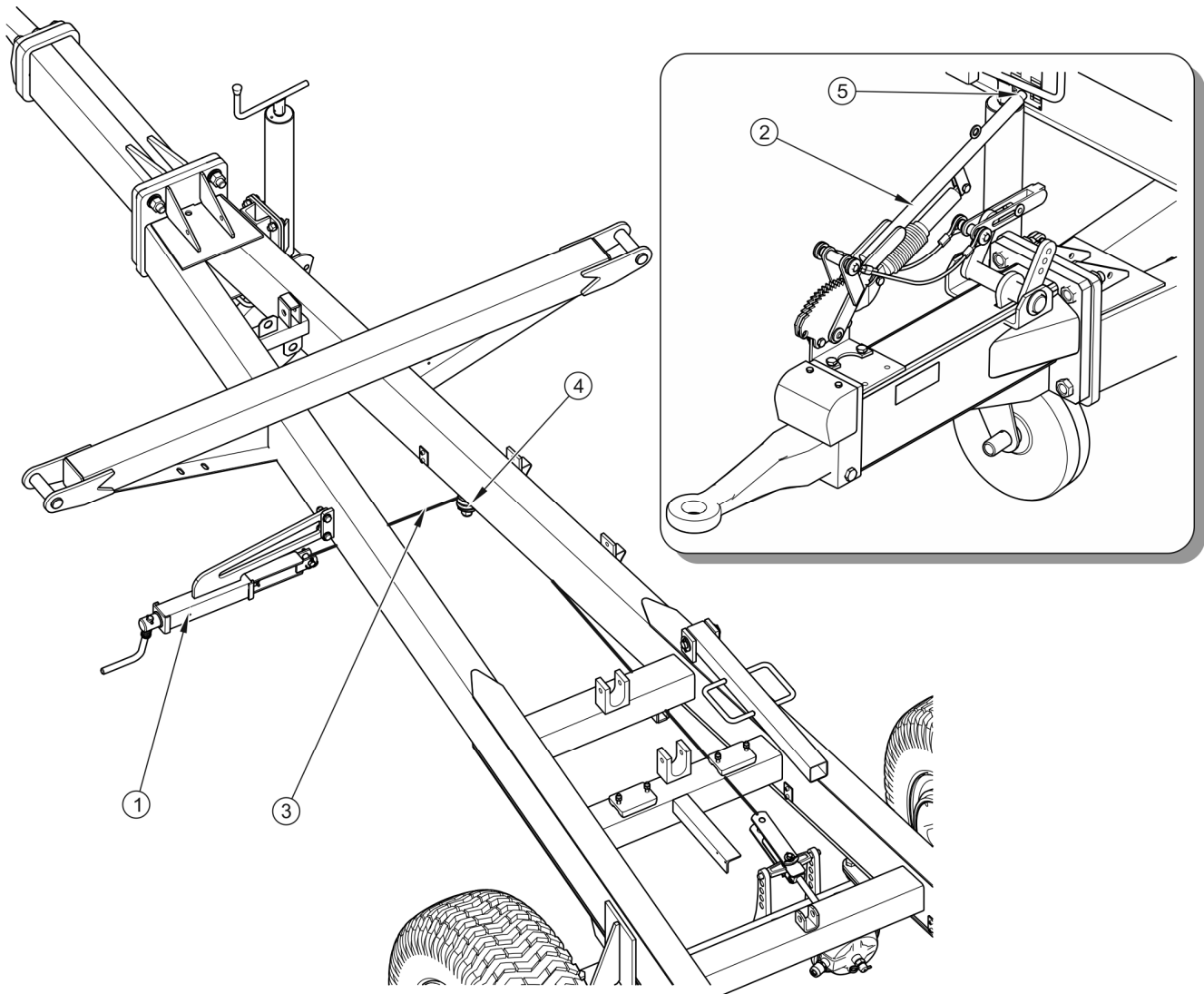
RYSUNEK 3.12 Budowa hamulca postojowego
