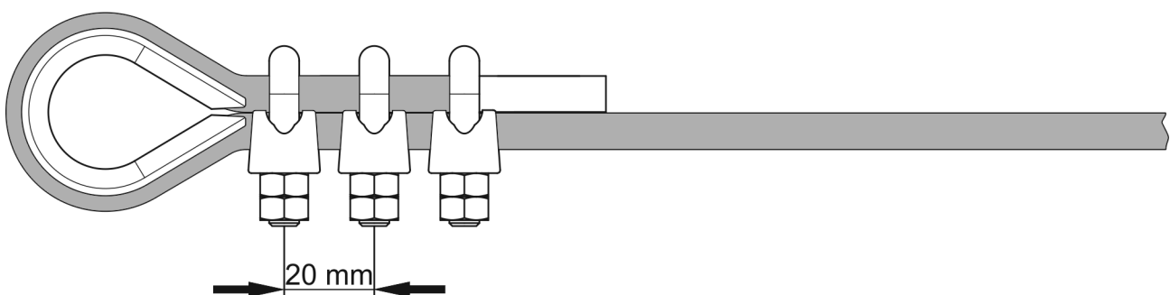
RYСУNEK 5.9 Montaż zacisków linki hamulcowej
