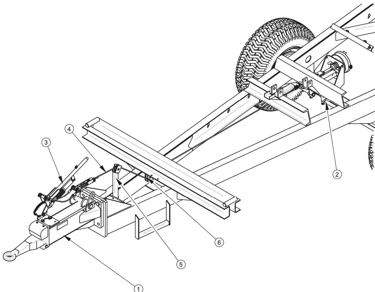
Obrázek 3.9 Nájezdová brzda
