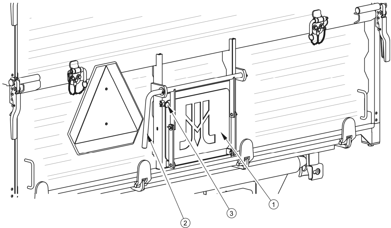
Obrázek 3.5 Dvířka zadní bočnice
