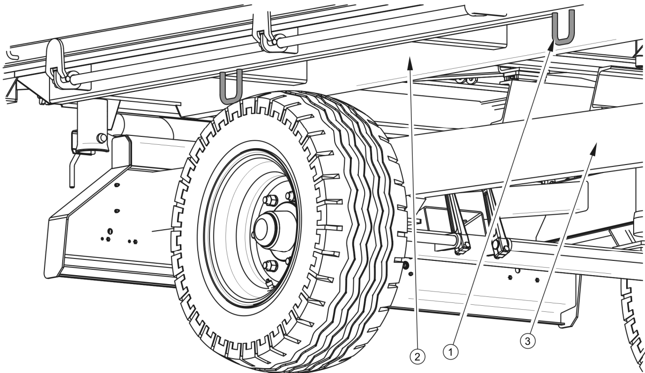
Obrázek 1.3 Rozmístění přepravních držáků
