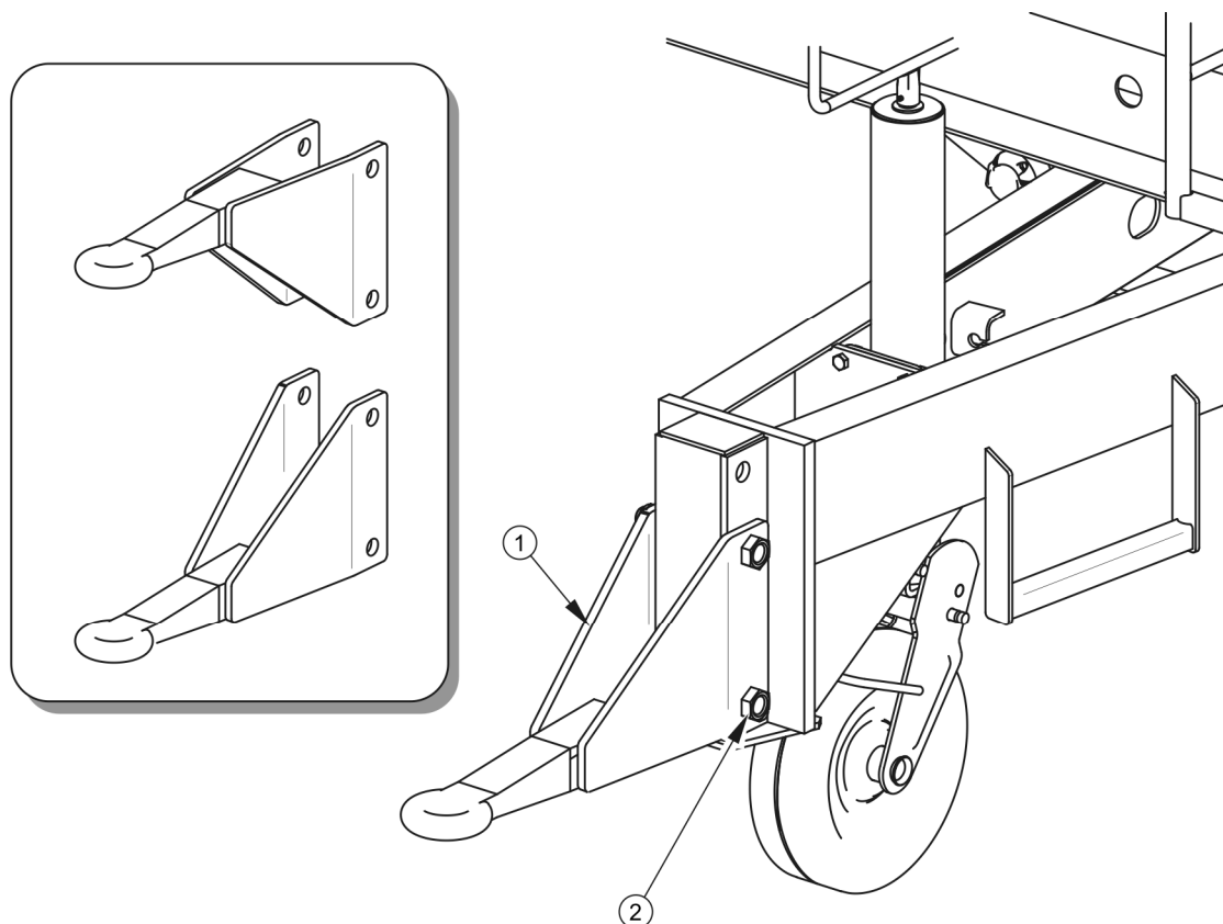
Obrázek 5.12 Seřízení polohy oje
