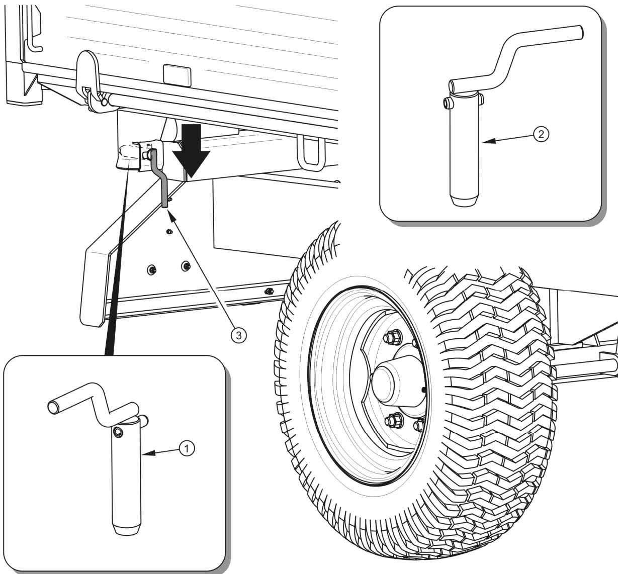
Obrázek 4.3 Zajišťování čepů sklápění
