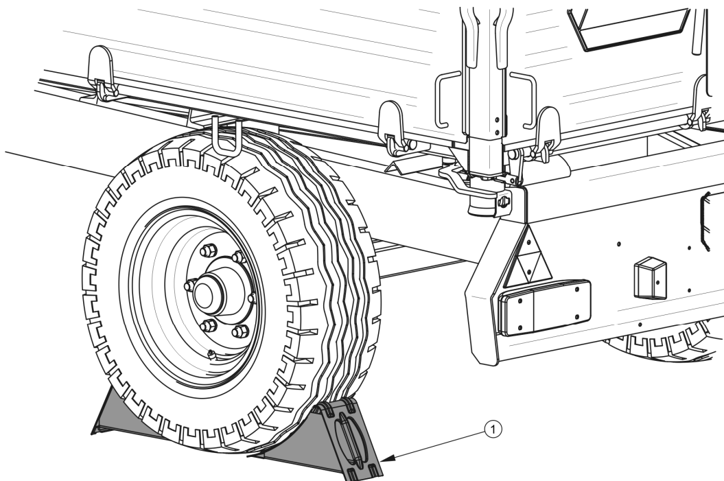
Obrázek 2.1 Správný způsob podložení klínů
