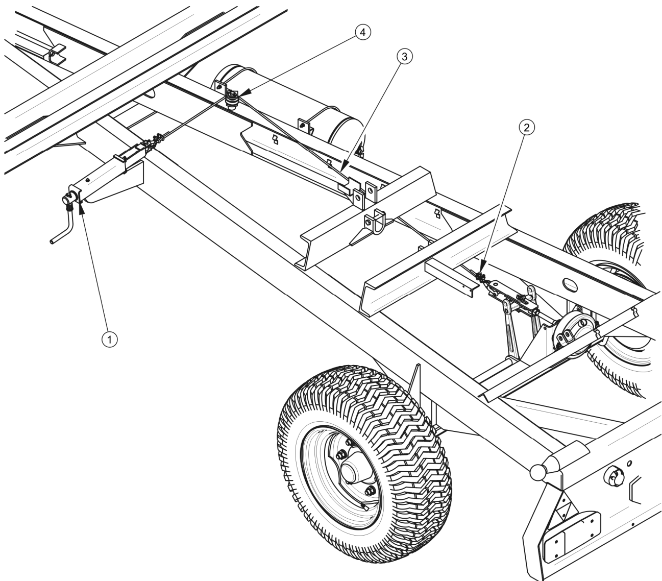
Obrázek 5.6 Seřízení napnutí lanka parkovací brzdy
