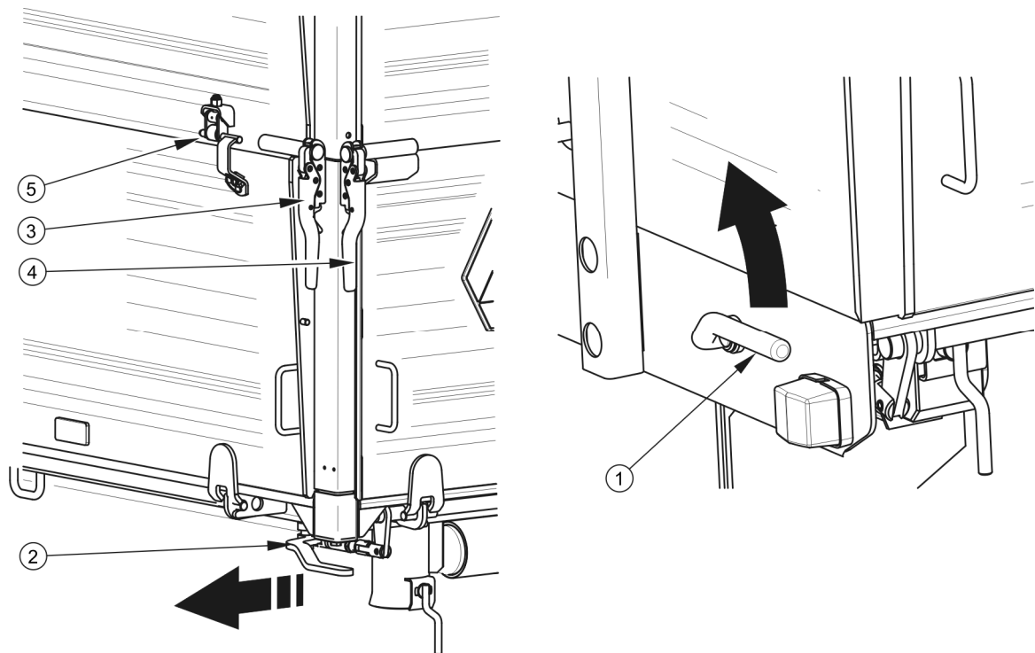
Obrázek 4.4 Zámky bočnic a skříňových nástavek
