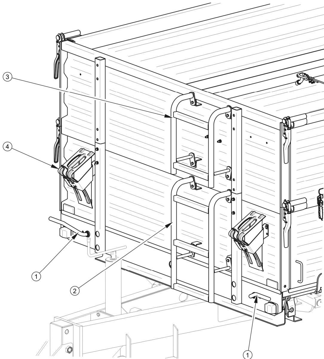
Obrázek 3.4 Korba – pohled zepředu
