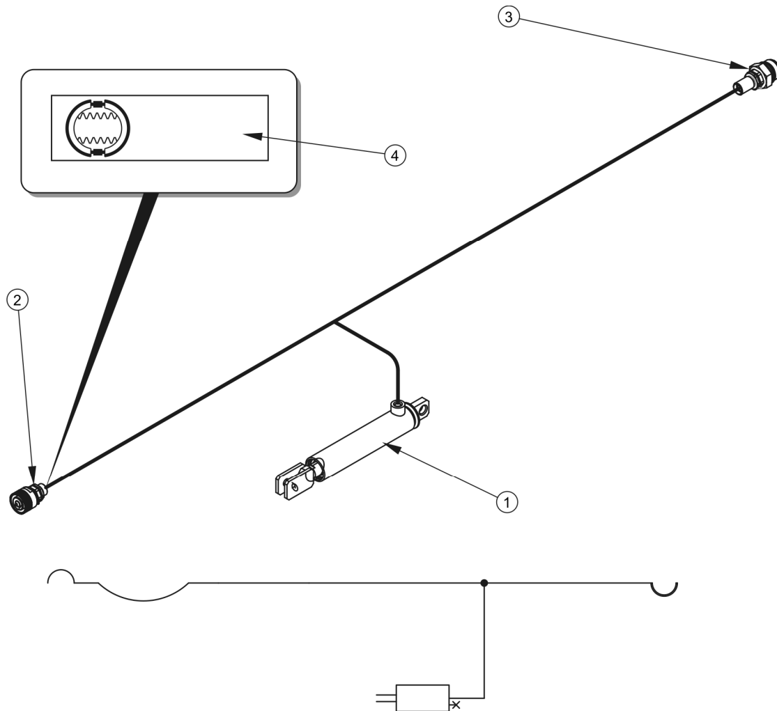
Obrázek 3.8 Konstrukce a schéma hydraulické brzdové instalace
