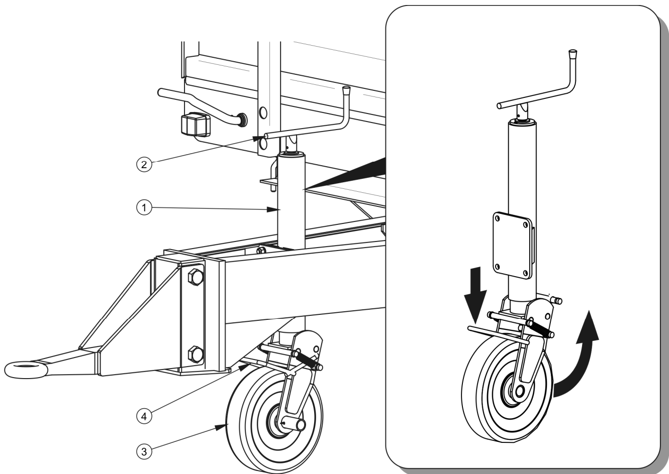
Obrázek 4.1 Podpěra přívěsu
