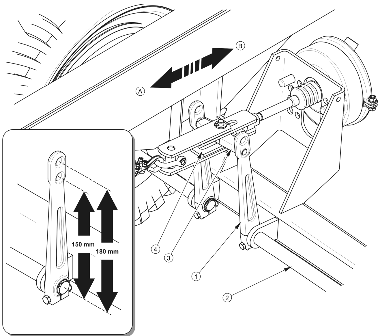
Obrázek 5.4 Seřízení mechanických brzd pojezdové nápravy
