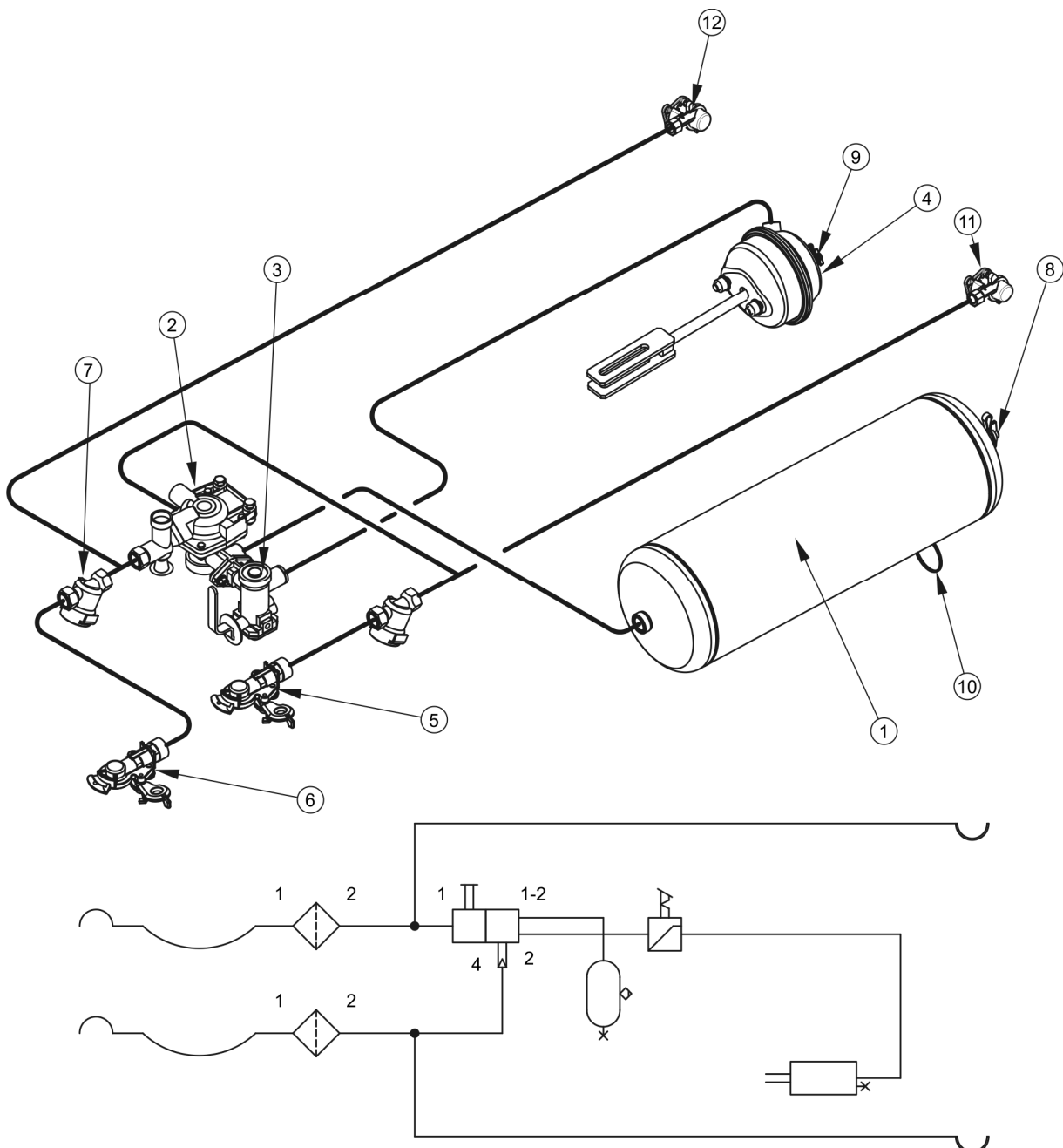
Obrázek 3.6 Konstrukce a schéma vzduchové brzdové dvouhadicové instalace
