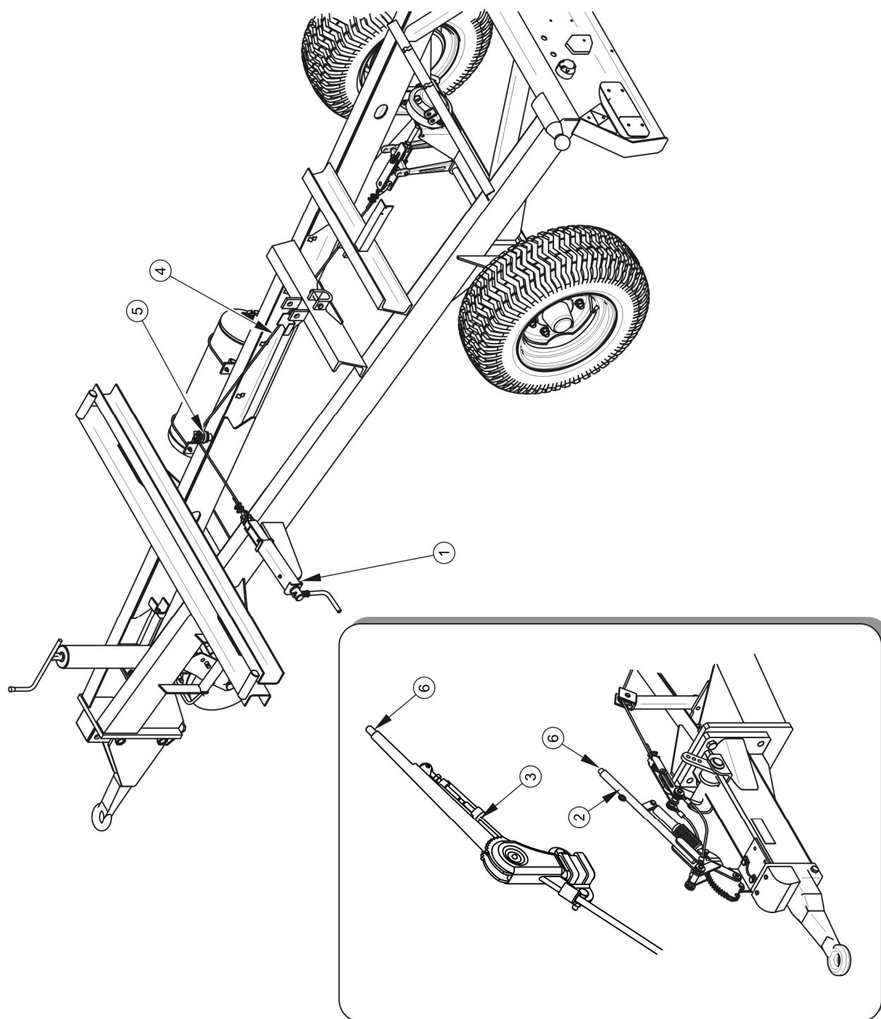
Obrázek 3.12 Konstrukce parkovací brzdy s klikovým mechanismem
