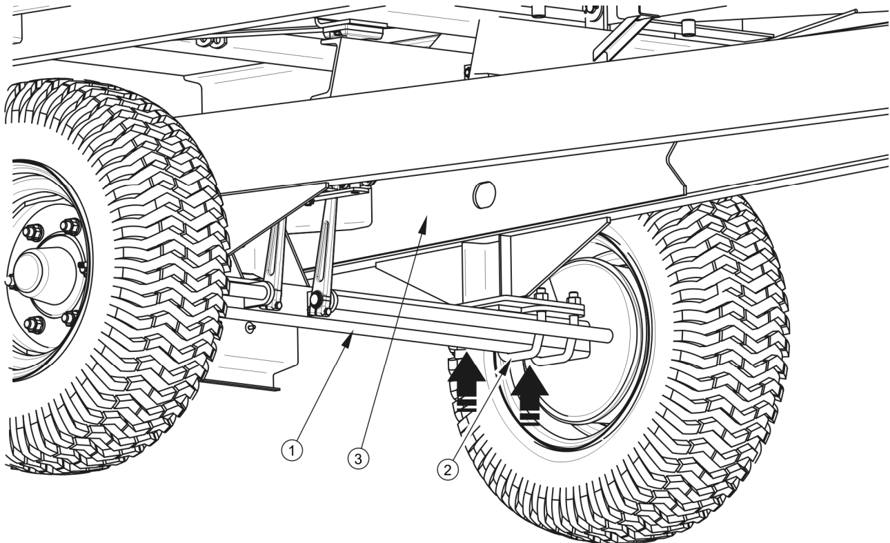
Obrázek 5.1 Podpěrný bod zvedáku
