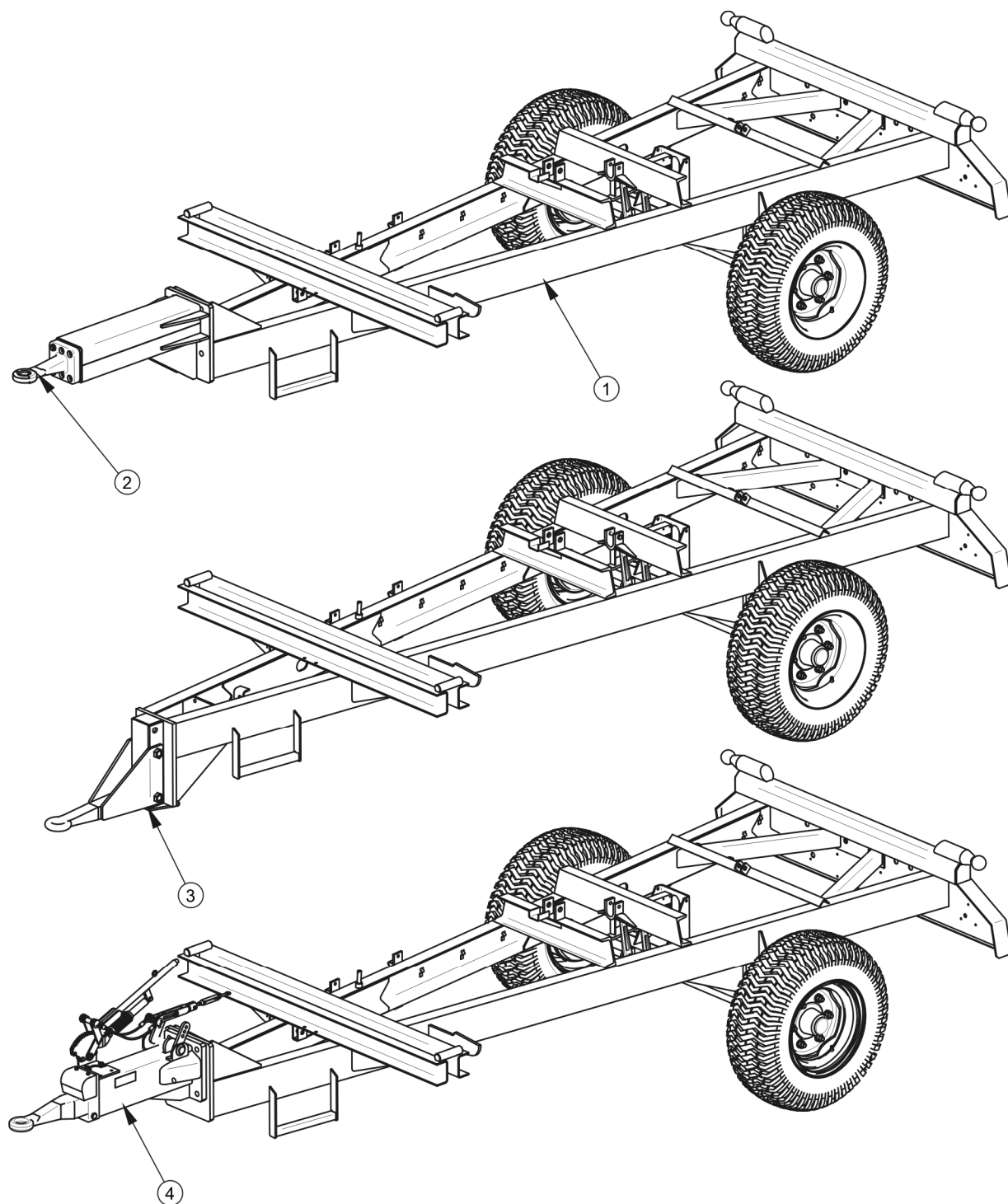
Obrázek 3.2 Varianty spodního rámu
