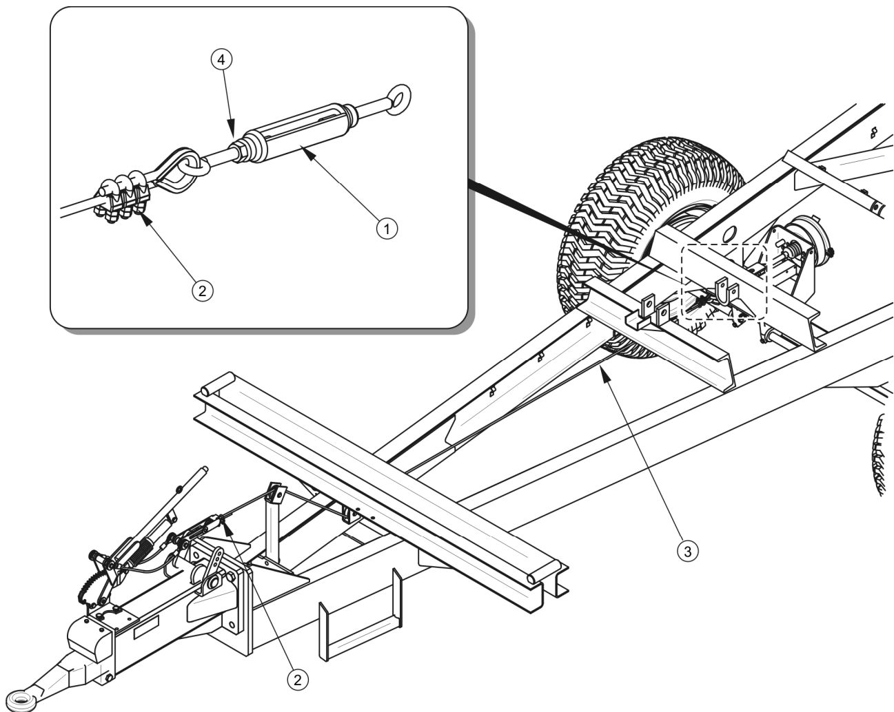
Obrázek 5.5 Seřízení napnutí lanka nájezdové brzdy
