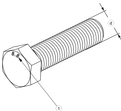
Obrázek 5.11 Šroub s metrickým závitem
