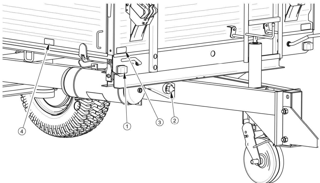
Obrázek 3.15 Rozmístění prvků elektroinstalace a odrazových skel – pohled zepředu
