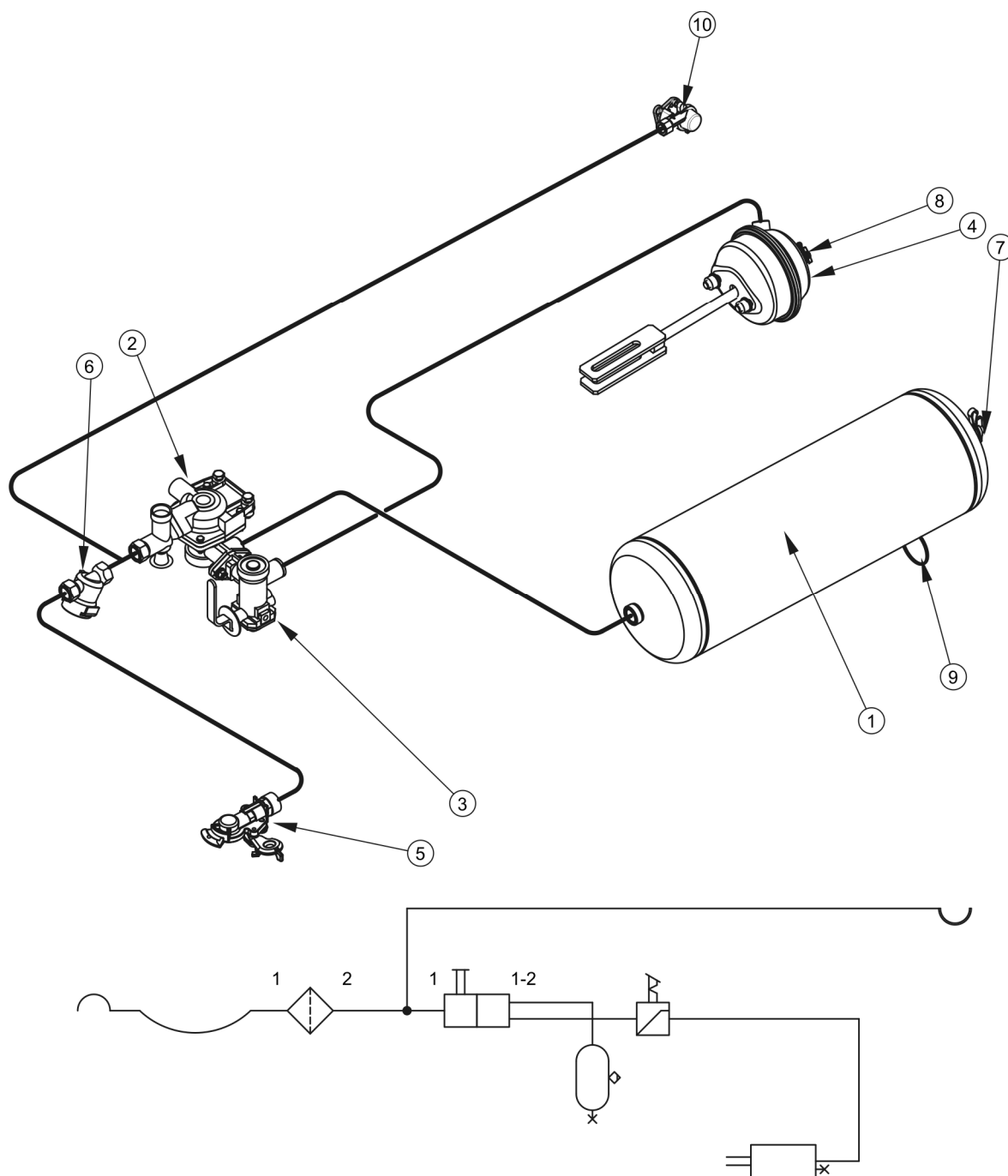
Obrázek 3.7 Konstrukce a schéma vzduchové jednohadicové brzdové instalace
