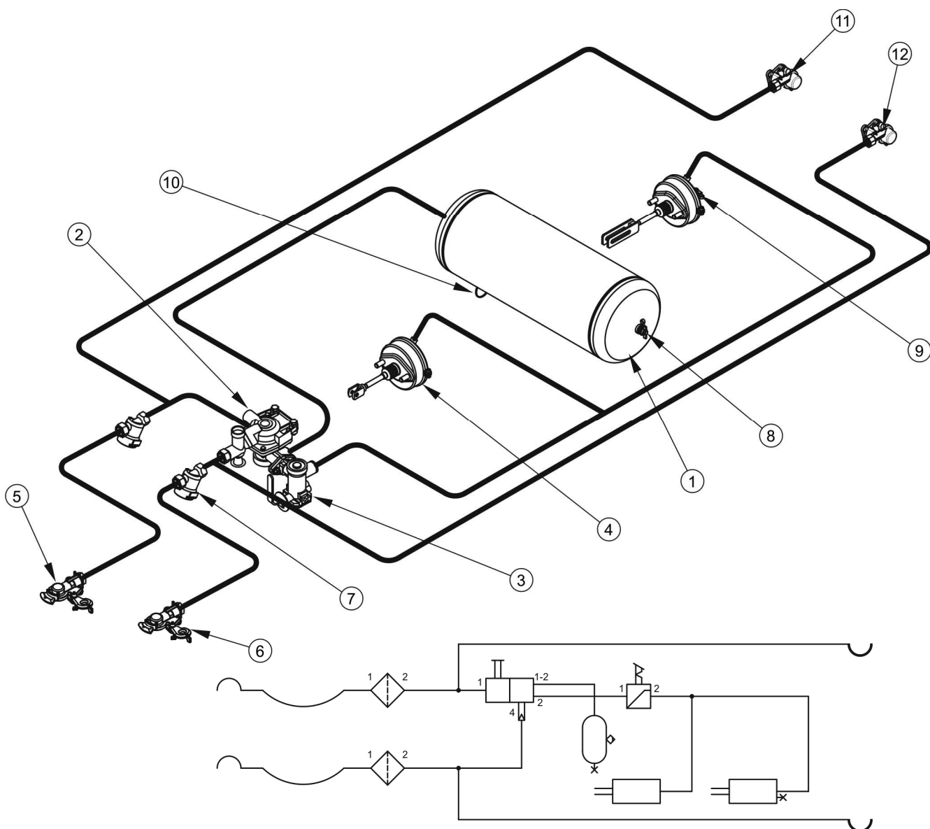
Obrázek 3.5 Konstrukce a schéma vzduchové brzdové dvouhadicové instalace
