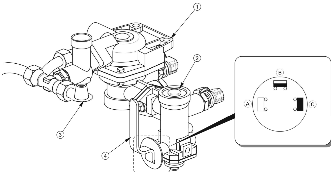
Obrázek 3.9 Ovládací ventil a regulátor brzdné síly
