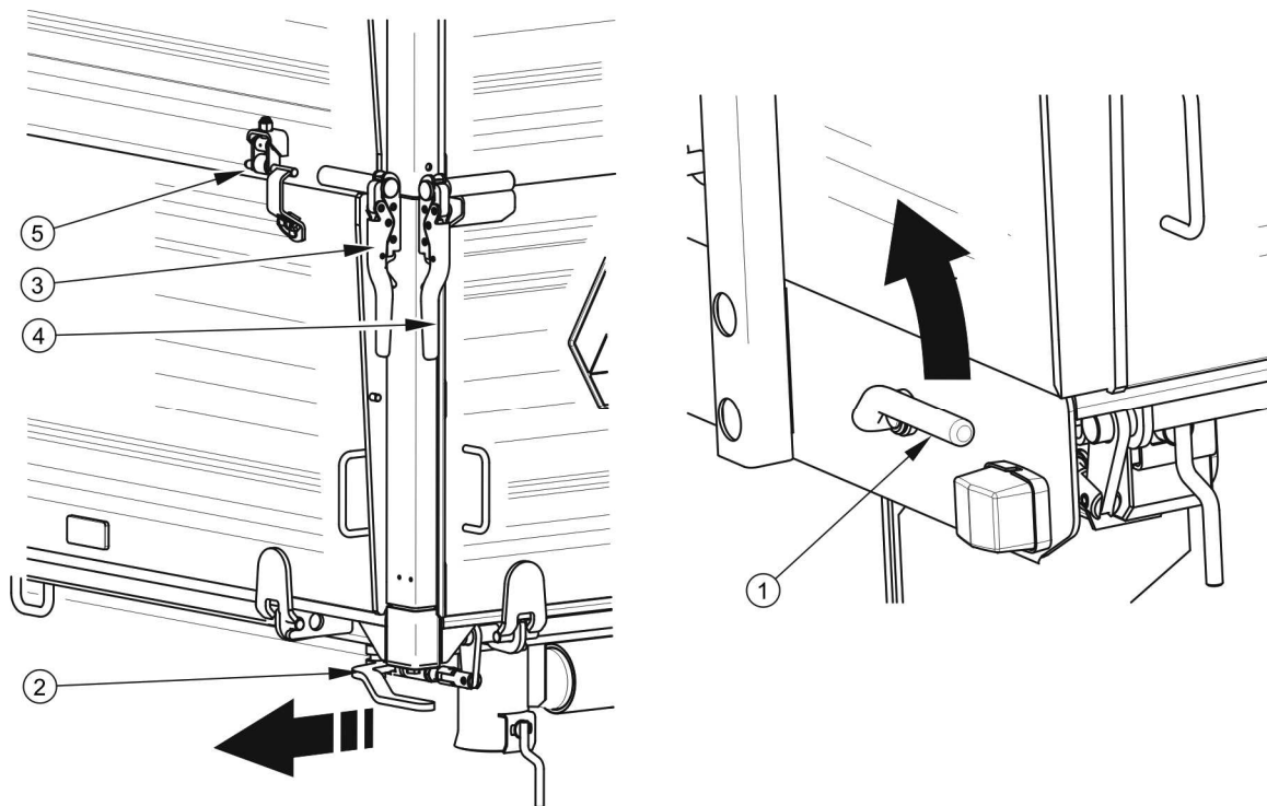
Obrázek 4.4 Zámky bočnic a skříňových nástavek
