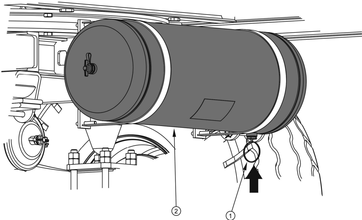
Obrázek 5.8 Odvodňování vzdušníku
