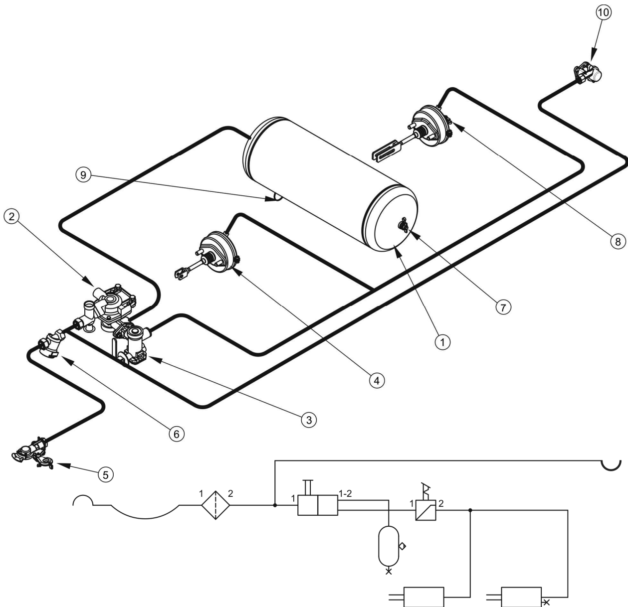
Obrázek 3.6 Konstrukce a schéma vzduchové jednohadicové brzdové instalace
