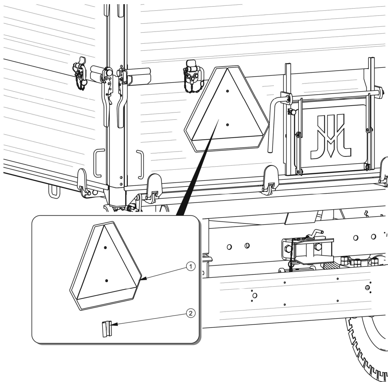
Obrázek 2.2 Místo montáže tabulky označující pomalá vozidla
