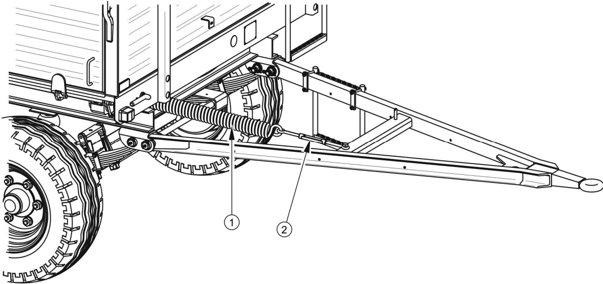
Obrázek 5.14 Seřízení polohy oje
