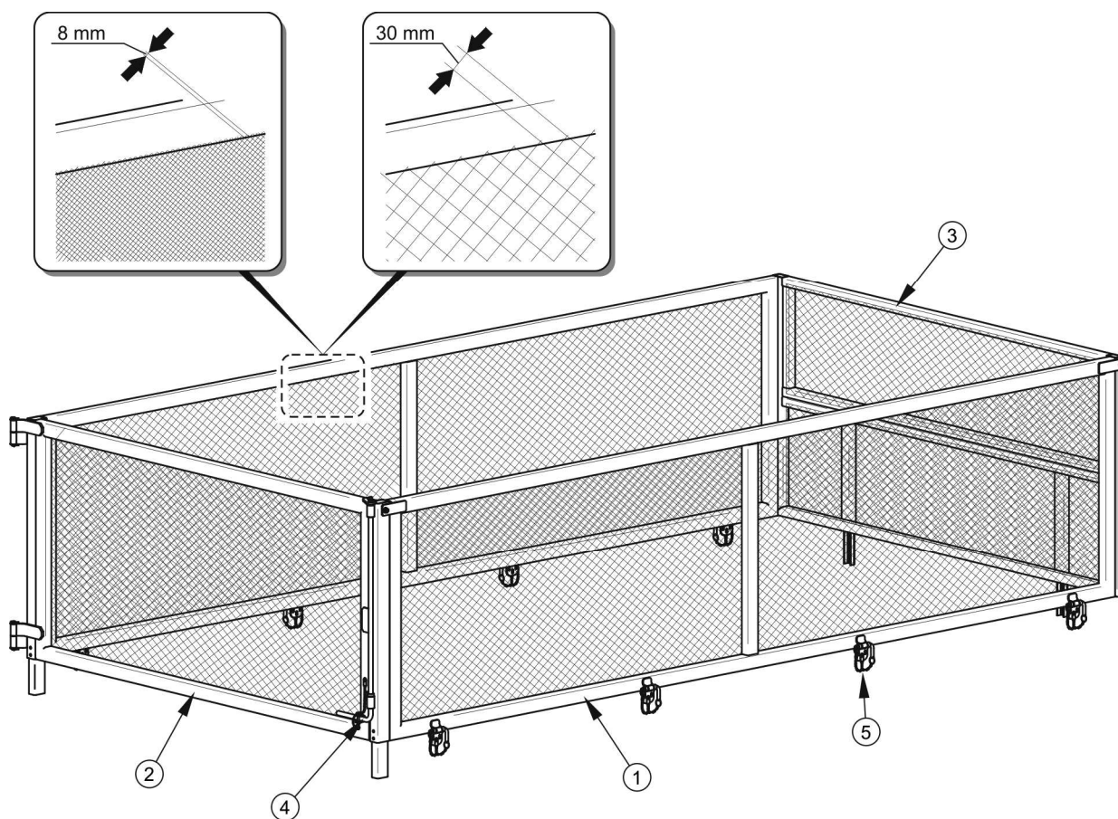
Obrázek 3.4 Pletivové nástavky 1 000 mm.
