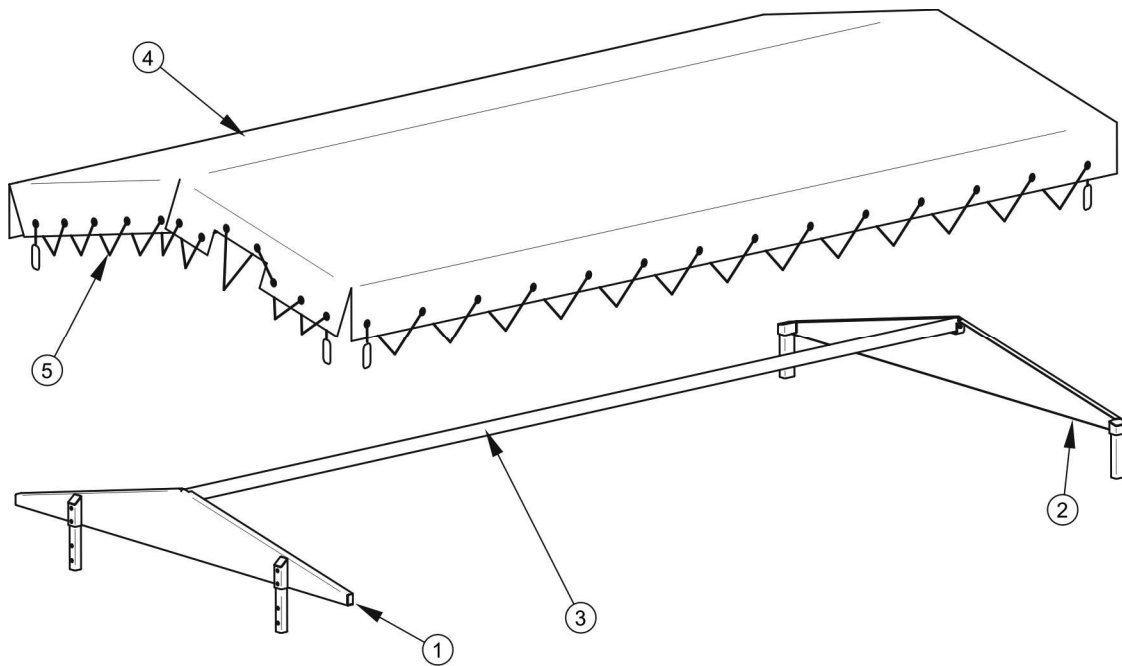
Obrázek 5.13 Podpěrná konstrukce s plachtou
