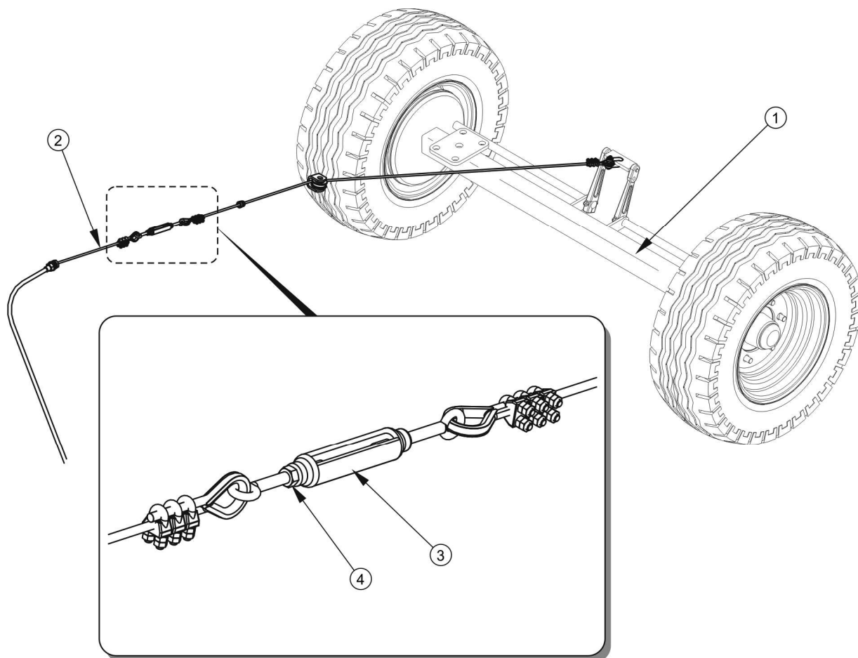
Obrázek 5.5 Seřízení napnutí lanka nájezdové brzdy
