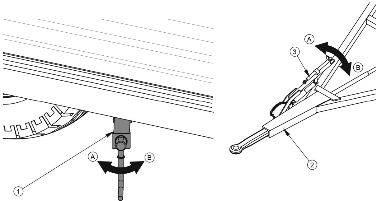
Obrázek 4.1 Parkovací brzda
