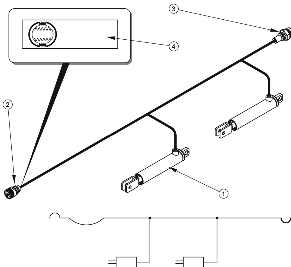
Obrázek 3.7 Konstrukce a schéma hydraulické brzdové instalace
