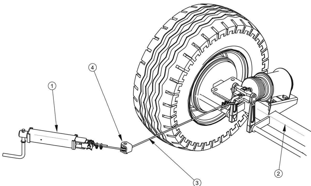
Obrázek 3.11 Konstrukce parkovací brzdy s klikovým mechanismem
