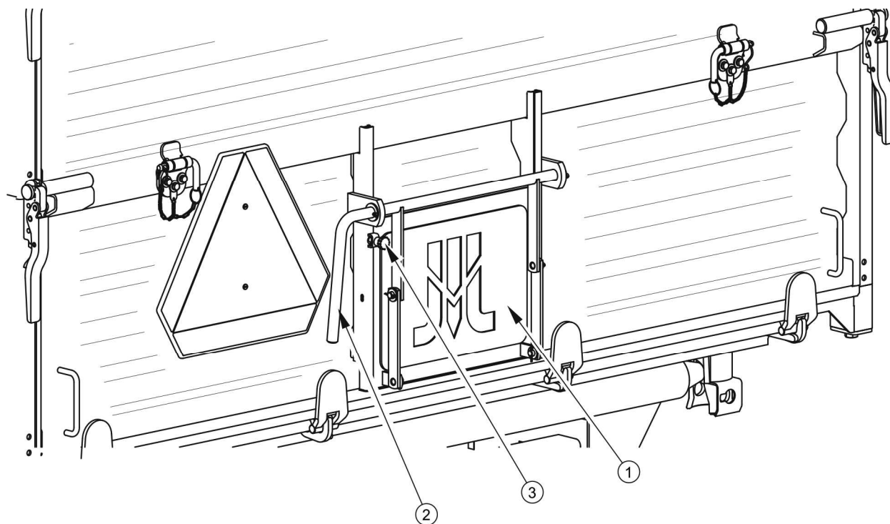
Obrázek 3.3 Dvířka zadní bočnice
