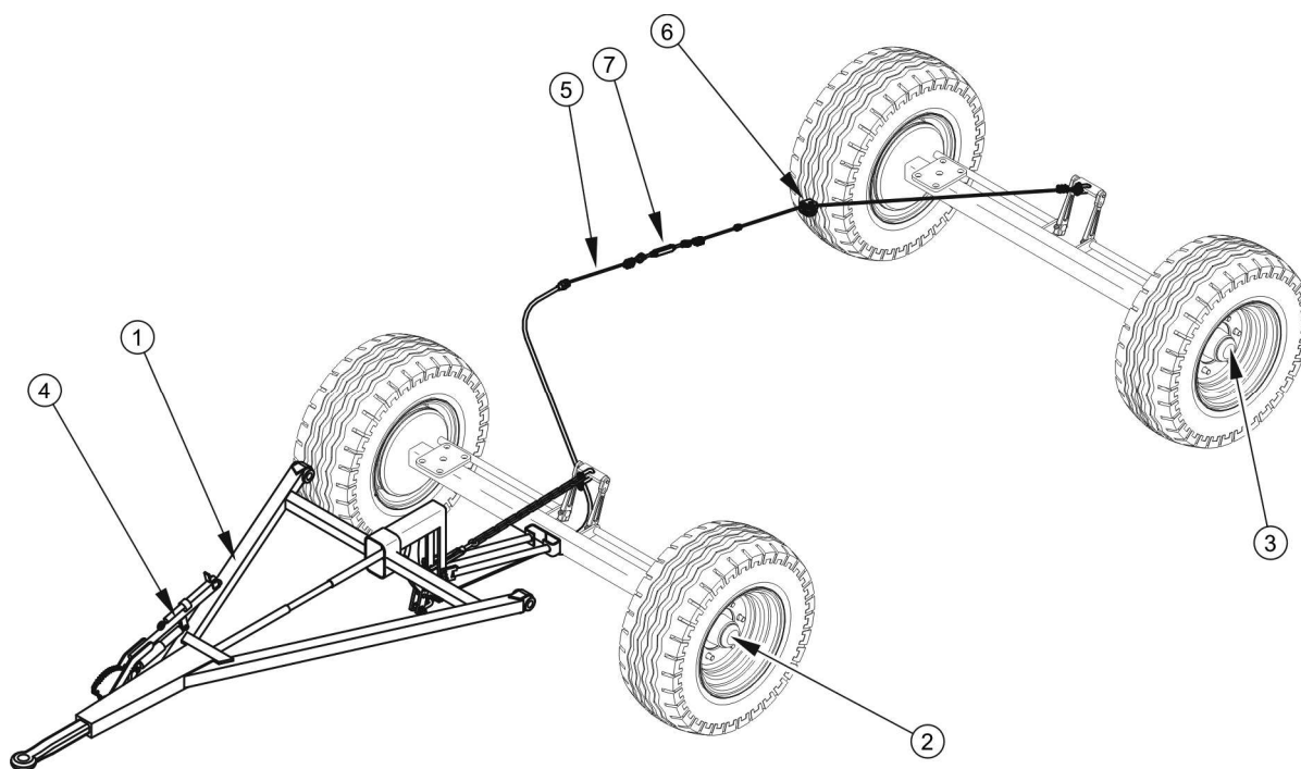
Obrázek 3.8 Nájezdová brzda
