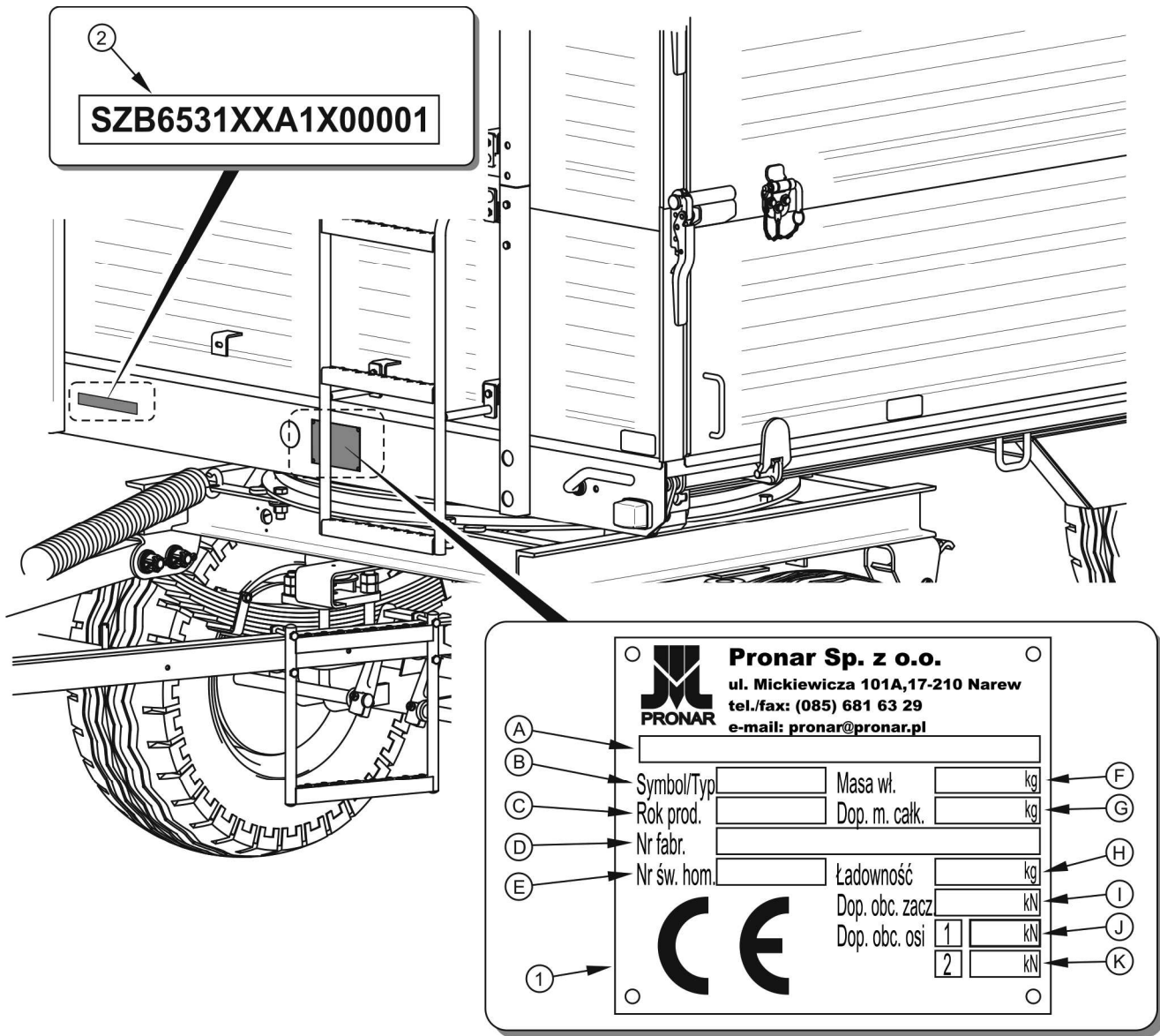
Obrázek 1.1 Místa umístění údajového štítku a vyražení výrobního čísla
