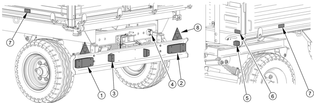
Obrázek 5.9 Součástí elektrovybavení a odrazová světla.
