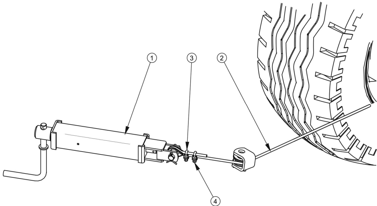
Obrázek 5.6 Seřízení napnutí lanka parkovací brzdy
