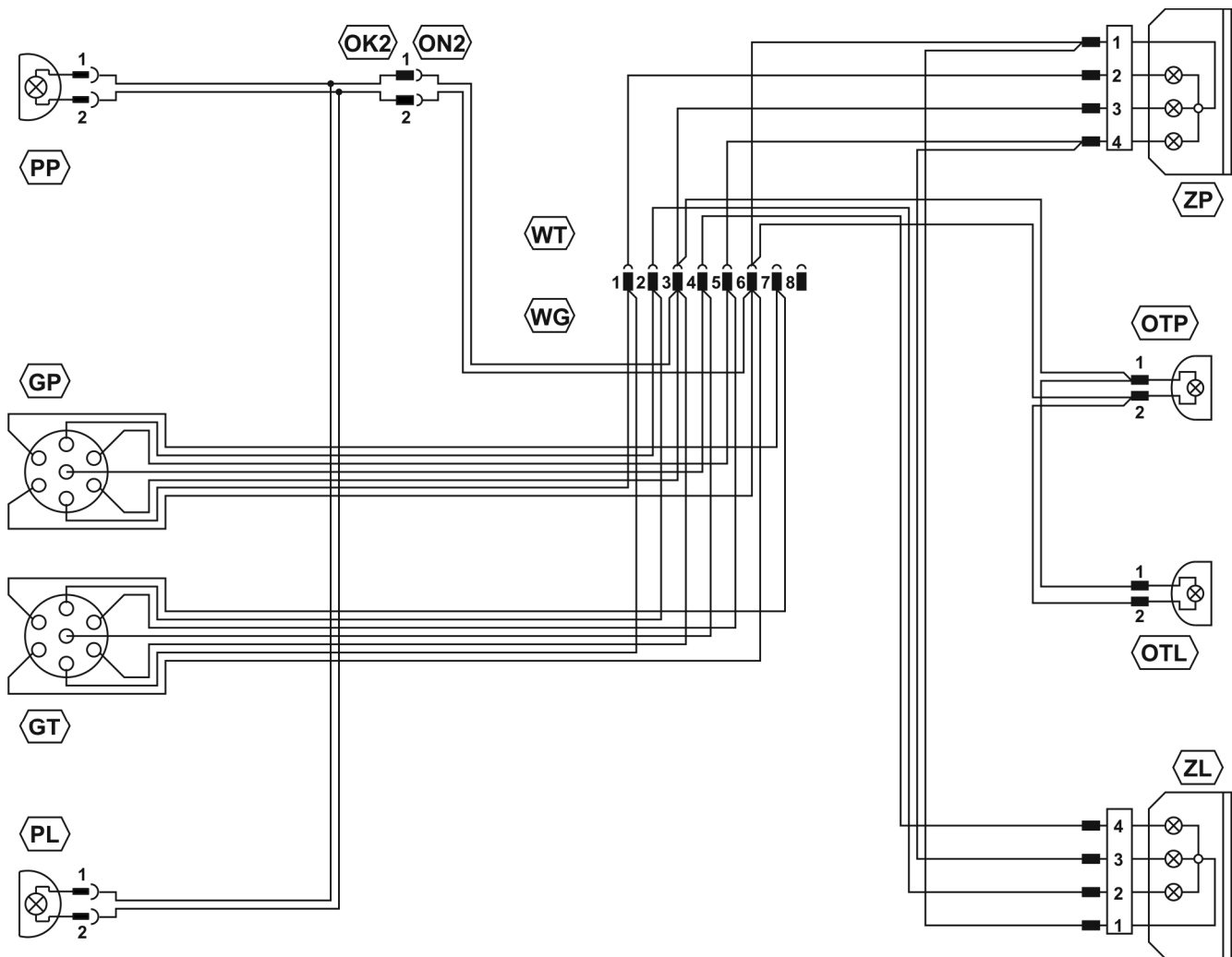
Obrázek 3.12 Ideové schéma elektroinstalace
