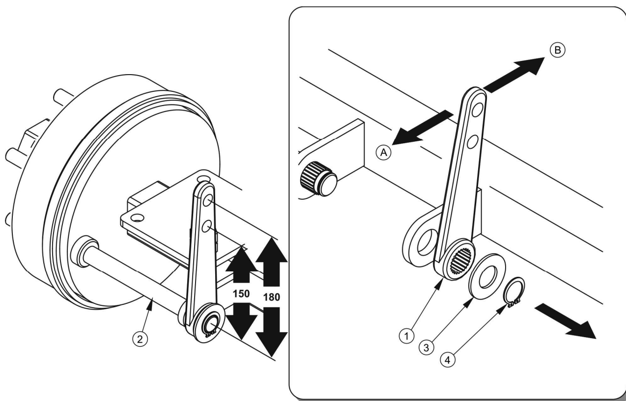
Obrázek 5.4 Seřízení mechanických brzd pojezdových náprav
