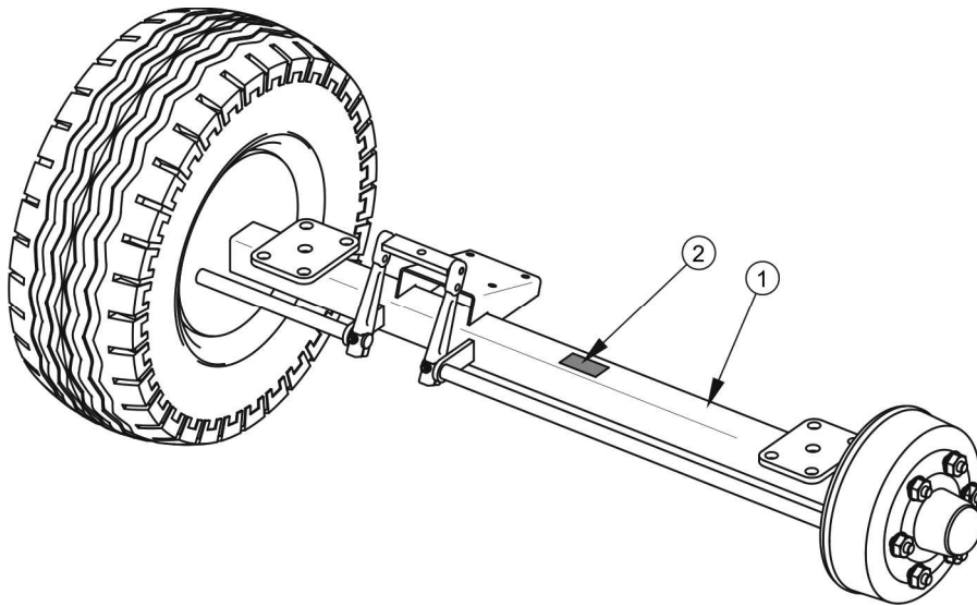
Obrázek 1.2 Místo umístění údajového štítku nápravy
