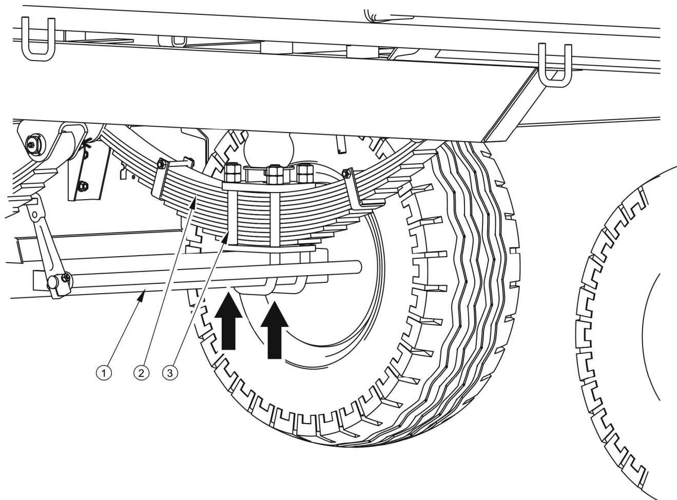
Obrázek 5.1 Podpěrný bod zvedáku
