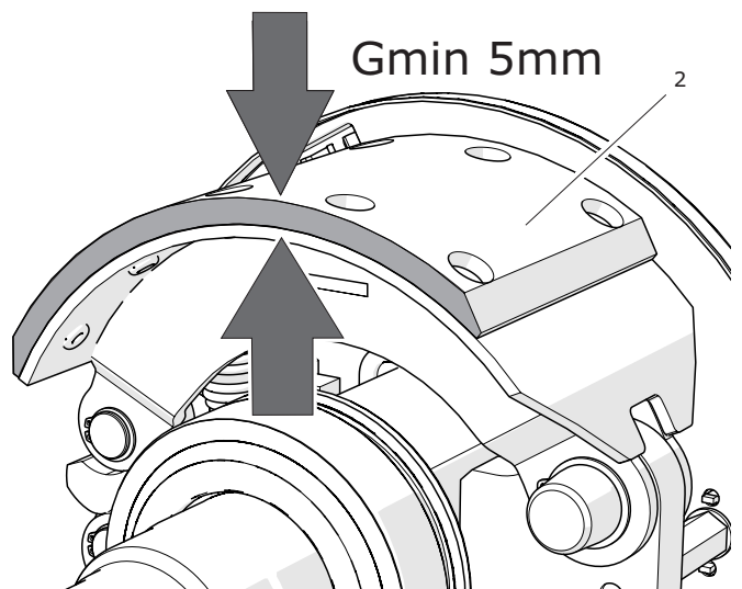
Figura 5.9 Control de los revestimientos de frenos (1) tapón (2) revestimiento de freno
