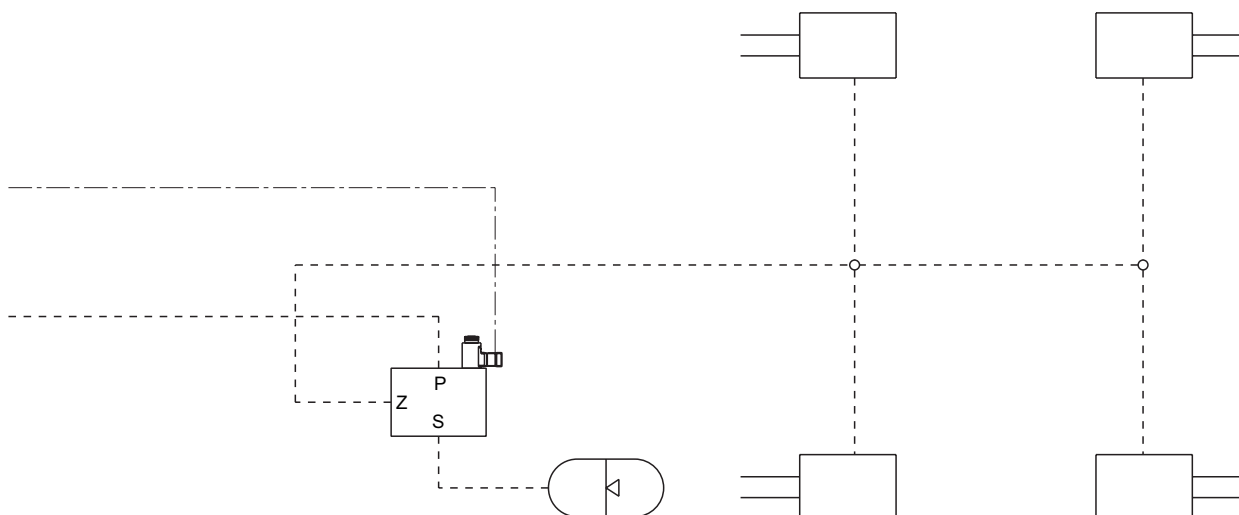
Figura 3.13 Esquema de la instalación hidráulica con el regulador de fuerza de frenos.
