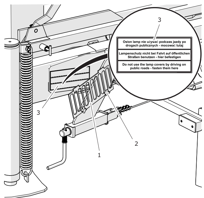
Figura 4.23 Toma de la rejilla protectora (1) rejilla protectora (2) tornillo (3) etiqueta
