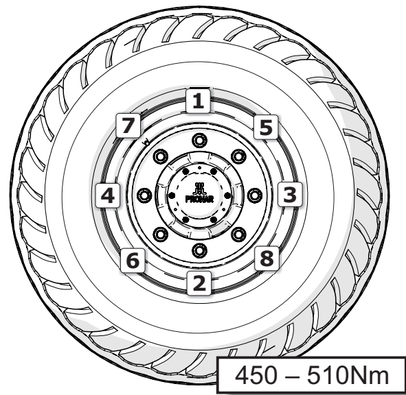
Figura 5.23 Modo de enrosque de la rueda
