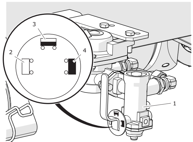
Figura 4.22 Regulador de la fuerza de frenado (1) regulador (2) posición SIN CARGA (3) posición MEDIA CARGA (4) posición CARGA LLENA
