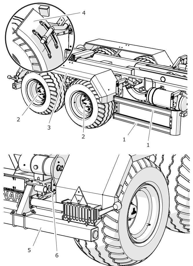
Figura 5.5 Tapas de remolque
