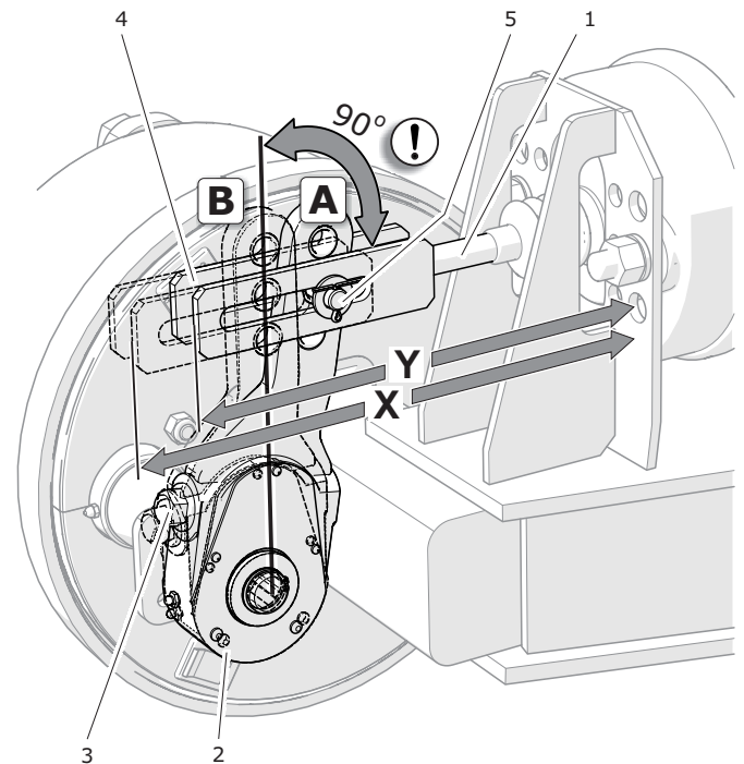
Figura 5.11 Control de freno
