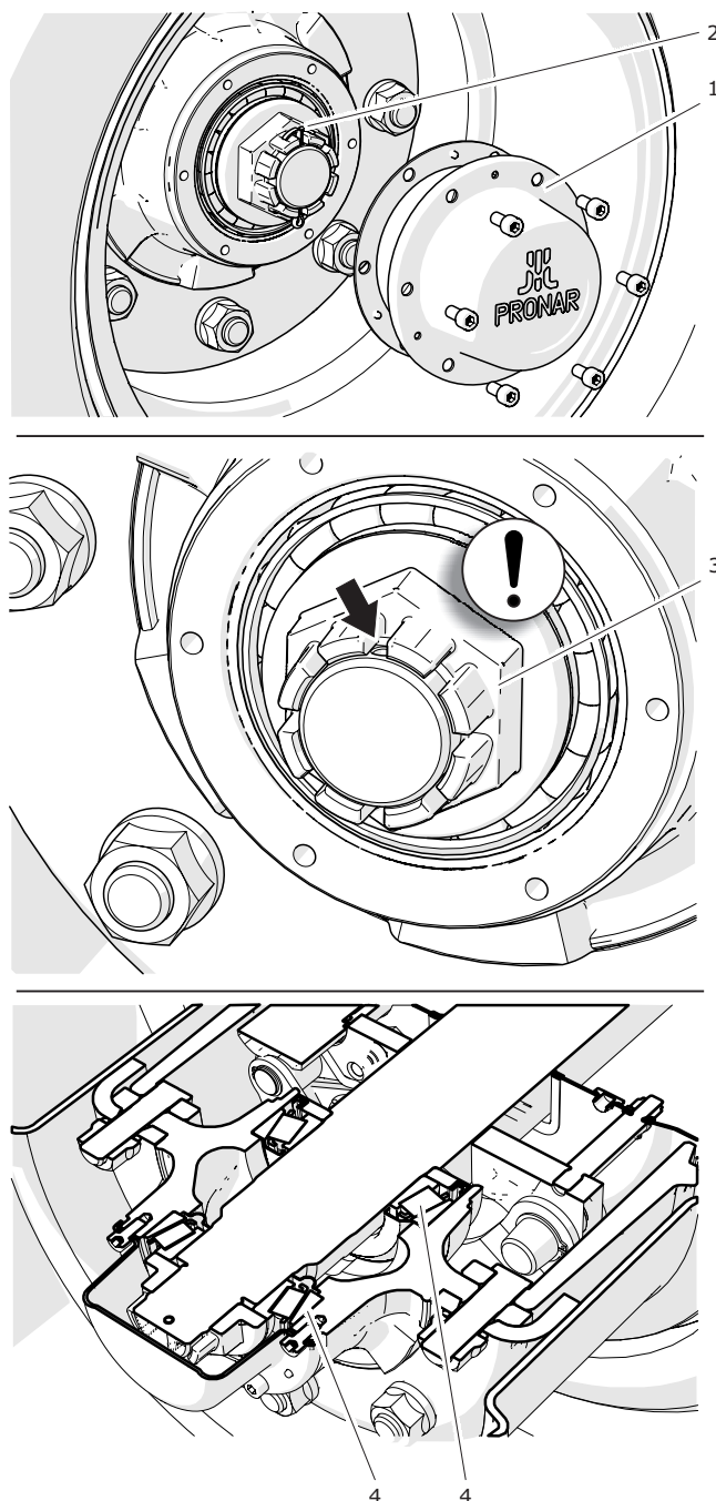
Figura 5.17 Zasada regulacji luzu łożysk
