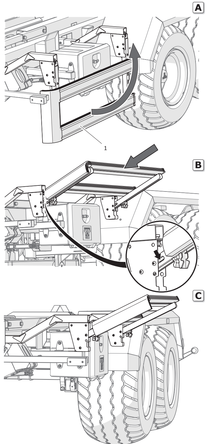
Figura 4.5 Prawa osłona najazdowa
