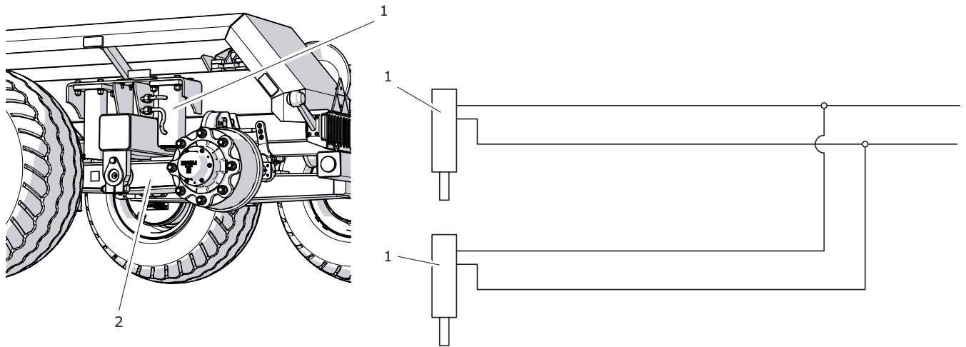
Figura 3.19 Esquema de la instalación de bloqueo de los brazos transversales.
