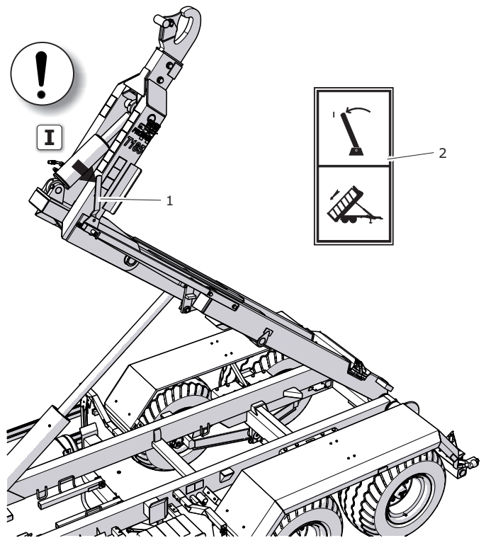
Figura 3.5 Elevación del bastidor basculante
