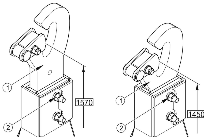
RYСУNEK 4.6A REGULACJA POŁOŻENIA HAKA
