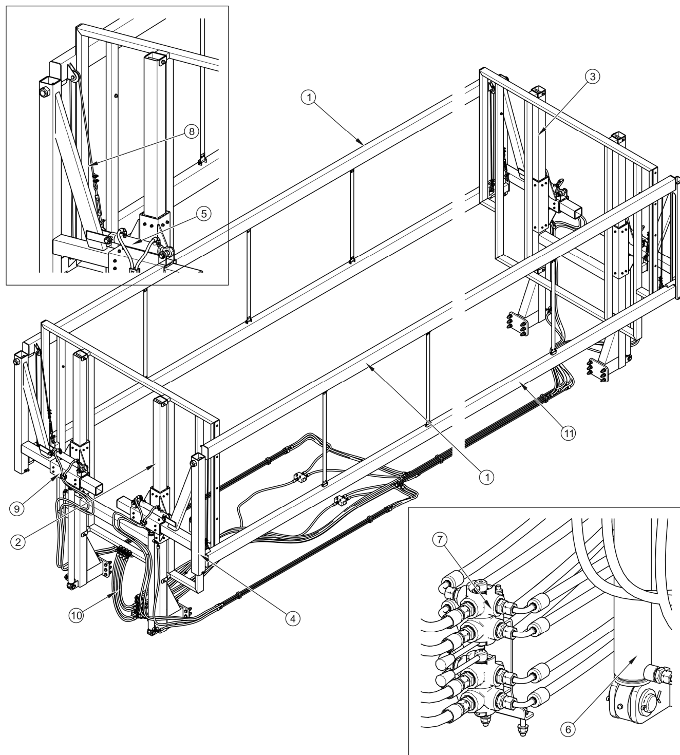
RYSUNEK 3.11 Budowa instalacji hydraulicznej unoszenia ścian
