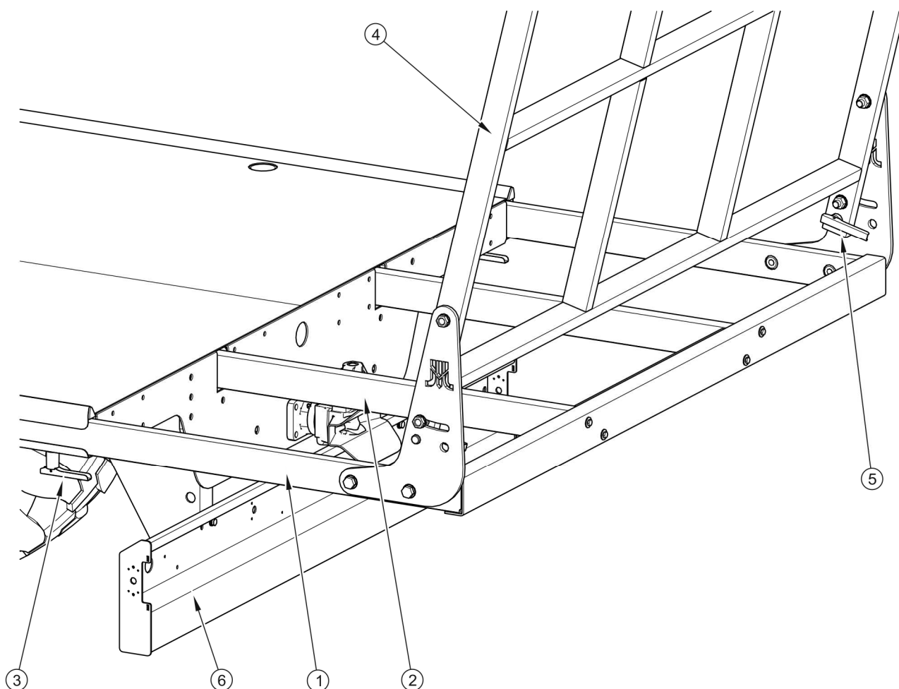
RYSUNEK 3.4 Rama wysuwna
