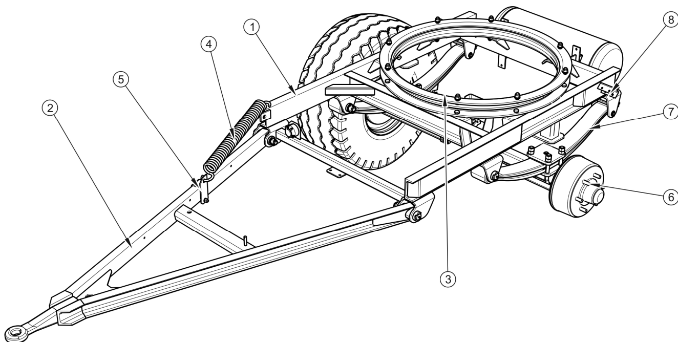
RYСУNEK 3.6 Zawieszenie przednie
