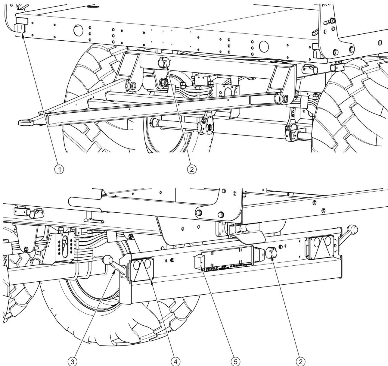
RYSUNEK 3.13 Rozmieszczenie elementów instalacji elektrycznej
