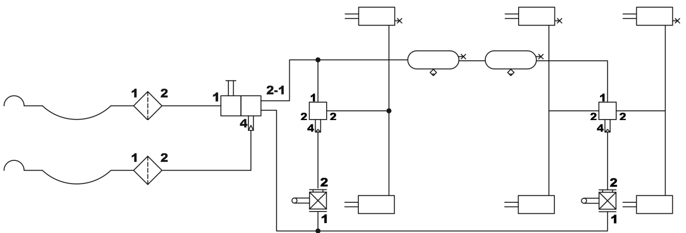
RYSUNEK 3.8 Schemat instalacji pneumatycznej dwuprzewodowej z automatycznym regulatorem siły hamowania
