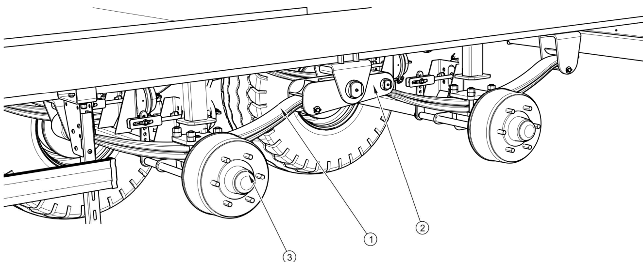
RYСУNEK 3.5 Zawieszenie tylne
