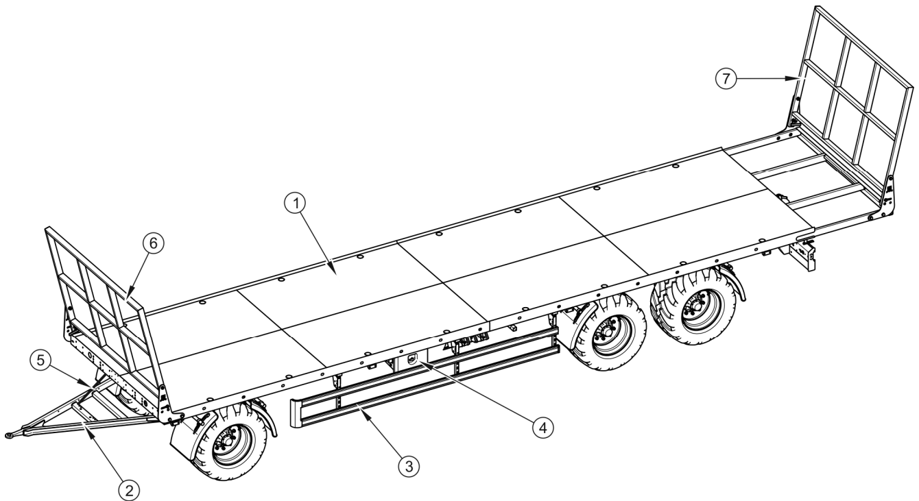
RYСУNEK 3.1 Budowa przyczepy w wersji podstawowej z drabinkami
