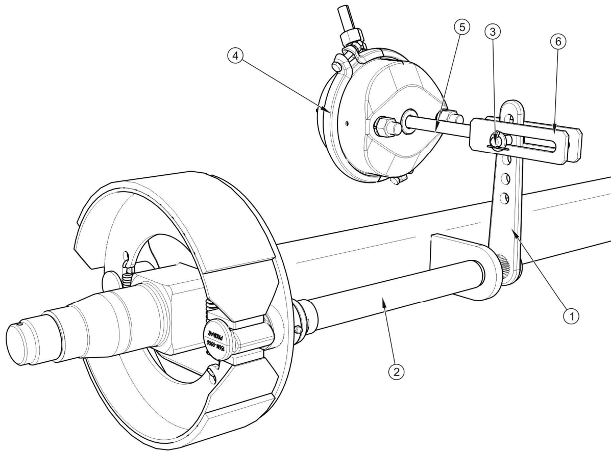
RYСУNEK 5.6 Budowa hamulca osi jezdnej
