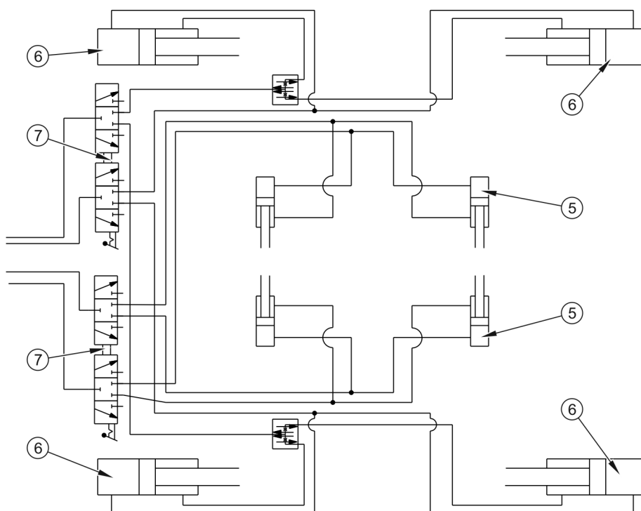
RYSUNEK 3.12 Schéma hydraulického zvedání stěn
