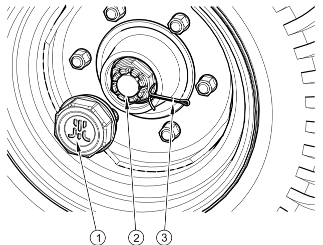
RYSUNEK 5.3 Seřízení vůle
