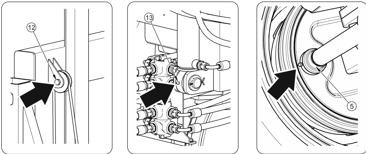
RYSUNEK 5.11 Mazací místa přívěsu
