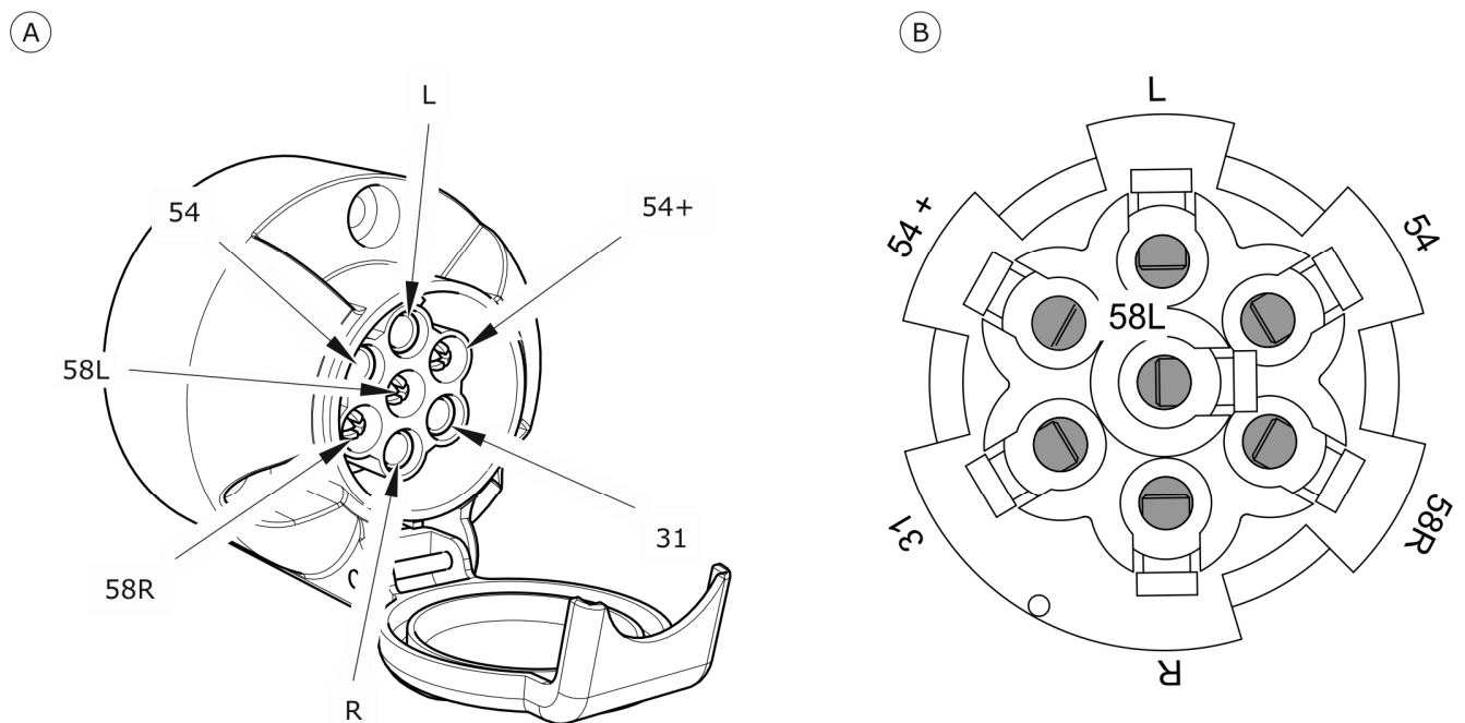
RYSUNEK 3.19 Gniazdo przyłączeniowe
