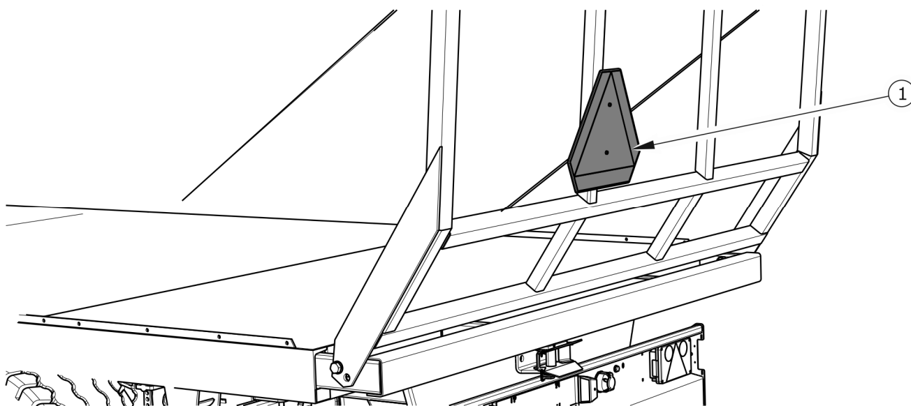
RYSUNEK 2.1 Miejsce montażu tablicy
