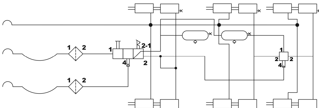
RYСУNEK 3.11 Schemat instalacji pneumatyczno hydraulicznej
