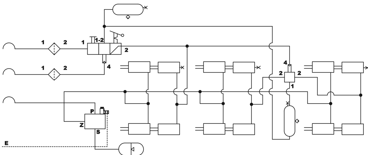
RYСУNEK 3.12 Schemat instalacji pneumatyczno hydraulicznej z zabezpieczeniem elektrycznym
