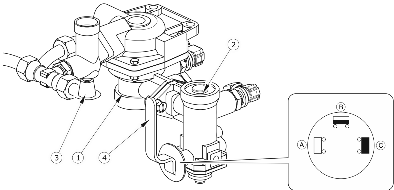
RYSUNEK 3.15 Zawór sterujący i regulator siły hamowania
