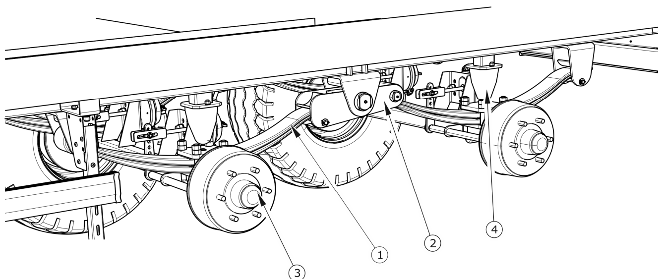
RYSUNEK 3.4 Zawieszenie tylne
