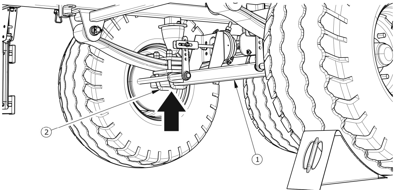
RYSUNEK 5.1 Punkt podparcia podnośnika
