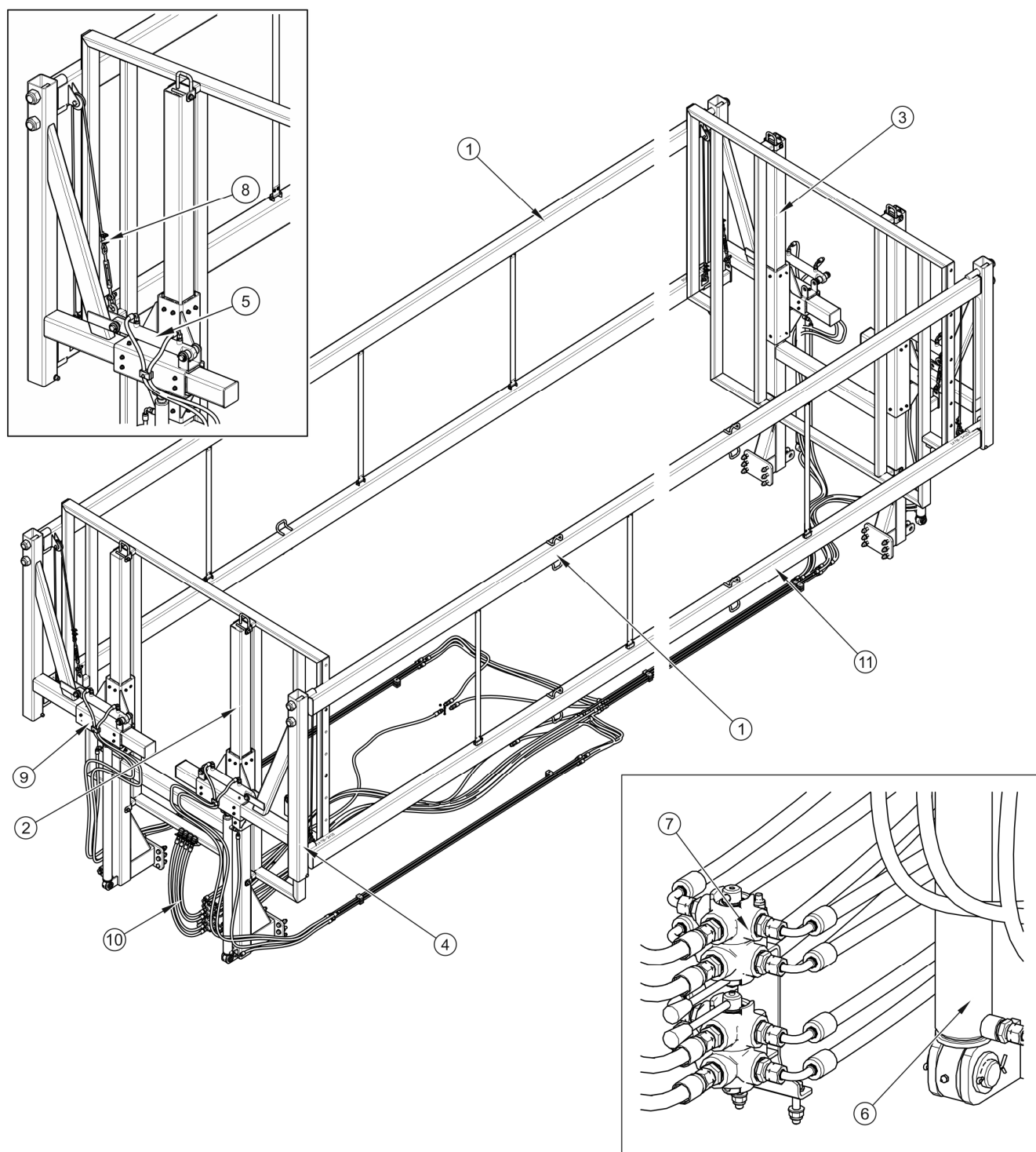
RYСУNEK 3.16 Budowa instalacji hydraulicznej unoszenia ścian
