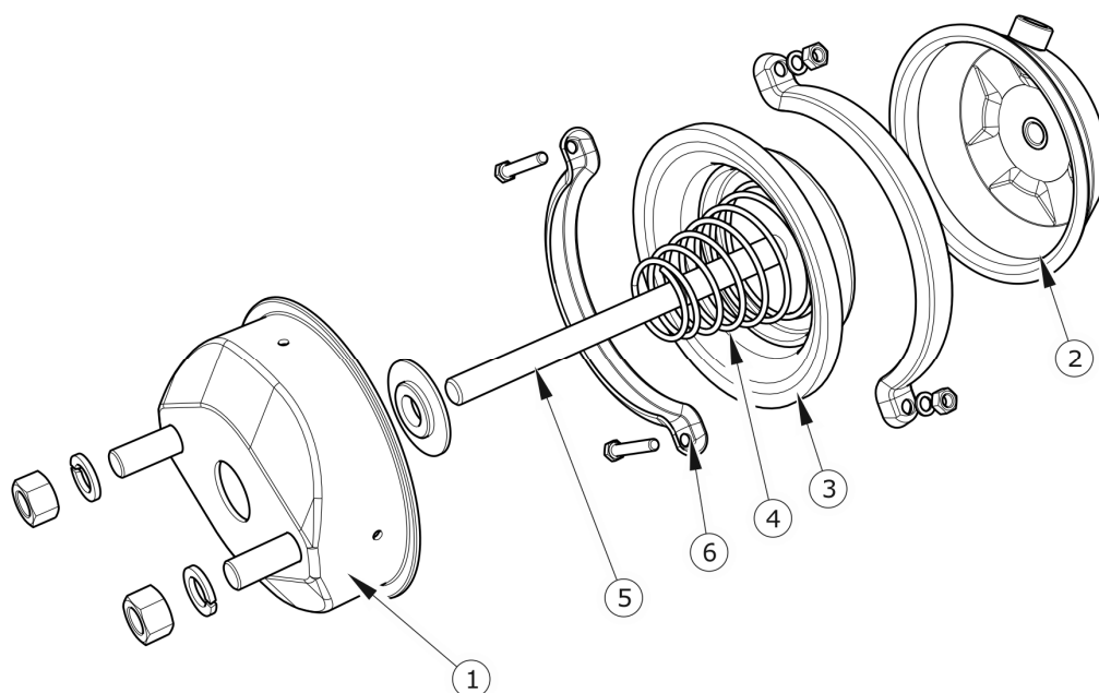
RYСУNEK 3.14 Budowa siłownika pneumatycznego
