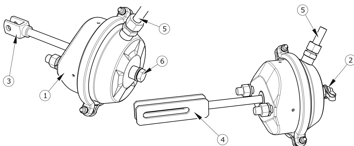
RYСУNEK 3.13 Siłowniki pneumatyczne hamulcowe
