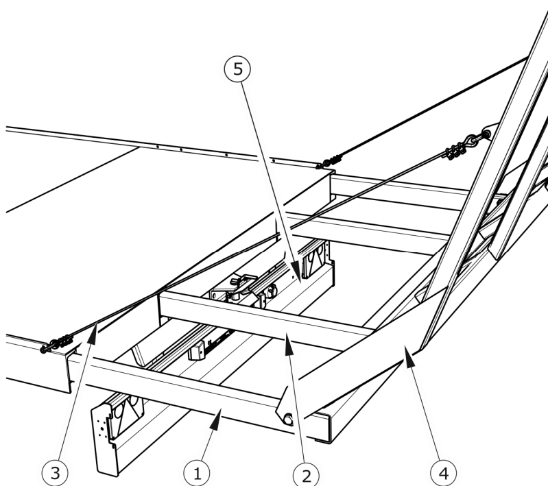
RYSUNEK 3.3 Rama wysuwna
