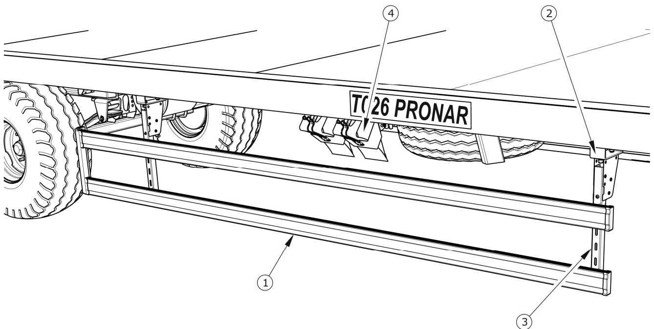
RYSUNEK 3.6 Boczne osłony najazdowe
