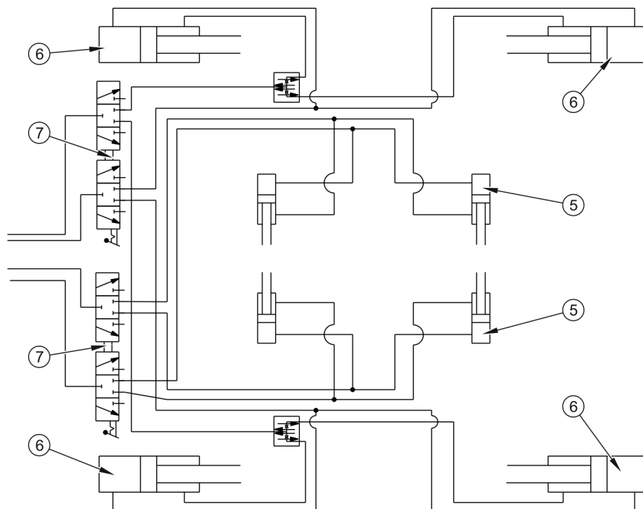
RYСУNEK 3.17 Schemat instalacji hydraulicznej unoszenia ścian
