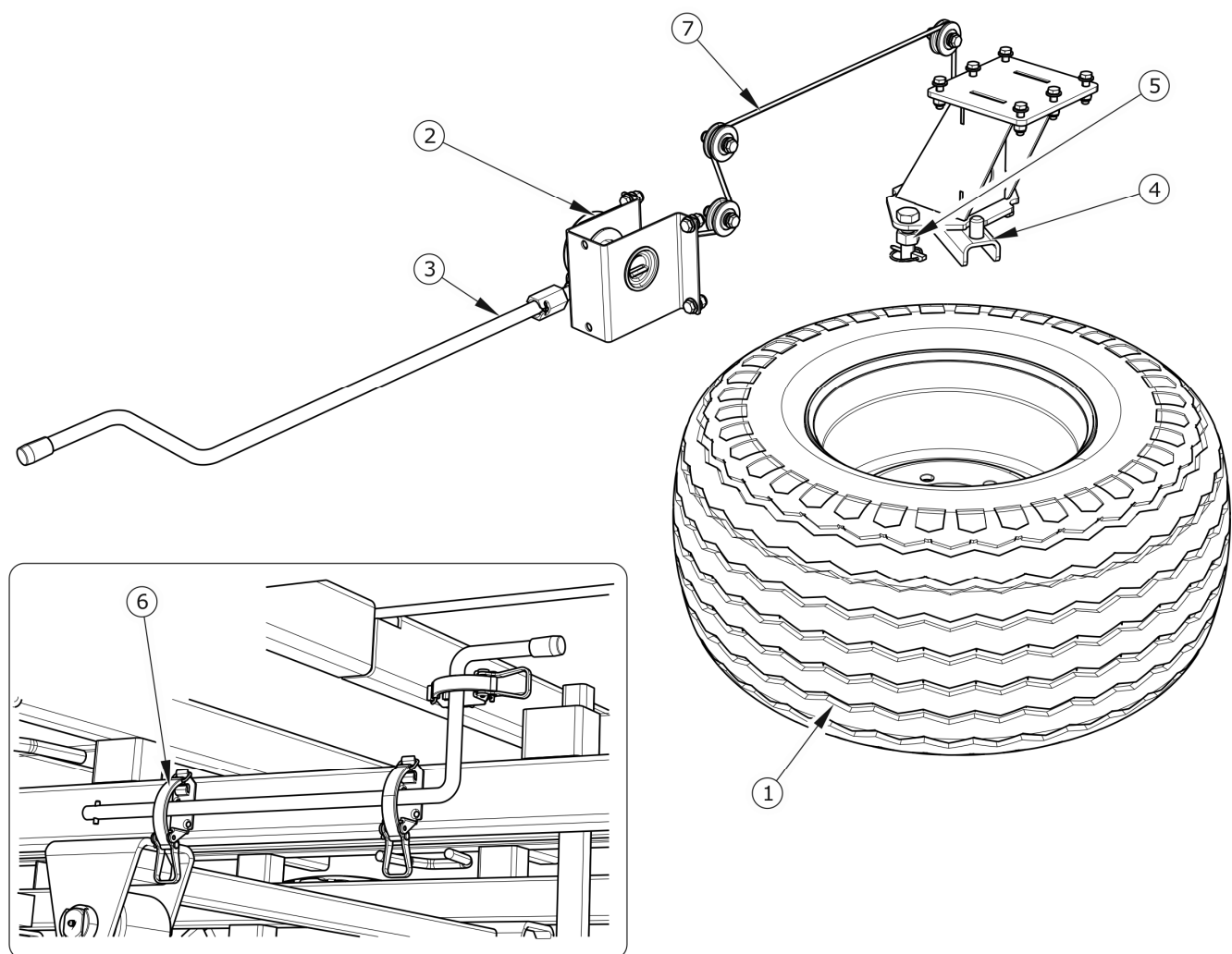
RYСУNEK 3.15 Budowa wciągarki koła zapasowego
