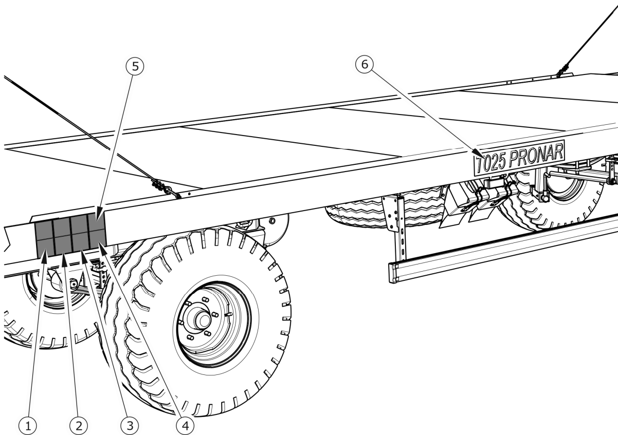
RYSUNEK 2.2 Rozmieszczenie naklejek informacyjnych i ostrzegawczych
