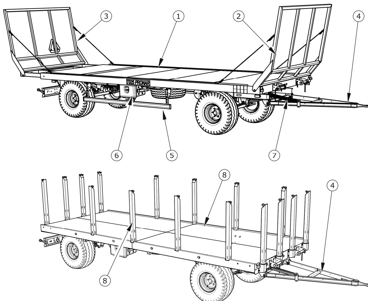
RYSUNEK 3.1 Budowa przyczepy
