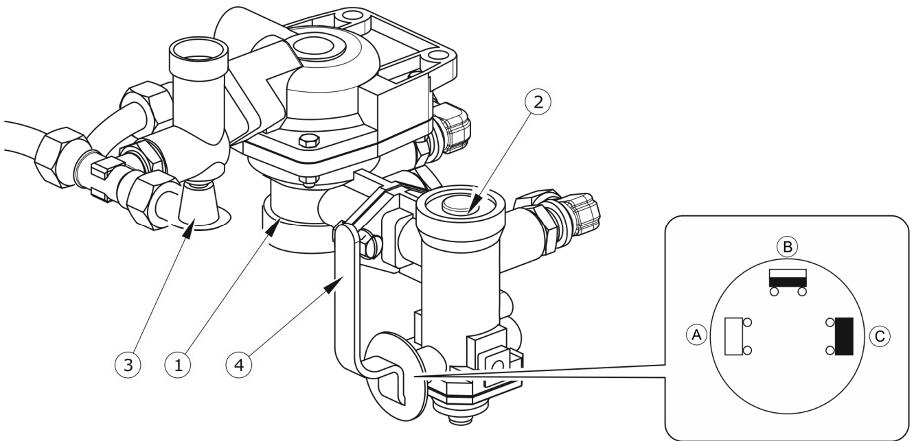
RYSUNEK 3.12 Zawór sterujący i regulator siły hamowania
