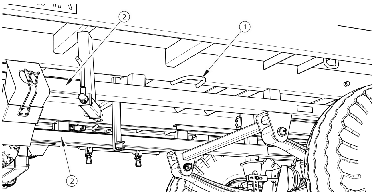
RYSUNEK 1.3 Uchwyty transportowe
